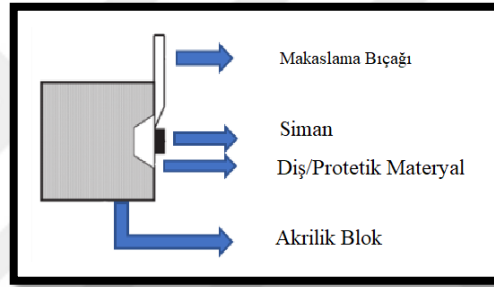
Şekil 2.17. Makaslama test düzeneği 119
