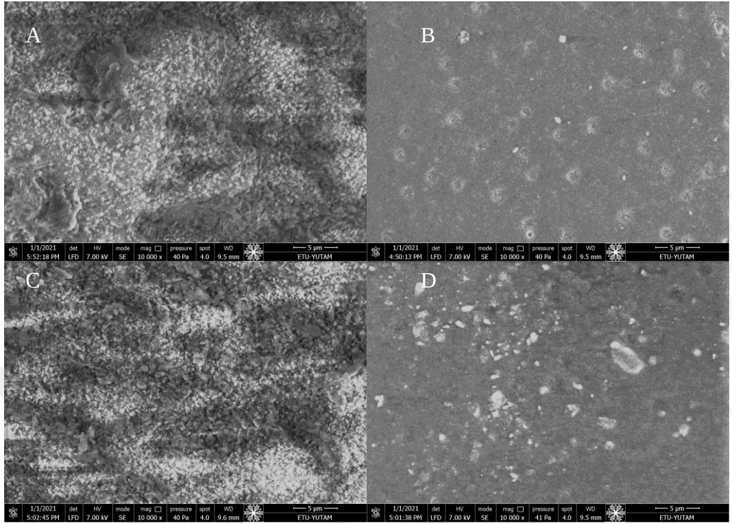
Şekil 4.15. Yüzey işlemleri sonrası GC materyal yüzeylerinde elde edilen ESEM görüntüsü 10000×
