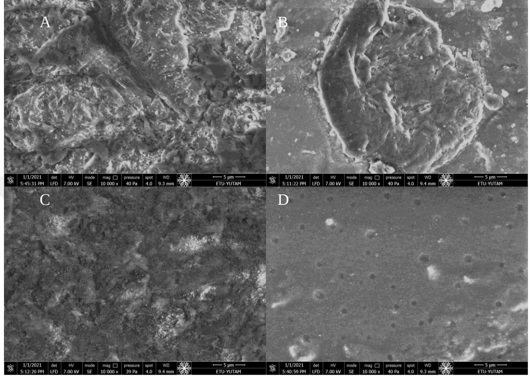
Şekil 4.12. Yüzey işlemleri sonrası PEEK materyal yüzeylerinde elde edilen ESEM görüntüsü 10000×
