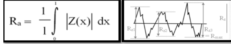
Şekil 2.12. Yüzey pürüzlülüğü parametreleri ( R_a , R_z , R_{max} ) 100
