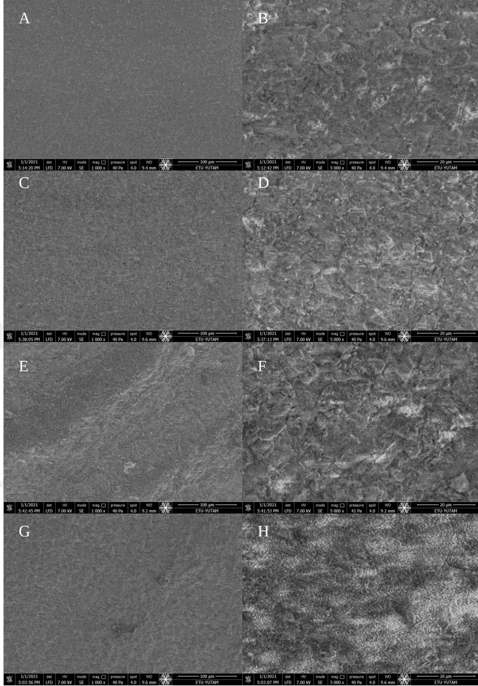
Şekil 4.10. CoJet grubunda materyal yüzeylerinde elde edilen ESEM görüntüleri A: PEEK 1000×, B: PEEK 5000×, C: PEKK 1000×, D: PEKK 5000×, E: VITA 1000×, F: VITA 5000×, G: CERASMART 1000×, H: CERASMART 5000×
