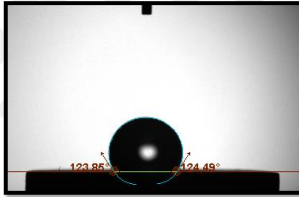
Şekil 4.4. PEKK kumlama, adeziv – grubunun temas açısı görünümü
