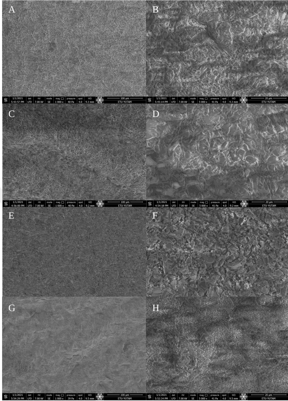
Şekil 4.8. Kumlama grubunda materyal yüzeylerinde elde edilen ESEM görüntüleri A: PEEK 1000×, B: PEEK 5000×, C: PEKK 1000×, D: PEKK 5000×, E: VITA 1000×, F: VITA 5000×, G: CERASMART 1000×, H: CERASMART 5000×
