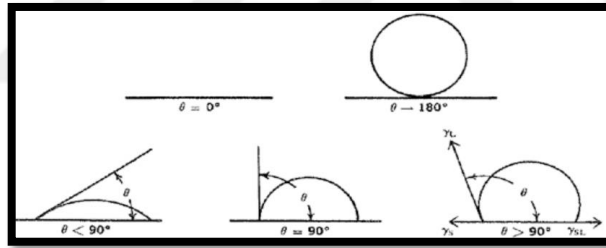
Şekil 2.14. Katı-sıvı arasında meydana gelen değim açısı 109
