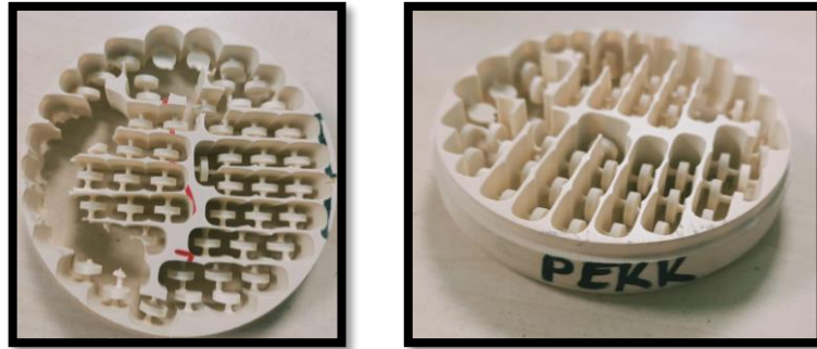
Şekil 3.5. K5 vhf kazıma cihazında hazırlanan PEEK ve PEKK örnekler
