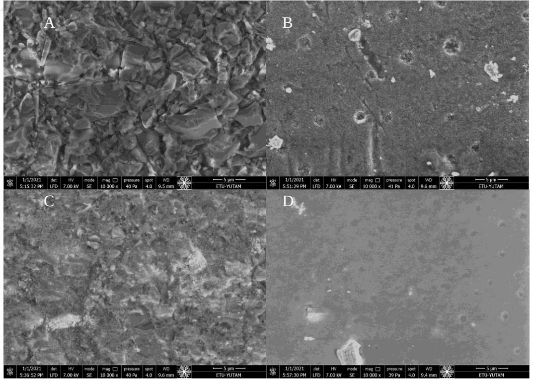
Şekil 4.14. Yüzey işlemleri sonrası VITA materyal yüzeylerinde elde edilen ESEM görüntüsü 10000×
