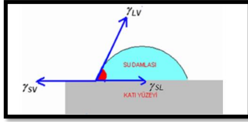
Şekil 2.13. Değim açısı 109
