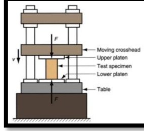
Şekil 2.20. Basma deneyi test düzeneği 125
