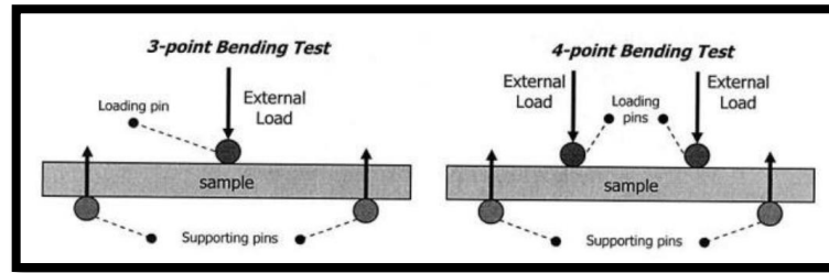
Şekil 2.19. 3 nokta ve 4 nokta bükülme testleri 123
