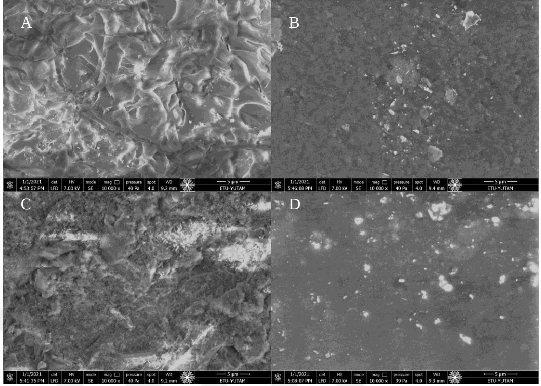
Şekil 4.13. Yüzey işlemleri sonrası PEKK materyal yüzeylerinde elde edilen ESEM görüntüsü 10000×
