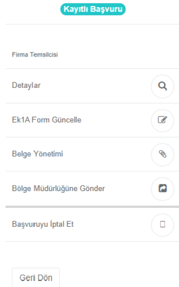
Şekil 11. Seçenekler menüsü
