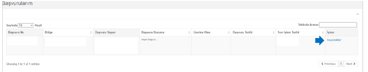
Şekil 10. Seçenekler
