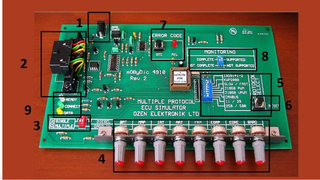
Şekil 3.18. Mobydic 4910 simülasyon cihazı
