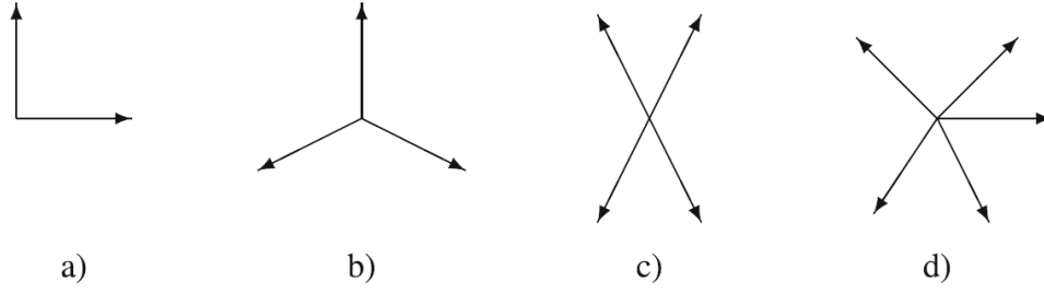
Şekil 3.1 Düzlemde bazı pozitif taban örnekleri (Audet ve Hare, 2014).
