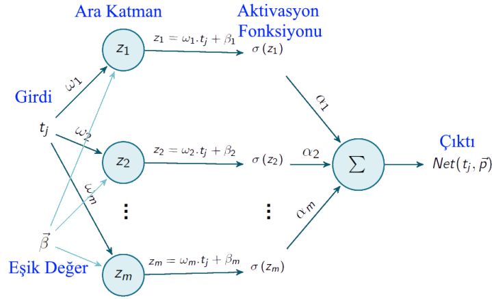
Şekil 4.2 İleri beslemeli yapay sinir ağı topolojik yapısı.
