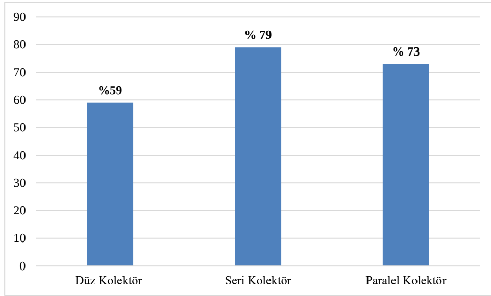
Şekil 5.28. Seri, paralel ve düz kolektörün 6,5m/s hızda radyasyon değerlerine göre verim grafiği
