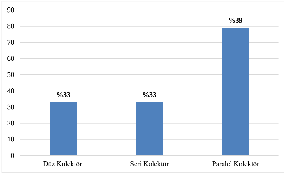
Şekil 5.29. Seri, paralel ve düz kollektörün 3m/s hızda radyasyon değerlerine göre verim grafiği
