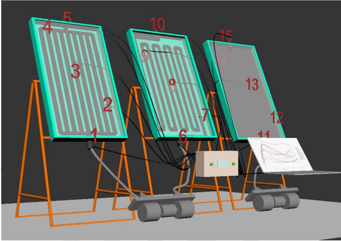
Şekil 5.16. Hava akışkanlı güneş kolektörlerinin ölçüm aletleri ile kurulumu.
