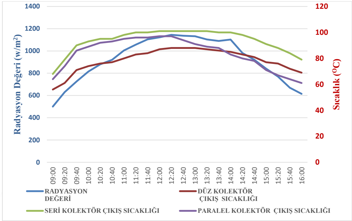
Şekil 5.24. Seri kollektör 41° ve 3 m/s hızda radyasyon değerlerine göre sıcaklık farkı grafiği
