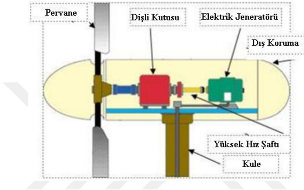
Şekil 3.4. Rüzgâr enerjisi üretim şeması (Adıyaman, 2012)
