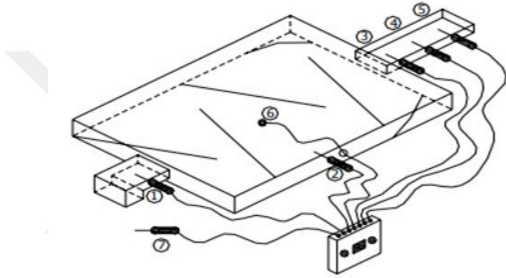
Şekil 2.1. Sıcaklık ölçümü yapılan noktalar (İnalı ve ark., 2001)
