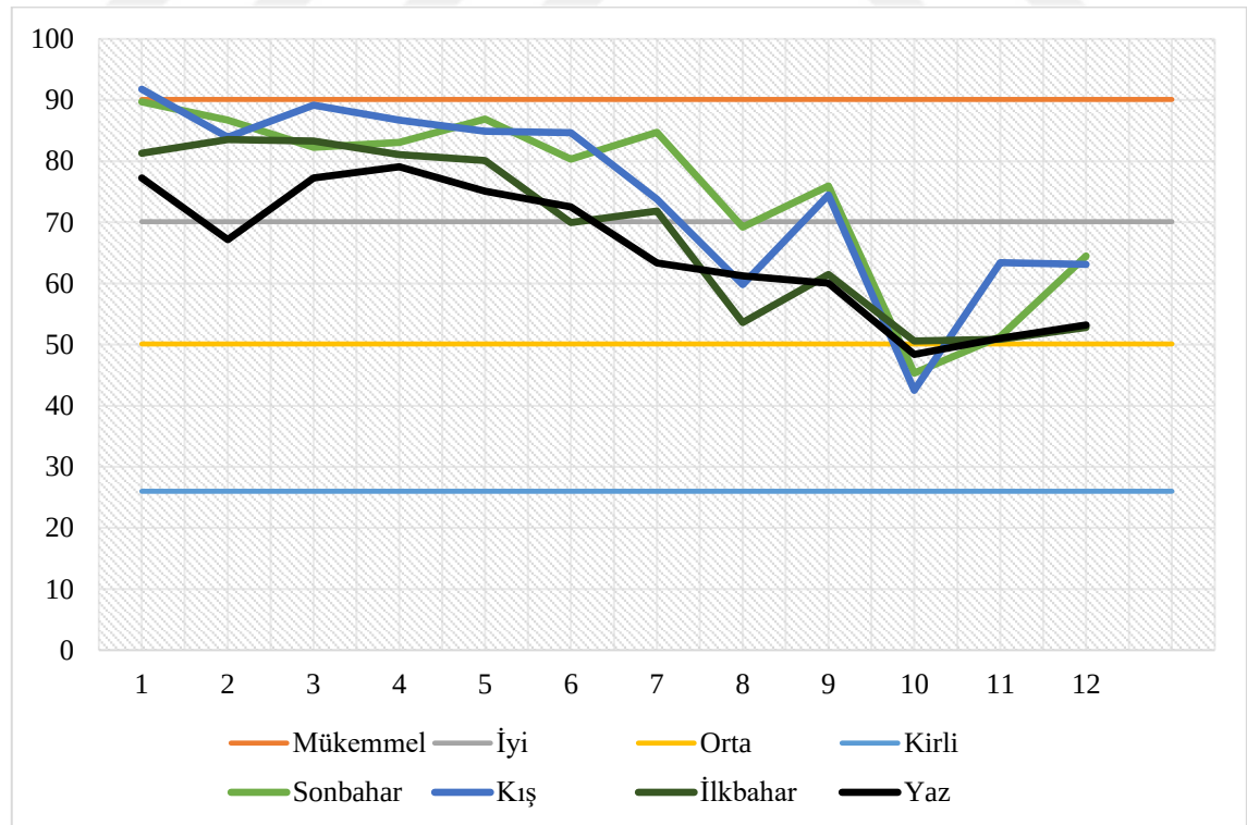
Şekil 4.20. Tüm mevsimlerde ölçülen NSF-WQI değerleri
