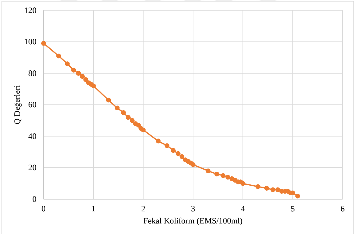
Şekil 2.8. Fekal koliiform için Q değerleri (Fekal koliiform > 100.000/100 ml olduğunda Q=2 )
