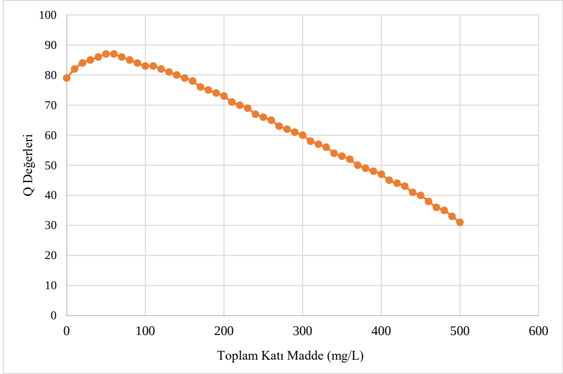
Şekil 2.9. Toplam katı madde için Q değerleri ( TKM > 500 \text{ mg/L} olduğunda Q=20 )
