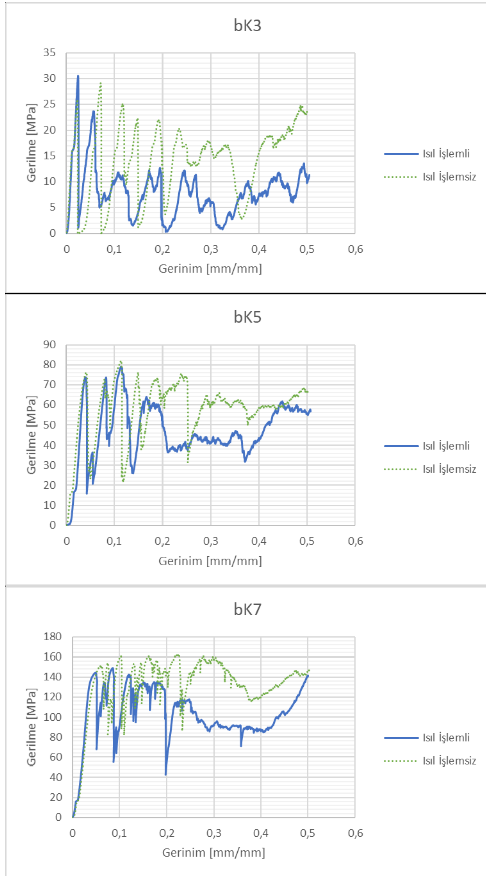
Şekil 4.38. Kübik numunelerin ısıtıl işlem farkını gösteren basma deneyi gerilme-gerinim grafiği
