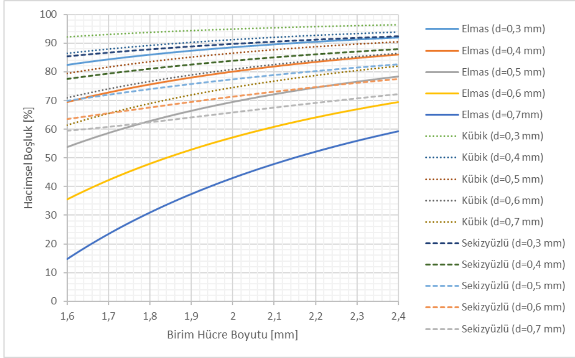
Şekil 4.7. Belirli kolon kalınlıkları için birim hücre boyutuna bağlı hacimsel boşluk oranları
