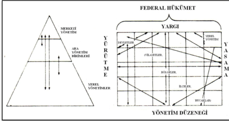
Şekil 4.1: Elazar'ın matrisi
