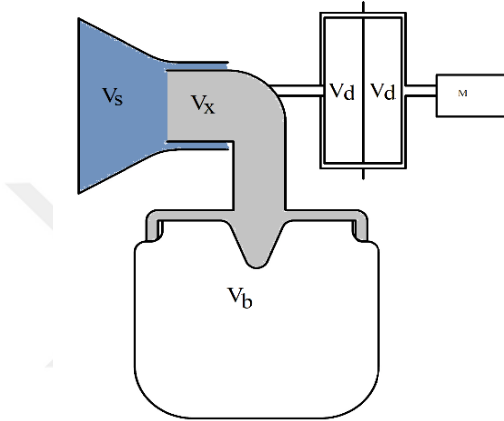
Şekil 4.1 Meme pompası tasarımı için hesaplanan hacim şeması. (V s : Meme flanşı hacmi, V x : Flanş, şişe ve pompa arasındaki Konektörlerin Hacmi, V d : Yarım Pompa Hacmi. V b :Şişe hacmi)
