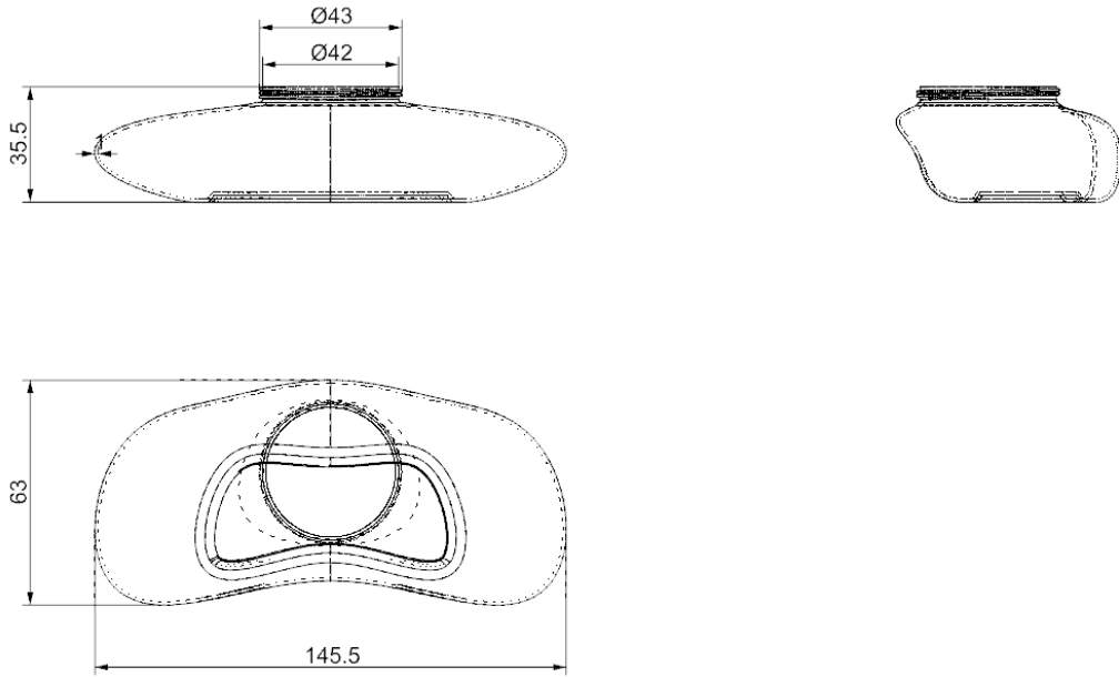
Şekil 4.5 Süt haznesi ölçüler
