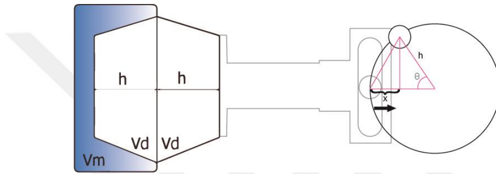
Şekil 5. 14 Diyafram hareketi ve servo motor açısı ile oluşturulan hacim illüstrasyonu
