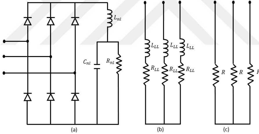
Şekil 22. Yükler: (a) doğrusal olmayan yük, (b) endüktif yük, (c) omik yük
