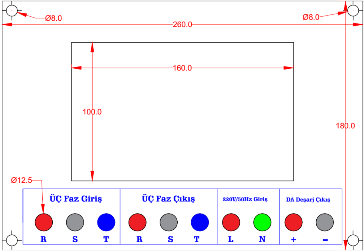
Ek Şekil 4. KGK ön panel giriş ve çıkışları
