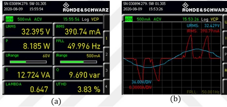
Şekil 86. Doğrusal olmayan yük altında CCS-MPC ile KGK çıkış gerilimi performansı (a) ve yük akımı, çıkış gerilimi dalga biçimi (b), ( \eta=7.8 , V_d^* = 50V , \%THD = 3.83 )
