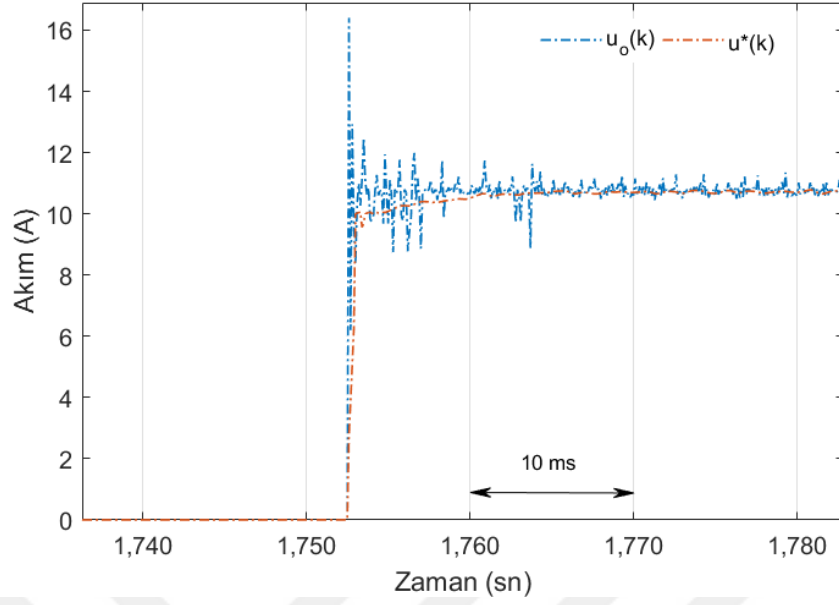
Şekil 77. u_o(k) ve u^*(k) kontrol girişleri ile omik yük akımının geçiş cevabı ( \eta=2.5 , u^*(k) ile THD = %1, u_o(k) ile THD = %2.2)
