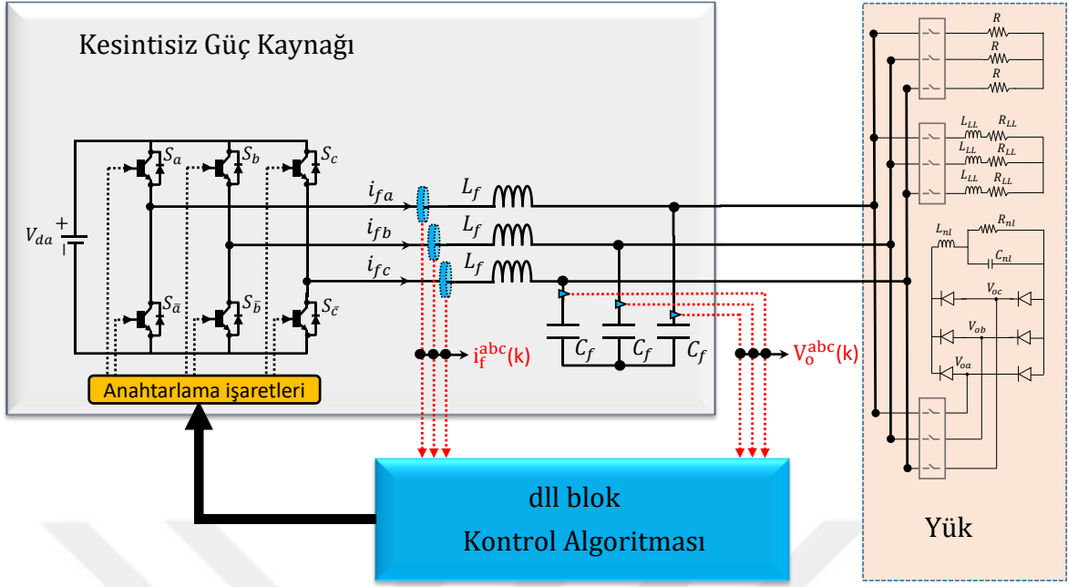
Şekil 21. PSIM'de oluşturulan KGK benzetim modeli
