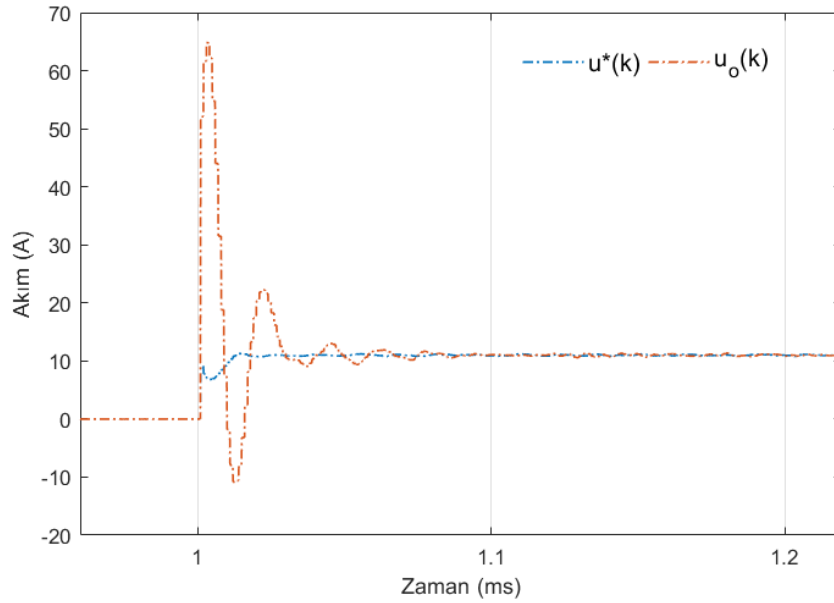
Şekil 23. u_o(k) ve u^*(k) kontrol girişleri ile omik yük akımının geçiş cevabı ( \eta=2.5 , u^*(k) ile THD = %1, u_o(k) ile THD = %2.2)
