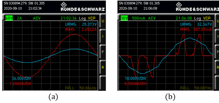
Şekil 88. KGK çıkış gerilimi ve bir faza ait akım (a) doğrusal yük altında, (b) doğrusal olmayan yük altında
