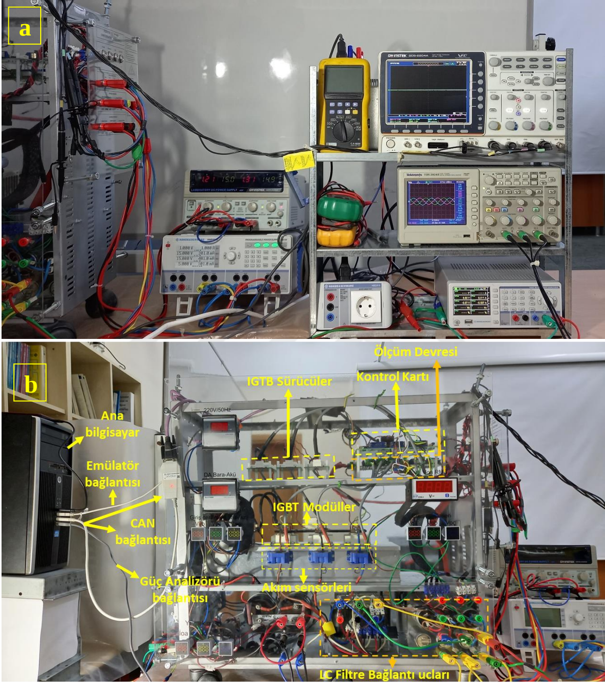
Ek Şekil 7. Deney Düzeneği (a) Ölçüm Seti (b) KKG cihazı
