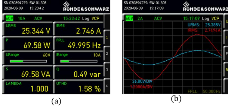
Şekil 85. CCS-MPC ile (a) KGK çıkış gerilimi THD'si, (b) akım ve gerilim dalga biçimi ( C_f = 33\mu F )
