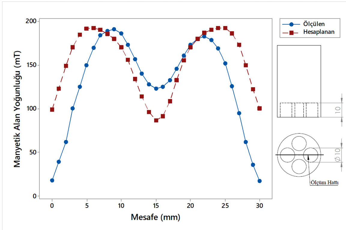
Şekil 5.10. 1 nolu takıma ait kutup boyunca manyetik alan yoğunluğunun değişimi
