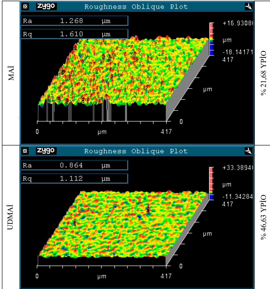
Resim 1.4. 4. deneylere ait numunelerin 3B yüzey topografyası
