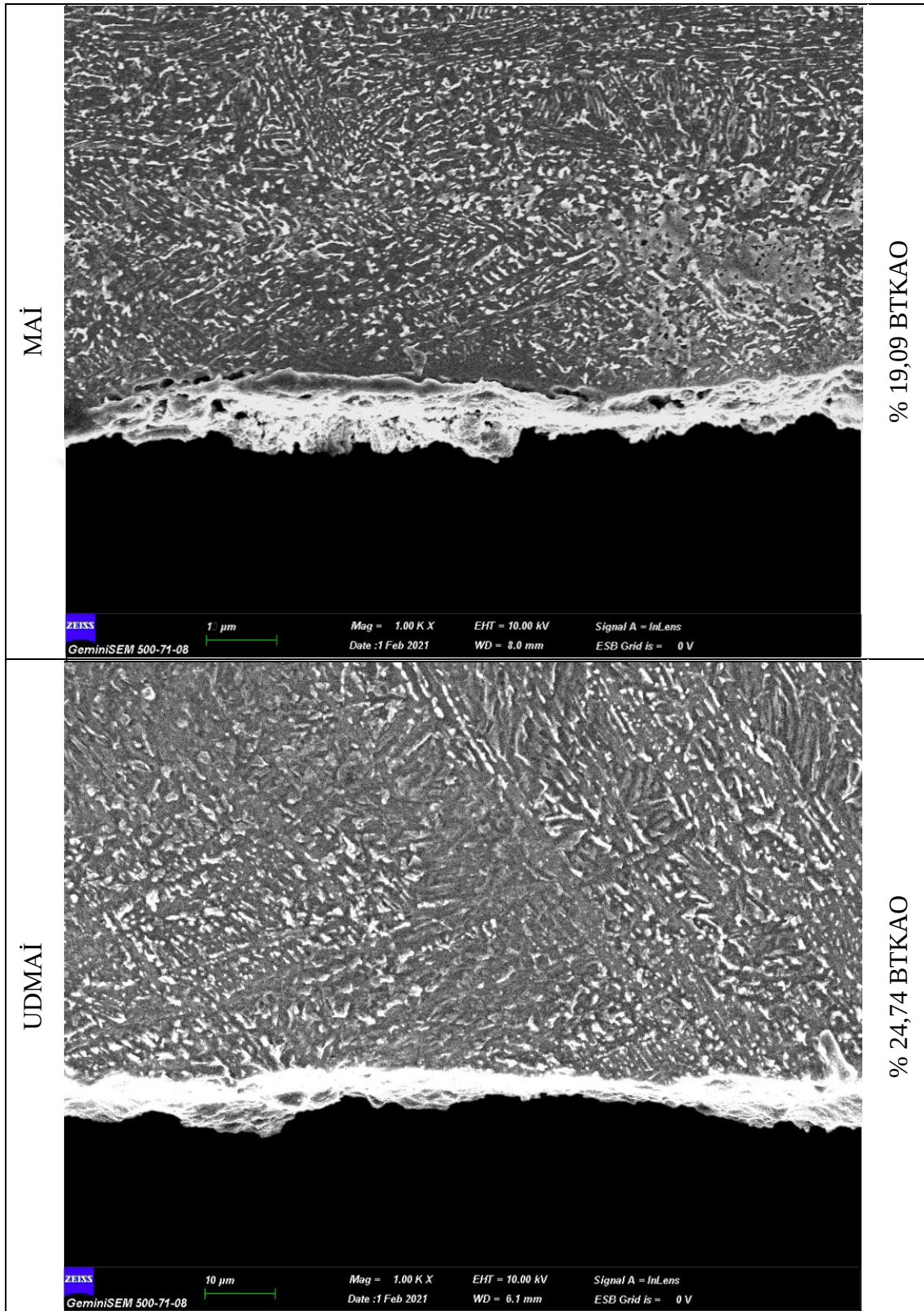
Resim 6.5. En düşük BTKAO değerine sahip numunelere ait SEM görüntüleri
