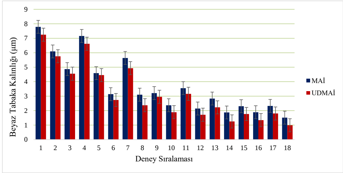
Şekil 6.10. MAİ/UDMAİ deneylerine ait beyaz tabaka kalınlık grafiği
