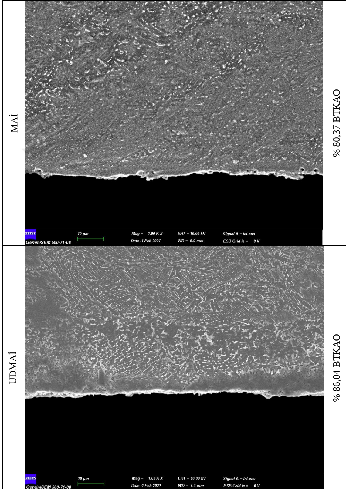
Resim 2.16. 16. deneylere ait beyaz tabaka görüntüleri
