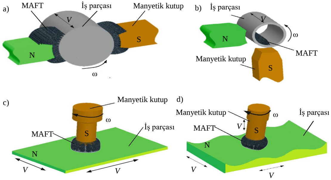
Şekil 3.1. MAİ yönteminin farklı yüzeylerde uygulanışı: a: silindirik dış yüzeyler, b: silindirik iç yüzeyler, c: düzlemsel yüzeyler, d: serbest formlu yüzeyler [35]
