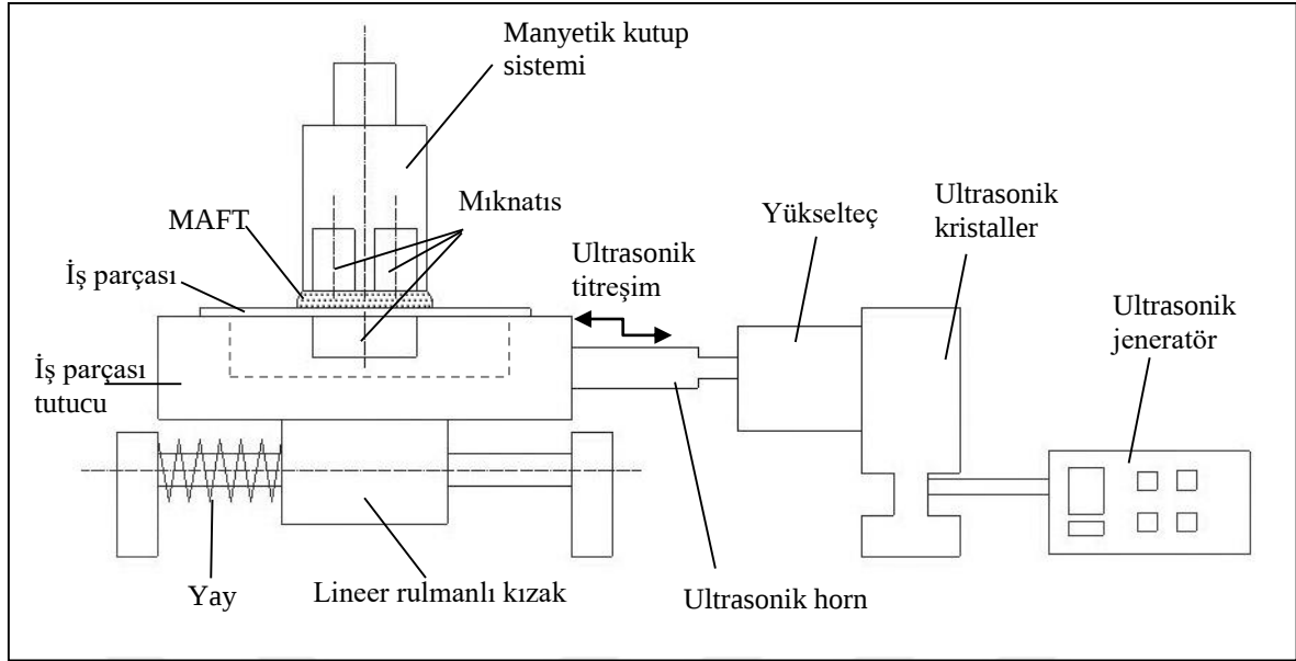
Şekil 5.2. Deney düzeneğinin şematik gösterimi
