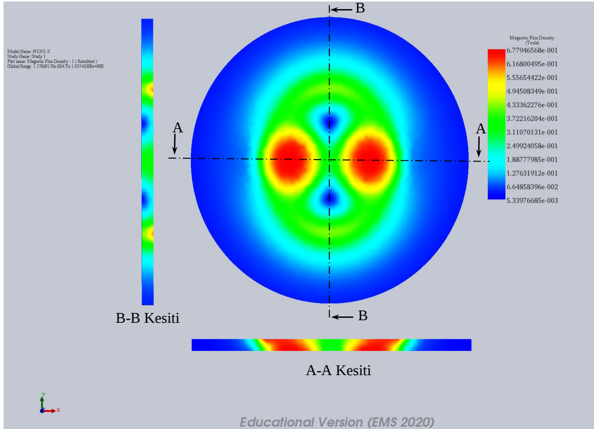
Şekil 5.6. NSNS-S oryantasyonuna sahip kutup sisteminde iş parçasına etkiyen manyetik alan
