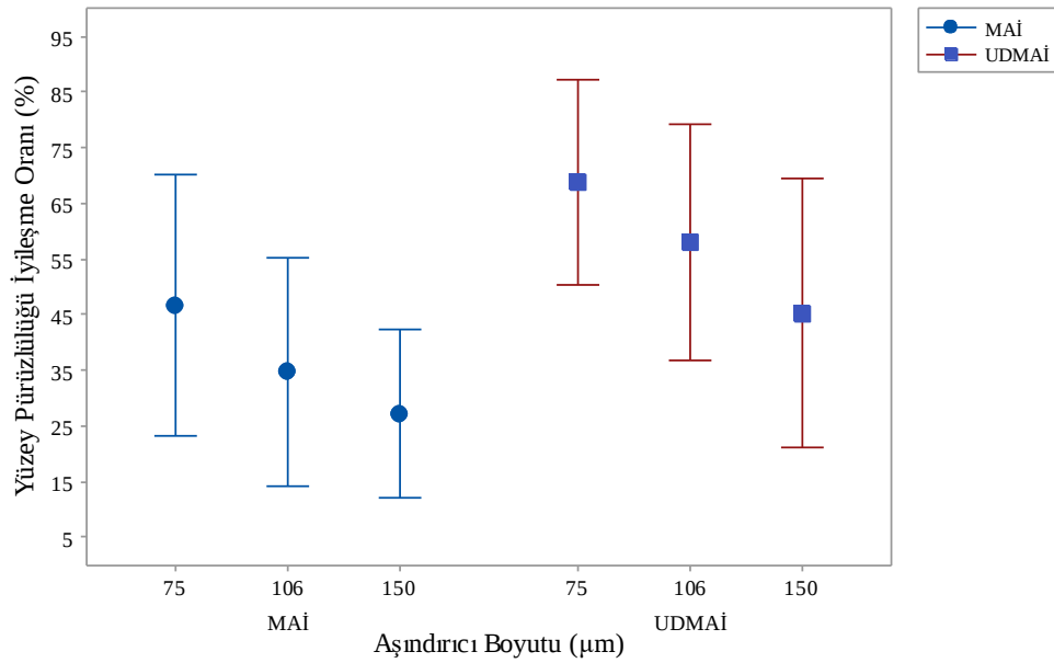
Şekil 6.7. MAİ ve UDMAİ yönteminde aşındırıcı boyutunun YPİO üzerine etkisi
