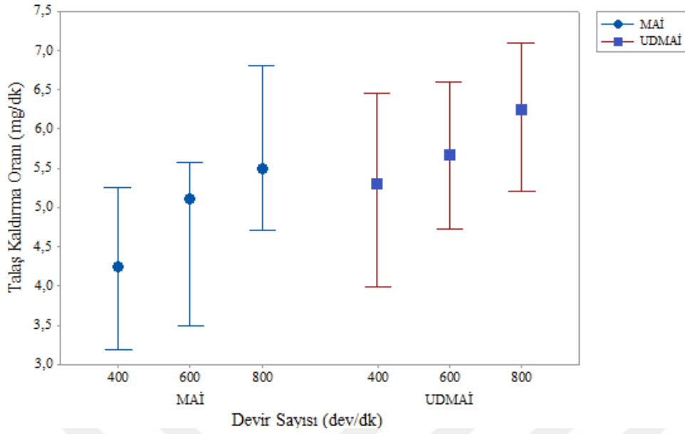
Şekil 6.3. MAİ ve UDMAİ yönteminde devir sayısının TKO üzerine etkisi
