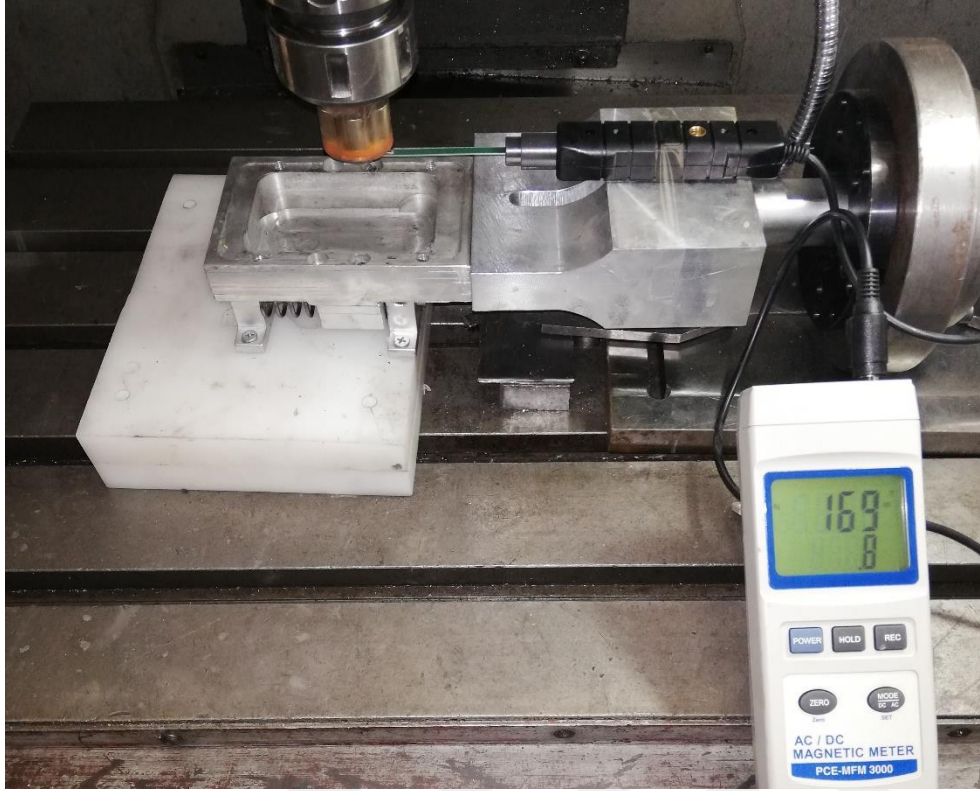
Resim 5.3. Manyetik kutup boyunca manyetik alan yoğunluğunun ölçülmesi
