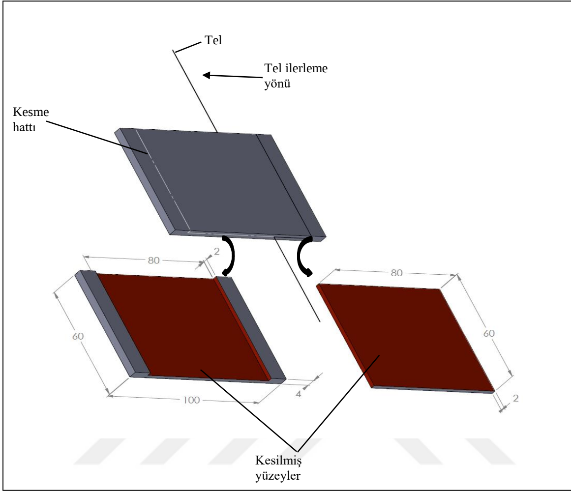
Şekil 5.1. Numunelerin TEİ yöntemiyle kesilmesi
