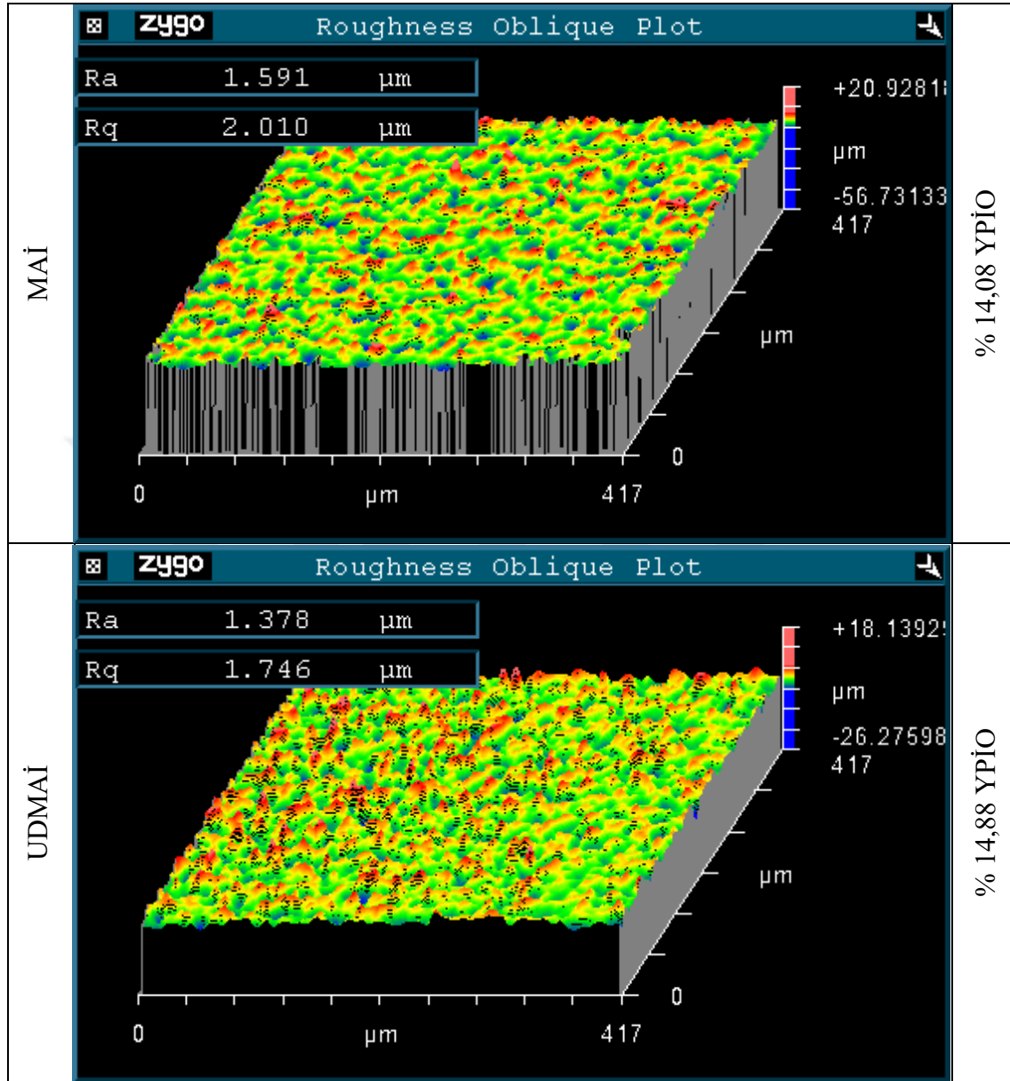
Resim 1.9. 9. deneylere ait numunelerin 3B yüzey topografyası
