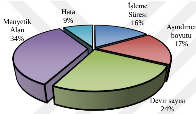
Şekil 7.4. UDMAİ yönteminde işlem parametrelerinin TKO üzerindeki katkıları
