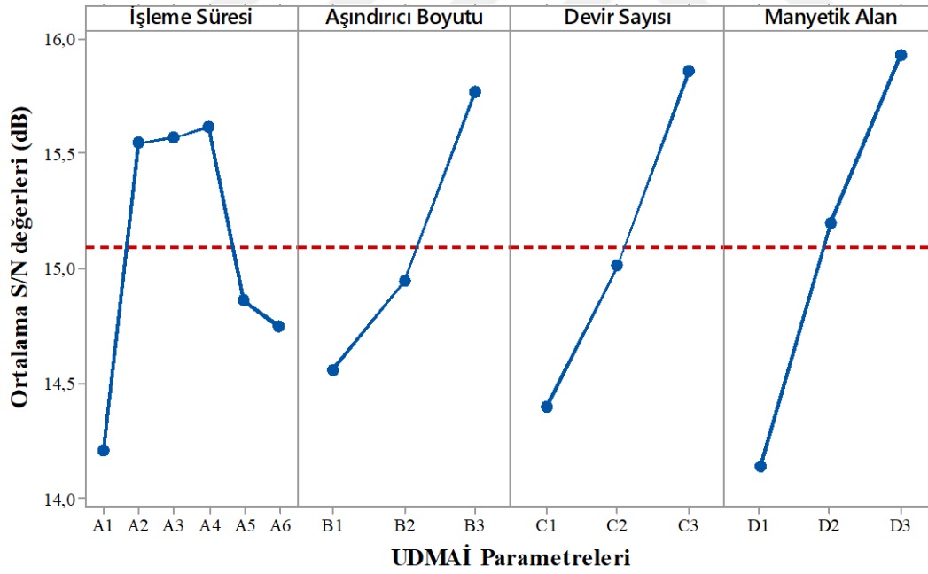
Şekil 7.2. UDMAİ yönteminde işleme parametrelerinin talaş kaldırma oranına etkisi
