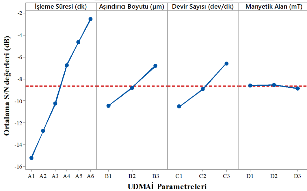
Şekil 7.10. UDMAİ yönteminde işleme parametrelerinin beyaz tabaka kalınlığı üzerindeki etkisi
