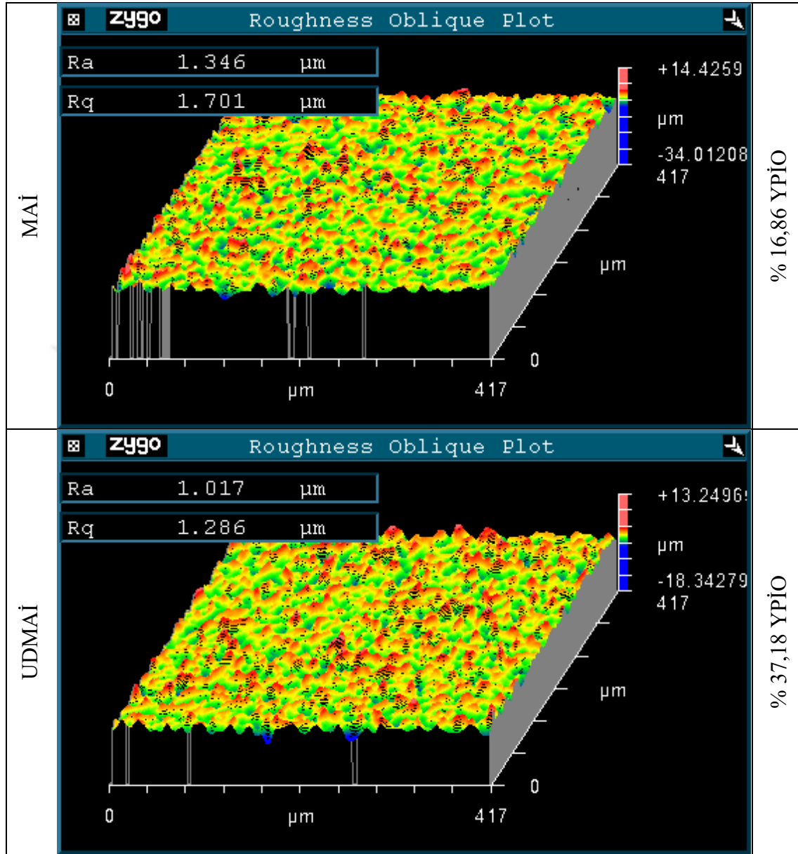
Resim 1.5. 5. deneylere ait numunelerin 3B yüzey topografyası
