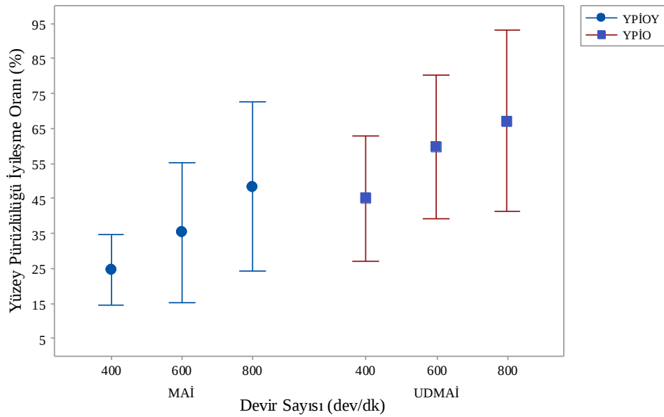
Şekil 6.8. MAİ ve UDMAİ yönteminde devir sayısının YPİO üzerine etkisi
