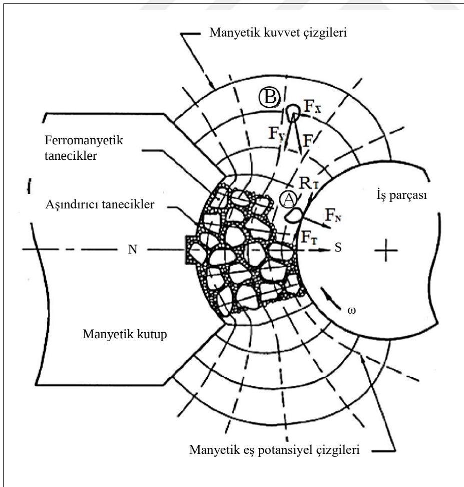
Şekil 3.3. MAİ yönteminde manyetik alan dağılımı ve taneciklere etki eden kuvvetler [1]
