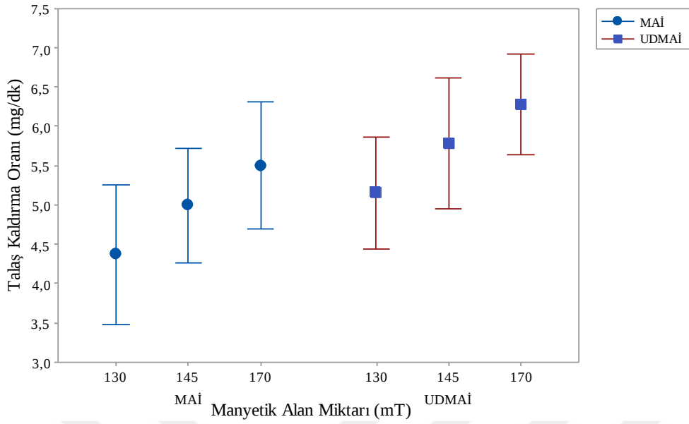
Şekil 6.4. MAİ ve UDMAİ yönteminde manyetik alan miktarının TKO üzerine etkisi
