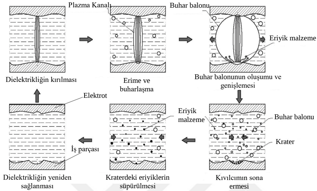
Şekil 2.1. EEİ yönteminde talaş kaldırma mekanizması [27]
