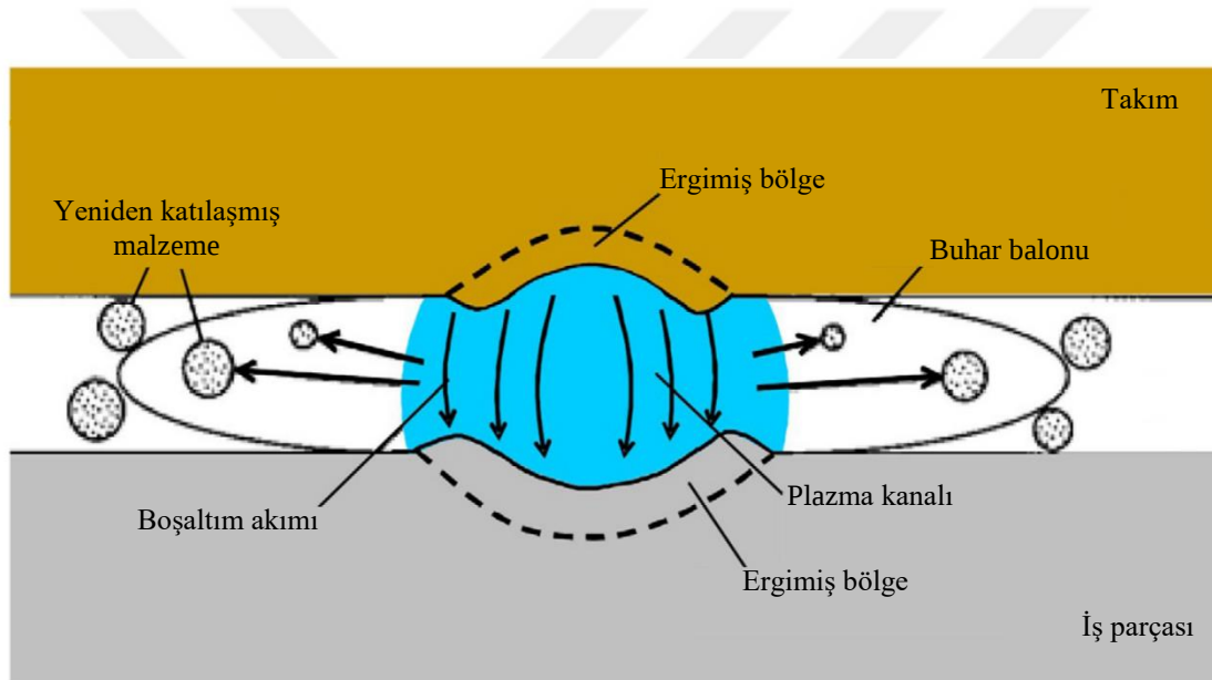
Şekil 2.2. Boşaltım noktasının detaylı modeli [30]
