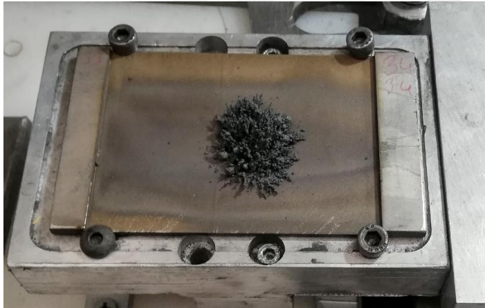
Resim 5.8. Numune üzerinde fırça şeklini alan manyetik aşındırıcı karışımı
