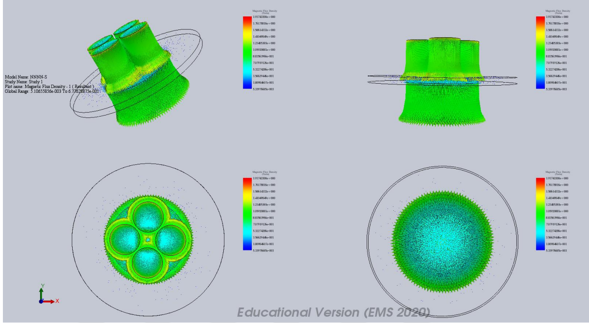
Şekil 5.9. NNNN-S oryantasyonuna sahip kutup sisteminde manyetik alan yoğunluğu
