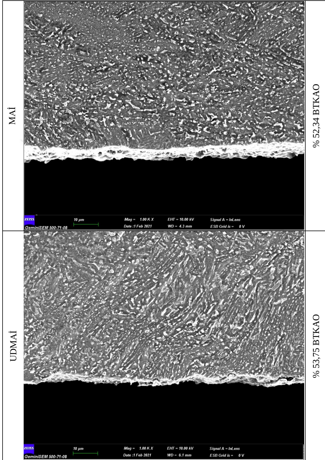
Resim 2.5 5. deneylere ait beyaz tabaka görüntüleri
