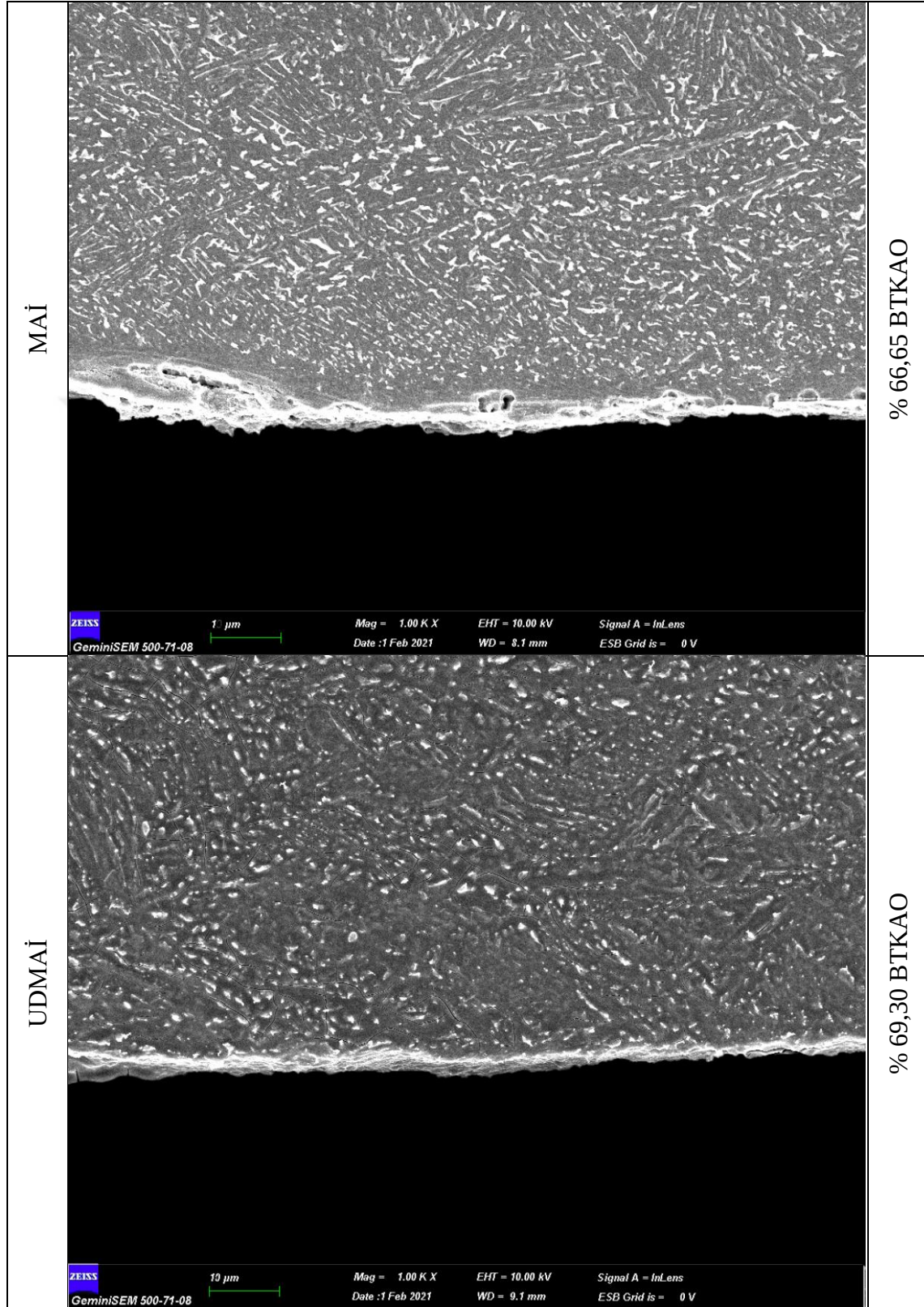
Resim 2.9. 9. deneylere ait beyaz tabaka görüntüleri
