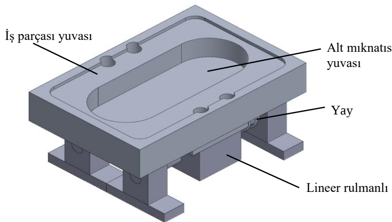
Şekil 5.3. İş parçası tutucusu
