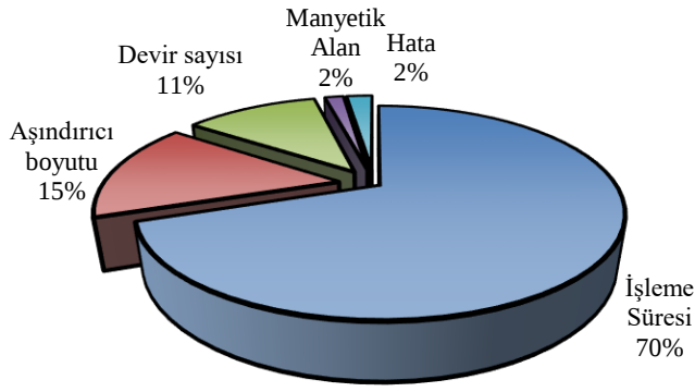
Şekil 7.11. MAİ yönteminde işleme parametrelerinin beyaz tabaka kalınlığı üzerindeki katkıları
