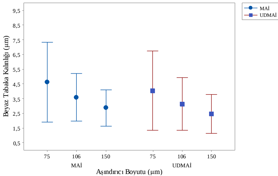
Şekil 6.12. MAİ ve UDMAİ yönteminde aşındırıcı boyutunun beyaz tabaka kalınlığı üzerine etkisi
