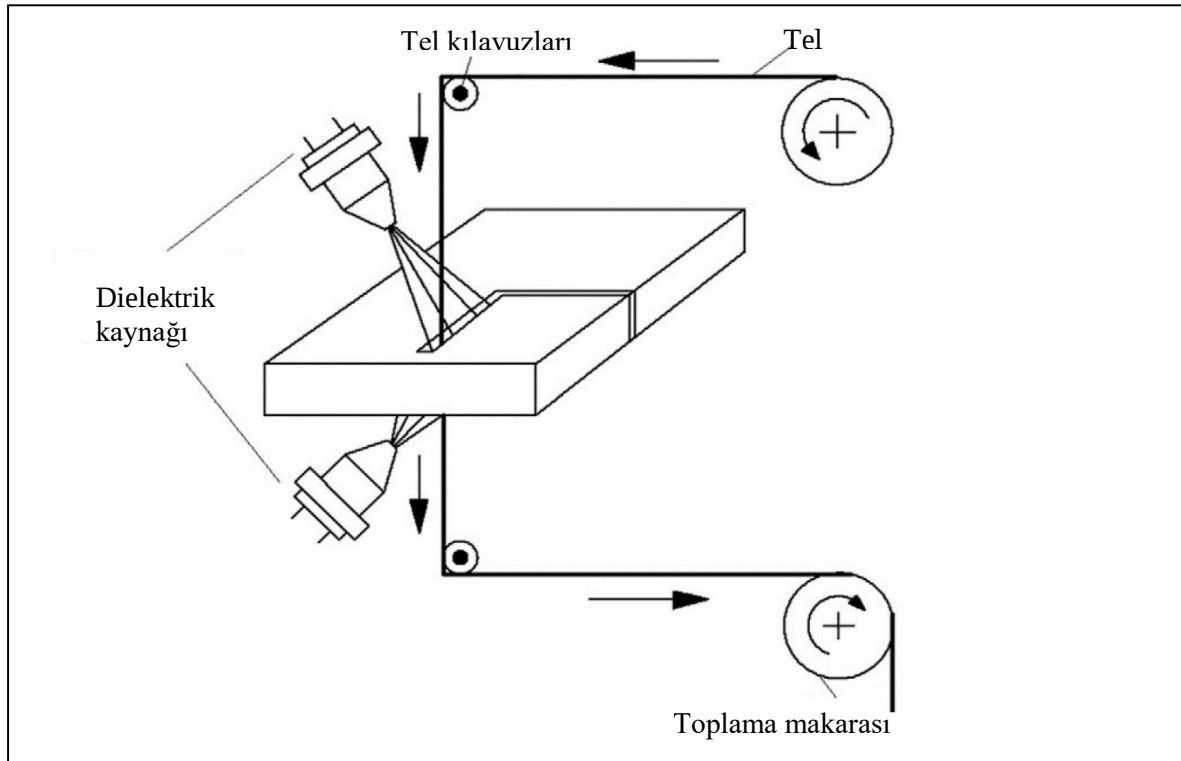
Şekil 2.4. TEİ yönteminin çalışma prensibinin şematik gösterimi [27]
