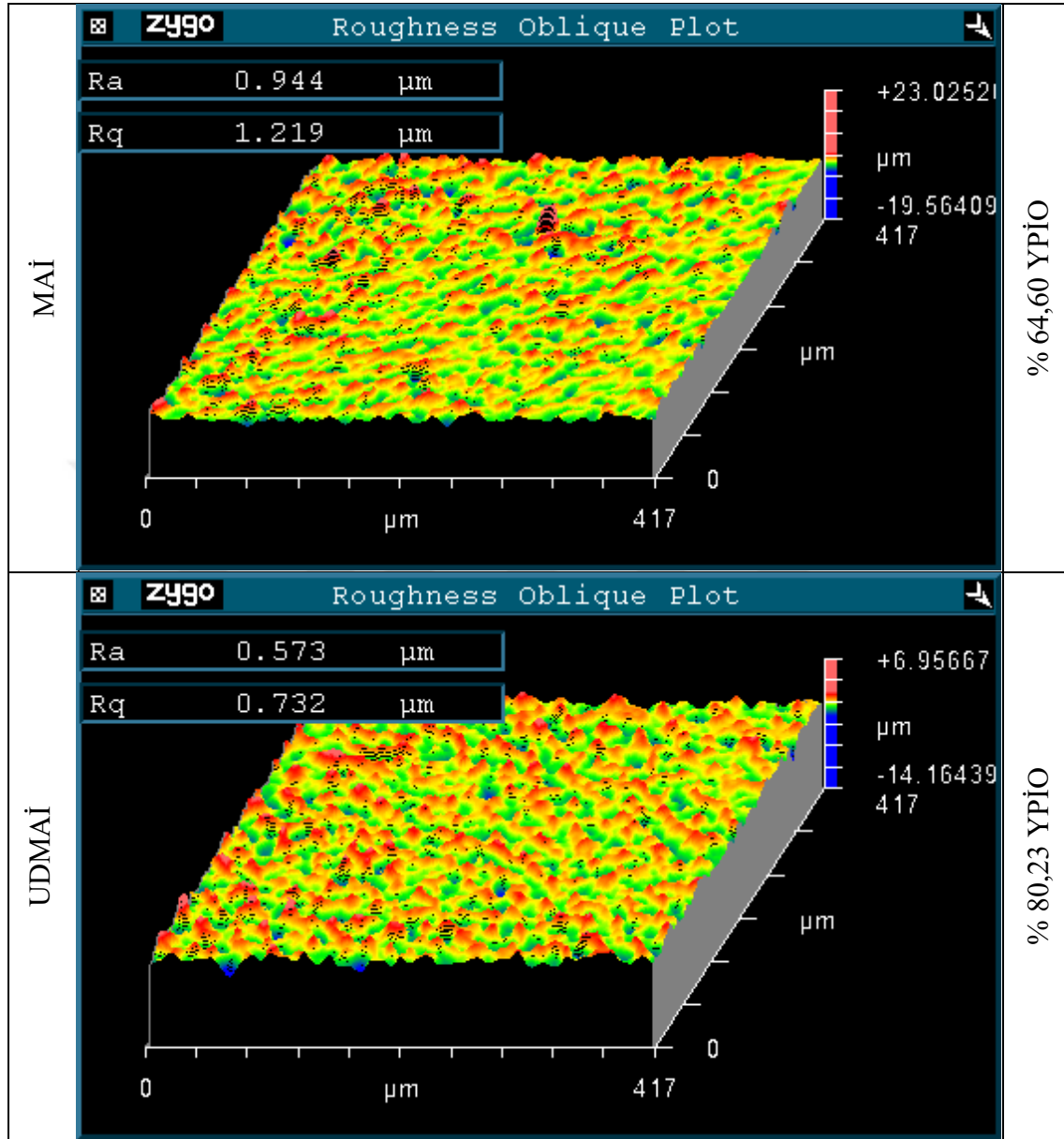
Resim 1.8. 8. deneylere ait numunelerin 3B yüzey topografyası
