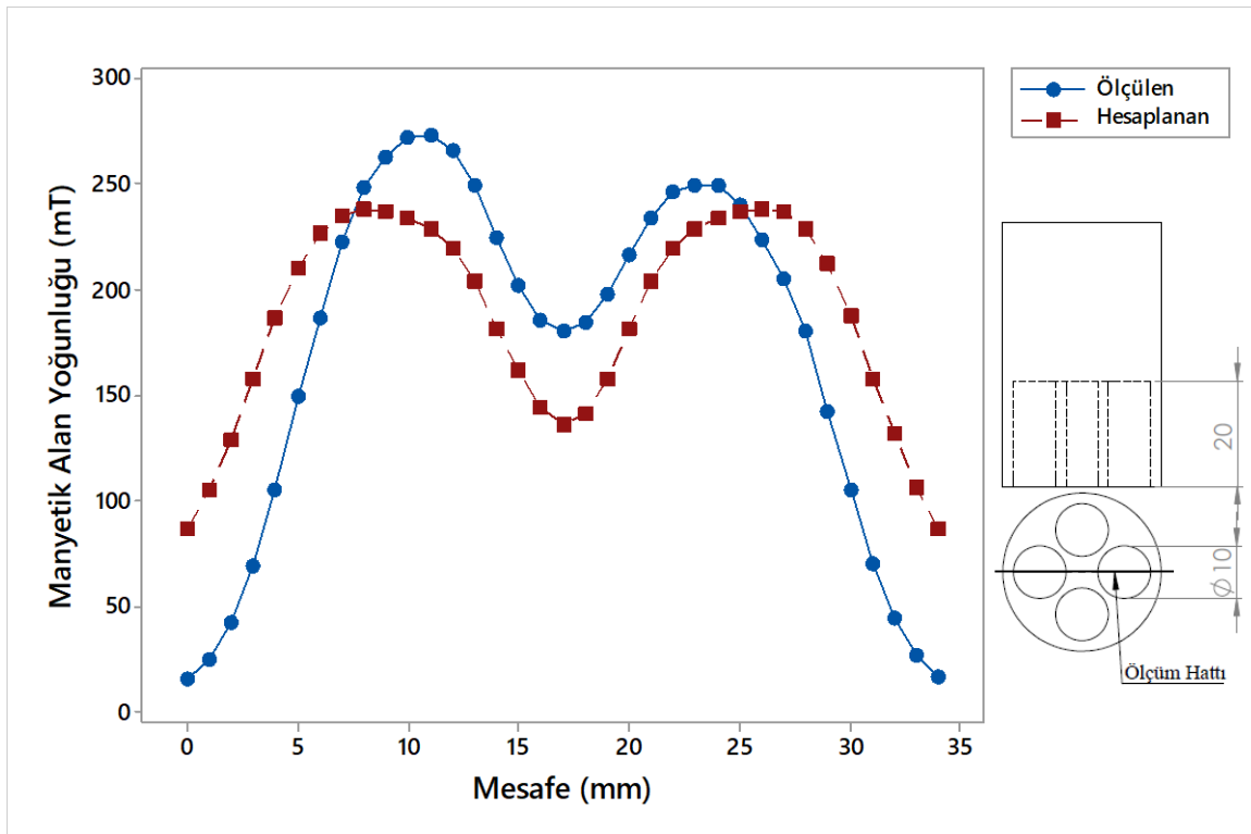
Şekil 5.12. 3 nolu takıma ait kutup boyunca manyetik alan yoğunluğunun değişimi
