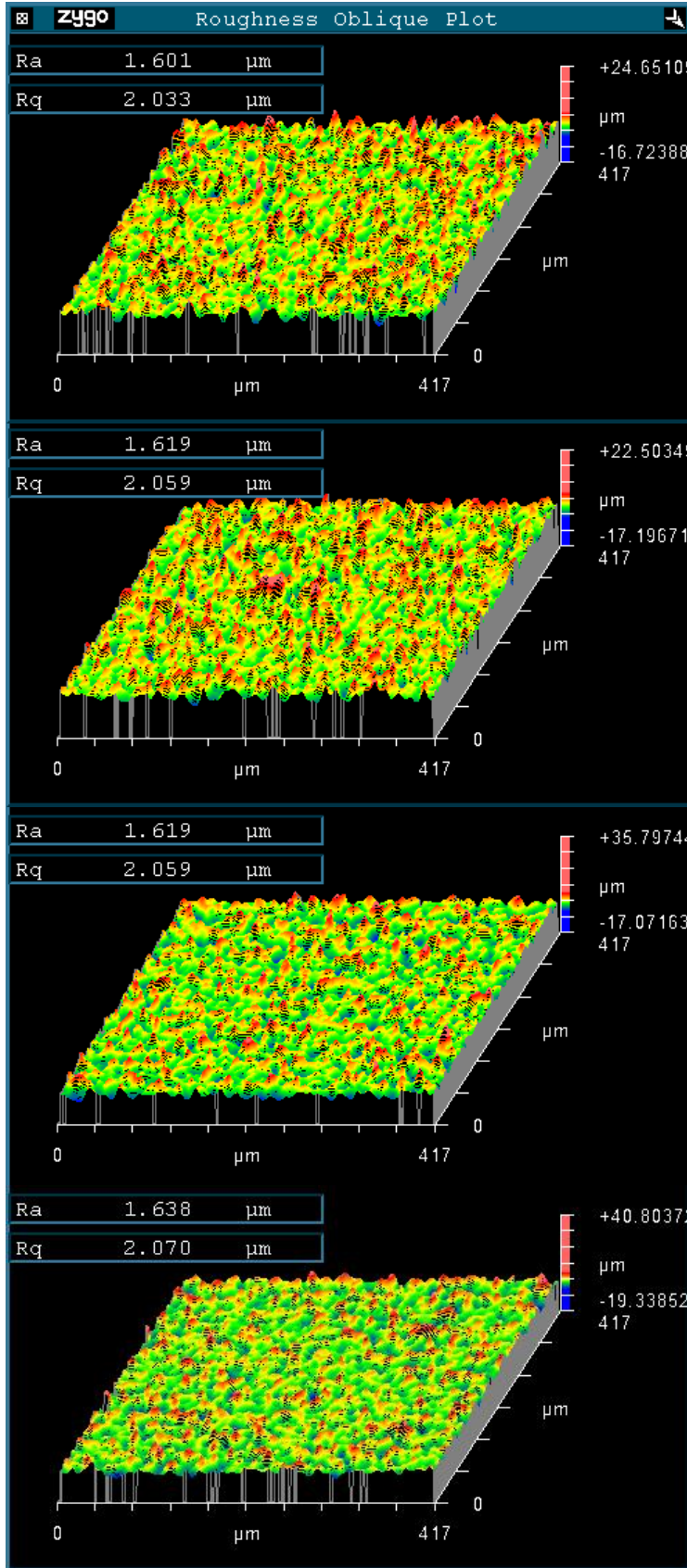
Resim 6.1. TEİ işlemi sonrası numunelerin 3B yüzey topografyası
