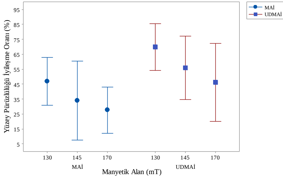
Şekil 6.9. MAİ ve UDMAİ yönteminde manyetik alan miktarının YPİO üzerine etkisi
