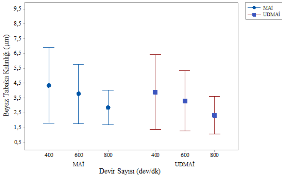
Şekil 6.13. MAİ ve UDMAİ yönteminde devir sayısının beyaz tabaka kalınlığı üzerine etkisi
