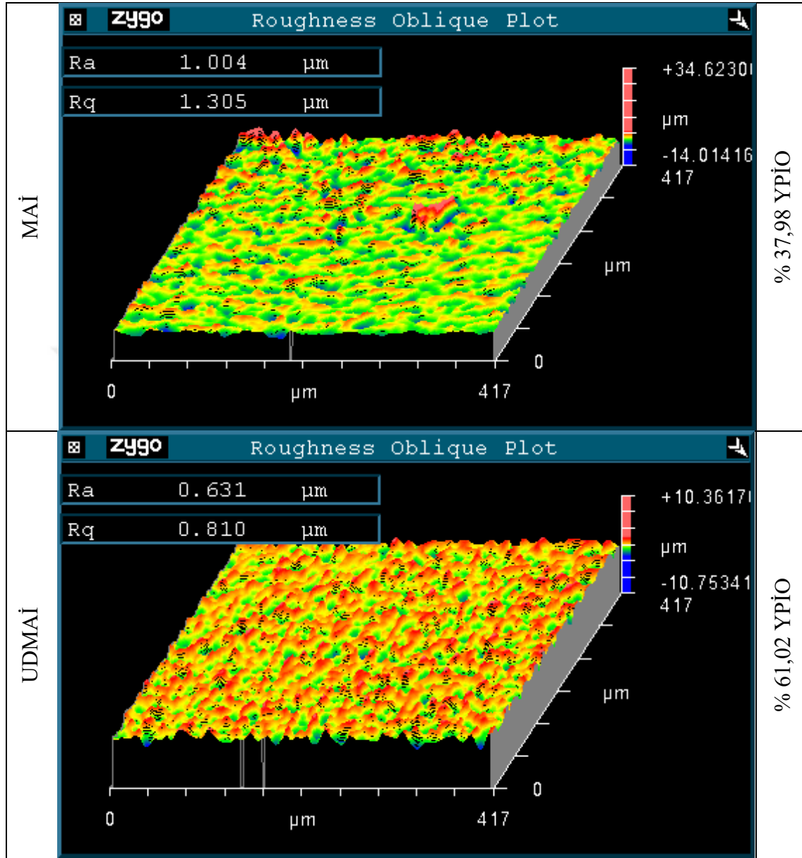
Resim 1.6. 6. deneylere ait numunelerin 3B yüzey topografyası
