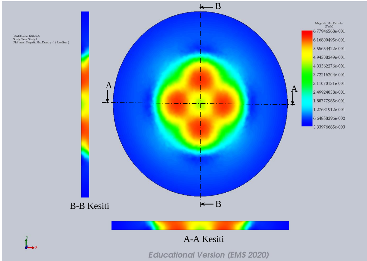
Şekil 5.7. NNNN-S oryantasyonuna sahip kutup sisteminde iş parçasına etkiyen manyetik alan
