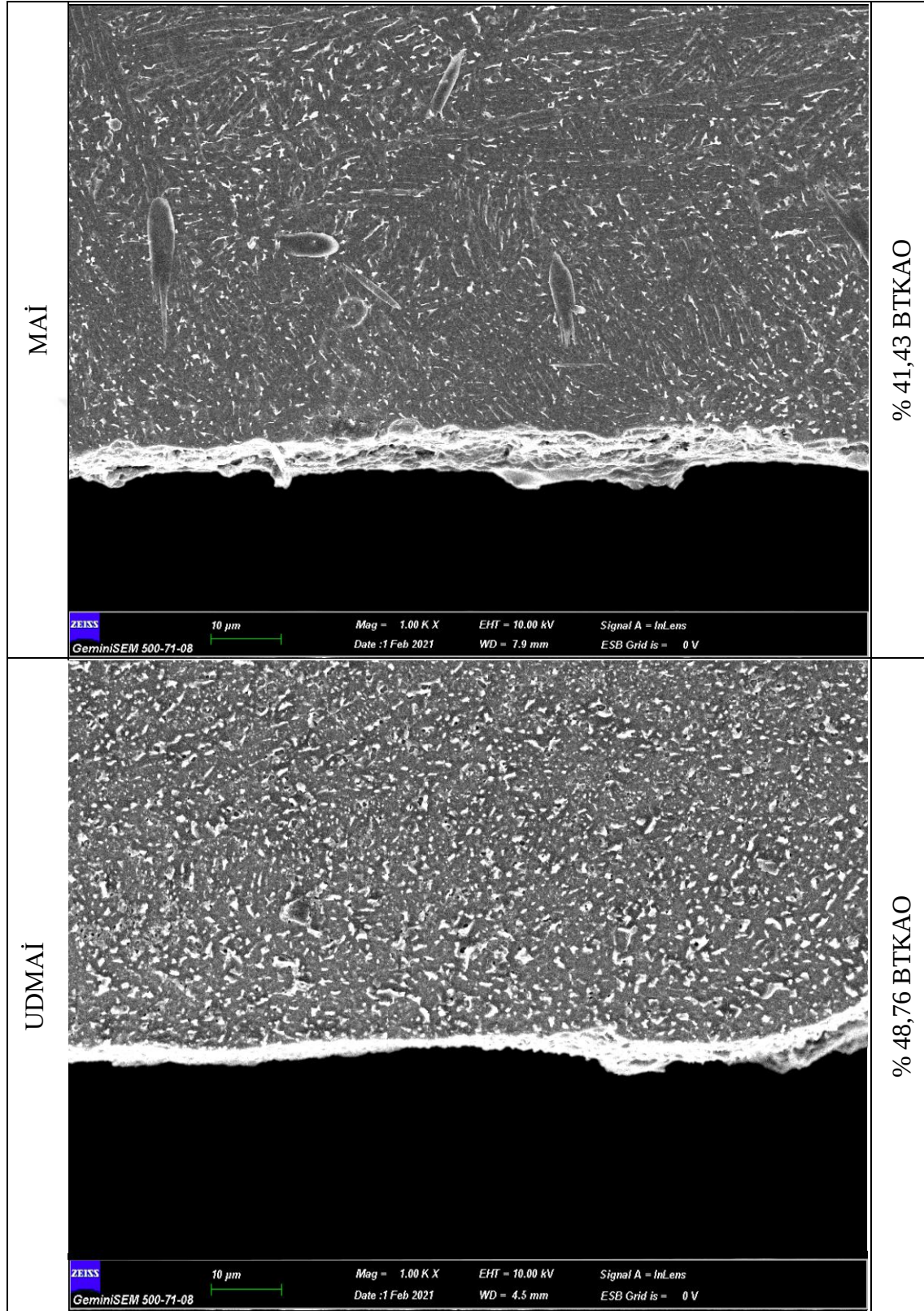
Resim 2.7. 7. deneylere ait beyaz tabaka görüntüleri
