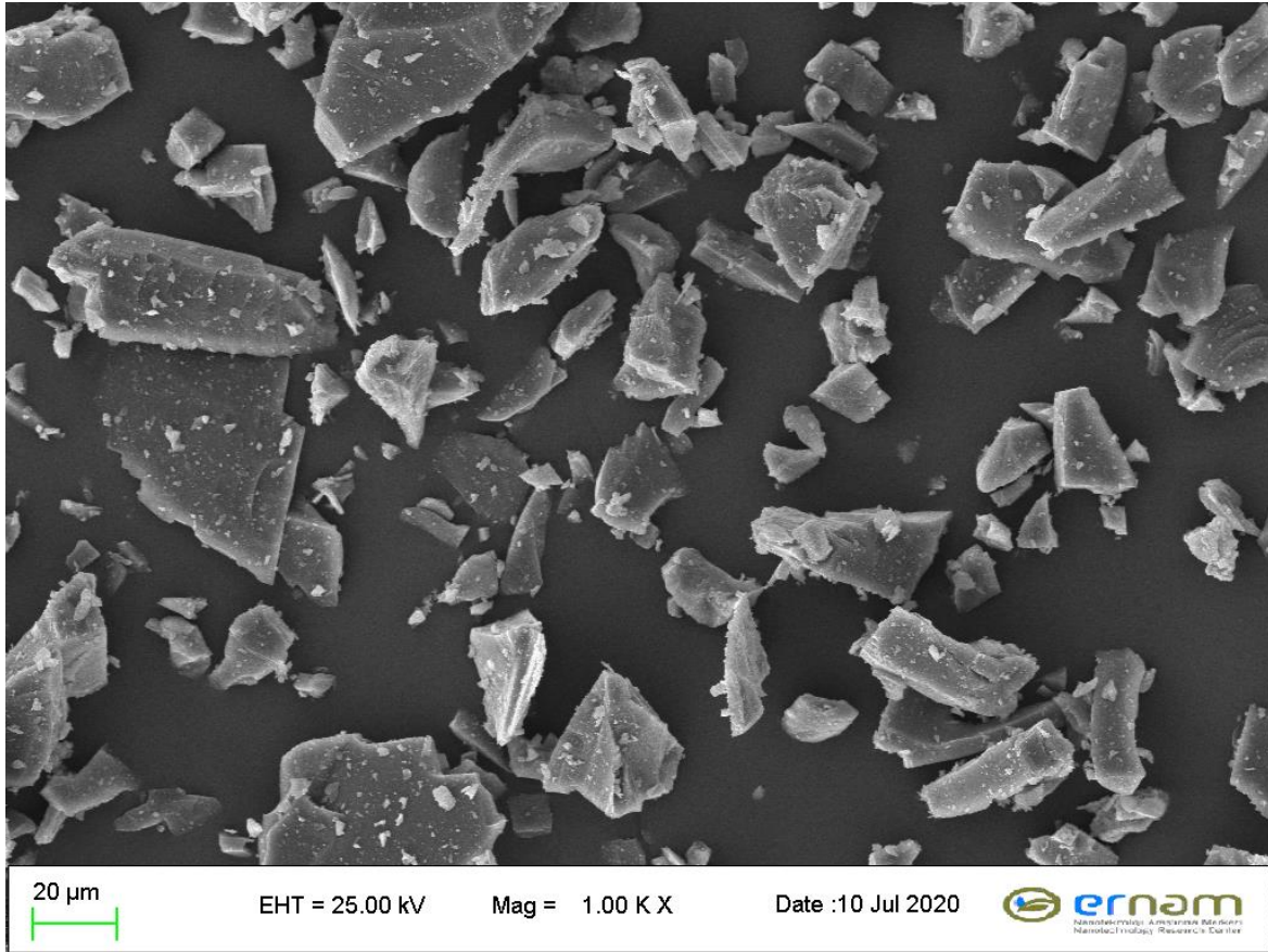
Resim 5.6. SiC taneciklerin SEM görüntüsü
