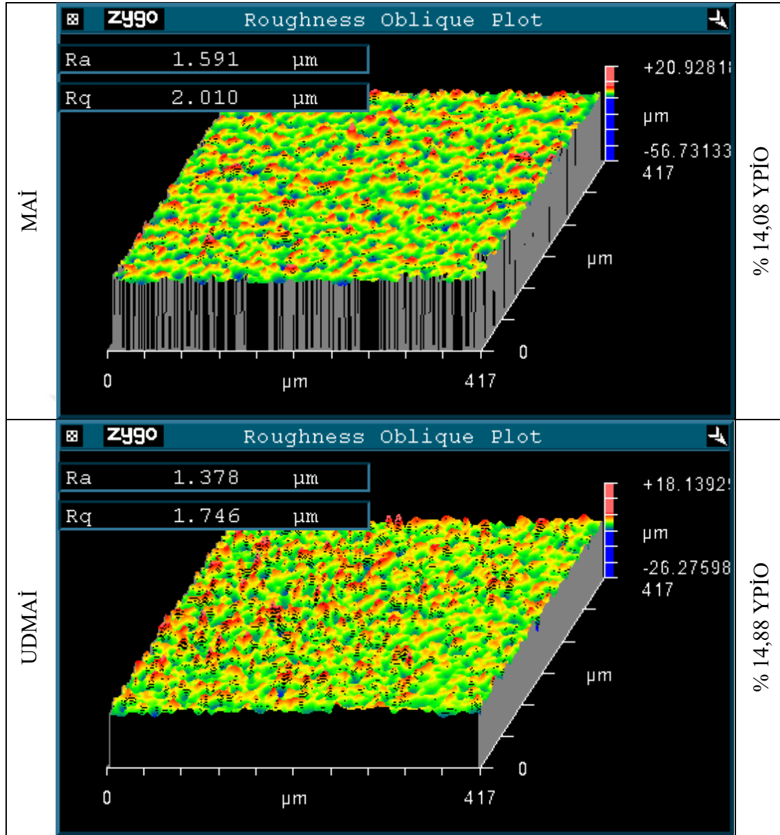
Resim 6.2. En düşük YPİO değerine sahip numunelerin 3B yüzey topografyası
