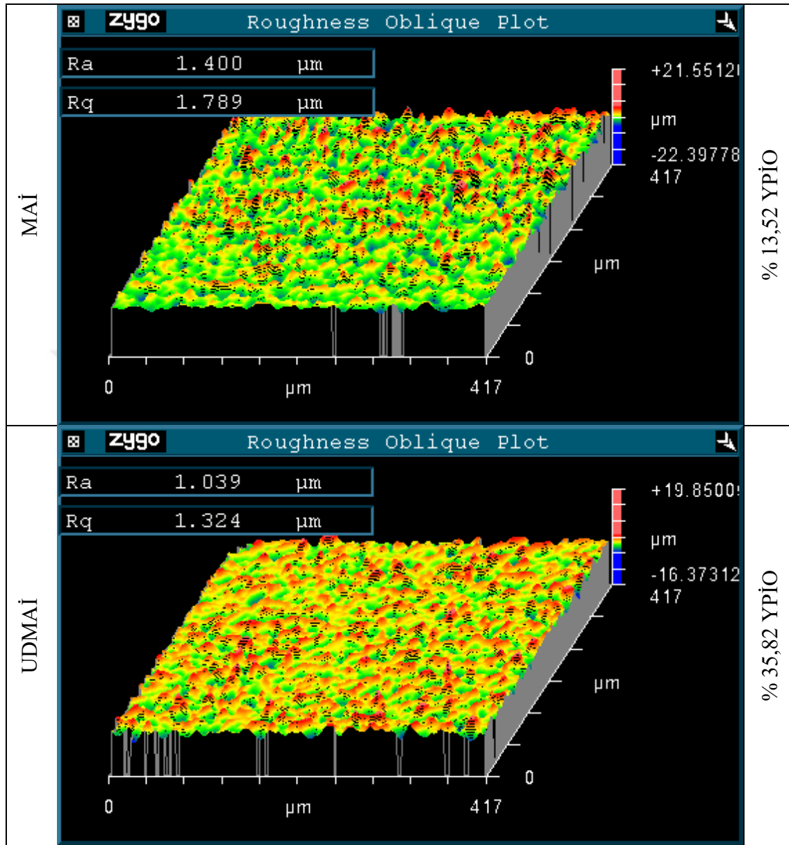
Resim 1.2. 2. deneylere ait numunelerin 3B yüzey topografyası
