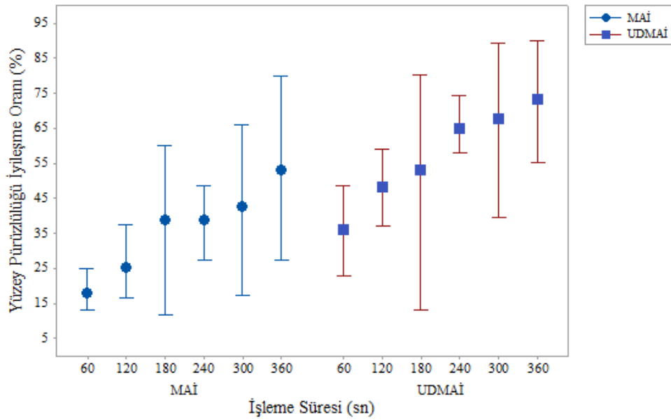
Şekil 6.6. MAİ ve UDMAİ yönteminde işleme süresinin YPİO üzerine etkisi
