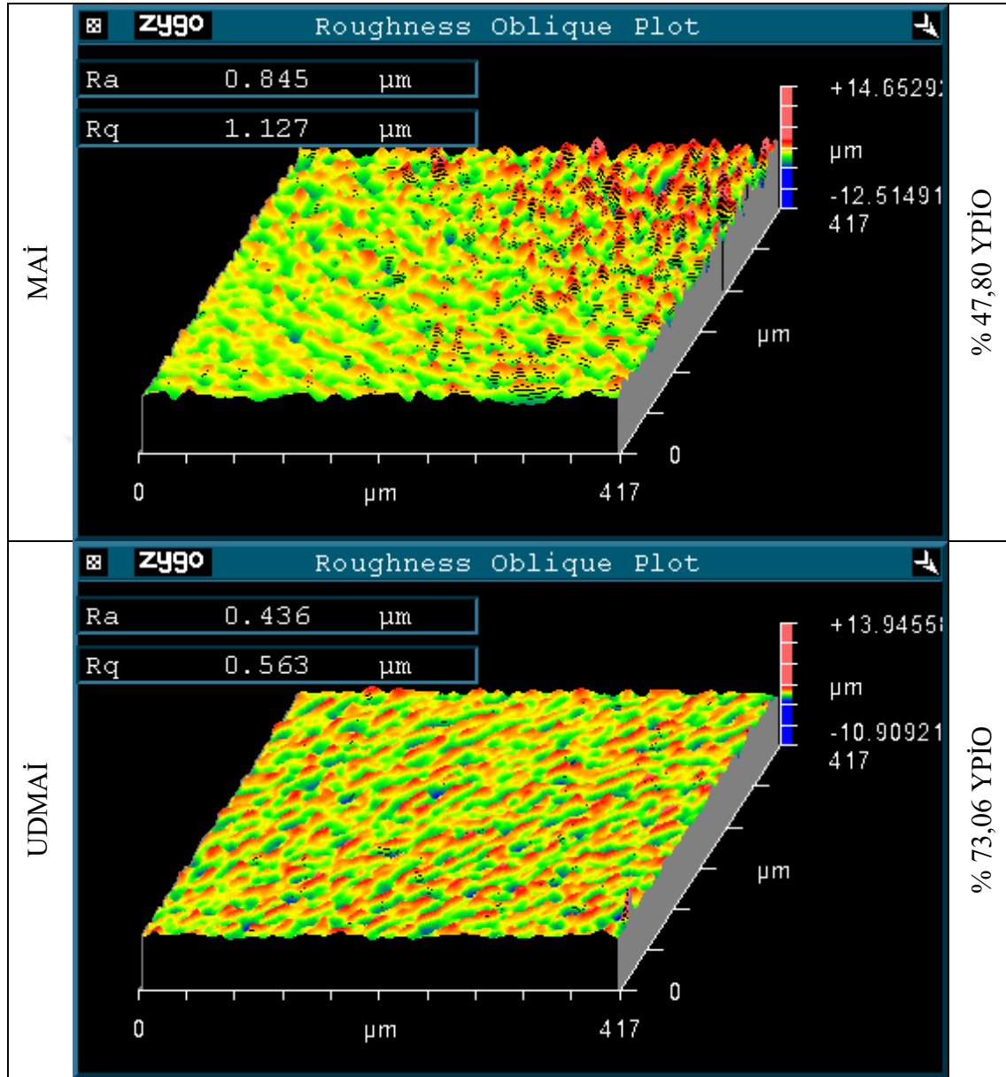
Resim 1.10. 10. deneylere ait numunelerin 3B yüzey topografyası
