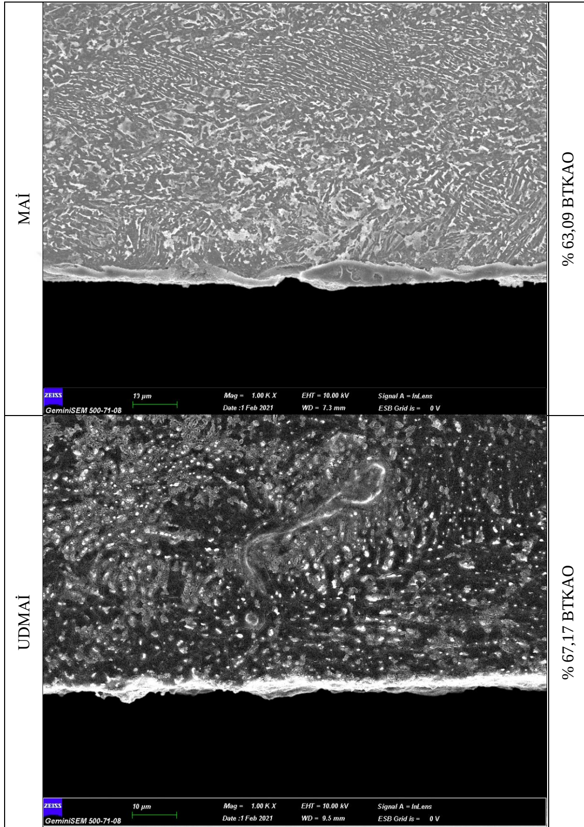
Resim 2.11. 11. deneylere ait beyaz tabaka görüntüleri
