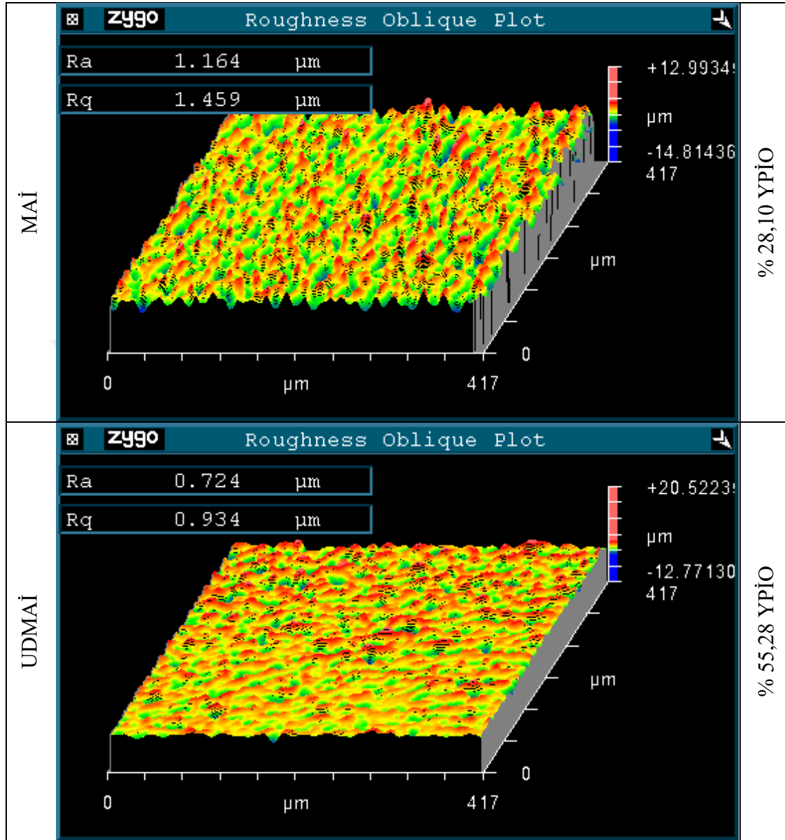
Resim 1.17. 17. deneylere ait numunelerin 3B yüzey topografyası
