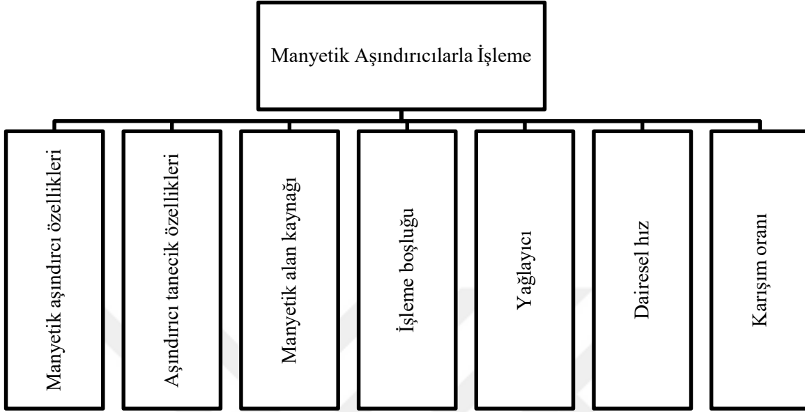
Şekil 3.6. MAİ yöntemini etkileyen parametreler
