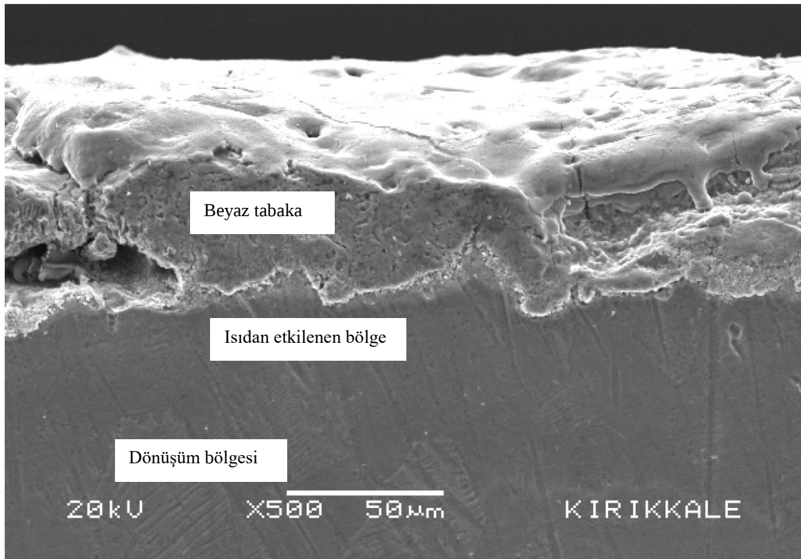
Resim 2.1. EEİ ile işlenmiş bir yüzeyin komşu yüzeyinin SEM görüntüsü [23]
