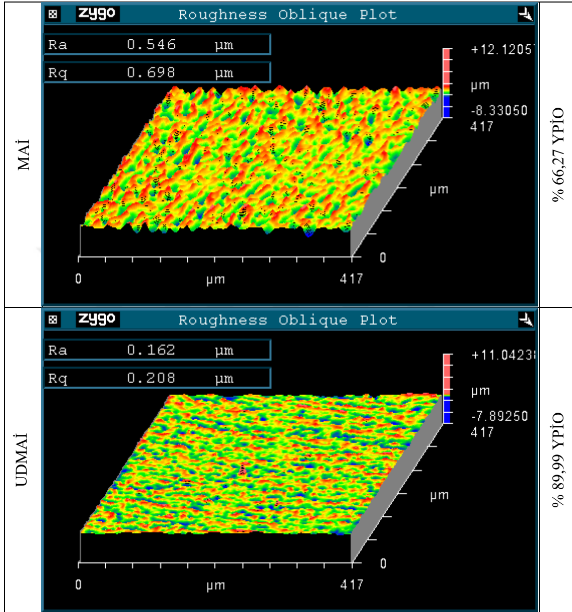
Resim 1.14. 14. deneylere ait numunelerin 3B yüzey topografyası
