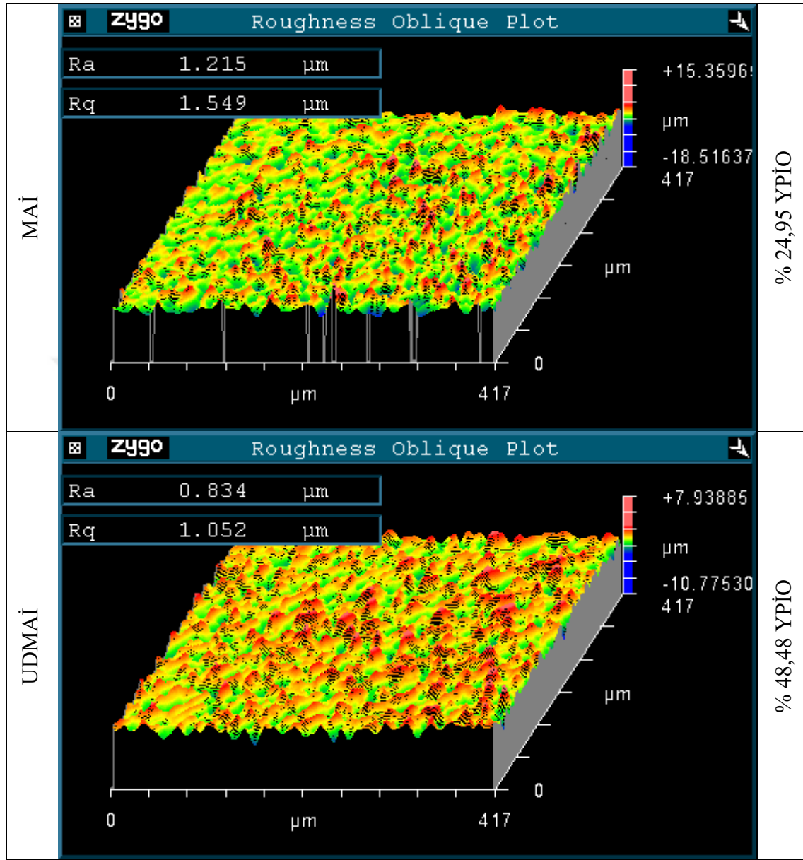
Resim 1.1. 1. deneylere ait numunelerin 3B yüzey topografyası
