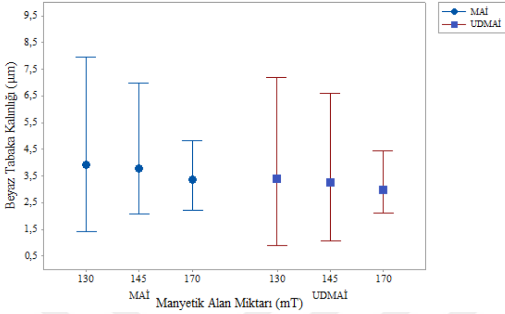
Şekil 6.14. MAİ ve UDMAİ yönteminde manyetik alan miktarının beyaz tabaka kalınlığı üzerine etkisi
