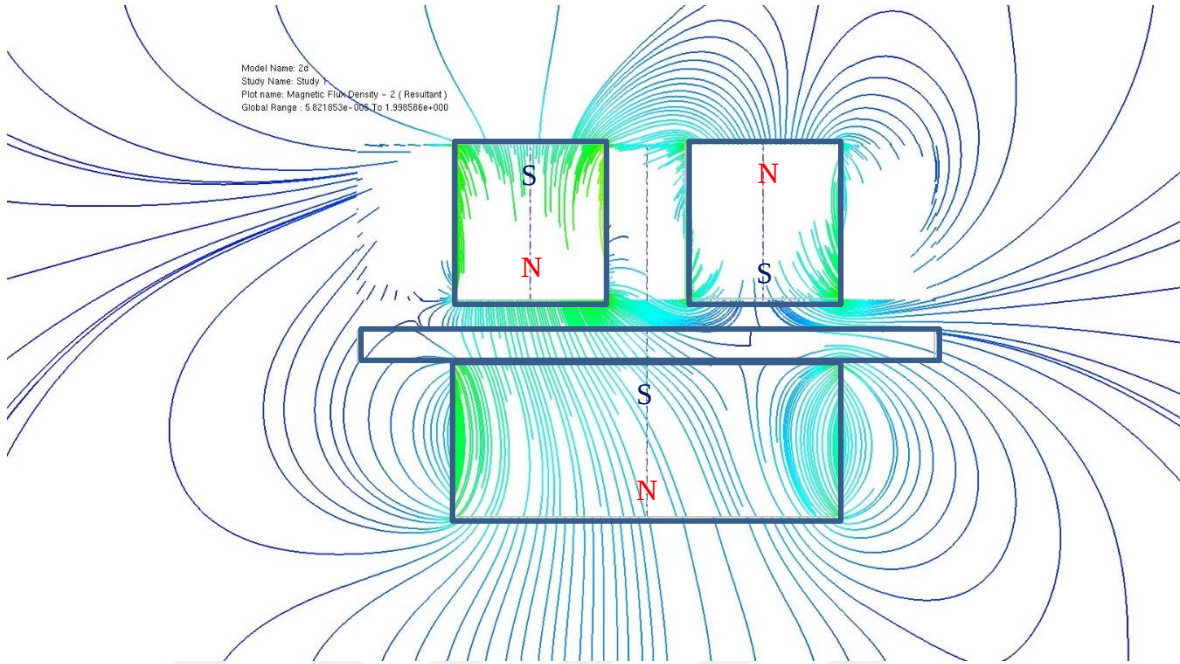
Şekil 5.4. NSNS-S manyetik kutup sistemine ait manyetik alan çizgileri
