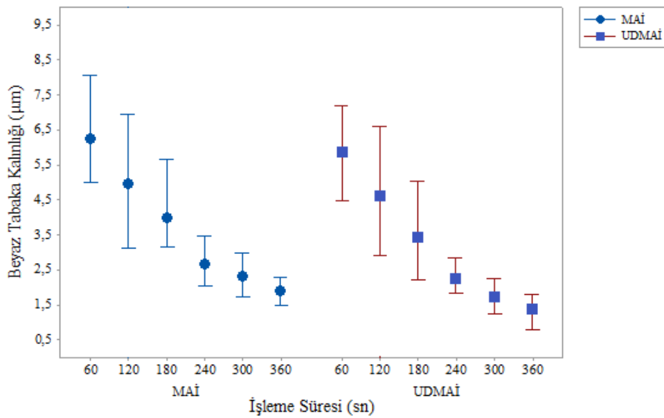
Şekil 6.11. MAİ ve UDMAİ yönteminde işleme süresinin beyaz tabaka kalınlığı üzerine etkisi
