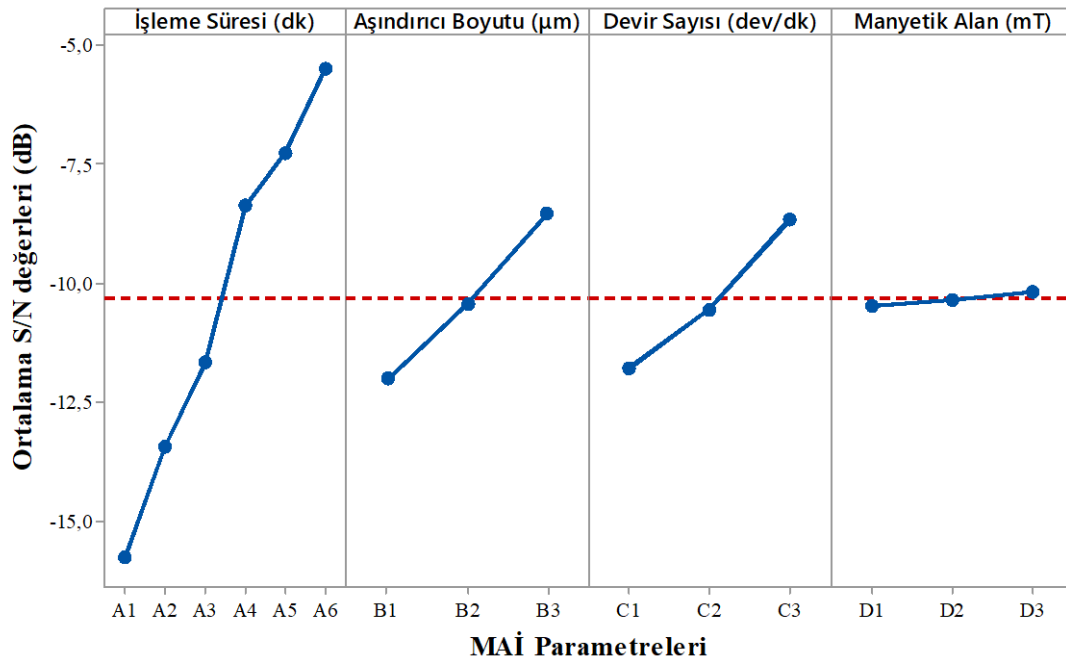
Şekil 7.9. MAİ yönteminde işleme parametrelerinin beyaz tabaka kalınlığı üzerindeki etkisi
