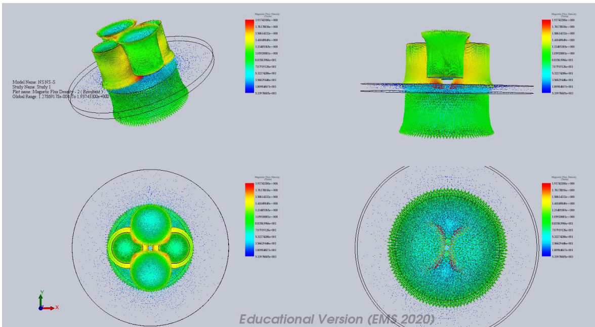
Şekil 5.8. NSNS-S oryantasyonuna sahip kutup sisteminde manyetik alan yoğunluğu
