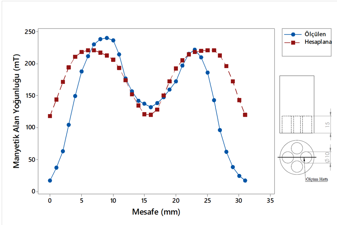
Şekil 5.11. 2 nolu takıma ait kutup boyunca manyetik alan yoğunluğunun değişimi
