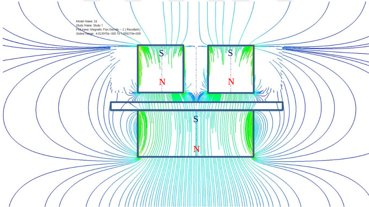
Şekil 5.5. NNNN-S manyetik kutup sistemine ait manyetik alan çizgileri
