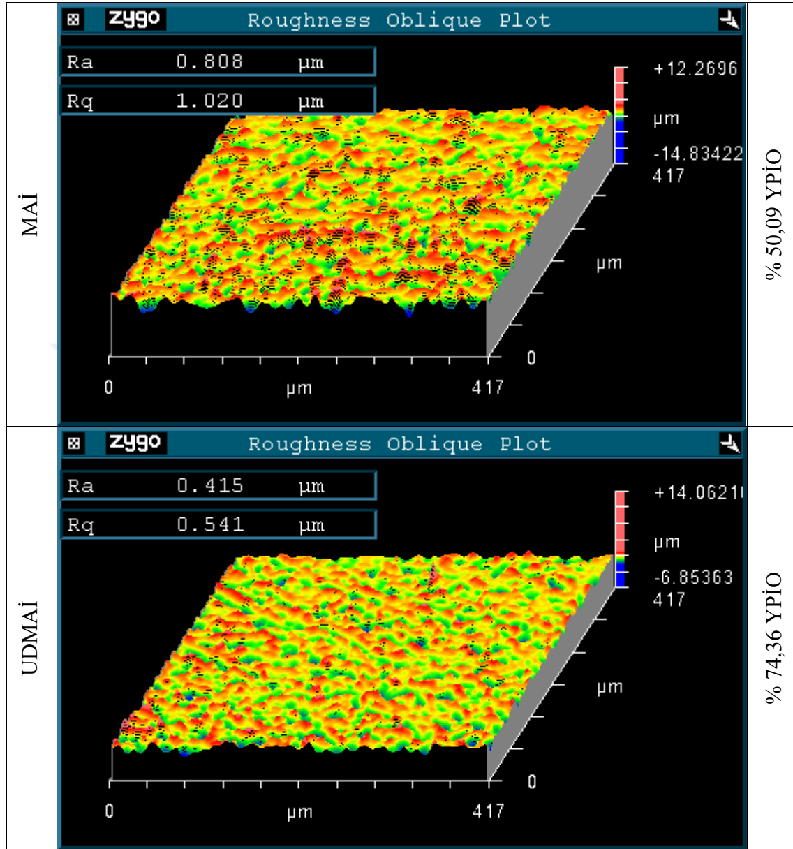
Resim 1.18. 18. deneylere ait numunelerin 3B yüzey topografyası
