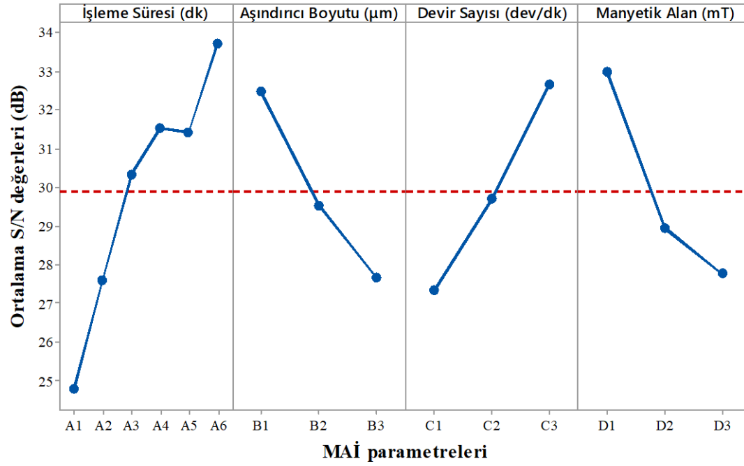
Şekil 7.5. MAİ yönteminde işleme parametrelerinin yüzey pürüzlülüğü iyileşme oranına etkisi
