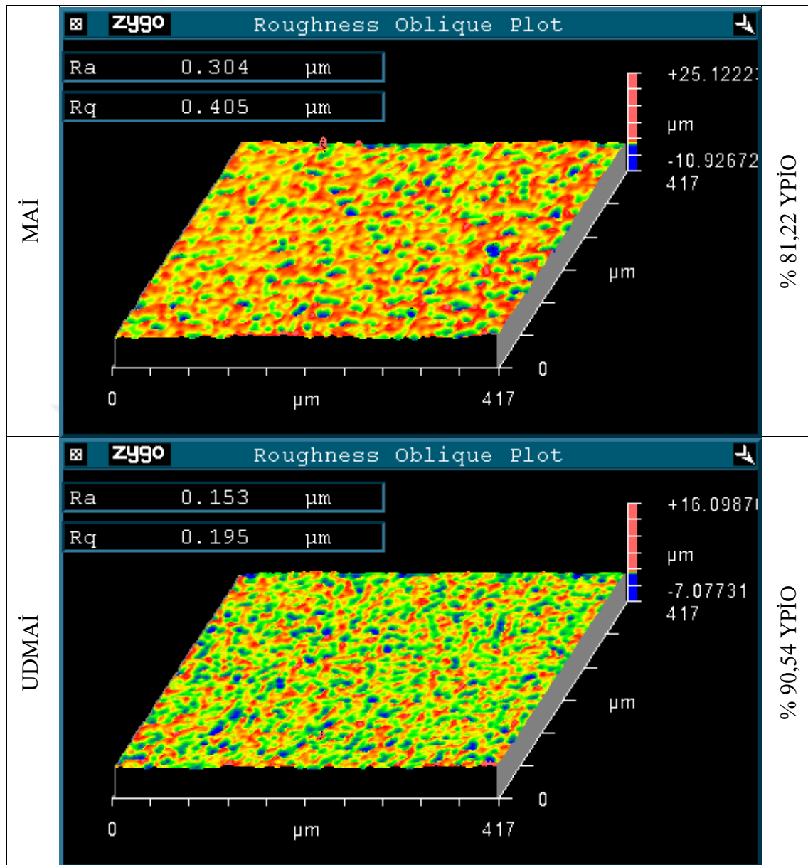
Resim 6.3. En yüksek YPİO değerine sahip numunelerin 3B yüzey topografyası
