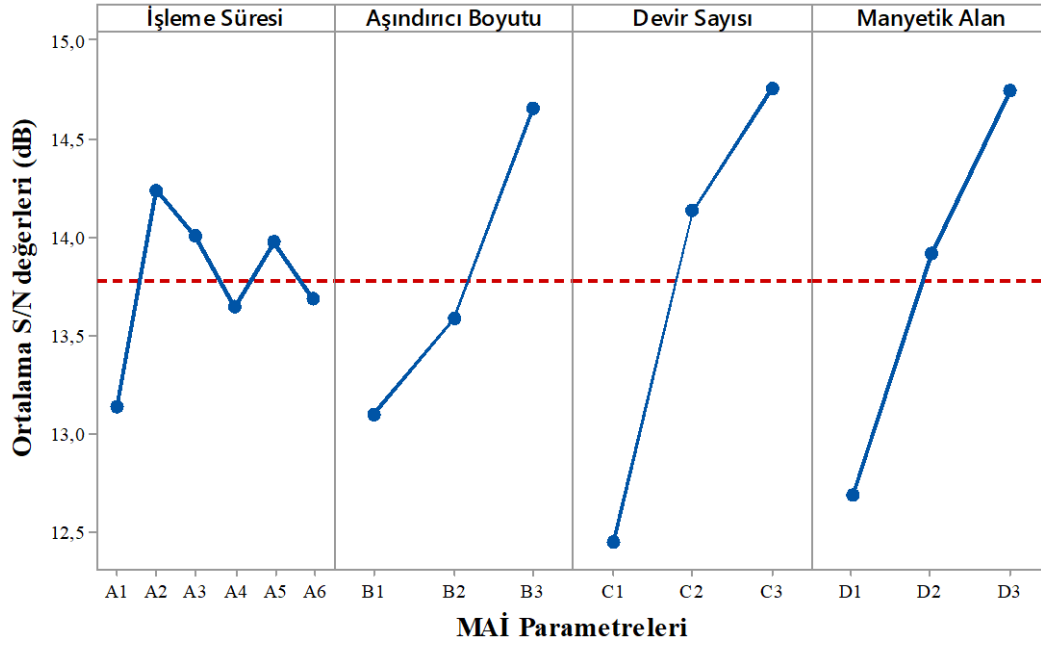
Şekil 7.1. MAİ yönteminde işleme parametrelerinin talaş kaldırma oranına etkisi
