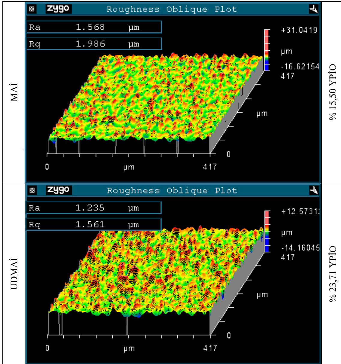
Resim 1.3. 3. deneylere ait numunelerin 3B yüzey topografyası
