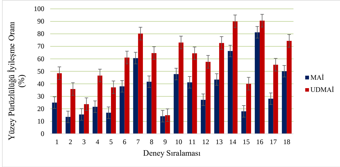
Şekil 6.5. MAİ/UDMAİ deneylerine ait YPİÖ grafiği
