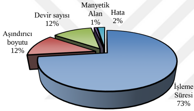
Şekil 7.12. UDMAİ yönteminde işleme parametrelerinin beyaz tabaka kalınlığı üzerindeki katkıları
