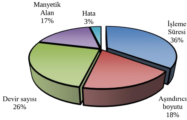
Şekil 7.7. MAİ yönteminde işleme parametrelerinin YPIÖ üzerindeki katkıları
