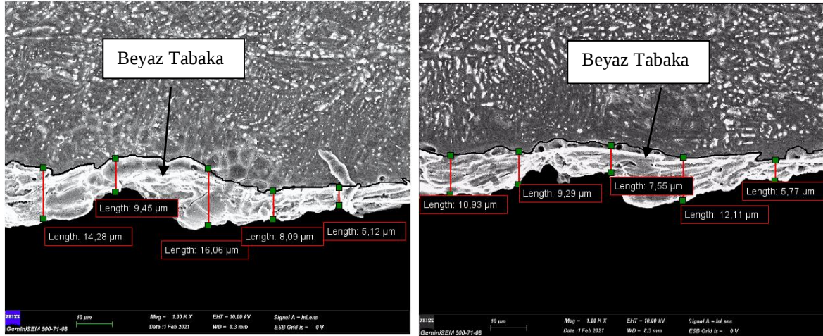
Resim 6.4. TEİ işlemi sonrası yüzeyde oluşan beyaz tabaka görüntüleri
