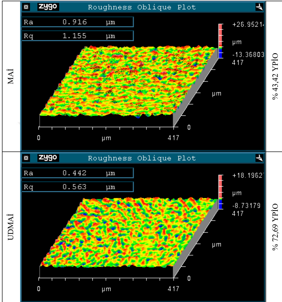
Resim 1.13. 13. deneylere ait numunelerin 3B yüzey topografyası
