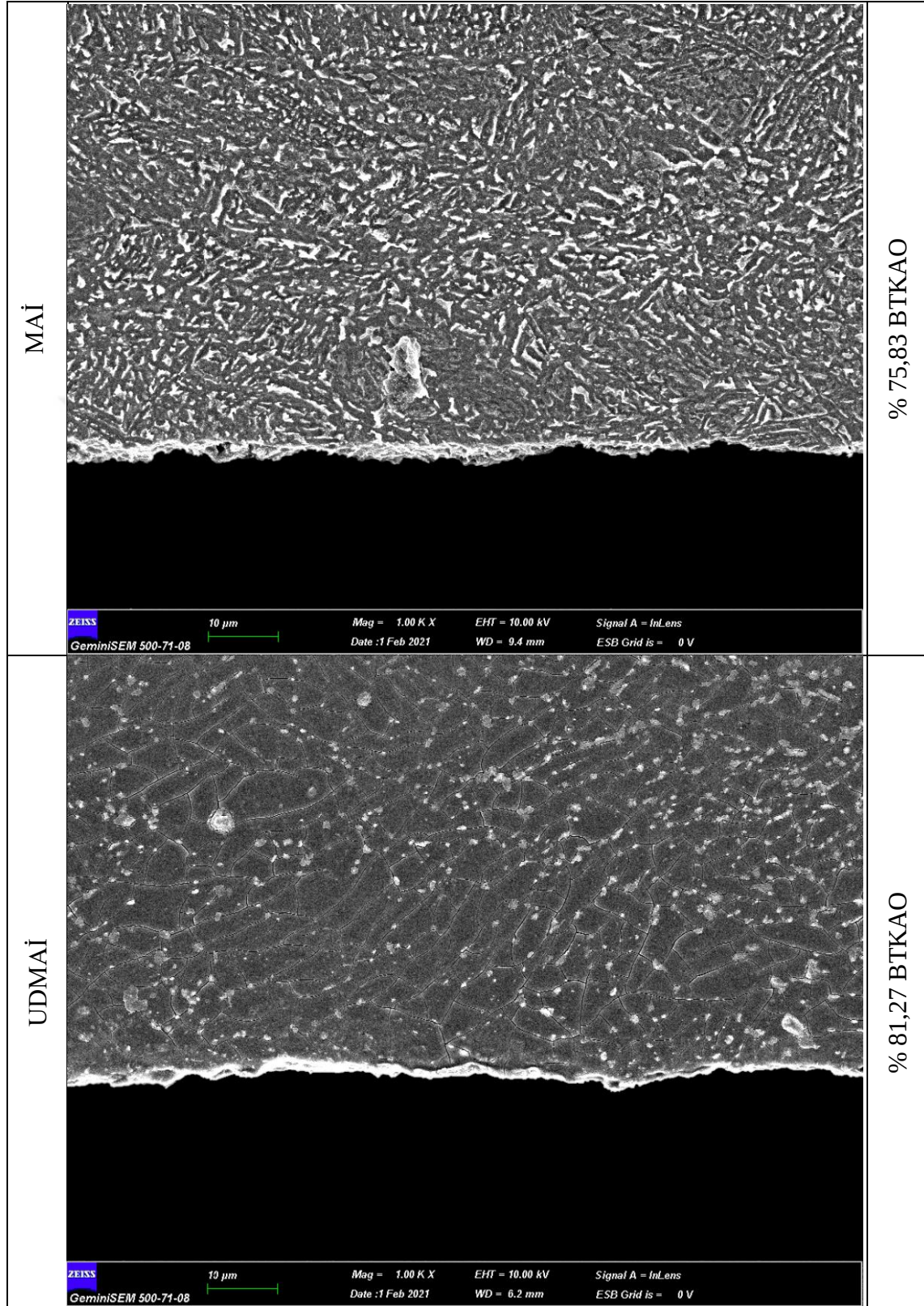
Resim 2.17. 17. deneylere ait beyaz tabaka görüntüleri
