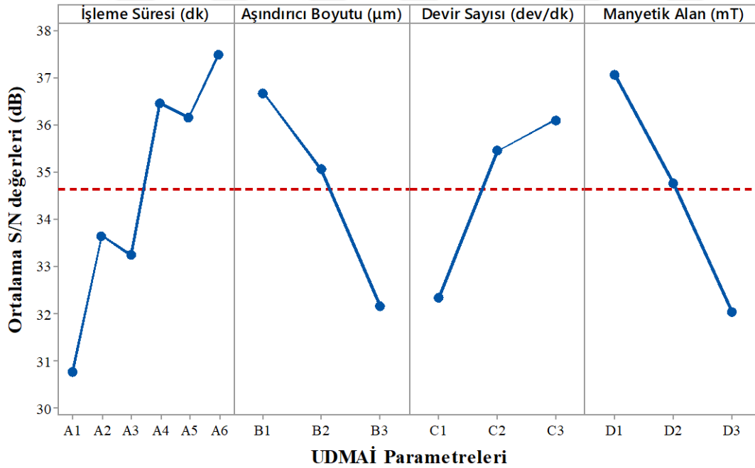
Şekil 7.6. UDMAİ yönteminde işleme parametrelerinin yüzey pürüzlülüğü iyileşme oranına etkisi
