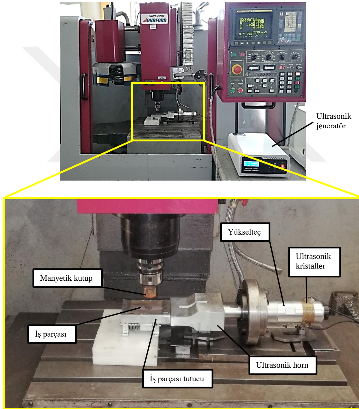
Resim 5.5. Deney düzeneğinin fotoğrafı
