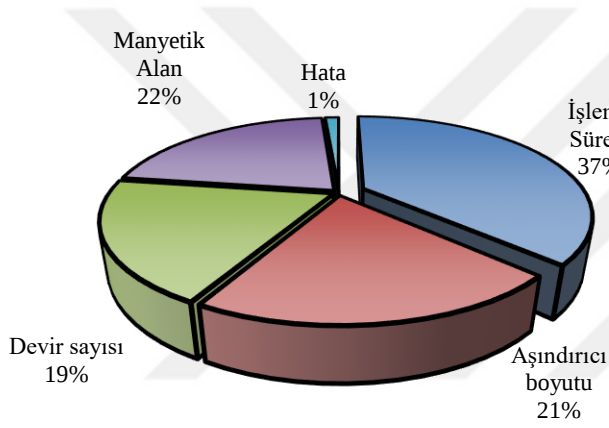
Şekil 7.8. UDMAİ yönteminde işleme parametrelerinin YPIÖ üzerindeki katkıları
