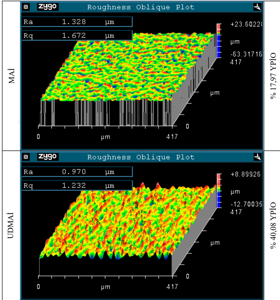
Resim 1.15. 15. deneylere ait numunelerin 3B yüzey topografyası
