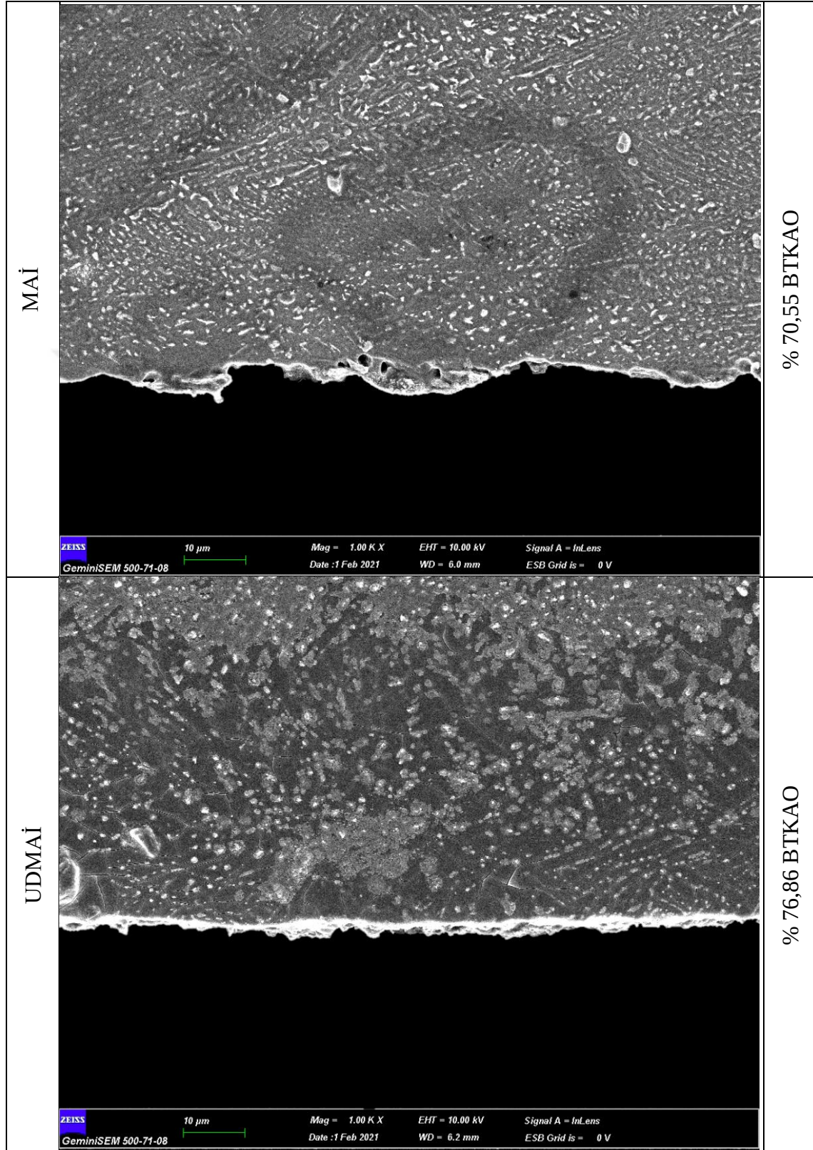
Resim 2.13. 13. deneylere ait beyaz tabaka görüntüleri
