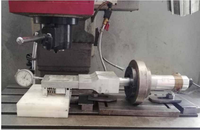
Resim 5.4. İş parçası genliğinin ölçülmesi
