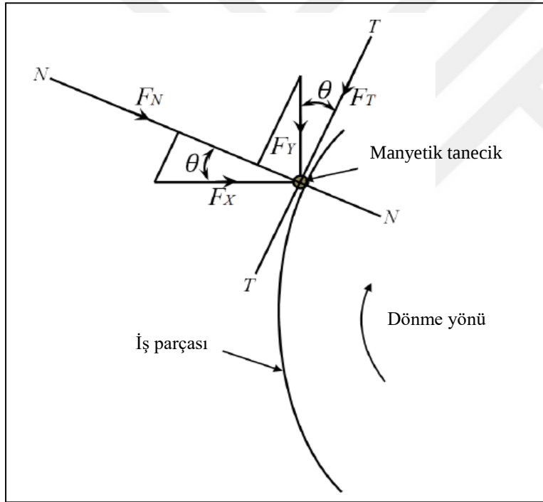
Şekil 3.5. MAİ yönteminde manyetik tanecik üzerine etki eden kuvvetlerin şematik gösterimi [42]
