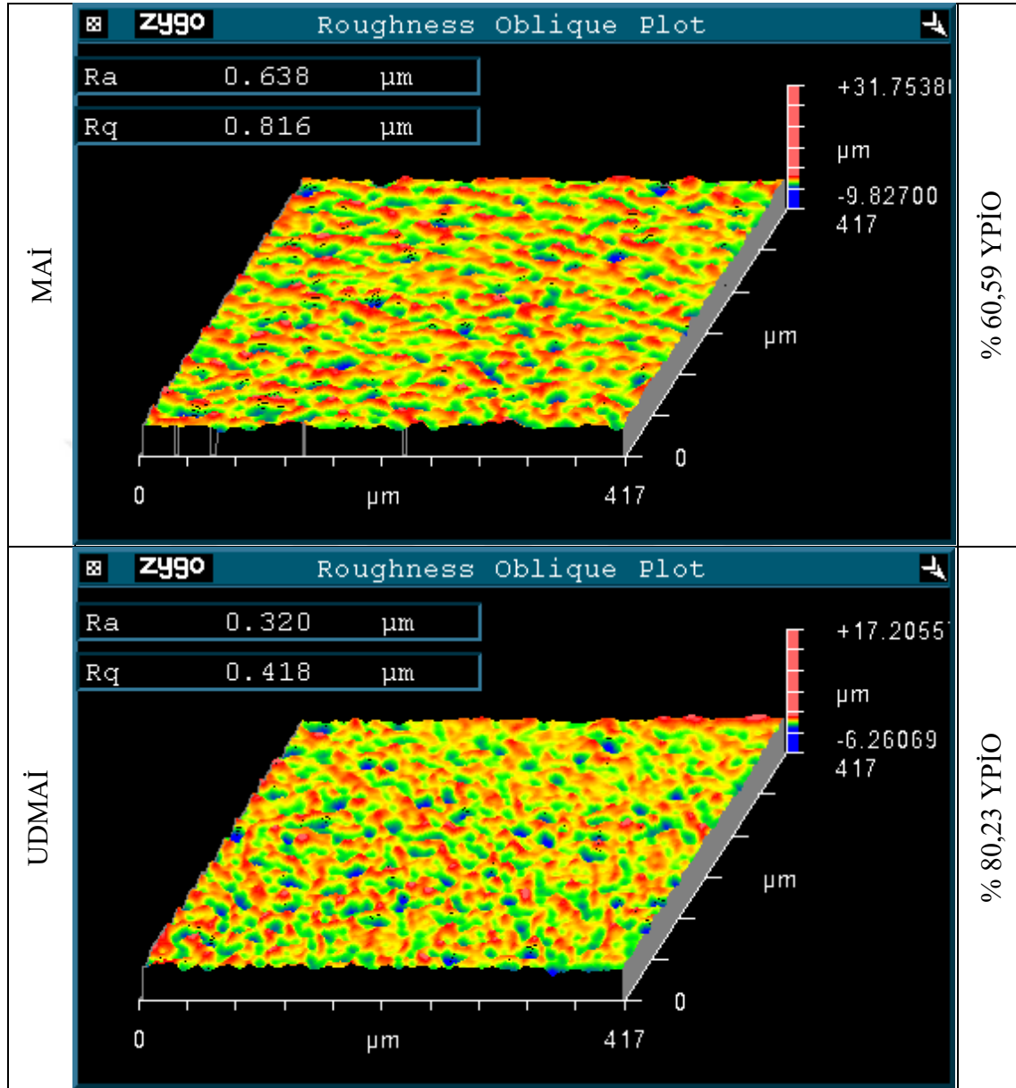
Resim 1.7. 7. deneylere ait numunelerin 3B yüzey topografyası
