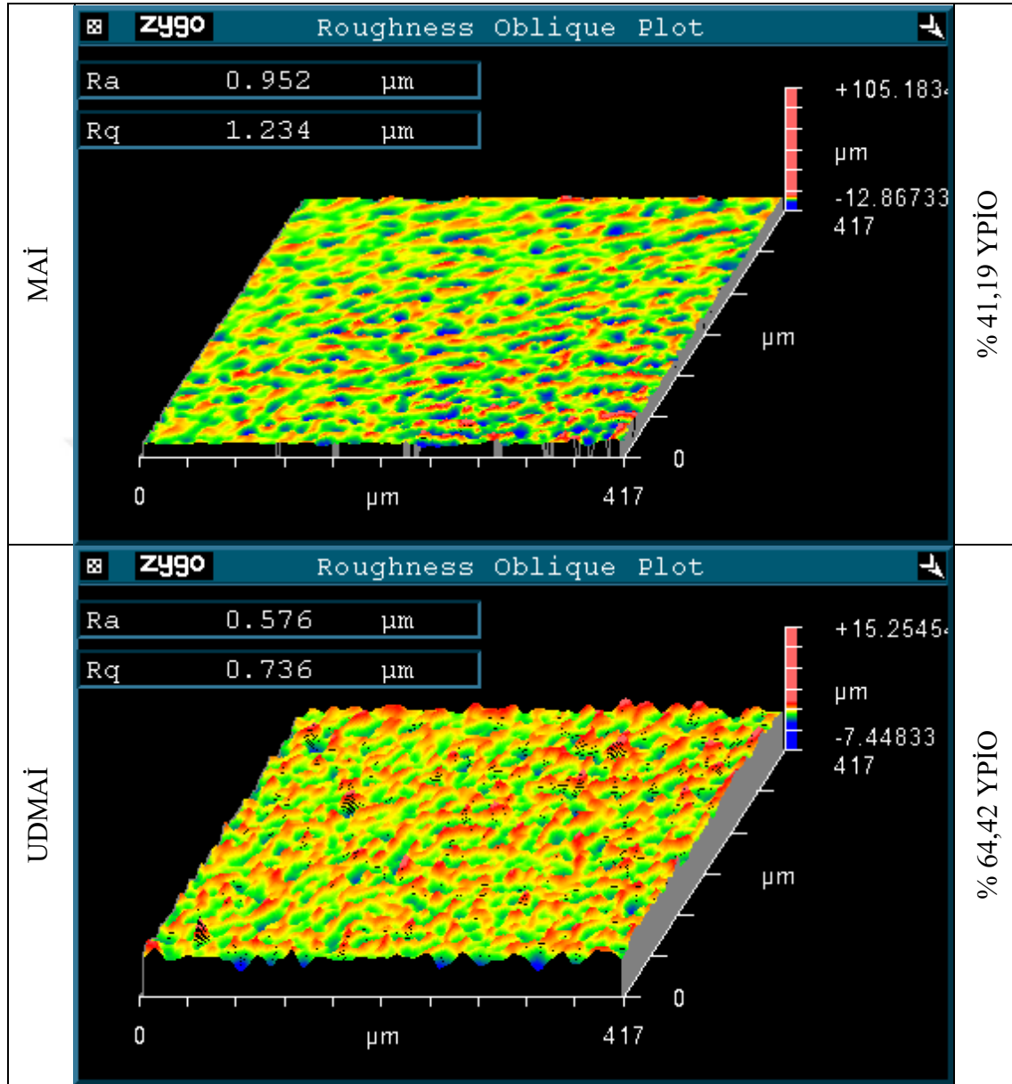
Resim 1.11. 11. deneylere ait numunelerin 3B yüzey topografyası
