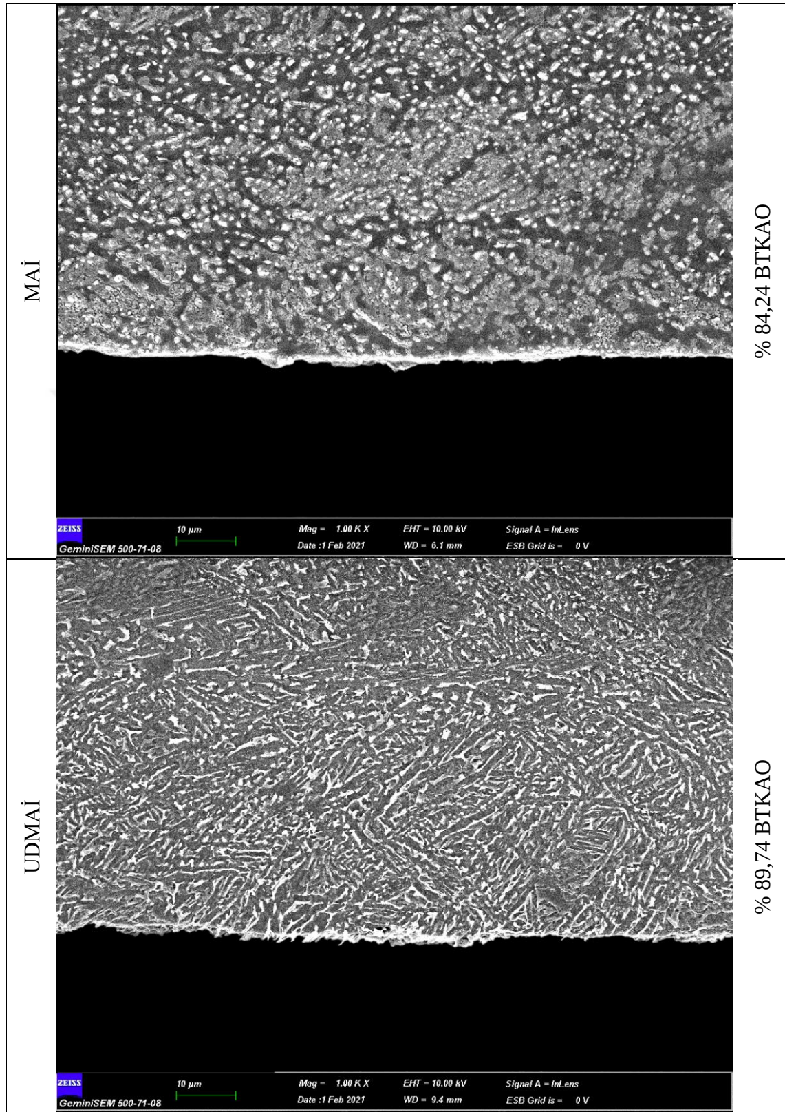
Resim 6.6 En yüksek BTKAO değerine sahip numunelere ait SEM görüntüleri
