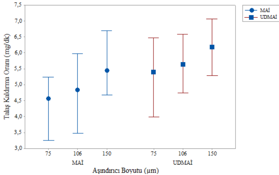
Şekil 6.2. MAİ ve UDMAİ yönteminde aşındırıcı boyutunun TKO üzerine etkisi
