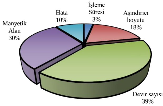
Şekil 7.3. MAİ yönteminde işlem parametrelerinin TKO üzerindeki katkıları
