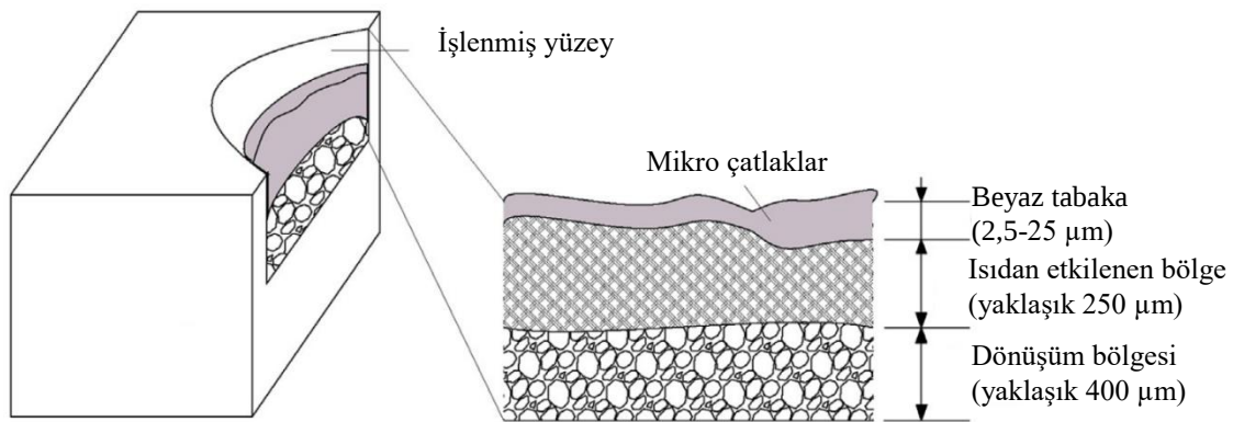
Şekil 2.3. EEİ ile işlenmiş bir yüzeyin ve komşu yüzeyin şematik gösterimi [27]
