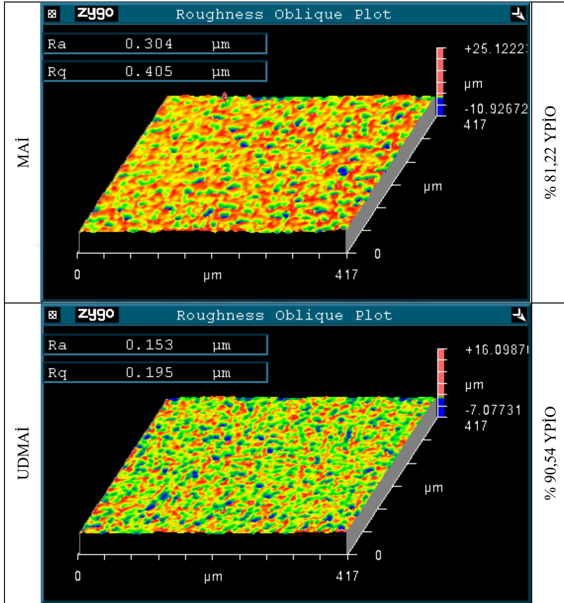
Resim 1.16. 16. deneylere ait numunelerin 3B yüzey topografyası
