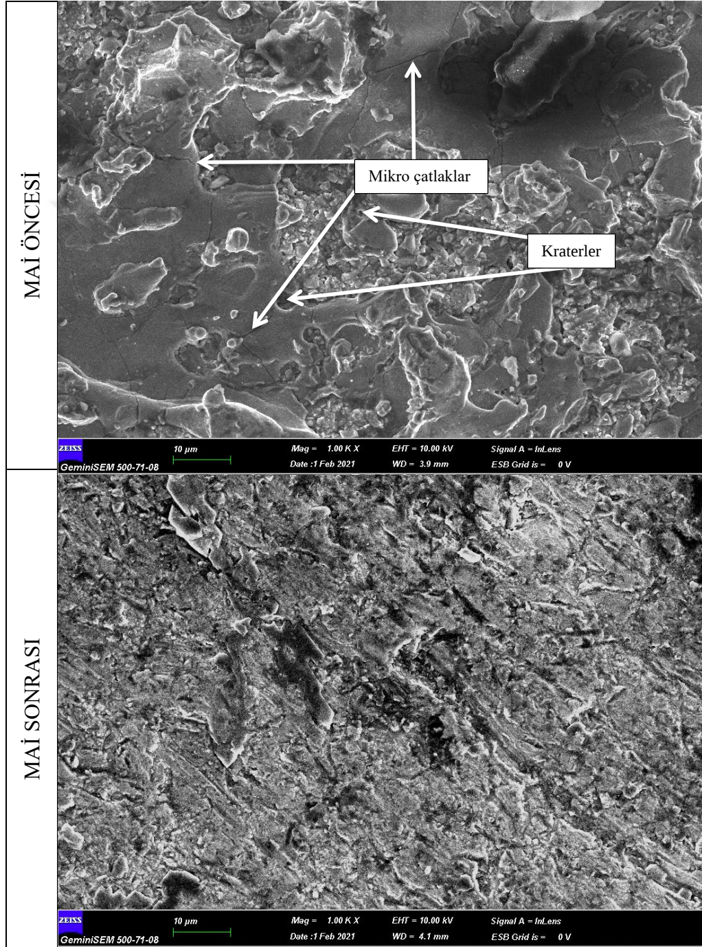
Resim 6.7. MAİ işleminin yüzey yapıları üzerindeki etkisi
