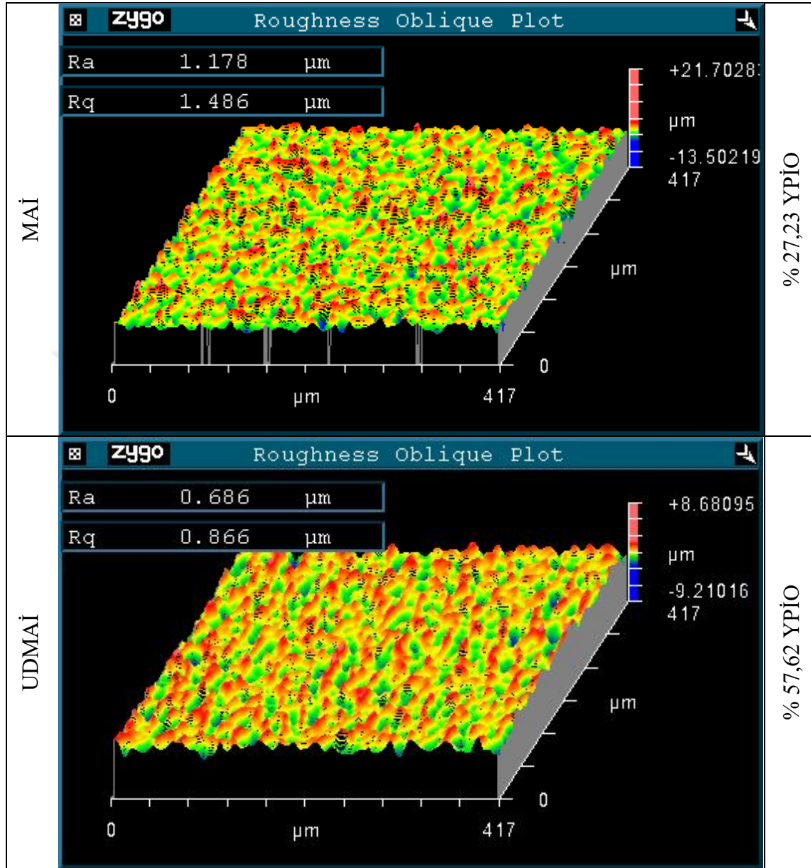
Resim 1.12. 12. deneylere ait numunelerin 3B yüzey topografyası
