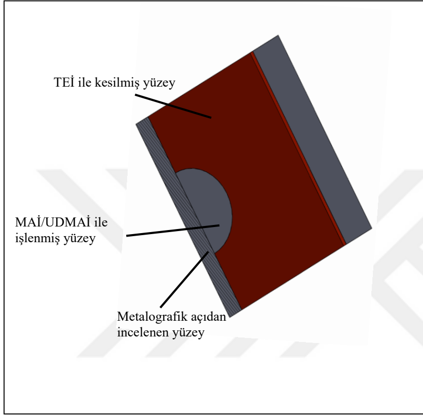
Şekil 5.13. Metalografik inceleme bölgeleri
