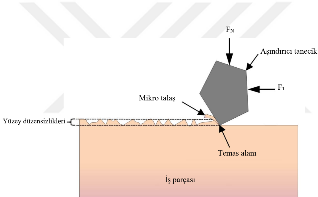
Şekil 3.4. MAİ yönteminde talaş kaldırma sırasında aşındırıcı taneciklere etki eden kuvvetler [35]
