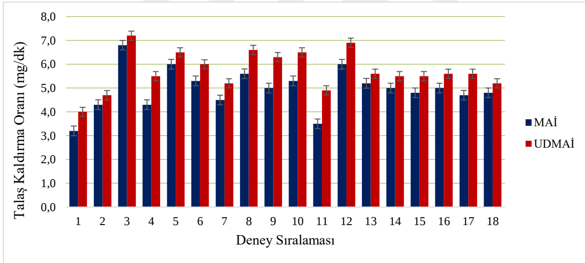
Şekil 6.1. MAİ/UDMAİ deneylerine ait TKO grafiği
