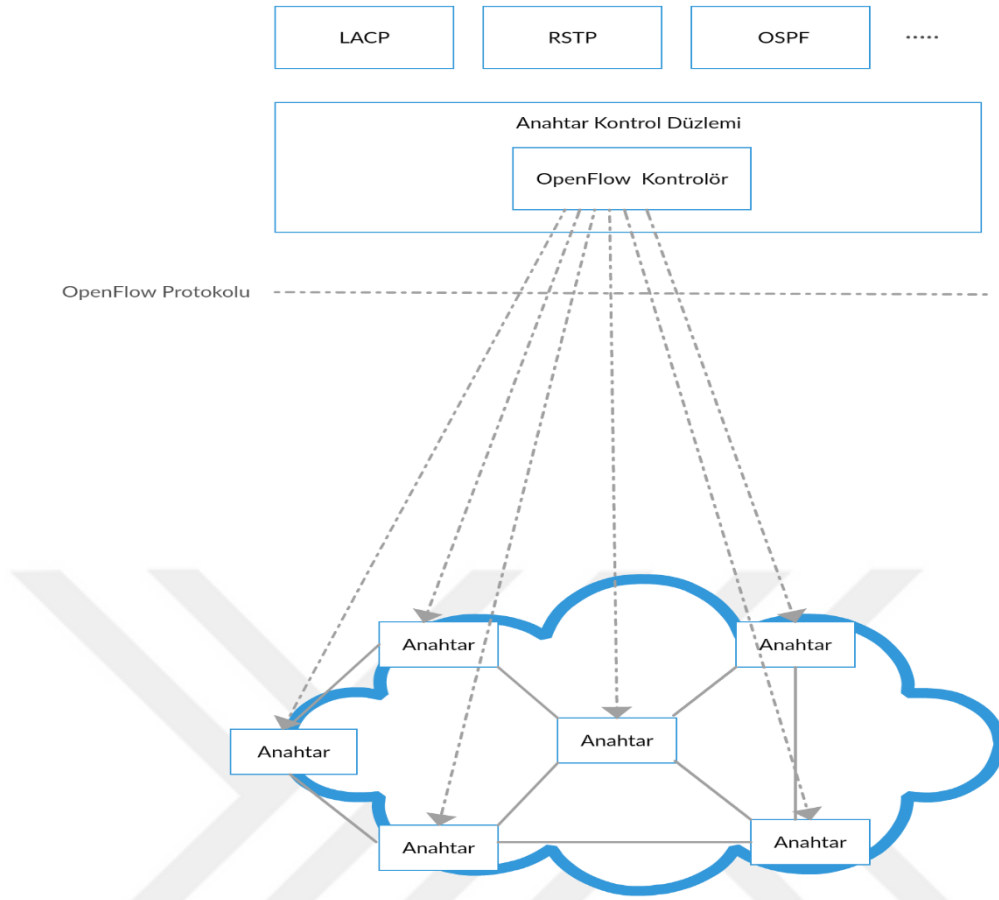
Şekil 7:OpenFlow mimarisi(Bazı kontrol düzlemi uygulamalarının,geleneksel kontrol düzlemi uygulamalarının davranışını taklit eden denetleyicinin ÜSTÜ üzerinde süreceği görüşünde)
