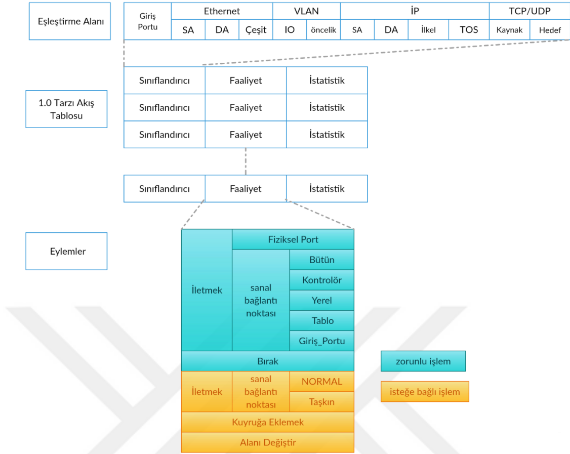
Şekil 9:OpenFlow(telli)sürüm 1.0 ilkeleri
