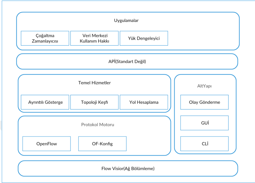
Şekil 8:OpenFlow denetleyici bileşenleri(FlowVisor ve uygulamaları ayrı varlıklardır)
