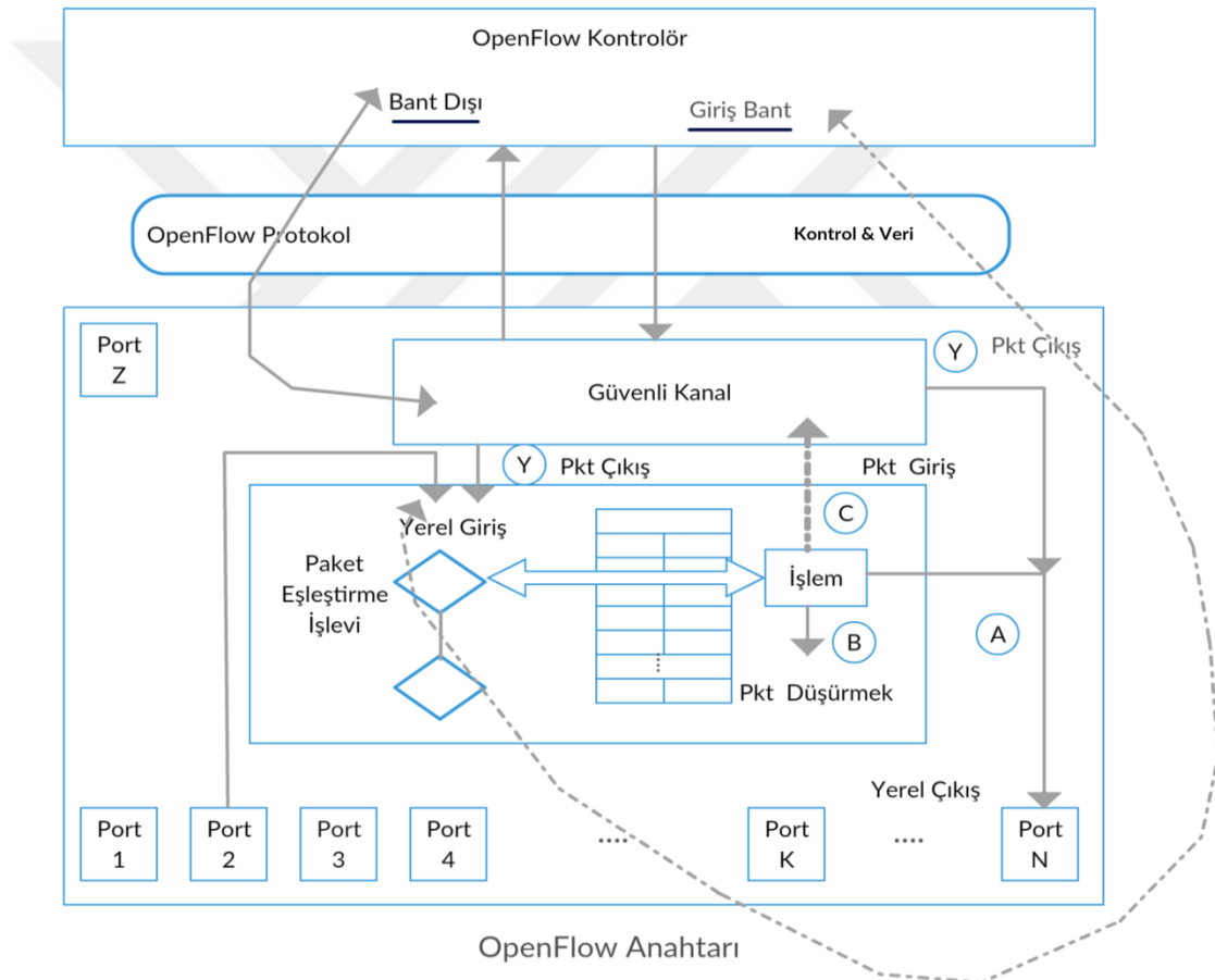
Şekil 11:OpenFlow Kontrolör-Anahtar Güvenli Kanal
