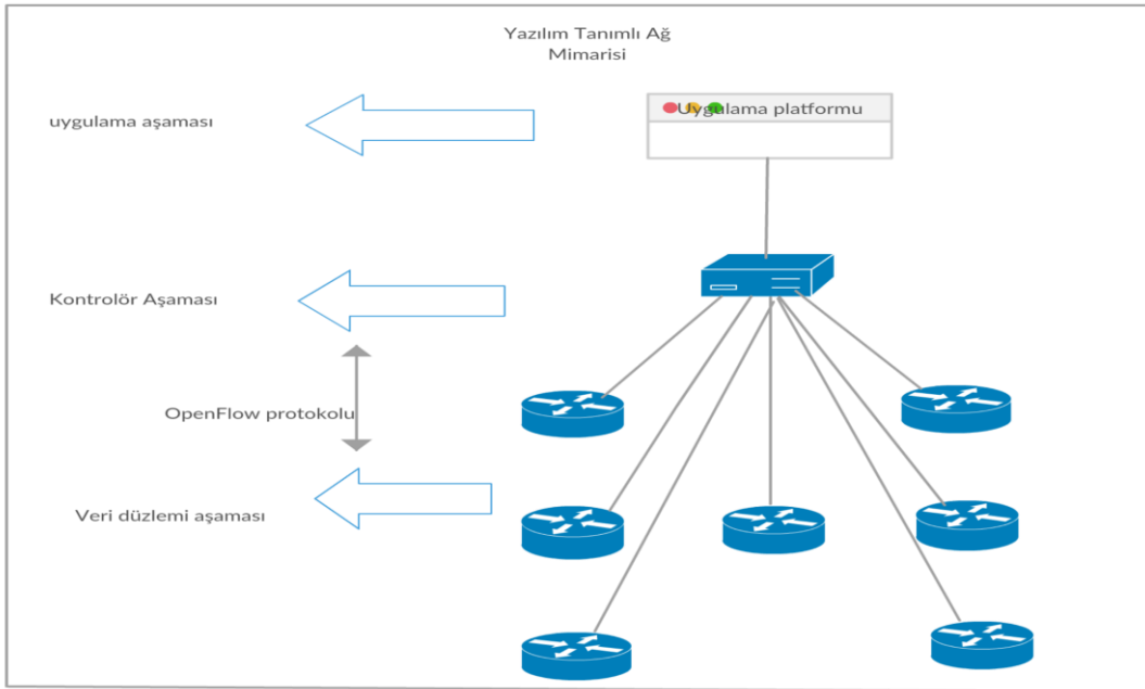
Şekil 1: SDN Mimarisi
