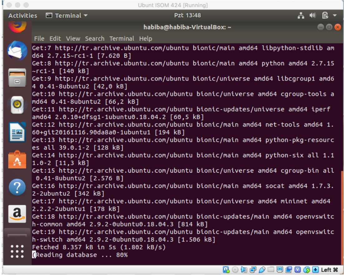
Şekil 45:Mininet kurulumuna devam etmek istedikten sonra
