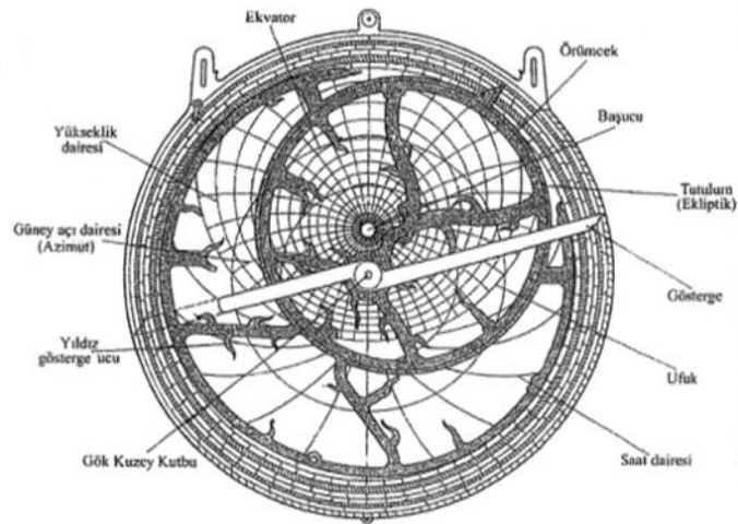
Fotoğraf 8:Usturlabın Ön Yüzü 251
