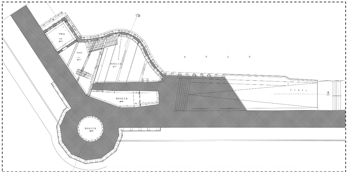
Şekil 3.183 Alay Köşkü asma kat plan şeması (İRAM)
