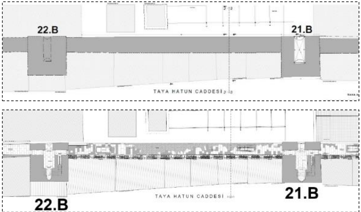
Şekil 3.225 21 nolu burç ile 22 nolu burç arasındaki kısmın alt ve üst kot rölöve plan şemaları (İRAM)
