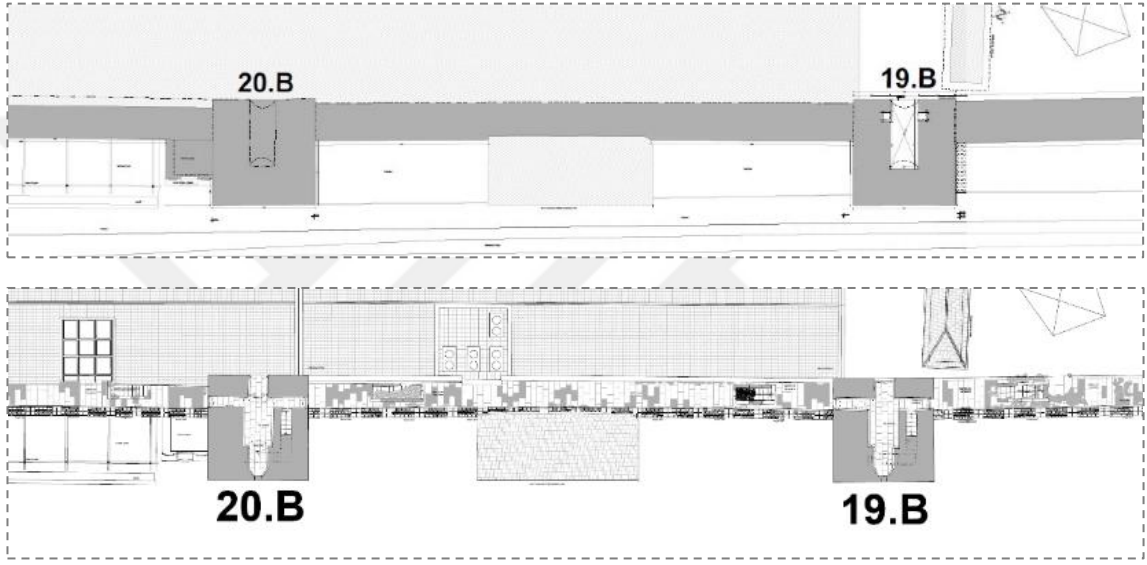
Şekil 3.205. 19 nolu burç ile 20 nolu burç arasındaki kısmın alt ve üst kot rölöve plan şemaları (İRAM).
