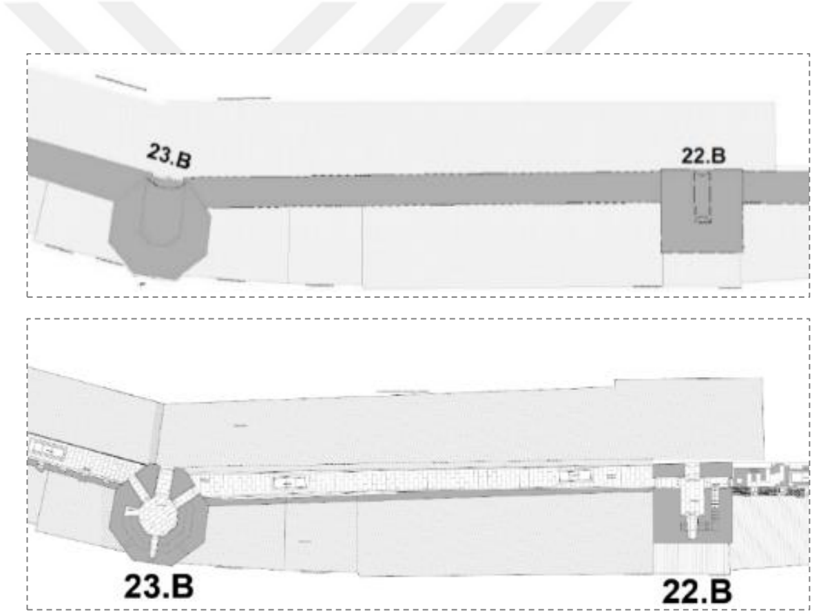
Şekil 3.233: 22 nolu burç ile 23 nolu burç arasındaki kısmın alt ve üst kot plan şemaları (İRAM)
