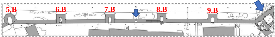
Şekil 3.59. 5 nolu sekizgen burç ile Bab-ı Hümayun arasındaki kısmın rölövesi, 2015 (İRAM).
