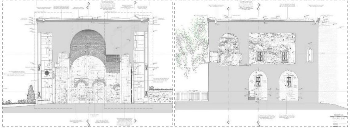
Şekil 3.88. Bab-ı Hümayun'a ilişkin enine kesitler 3-3 (soldaki) ve 5-5 kesitleri, 2015 (İRAM). 96
