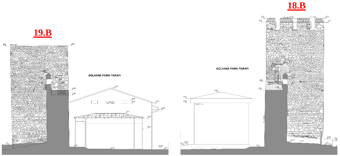
Şekil 3.199: 18 ve 19 nolu burçlar arası kısımda “4-4” (soldaki) ve “5-5” (sağdaki) kesitleri (İRAM).
