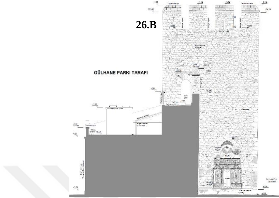
Şekil 3.272 26 nolu burç ile Demirkapı arasındaki “1-1” kesiti (İRAM) 154
