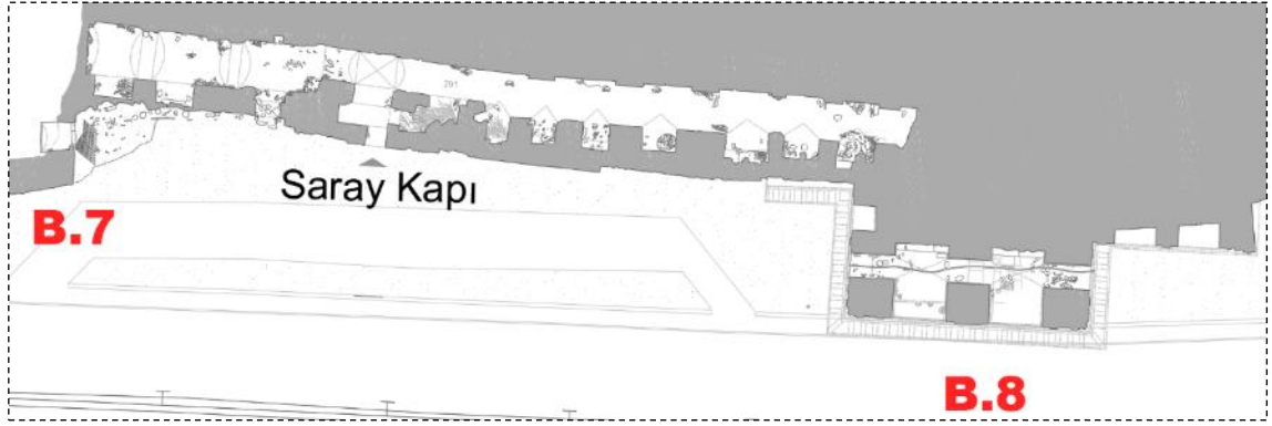
Şekil 3.407 B.7 ile B.8 arasına ilişkin ara kesit röleve plan şeması (İRAM; Soyal)
