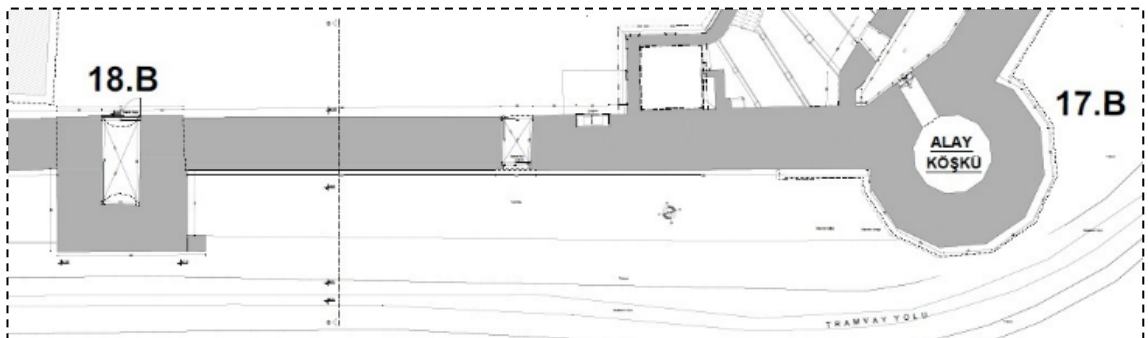
Şekil 3.188. 17 nolu burç (Alay Köşkü) ile 18 nolu burç arası rölöve çizimi (İRAM).
