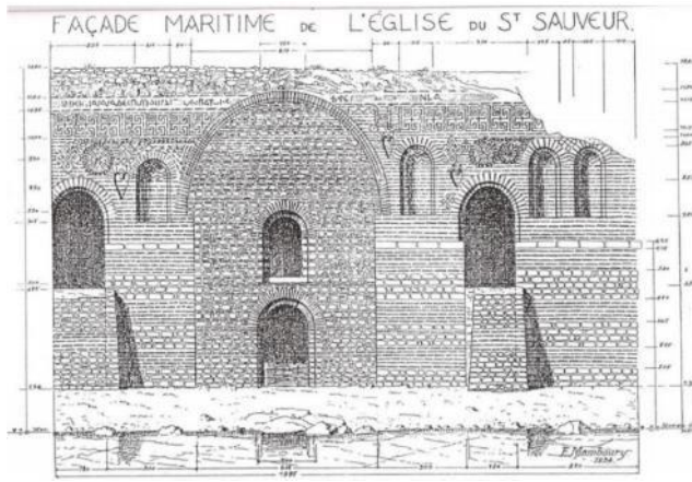
Şekil 3.376 B.9 bitişiğindeki Bizans yapı kalıntısına ilişkin cephe ve plan şeması (Demangel-Mamboury)
