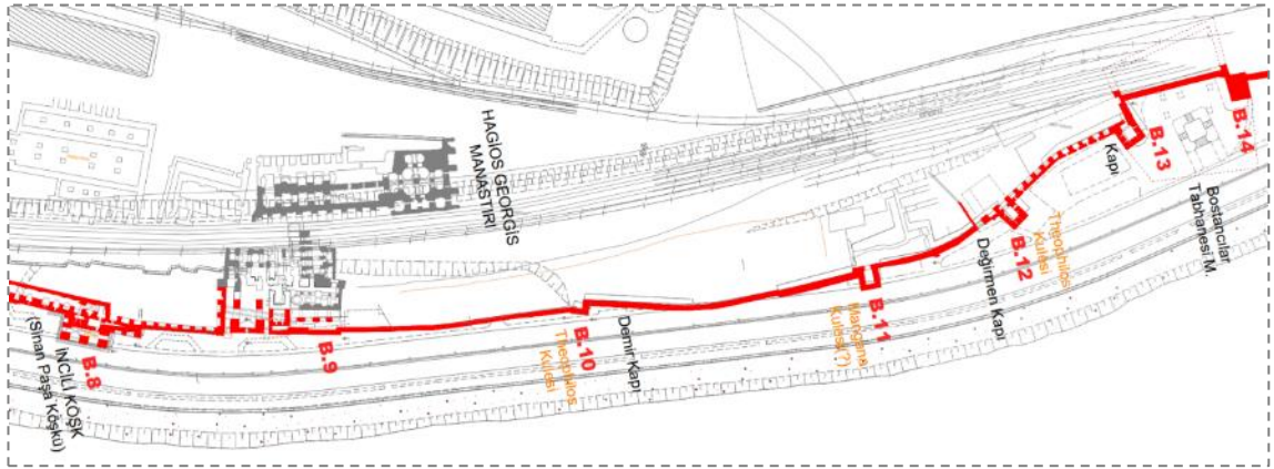
Şekil 3.331 B.14 burcu ile İncili Köşk (B.8) arasındaki bölümün vaziyet planı (İRAM) 198
