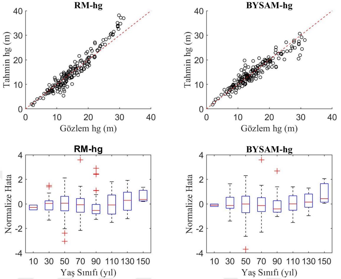
Şekil 3.16 Meşcere orta boyu modellerinin hata dağılımları ve gözlemlere karşı tahmin grafikleri
