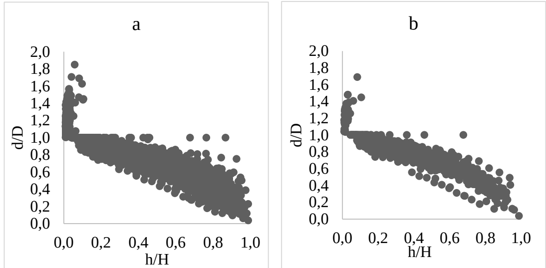
Şekil 2.5 Modellerin oluşturulmasında (a) ve uygunluğunun test edilmesinde (b) kullanılan verilerin oransal çap değerlerinin oransal boy değerlerine göre dağılımı
