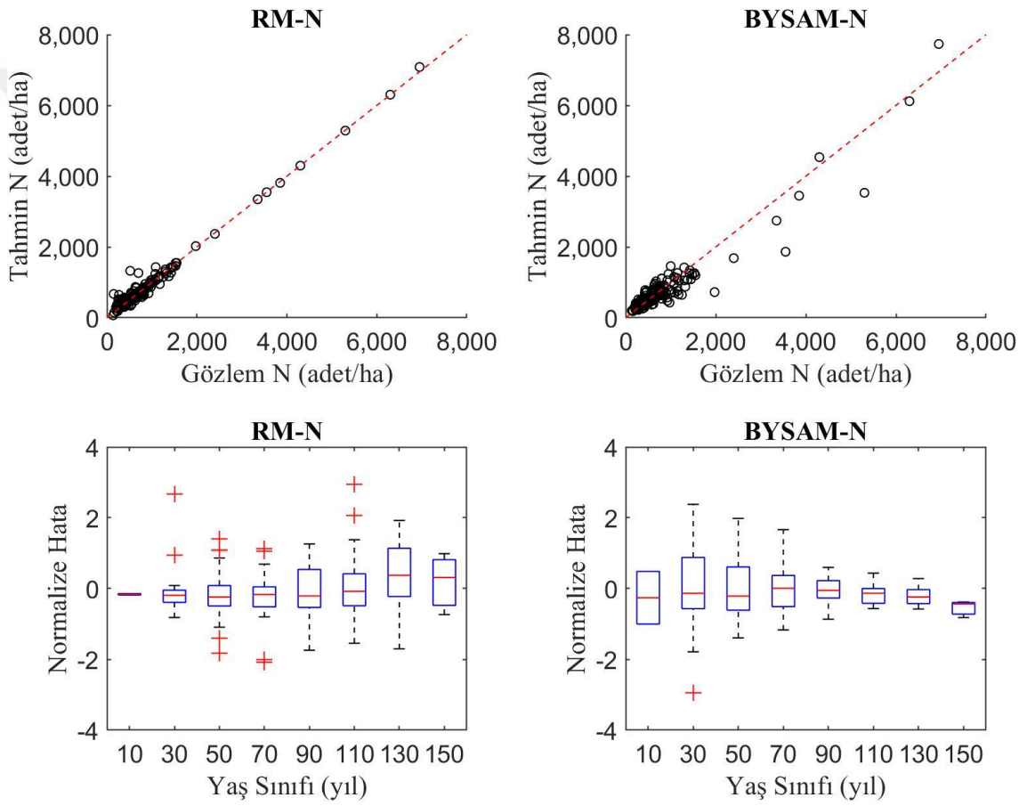
Şekil 3.17 Meşcere ağaç sayısı modellerinin hata dağılımları ve gözlemlere karşı tahmin grafikleri
