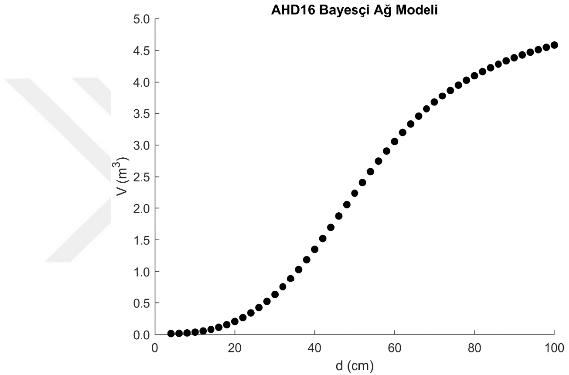
Şekil 3.3 Göğüs yüksekliği çapını esas alan BYSAM'nin simülasyon veri setindeki davranışı
