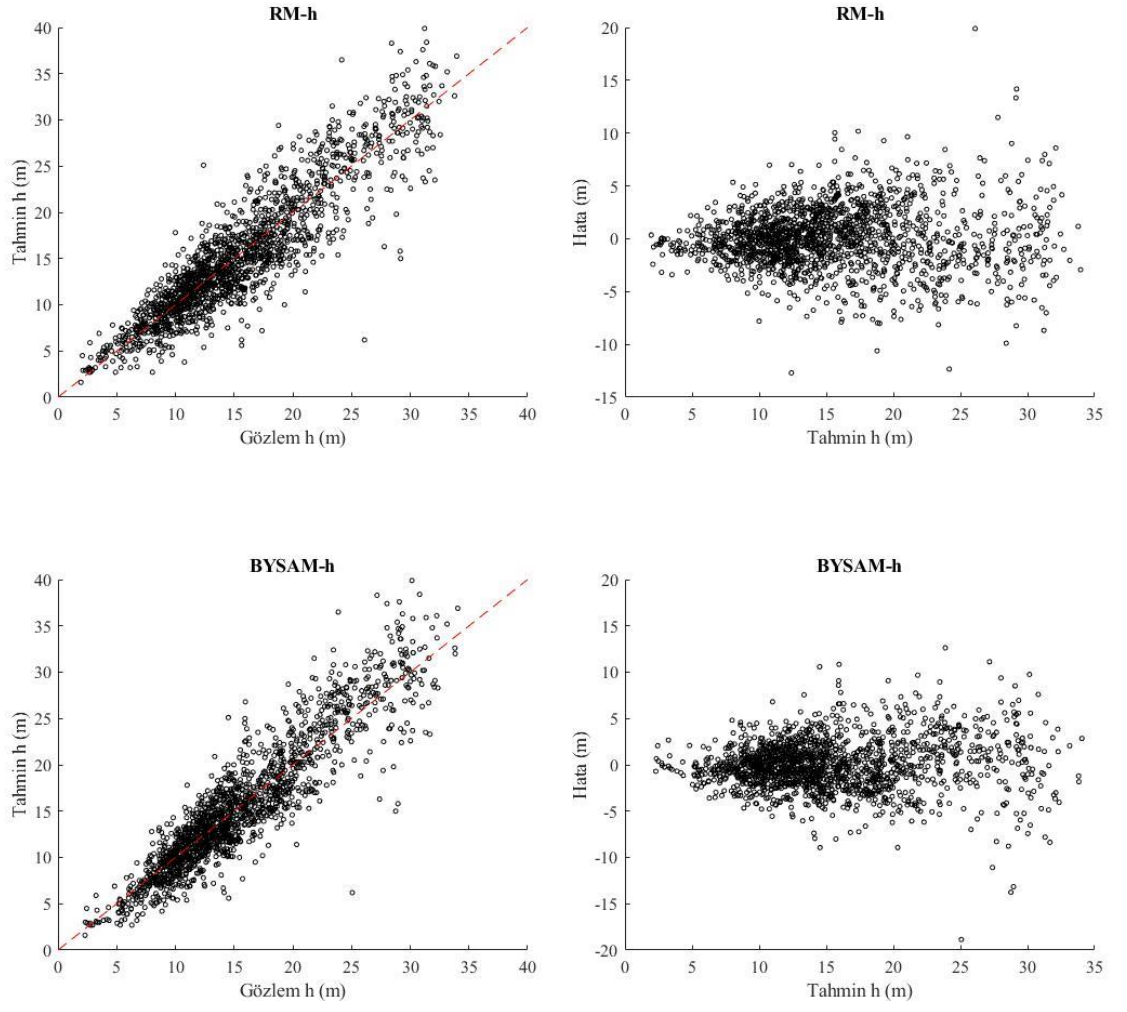
Şekil 3.9 Genelleştirilmiş çap-boy modellerine ilişkin hata dağılımları ve gözlem-tahmin grafikleri
