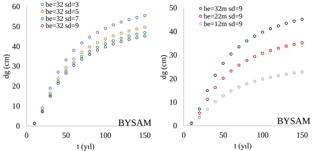
Şekil 3.25 Meşcere orta çapının (cm) iyi bonitet sınıfında ( be=32m ) yaş ve sıklık derecelerine (sol) ve sıklık derecesi=9 (Normal Sıklık) olan meşcerelerde yaş ve bonitet sınıfına göre (sağ) değişimi
