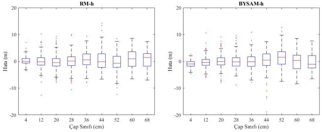
Şekil 3.10 Genelleştirilmiş çap-boy modellerinin çap sınıflarına göre hata dağılımları
