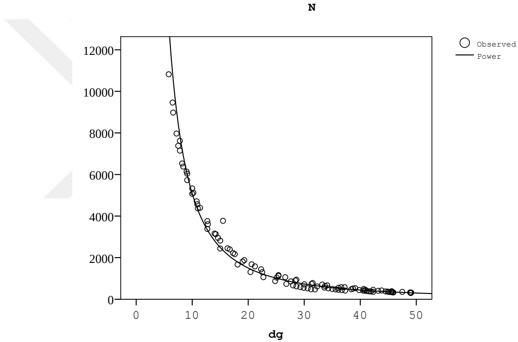
Şekil 3.12 Kalıpsız (1963)’den elde edilen meşcere orta çapının meşcere ağaç sayısı ile ilişkisi
