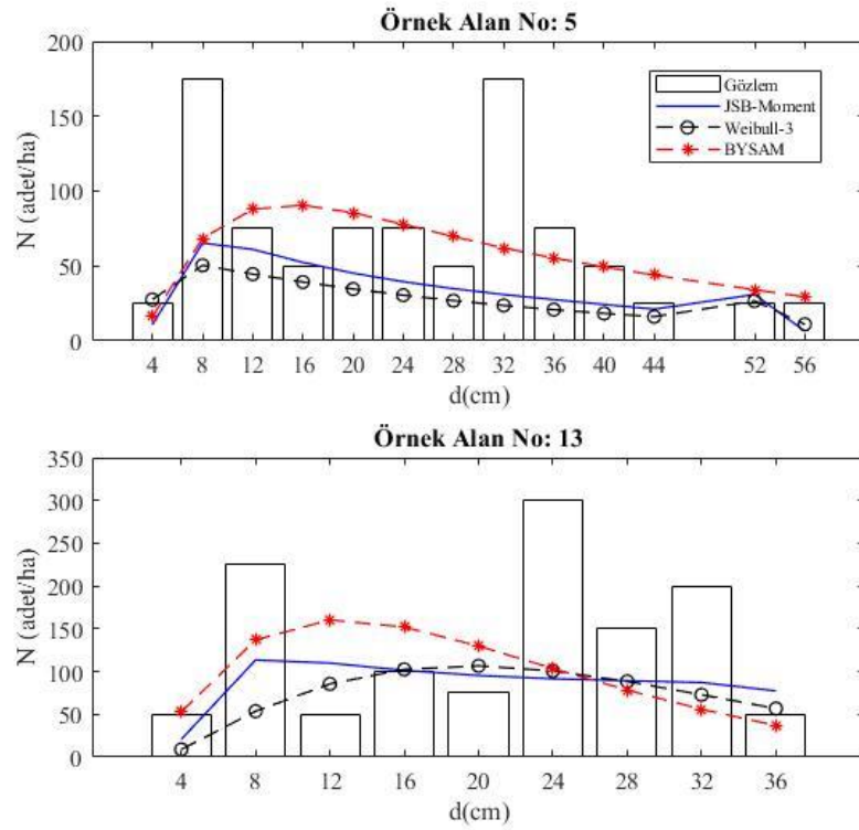
Şekil 3.35 Standart sapması yüksek olan iki örnek alanda çap dağılım modellerinin davranışı
