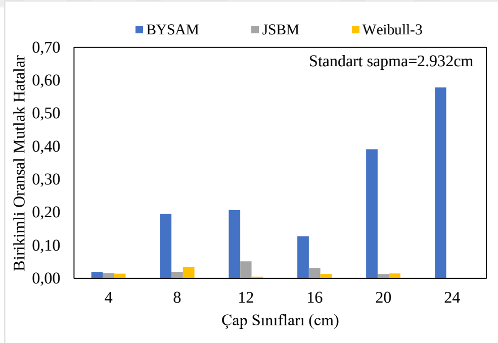
Şekil 3.32 132 numaralı örnek alanda çap dağılım modellerinin birikimli oransal mutlak hataları
