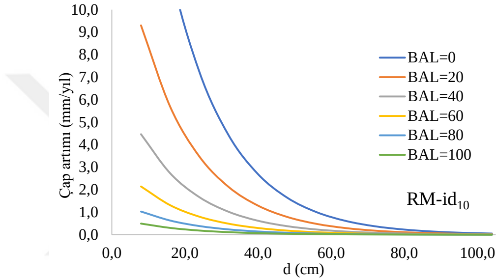
Şekil 3.42 RM ile elde edilen tek ağaç çap artımlarının BAL değişkenine göre değişimi (Meşcere özellikleri be=32 m, dg=30 cm, sd=9 ve G=30 m 2 /ha)
