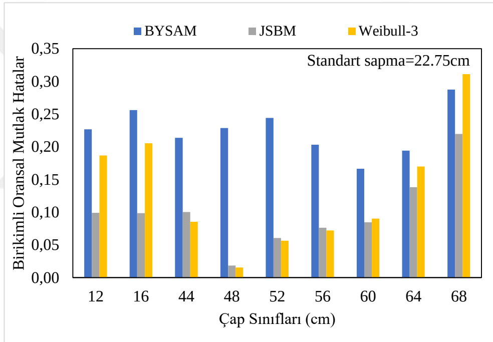
Şekil 3.30 66 numaralı örnek alanda çap dağılım modellerinin birikimli oransal mutlak hataları
