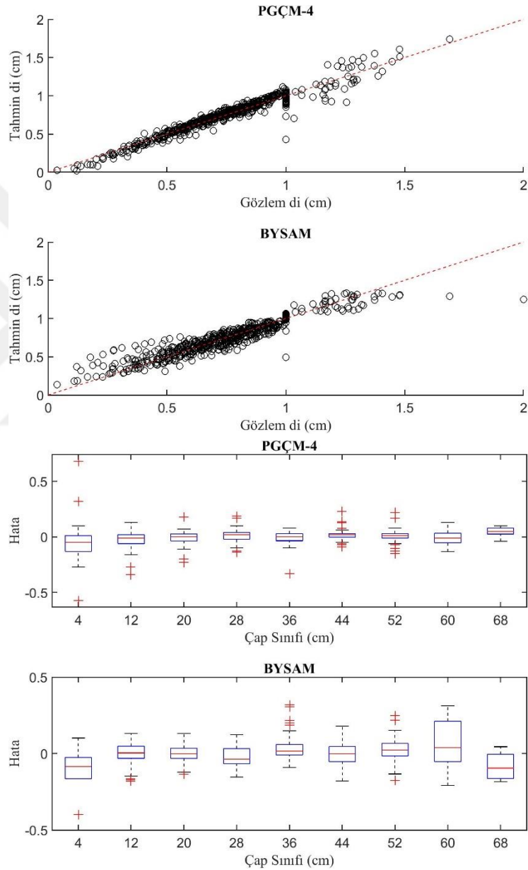
Şekil 3.1 PGÇM-4 ve BYSAM'nin hata dağılımları ve tahmin-gözlem grafikleri
