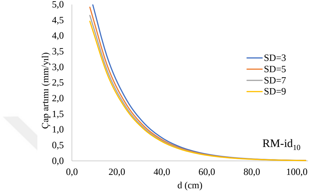
Şekil 3.40 RM ile elde edilen tek ağaç çap artışlarının sıklığa göre değişimi (Meşcere özellikleri be=32m , dg=30\text{ cm} , BAL=40\text{ m}^2 ve G=30\text{ m}^2/ha )
