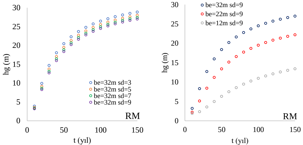
Şekil 3.21 Meşcere orta boyunun (m) iyi bonitet sınıfında ( be=32m ) yaş ve sıklık derecelerine (sol) ve sıklık derecesi=9 (Normal Sıklık) olan meşcerelerde yaş ve bonitet sınıfına göre (sağ) değişimi
