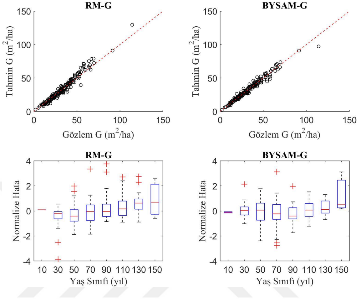
Şekil 3.18 Meşcere göğüs yüzeyi modellerinin hata dağılımları ve gözlemlere karşı tahmin grafikleri
