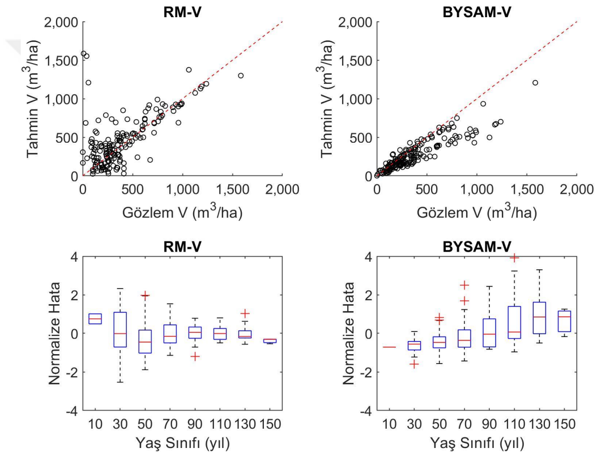
Şekil 3.19 Meşcere hacim modellerinin hata dağılımları ve gözlemlere karşı tahmin grafikleri
