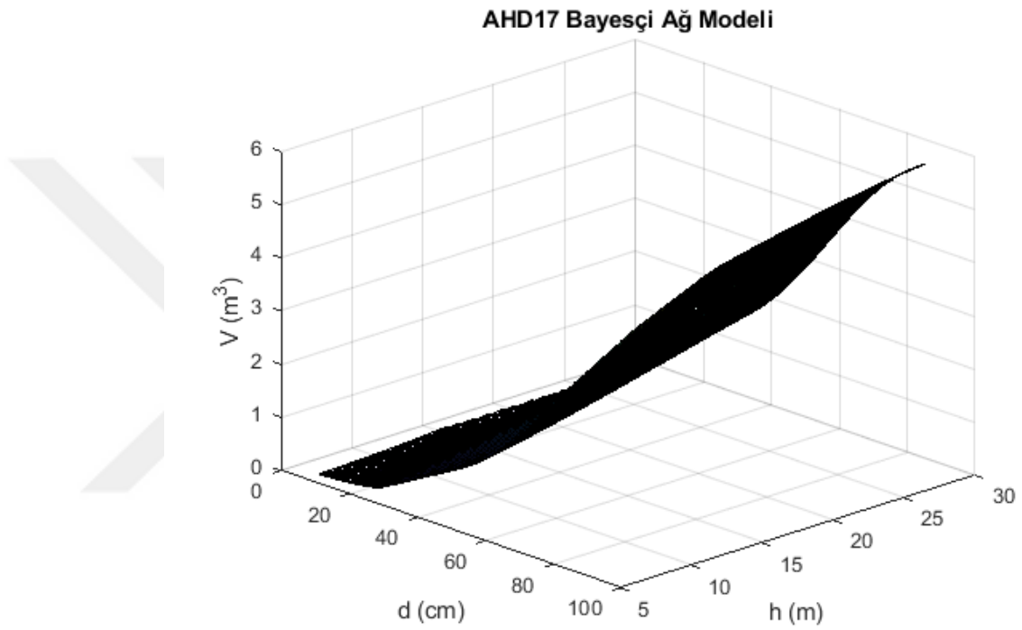
Şekil 3.4 Göğüs yüksekliği çapını ve toplam ağaç boyunu esas alan BYSAM'nin simülasyon veri setindeki davranışı
