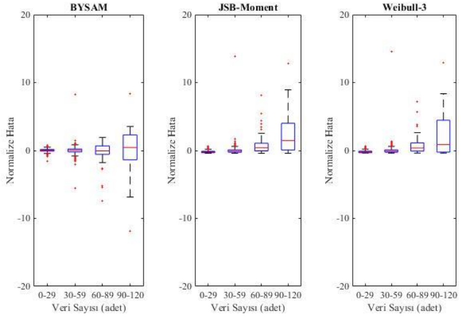
Şekil 3.34 Çap dağılım modellerinin veri sayısına göre hata dağılımları
