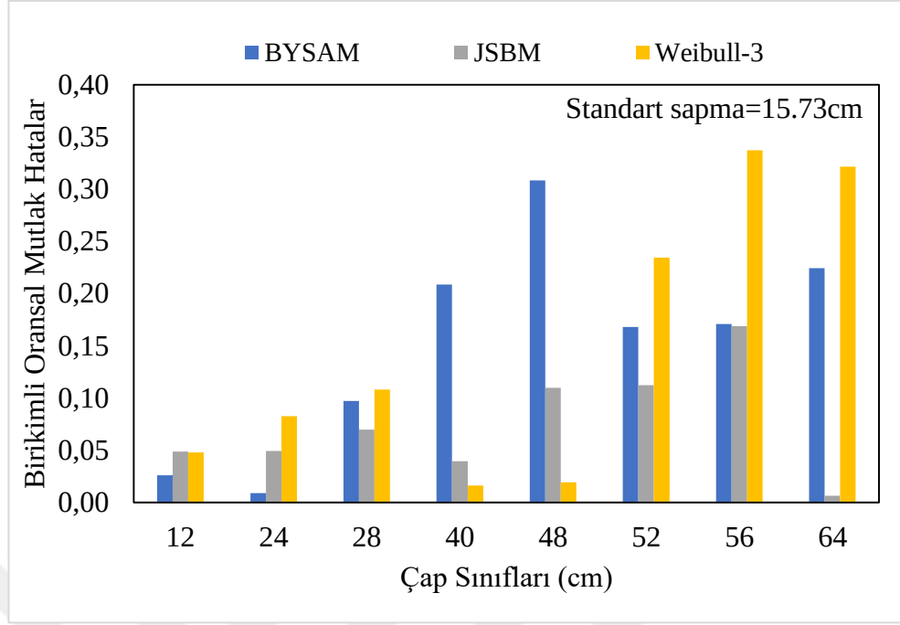
Şekil 3.31 8 numaralı örnek alanda çap dağılım modellerinin birikimli oransal mutlak hataları
