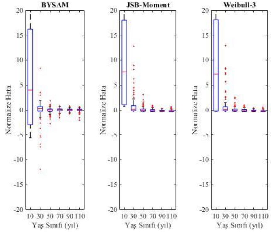
Şekil 3.33 Çap dağılım modellerinin yaş sınıflarına göre hata dağılımları
