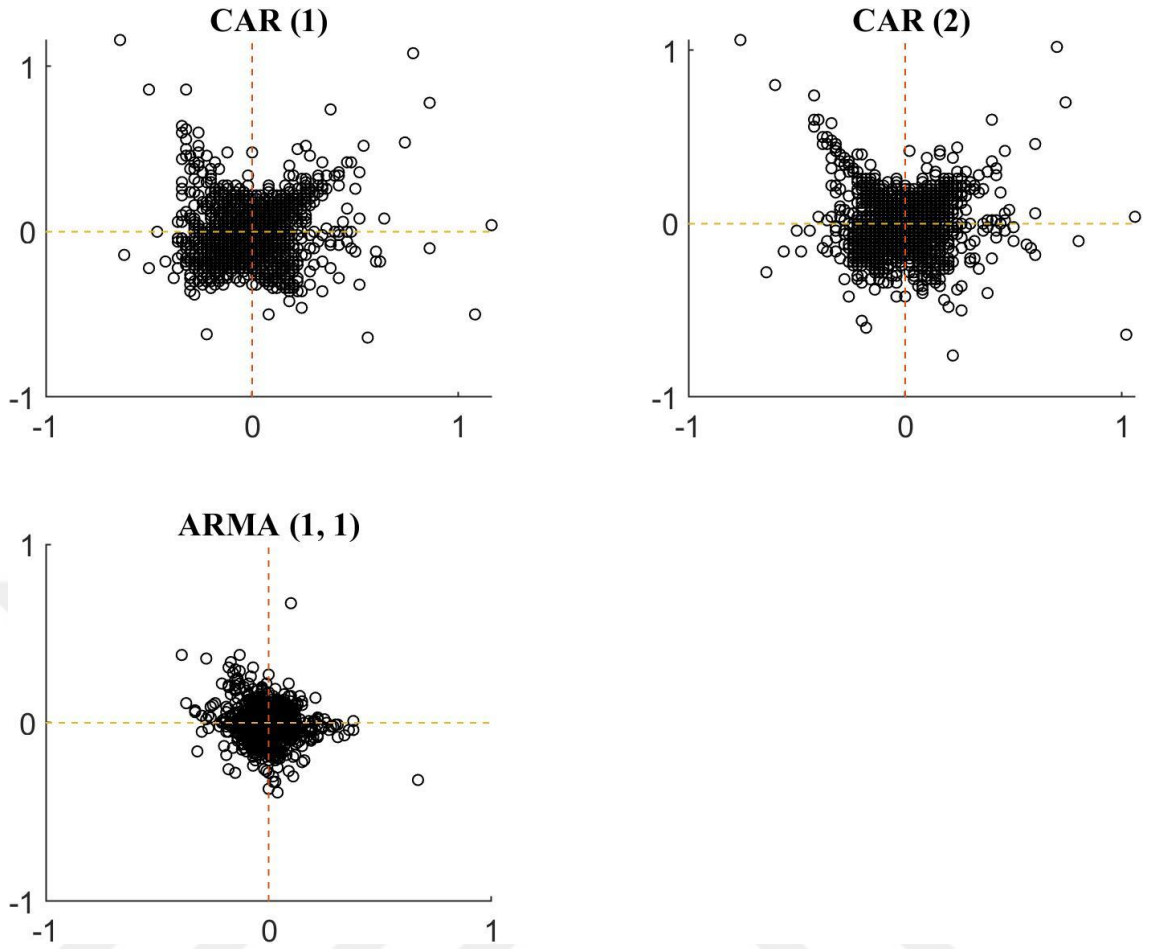
Şekil 3.2 Parçalı gövde çapı modellerinin gecikmeli hata dağılımları
