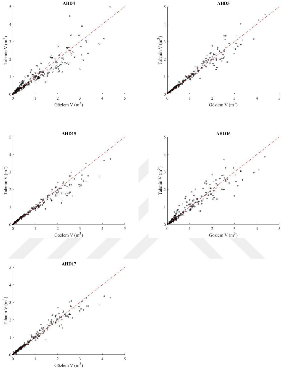
Şekil 3.5 Ağaç hacim modellerinin gözlemlere karşı tahminlerin dağılımları
