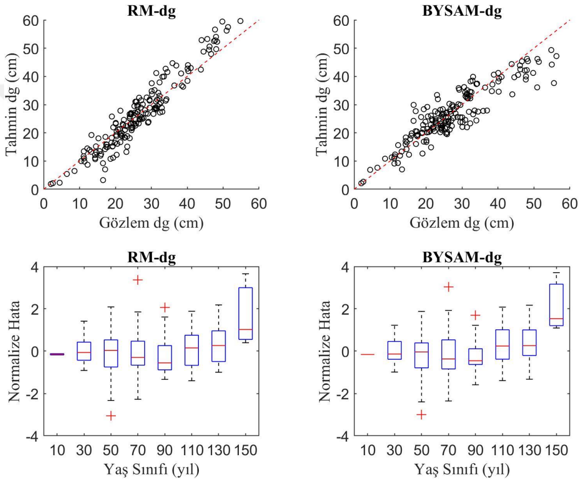
Şekil 3.15 Meşcere orta çapı modellerinin hata dağılımları ve gözlemlere karşı tahmin grafikleri
