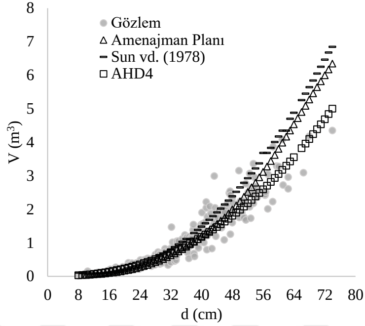
Şekil 3.7 Çalışma kapsamında geliştirilen tek girişli ağaç hacim modelinin amenajman planı ve Sun vd. (1978) ile karşılaştırılması
