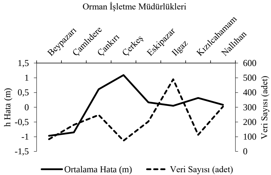
Şekil 3.11 Genelleştirilmiş çap-boy modellerinin orman işletme müdürlüklerine göre hata dağılımları
