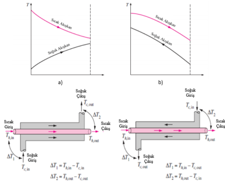
Şekil 4.1. a) Paralel akışlı ısı değiştirici, b) Ters akışlı ısı değiştirici (Incropera, F.P., vd., 2007).
