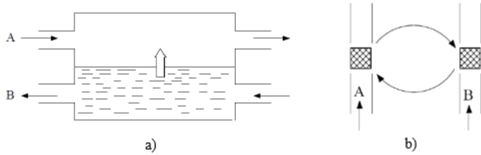
Şekil 3.2. a) Reküperatör ısı değiştiricisi, b) Rejeneratör ısı değiştiricisi (Bott vd., 1994).
