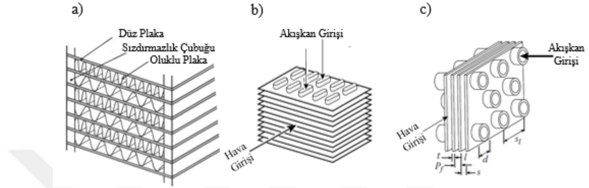
Şekil 3.11. Genişletilmiş yüzeyli ısı değıştircileri: a) plakalı kanatlı, b) lamelli boru kanatlı, c) yuvarlak boru kanatlı (Kakaç vd., 2012).
