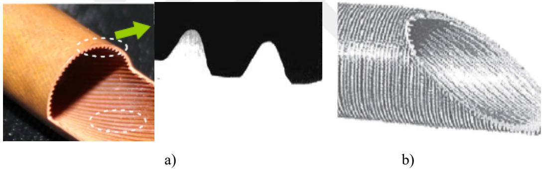
Şekil 3.15. Daha önce yayınlanmış çalışmalarda kullanılan mikro kanatlı borular: a) (Eiamsa-Ard ve Wongcharee, 2012), b) (Nagarajan vd., 2010).
