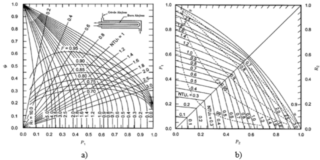
Şekil 4.2. 1-2 TEMA E tipi gövde borulu ısı değiştiricide, a) \psi değişimi (Roetzel ve Spang,1983), b) P_1 - P_2 değişimi (Roetzel ve Spang,1993).
