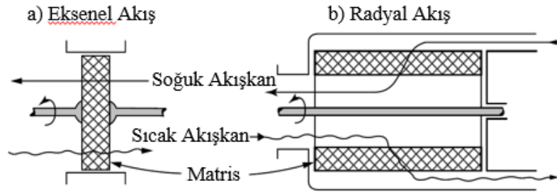
Şekil 3.3. Döner rejeneratörler: a) disk tipi, b) tambur tipi (Kakaç vd., 1987).
