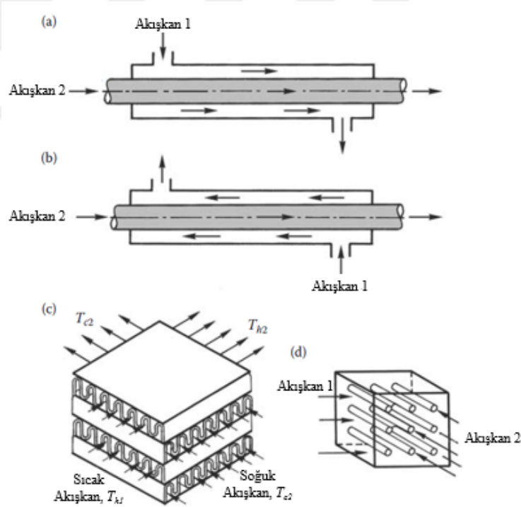
Şekil 3.13. Akış düzenlemesine göre ısı değiştiricilerinin sınıflandırılması: a) paralel akış, b) ters akış, c) her iki sıvı karıştırılmadan çapraz akış, d) çapraz akış, akışkan 1 karışık, akışkan 2 karıştırılmamış (Kakaç vd., 2012).
