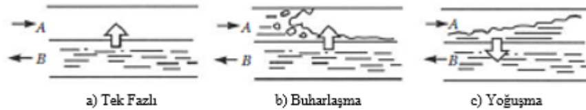
Şekil 3.12. Isı transfer mekanizmalarına göre ısı değıştirciler: a) tek fazlı taşınım b) buharlaşma çift fazlı taşınım c) yoğuşma çift fazlı taşınım (Bott vd., 1994).
