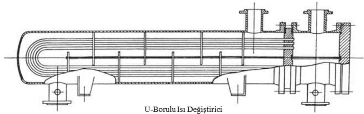
Şekil 3.8. U borulu, bölmeli tek geçişli gövde borulu ısı değıştircisi (TEMA Inc., 2007).
