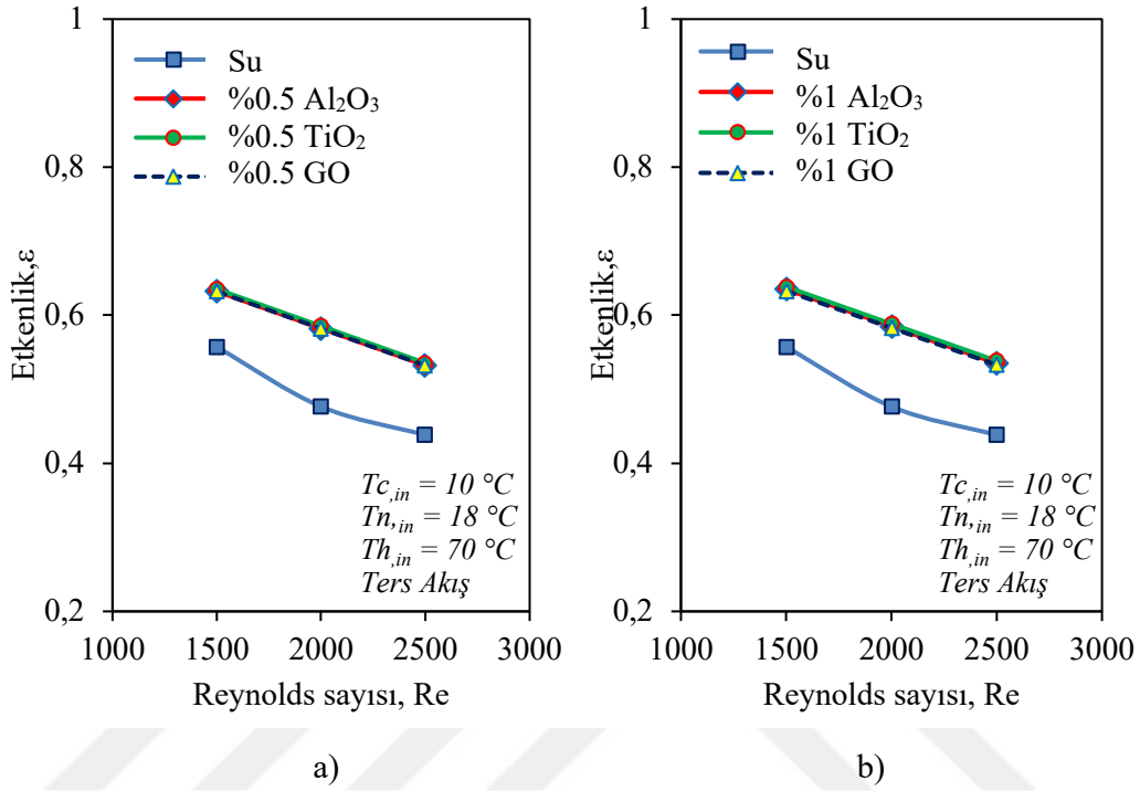
Şekil 7.4. Üç borulu ısı değıştircisi etkenliđi, a) %0,5 Al_2O_3 -su, %0,5 TiO_2 -su ve %0,5 GO-su nanoakışkanları, b) %1 Al_2O_3 -su, %1 TiO_2 -su ve %1 GO-su nanoakışkanları.
