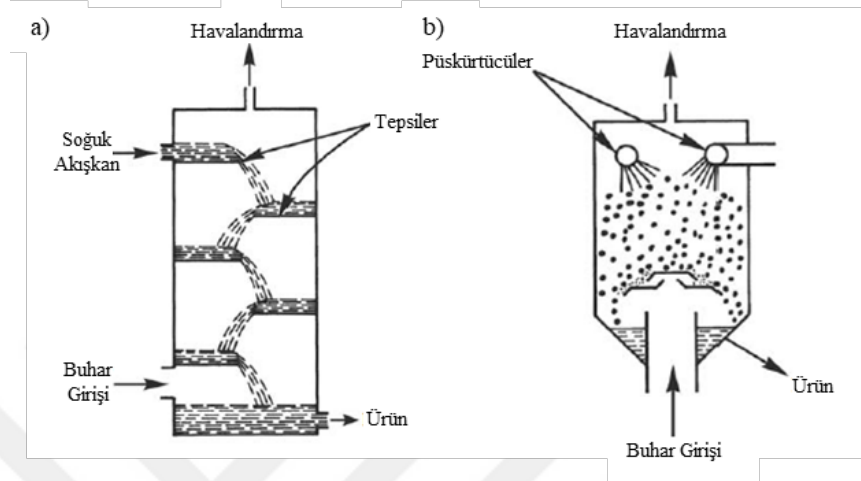
Şekil 3.4. Doğrudan temaslı ısı değıştircileri: a) tepsili kondenser, b) sprey yoğunlaştırıcı (Kakaç, 1992).
