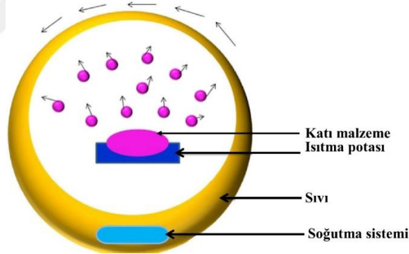
Şekil 5.2. Buharlaştırma yöntemi ile nanoakışkanın hazırlanması (Dağdevir, 2020).
