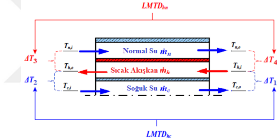
Şekil 6.9. Ortalama logaritmik sıcaklık farkı yöntemi ( LMTD_{ort} ).
