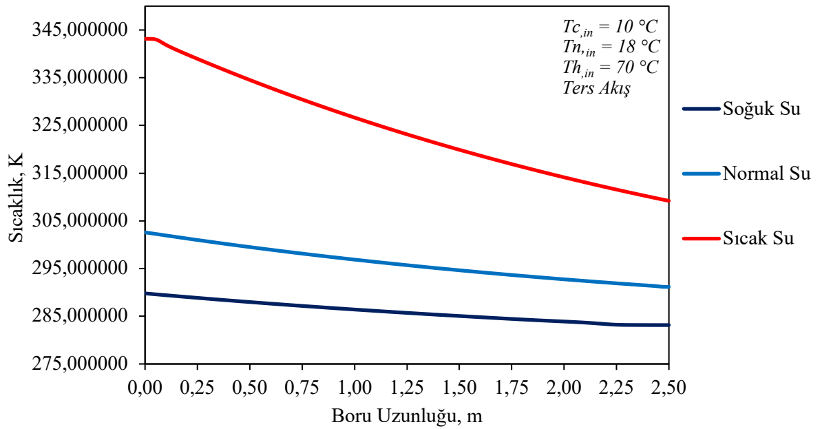
Şekil 6.8. Isı değıştircisinin boru uzunluğu boyunca merkezindeki sıcaklık dağılımları.
