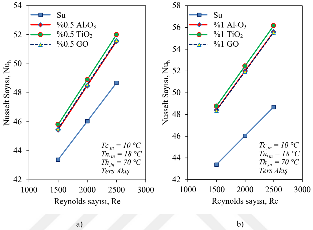
Şekil 7.1. Farklı Re sayılarında Nu sayısının değişimi, a) \%0,5 Al_2O_3 -su, \%0,5 TiO_2 -su ve \%0,5 GO-su nanoakışkanları, b) \%1 Al_2O_3 -su, \%1 TiO_2 -su ve \%1 GO-su nanoakışkanları.
