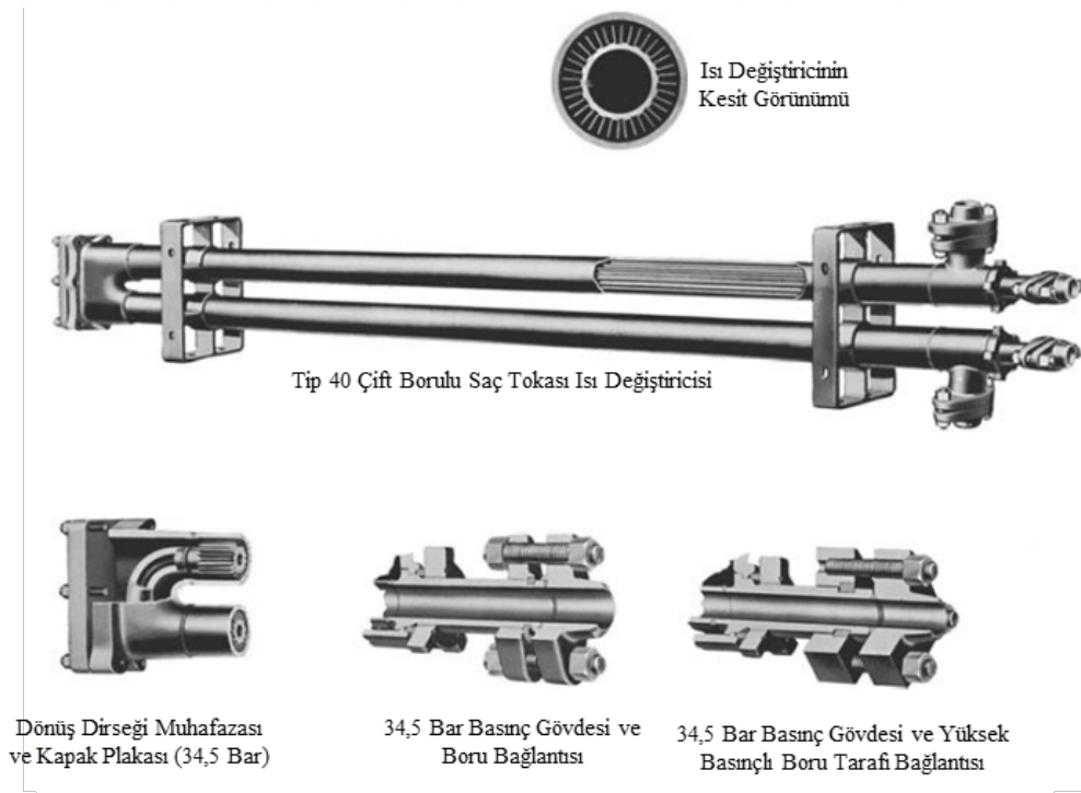
Şekil 3.6. Enine kesit görünümüne ve dönüş dirsek muhafazasına sahip çift borulu U tipi ısı değıştircisi (Kakaç vd., 1987).
