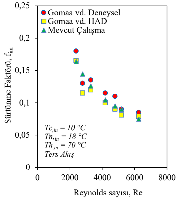
Şekil 6.6. Reynolds sayısı ve sürtünme faktörü değerleri için karşılaştırma.
