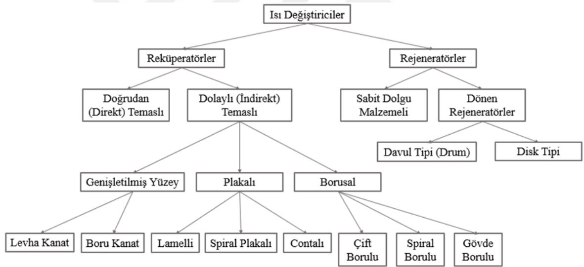
Şekil 3.1. Isı değıştircilerinin sınıflandırılması (Kakaç vd., 2012).
