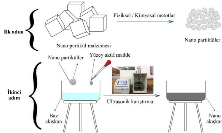
Şekil 5.3. İki adım yöntemi ile nanoakışkanın hazırlanması (Dağdevir, 2020).
