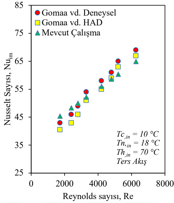
Şekil 6.5. Reynolds ve Nusselt sayıları için karşılaştırma.
