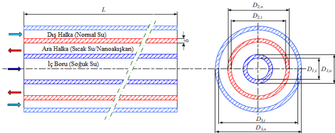
Şekil 6.1. Eş merkezli üç borulu ısı değiştiricisinin şematik akış diyagramı.
