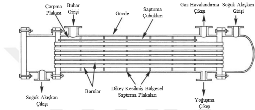
Şekil 3.7. Gövde borulu ısı değıştircisi (Kakaç vd., 1987).
