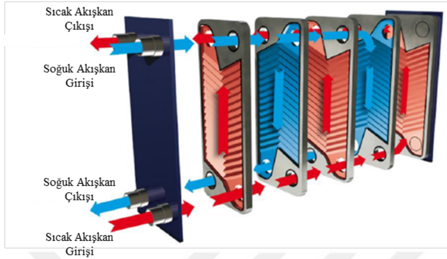
Şekil 3.10. Plakalı ısı değiştiricisi (“Kimya Teknolojisi |Megep”, 2021).
