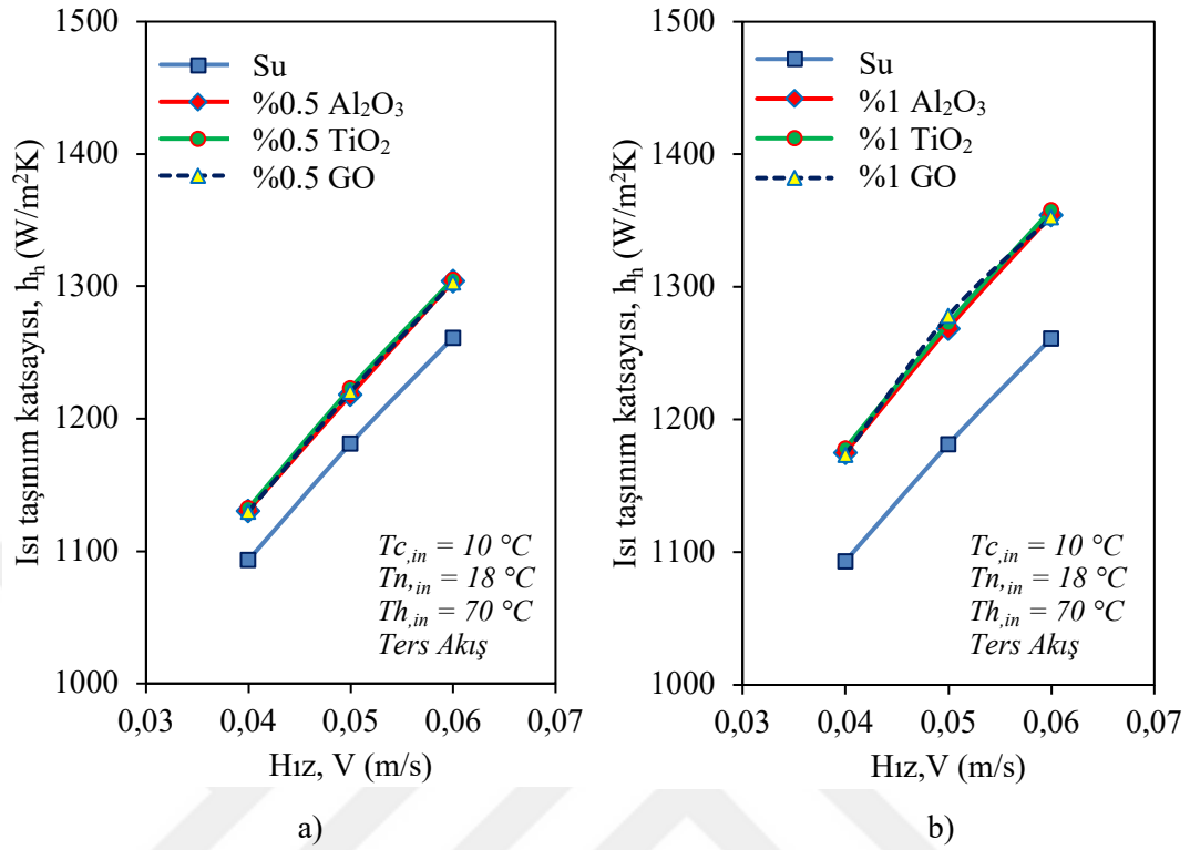
Şekil 7.3. Sıcak akışkanın 0,04, 0,05 ve 0,06 m/s giriş hızları için ısı taşınım katsayısının değişimi, a) %0,5 Al_2O_3 -su, %0,5 TiO_2 -su ve %0,5 GO-su nanoakışkanları, b) %1 Al_2O_3 -su, %1 TiO_2 -su ve %1 GO-su nanoakışkanları.
