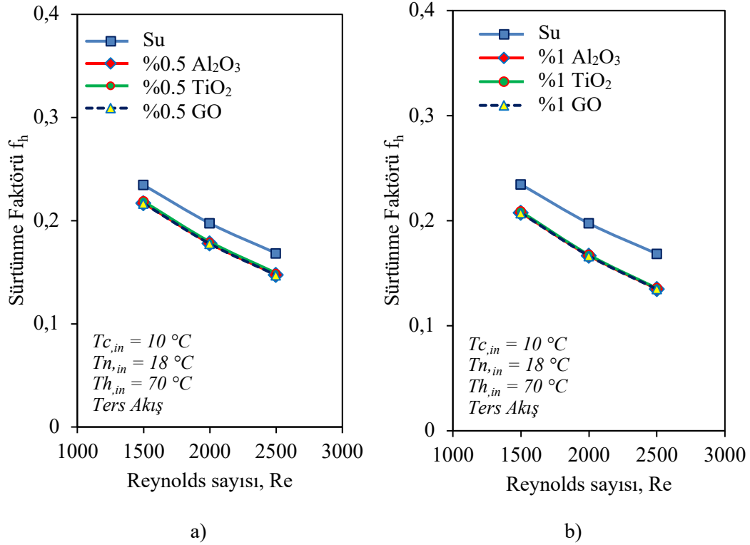
Şekil 7.2. Farklı Re sayılarında sürtünme faktörünün değişimi, a) %0,5 Al_2O_3 -su, %0,5 TiO_2 -su ve %0,5 GO-su nanoakışkanları, b) %1 Al_2O_3 -su, %1 TiO_2 -su ve %1 GO-su nanoakışkanları.
