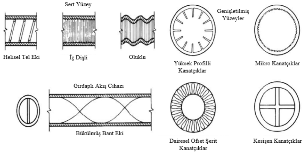
Şekil 3.14. Boru içi iyileştirme yöntemleri örnekleri (Kakaç, 1992).
