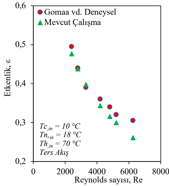
Şekil 6.7. Reynolds sayısı ve ısı değıştircisi etkenlik değeri için karşılaştırma.
