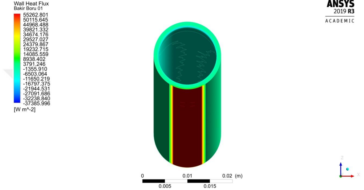
Şekil 4.36. 0.0017 kg/s debi için odak borusu ısı dağılımı
