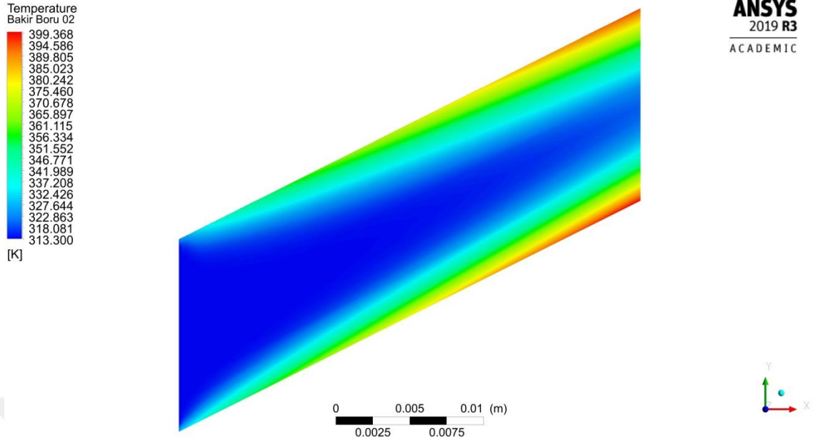
Şekil 4.47. 0.0033 kg/s debide boru merkez çizgisi boyunca kesitinin sıcaklığı dağılımı
