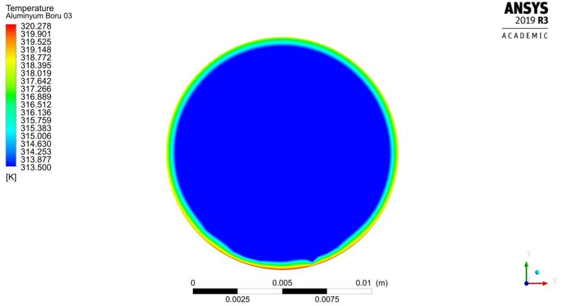
Şekil 4.87. 0.005 kg/s debide akışkan giriş sıcaklığı dağılımı
