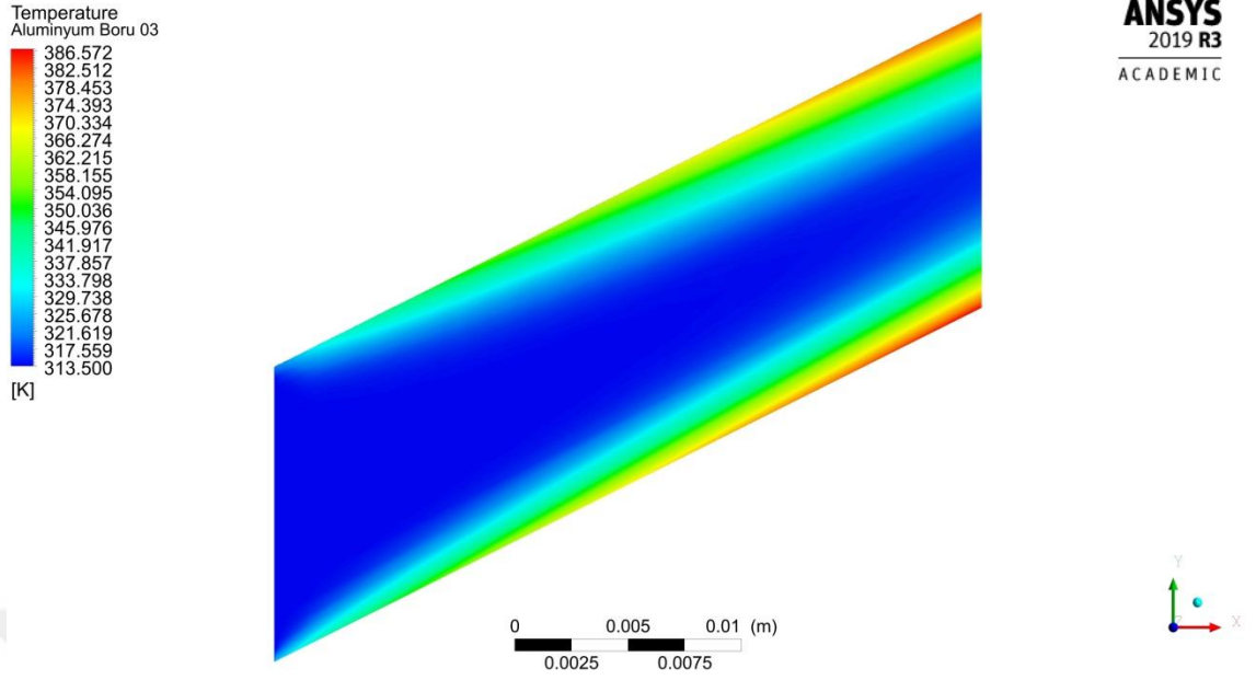
Şekil 4.89. 0.0050 kg/s debide boru merkez çizgisi boyunca kesitinin sıcaklığı dağılımı
