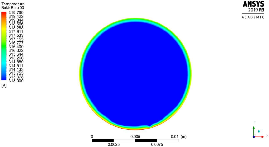
Şekil 4.52. 0.0050 kg/s debide akışkan giriş sıcaklığı dağılımı
