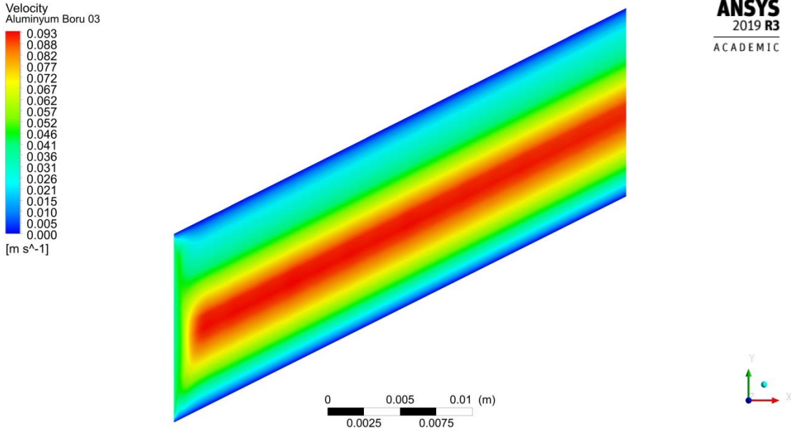
Şekil 4.90. 0.0050 kg/s debide boru merkez çizgisi boyunca kesitin hız dağılımı
