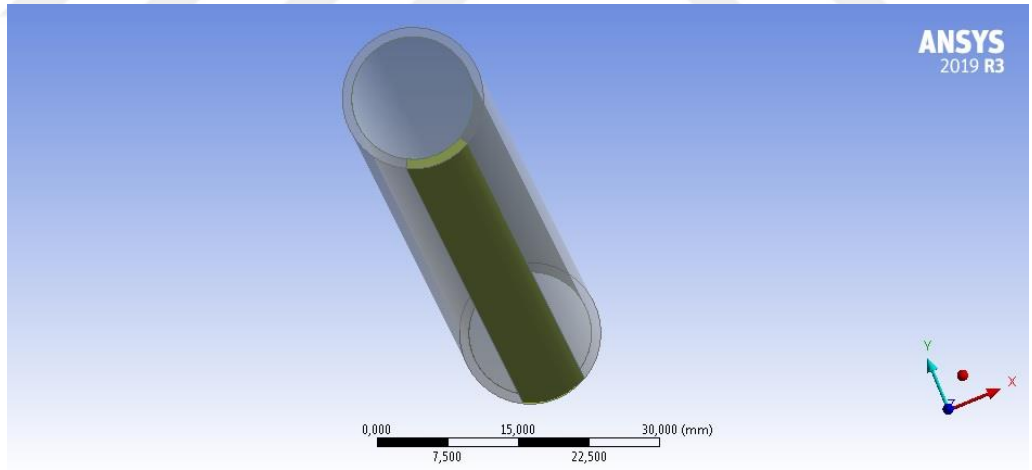
Şekil 4.26. Bakır boruya güneş ışınlarının odaklandığı bölge
