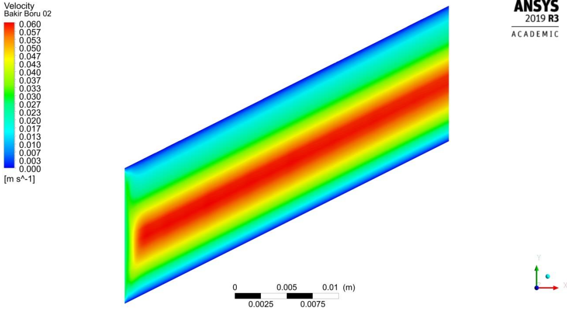
Şekil 4.48. 0.0033 kg/s debide boru merkez çizgisi boyunca kesitin hız dağılımı
