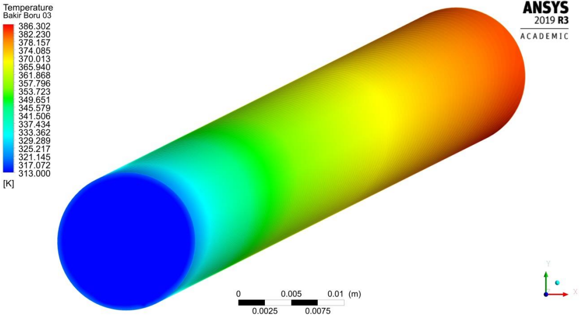
Şekil 4.51. 0.0050 kg/s debide akışkan sıcaklık dağılımı
