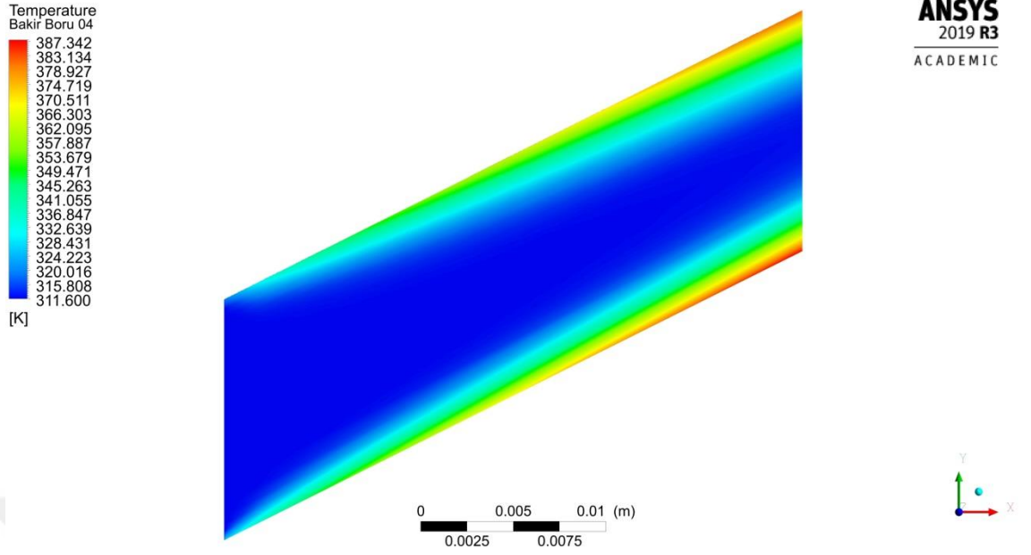
Şekil 4.61. 0.0067 kg/s debide boru merkez çizgisi boyunca kesitinin sıcaklığı dağılımı
