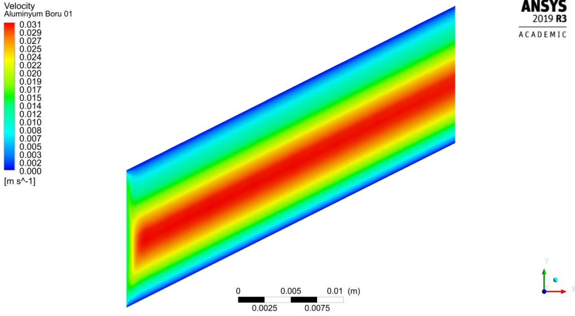
Şekil 4.76. 0.0017 kg/s debide boru merkez çizgisi boyunca kesitin hız dağılımı
