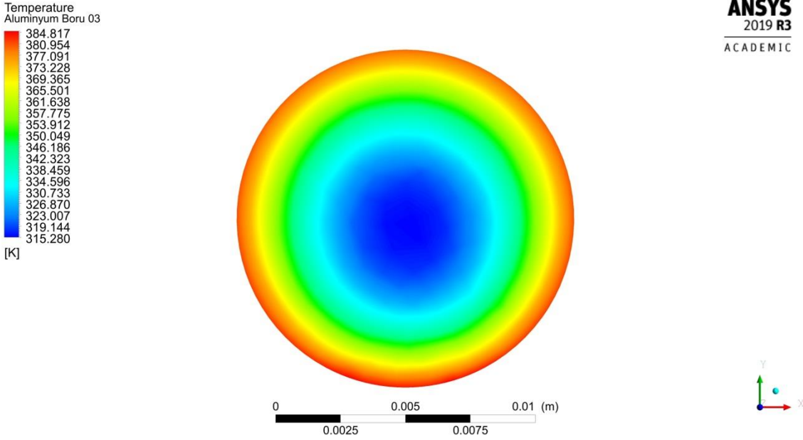
Şekil 4.88. 0.0050 kg/s debide akışkan çıkış sıcaklığı dağılımı
