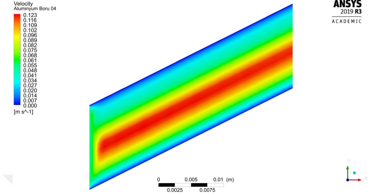
Şekil 4.97. 0.0067 kg/s debide boru merkez çizgisi boyunca kesitin hız dağılımı
