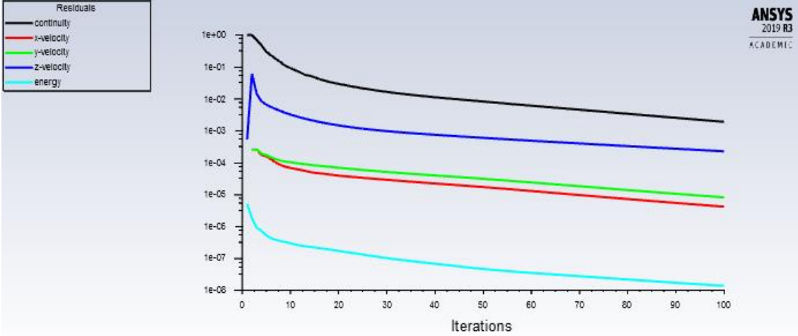
Şekil 4.35. Çözümleme ve iterasyon grafiği
