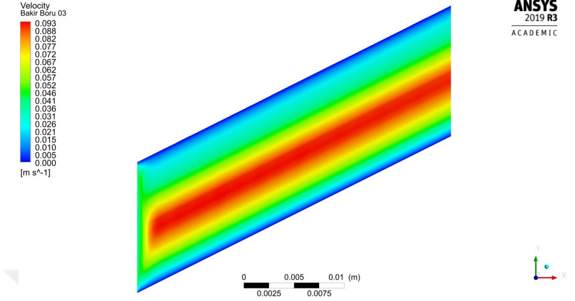
Şekil 4.55. 0.0050 kg/s debide boru merkez çizgisi boyunca kesitin hız dağılımı
