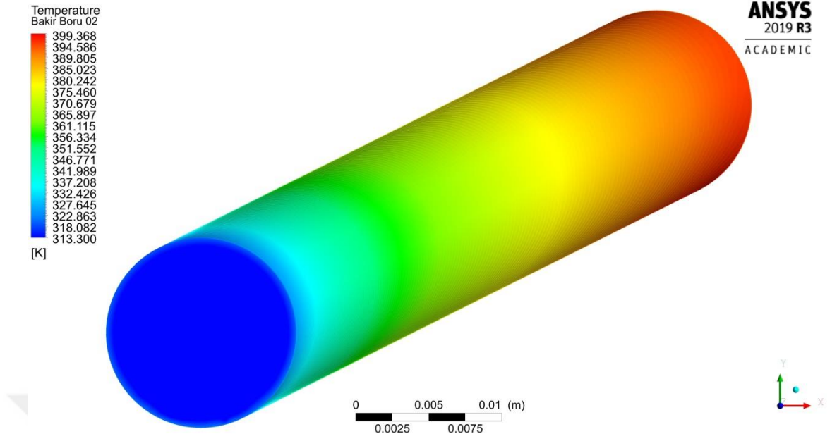
Şekil 4.44. 0.0033 kg/s debide akışkan sıcaklık dağılımı
