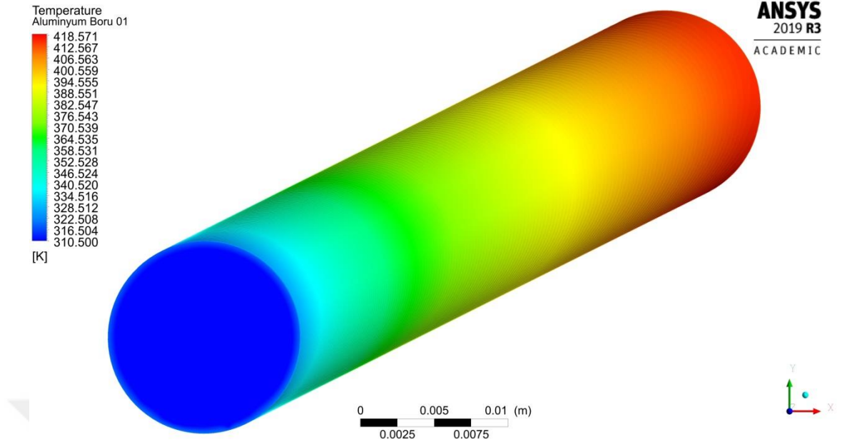
Şekil 4.72. 0.0017 kg/s debide akışkan sıcaklık dağılımı
