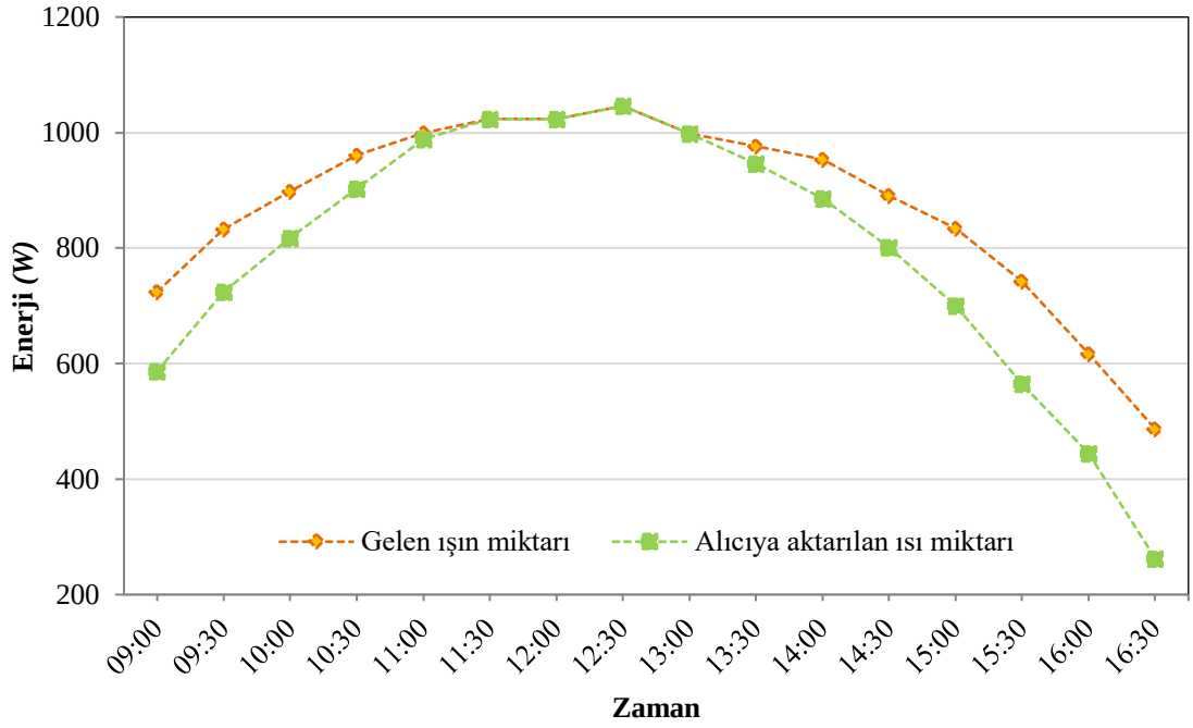
Şekil 5.3. Işın sapma miktarı
