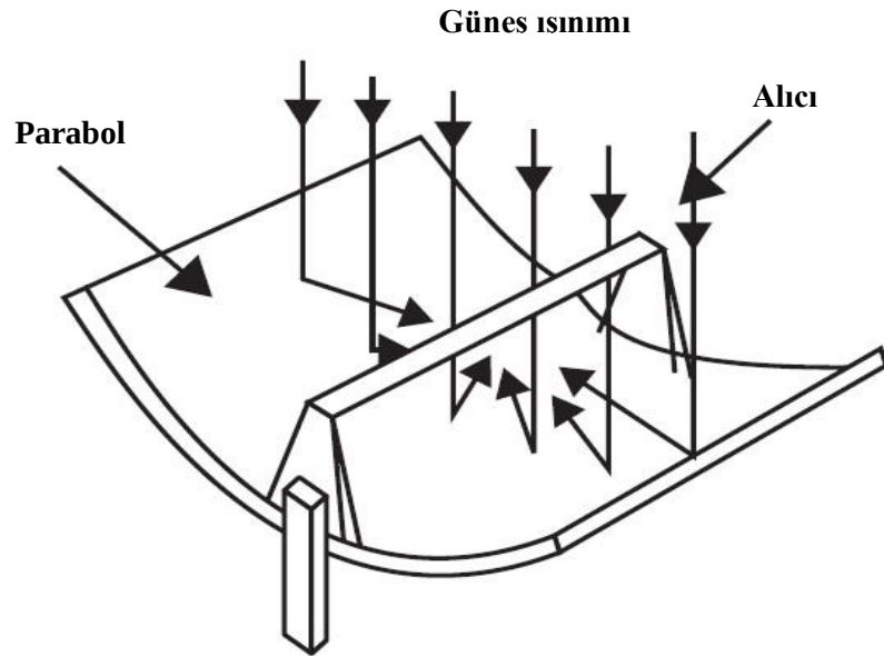
Şekil 1.12. Parabolik oluklu güneş kolektör reflektörü için bir ışın izi diyagramı (Kaloigoru 2009)
