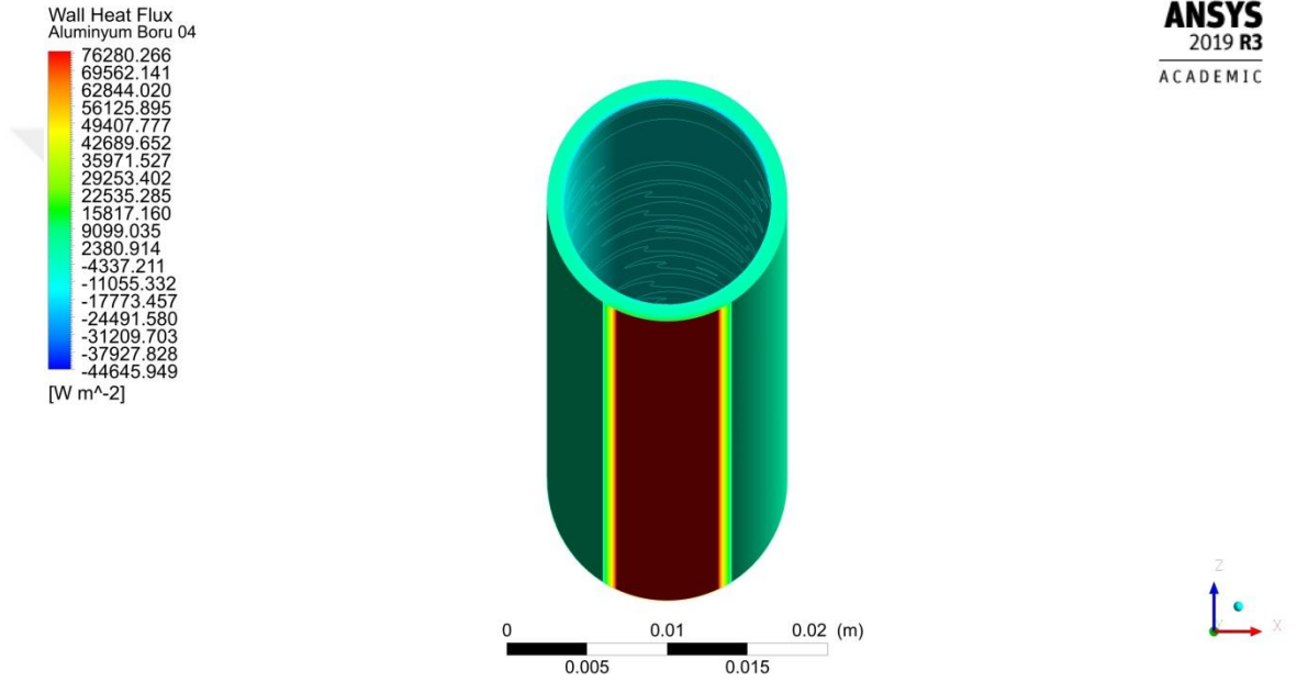
Şekil 4.92. 0.0067 kg/s debi için odak borusu ısı dağılımı
