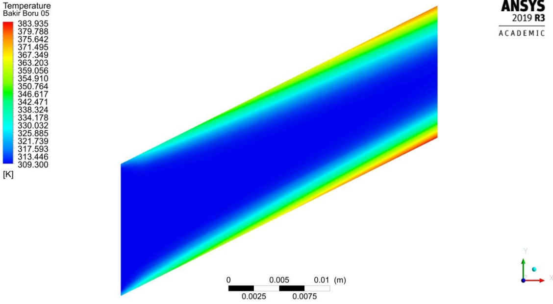
Şekil 4.68. 0.0083 kg/s debide boru merkez çizgisi boyunca kesitin sıcaklığı dağılımı
