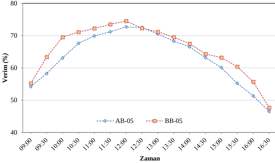
Şekil 5.2. AB-05 ve BB-05 verim karşılaştırılması
