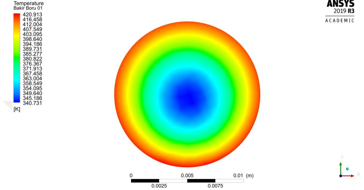
Şekil 4.39. 0.0017 kg/s debide akışkan çıkış sıcaklığı dağılımı
