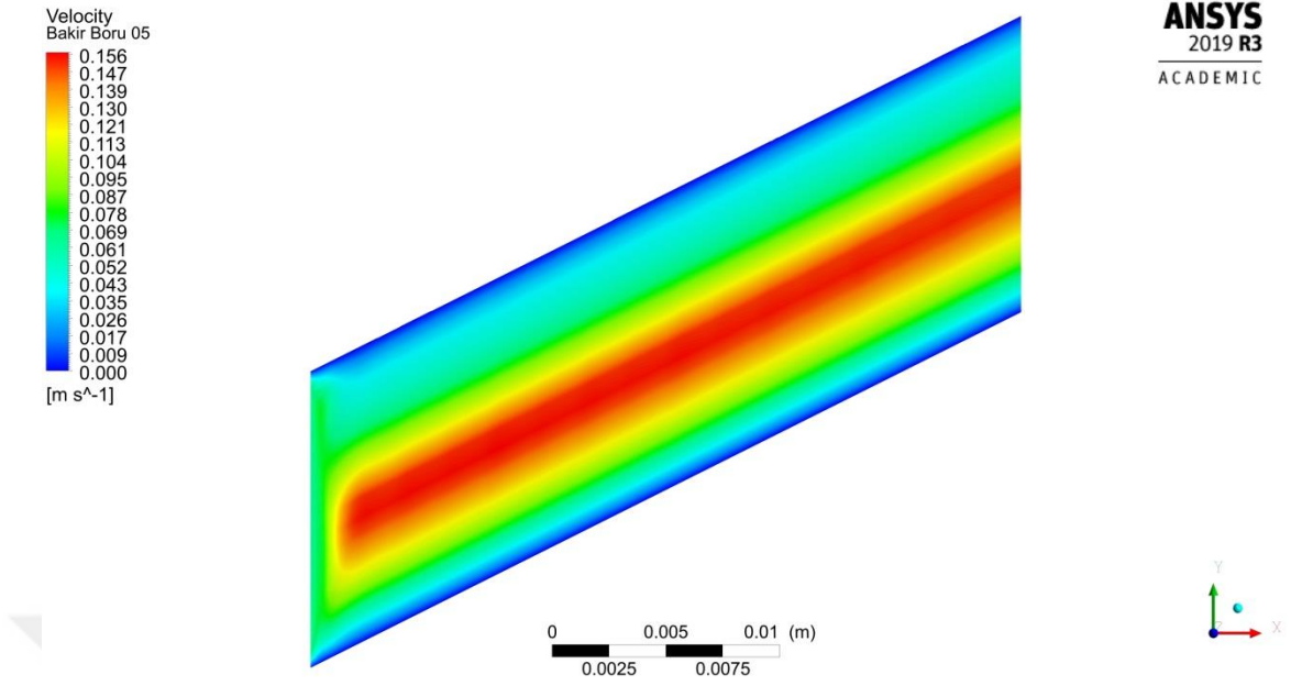
Şekil 4.69. 0.0083 kg/s debide boru merkez çizgisi boyunca kesitin hız dağılımı
