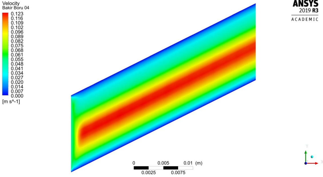
Şekil 4.62. 0.0067 kg/s debide boru merkez çizgisi boyunca kesitin hız dağılımı
