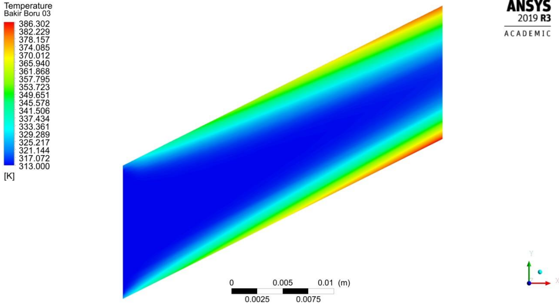
Şekil 4.54. 0.0050 kg/s debide boru merkez çizgisi boyunca kesitin sıcaklığı dağılımı
