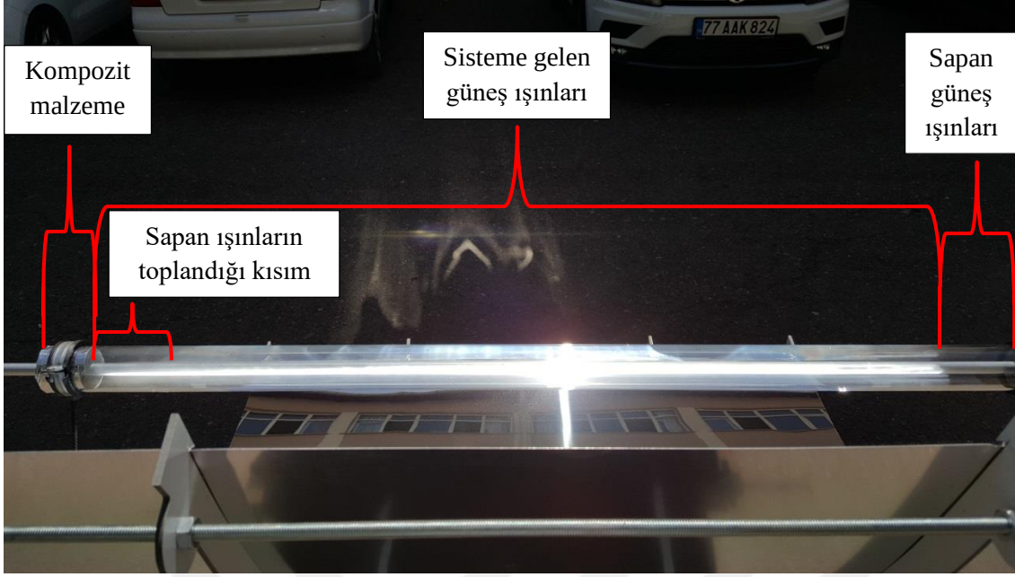
Şekil 4.19. Güneş ışınlarının sapması
