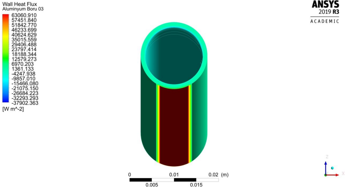
Şekil 4.85. 0.0050 kg/s debi için odak borusu ısı dağılımı
