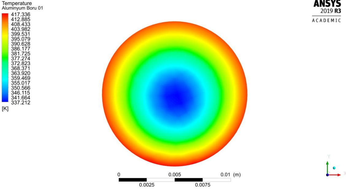
Şekil 4.74. 0.0017 kg/s debide akışkan çıkış sıcaklığı dağılımı
