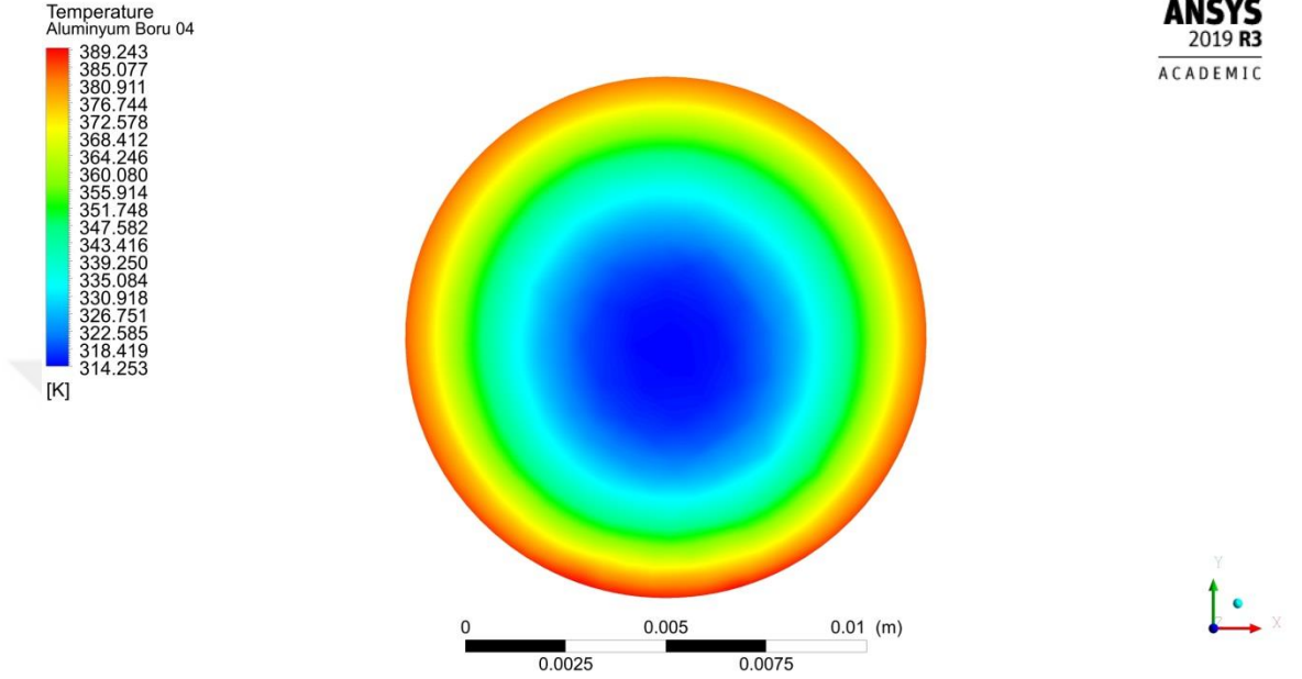
Şekil 4.95. 0.0067 kg/s debide akışkan çıkış sıcaklığı dağılımı
