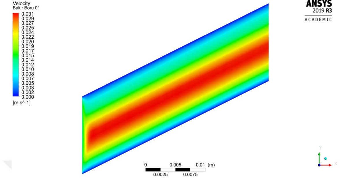
Şekil 4.41. 0.0017 kg/s debide boru merkez çizgisi boyunca kesitinin hız dağılımı
