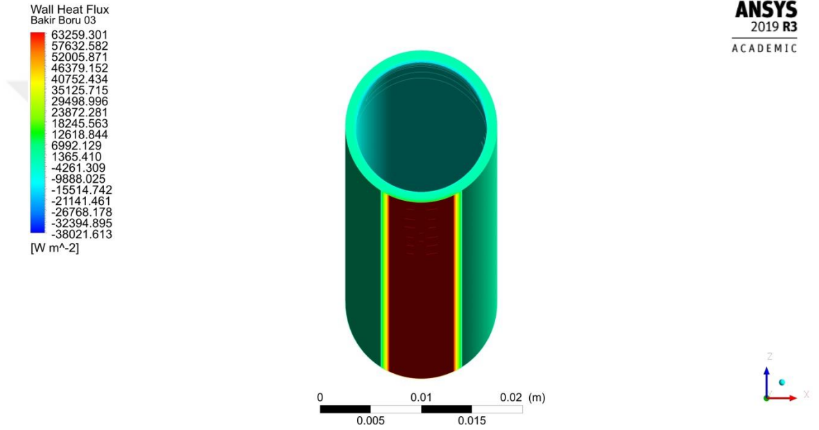
Şekil 4.50. 0.0050 kg/s debi için odak borusu ısı dağılımı
