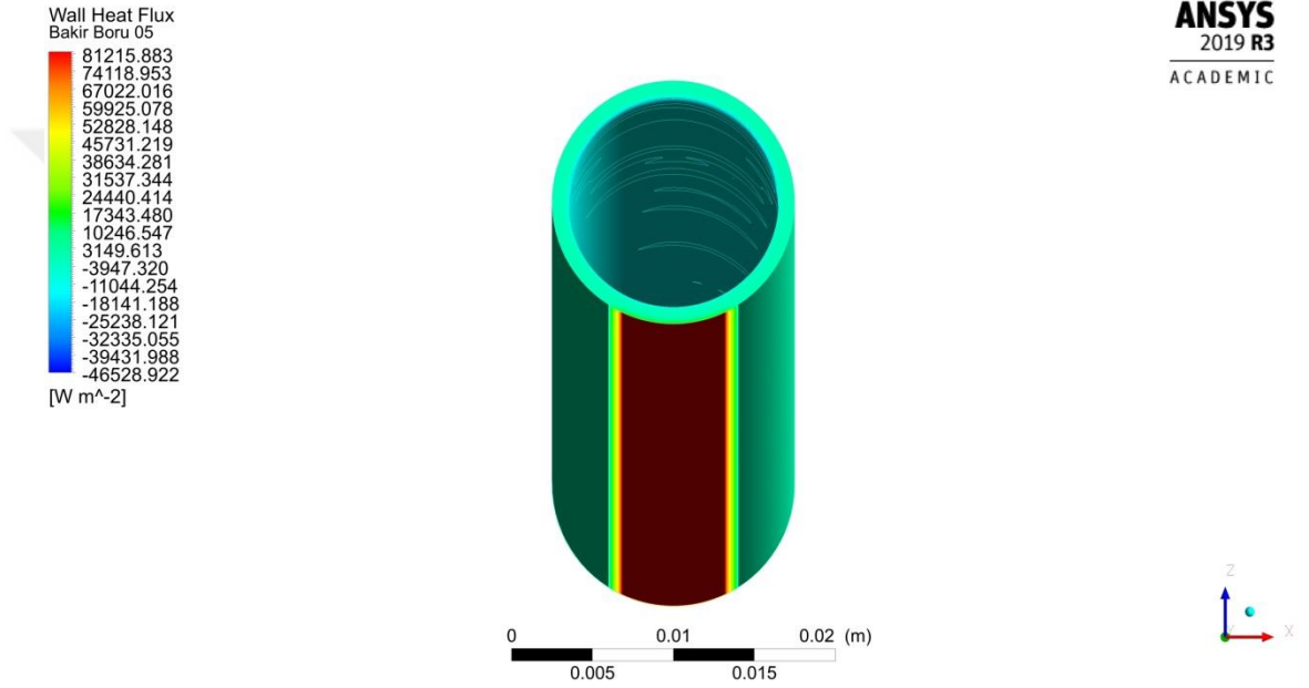
Şekil 4.64. 0.0083 kg/s debi için odak borusu ısı dağılımı
