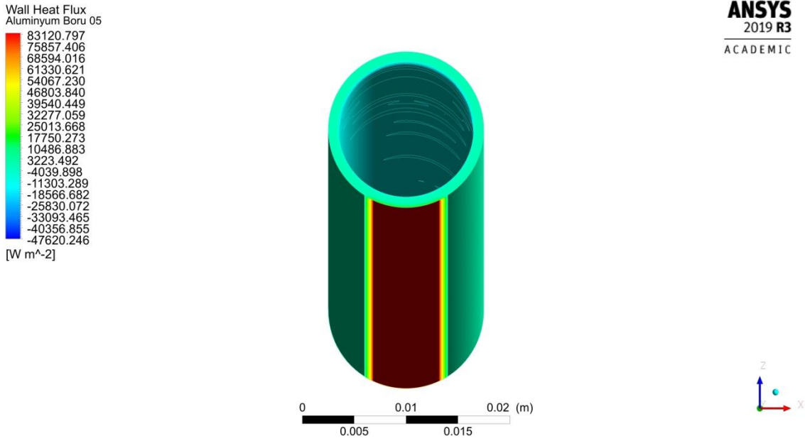
Şekil 4.99. 0.0083 kg/s debi için odak borusu ısı dağılımı
