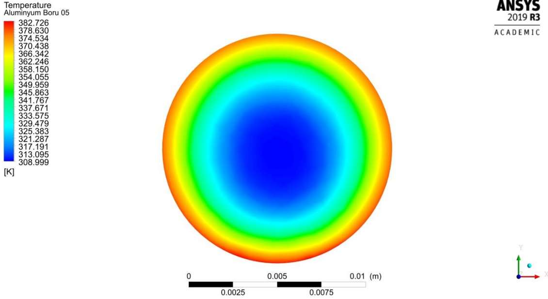
Şekil 4.102. 0.0083 kg/s debide akışkan çıkış sıcaklığı dağılımı
