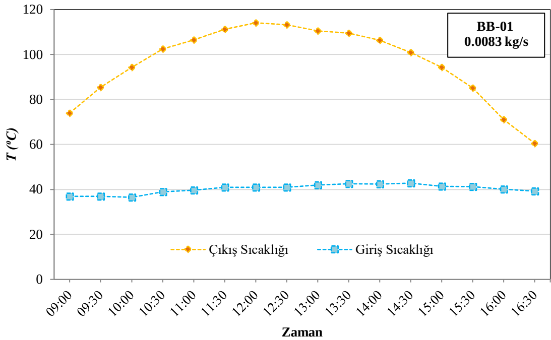
Şekil 4.1. BB-01 0.0083 kg/s debide sisteme suyun giriş ve çıkış sıcaklıkları
