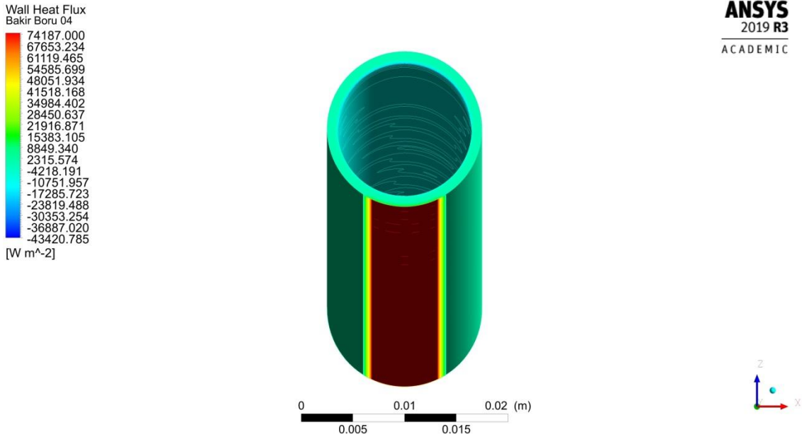
Şekil 4.57. 0.0067 kg/s debi için odak borusu ısı dağılımı
