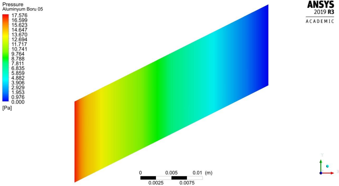
Şekil 4.105. 0.0083 kg/s debide boru merkez çizgisi boyunca kesitin basınç dağılımı
