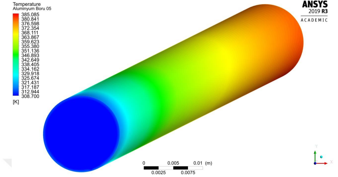
Şekil 4.100. 0.0083 kg/s debide akışkan sıcaklık dağılımı
