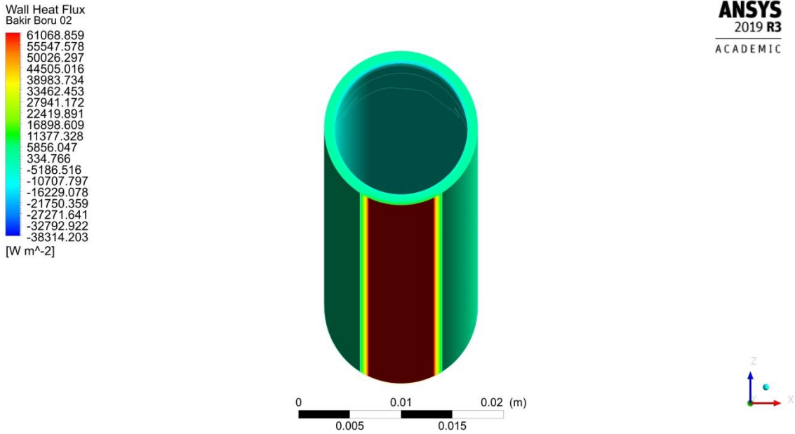
Şekil 4.43. 0.0033 kg/s debi için odak borusu ısı dağılımı
