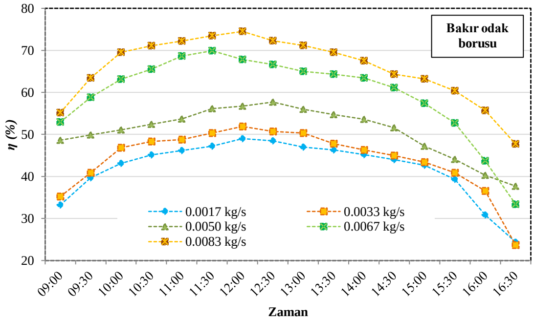
Şekil 4.7. Bakır odak borulu deney düzeneği ile yapılan deneylerin verim-zaman grafiği
