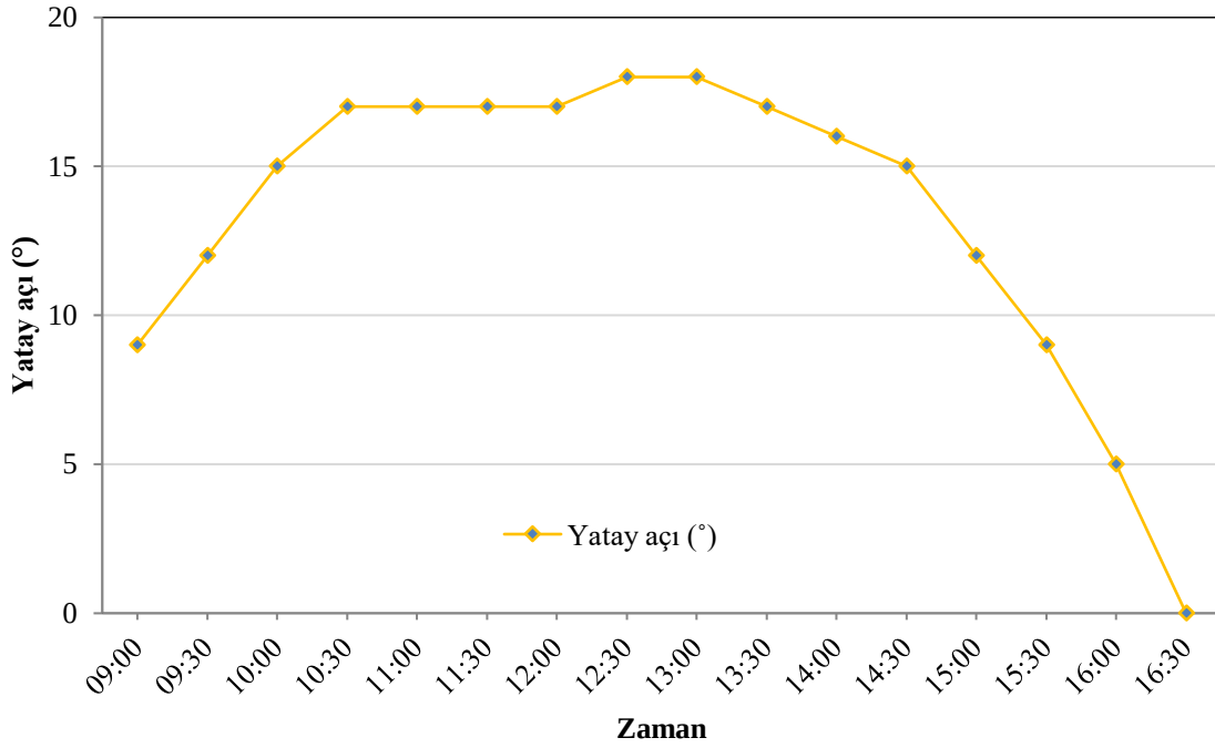
Şekil 4.2. Yatay açının zamanla değişimi
