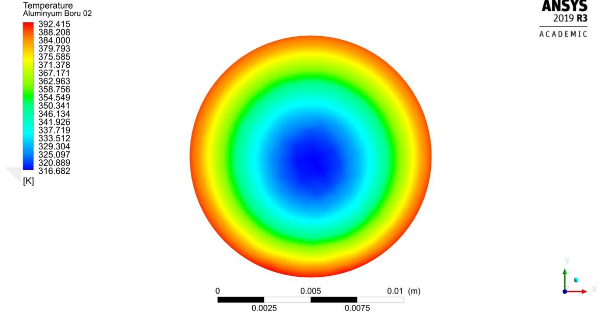
Şekil 4.81. 0.0033 kg/s debide akışkan çıkış sıcaklığı dağılımı
