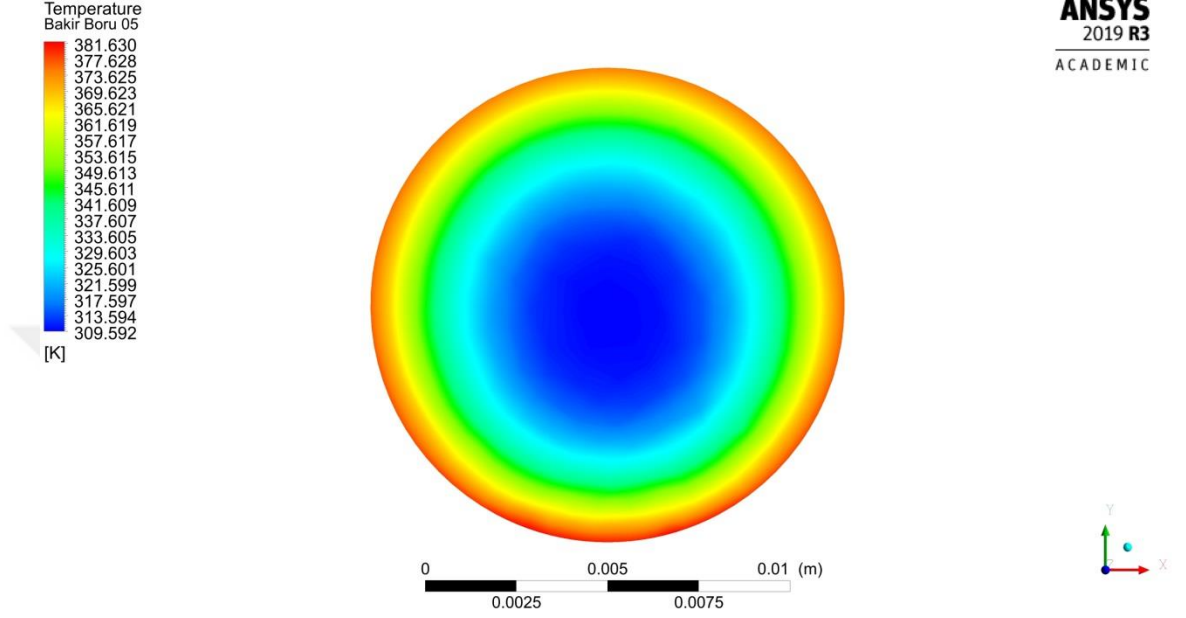
Şekil 4.67. 0.0083 kg/s debide akışkan çıkış sıcaklığı dağılımı
