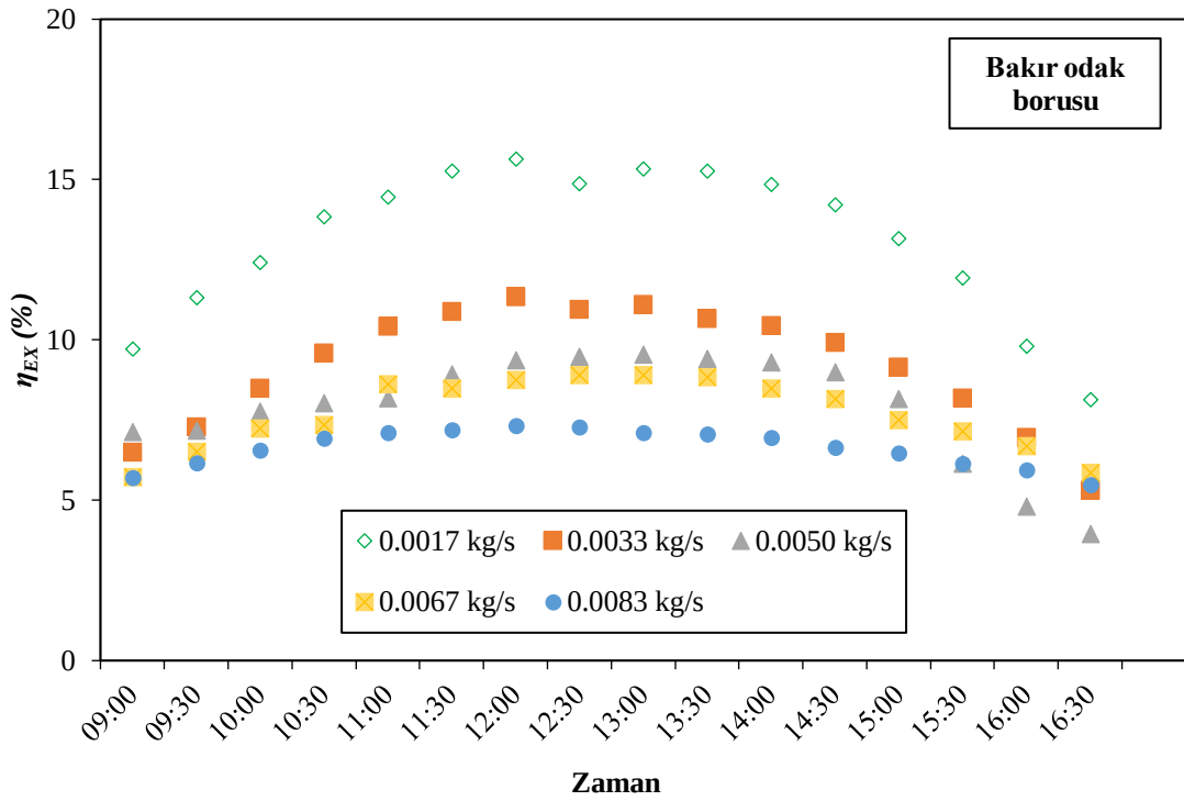
Şekil 4.8. Bakır boru ekserji verimi – zaman grafiği
