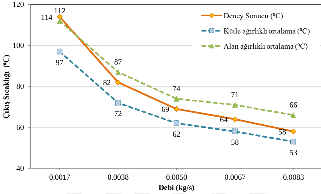
Şekil 4.107. Bakır boru deney ve simülasyon çıkış sıcaklıkları
