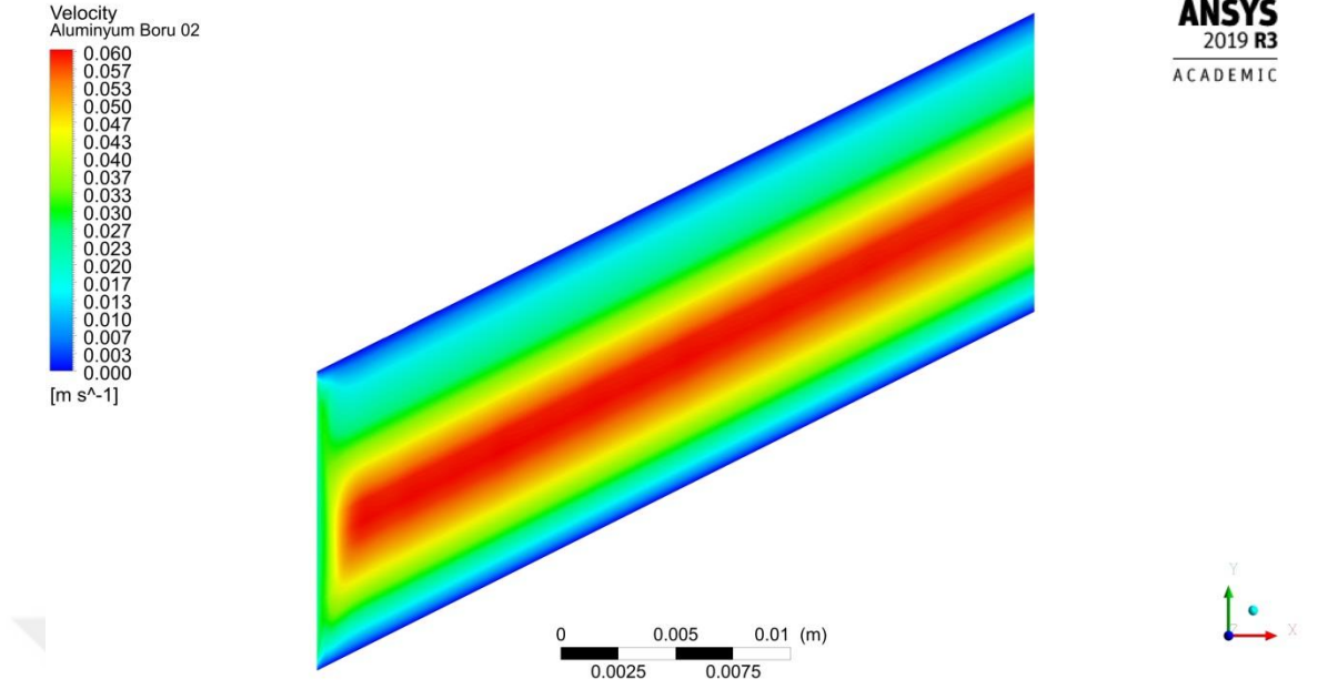
Şekil 4.83. 0.0033 kg/s debide boru merkez çizgisi boyunca kesitin hız dağılımı
