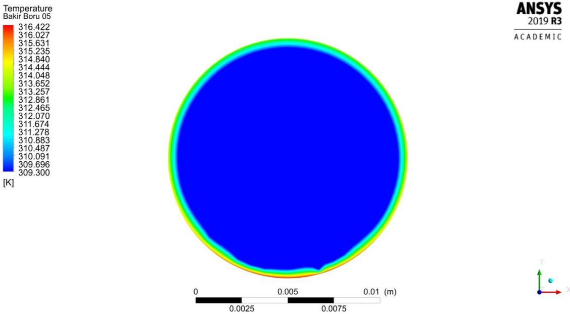
Şekil 4.66. 0.0083 kg/s debide akışkan giriş sıcaklığı dağılımı
