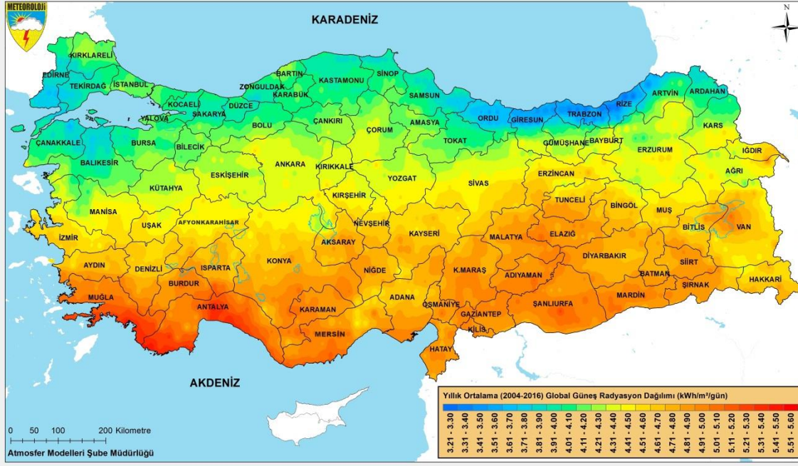
Şekil 1.2. Türkiye’de global güneş radyasyon dağılımı (kWh/m 2 /gün) (MGM 2016)
