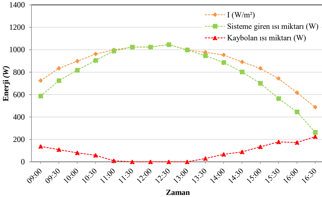
Şekil 4.20. BB-05 deneyi sapmadan kaynaklanan enerji kayıpları
