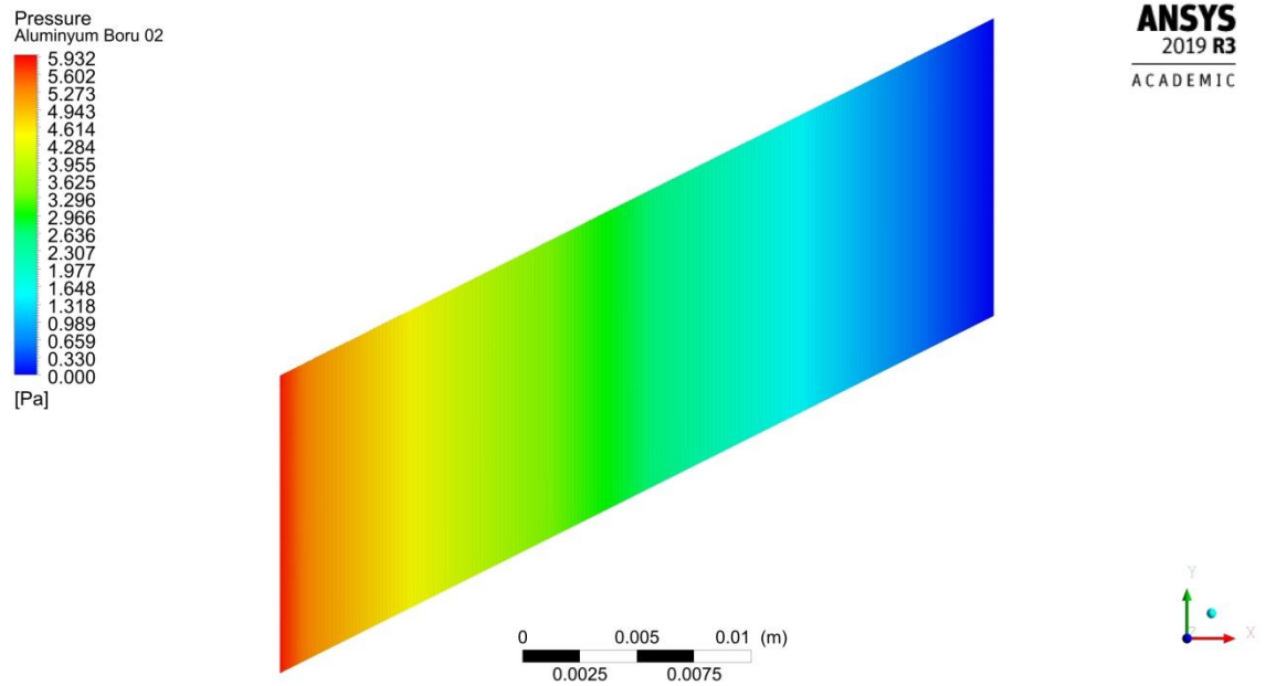
Şekil 4.84. 0.0033 kg/s debide boru merkez çizgisi boyunca kesitin basınç dağılımı
