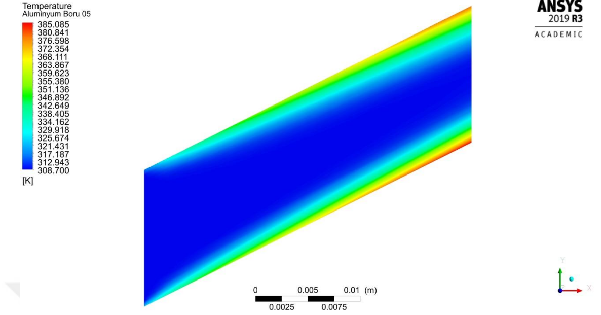
Şekil 4.103. 0.0083 kg/s debide boru merkez çizgisi boyunca kesitin sıcaklığı dağılımı
