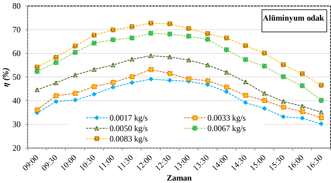
Şekil 4.11. Alüminyum odak borulu deney düzeneği ile yapılan deneylerin verim-zaman grafiği
