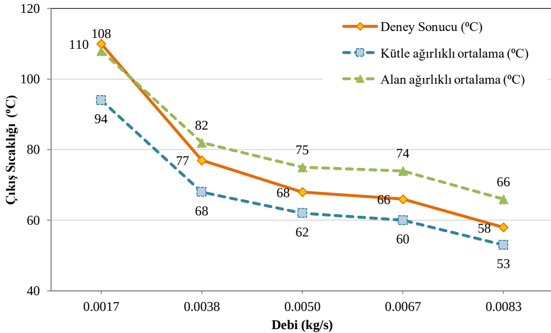
Şekil 4.108. Alüminyum boru deney ve simülasyon çıkış sıcaklıkları
