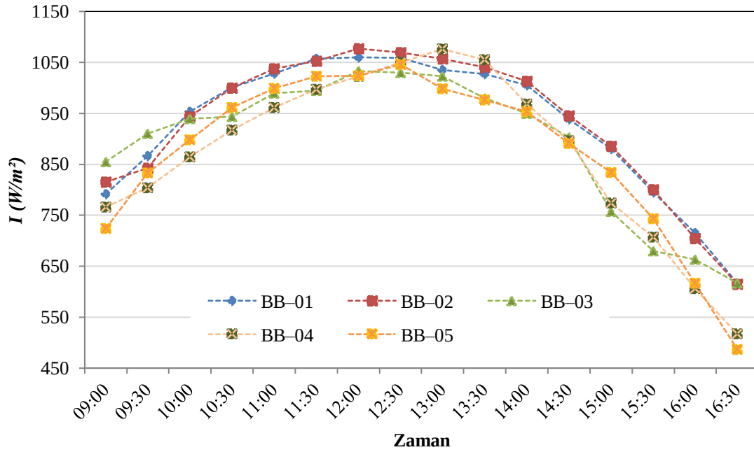
Şekil 4.3. Bakır odak borusunun güneş ısıtım değerlerinin zamanla değişimi
