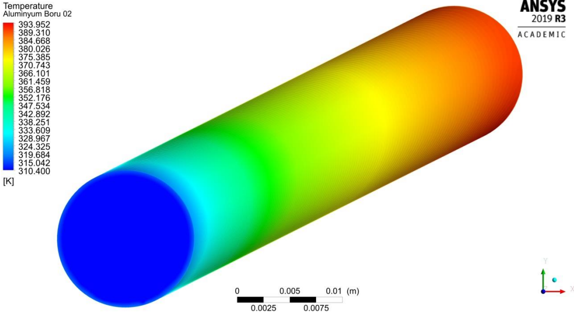
Şekil 4.79. 0.0033 kg/s debide akışkan sıcaklık dağılımı
