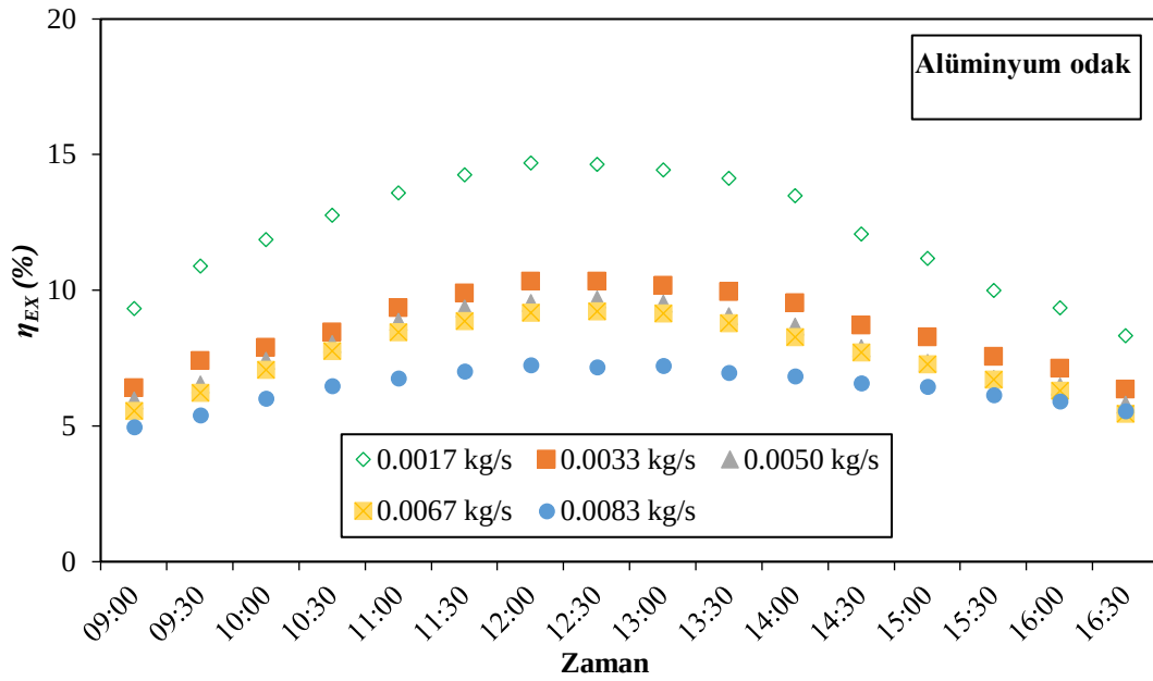
Şekil 4.12. Alüminyum boru ekserji verimi – zaman grafiği
