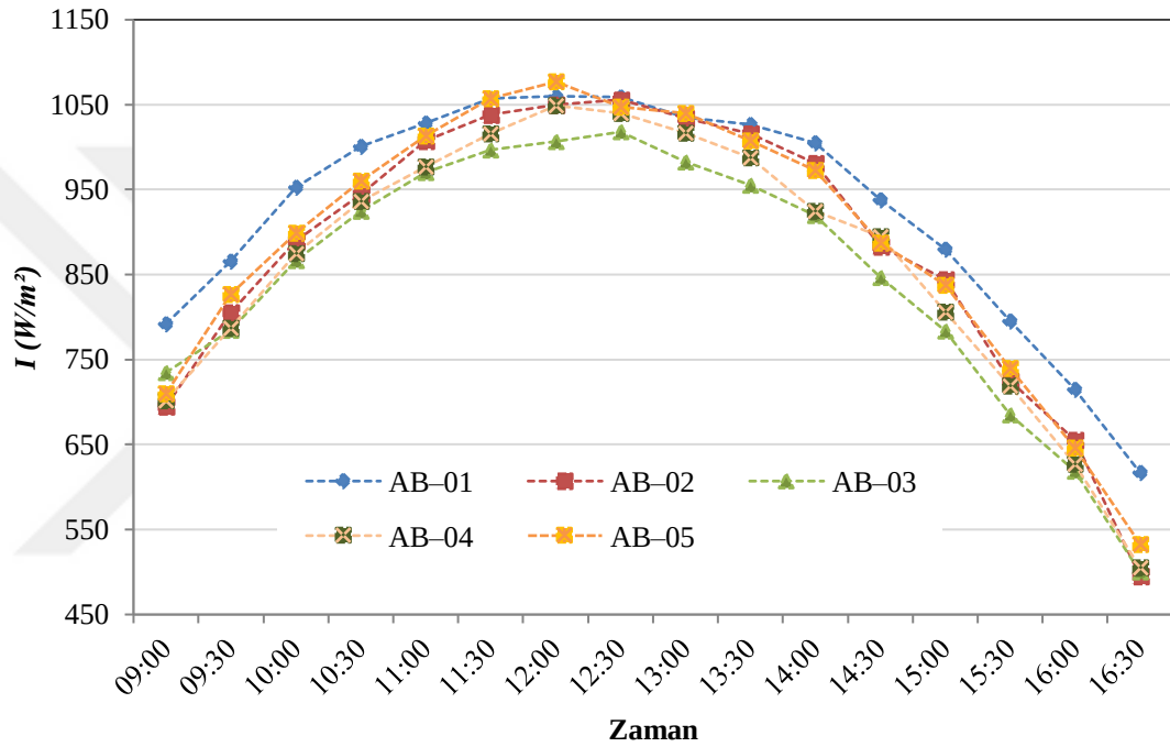
Şekil 4.4. Alüminyum odak borusunun güneş ışınlam değerlerinin zamanla değişimi
