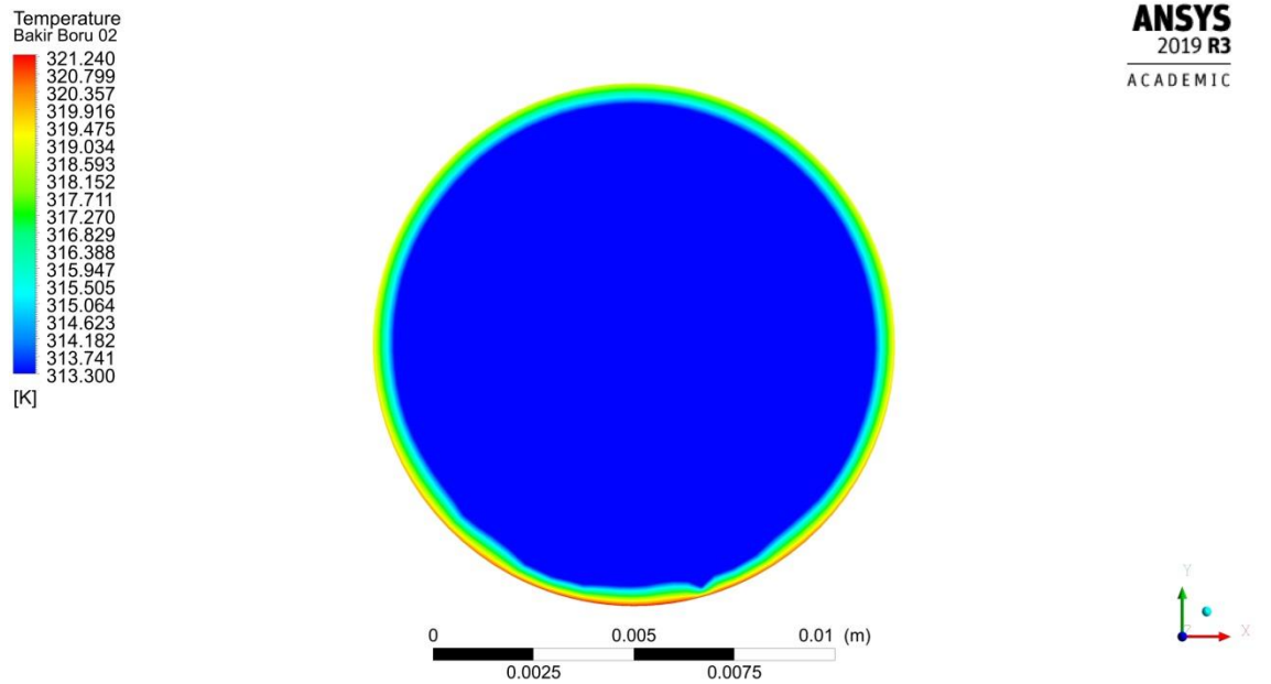
Şekil 4.45. 0.0033 kg/s debide akışkan giriş sıcaklığı dağılımı
