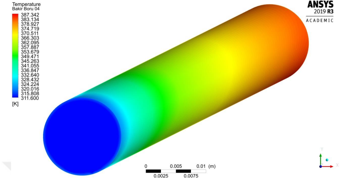
Şekil 4.58. 0.0067 kg/s debide akışkan sıcaklık dağılımı
