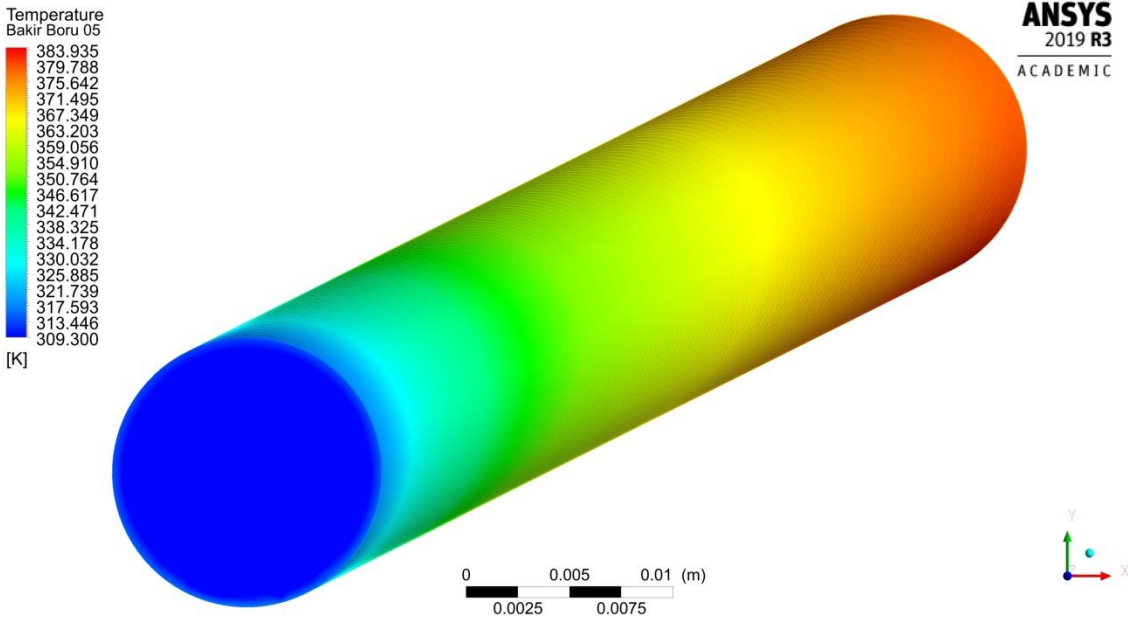
Şekil 4.65. 0.0083 kg/s debide akışkan sıcaklık dağılımı
