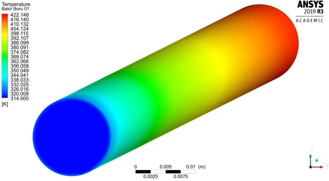
Şekil 4.37. 0.0017 kg/s debide akışkan sıcaklık dağılımı
