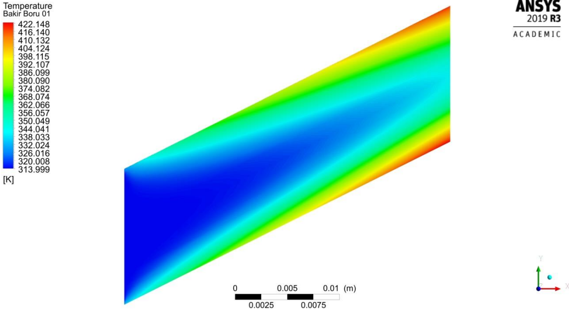
Şekil 4.40. 0.0017 kg/s debide boru merkez çizgisi boyunca kesitin sıcaklığı dağılımı
