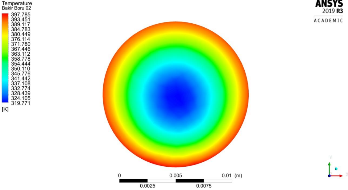
Şekil 4.46. 0.0033 kg/s debide akışkan çıkış sıcaklığı dağılımı
