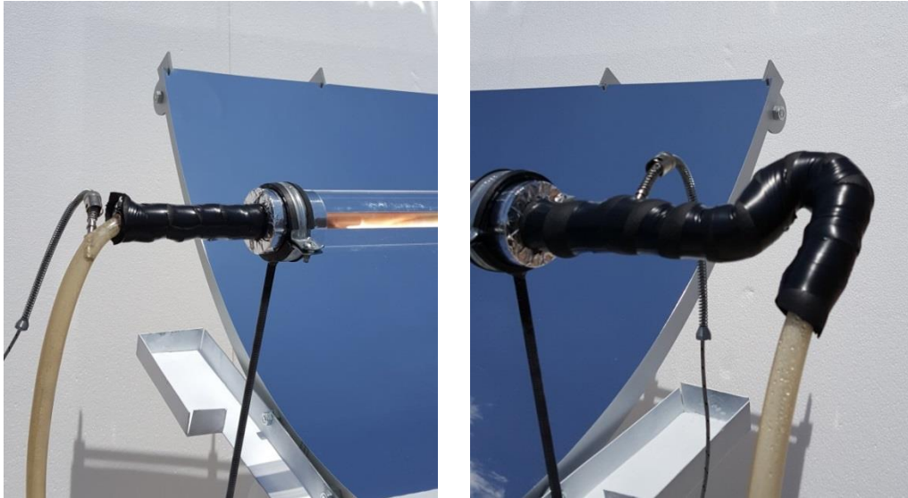
Şekil 3.9. Dijital proplu termometre ile giriş ve çıkış sıcaklıklarının ölçümü
