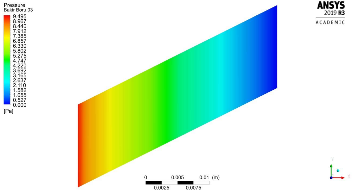
Şekil 4.56. 0.0050 kg/s debide boru merkez çizgisi boyunca kesitin basınç dağılımı
