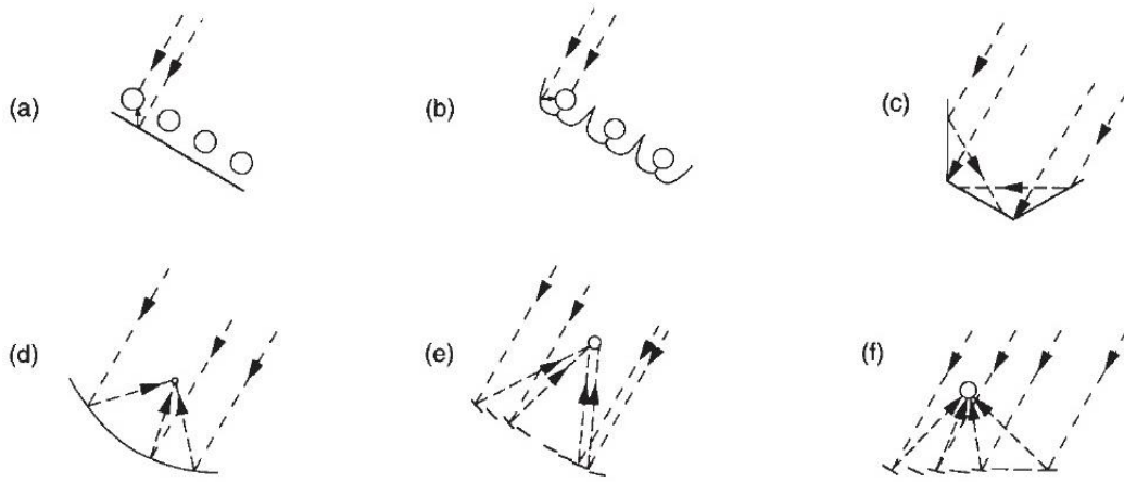
Şekil 1.5. Yoğunlaştırıcı kolektör konfigürasyonları (a) Arkadan yansıtıcı borulu emiciler; (b) Tepe yansıtıcı tüplü emiciler; (c) Düzlemsel yansıtıcı yoğunlaştırıcı; (d) Parabolik yoğunlaştırıcı; (e) Fresnel yansıtıcı; (f) Merkezi alıcıya sahip heliostat dizisi (Duffie ve Beckman 2005)
