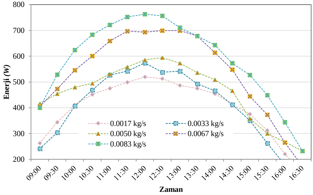
Şekil 4.6. BB suya aktarılan ısı-zaman grafiği
