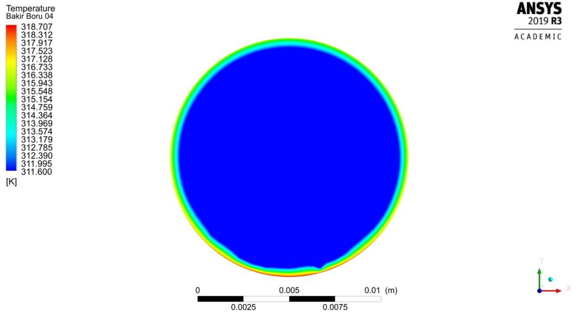
Şekil 4.59. 0.0067 kg/s debide akışkan giriş sıcaklığı dağılımı
