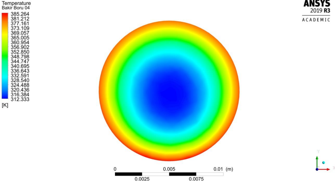
Şekil 4.60. 0.0067 kg/s debide akışkan çıkış sıcaklığı dağılımı
