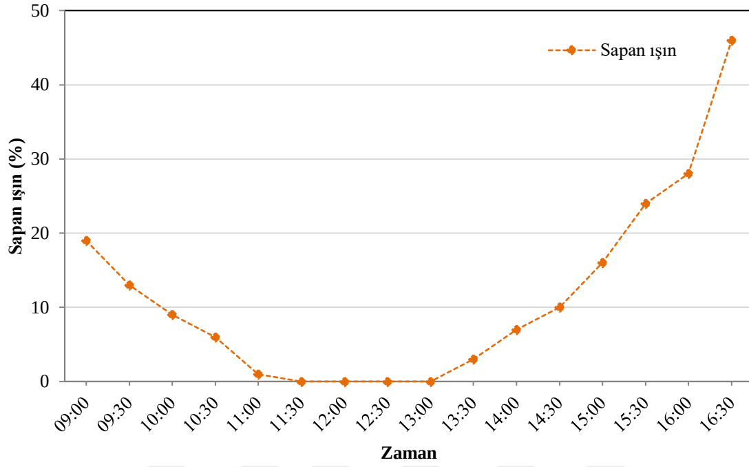
Şekil 4.16. Gün içerisinde sapan ışı-zaman grafiği
