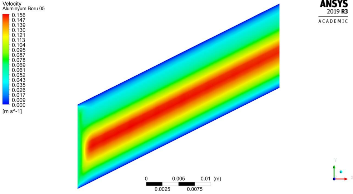
Şekil 4.104. 0.0083 kg/s debide boru merkez çizgisi boyunca kesitin hız dağılımı
