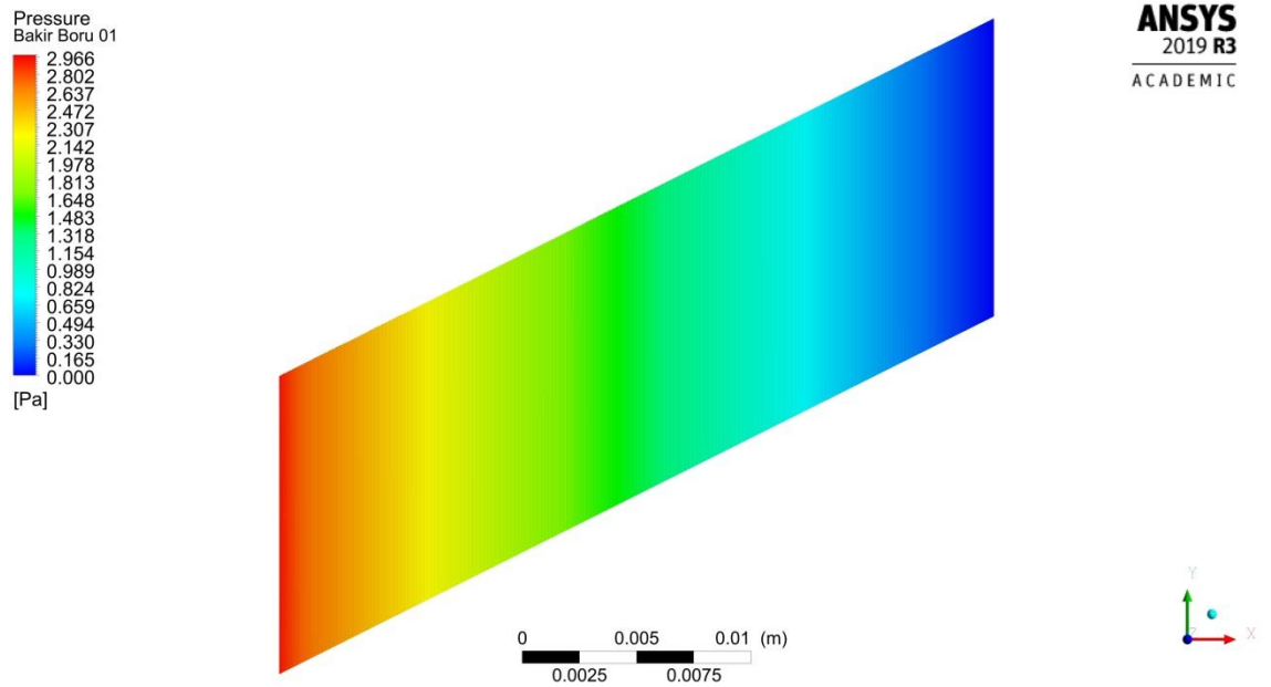
Şekil 4.42. 0.0017 kg/s debide boru merkez çizgisi boyunca kesitinin basınç dağılımı
