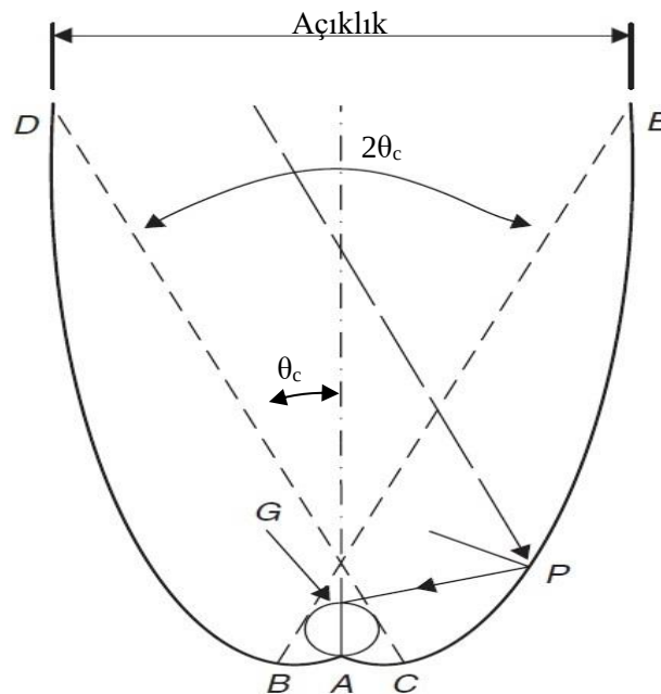
Şekil 3.21. POGK'nun parabol açıklığı şematik gösterimi (Kalogirou 2009)
