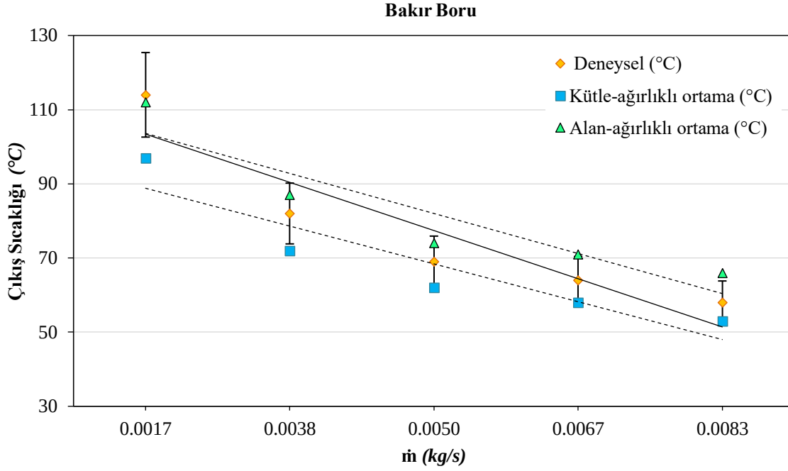
Şekil 5.4. Bakır boru deney ve simülasyon çıkış sıcaklıkları hata okuma
