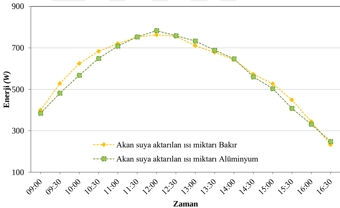
Şekil 5.1. Alüminyum ve bakır boru malzemeleri ile suya ısı aktarımının karşılaştırılması
