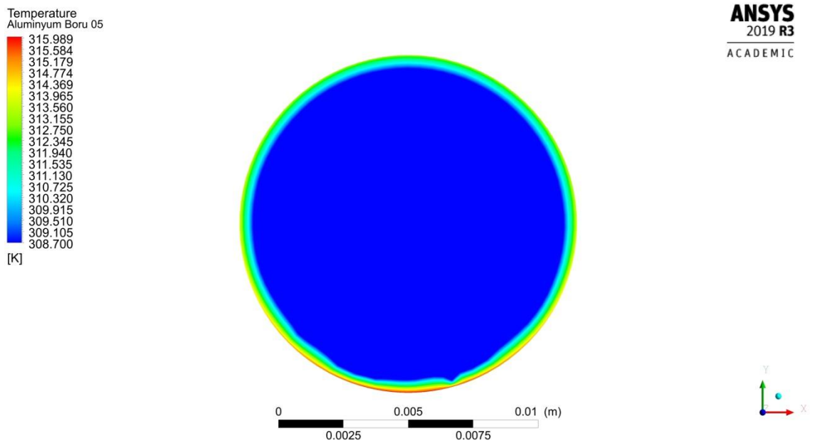
Şekil 4.101. 0.0083 kg/s debide akışkan giriş sıcaklığı dağılımı
