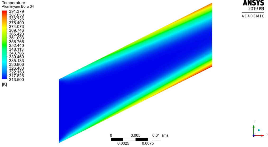
Şekil 4.96. 0.0067 kg/s debide boru merkez çizgisi boyunca kesitin sıcaklığı dağılımı
