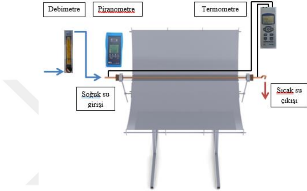
Şekil 3.10. Deney seti düzeneği ve ölçüm cihazları
