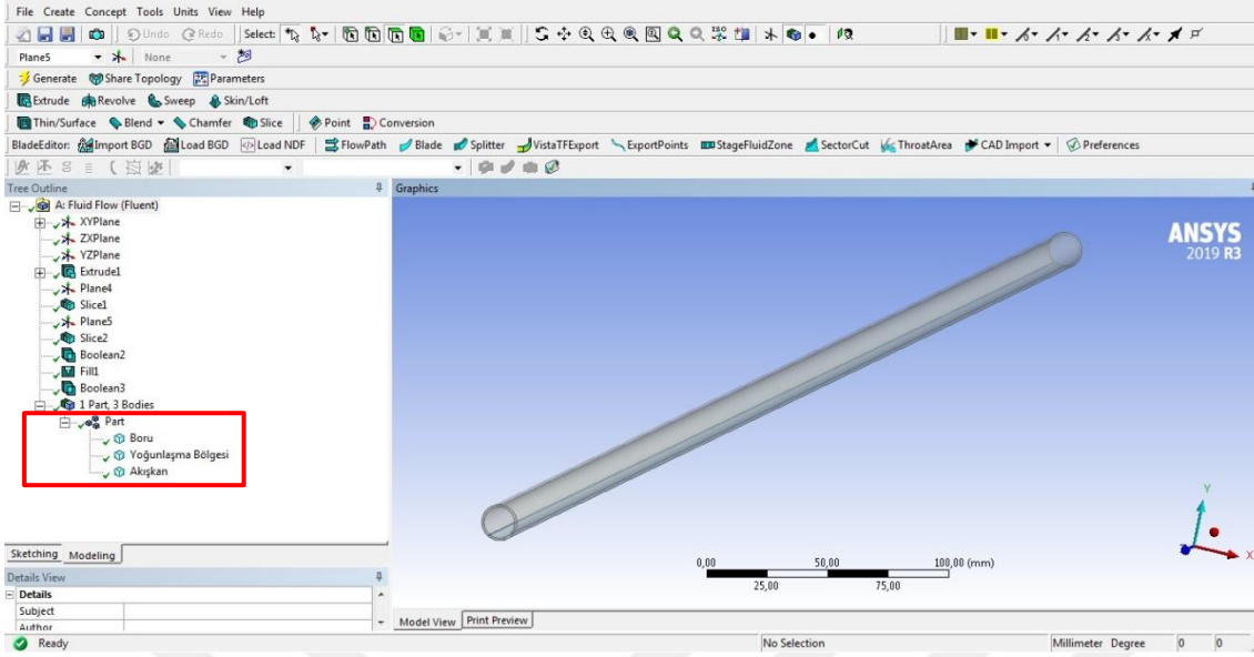
Şekil 4.27. Materyal sınır bölgelerinin belirlenmesi
