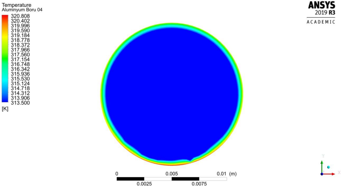
Şekil 4.94. 0.0067 kg/s debide akışkan giriş sıcaklığı dağılımı
