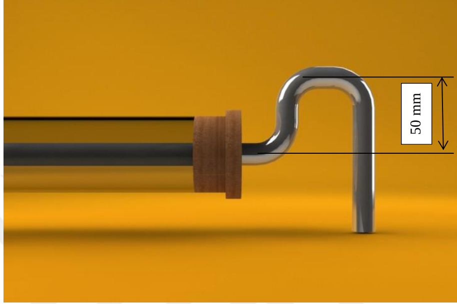
Şekil 3.14. Odak borusu kot farkı
