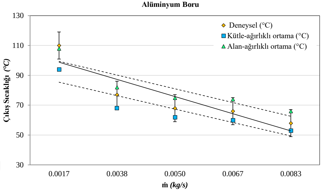
Şekil 5.5. Alüminyum malzeme boru deney ve simülasyon çıkış sıcaklıkları hata okuma
