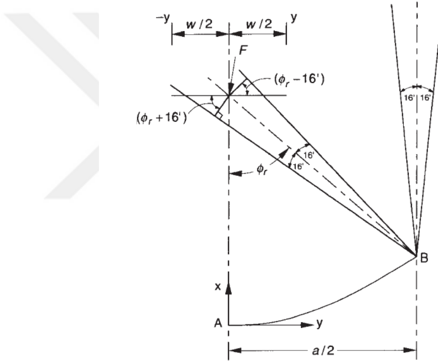
Şekil 3.12. Odaklanma çapı ile ilgili geometrik açılar (Duffie ve Beckman 2005)
