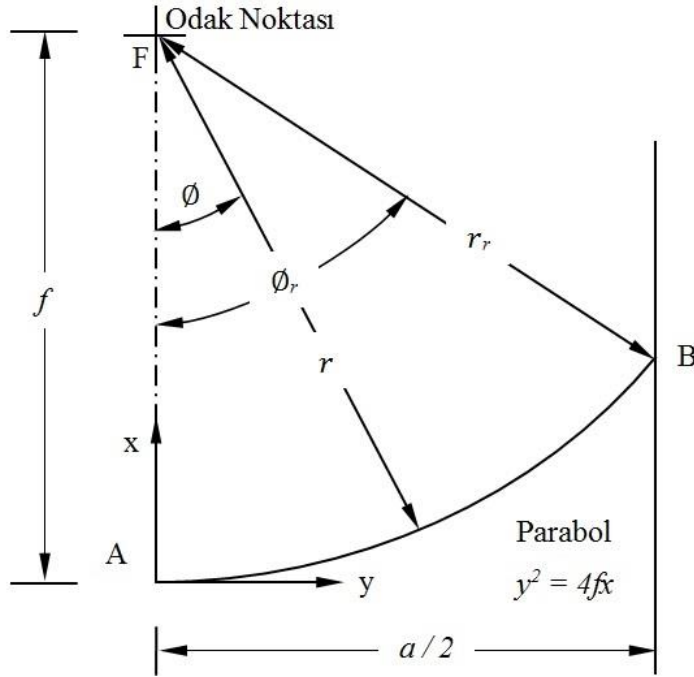
Şekil 3.20. Parabolik oluk geometrisi (Duffie ve Beckman 2005)
