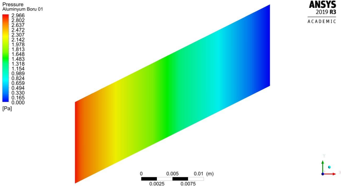
Şekil 4.77. 0.0017 kg/s debide boru merkez çizgisi boyunca kesitin basınç dağılımı
