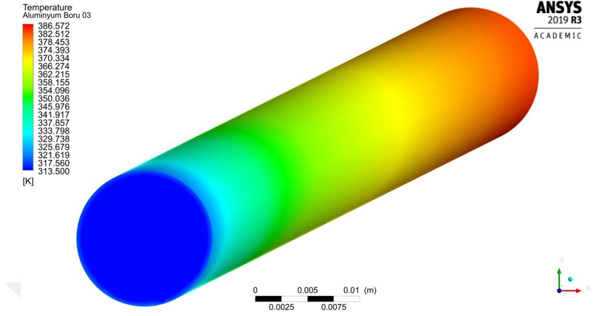
Şekil 4.86. 0.0050 kg/s debide akışkan sıcaklık dağılımı
