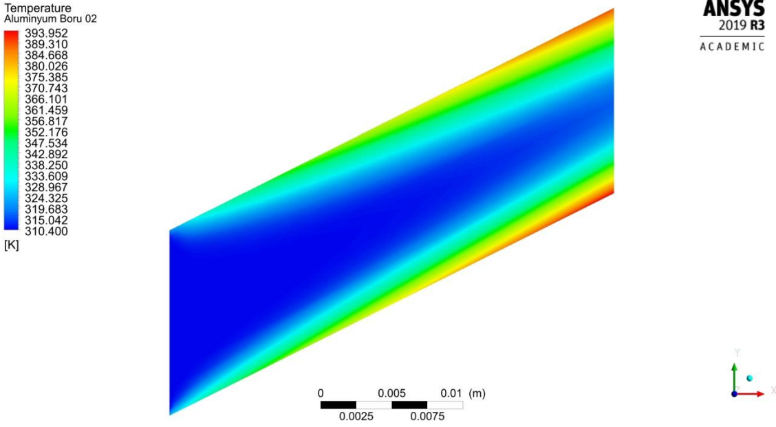
Şekil 4.82. 0.0033 kg/s debide boru merkez çizgisi boyunca kesitin sıcaklığı dağılımı
