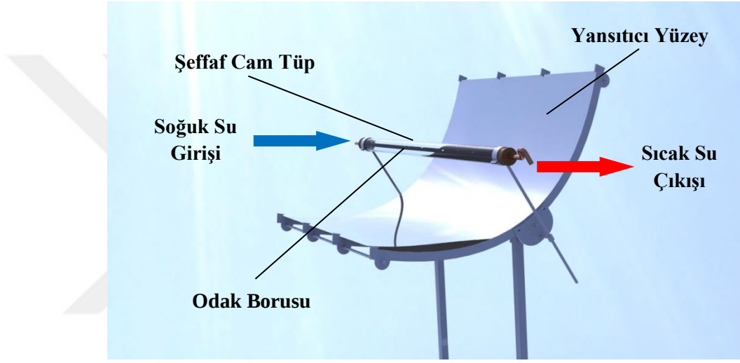
Şekil 1.14. Parabolik oluklu kollektör şematik gösterimi
