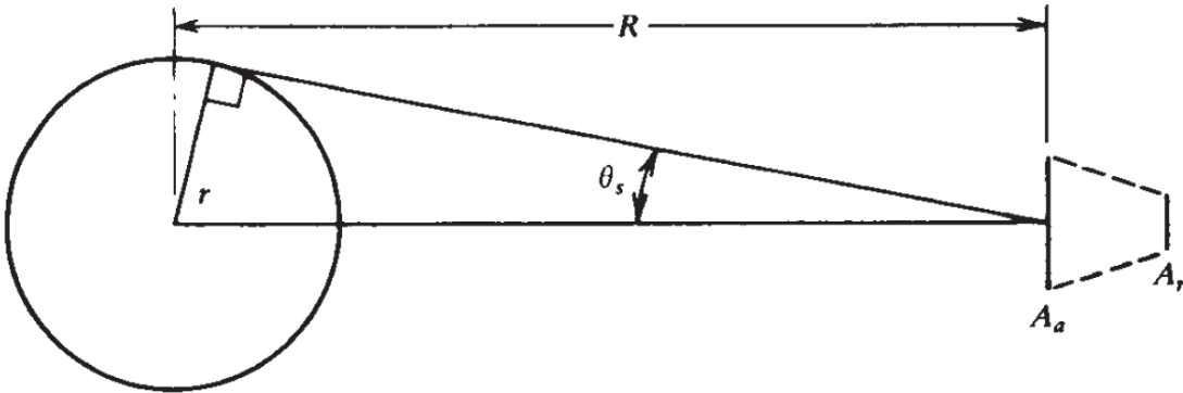
Şekil 3.23. Güneş ışınlarının yoğunlaşmasının şematik gösterimi (Duffie ve Beckman 2005)
