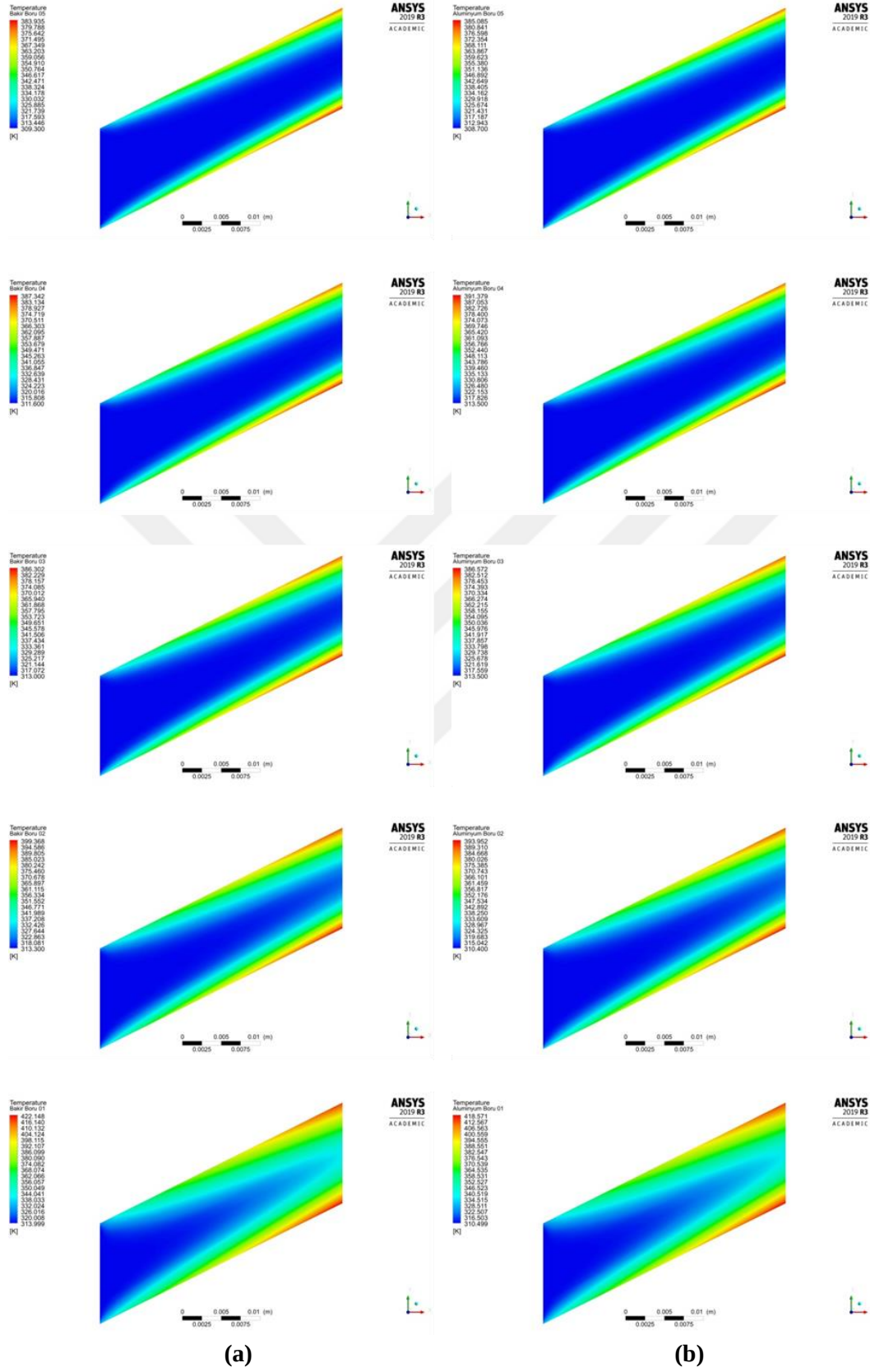
Şekil 4.109. Artan debiye göre (a) Bakır boru (b) Alüminyum boru için merkez çizgisi boyuna kesit sıcaklık dağılımları
