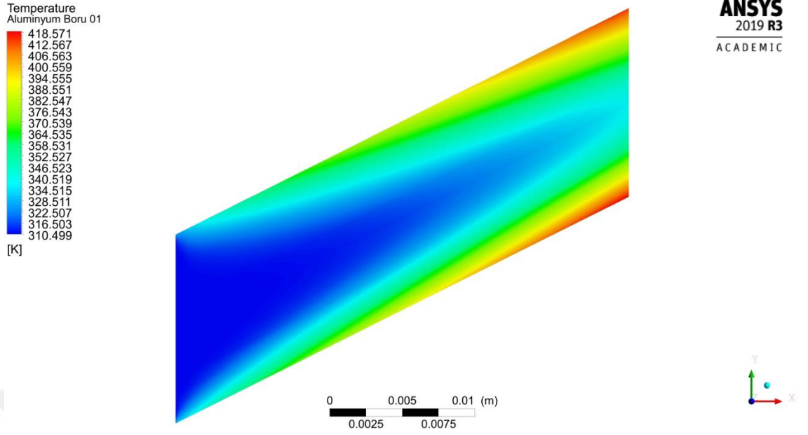
Şekil 4.75. 0.0017 kg/s debide boru merkez çizgisi boyunca kesitinin sıcaklığı dağılımı
