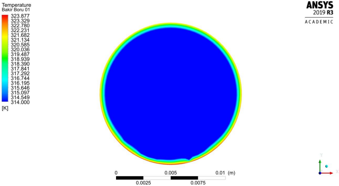
Şekil 4.38. 0.0017 kg/s debide akışkan giriş sıcaklığı dağılımı
