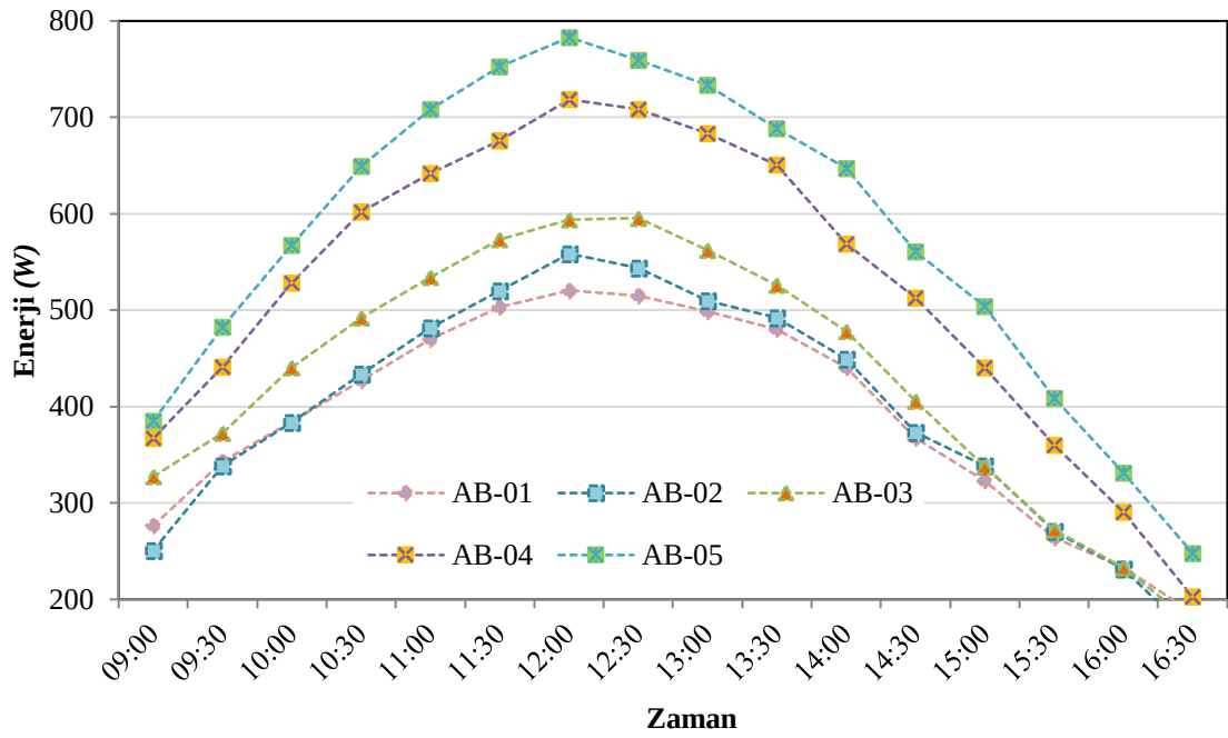
Şekil 4.10. AB suya aktarılan ısı-zaman grafiği
