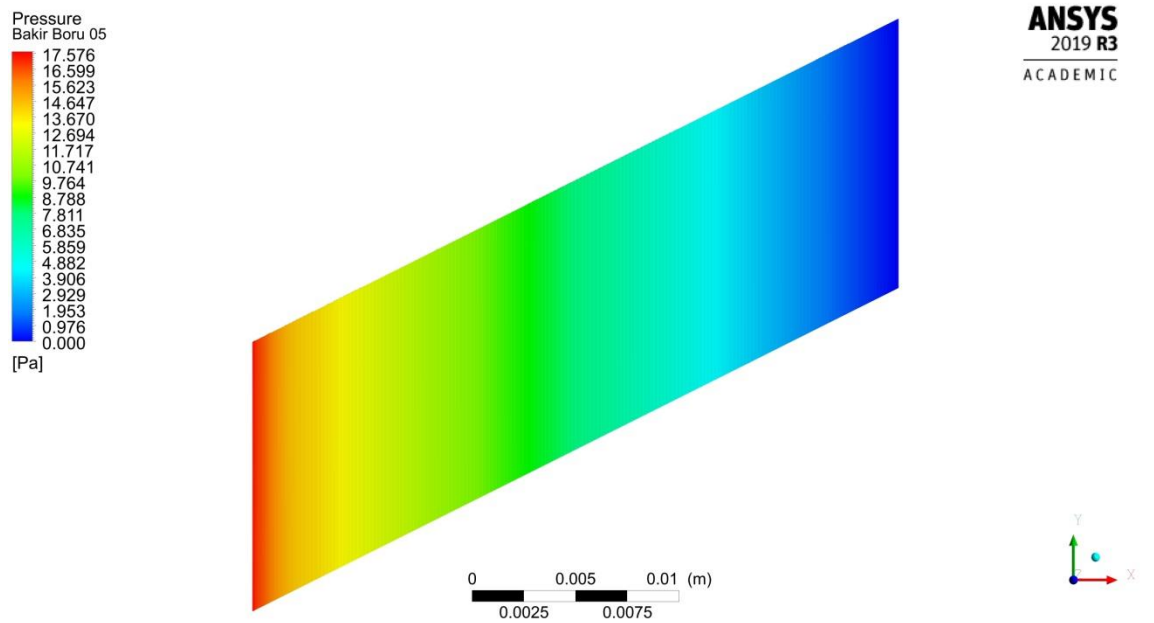
Şekil 4.70. 0.0083 kg/s debide boru merkez çizgisi boyunca kesitin basınç dağılımı
