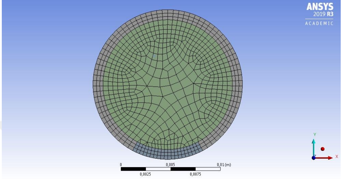
Şekil 4.29. Giriş sınırında boru, akışkan ve ısı transfer bölgesinin eleman bölümü
