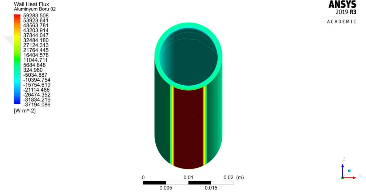
Şekil 4.78. 0.0033 kg/s debi için odak borusu ısı dağılımı
