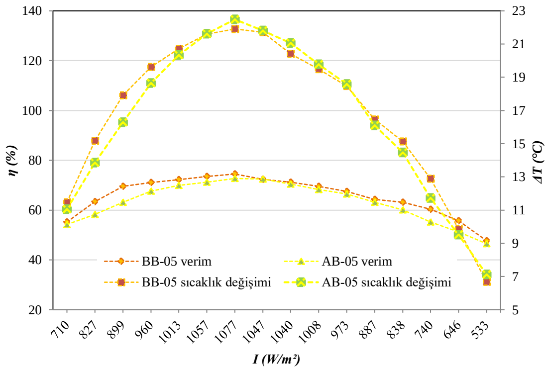
Şekil 4.14. AB-05 ve BB-05 deneylerinde güneş ışınımı ve sıcaklık farkının verime etkisi
