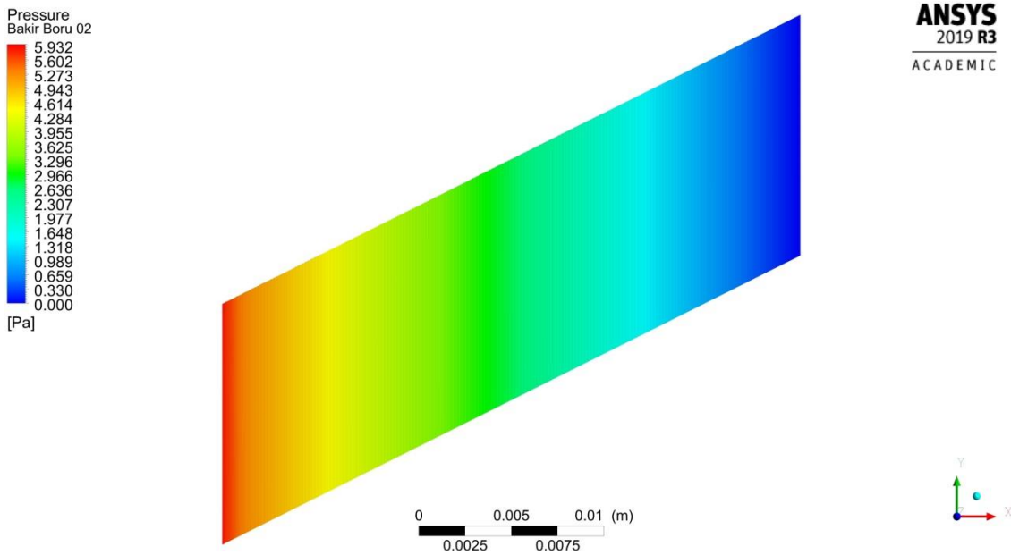
Şekil 4.49. 0.0033 kg/s debide boru merkez çizgisi boyunca kesitin basınç dağılımı
