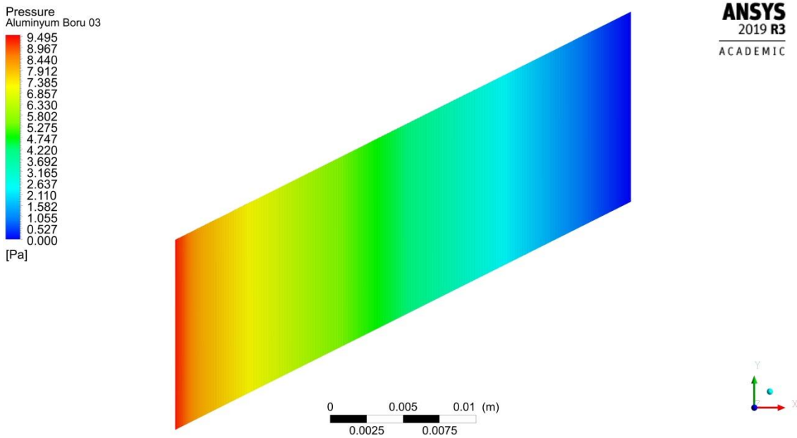
Şekil 4.91. 0.0050 kg/s debide boru merkez çizgisi boyunca kesitin basınç dağılımı
