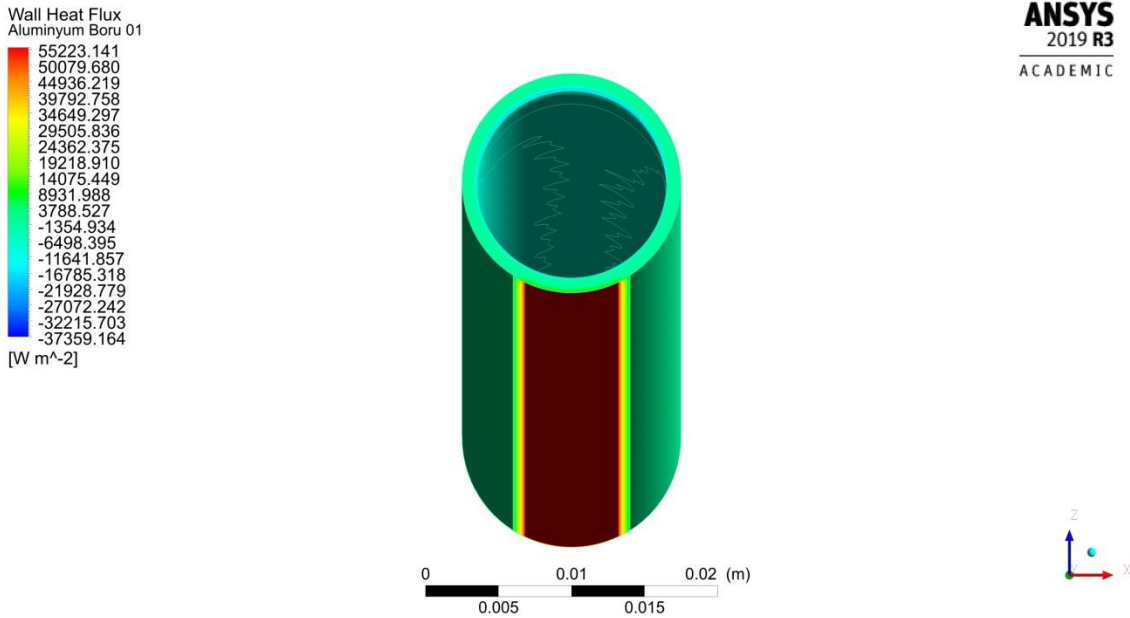
Şekil 4.71. 0.0017 kg/s debi için odak borusu ısı dağılımı
