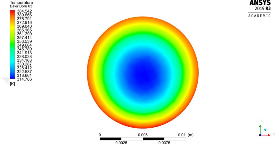
Şekil 4.53. 0.0050 kg/s debide akışkan çıkış sıcaklığı dağılımı
