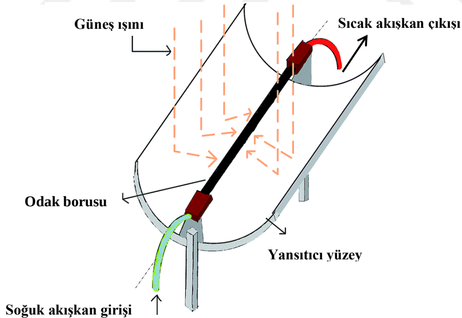
Şekil 1.13. Parabolik oluk güneş kollektörü şematik gösterimi (Dabiri ve Rahimi 2016)
