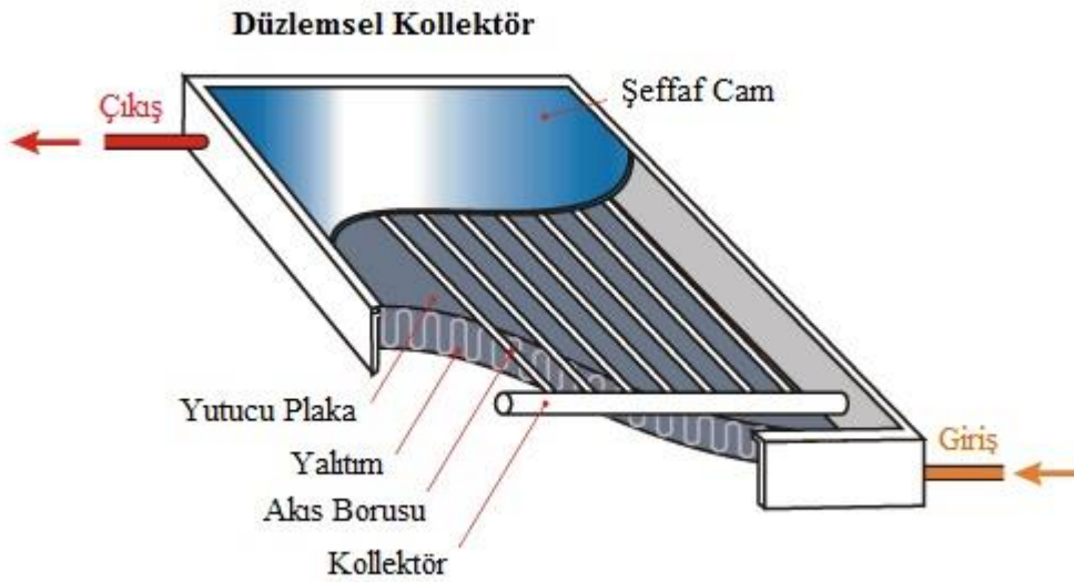
Şekil 1.4. Düzlemsel kollektörün yapısı (SOLAR ADVİCE 2020)
