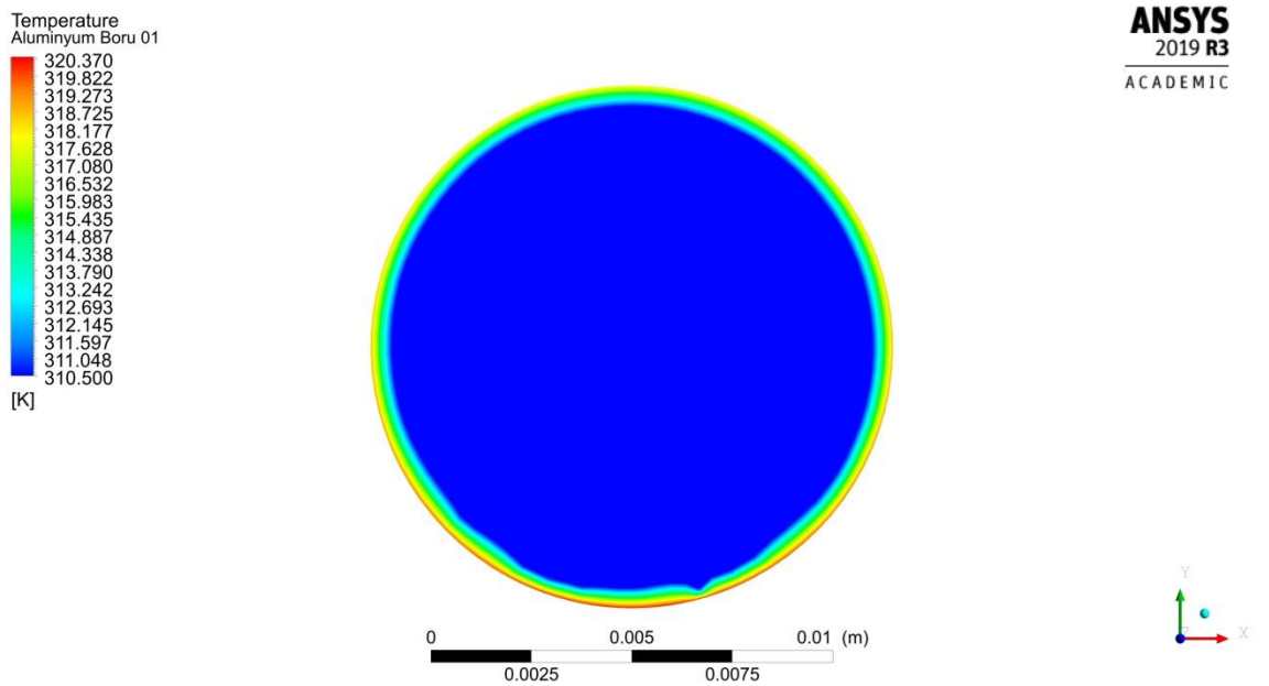
Şekil 4.73. 0.0017 kg/s debide akışkan giriş sıcaklığı dağılımı
