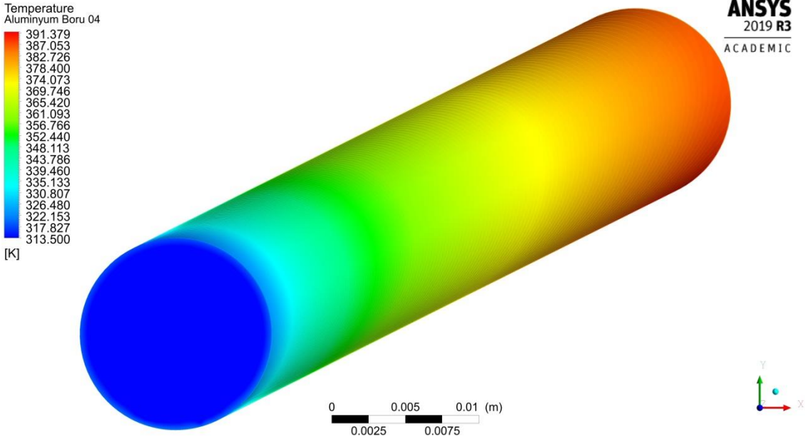
Şekil 4.93. 0.0067 kg/s debide akışkan sıcaklık dağılımı
