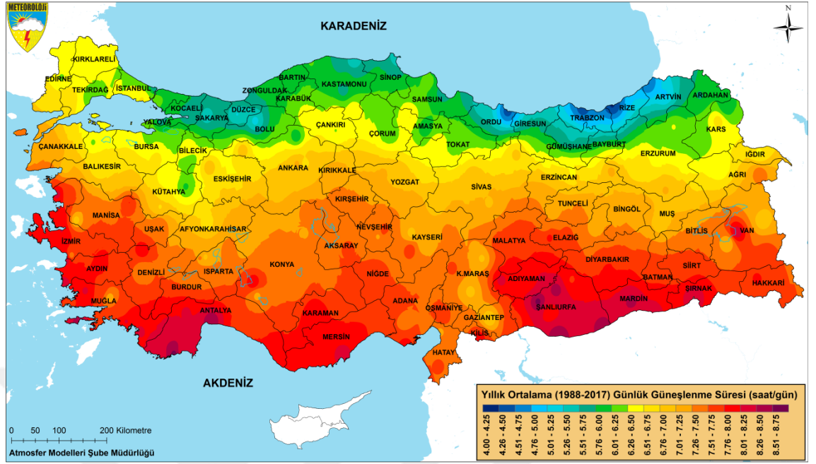
Şekil 1.1. Türkiye’de günlük güneşlenme süresi (saat/gün) (MGM 2017)
