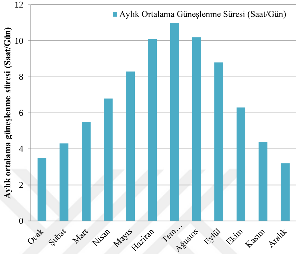
Şekil 1.3. Türkiye’de aylık ortalama güneşlenme süresi (saat/gün) (MGM 2016)
