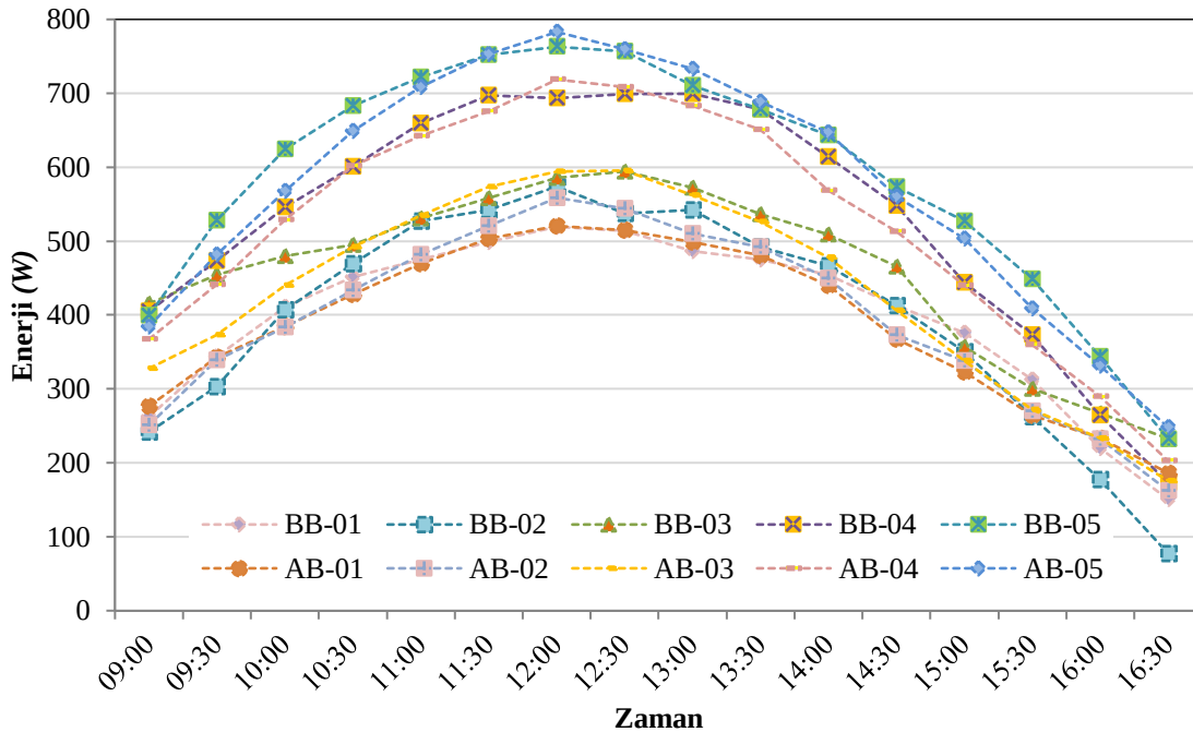
Şekil 4.13. Bakır - Alüminyum suya aktarılan ısı miktarları
