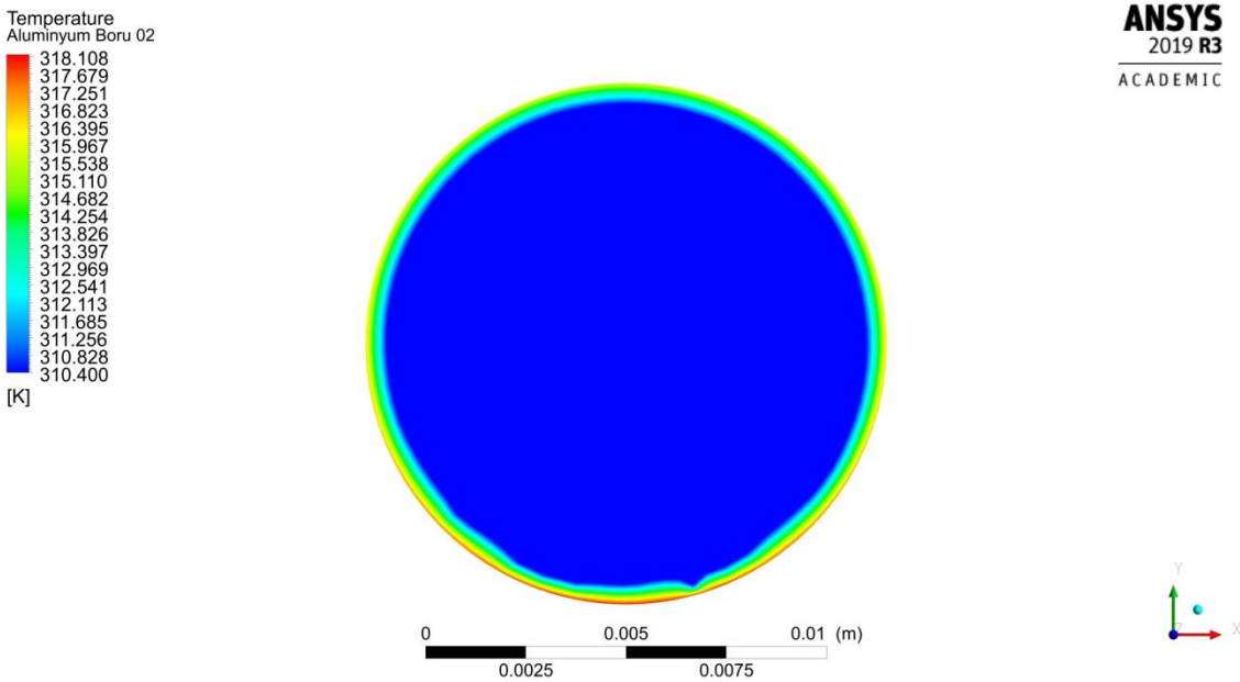
Şekil 4.80. 0.0033 kg/s debide akışkan giriş sıcaklığı dağılımı
