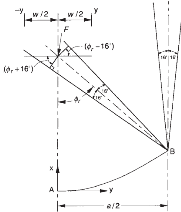
Şekil 3.22. Doğrusal bir yoğunlaştırıcı için görüntü boyutları (Duffie ve Beckman 2005)
