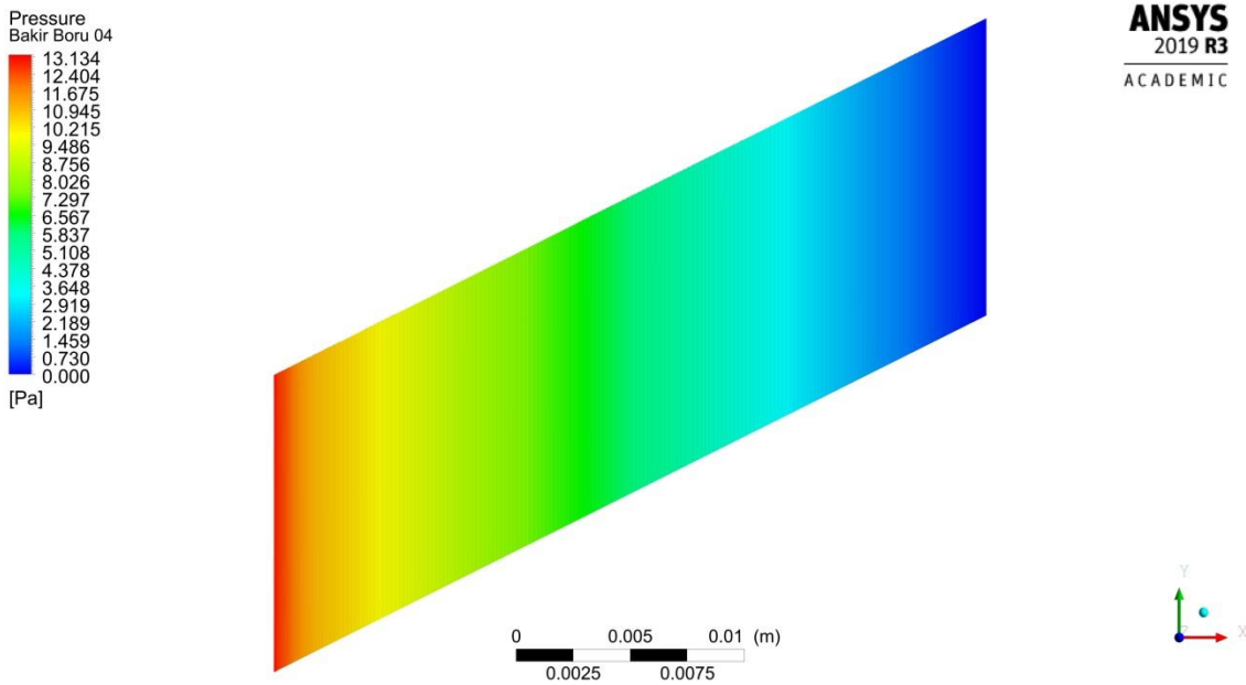
Şekil 4.63. 0.0067 kg/s debide boru merkez çizgisi boyunca kesitin basınç dağılımı
