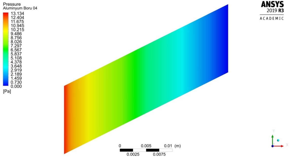
Şekil 4.98. 0.0067 kg/s debide boru merkez çizgisi boyunca kesitin basınç dağılımı
