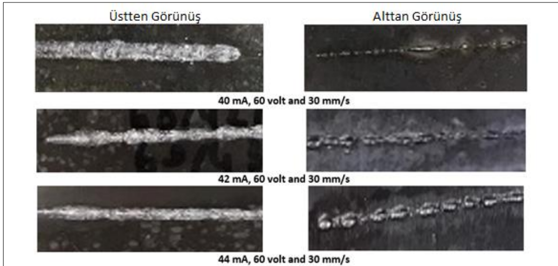
Şekil 7.2. Kaynaklı parçaların üstten ve alttan görünüşü
