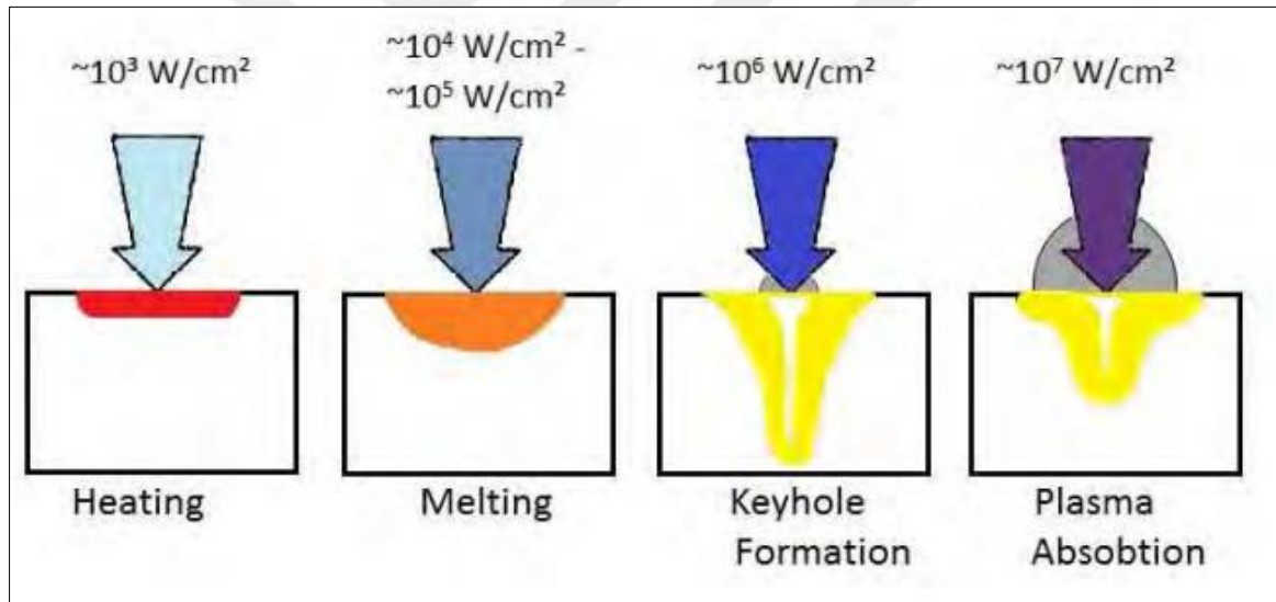
Şekil 3.7. Güç yoğunluğu
