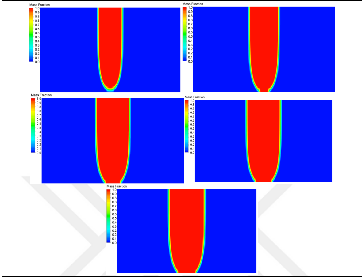
Şekil 7.1. Kaynak parametrelerinden akımın ergime üzerindeki etkisi
