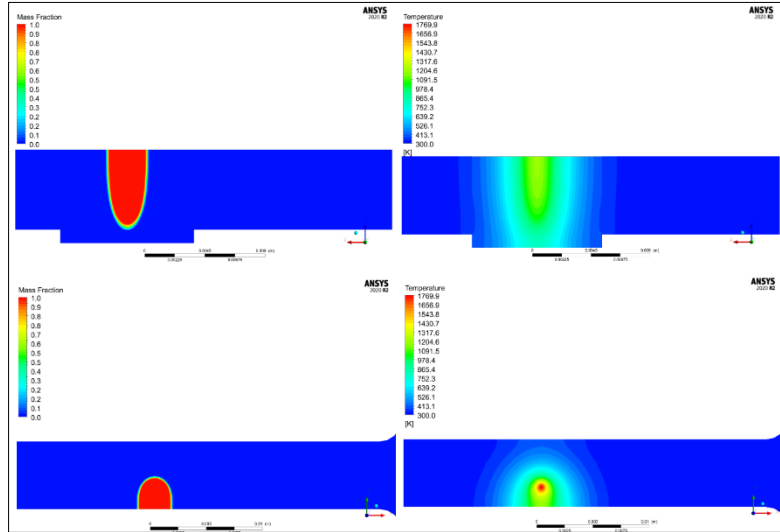
Şekil 5.15. Parametre – 11: 57kV – 40 mA – 30 mm/s
