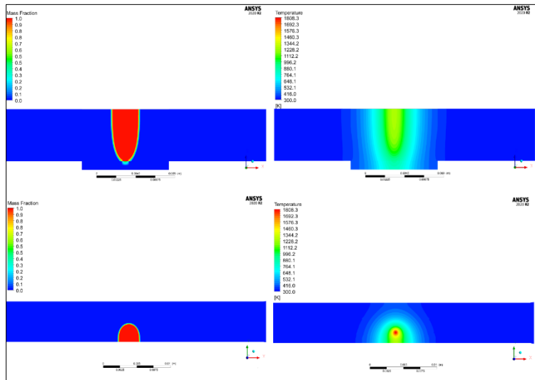
Şekil 5.14. Parametre – 10: 57kV – 40 mA – 27 mm/s
