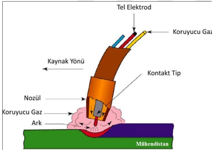
Şekil 2.3. MIG kaynağı şematik gösterimi
