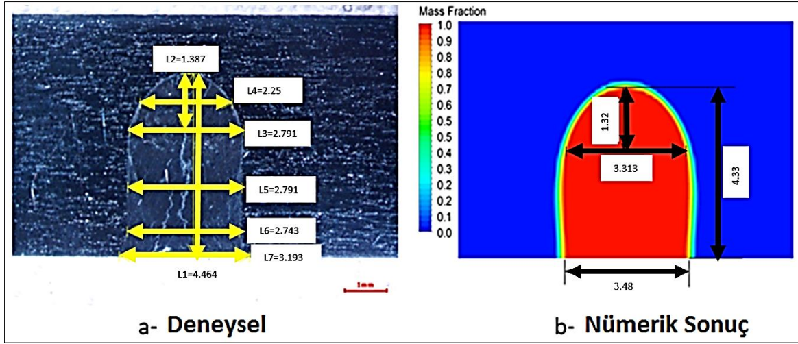
Şekil 5.4. Deneysel ve sayısal sonuçların karşılaştırılması
