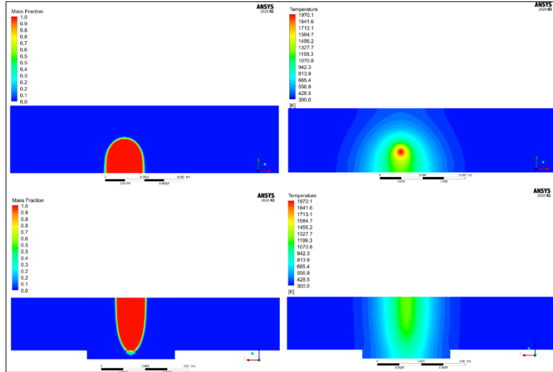
Şekil 5.31. Parametre – 27 60kV – 44 mA – 33 mm/s
