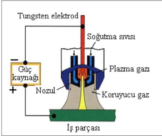
Şekil 2.4. Plazma ark kaynağı şematik gösterişi
