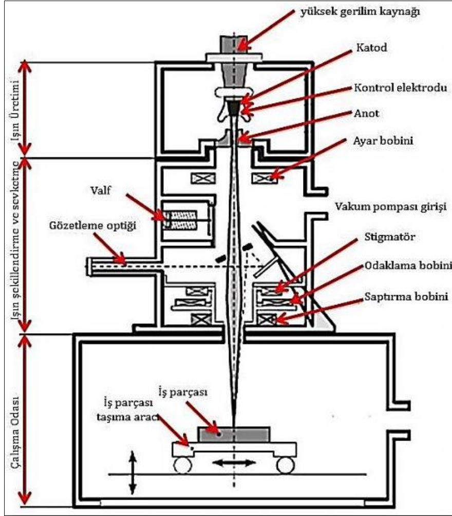
Şekil 3.1. Elektron ışın kaynağı makinesinin şematik gösterimi
