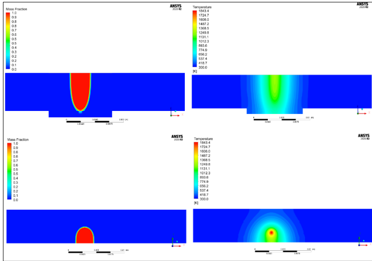
Şekil 5.18. Parametre – 14: 57kV – 42 mA – 30 mm/s
