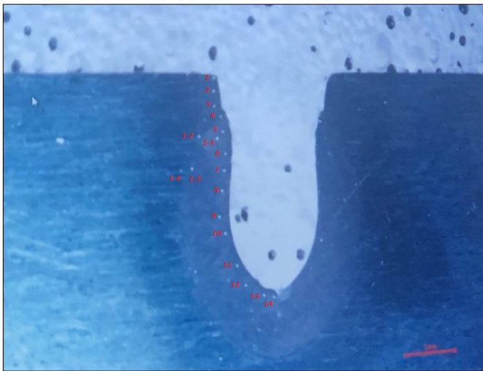
Resim 6.19. Yarım yapılan kaynağın mikroskop altındaki görünüşü
