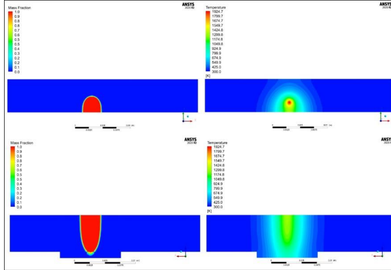
Şekil 5.27. Parametre – 23 60kV – 42 mA – 30 mm/s
