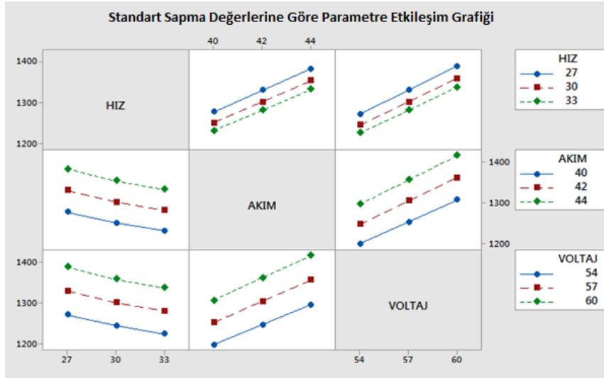
Şekil 5.33. Standart sapma değerlerine göre parametre etkileşim grafiği
