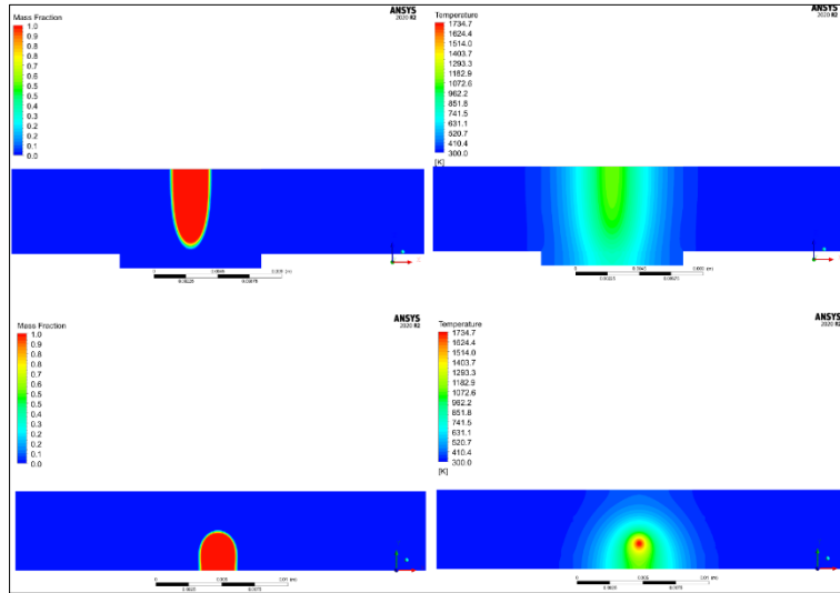
Şekil 5.10. Parametre – 6: 54kV – 42 mA – 33 mm/s
