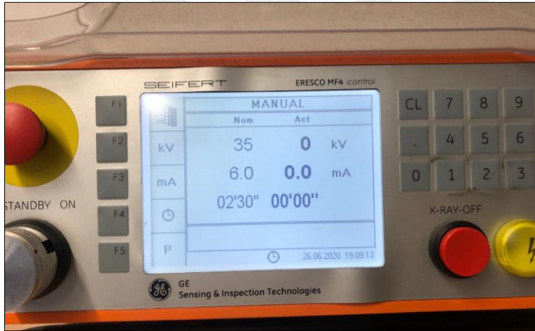
Resim 6.8. Radyografi parametreleri
