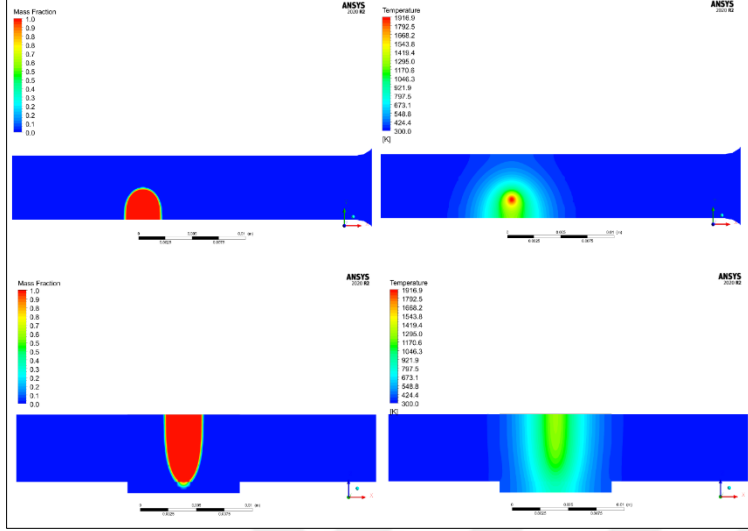
Şekil 5.21. Parametre – 17: 57kV – 44 mA – 30 mm/s
