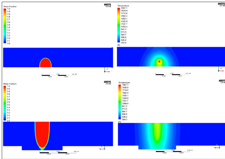
Şekil 5.26. Parametre – 22 60kV – 42 mA – 27 mm/s
