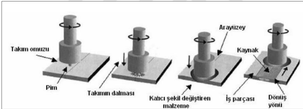
Şekil 2.6. Sürtünme kaynağının işlem sıralamaları
