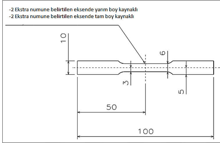
Şekil 6.3. Ekstra numunelerdeki kaynak yönleri
