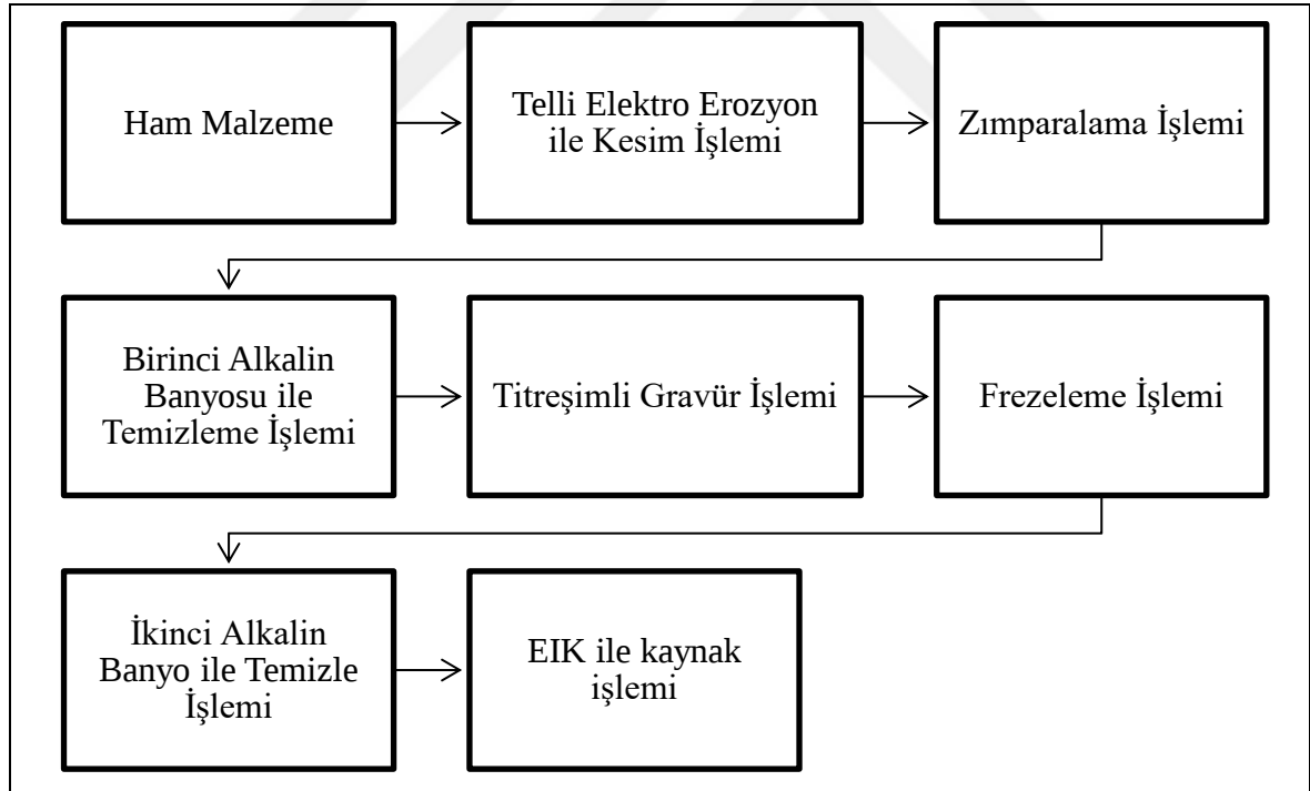
Şekil 6.2. Numune üretim süreci
