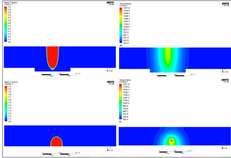
Şekil 5.11. Parametre – 7: 54kV – 44 mA – 27 mm/s
