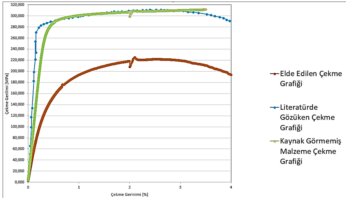
Şekil 6.7. En iyi parametre çekme sonuçları
