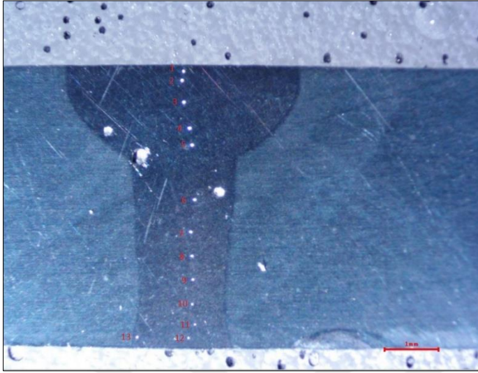
Resim 6.20. Tam yapılan kaynağın mikroskop altındaki görünüşü
