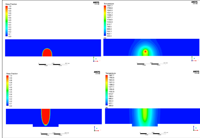
Şekil 5.23. Parametre – 19: 60kV – 40 mA – 27 mm/s
