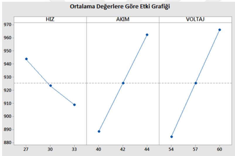
Şekil 5.34. Ortalama değerle göre etki grafiği
