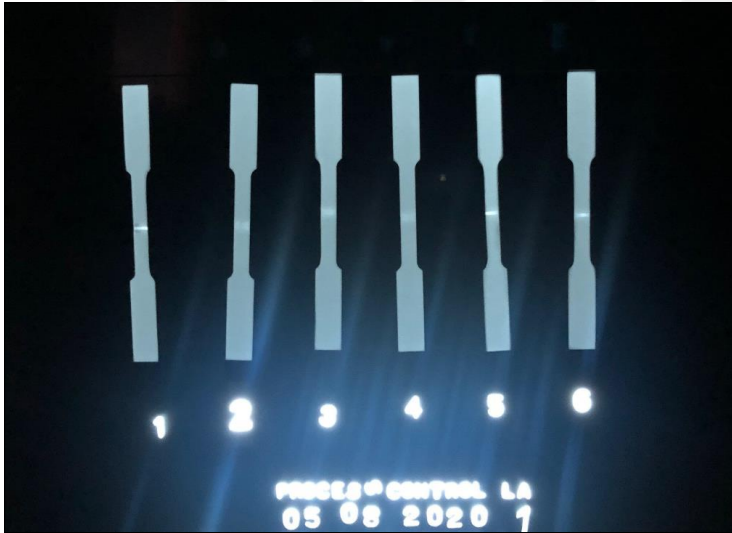
Resim 6.13. En iyi parametrelerin tek çekildiği radyografi sonucu
