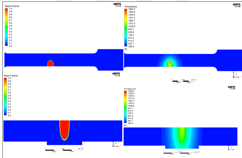
Şekil 5.6. Parametre – 2: 54kV – 40 mA – 30 mm/s
