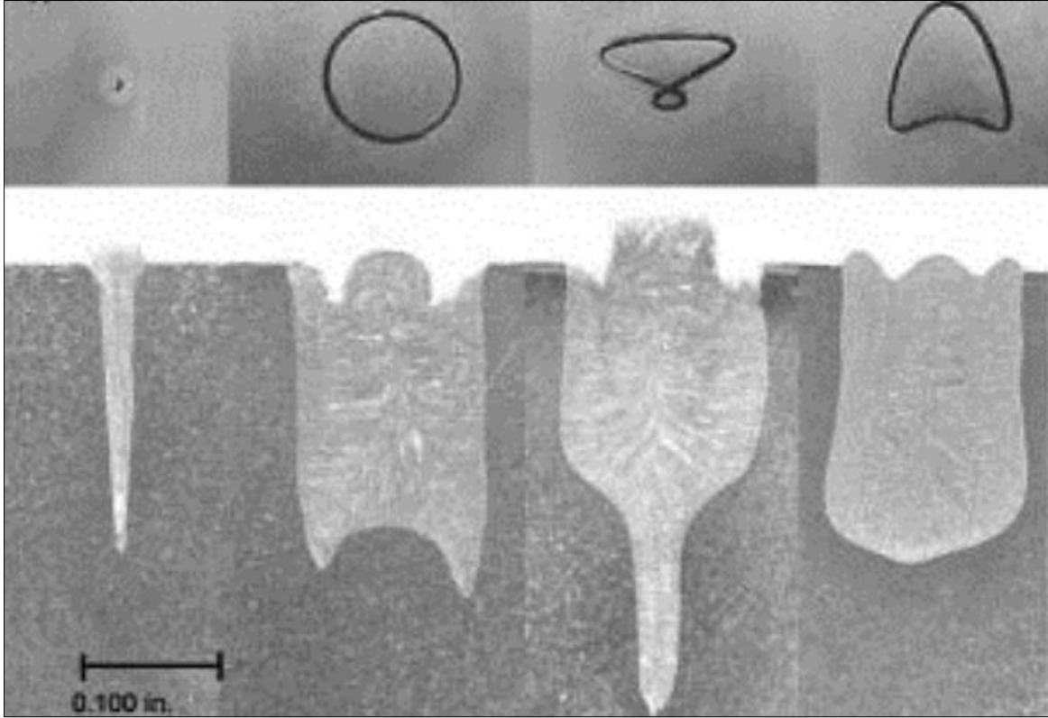
Şekil 3.6. Osilasyon tipleri - kesitten görünümü
