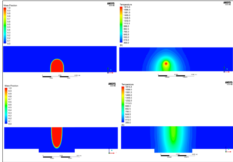
Şekil 5.19. Parametre – 15: 57kV – 42 mA – 33 mm/s
