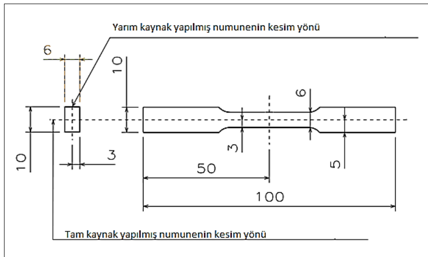
Şekil 6.4. Ekstra örneklerin kesim eksenleri
