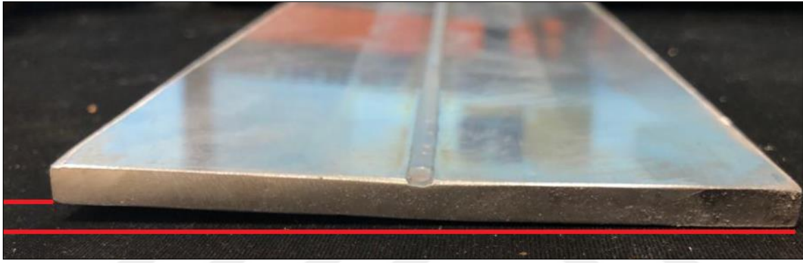
Resim 5.2. Fazla enerji kullanımında düzlemselliğin kaybolmasına örnek
