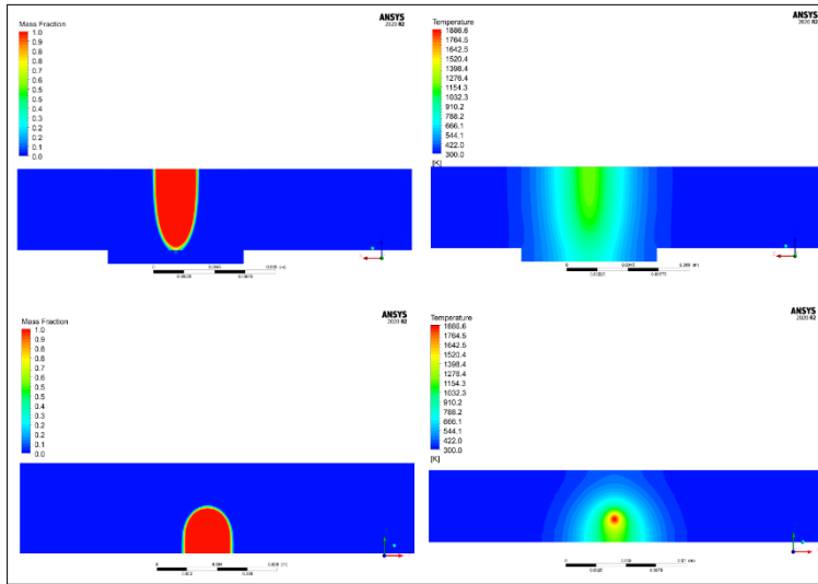
Şekil 5.22. Parametre – 18: 57kV – 44 mA – 33 mm/s
