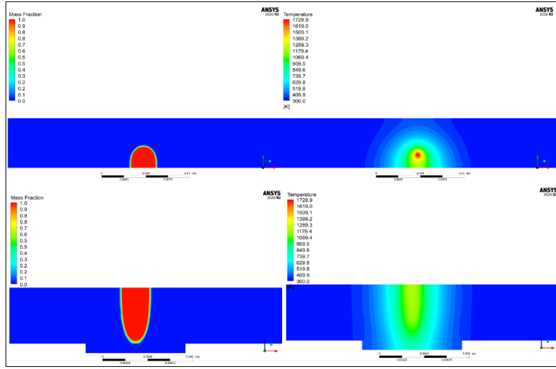
Şekil 5.5. Parametre – 1: 54 kV - 40 mA - 27 mm/s
