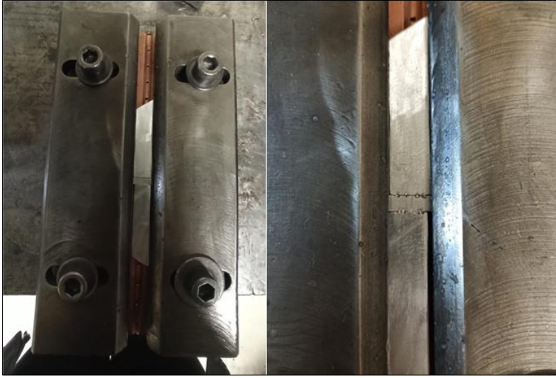
Resim 6.6. Kullanılan mengene ve numunenin mengenedeki görünüşü
