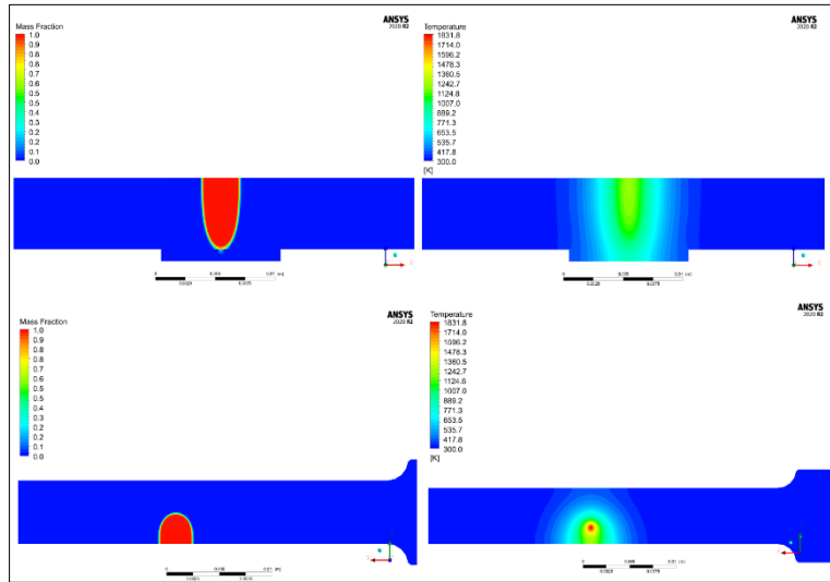
Şekil 5.12. Parametre – 8: 54kV – 44 mA – 30 mm/s
