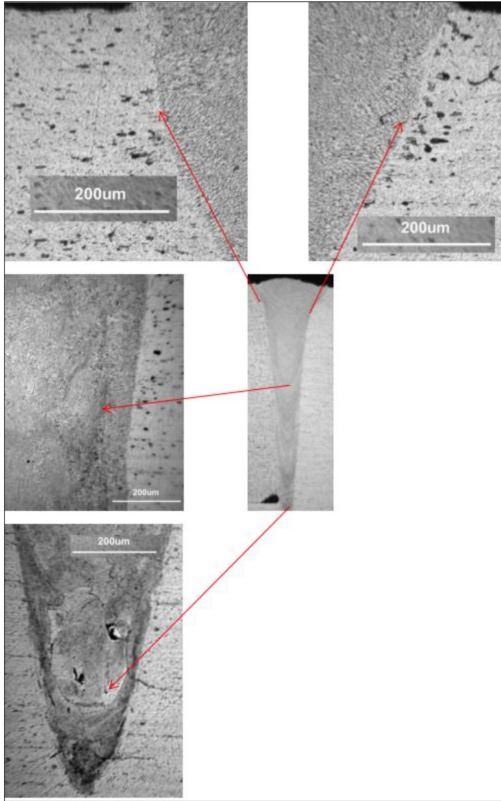
Resim 5.3. Örnek anahtar deliği şeklindeki kaynak görseli
