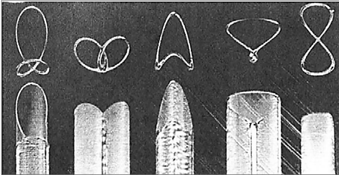
Şekil 3.5. Osilasyon tipleri - üstten görünüm
