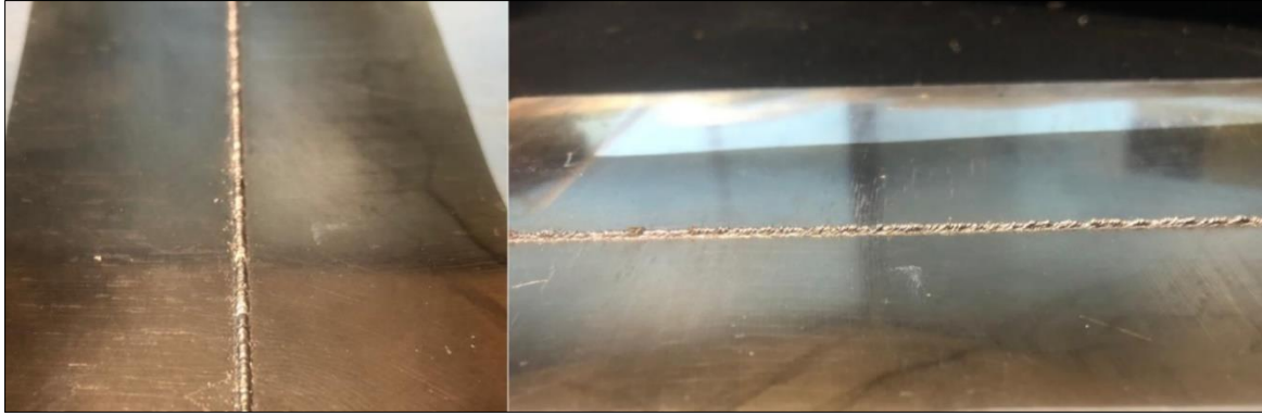
Resim 5.1. Fazla enerji kullanımında çentik etkisi yaratılmasına örnek
