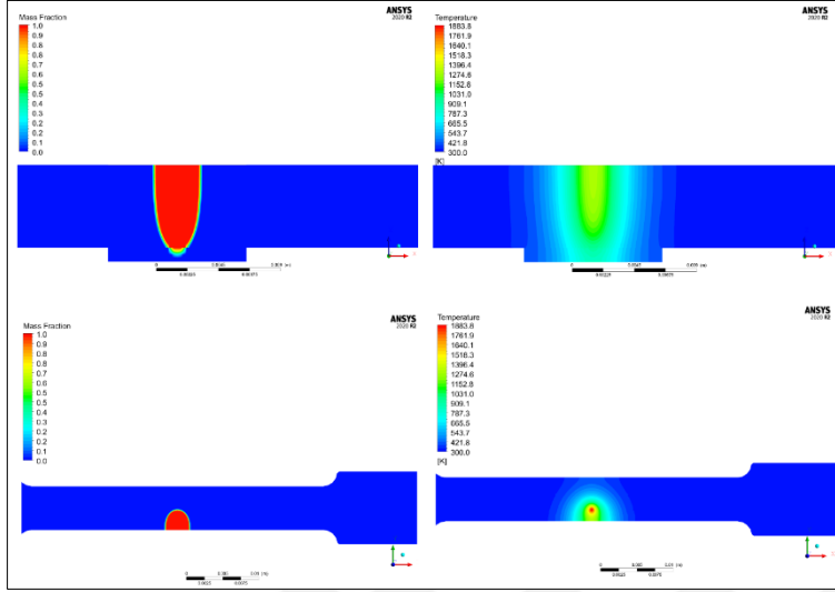
Şekil 5.17. Parametre – 13: 57kV – 42 mA – 27 mm/s
