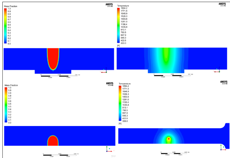
Şekil 5.28. Parametre – 24 60kV – 42 mA – 33 mm/s
