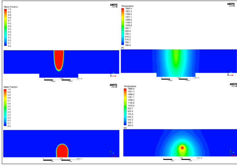
Şekil 5.7. Parametre – 3: 54kV – 40 mA – 33 mm/s
