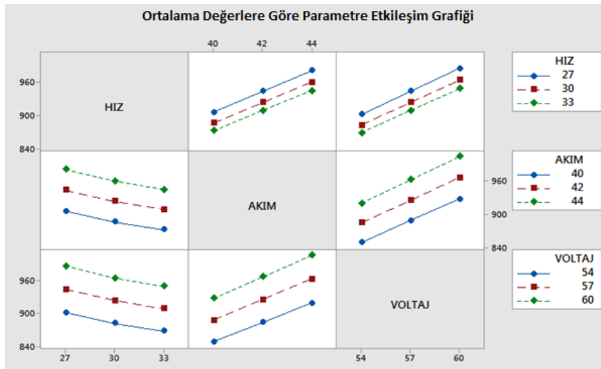
Şekil 5.32. Ortalama değerlere göre parametre etkileşim grafiği
