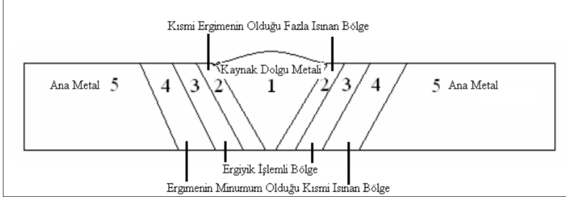
Şekil 2.1. Kaynaklı parçalardaki ısı bölgeleri
