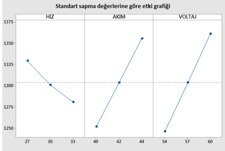
Şekil 5.35. Standart sapma değerlerine göre etki grafiği
