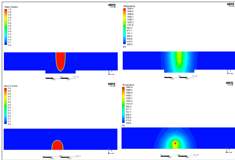
Şekil 5.8. Parametre – 4: 54kV – 42 mA – 27 mm/s
