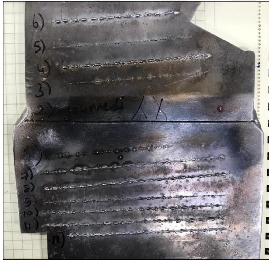
Resim 6.5. Levha denemeleri arkadan görünüş
