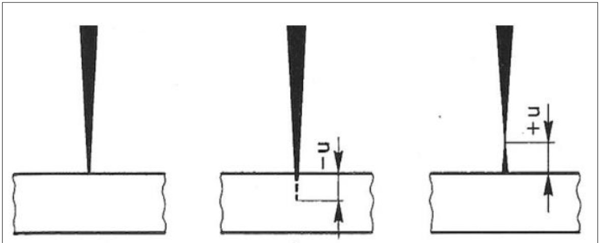
Şekil 3.4. Farklı odak konumları
