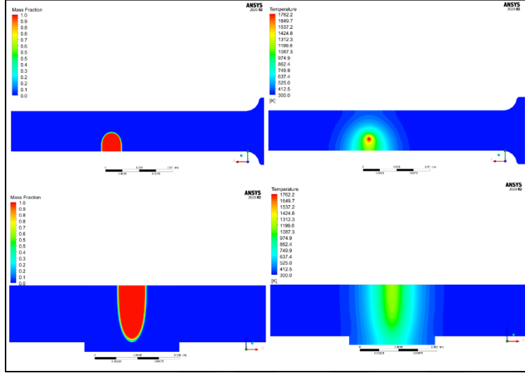
Şekil 5.9. Parametre – 5: 54kV – 42 mA – 30 mm/s
