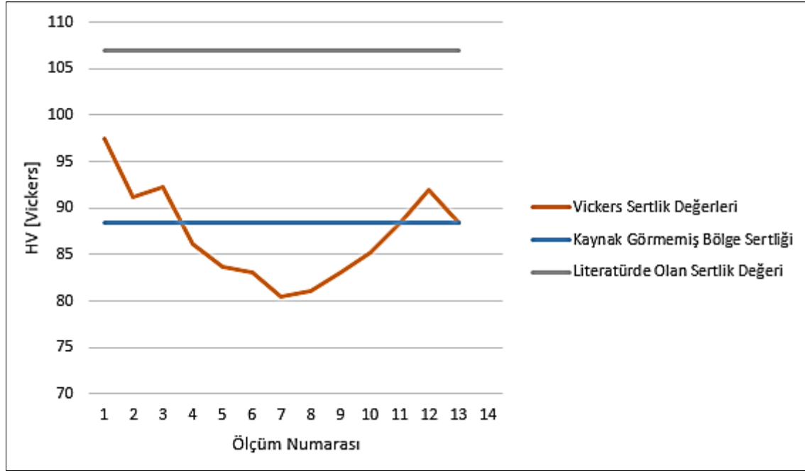
Şekil 6.6. Tam kaynak yapılan numune üzerindeki noktadaki sertlik değerleri grafiği
