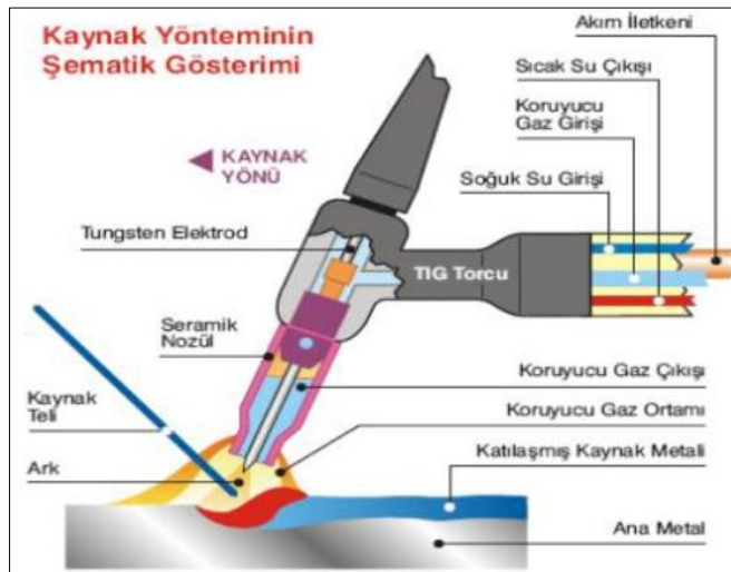
Şekil 2.2. TIG kaynağı şematik gösterimi
