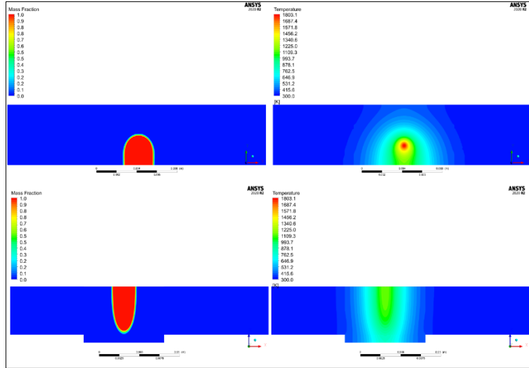
Şekil 5.13. Parametre – 9: 54kV – 44 mA – 33 mm/s
