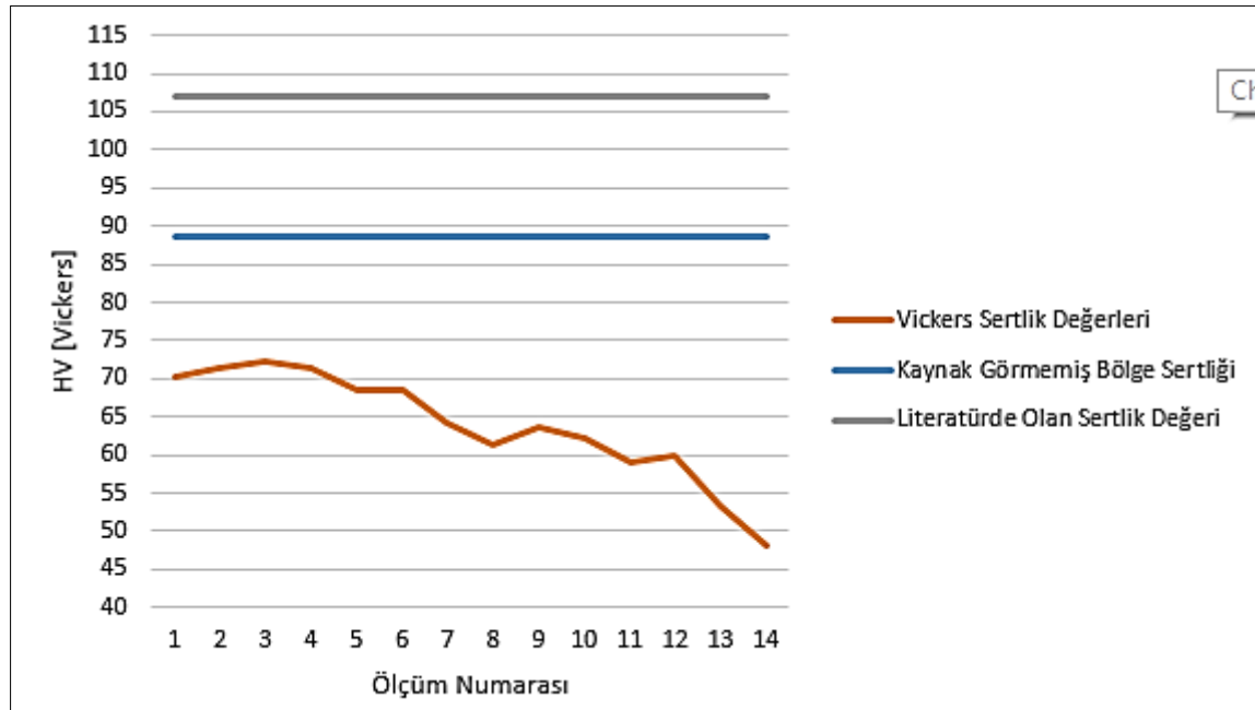
Şekil 6.5. Yarım kaynak yapılan numune üzerindeki noktalardaki sertlik değerleri grafiği
