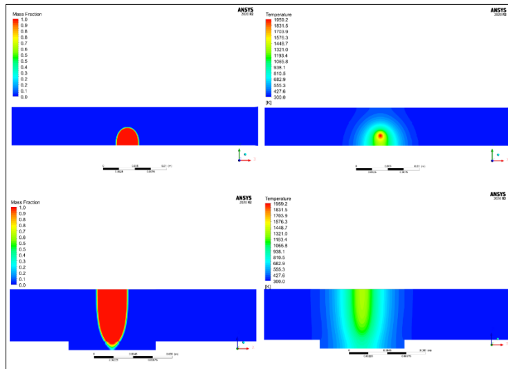
Şekil 5.20. Parametre – 16: 57kV – 44 mA – 27 mm/s
