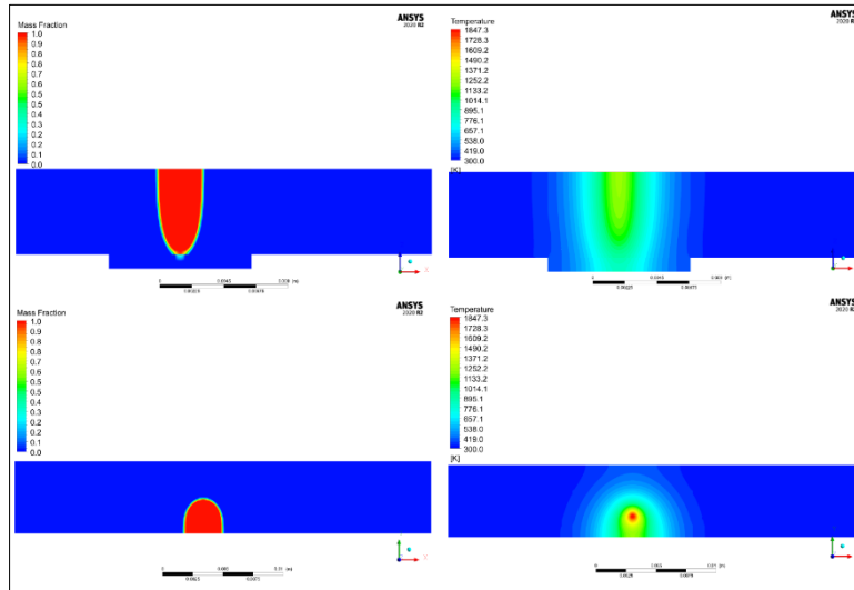
Şekil 5.24. Parametre – 20: 60kV – 40 mA – 30 mm/s
