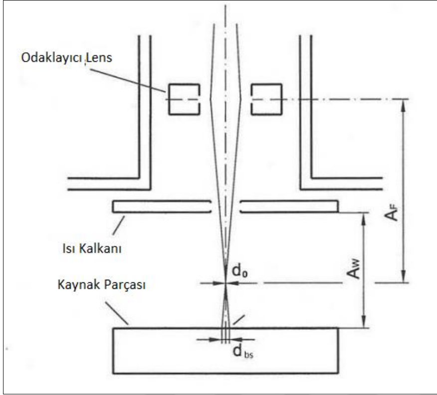
Şekil 3.3. Odak mesafesi ve konumu
