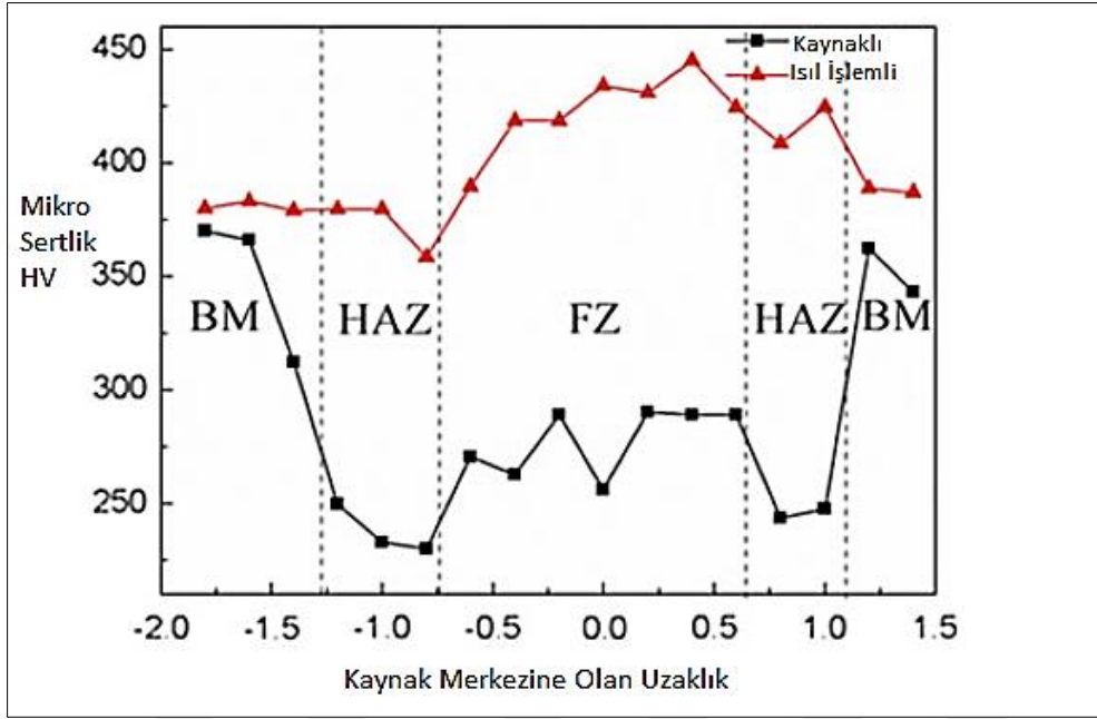
Şekil 4.1. Kaynak merkezine olan uzaklığa göre sertlik değişimi
