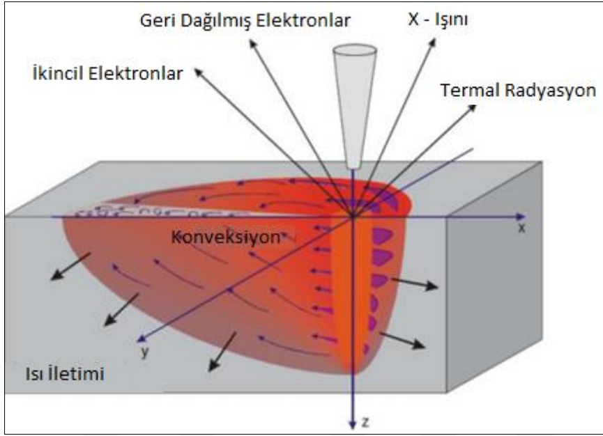
Şekil 3.2. İş parçası içinde elektron ışınının enerji dönüşümü
