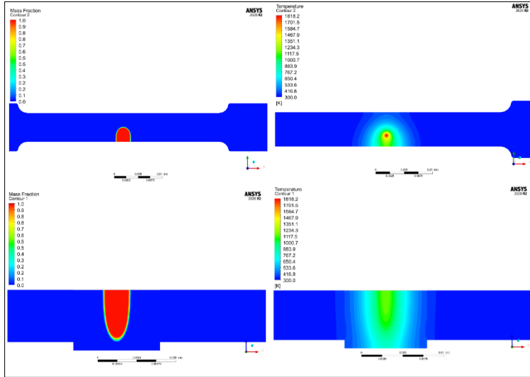
Şekil 5.25. Parametre – 21 60kV – 40 mA – 33 mm/s
