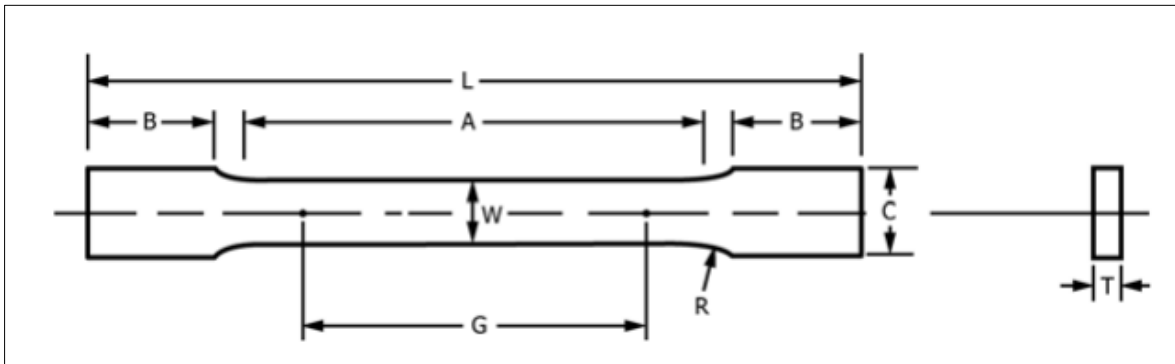
Şekil 6.1. ASTM E8/E8M – 16a düz tip numune boyutlandırma
