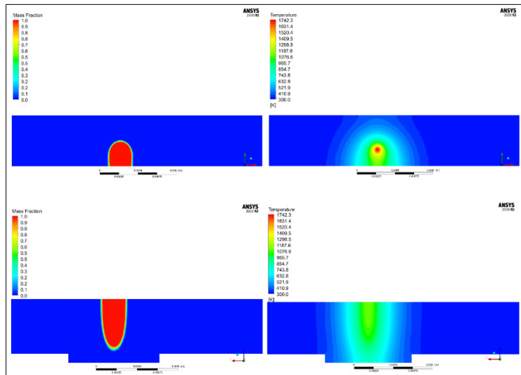
Şekil 5.16. Parametre – 12: 57kV – 40 mA – 33 mm/s
