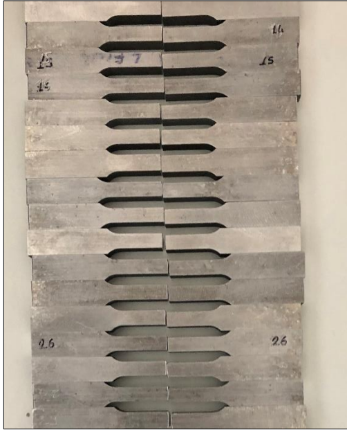
Resim 6.3. Freze işlemi sonrası numunelerin görünüşü
