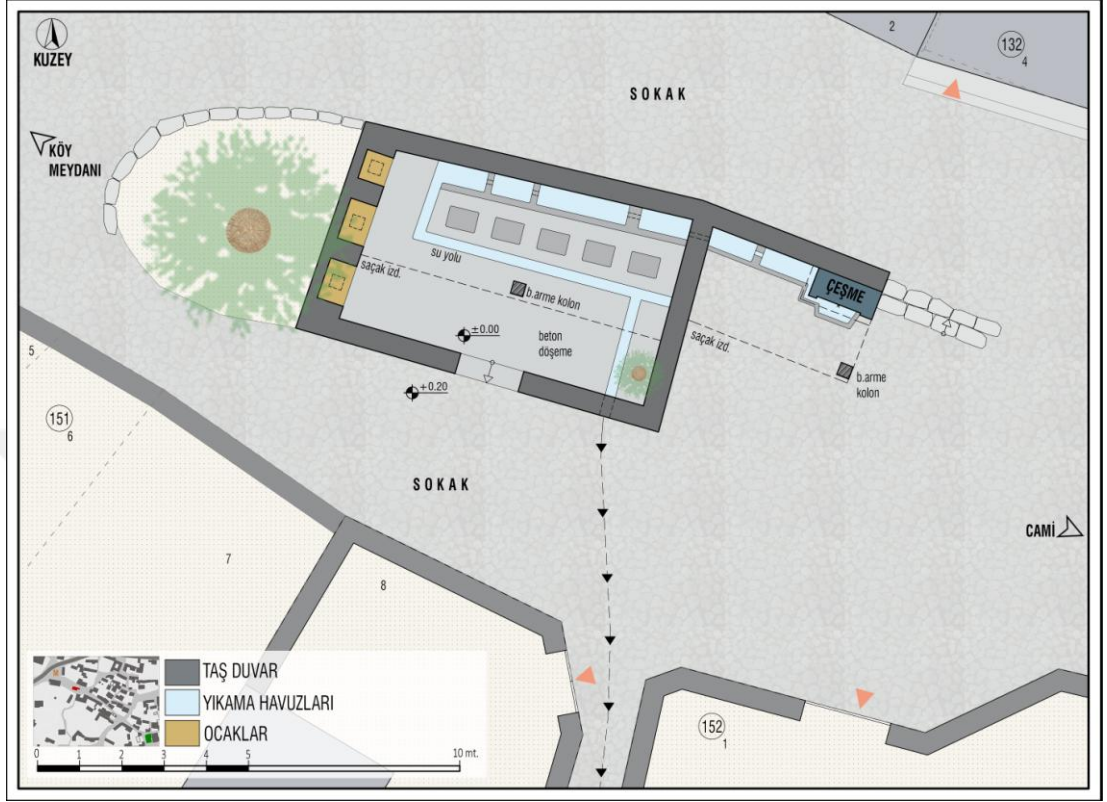
Şekil 4.21 : 159 Ada 1 Parselde Yer Alan Çamaşırhane Planı Rölövesi, 2019
