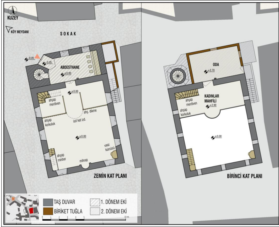
Şekil 4.31 : 168 Ada 1 Parselde Yer Alan Cami Planı
