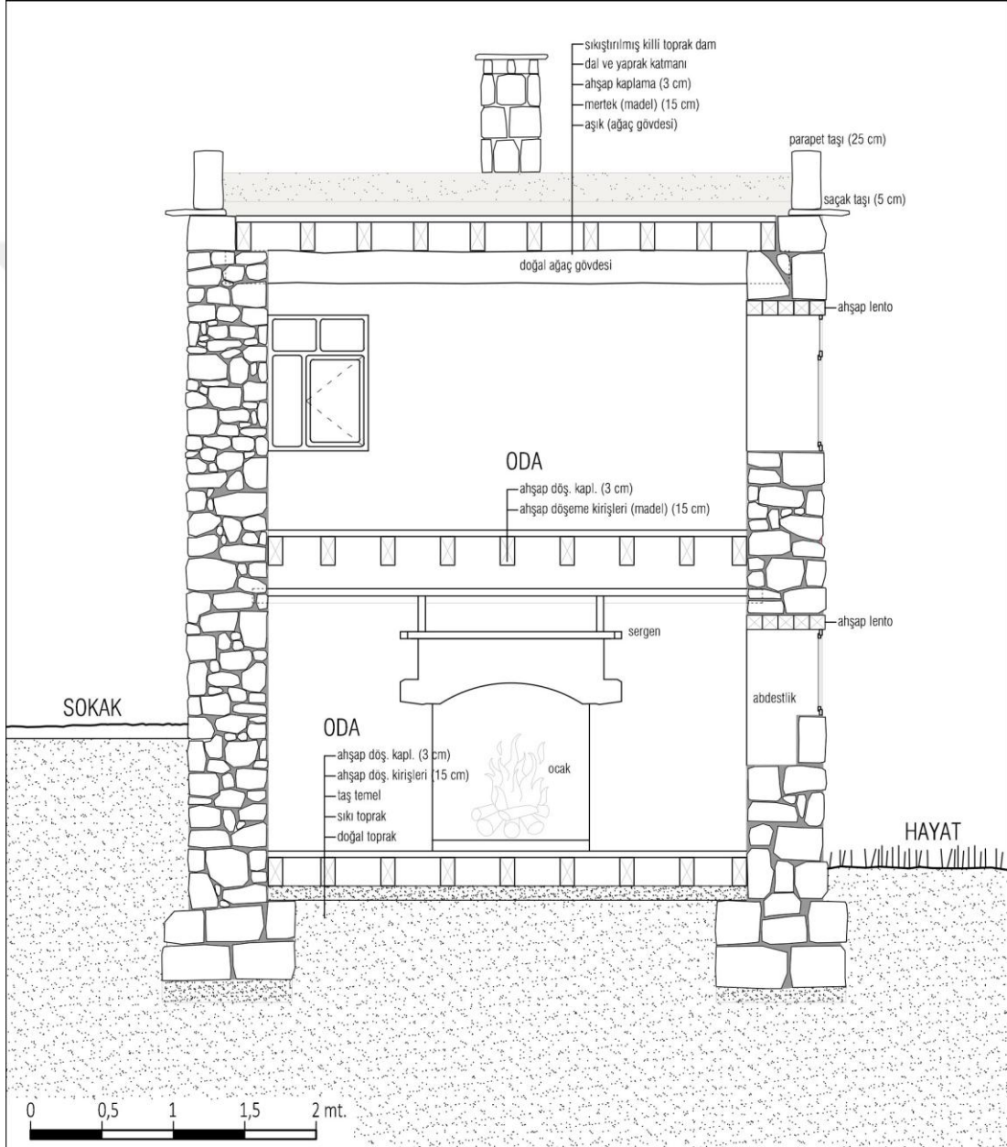
Şekil 4.70: Geleneksel Bir Yapının Kesiti
