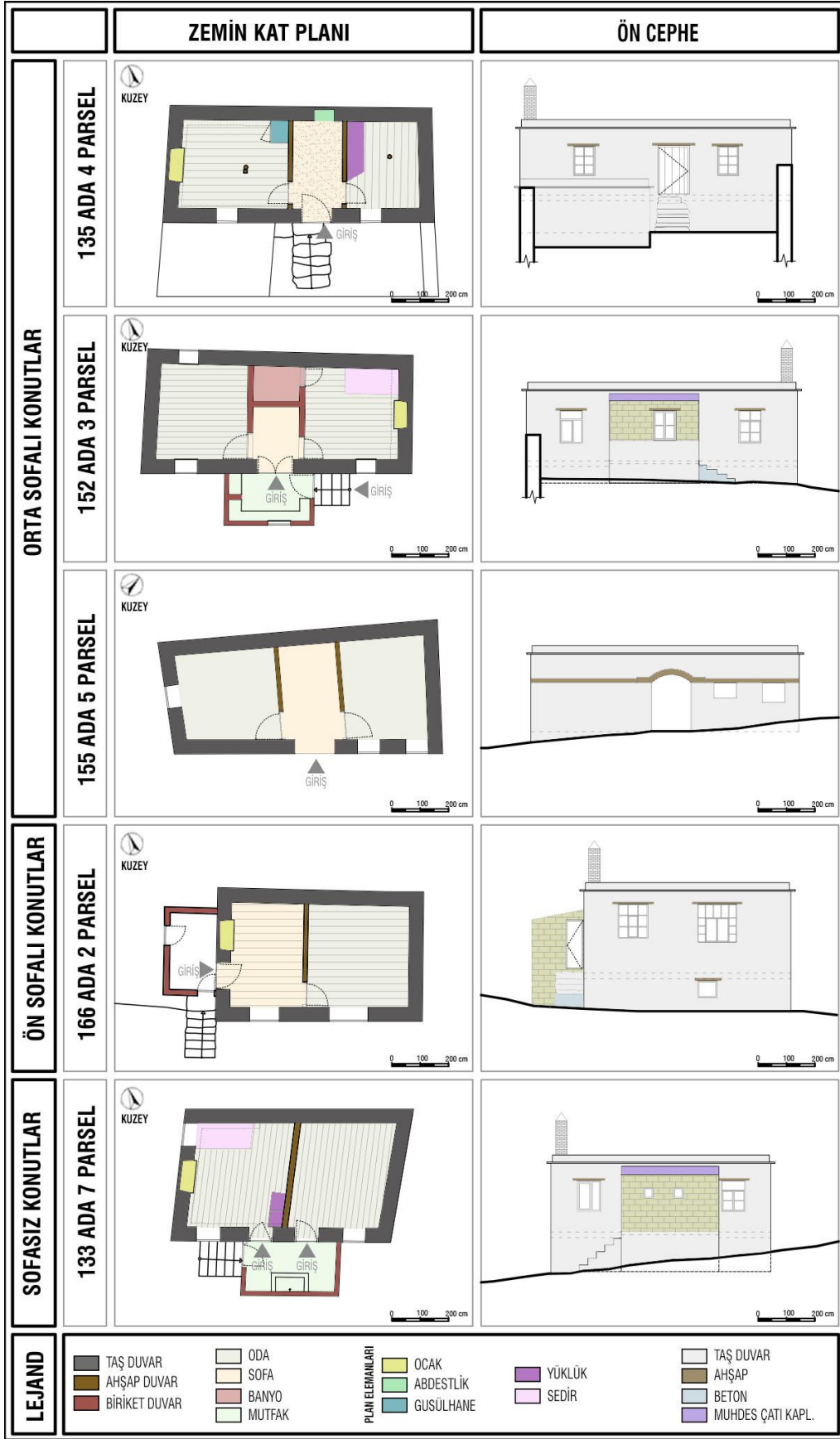
Şekil 4.50: Tek Katlı Geleneksel Konutlarda Plan Tipolojileri
