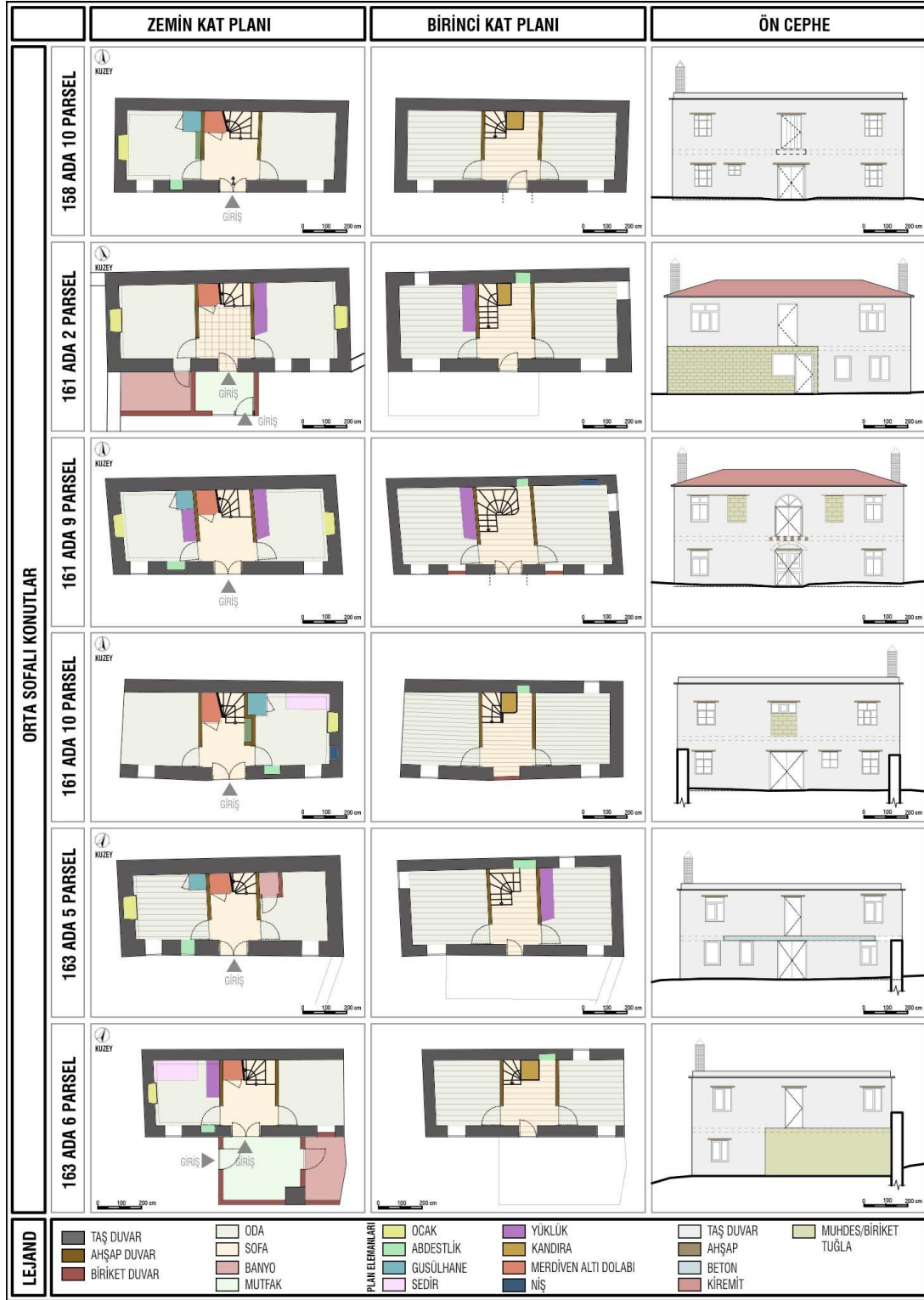
Şekil 4.48: İki Katlı Geleneksel Konutlarda Plan Tipolojileri
