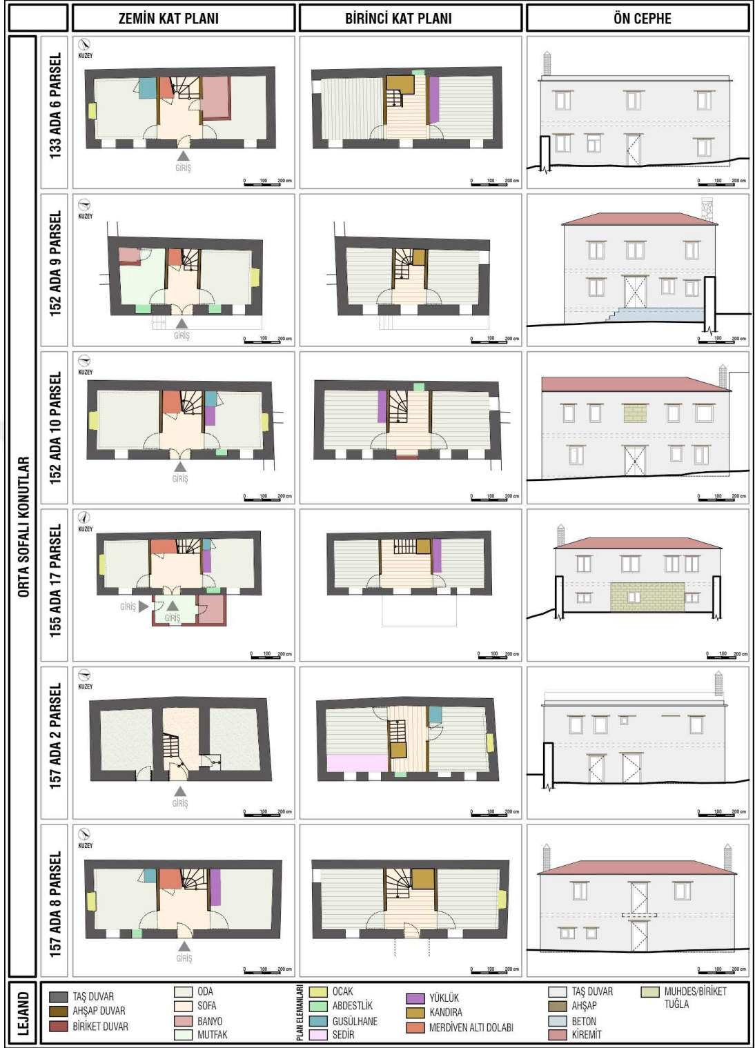
Şekil 4.47: İki Katlı Geleneksel Konutlarda Plan Tipolojileri
