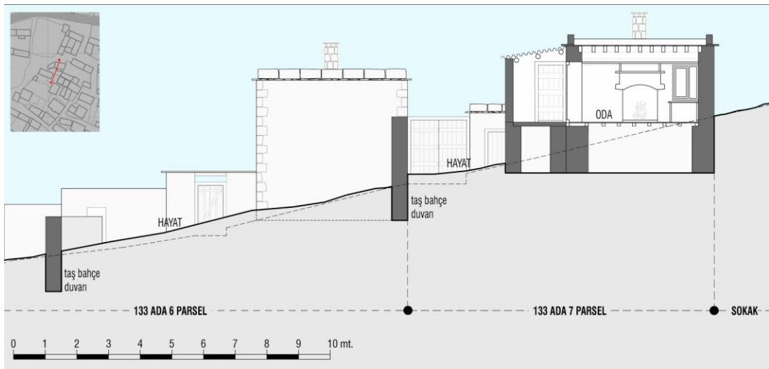
Şekil 4.9: Yerleşimde Bulunan Komşu İki Evin Topografyada Konumlanışı
