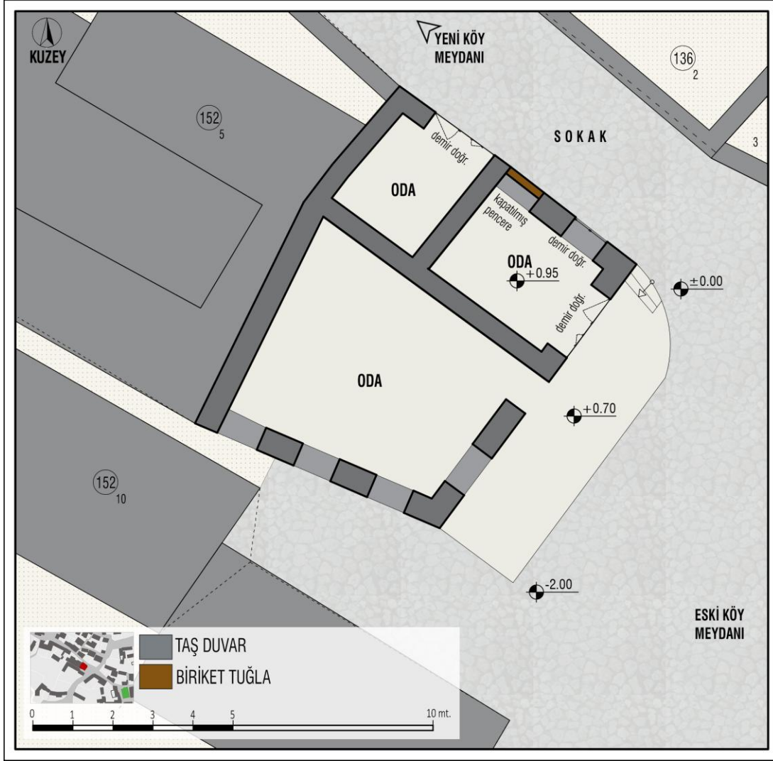
Şekil 4.28 : Eski Kahvehane Planı Rölövesi, 2019
