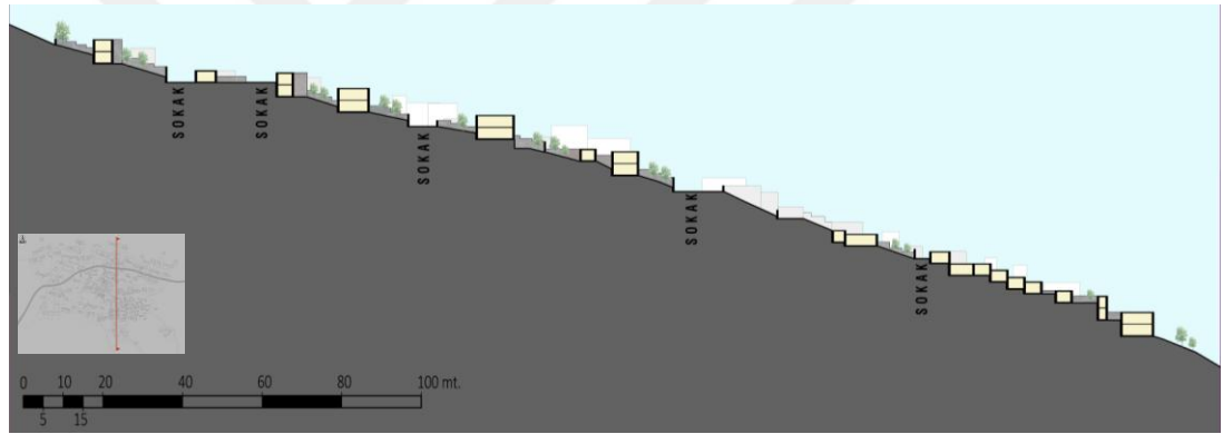
Şekil 4.8: Yapıların Arazideki Konumları Şeması
