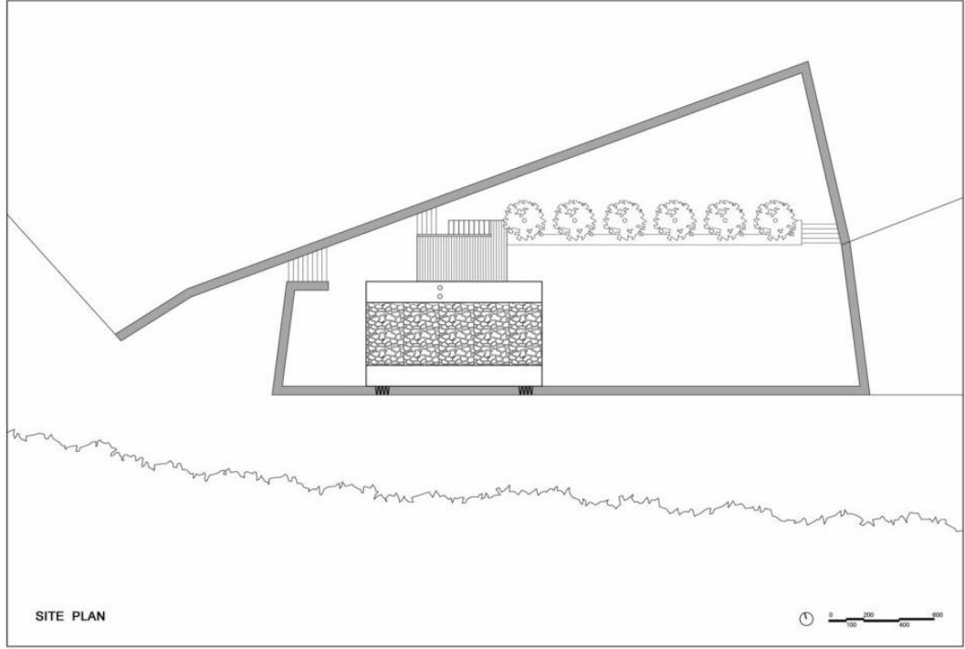
Şekil 4.92: B2 Evi Vaziyet Planı (URL-12)
