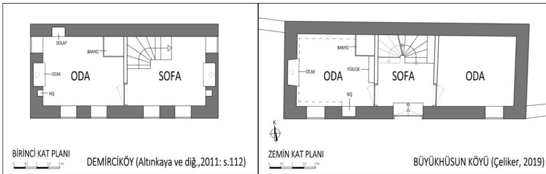
Şekil 4.82: Demirciköy ve Büyükhüsün Köyü Evlerinin Ortak Plan Elemanları
