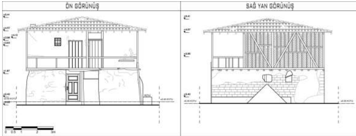
Şekil 4.43. 10 numaralı Alaçık meskeninin Güneydoğu ve Kuzeydoğu cephesi
