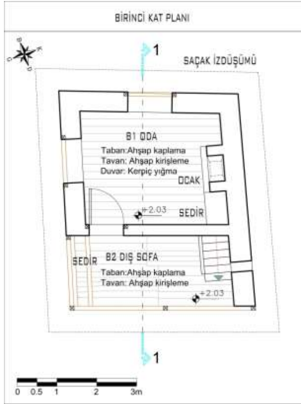
Şekil 4.2. 1 numaralı bağ evinin birinci kat planı
