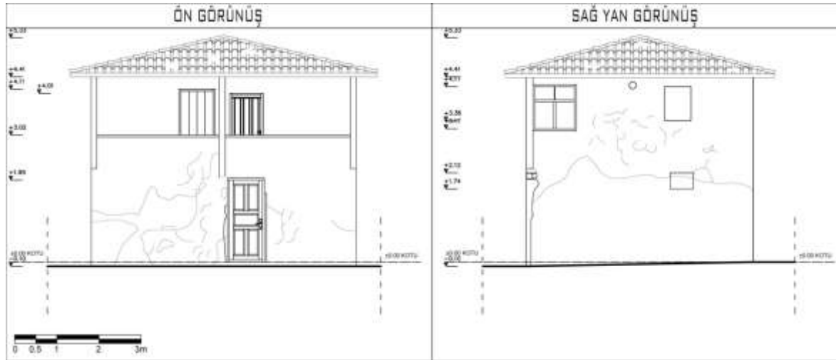
Şekil 4.57. 13 numaralı Alaçık meskeninin Güneydoğu ve Kuzeydoğu cephesi
