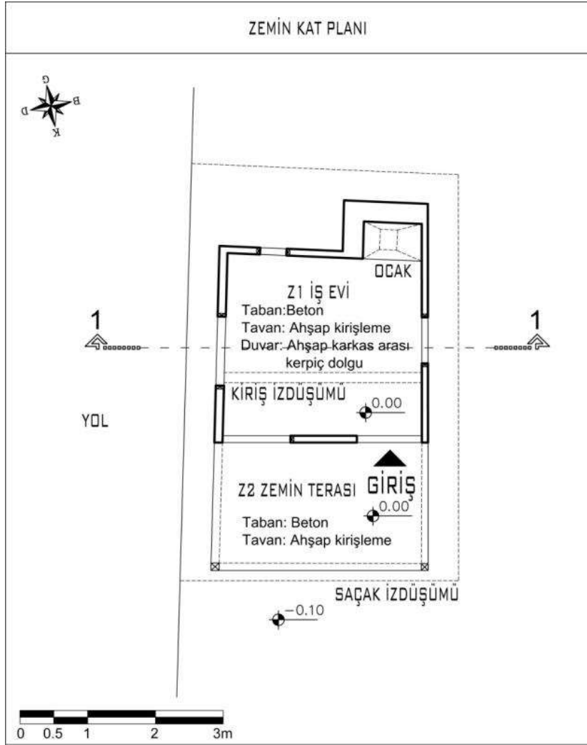
Şekil 4.30. 7 numaralı Gümelenin zemin kat planı
