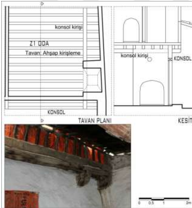
Şekil 5.18. Alpak ailesi Alaçık meskeni; döşeme kirişleri dışarı çıkan konsol detayı (Bkz. Katalog 17)
