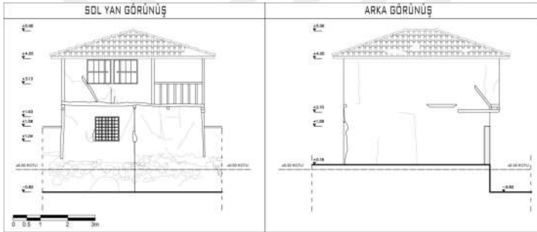
Şekil 4.9. 2 numaralı Gümelenin Kuzeydoğu ve Güneydoğu cephesi
