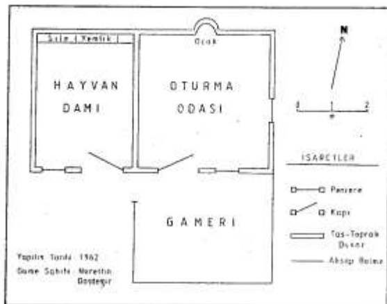
Şekil 3.7. Eski Gediz Kasabası'nda tek katlı güme planı örneği (sayfa 182) [34]
