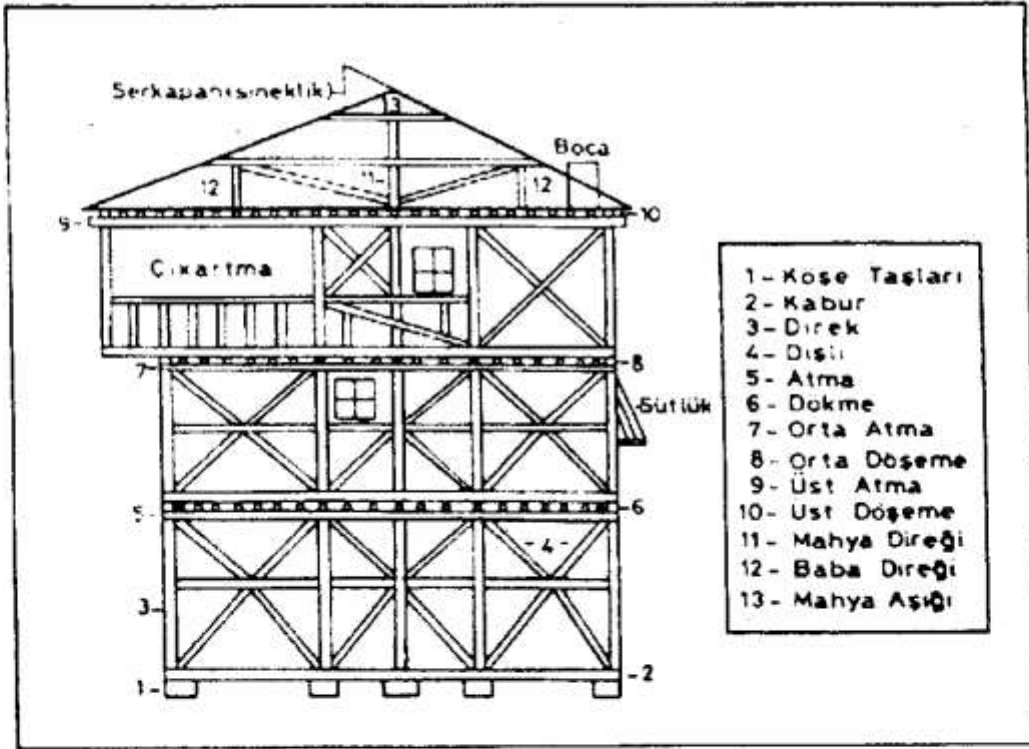
Şekil 3.3. Tosya çevresindeki örnek bir Gümelenin karkas sistemi (sayfa 17) [30]
