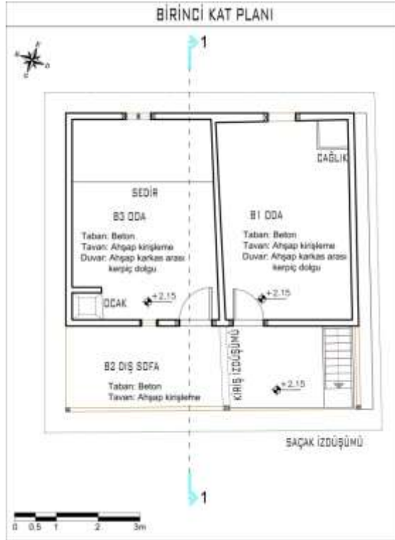
Şekil 4.42. 10 numaralı Alaçık meskeninin birinci kat planı
