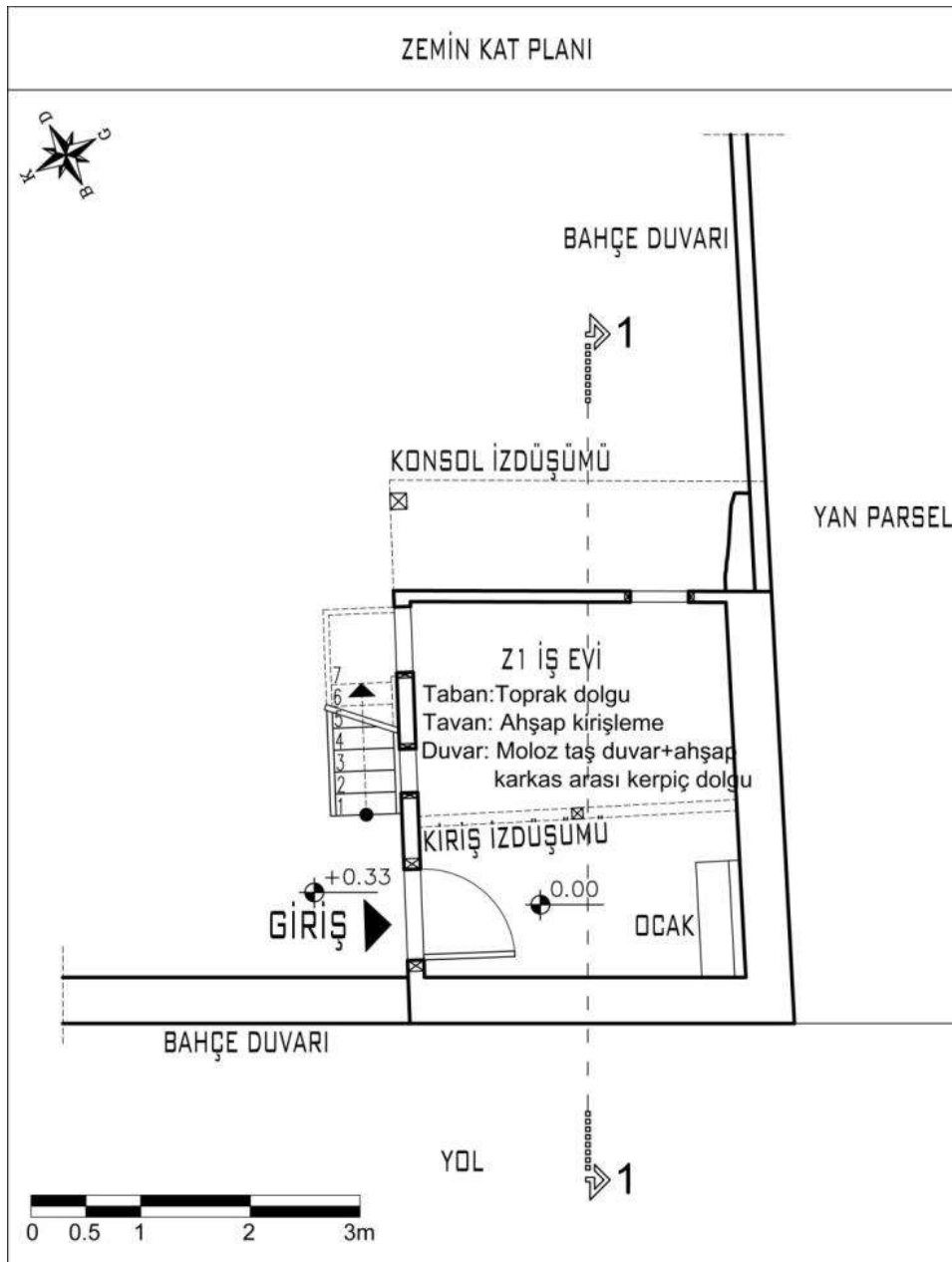
Şekil 4.16. 4 numaralı Gümelenin zemin kat planı
