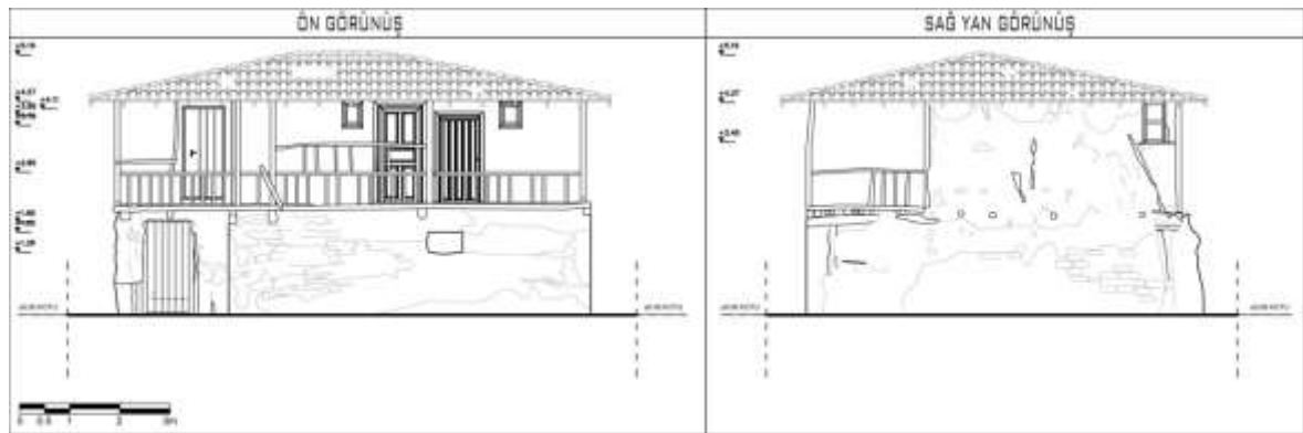
Şekil 4.48. 11 numaralı Alaçık meskeninin Güneydoğu ve Kuzeydoğu cephesi
