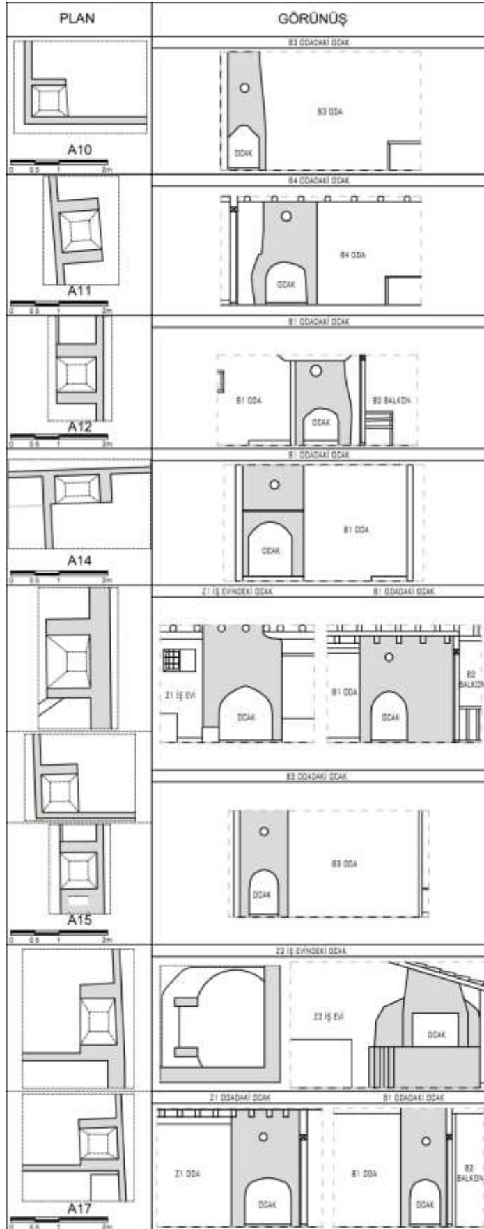
Şekil 5.7. Alaçık meskenlerinde ocaklar
