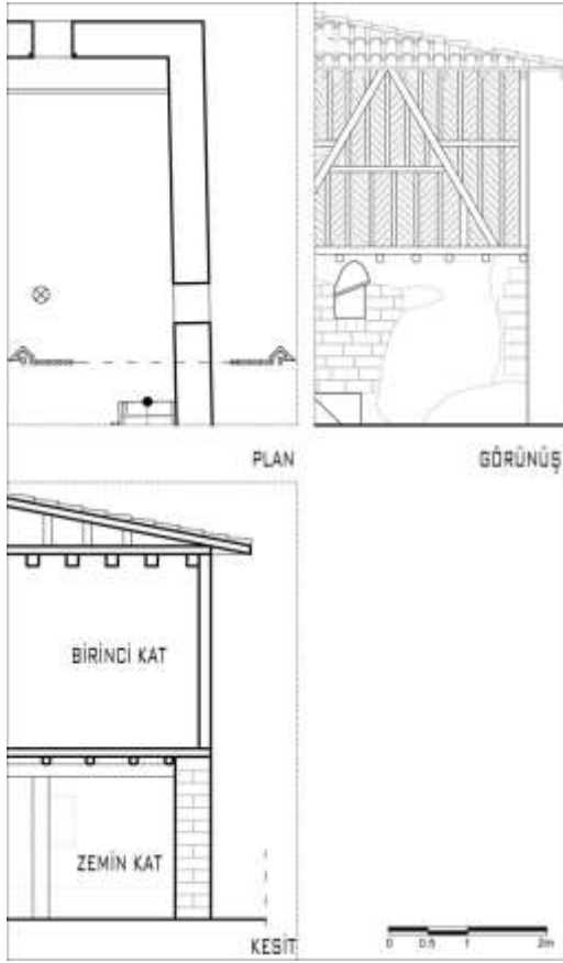
Şekil 5.17. Bağ evlerinde duvar detayı
