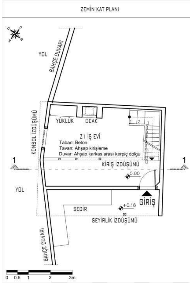
Şekil 4.6. 2 numaralı Gümelenin zemin kat planı
