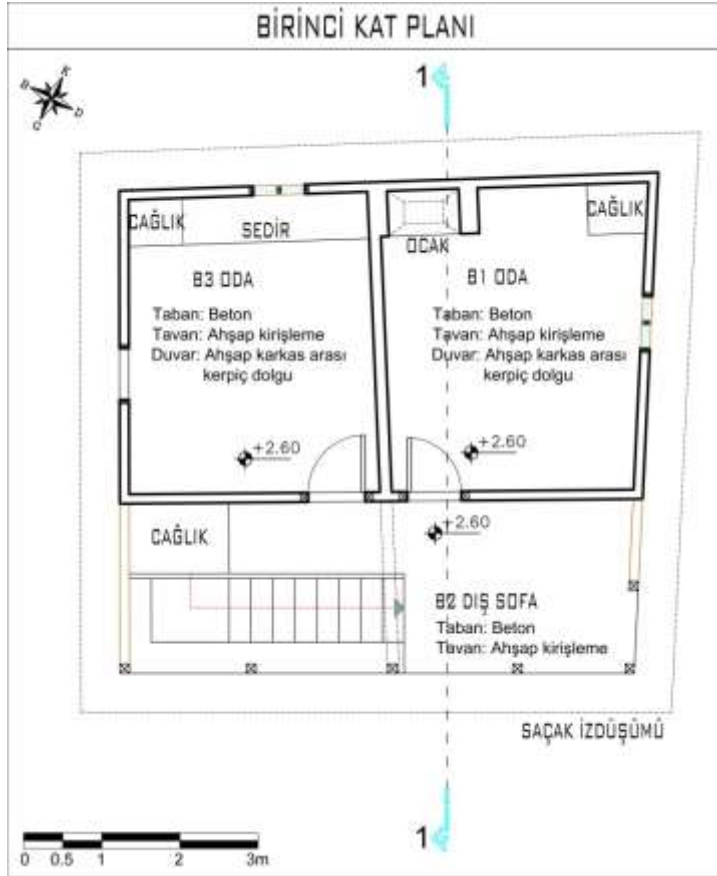
Şekil 4.61. 14 numaralı Alaçık meskeninin birinci kat planı
