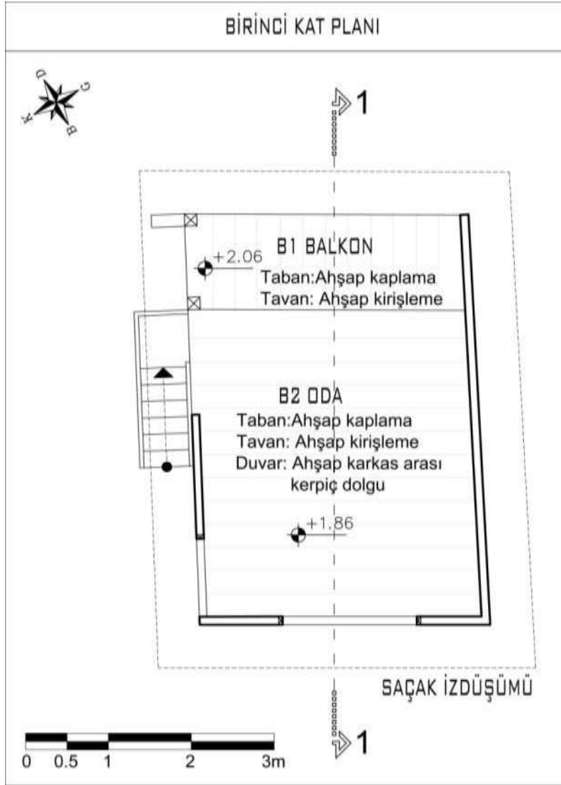
Şekil 4.17. 4 numaralı Gümelenin birinci kat planı
