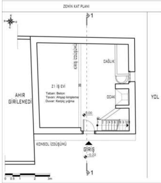
Şekil 4.65. 15 numaralı Alaçık meskeninin zemin kat planı
