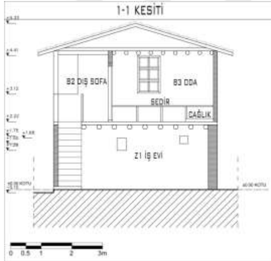
Şekil 4.59. 13 numaralı Alaçık meskeninin kesiti
