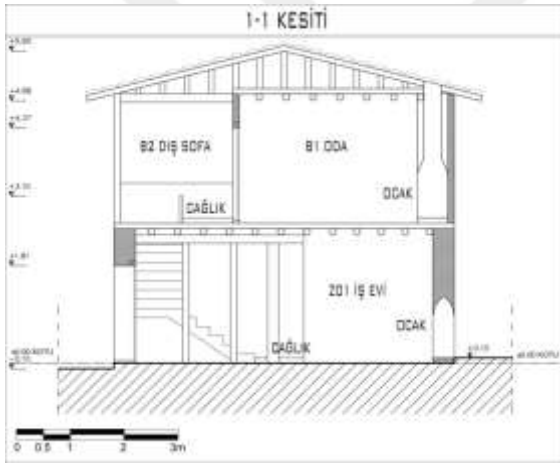
Şekil 4.64. 14 numaralı Alaçık meskeninin kesiti
