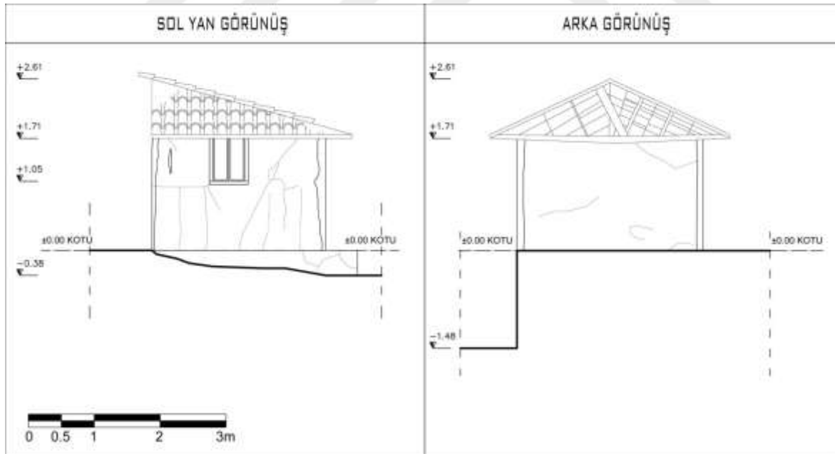
Şekil 4.36. 8 numaralı Gümelenin Kuzeybatı ve Kuzeydoğu cepheleri
