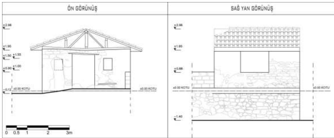
Şekil 4.27. 6 numaralı Gümelenin Kuzeydoğu ve Kuzeybatı cepheleri
