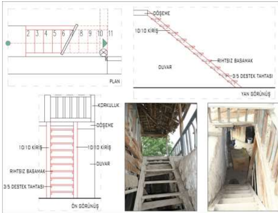
Şekil 5.5. Riht tahtası olmayan merdiven detayı (A11)
