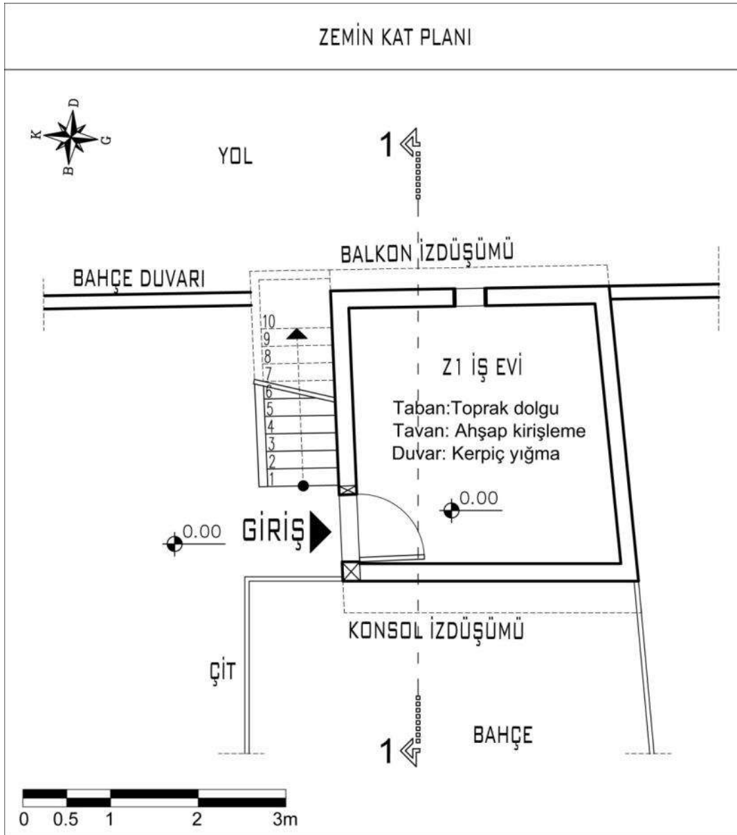
Şekil 4.21. 5 numaralı Gümelenin zemin kat planı
