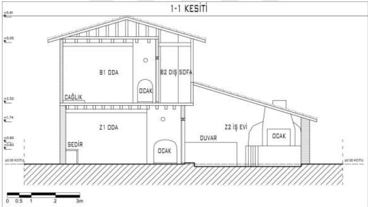
Şekil 4.76. 17 numaralı Alaçık meskeninin kesiti
