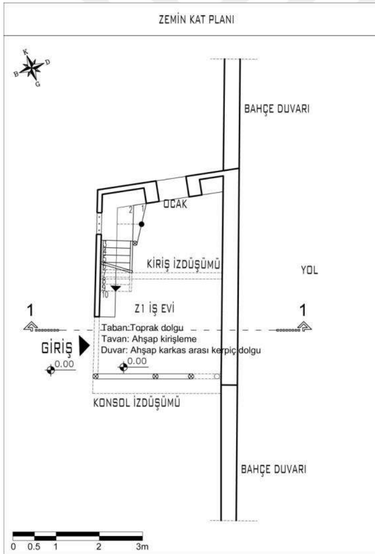
Şekil 4.11. 3 numaralı Gümelenin zemin kat planı
