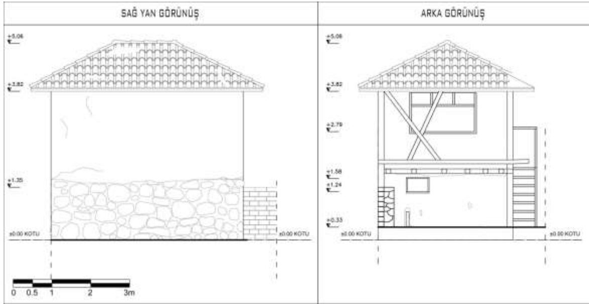
Şekil 4.19. 4 numaralı Gümelenin Güneybatı ve Güneydoğu cephesi
