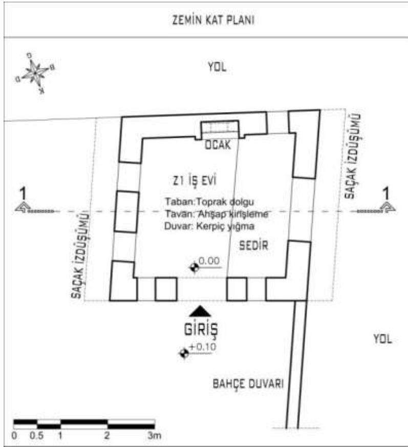
Şekil 4.26. 6 numaralı Gümelenin zemin kat planı
