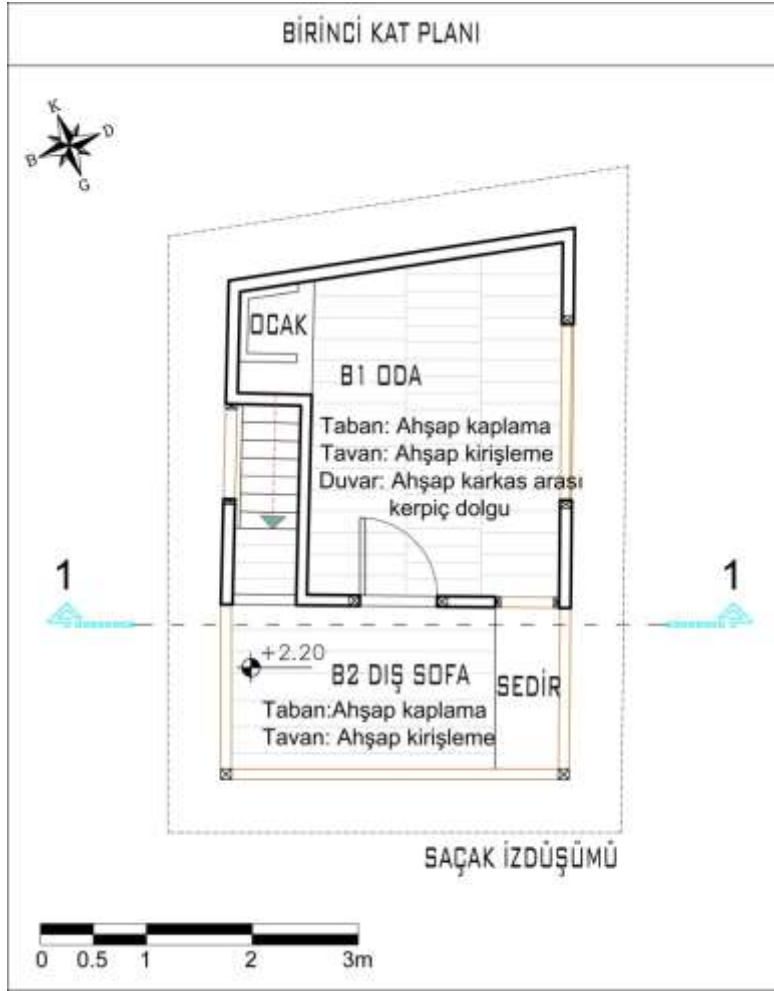
Şekil 4.12. 3 numaralı Gümelenin birinci kat planı
