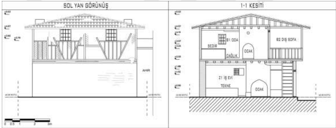
Şekil 4.68. 15 numaralı Alaçık meskeninin Kuzey cephesi ve 1-1 kesiti
