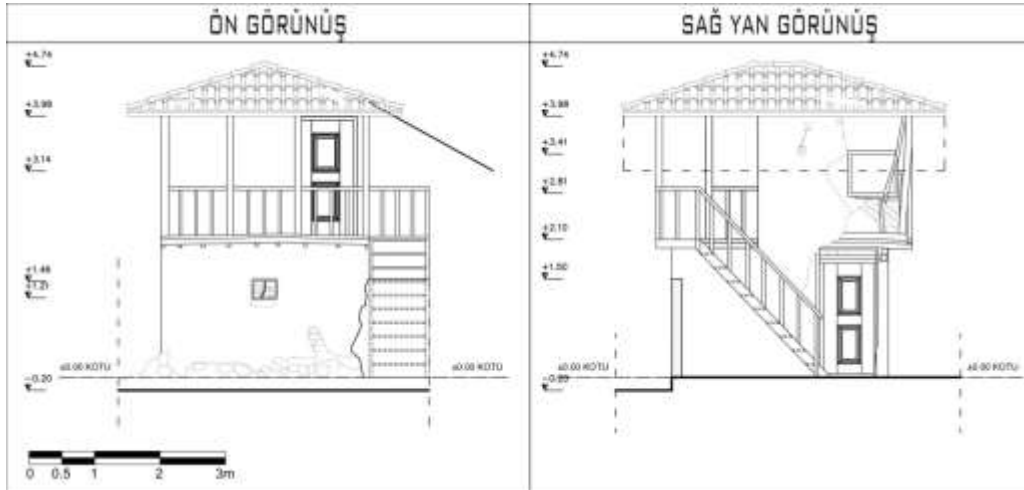
Şekil 4.23. 5 numaralı Gümelenin Doğu ve Kuzey cepheleri
