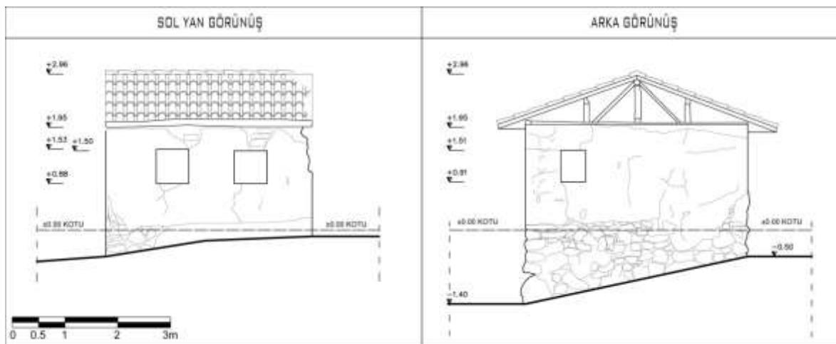
Şekil 4.28. 6 numaralı Gümelenin Güneydoğu ve Güneybatı cepheleri
