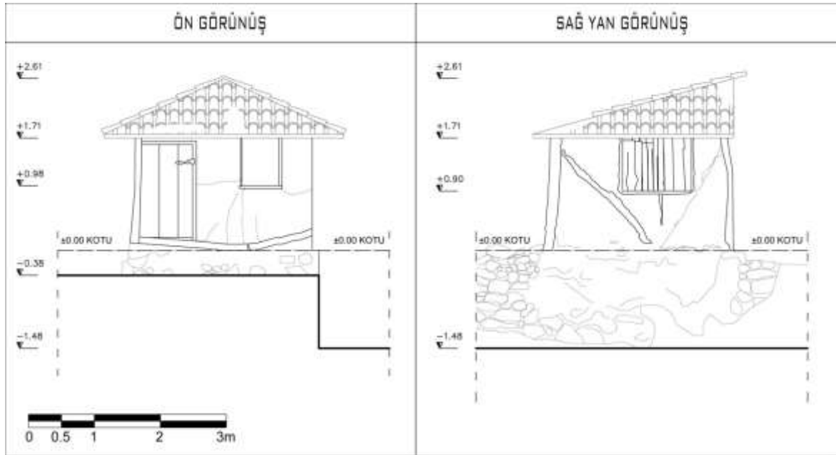
Şekil 4.35. 8 numaralı Gümelenin Güneybatı ve Güneydoğu cepheleri
