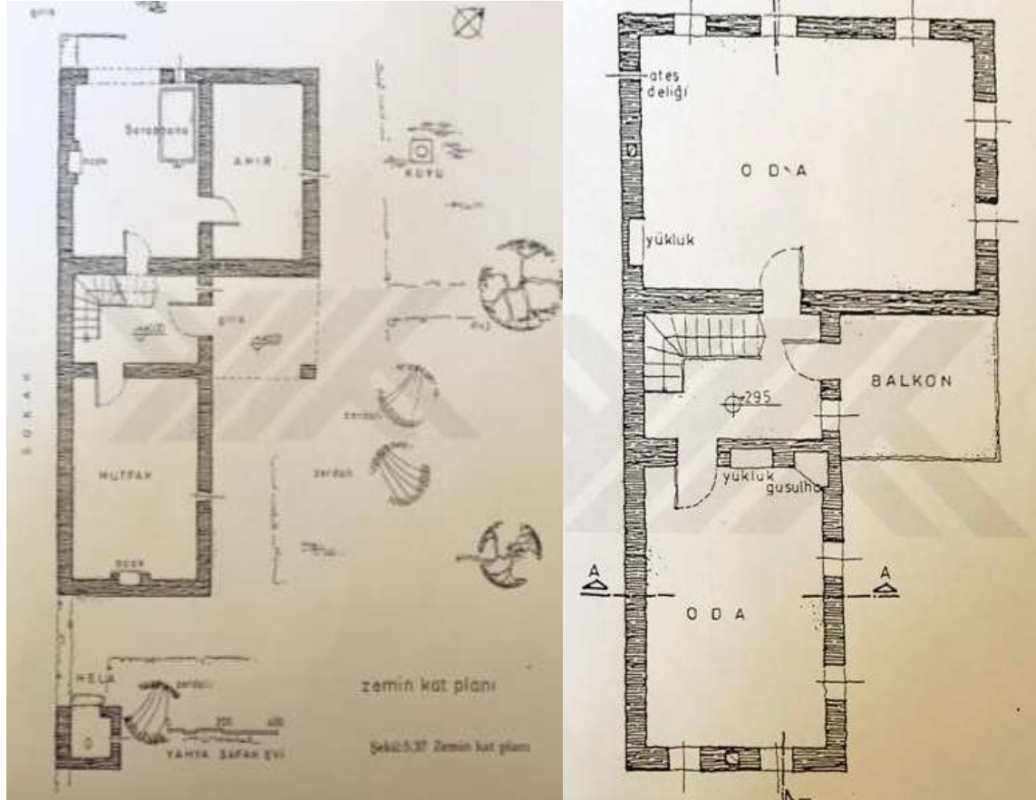
Şekil 3.12. Niğde çevresinde bir bağ evinin zemin ve üst kat planı (sayfa 115-116) [38]
