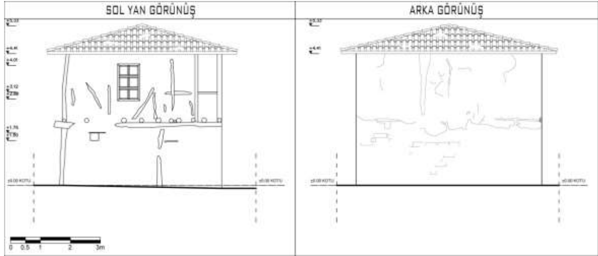
Şekil 4.58. 13 numaralı Alaçık meskeninin Güneybatı ve Kuzeybatı cephesi
