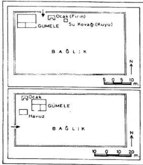
Şekil 3.2. Tosya çevresindeki Gümelelerin arsa üzerindeki vaziyet planı (sayfa 16) [30]
