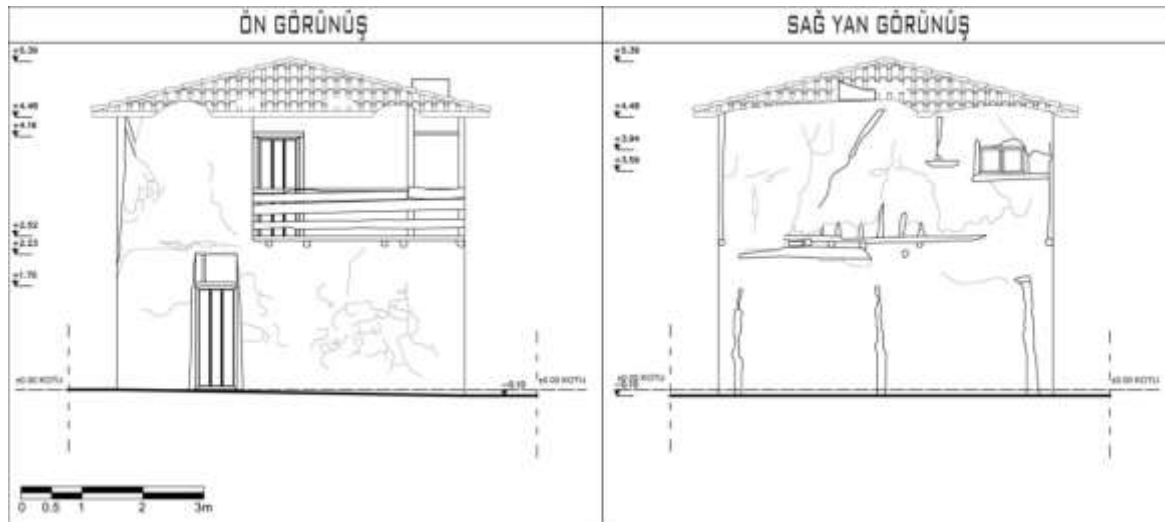
Şekil 4.53. 12 numaralı Alaçık meskeninin Güneydoğu ve Kuzeydoğu cephesi
