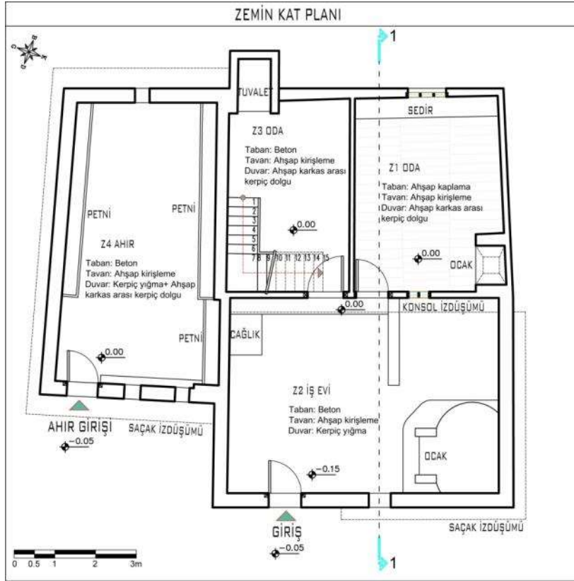
Şekil 4.73. 17 numaralı Alaçık meskeninin zemin kat planı
