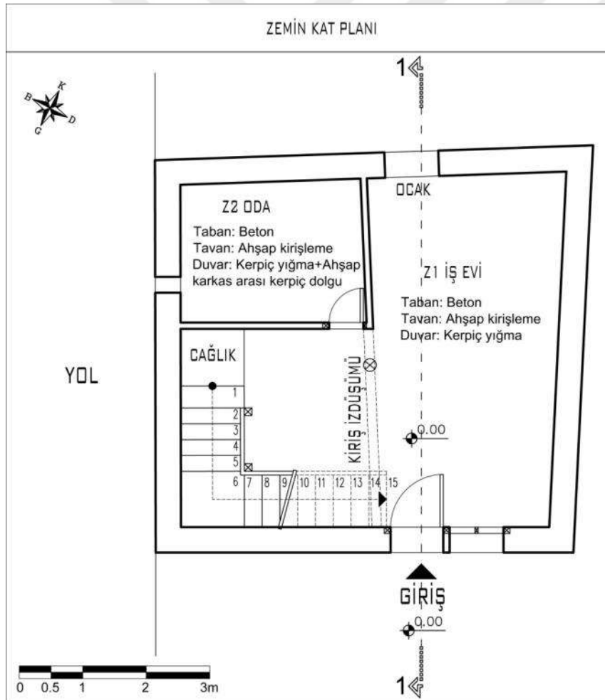
Şekil 4.60. 14 numaralı Alaçık meskeninin zemin kat planı
