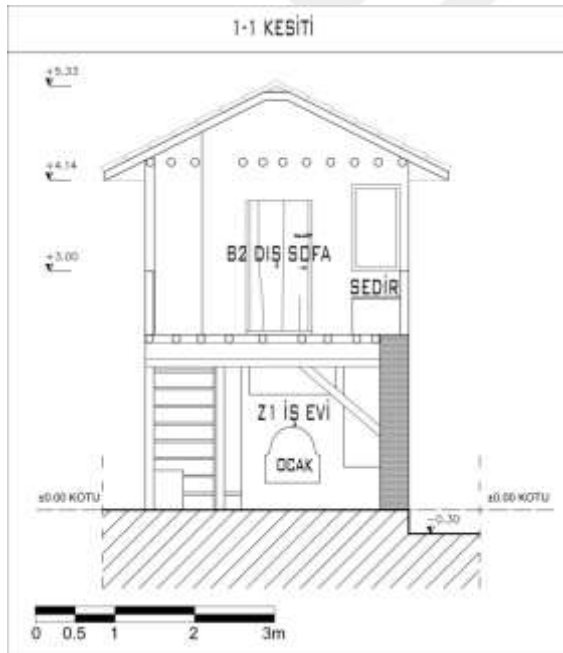
Şekil 4.15. 3 numaralı Gümelenin kesiti
