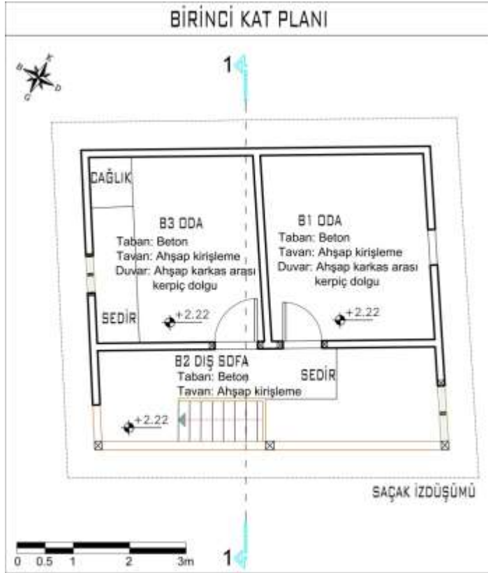
Şekil 4.56. 13 numaralı Alaçık meskeninin birinci kat planı
