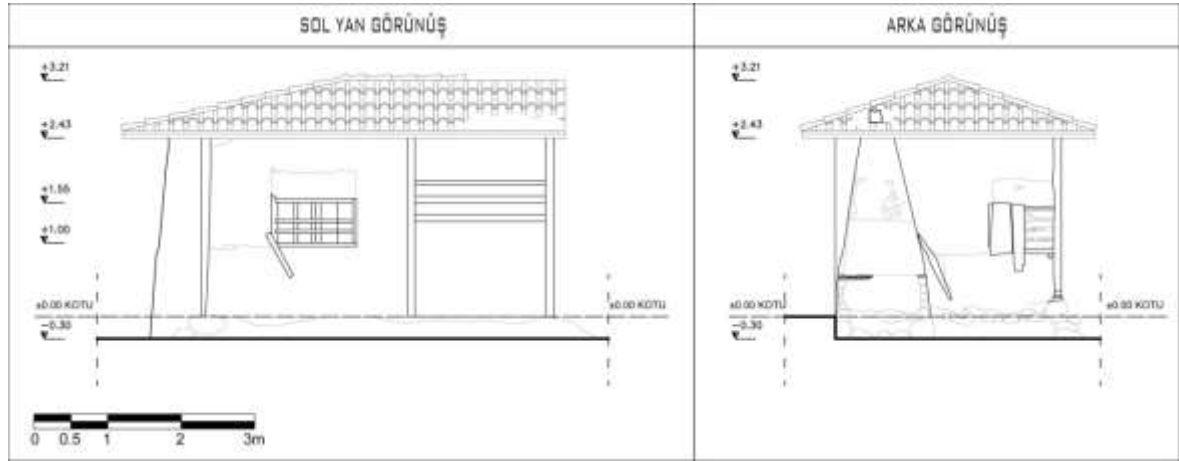
Şekil 4.32. 7 numaralı Gümelenin Güneydoğu ve Güneybatı cepheleri
