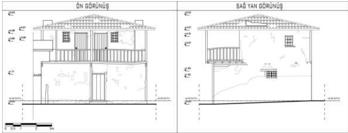
Şekil 4.67. 15 numaralı Alaçık meskeninin Güney ve Doğu cepheleri
