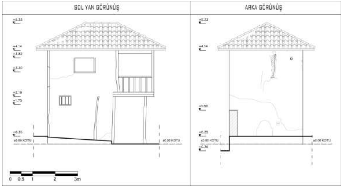
Şekil 4.14. 3 numaralı Gümelenin Kuzeybatı ve Kuzeydoğu cephesi
