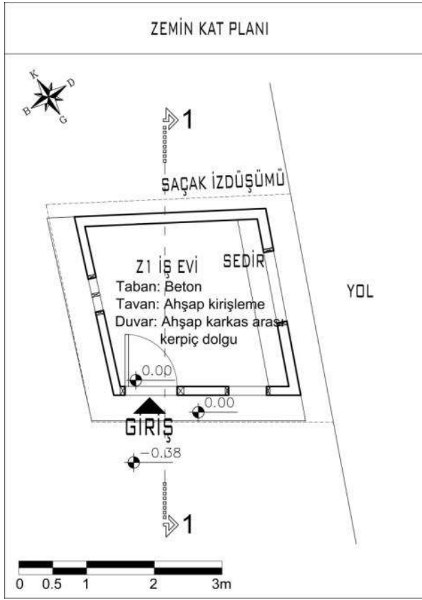
Şekil 4.34. 8 numaralı Gümelenin zemin kat planı
