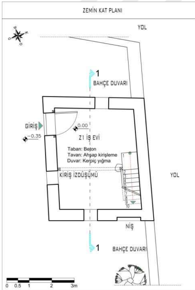
Şekil 4.1. 1 numaralı bağ evinin zemin kat planı
