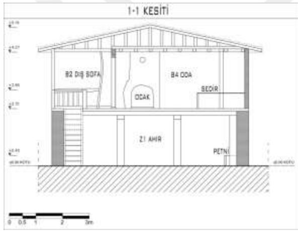
Şekil 4.50. 11 numaralı Alaçık meskeninin kesiti
