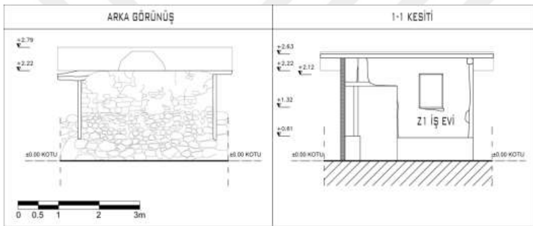
Şekil 4.40. 9 numaralı Gümelenin Batı cephesi ve 1-1 kesiti
