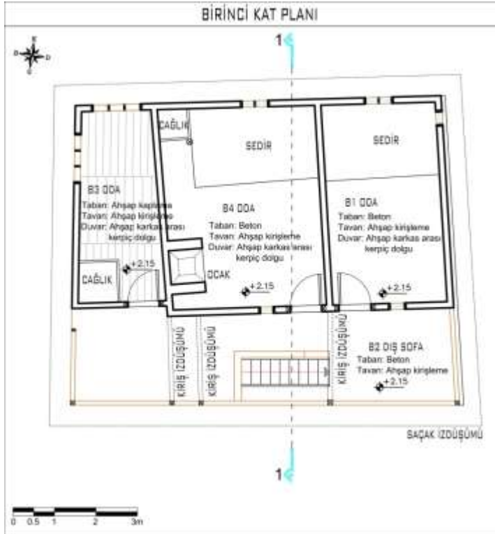
Şekil 4.47. 11 numaralı Alaçık meskeninin birinci kat planı
