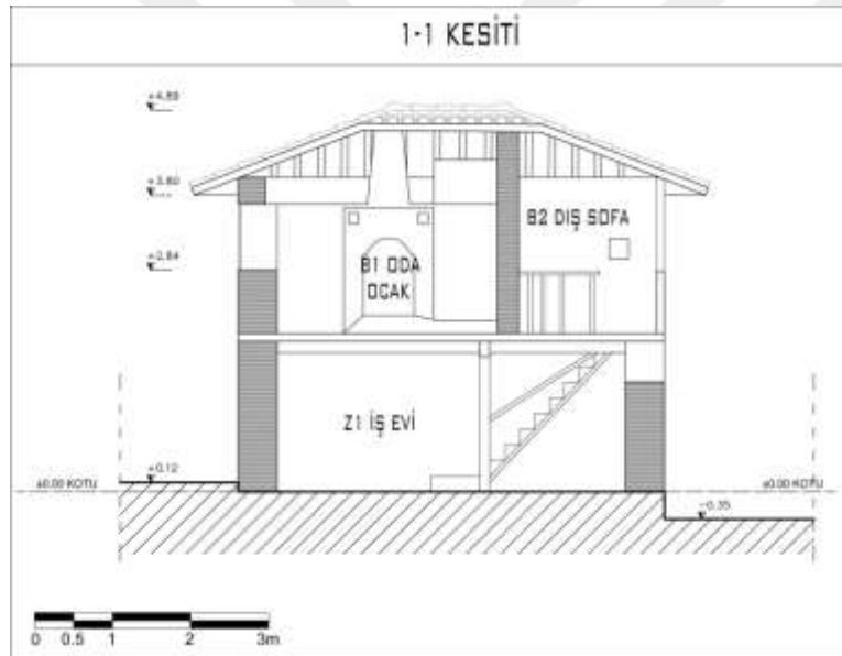
Şekil 4.5. 1 numaralı bağ evinin kesiti
