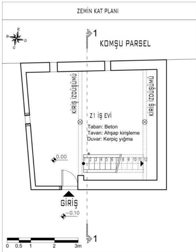
Şekil 4.51. 12 numaralı Alaçık meskeninin zemin kat planı
