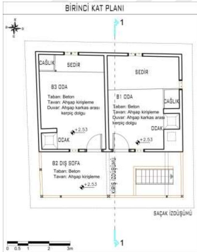
Şekil 4.66. 15 numaralı Alaçık meskeninin birinci kat planı
