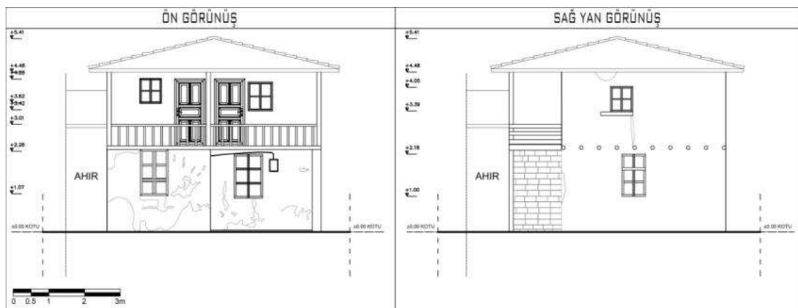
Şekil 4.71. 16 numaralı Alaçık meskeninin Güneydoğu ve Kuzeydoğu cephesi
