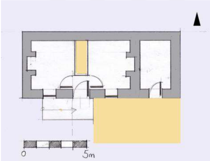
Şekil 3.10. İncirkırı evlerinde iki oda ve bir tuvalet/deposu olan üst kat tipolojisi (sayfa 278) [36]
