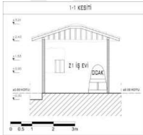
Şekil 4.33. 7 numaralı Gümelenin kesiti
