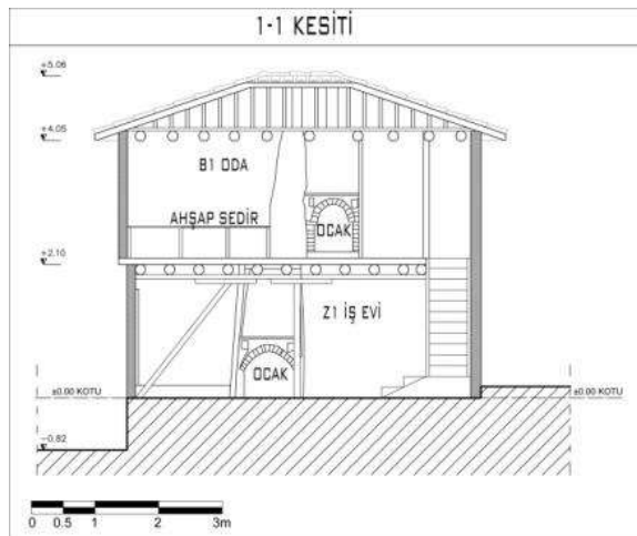
Şekil 4.10. 2 numaralı Gümelenin kesiti
