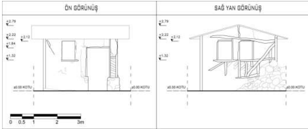
Şekil 4.39. 9 numaralı Gümelenin Doğu ve Kuzey cepheleri
