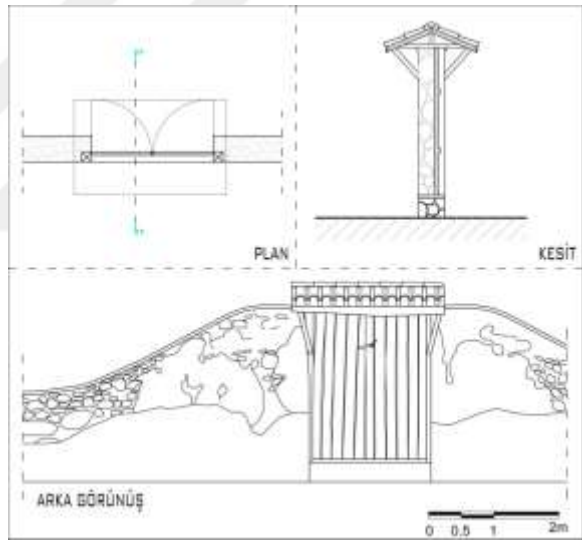
Şekil 5.10. G3 bahçe kapısı detayı
