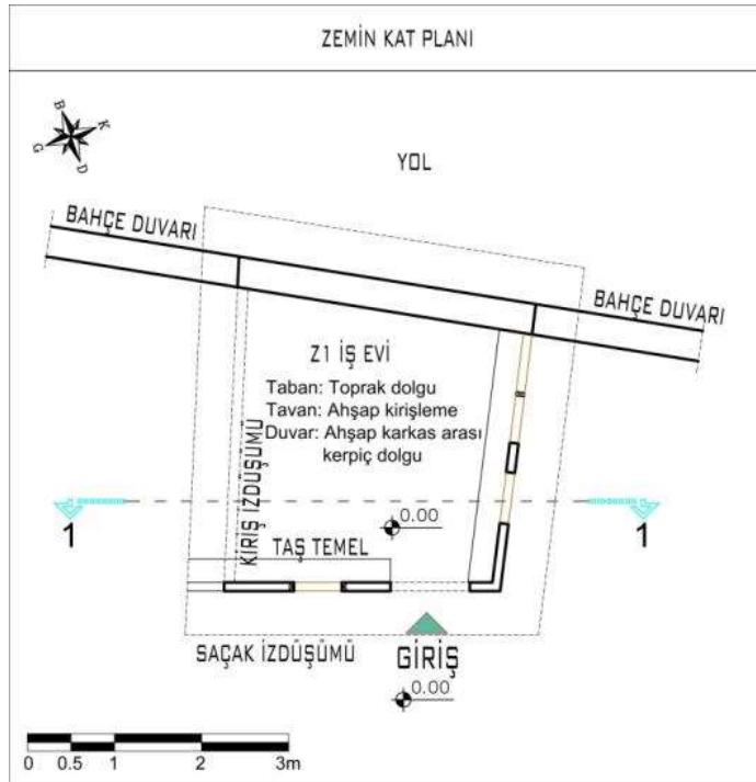
Şekil 4.38. 9 numaralı Gümelenin zemin kat planı
