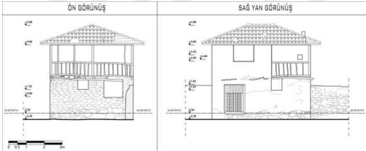
Şekil 4.3. 1 numaralı bağ evinin Güneydoğu ve Kuzeydoğu cephesi
