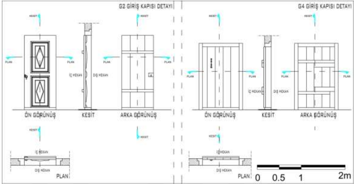
Şekil 5.11. Bağ evlerinde giriş kapısı detayları
