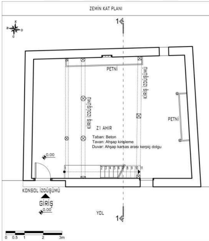
Şekil 4.46. 11 numaralı Alaçık meskeninin zemin kat planı
