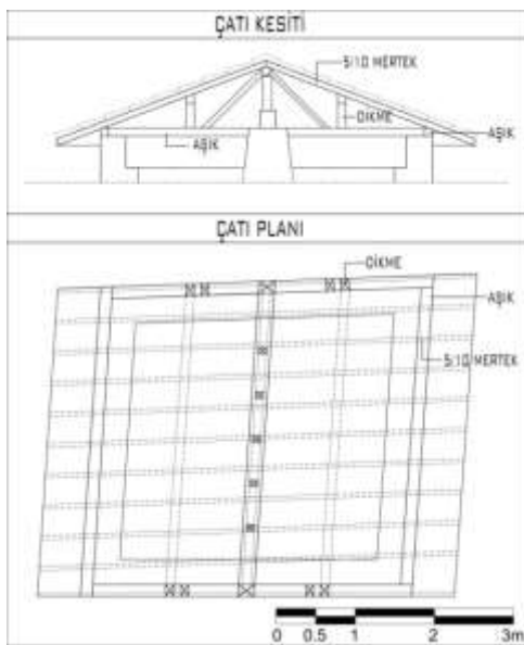
Şekil 5.19. Bağ evlerinde ahşap çatı elemanları
