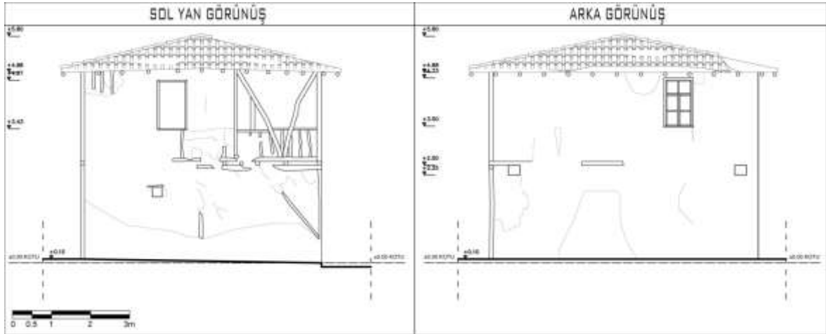
Şekil 4.63. 14 numaralı Alaçık meskeninin Güneybatı ve Kuzeybatı cephesi
