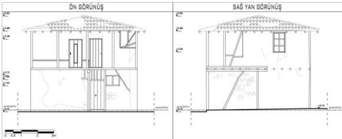
Şekil 4.62. 14 numaralı Alaçık meskeninin Güneydoğu ve Kuzeydoğu cephesi
