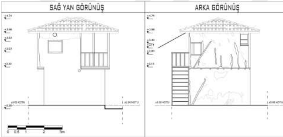
Şekil 4.24. 5 numaralı Gümelenin Güney ve Batı cepheleri
