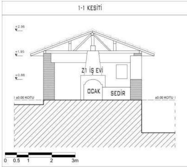
Şekil 4.29. 6 numaralı Gümelenin kesiti
