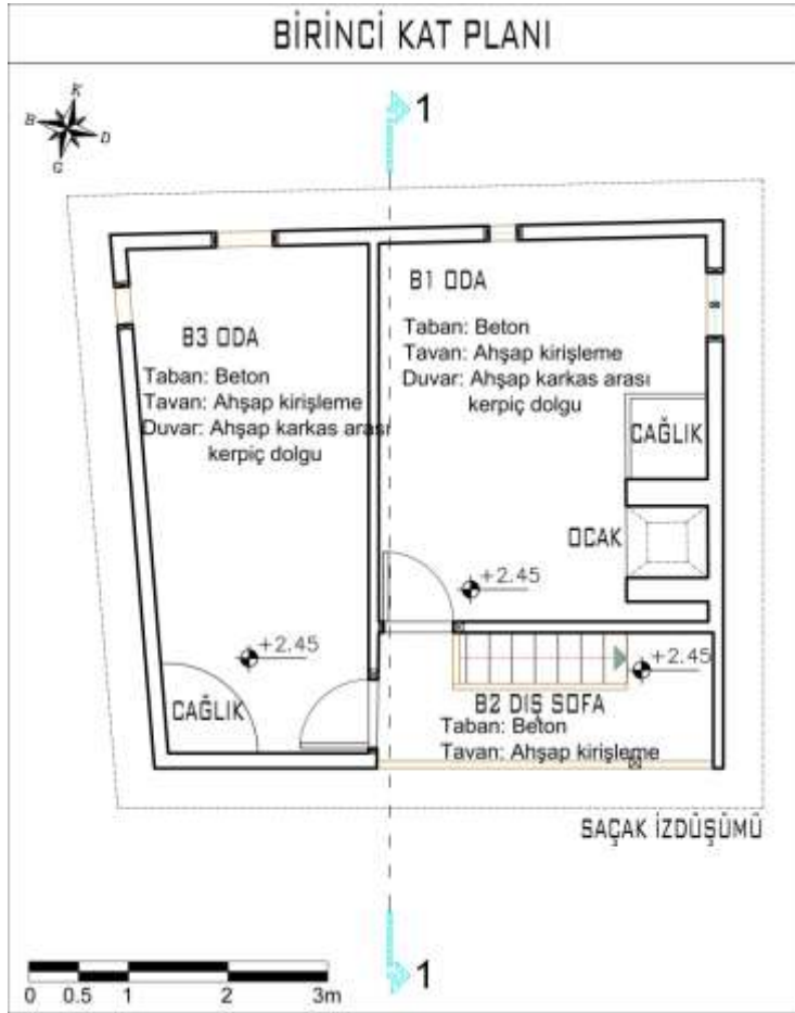
Şekil 4.52. 12 numaralı Alaçık meskeninin birinci kat planı
