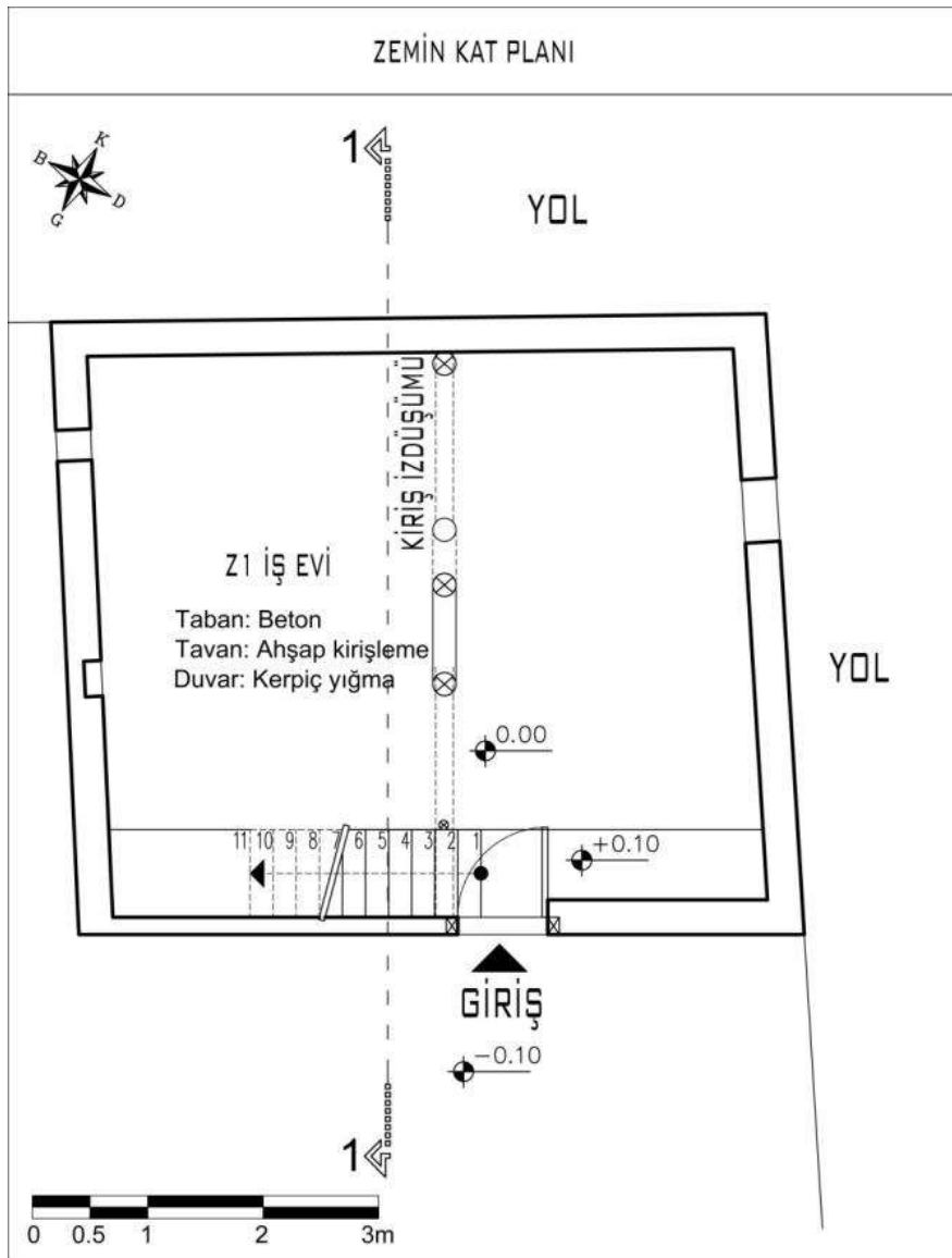
Şekil 4.55. 13 numaralı Alaçık meskeninin zemin kat planı
