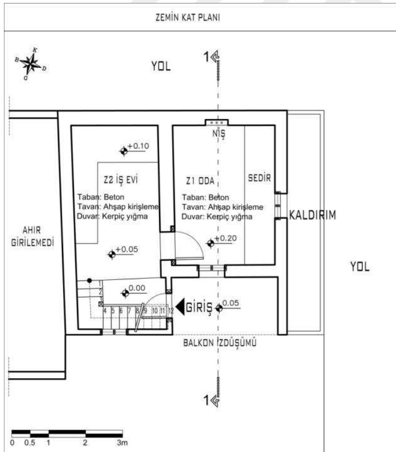
Şekil 4.69. 16 numaralı Alaçık meskeninin zemin kat planı
