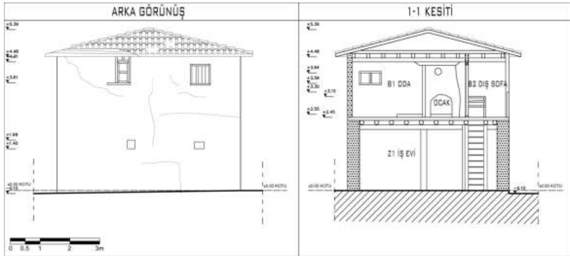
Şekil 4.54. 12 numaralı Alaçık meskeninin Kuzeybatı cephesi ve 1-1 kesiti
