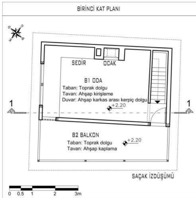
Şekil 4.7. 2 numaralı Gümelenin birinci kat planı
