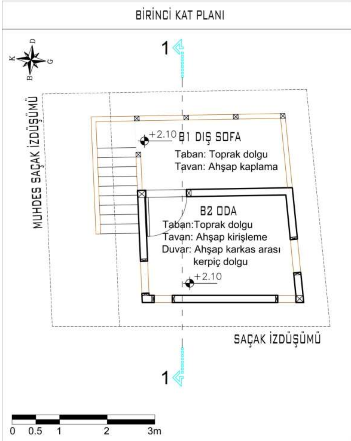
Şekil 4.22. 5 numaralı Gümelenin birinci kat planı
