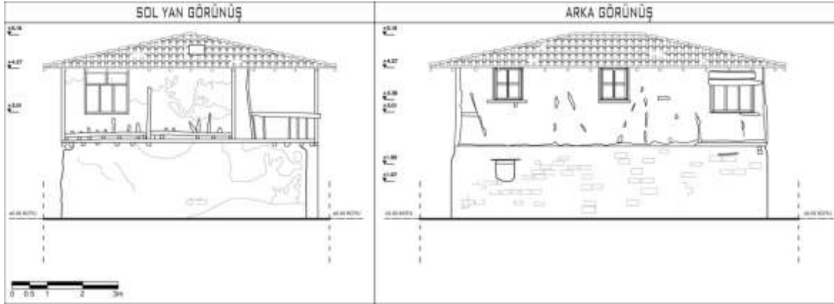
Şekil 4.49. 11 numaralı Alaçık meskeninin Güneybatı ve Kuzeybatı cephesi
