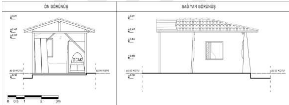
Şekil 4.31. 7 numaralı Gümelenin Kuzeydoğu ve Kuzeybatı cepheleri
