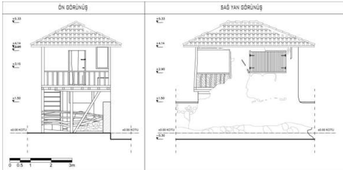
Şekil 4.13. 3 numaralı Gümelenin Güneybatı ve Güneydoğu cephesi
