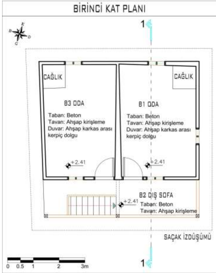
Şekil 4.70. 16 numaralı Alaçık meskeninin birinci kat planı
