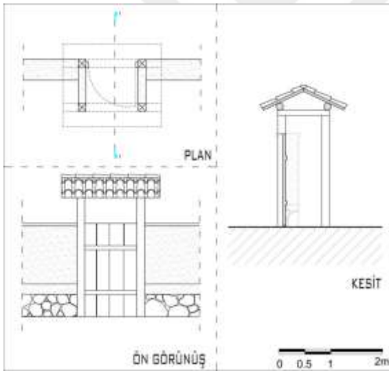
Şekil 5.9. G2 bahçe kapısı detayı
