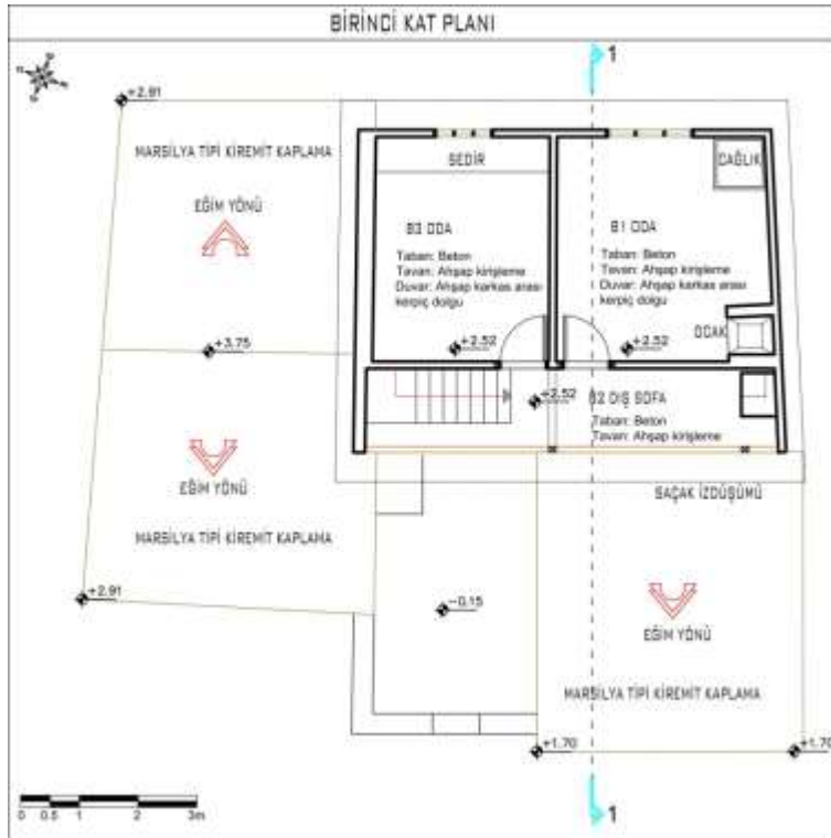
Şekil 4.74. 17 numaralı Alaçık meskeninin birinci kat planı
