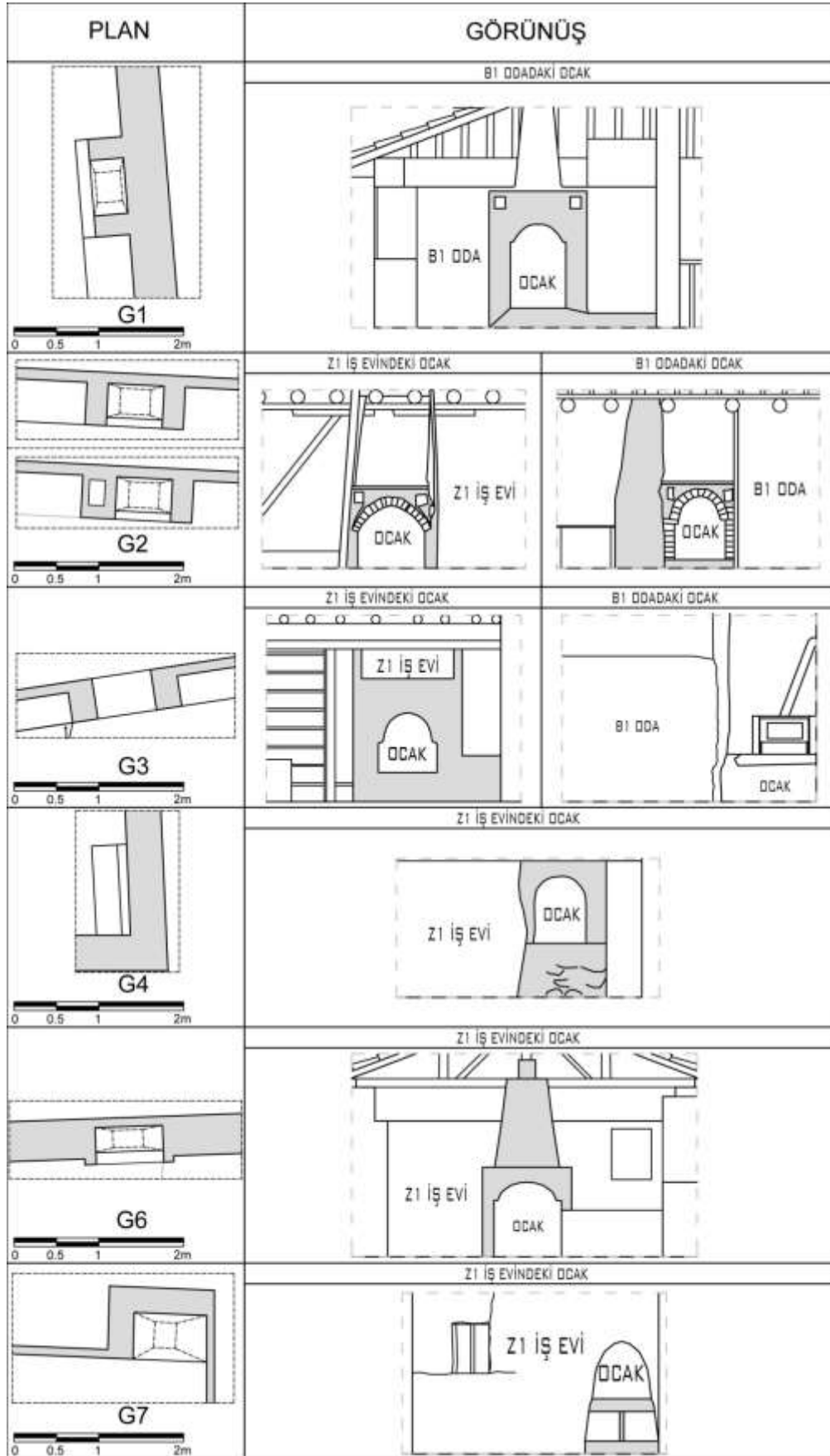
Şekil 5.6. Gümele meskenlerinde ocaklar
