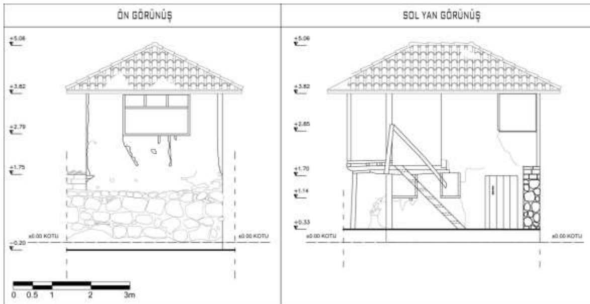
Şekil 4.18. 4 numaralı Gümelenin Kuzeybatı ve Kuzeydoğu cephesi
