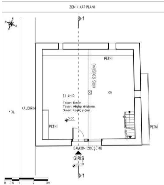
Şekil 4.41. 10 numaralı Alaçık meskeninin zemin kat planı
