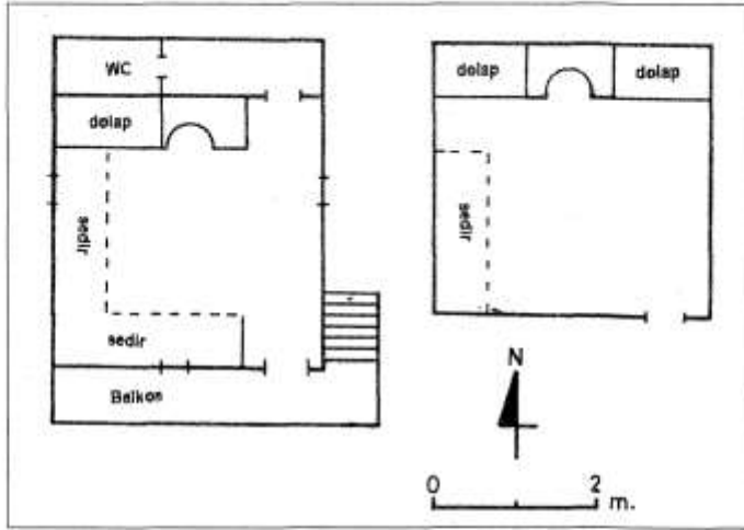
Şekil 3.5. Safranbolu platosunda iki katlı bir bağ evi örneği (sayfa 140) [33]
