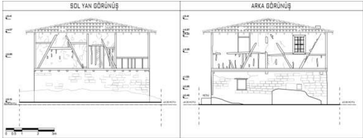
Şekil 4.44. 10 numaralı Alaçık meskeninin Güneybatı ve Kuzeybatı cephesi
