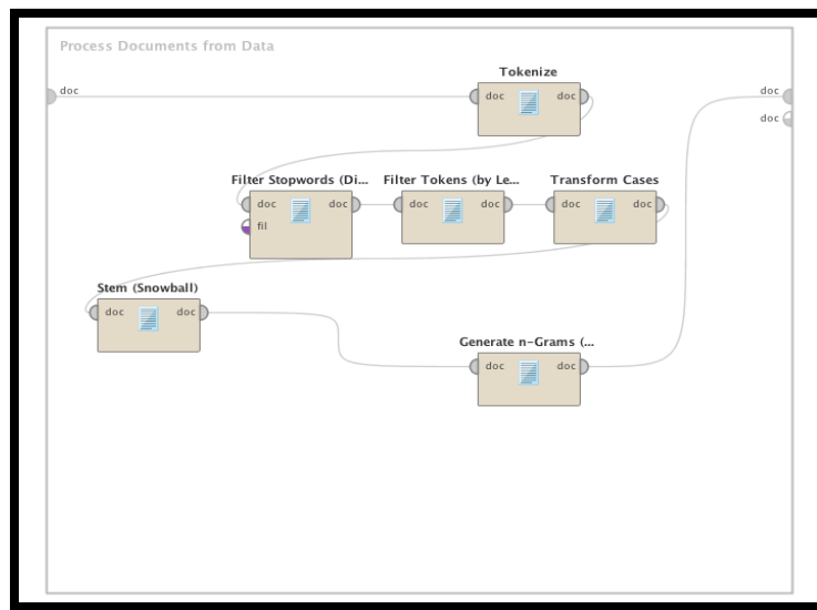
Şekil 16: RapidMiner Veri Ön İşleme Süreci
