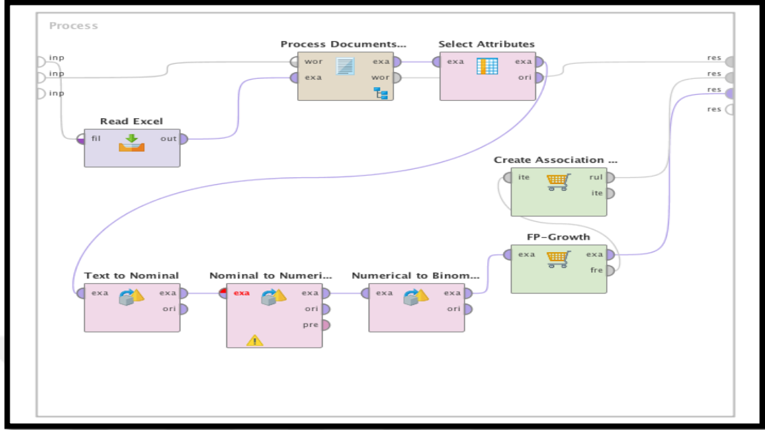
Şekil 17: Veri Madenciliği İşlemi
