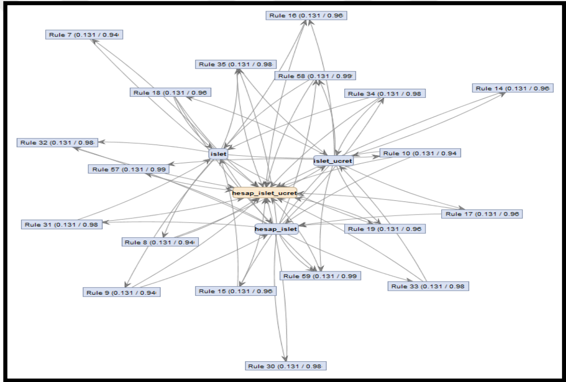
Şekil 19: Birliktelik Kuralının Grafik Olarak Gösterilmesi (Temmuz-Aralık Verisi)
