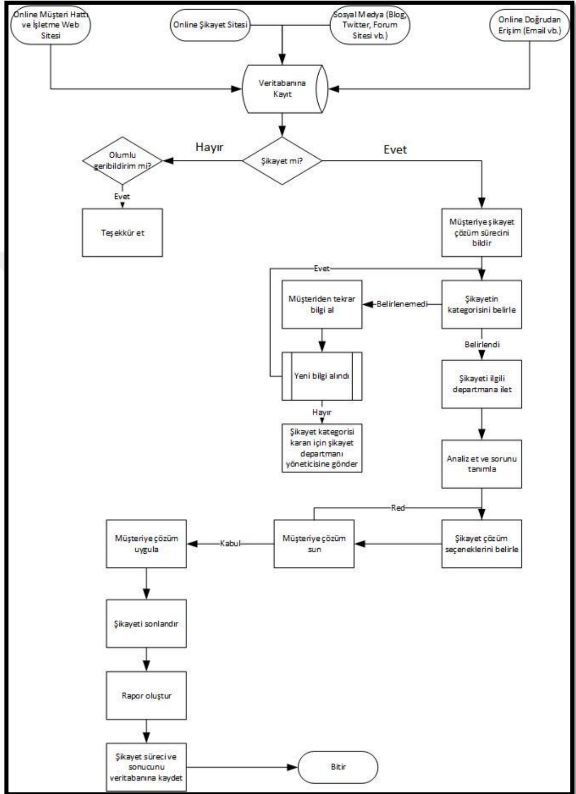
Şekil 9: Online Müşteri Yönetim Sistemi İş Akış Şeması
