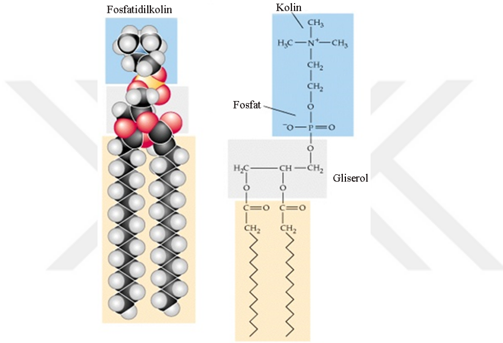
Şekil 1.8. Fosfatidilkolin yapısı
