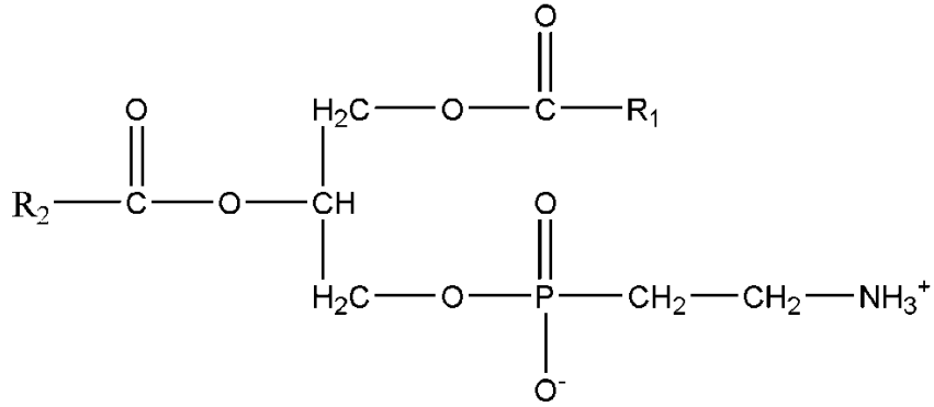
Şekil 1.9. Fosfatidiletanolamin yapısı
