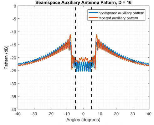
(d) Beamspace auxiliary patterns vs angles when D = 16
