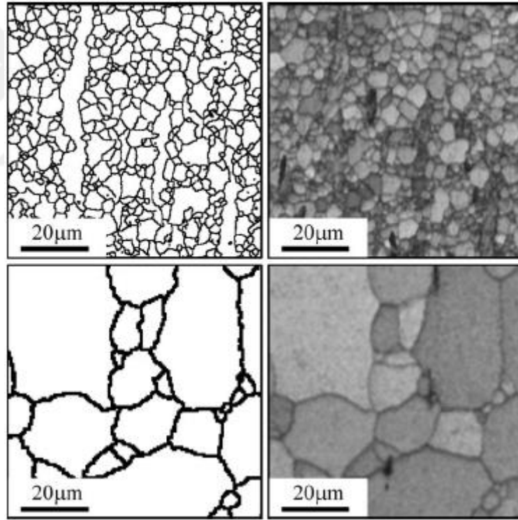
Görsel 3. 5 Üstte:, 220°C sıcaklıkta yapılmış ekstrüzyon+yenidenkristalleşme sonrası mikroyapı (tane boyutu=3µm); altta: 450°C sıcaklıkta yapılmış ekstrüzyon+yenidenkristalleşme sonrası mikroyapı (tane boyutu=16µm) [82].
