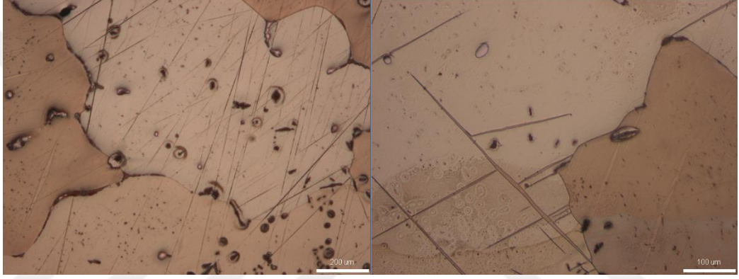
Görsel 3. 1 Mg-2Zn-1Ce-1Y-1Sn alaşımasının döküm mikroyapısı görüntüsü.
