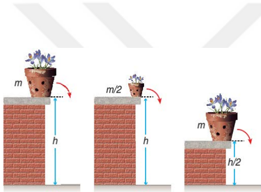
Şekil 4.5: Potansiyel enerji, cismin kütlesine ve yerden yüksekliğine göre değişir.
