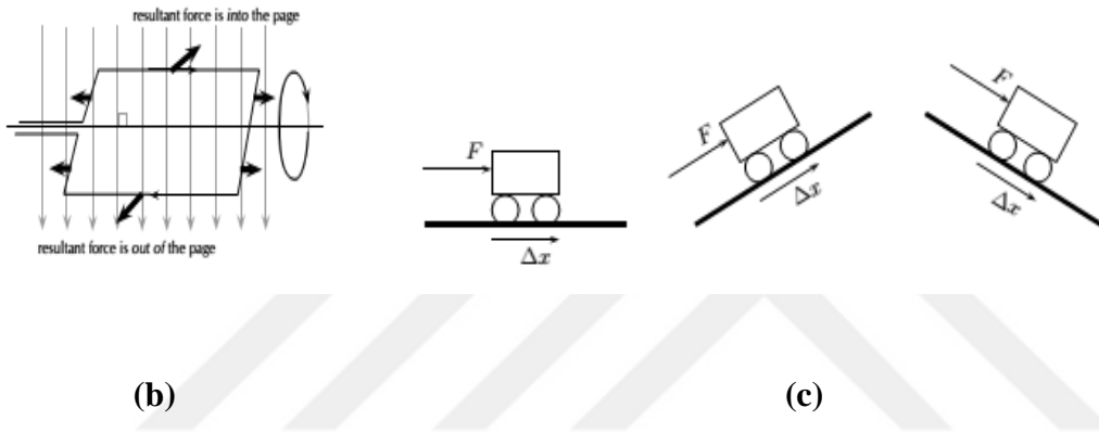
Şekil-4 a) Mercekler, b) Manyetik alanda akım taşıyan çerçeveye etki eden kuvvetler, c) İş' in tanımı ile ilgili görseller (Everything Science 12).
