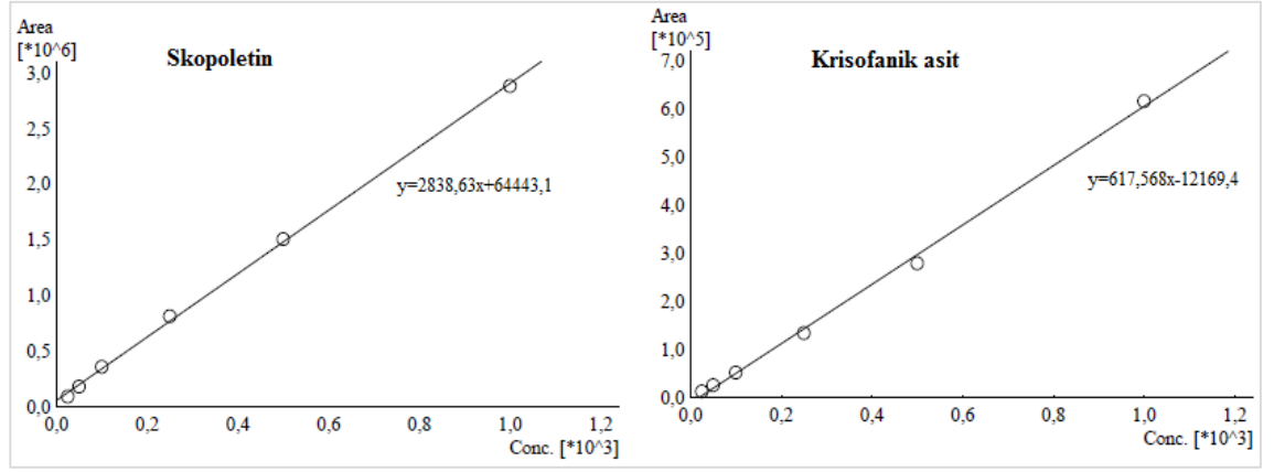
Ek 34. 11 Fitokimyasalın LC-MS/MS metodundaki analitlerin kalibrasyon grafikleri
