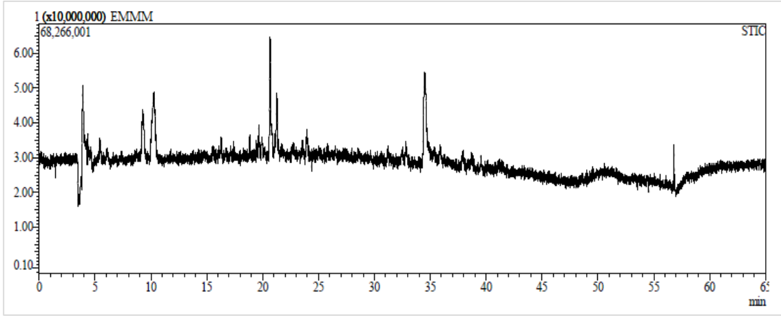
Ek 132. Malatya'dan toplanan E. macroclada 'nın karışık kısmının metanol ekstresinin LC- MS IT- TOF kromatogramı
