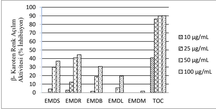
Ek 28. Diyarbakır'dan toplanan E. macroclada 'nın \beta -karoten renk açılım aktivitesi
