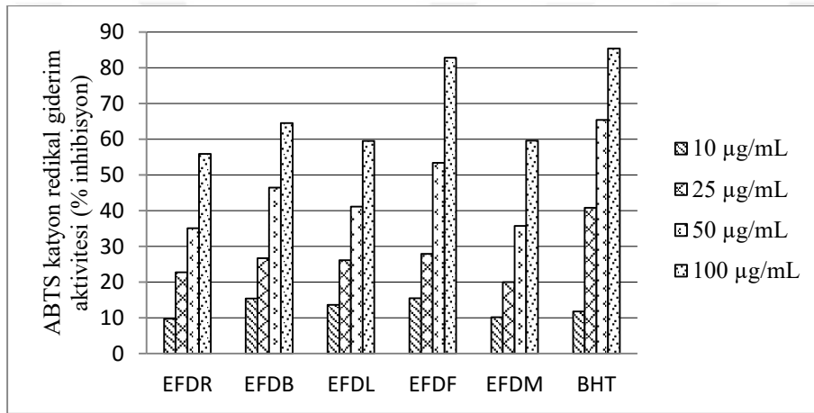
Ek 11. E. fistulosa 'nın ABTS katyon radikali giderim aktivitesi
