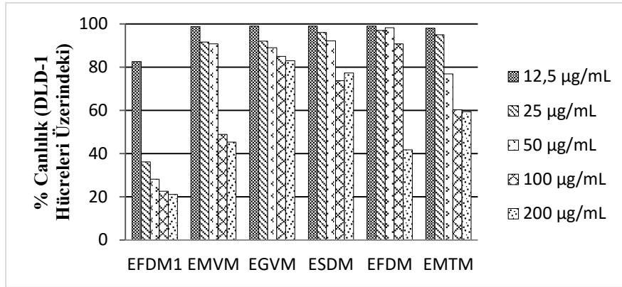
Şekil 4.4. EFDM 1 , EMVM, EGVM, ESDM, EFDM ve EMTM türlerinin kanserli hücre serisindeki stotoksik aktivitesi
