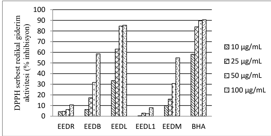
Ek 16. E. eriophora 'nın DPPH serbest radikali giderim aktivitesi
