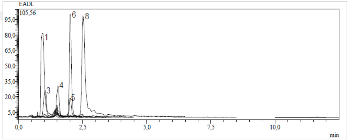
Ek 88. E. aleppica 'nın olgunlaşmış yaprak kısmının metanol ekstresinin kromatogramı
