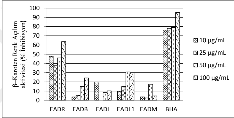
Ek 26. E. aleppica 'nın \beta -karoten renk açılım aktivitesi
