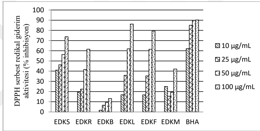
Ek 14. E. denticulata 'nın DPPH serbest radikali giderim aktivitesi
