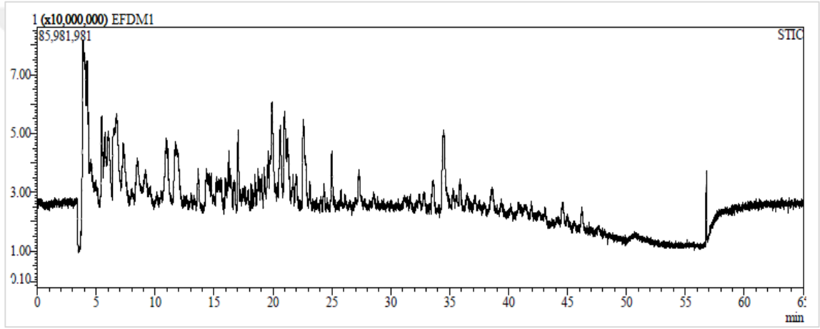
Ek 136. E. falcata 'nın karışık kısmının metanol ekstresinin LC- MS IT- TOF kromatogramı
