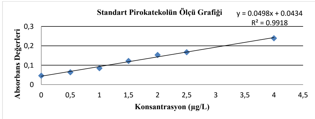
Şekil 3.3. Standart pirokatekolün ölçü grafiği
