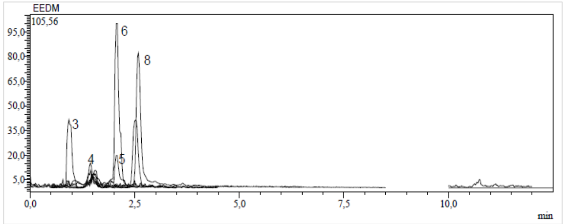
Ek 95. E. eriophora 'nın karışık kısmının metanol ekstresinin kromatogramı
