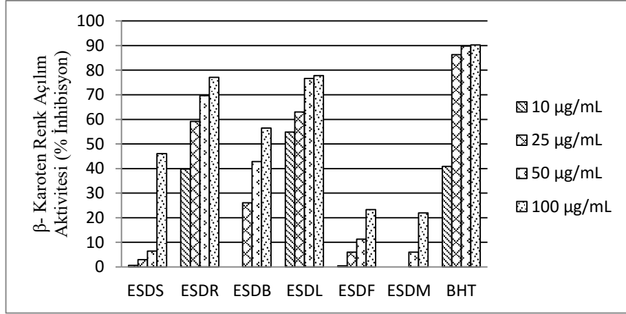
Ek 31. E. seguieriana subsp. seguieriana 'nın \beta -karoten renk açılım aktivitesi
