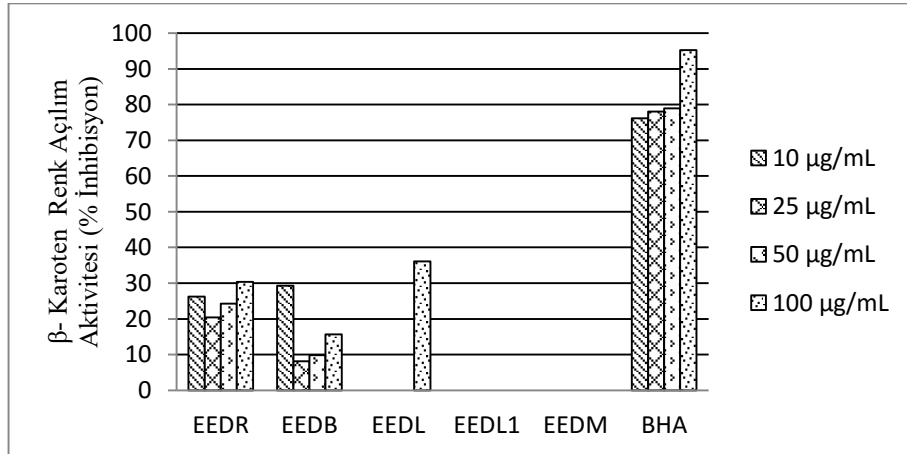
Ek 27. E. eriophora 'nın \beta -karoten renk açılım aktivitesi
