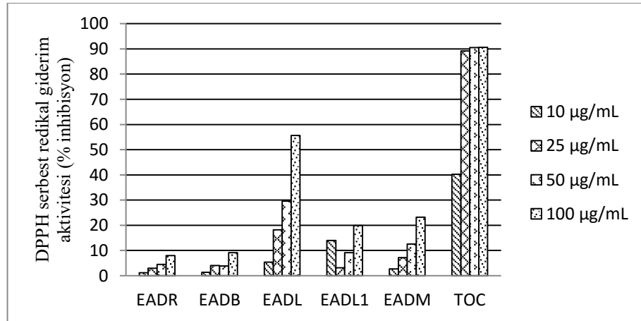
Ek 15. E. aleppica 'nın DPPH serbest radikali giderim aktivitesi
