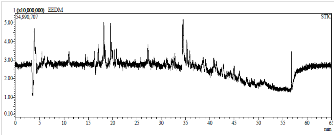
Ek 134. E. erophora 'nın karışık kısmının metanol ekstresinin LC- MS IT- TOF kromatogramı
