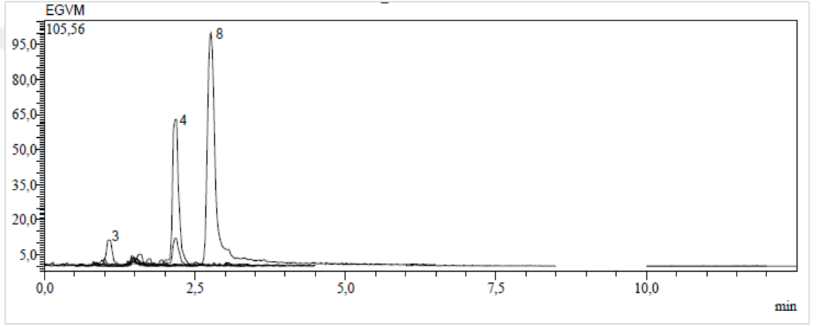
Ek 112. E. grisophylla 'nın karışık kısmının metanol ekstresinin kromatogramı
