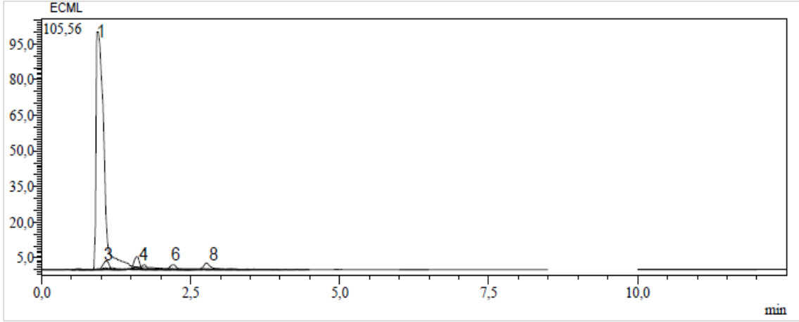
Ek 72. E. craspedia 'nın yaprak kısmının metanol ekstresinin kromatogramı
