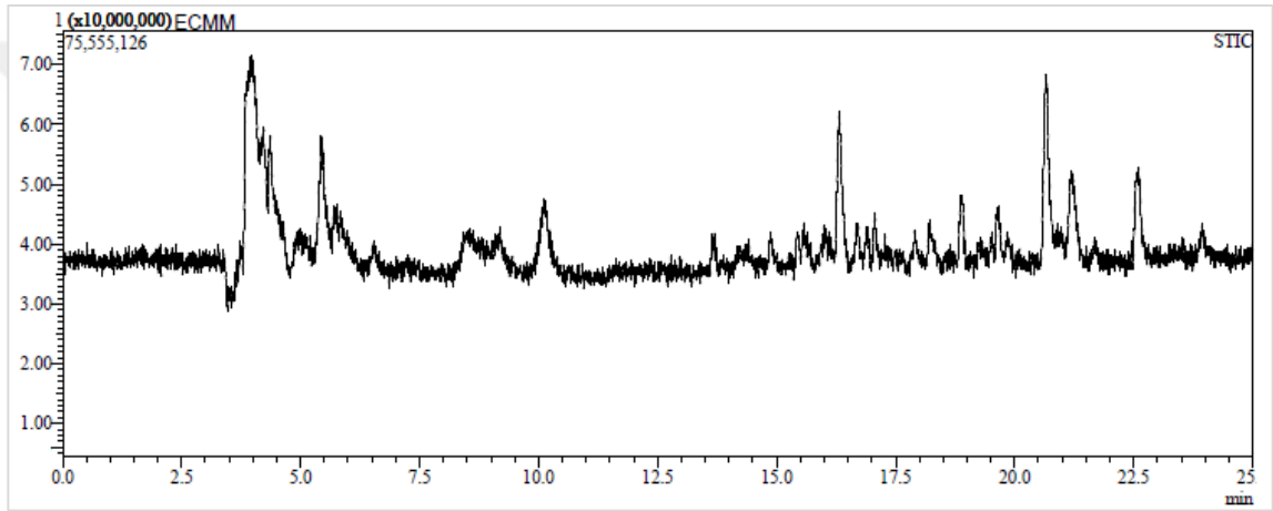
Ek 130. E. craspedia 'nın karışık kısmının metanol ekstresinin LC- MS IT- TOF kromatogramı
