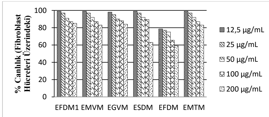
Şekil 4.2. EFDM 1 , EMVM, EGVM, ESDM, EFDM ve EMTM türlerinin canlı fibroblast hücre serisindeki stotoksik aktivitesi
