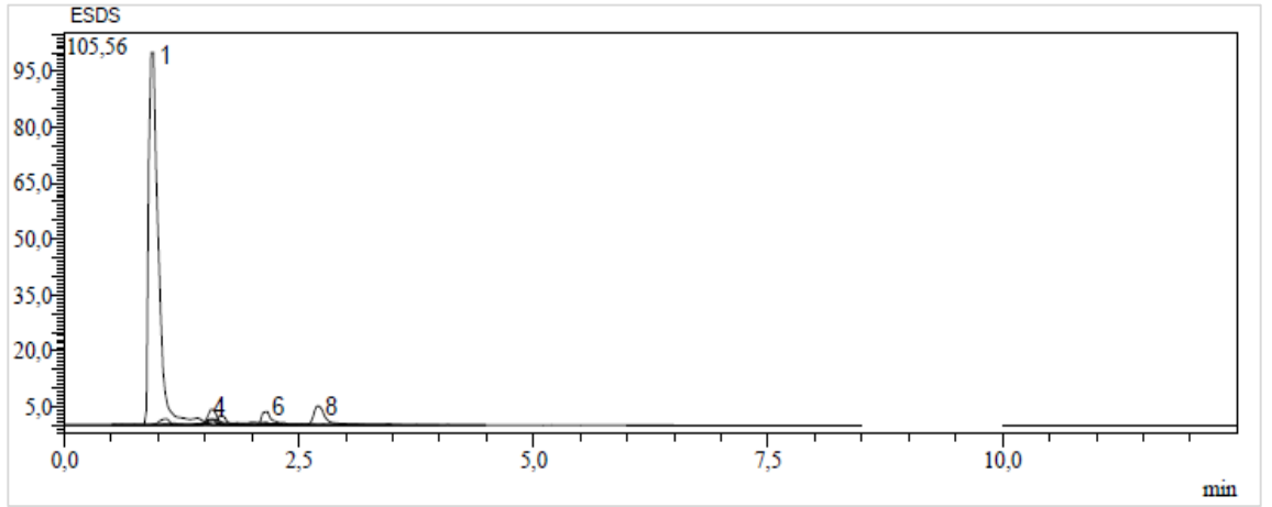
Ek 113. E. seguieriana subsp. seguieriana 'nın tohum kısmının metanol ekstresinin kromatogramı
