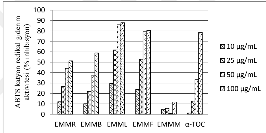
Ek 2. Malatya'dan toplanan E. macroclada 'nın ABTS kasyon radikali giderim aktivitesi
