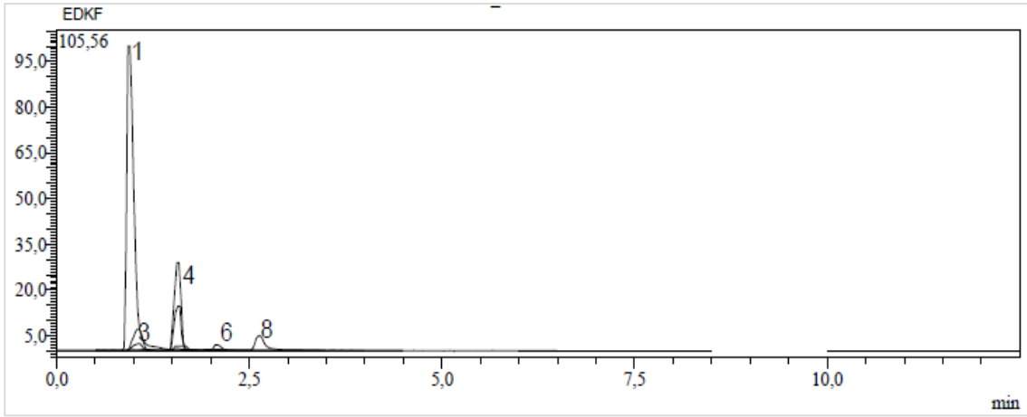
Ek 79. E. denticulata 'nın çiçek kısmının metanol ekstresinin kromatogramı
