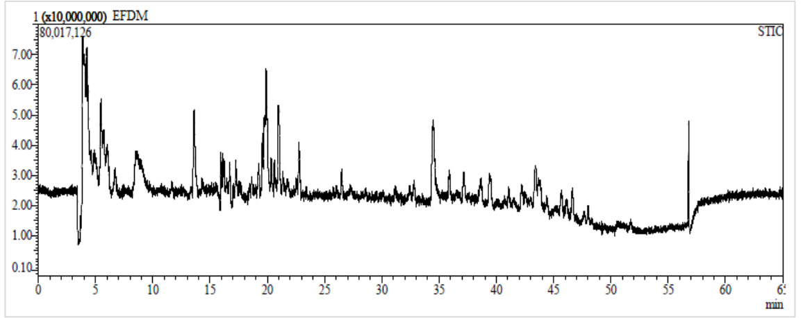
Ek 141. E. fistulosa 'nın karışık kısmının metanol ekstresinin LC- MS IT- TOF kromatogramı
