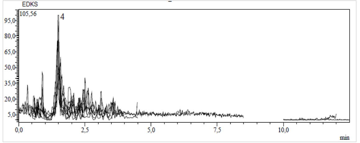
Ek 75. E. denticulata 'nın tohum kısmının metanol ekstresinin kromatogramı
