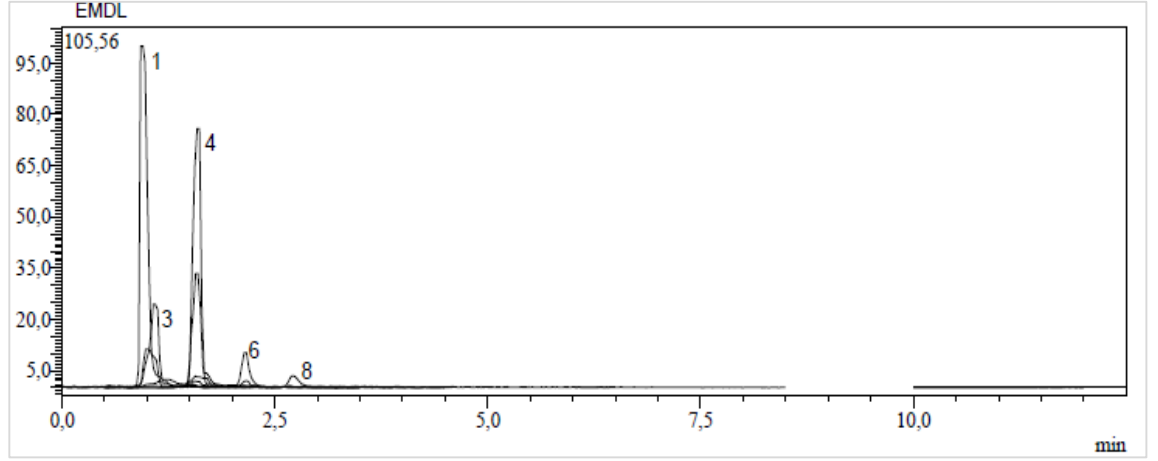
Ek 99. Diyarbakır'dan toplanan E. macroclada 'nın yaprak kısmının metanol ekstresinin kromatogramı
