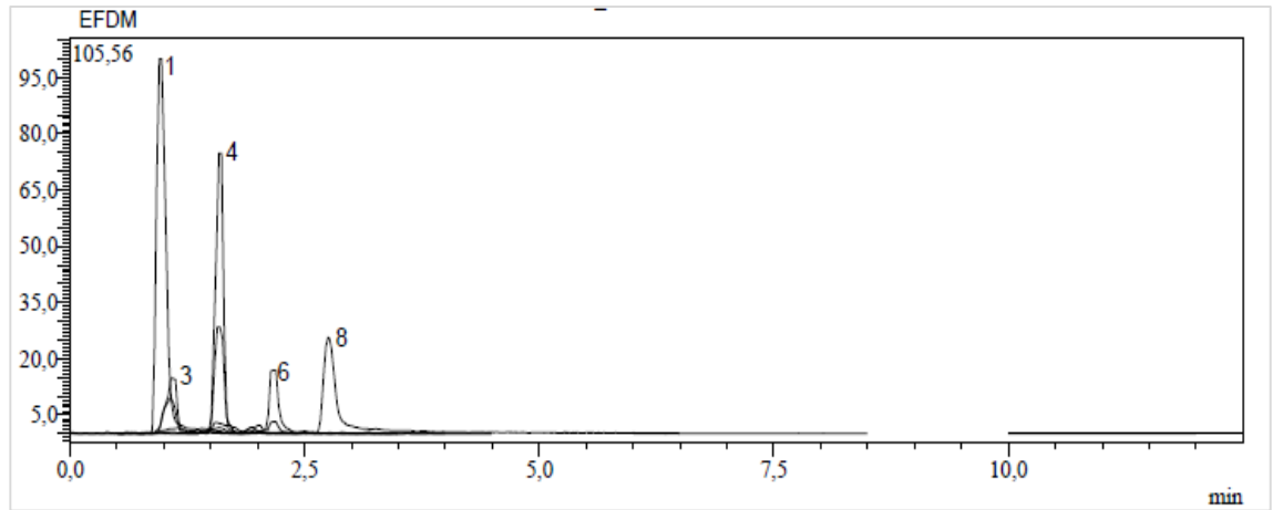
Ek 101. E. falcata 'nın karışık kısmının metanol ekstresinin kromatogramı
