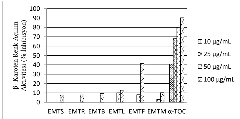
Ek 33. E. fistulosa 'nın \beta -karoten renk açılım aktivitesi
