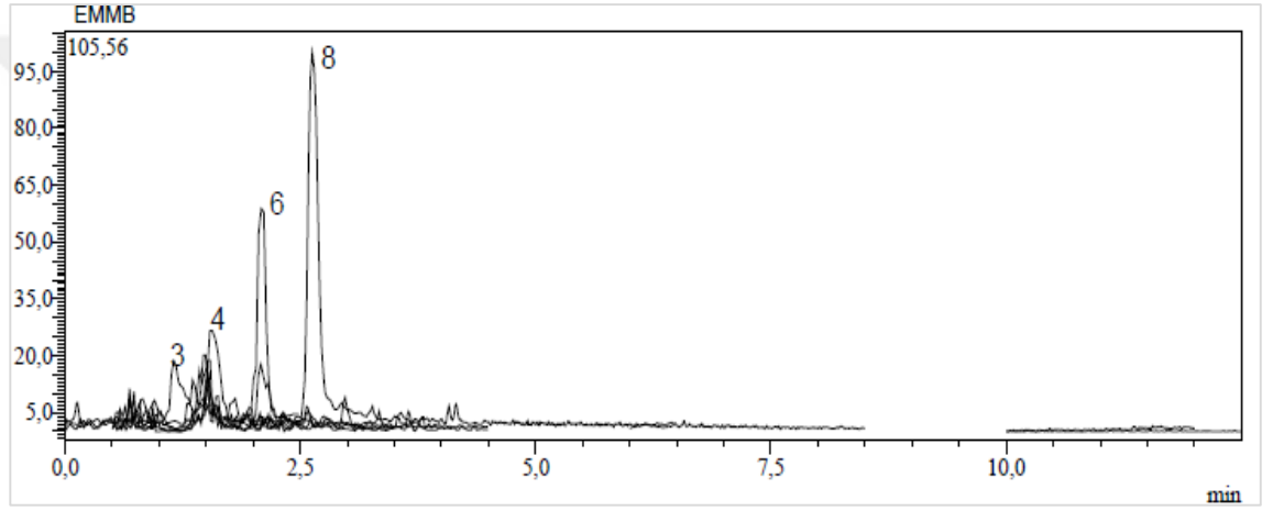
Ek 82. Malatya'dan toplanan E. macroclada 'nın dal kısmının metanol ekstresinin kromatogramı
