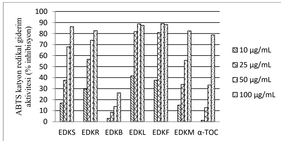
Ek 3. E. denticulata 'nın ABTS kasyon radikali giderim aktivitesi
