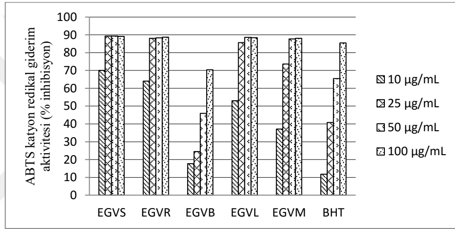
Ek 8. E. grisophylla 'nın ABTS katyon radikali giderim aktivitesi
