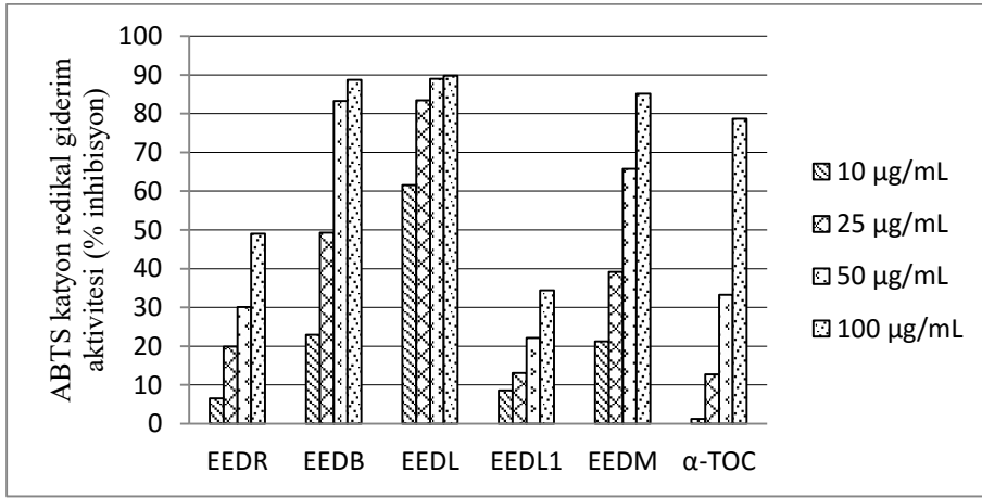
Ek 5. E. eriophora 'nın ABTS katyon radikali giderim aktivitesi
