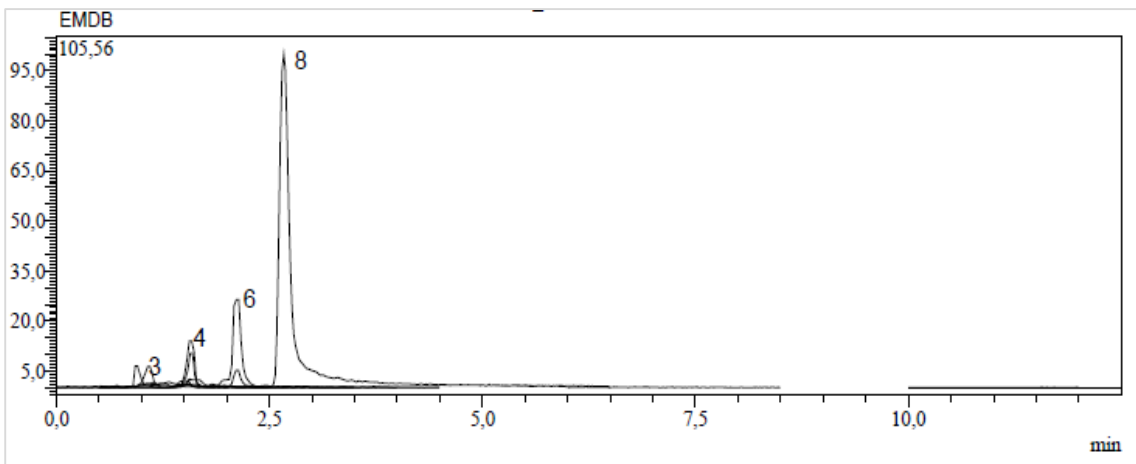
Ek 98. Diyarbakır'dan toplanan E. macroclada 'nın dal kısmının metanol ekstresinin kromatogramı
