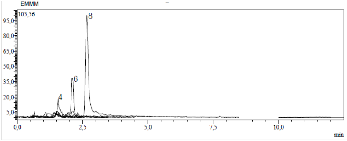
Ek 85. Malatya'dan toplanan E. macroclada 'nın karışık kısmının metanol ekstresinin kromatogramı
