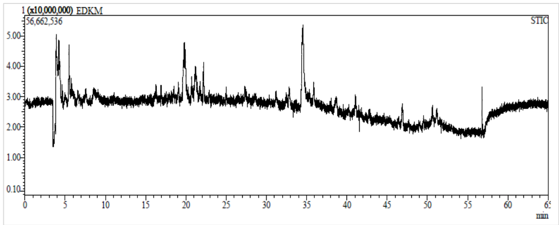
Ek 131. E. denticulata 'nın karışık kısmının metanol ekstresinin LC- MS IT- TOF kromatogramı
