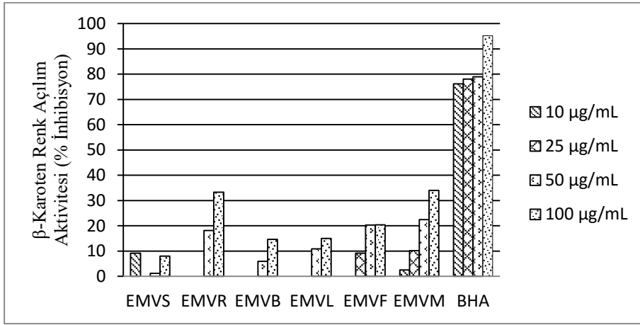
Ek 29. Van'dan toplanan E. macroclada 'nın \beta -karoten renk açılım aktivitesi
