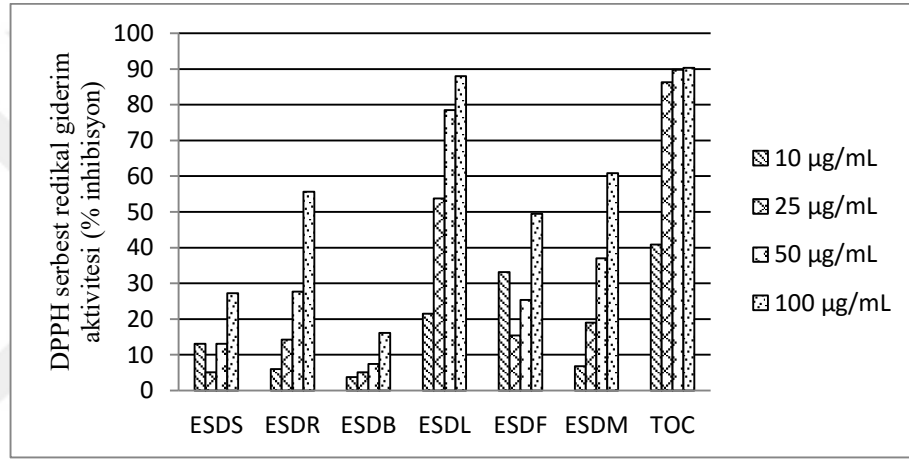
Ek 20. E. seguieriana subsp. seguieriana 'nın DPPH serbest radikali giderim aktivitesi
