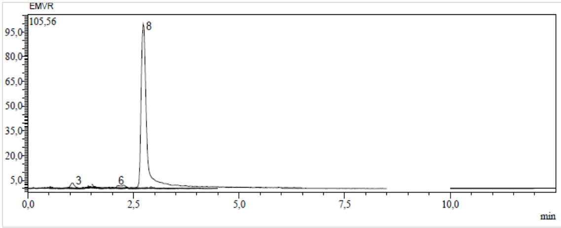
Ek 103. Van'dan toplanan E. macroclada 'nın kök kısmının metanol ekstresinin kromatogramı
