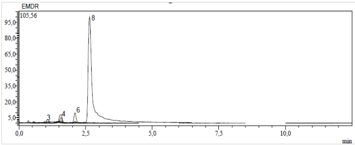
Ek 97. Diyarbakır'dan toplanan E. macroclada 'nın kök kısmının metanol ekstresinin kromatogramı
