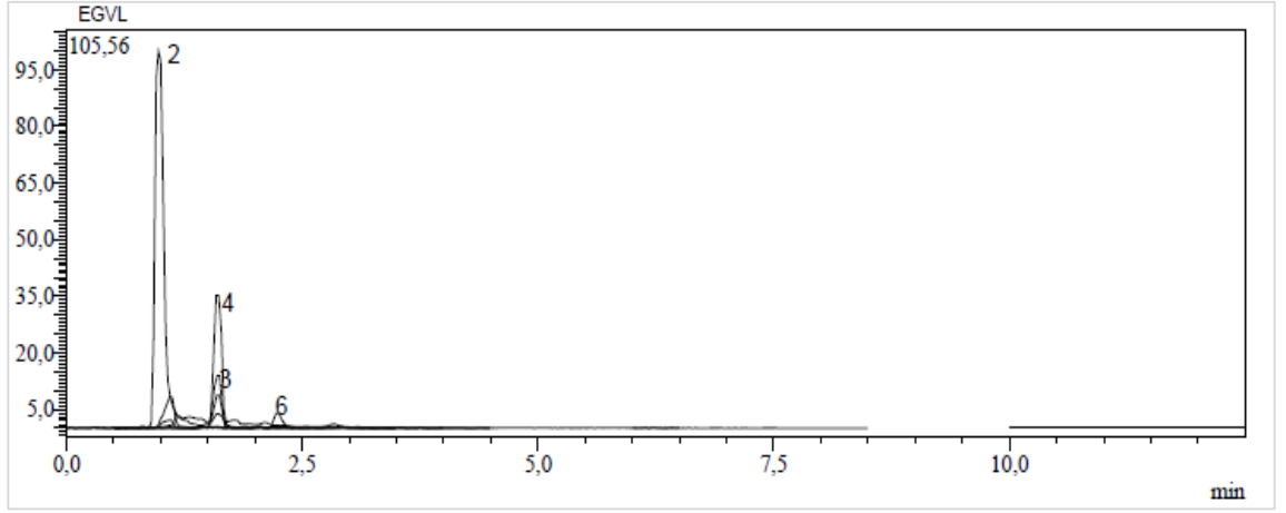
Ek 111. E. grisophylla 'nın yaprak kısmının metanol ekstresinin kromatogramı
