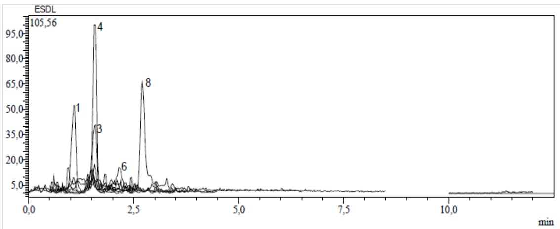
Ek 116. E. seguieriana subsp. seguieriana 'nın yaprak kısmının metanol ekstresinin kromatogramı
