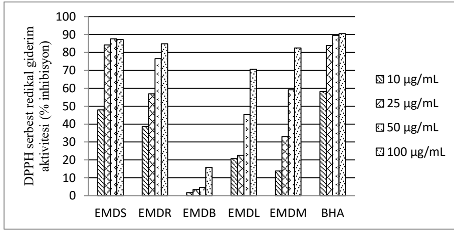
Ek 17. Diyarbakır'dan toplanan E. macroclada DPPH serbest radikali giderim aktivitesi
