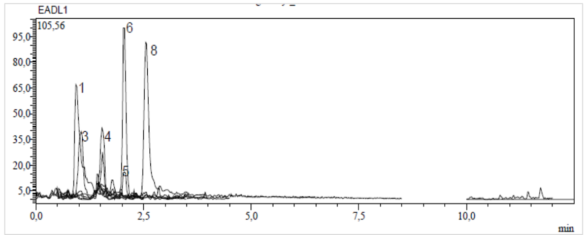
Ek 89. E. aleppica 'nın olgunlaşmamış yaprak kısmının metanol ekstresinin kromatogramı
