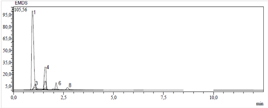
Ek 96. Diyarbakır'dan toplanan E. macroclada 'nın tohum kısmının metanol ekstresinin kromatogramı
