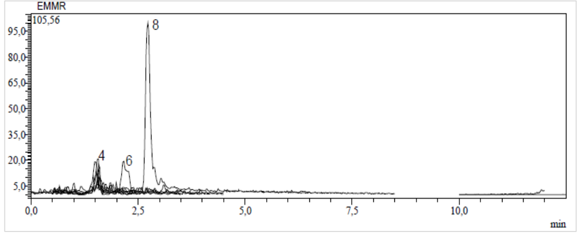
Ek 81. Malatya'dan toplanan E. macroclada 'nın kök kısmının metanol ekstresinin kromatogramı
