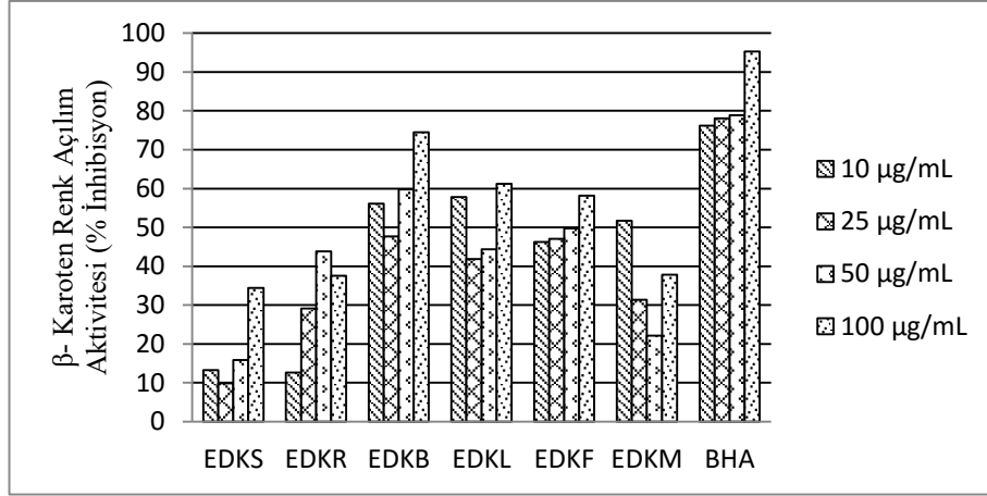
Ek 25. E. denticulata 'nın \beta -karoten renk açılım aktivitesi
