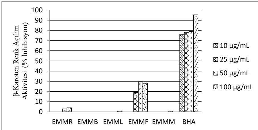
Ek 24. Malatya'dan toplanan E. macroclada 'nın β-karoten renk açılım aktivitesi
