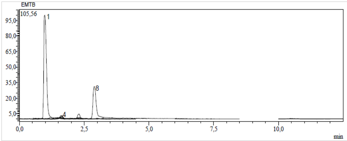
Ek 121. Trabzon'dan toplanan E. macroclada 'nın dal kısmının metanol ekstresinin kromatogramı
