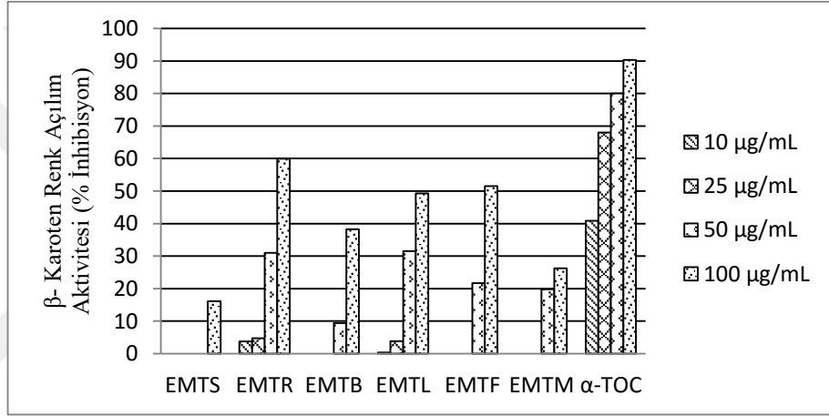
Ek 32. Trabzon'dan toplanan E. macroclada 'nın \beta -karoten renk açılım aktivitesi
