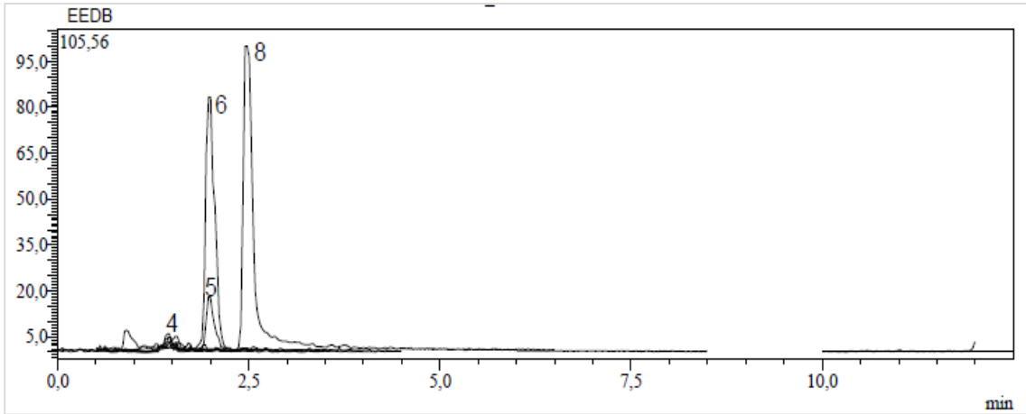
Ek 92. E. eriophora 'nın dal kısmının metanol ekstresinin kromatogramı
