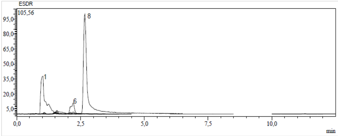
Ek 114. E. seguieriana subsp. seguieriana 'nın kök kısmının metanol ekstresinin
