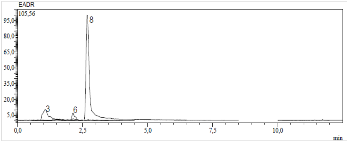
Ek 86. E. aleppica 'nın kök kısmının metanol ekstresinin kromatogramı
