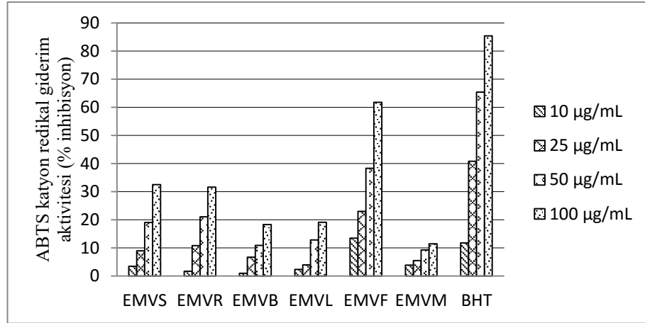
Ek 7. Van'dan toplanan E. macroclada 'nın ABTS katyon radikali giderim aktivitesi
