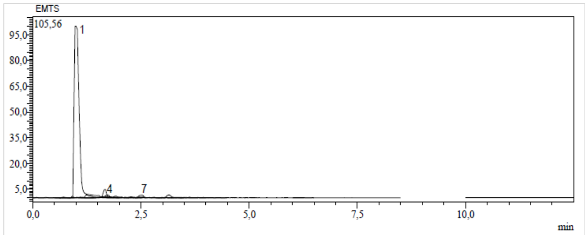
Ek 119. Trabzon'dan toplanan E. macroclada 'nın tohum kısmının metanol ekstresinin kromatogramı
