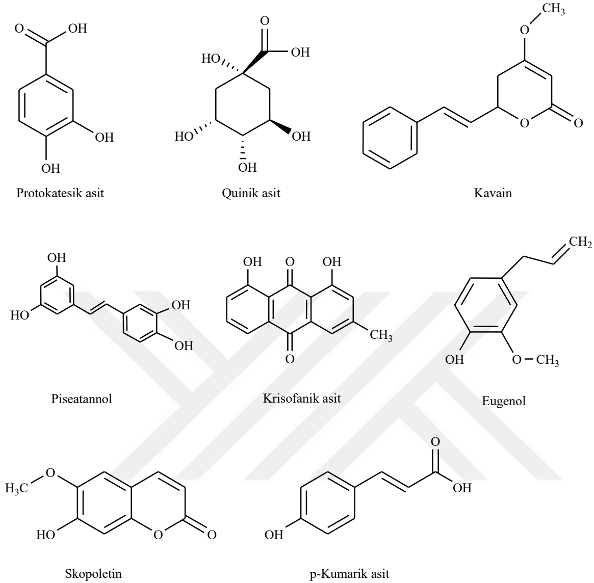
Şekil 3.6. LC-MS/MS metodunda kullanılan kimyasalların molekül yapıları
