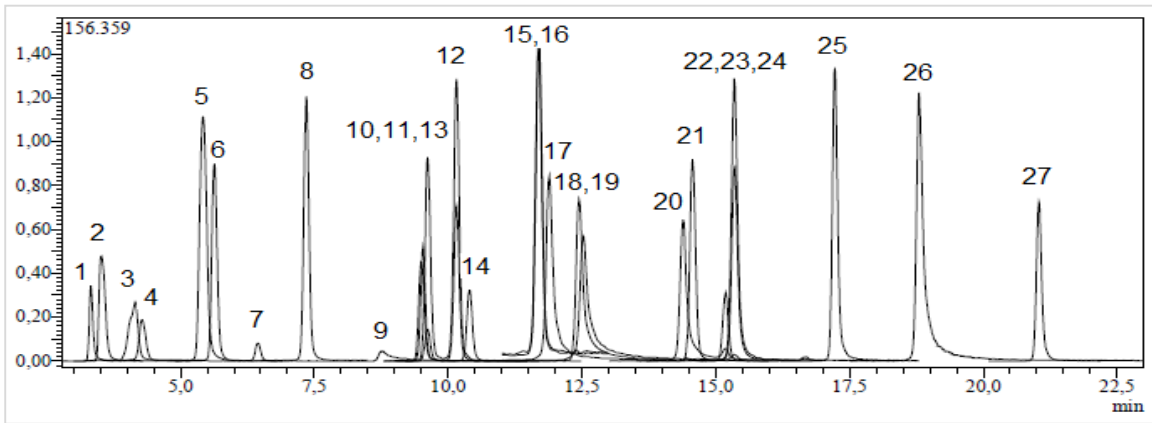
Şekil 4.8. 27 Fitokimyasal maddenin UHPLC-ESI-MS/MS kalibrasyon noktası 5'in standart kromatogramı
