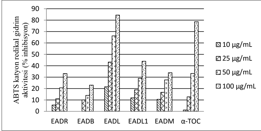
Ek 4. E. aleppica 'nın ABTS katyon radikali giderim aktivitesi
