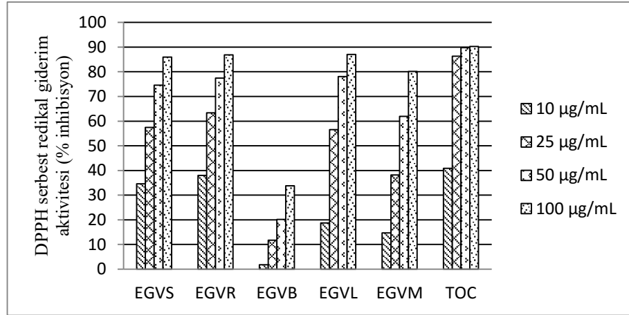
Ek 19. E. grisophylla 'nın DPPH serbest radikali giderim aktivitesi
