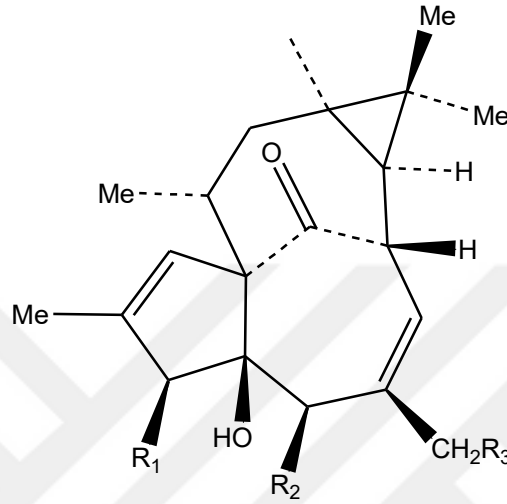
řekil 2.1. Ingenan diterpeninin iskelet yapısı (ingenol R 1 = R 2 = R 3 = OH)
