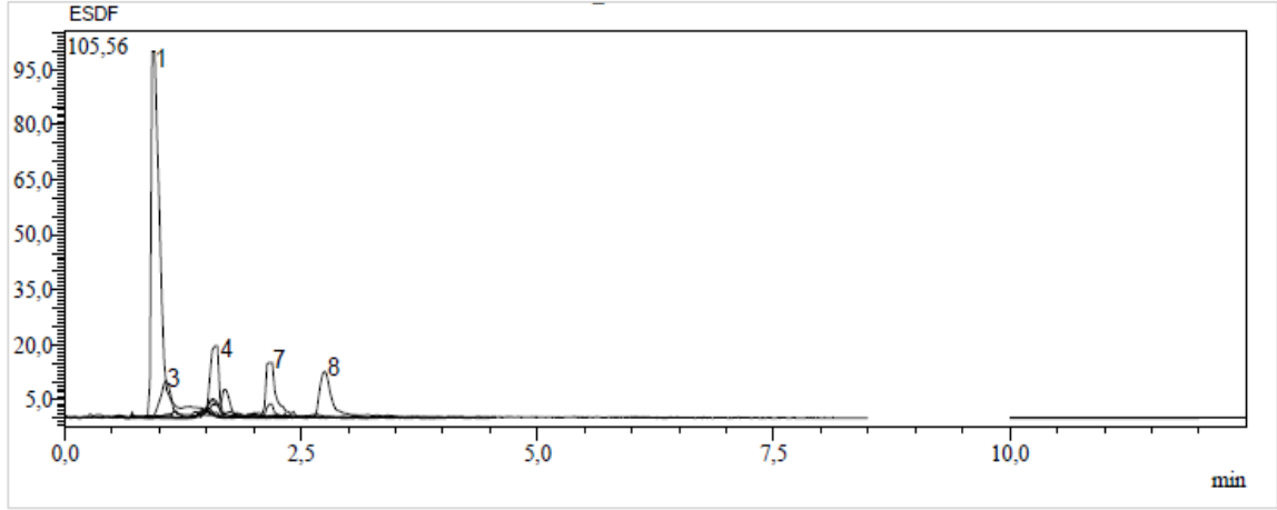
Ek 117. E. seguieriana subsp. seguieriana 'nın çiçek kısmının metanol ekstresinin kromatogramı
