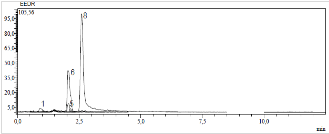
Ek 91. E. eriophora 'nın kök kısmının metanol ekstresinin kromatogramı
