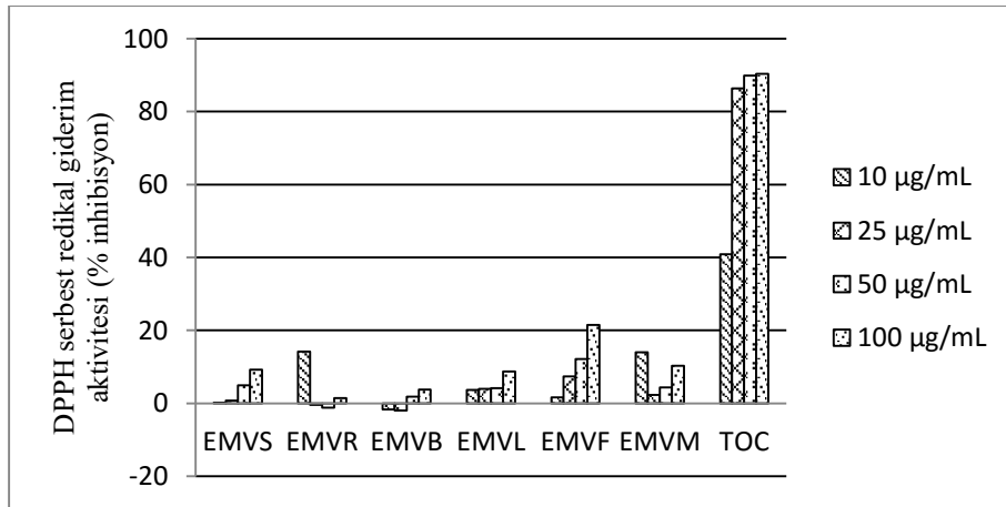
Ek 18. Van'dan toplanan E. macroclada 'nın DPPH serbest radikali giderim aktivitesi
