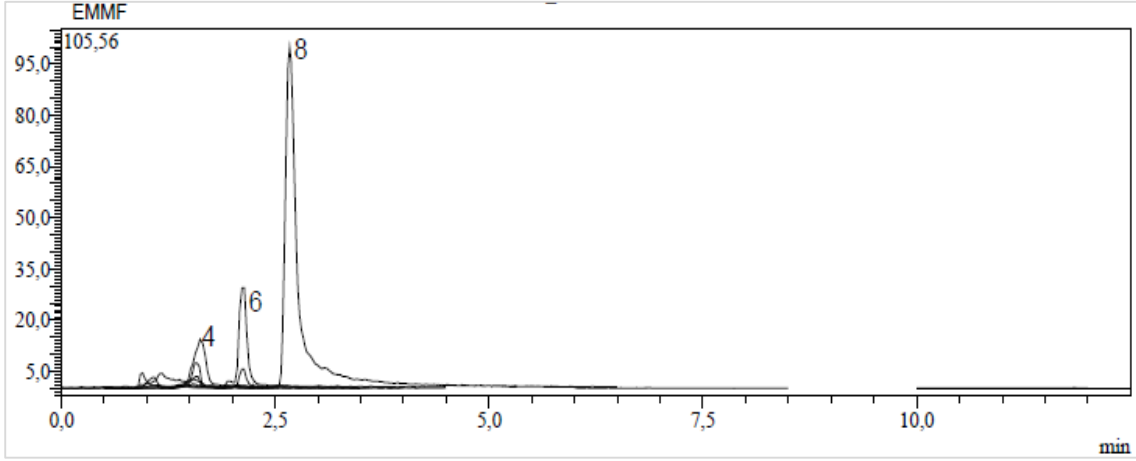
Ek 84. Malatya'dan toplanan E. macroclada 'nın çiçek kısmının metanol ekstresinin kromatogramı
