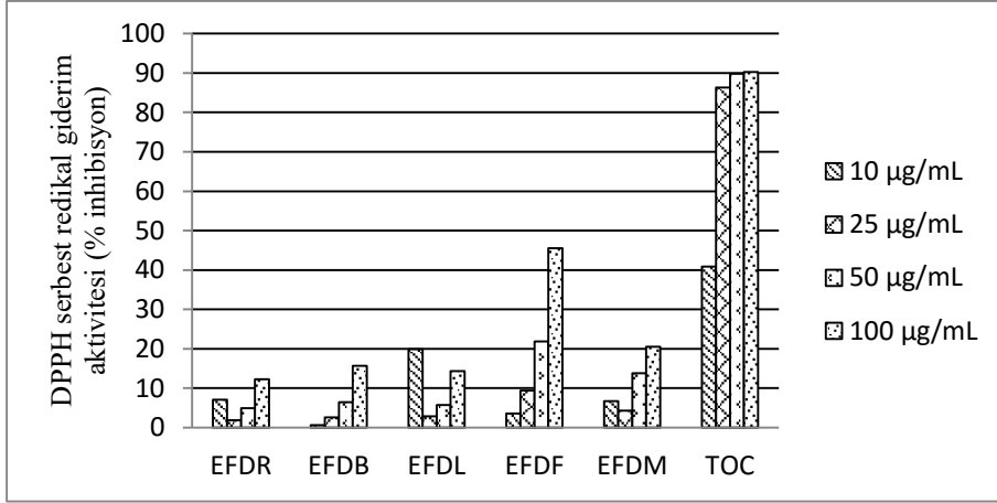
Ek 22. E. fistulosa 'nın DPPH serbest radikali giderim aktivitesi
