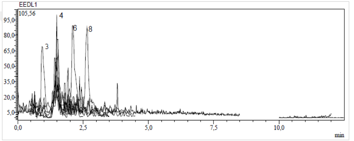
Ek 94. E. eriophora 'nın yaprak tozu kısmının metanol ekstresinin kromatogramı
