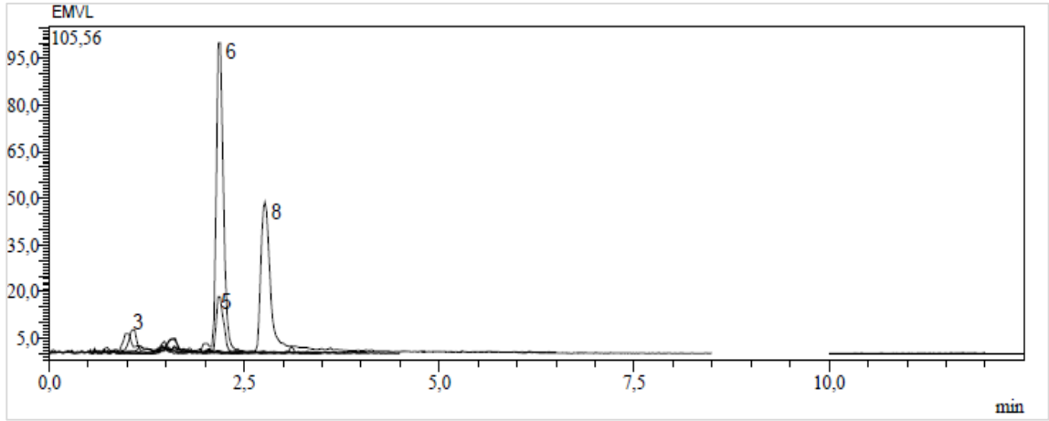
Ek 105. Van'dan toplanan E. macroclada 'nın yaprak kısmının metanol ekstresinin kromatogramı
