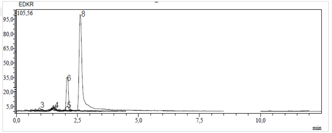
Ek 76. E. denticulata 'nın kök kısmının metanol ekstresinin kromatogramı
