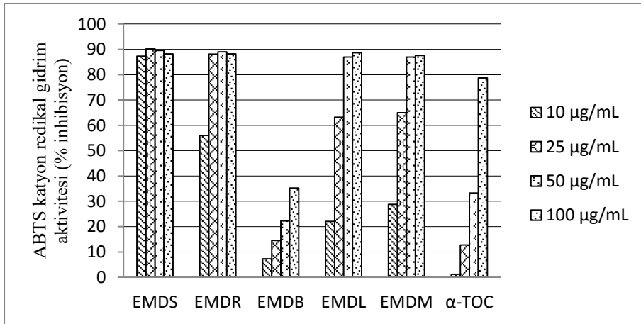
Ek 6. Diyarbakır'dan toplanan E. macroclada ABTS katyon radikali giderim aktivitesi
