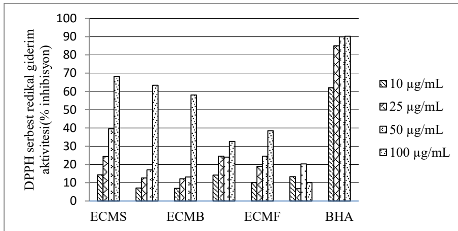
Ek 12. E. craspedia 'nin DPPH serbest radikali giderim aktivitesi
