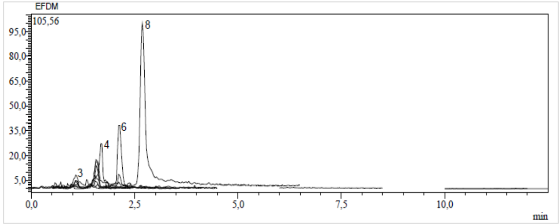
Ek 129. E. fistulosa 'nın karışık kısmının metanol ekstresinin kromatogramı
