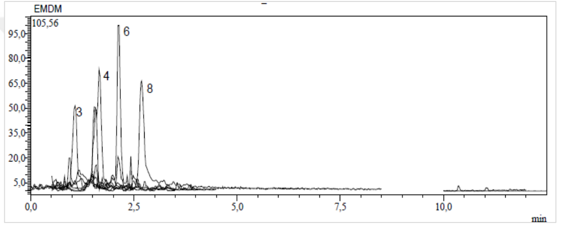
Ek 100. Diyarbakır'dan toplanan E. macroclada 'nın karışık kısmının metanol ekstresinin kromatogramı
