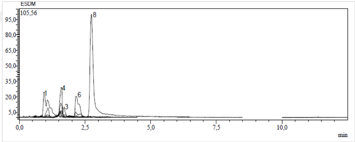
Ek 118. E. seguieriana subsp. seguieriana 'nın karışık kısmının metanol ekstresinin kromatogramı
