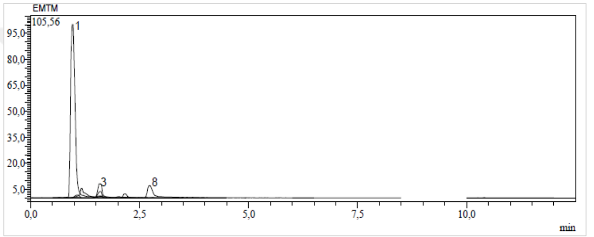
Ek 124. Trabzon'dan toplanan E. macroclada 'nın karışık kısmının metanol ekstresinin kromatogramı
