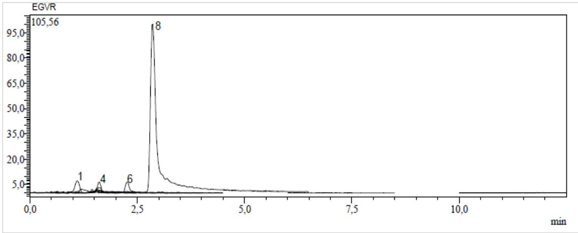
Ek 108. E. grisophylla 'nın tohum kısmının metanol ekstresinin kromatogramı
