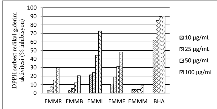
Ek 13. Malatya'dan toplanan E. macroclada 'nın DPPH serbest radikali giderim aktivitesi
