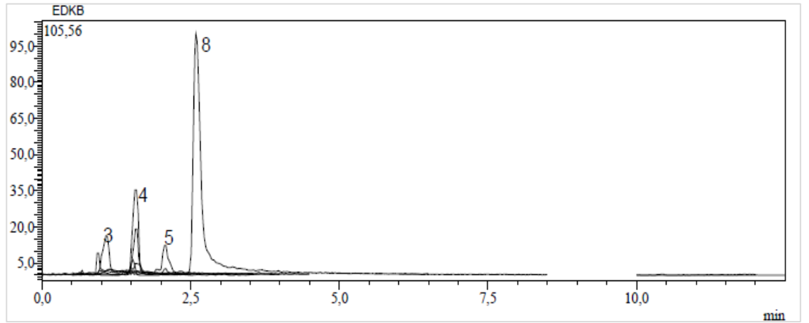
Ek 77. E. denticulata 'nın dal kısmının metanol ekstresinin kromatogramı
