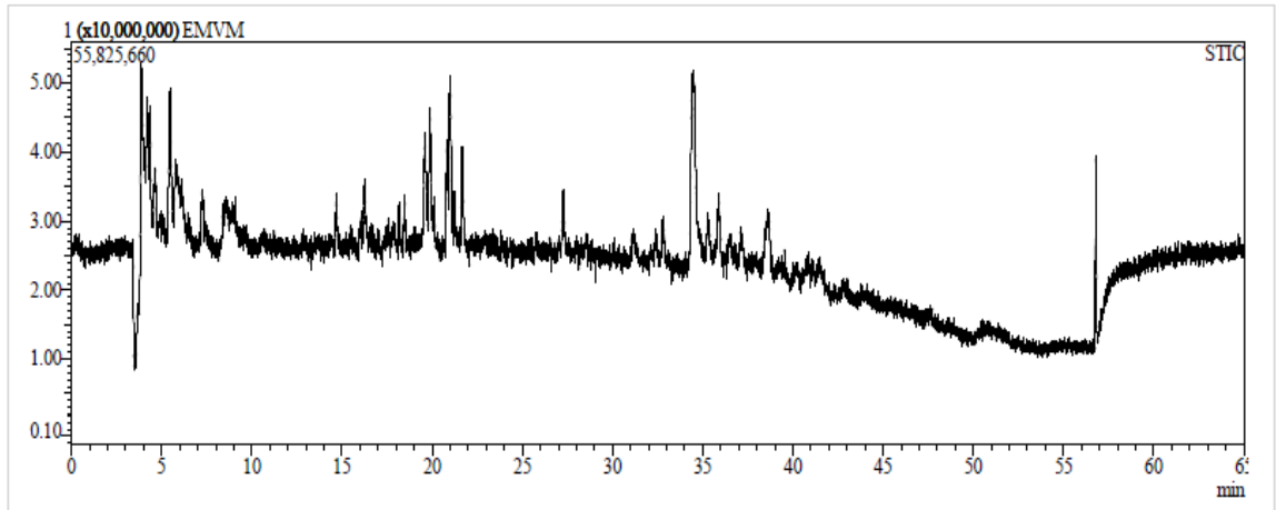
Ek 137. Van'dan toplanan E. macroclada 'nın karışık kısmının metanol ekstresinin LC- MS IT- TOF kromatogramı
