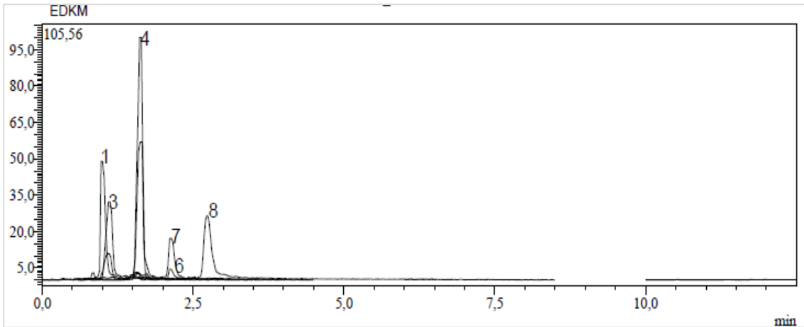
Ek 80. E. denticulata 'nın karışık kısmının metanol ekstresinin kromatogramı
