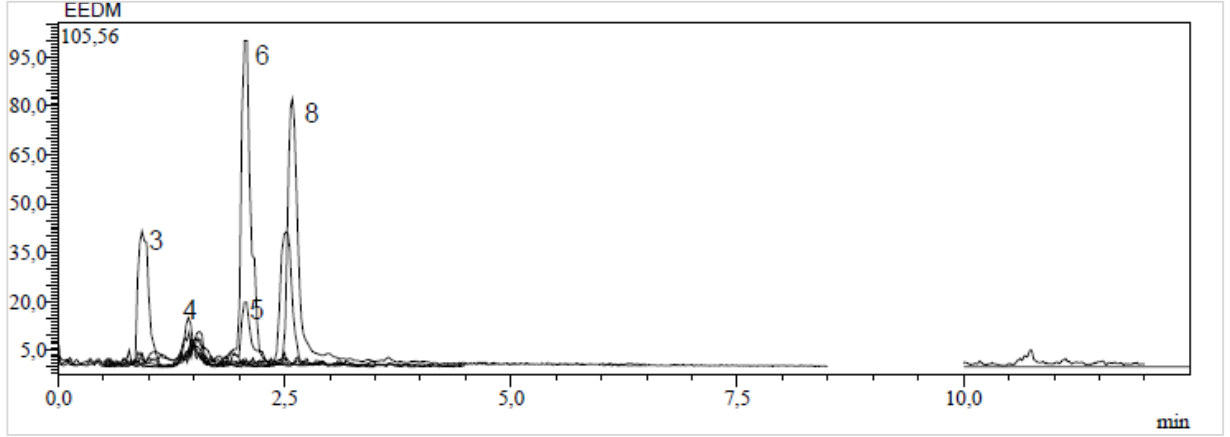
Şekil 4.7. E. eriophora karışık kısmının metanol ekstresinin standart kromatogramı
