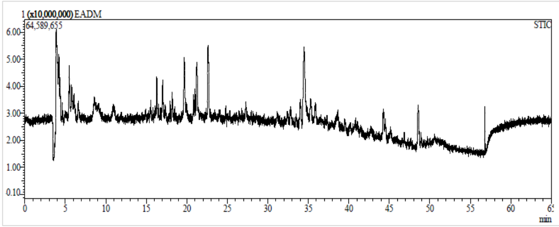
Ek 133. E. aleppica 'nın karışık kısmının metanol ekstresinin LC- MS IT- TOF kromatogramı
