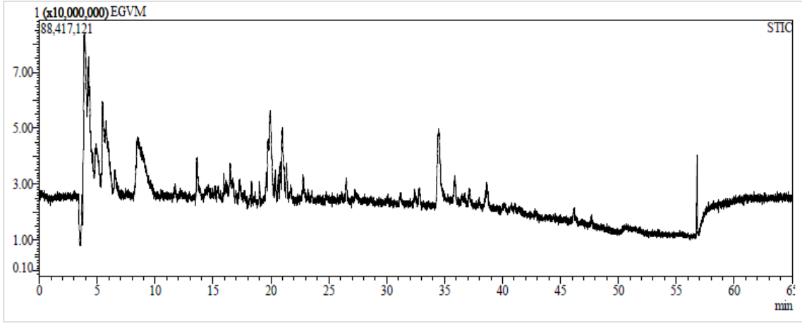
Ek 138. E. grisophylla 'nın karışık kısmının metanol ekstresinin LC- MS IT- TOF kromatogramı
