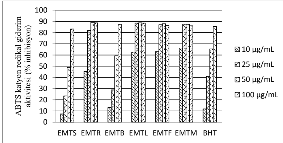
Ek 10. Trabzon'dan toplanan E. macroclada 'nın ABTS katyon radikali giderim aktivitesi
