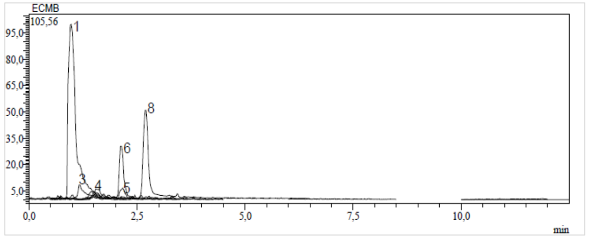
Ek 71. E. craspedia 'nın dal kısmının metanol ekstresinin kromatogramı
