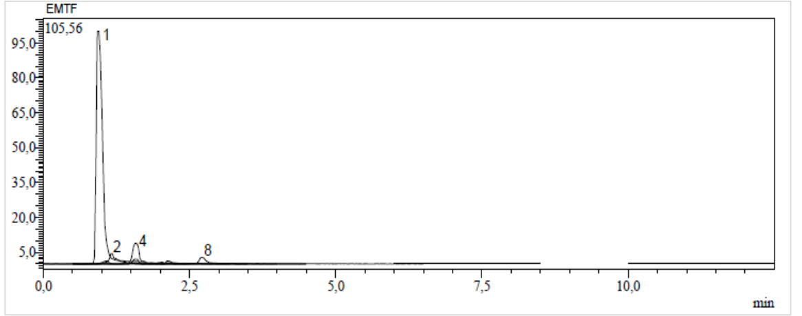
Ek 123. Trabzon'dan toplanan E. macroclada 'nın çiçek kısmının metanol ekstresinin kromatogramı
