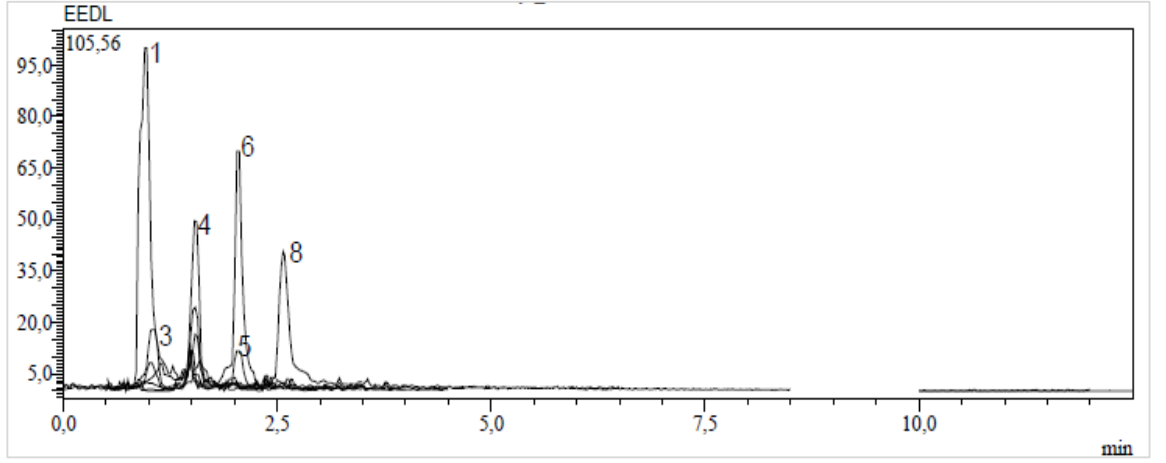
Ek 93. E. eriophora 'nın yaprak kısmının metanol ekstresinin kromatogramı
