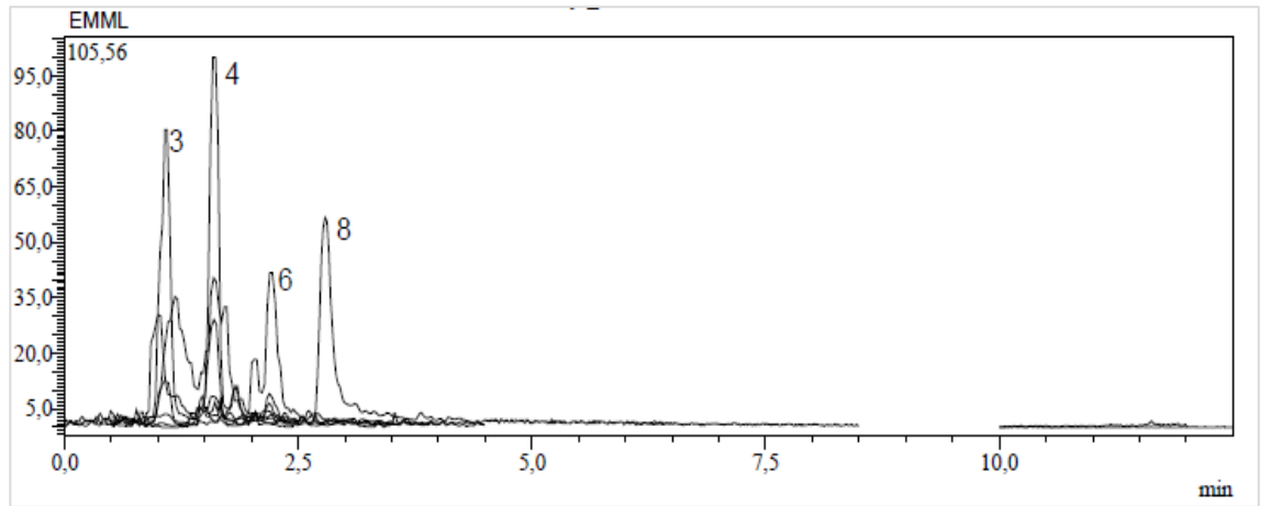
Ek 83. Malatya'dan toplanan E. macroclada 'nın yaprak kısmının metanol ekstresinin kromatogramı
