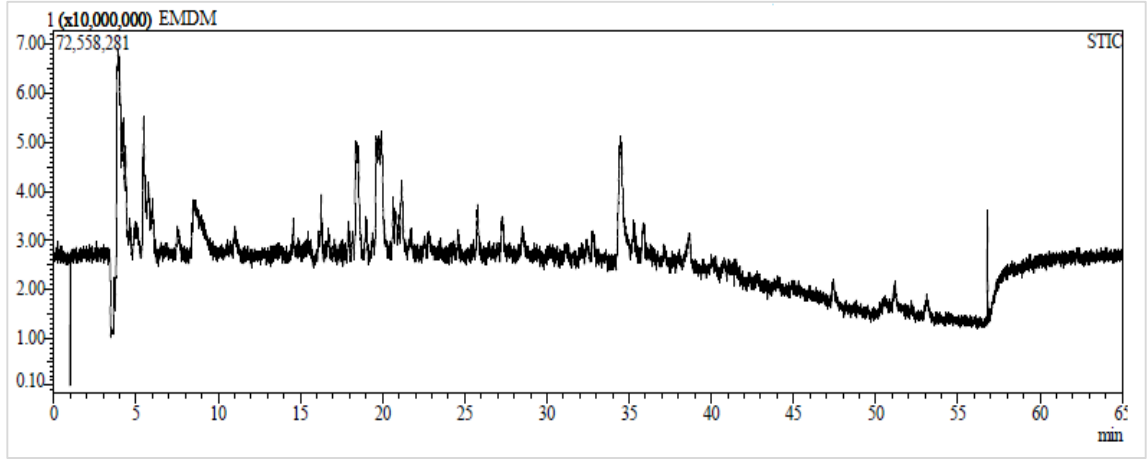
Ek 135. Diyarbakır'dan toplanan E. macroclada 'nın karışık kısmının metanol ekstresinin LC- MS IT- TOF kromatogramı
