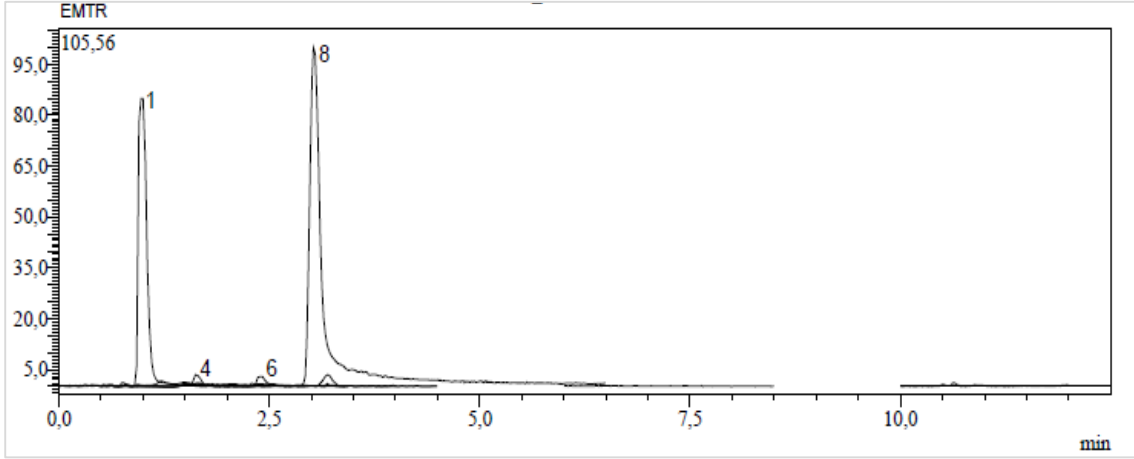
Ek 120. Trabzon'dan toplanan E. macroclada 'nın kök kısmının metanol ekstresinin kromatogramı
