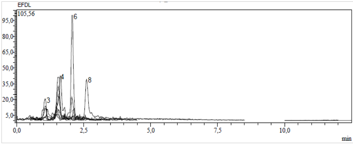
Ek 127. E. fistulosa 'nın yaprak kısmının metanol ekstresinin kromatogramı
