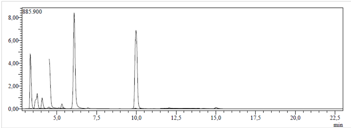
Şekil 4.9. Trabzon'dan toplanan E macroclada yaprak kısmının metanol ekstresinin standart kromatogramı
