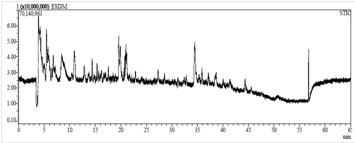
Ek 139. E. seguieriana subsp. seguieriana 'nın karışık kısmının metanol ekstresinin LC- MS IT- TOF kromatogramı
