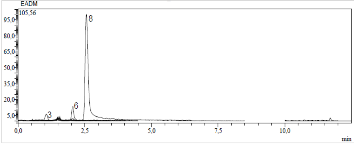
Ek 90. E. aleppica 'nın karışık kısmının metanol ekstresinin kromatogramı
