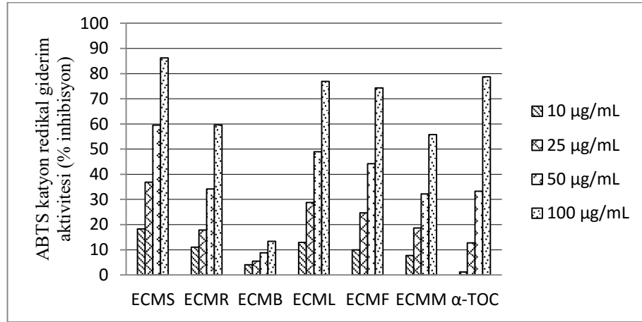
Ek 1. E. craspedia 'nın ABTS kasyon radikali giderim aktivitesi
