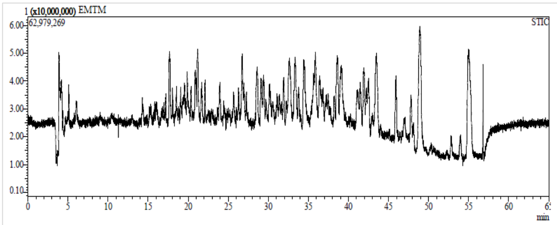
Ek 140. Trabzon'dan toplanan E. macroclada 'nın karışık kısmının metanol ekstresinin LC- MS IT- TOF kromatogramı
