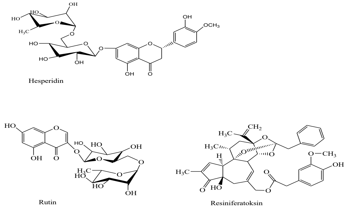
Şekil 3.5. LC-MS/MS metod validasyonu yapılan kimyasalların molekül yapıları
