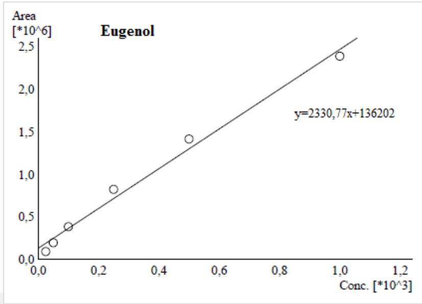
Şekil 4.5. LC-MS/MS metodundaki eugenol analitinin kalibrasyon grafiği
