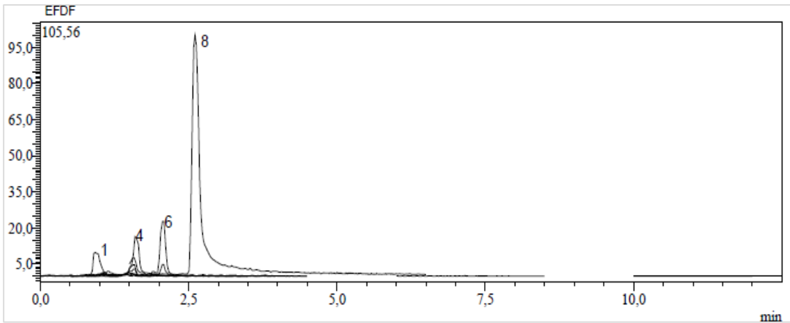
Ek 128. E. fistulosa 'nın çiçek kısmının metanol ekstresinin kromatogramı
