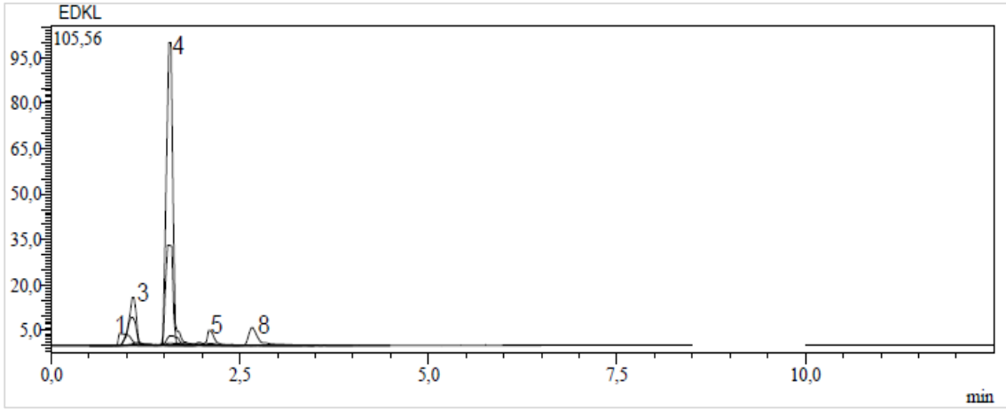
Ek 78. E. denticulata 'nın yaprak kısmının metanol ekstresinin kromatogramı
