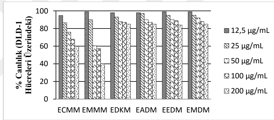
Şekil 4.3. ECMM, EMMM, EDKM, EADM, EEDM ve EMDM türlerinin kanserli hücre serisindeki stotoksik aktivitesi
