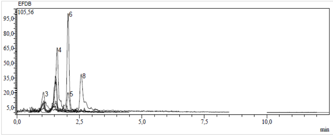
Ek 126. E. fistulosa 'nın dal kısmının metanol ekstresinin kromatogramı
