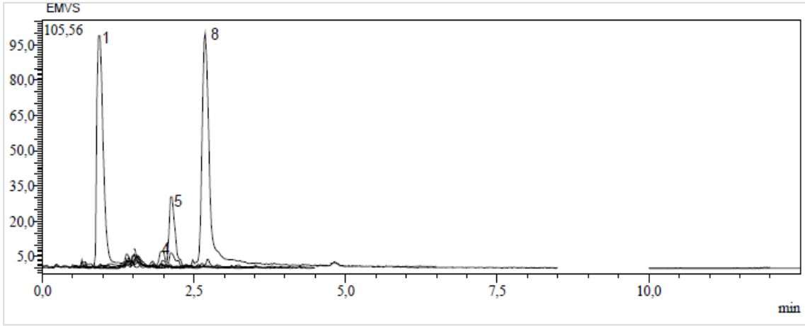
Ek 102. Van'dan toplanan E. macroclada 'nın tohum kısmının metanol ekstresinin kromatogramı
