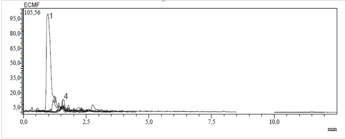
Ek 73. E. craspedia 'nın çiçek kısmının metanol ekstresinin kromatogramı
