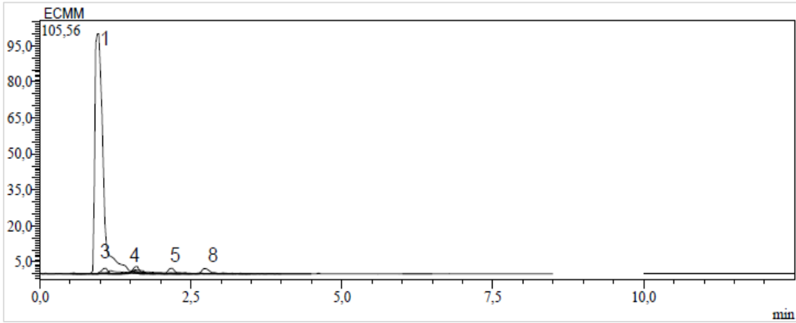
Ek 74. E. craspedia 'nın karışık kısmının metanol ekstresinin kromatogramı
