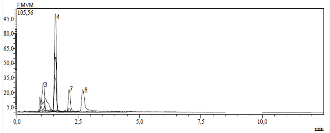
Ek 107. Van'dan toplanan E. macroclada 'nın karışık kısmının metanol ekstresinin kromatogramı
