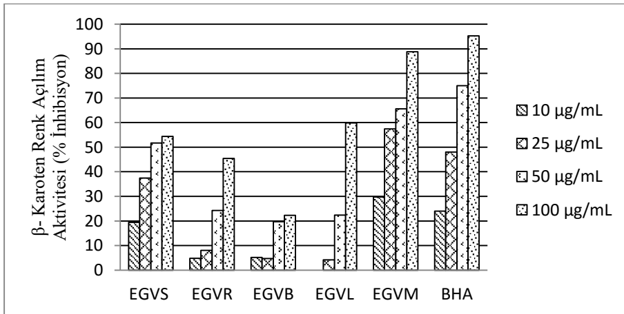
Ek 30. E. grisophylla 'nın \beta -karoten renk açılım aktivitesi
