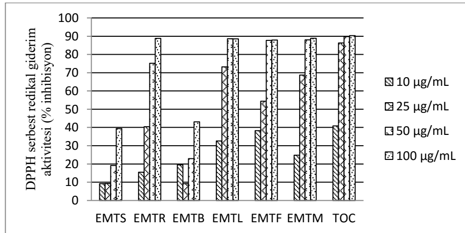
Ek 21. Trabzon'dan toplanan E. macroclada 'nın DPPH serbest radikali giderim aktivitesi
