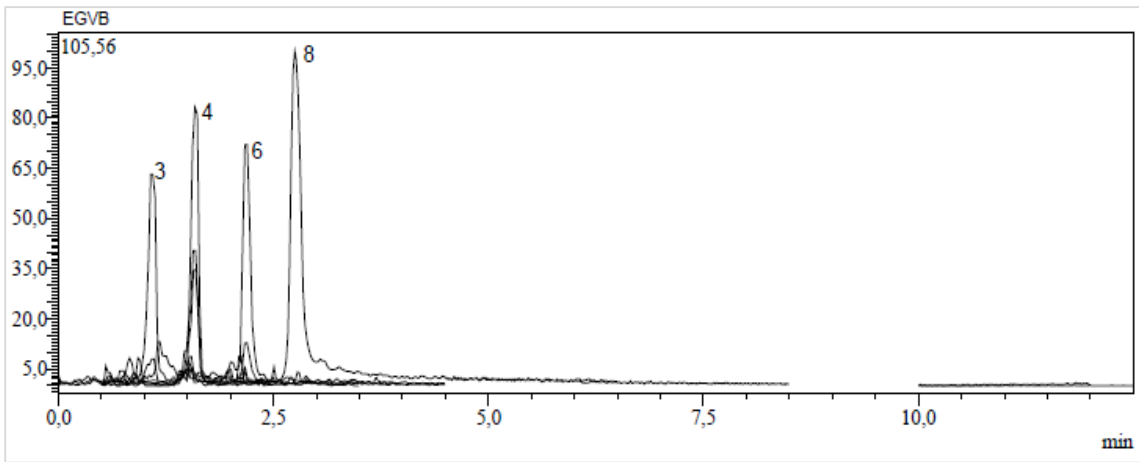
Ek 110. E. grisophylla 'nın dal kısmının metanol ekstresinin kromatogramı
