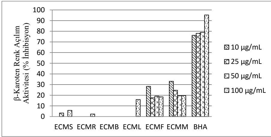
Ek 23. E. craspedia 'nın β-karoten renk açılım aktivitesi
