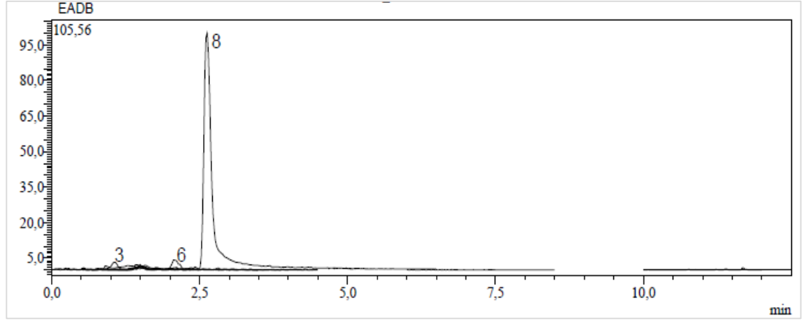
Ek 87. E. aleppica 'nın dal kısmının metanol ekstresinin kromatogramı
