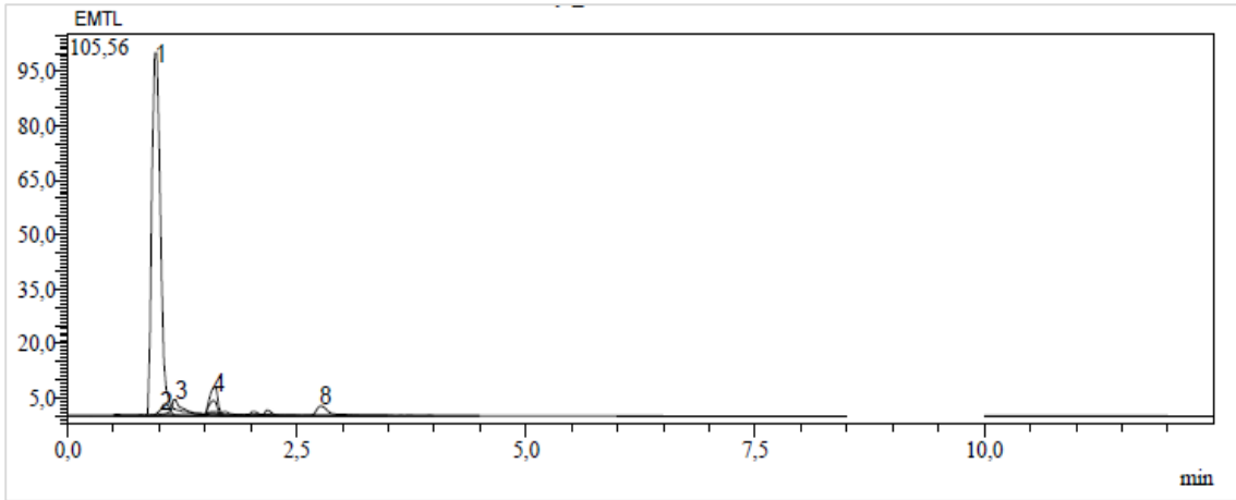
Ek 122. Trabzon'dan toplanan E. macroclada 'nın yaprak kısmının metanol ekstresinin kromatogramı
