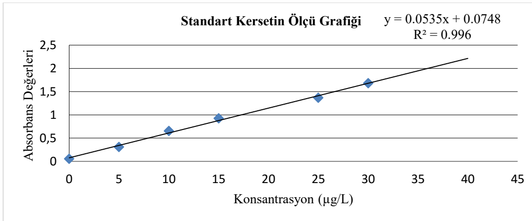
Şekil 3.4. Standart kersetinin ölçü grafiği
