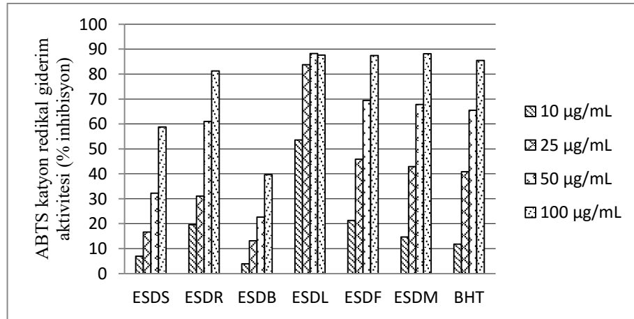
Ek 9. E. seguieriana subsp. seguieriana 'nın ABTS katyon radikali giderim aktivitesi
