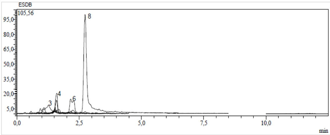
Ek 115. E. seguieriana subsp. seguieriana 'nın dal kısmının metanol ekstresinin kromatogramı
