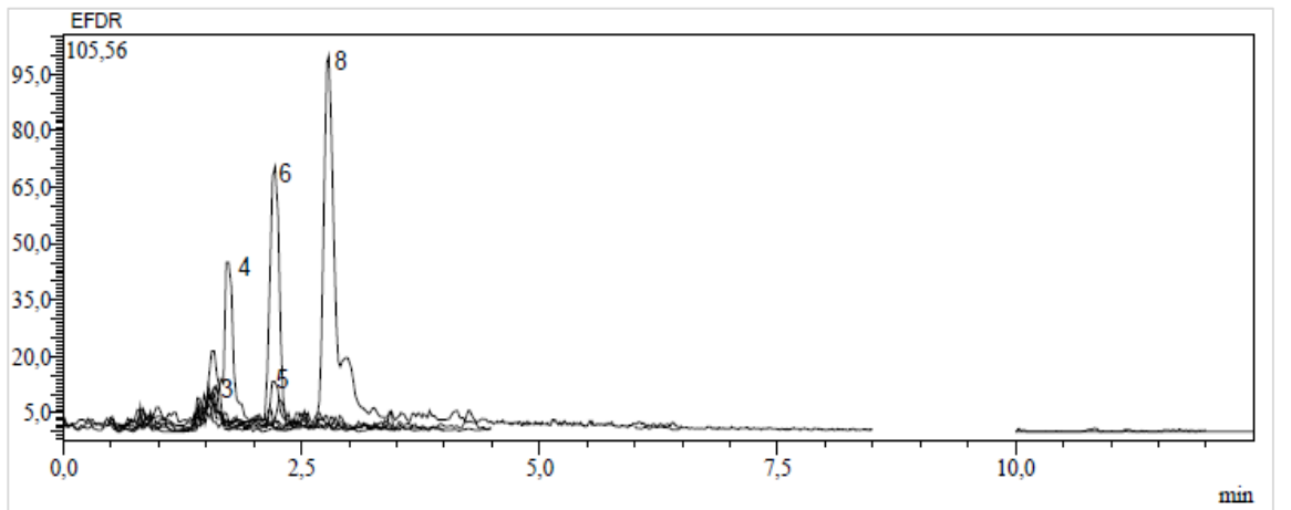
Ek 125. E. fistulosa 'nın kök kısmının metanol ekstresinin kromatogramı
