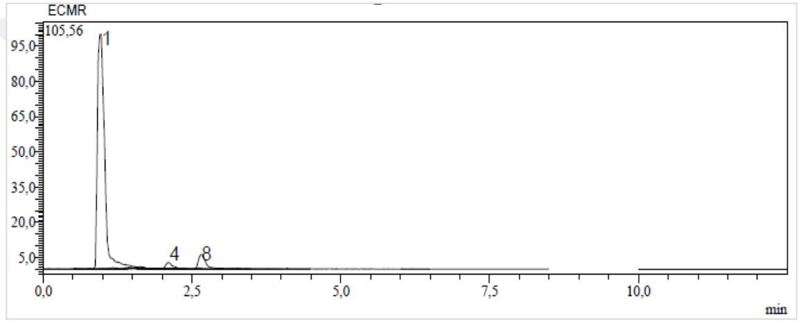
Ek 70. E. craspedia 'nın kök kısmının metanol ekstresinin kromatogramı
