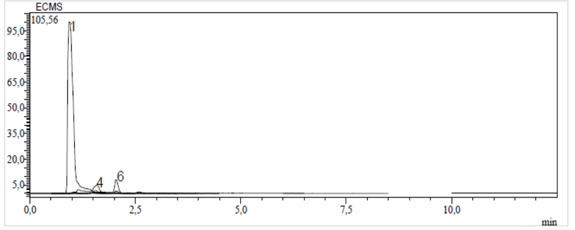
Ek 69. E. craspedia 'nın tohum kısmının metanol ekstresinin kromatogramı
