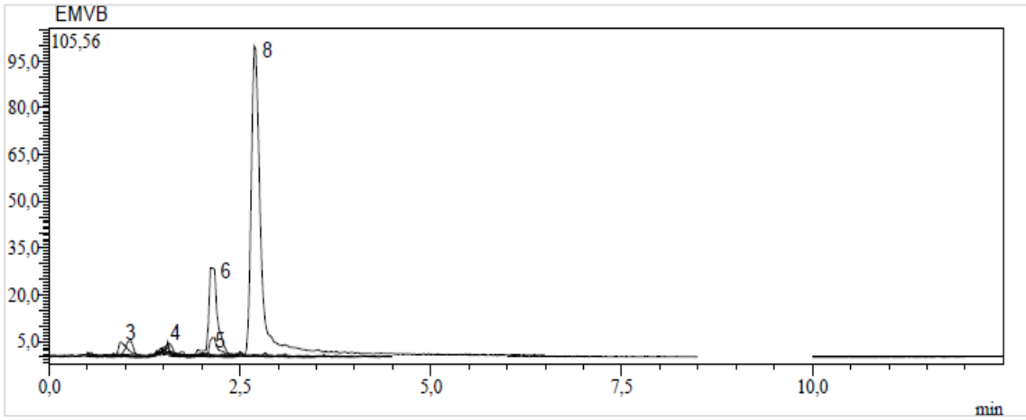
Ek 104. Van'dan toplanan E. macroclada 'nın dal kısmının metanol ekstresinin kromatogramı
