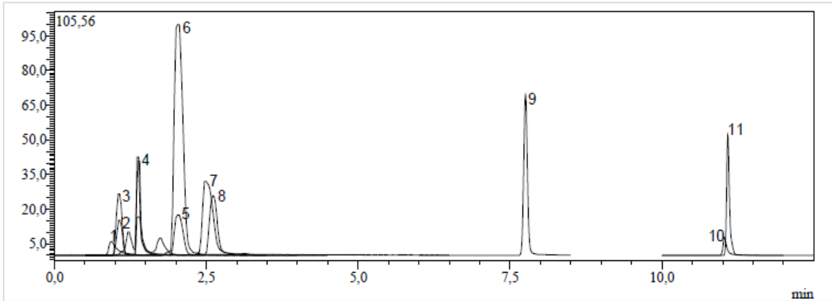
Şekil 4.6. Kalibrasyon noktası 5'in standart kromatogramı
