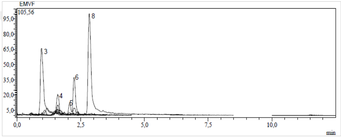
Ek 106. Van'dan toplanan E. macroclada 'nın çiçek kısmının metanol ekstresinin kromatogramı
