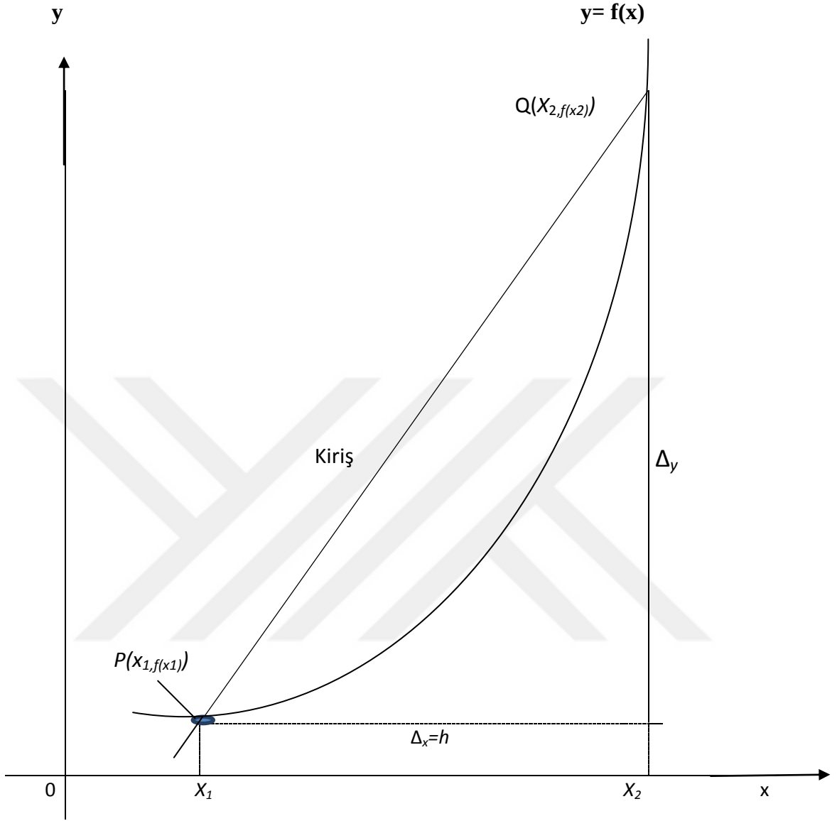
Grafik.1. y = f(x) grafiğinin bir kirişi. Eğimi \frac{\Delta y}{\Delta x} , f' 'nin [x_1, x_2] aralığındaki ortalama değişim oranıdır.
