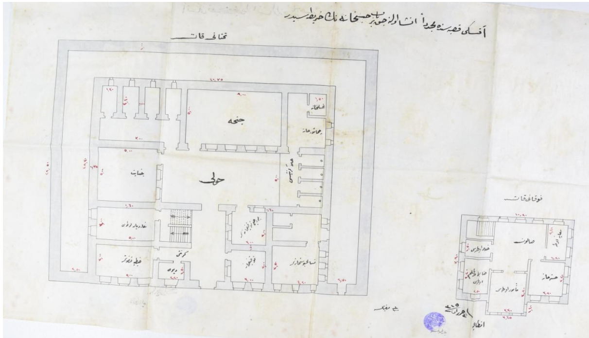
Akseki kazasında inşa edilecek olan hapishanenin planı (BOA, DH, TMIK. S, nr. 26/24, lef. 1.)
