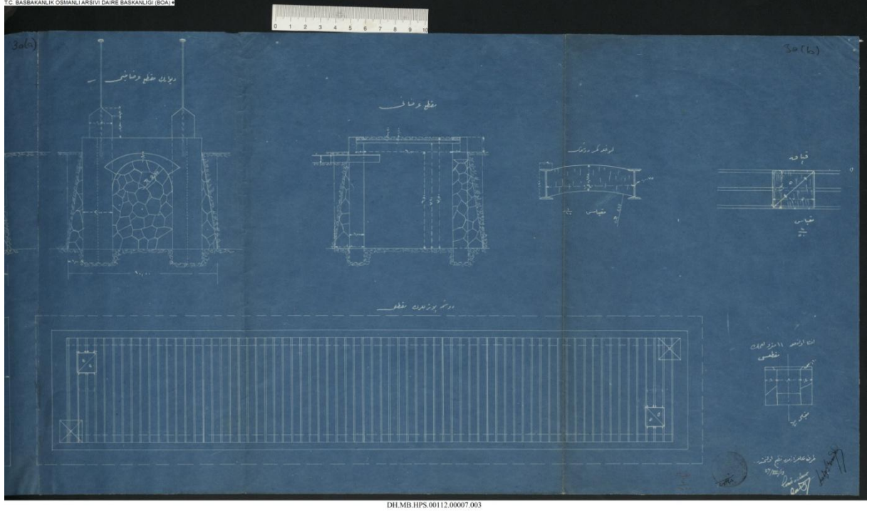
EK-XII: Bozkır Hapishanesinde yapılacak tamir ve inşaat faaliyetlerine dair kroki. BOA, DH. MB. HPS, 112. 7./3, Lef. 2.
