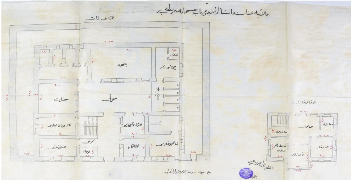
Alanya kazasında inşa edilecek olan hapishanenin planı. (BOA, DH. TMIK. S, nr. 26/14, lef. 37.)
