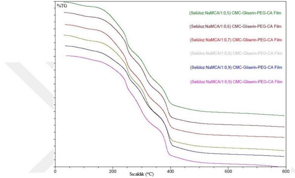
Şekil 5.9. Çeşitli Selüloz:NaMCA Oranlarında Sentezlenen CMC ile Hazırlanan Gliserin, PEG ve CA Katkılı Filmlerin TGA Sonucu
