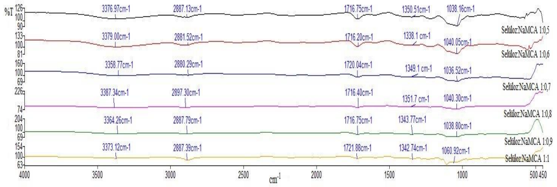
Şekil 5.5. Çeşitli Selulöz:NaMCA Oranlarında Sentezlenen CMC ile Hazırlanan Gliserin, PEG ve CA Katkılı Filmlerin FTIR Spektrumları
