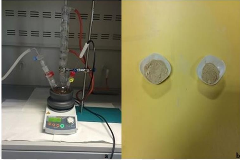
Görsel 4.2. Selülozun CMC'ye Dönüştürülmesinde Kullanılan Deney Düzeneği (a) ve Deneyler Sonucu Sentezlenen CMC (b)
