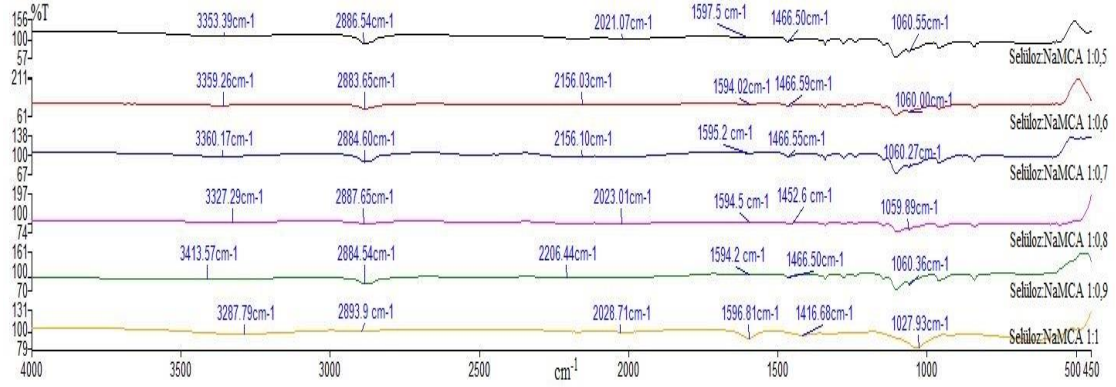
Şekil 5.4. Çeşitli Selüloz:NaMCA Oranlarında Sentezlenen CMC ile Hazırlanan Gliserin ve PEG Katkılı Filmlerin FTIR Spektrumları
