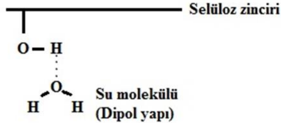
Şekil 2.3. Selülozun Su Molekülüne Hidrojen Köprüsü Oluşturarak Bağlanması [15]
