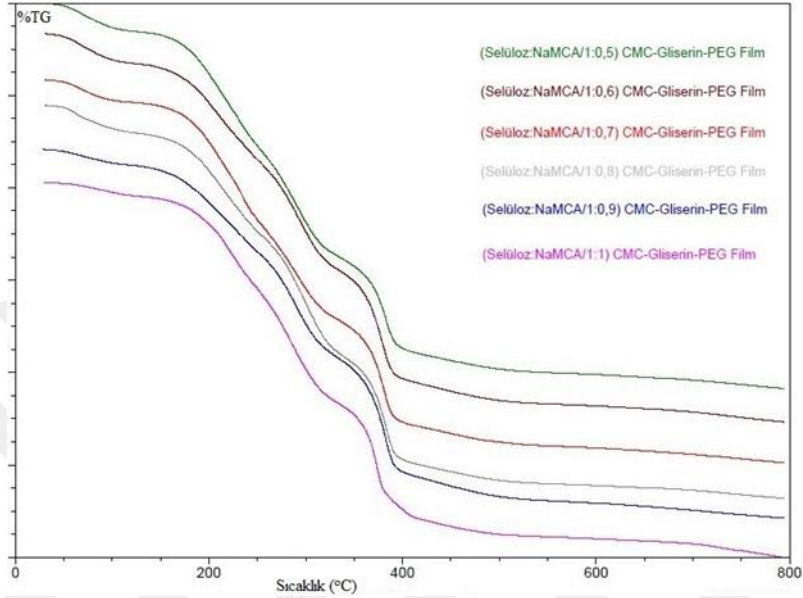
Şekil 5.8. Çeşitli Selüloz:NaMCA Oranlarında Sentezlenen CMC ile Hazırlanan Gliserin ve PEG Katkıli Filmlerin TGA Sonucu
