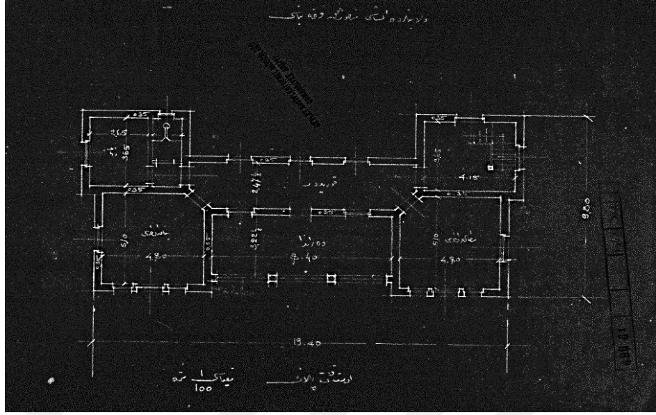
Şekil 3.25. Halkevi 1. Kat Planı [72]
