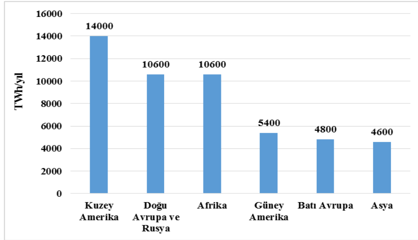
Şekil-17 Dünya Teknik Rüzgâr Potansiyelinin Bölgesel Dağılımı
