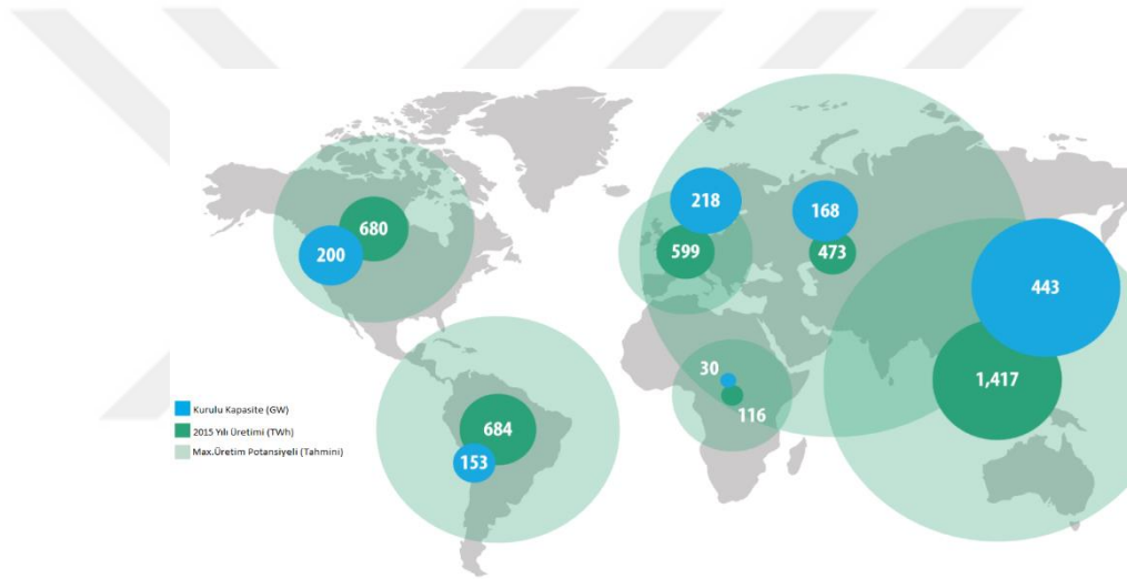
Şekil-12 Küresel Hidroelektrik Kurulu Kapasite, Elektrik Üretimi ve Teknik Potansiyeli
