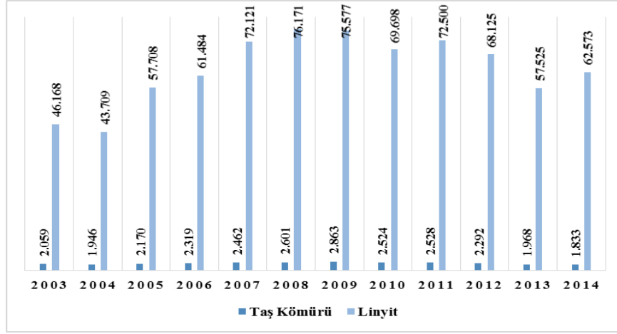
Şekil-3 2003-2014 Türkiye Yerli Kömür Üretimi (Bin Ton)
