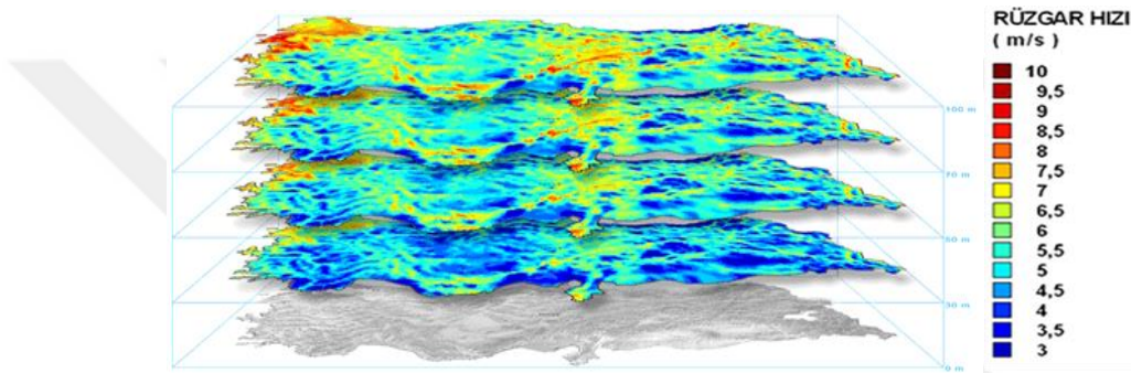
Şekil-19 Türkiye Rüzgâr Enerji Potansiyeli Atlası (REPA)
