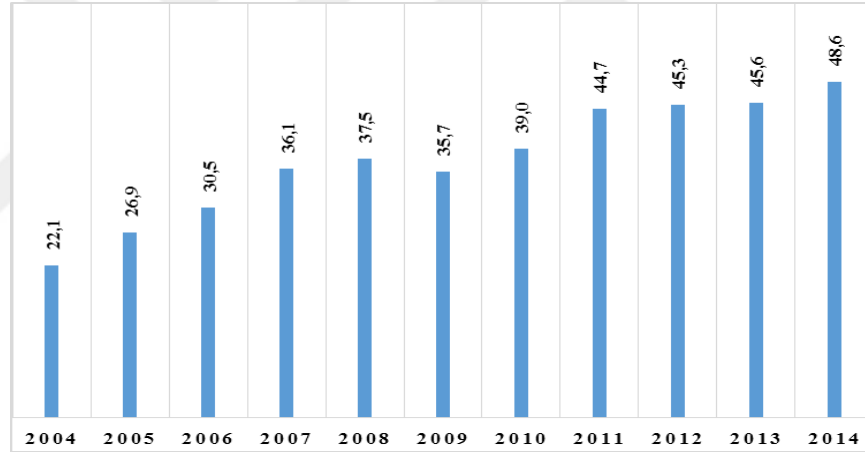
Şekil-8 2004-2014 Türkiye Doğal Gaz Tüketimi (Milyar m 3 )
