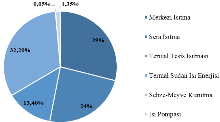
Şekil-16 Türkiye Jeotermal Enerjisi Doğrudan Kullanım Dağılımı
