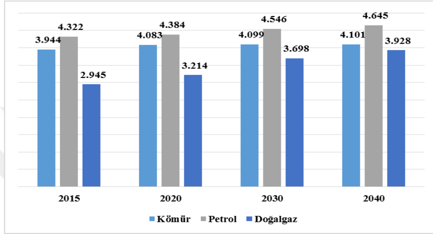
Şekil-1 Kömür, Petrol ve Doğal Gazın Enerji Kaynakları İçindeki Paylarının Değişimi (MTEP)
