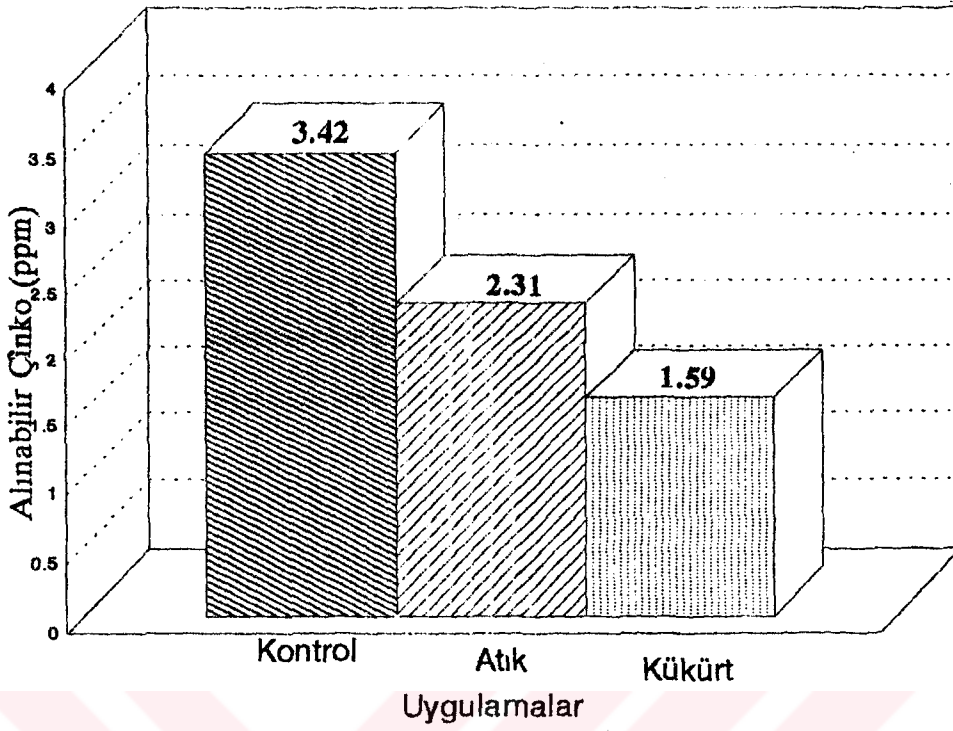
Şekil 4.7. Deneme Toprağının Uygulamaların Ortalamalarına Bağlı Olarak Alınabilir Çinko Kapsamının Kontrole Göre Değişimi
