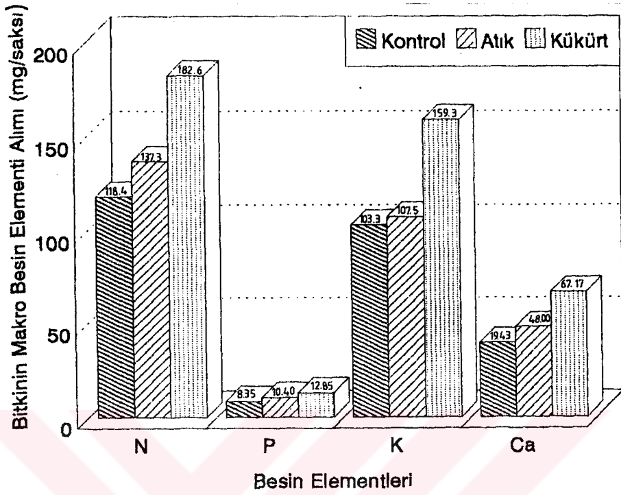
Şekil 4.8. Uygulamaların Ortalamalarına Bağlı Olarak Bitkinin Makro Besin Elementi Alımı
