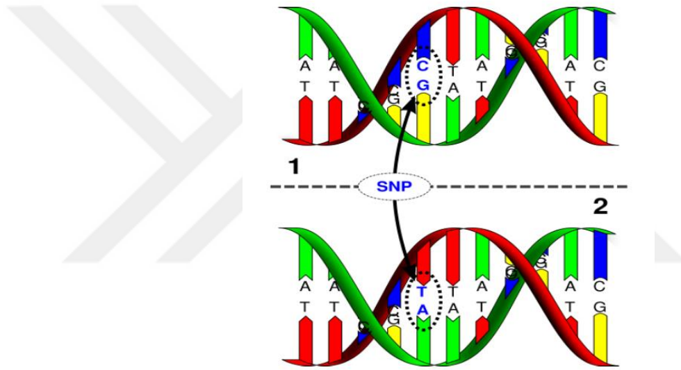
Şekil 11-Single Nucleotide Polymorphism-Tek Nükleotid Polimorfizm
