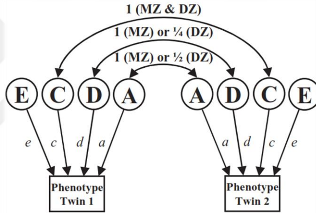
Şekil 10- Path Diyagramı İle Klasik İkiz Çalışması Modeli (Rijsdijk, 2002, 121)
