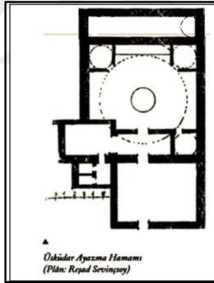
Şekil 26: Ayazma Hamamı Planı(Reşad Sevinçsoy'dan İşlenerek)
