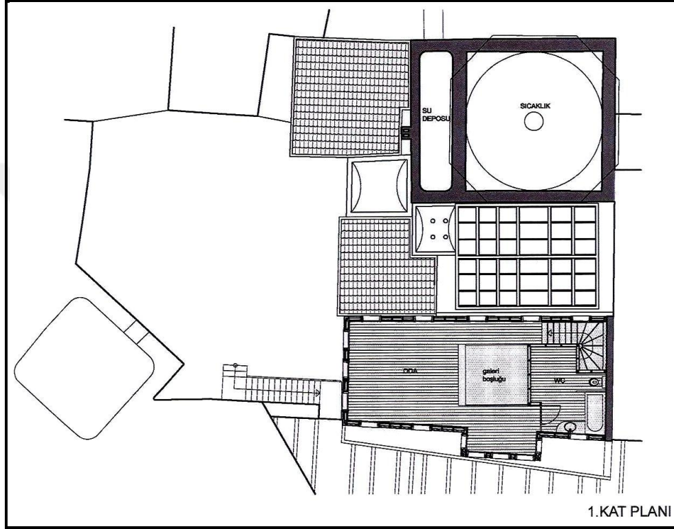
Şekil 40: Kuzguncuk Batak Hamam 1. Kat Planı (6.Kurul Arşivi)
