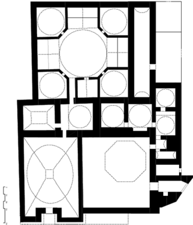
Şekil 19: Ağa Hamamı Planı
