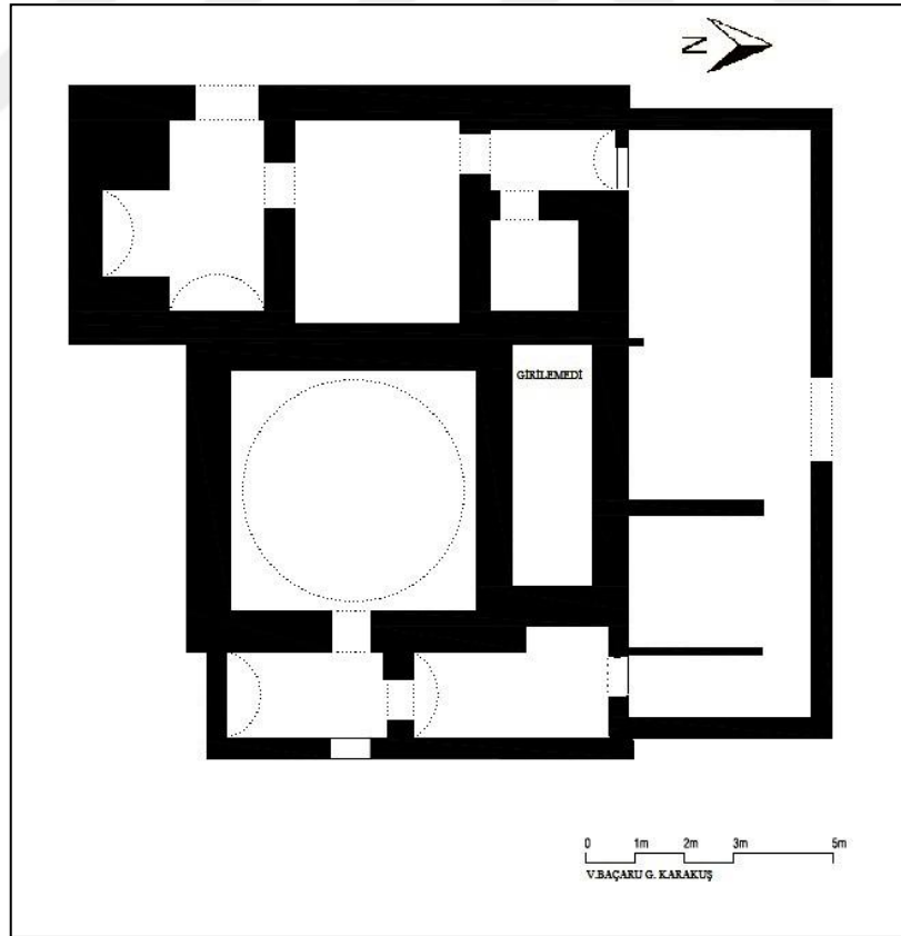
Şekil 33: Kuleli Hamamı Planı
