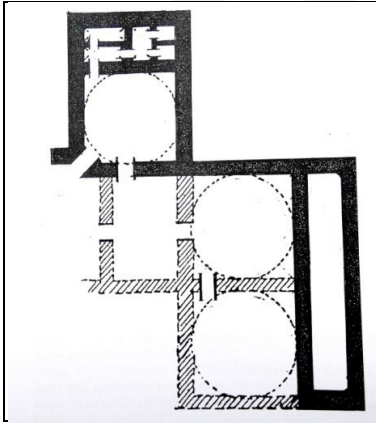
Şekil 2: Çengelköy Hamamı Planı (1948 R. Sevinçsoy)
