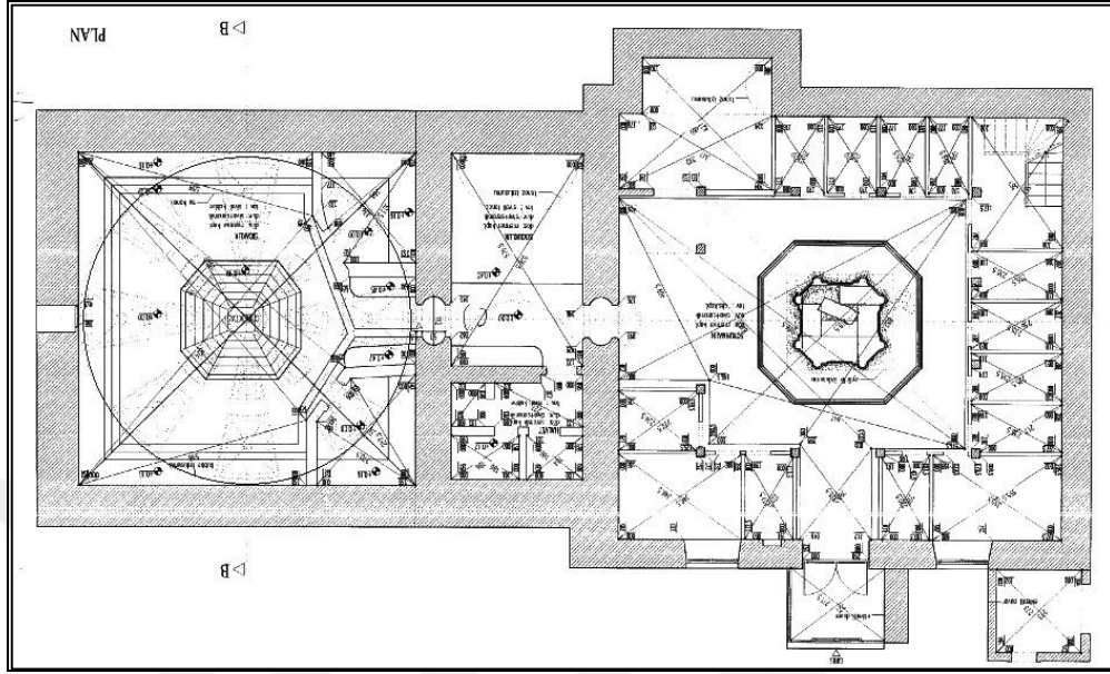
Şeki 35: İcadiye Dağ Hamamı Planı (İst. 6 No.lu KVKBK Arşivi'nden)
