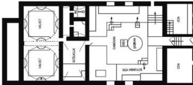
Şekil 22: Bulgurlu Köyü Hamamı Planı(A.B. KOÇU'dan İşlenerek)
