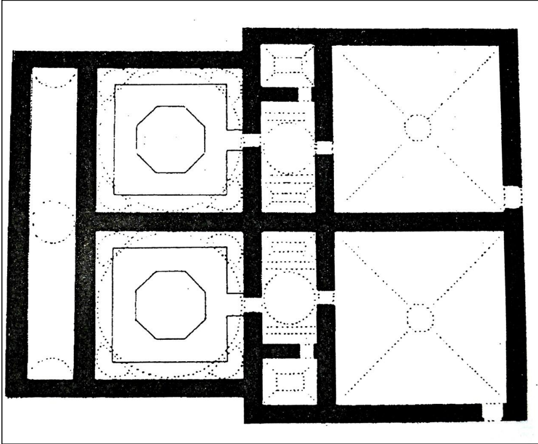
Şekil 17: Valide-i Atik Hamamı Planı (Abdullah Kuran’dan- Nermi Haskan’ın İst. Hamamları Kitabında)
