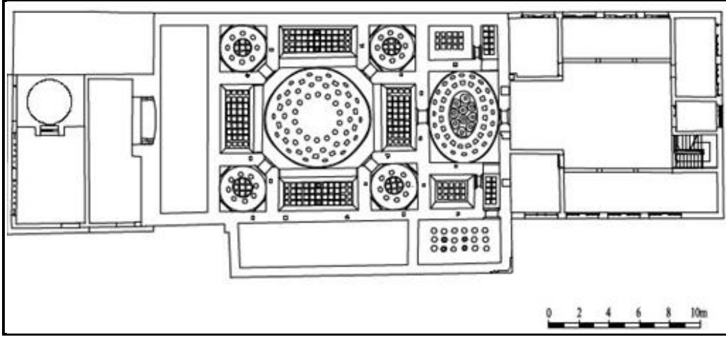
Şekil 30: Selimiye Hamamı Planı (İst. 6 No.lu KVKBK Arşivi)
