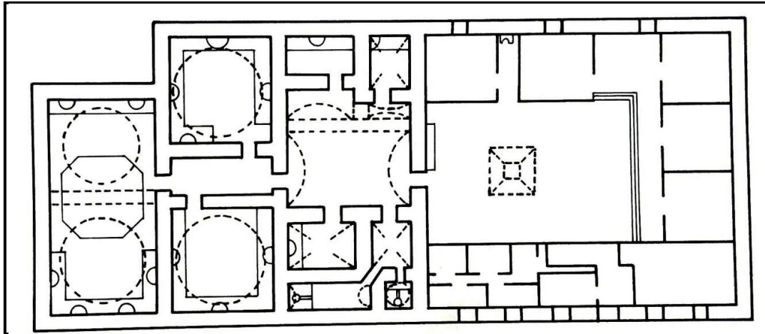
Şekil 28: Beylerbeyi Hamamı Planı (Rezan Çelebi, Düünden Bugüne İst. Ans.)
