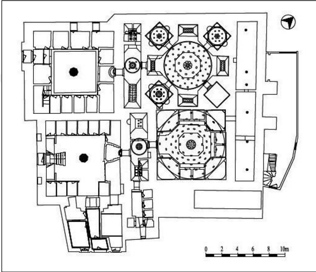
Şekil 24: Mahpeyker Kösem Valide Sultan Hamamı-Çinili Hamamı
