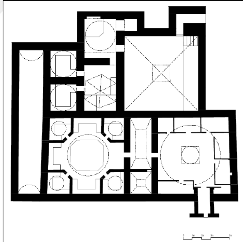
Şekil 11: Rum Mehmed Paşa Hamamı Planı ( Erkekler Kısım Ömel Tel'den İşlenerek, Kadınlar Kısım: V.Baçaru-G.Karakuş)
