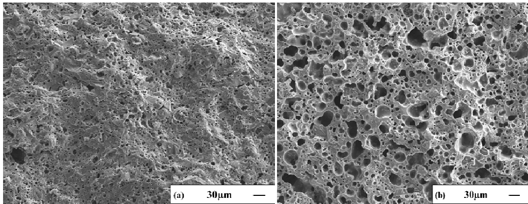
Görsel 7.13. (a)1210 ( \rho:1,77\text{gr/cm}^3 ), ve (b)1220°C ( \rho:1,55\text{gr/cm}^3 ), tepe sıcaklığında sinterlenen S-0,15-S9 kodlu bünyelerin genel mikroyapıları
