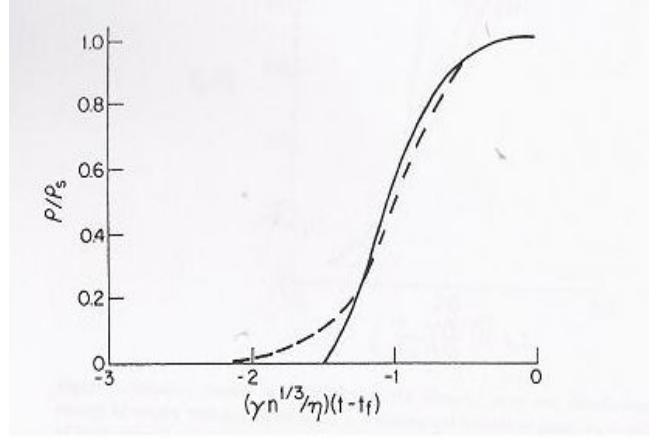
Şekil 4.3. Mackenzie-Shuttleworth modeline göre azalan zamana karşı relatif yoğunluk grafiği. (Düz grafik), Scherer'in silindir modeli (kesikli grafik) [55].
