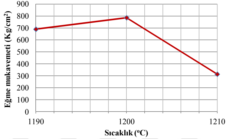
Şekil 7.11. CeO_2 katkılı bünyelerin sıcaklığa bağlı mukavemetteki değişimi
