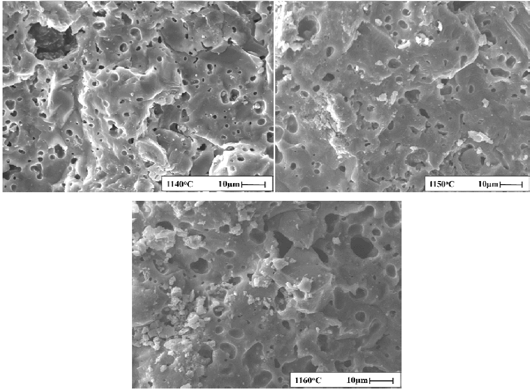
Görsel 7.24. Yüksek büyütmede BM+0,1Sika kodlu karoların sıcaklığa bağlı mikroyapı gelişimi ( \rho_{1140} :1,97gr/cm 3 , \rho_{1150} :2,30gr/cm 3 , \rho_{1160} :2,38gr/cm 3 )
