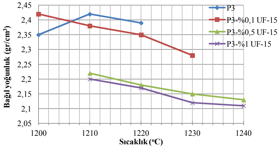
Şekil 7.82. P3 ve SiC (UF-15) katkılı P3 bünyelerinin sinterlenme sıcaklığına bağlı yoğunluk değerleri
