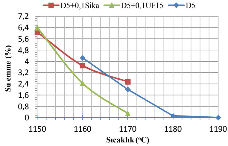
Şekil 7.67. D5 ve SiC katkılı D5 bünyelerinin sıcaklığa bağlı % su emme değişimi
