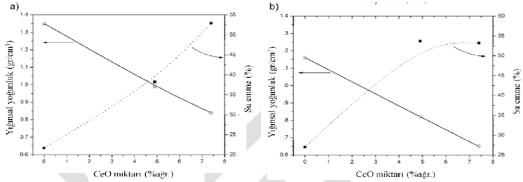
Şekil 5.3. %1 ağırl. \text{Si}_3\text{N}_4 içeren bünyelerde \text{CeO}_2 miktarına bağlı su emme ve yoğunluktaki değişim: (a) 1220^\circ\text{C} ; (b) 1240^\circ\text{C} [92].
