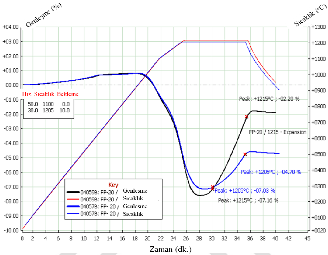
Şekil 7.13. %20 oranında parlatma atığı katkılı bünyenin 1205 ve 1215°C tepe sıcaklığında sinterlenme davranışının incelenmesi.
