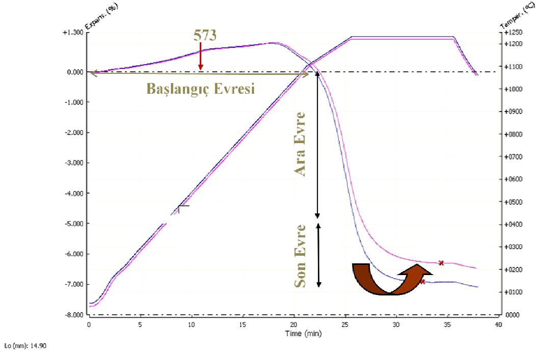
Şekil 4.4. Porselen karo bünyeleri sinterlenme aşamaları [63].
