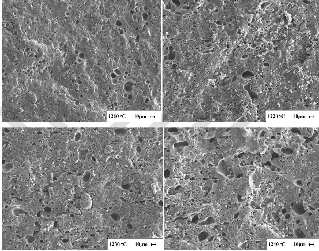
Görsel 7.33. %0,5 Sika katkılı P3 bünyesinin sıcaklığa bağlı mikroyapı gelişimi
