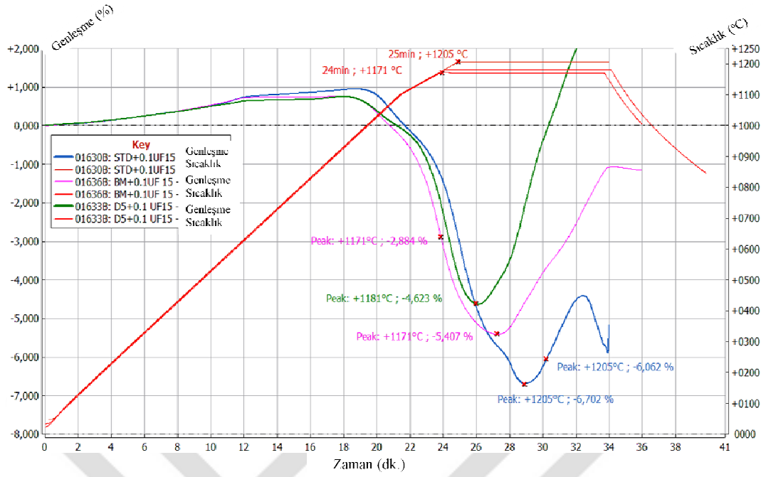
Şekil 7.74. %0,1 oranında UF15 içeren D5, BM ve STD bünyelerinin sinterlenme davranışının karşılaştırılması
