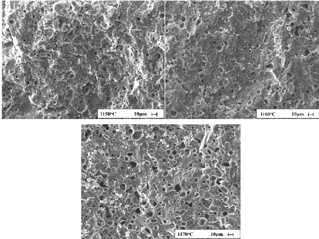
Görsel 7.27. D5+0,1SiC kodlu karoların sıcaklığa bağlı mikroyapı gelişimi ( \rho_{1150} : 2,46gr/cm 3 , \rho_{1160} : 2,37gr/cm 3 , \rho_{1170} : 1,91gr/cm 3 )
