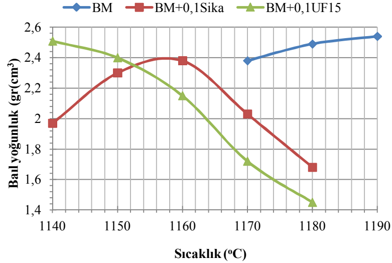
Şekil 7.64. BM ve SiC katkılı BM bünyelerinin sıcaklığa bağlı yoğunluk değişimi
