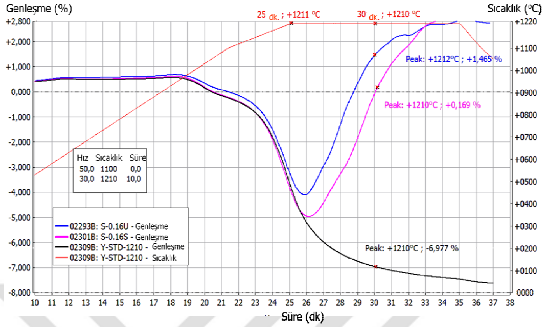
Şekil 7.49. Farklı tane boyutunda %0,16 oranında SiC (Sika, UF-15) içeren bünyelerin 1210°C tepe sıcaklığında sinterlenme davranışının incelenmesi
