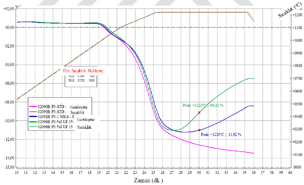
Şekil 7.89. %1 oranında Sika ve UF-15 kodlu SiC içeren P3 bün-yeleri sinterlenme davranışının karşılaştırılması
