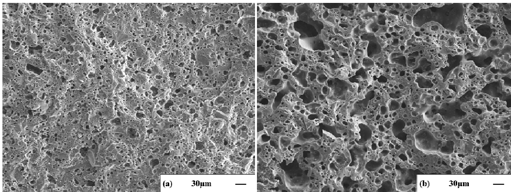
Görsel 7.16. (a) 1210 ( \rho: 1,76 \text{ gr/cm}^3 ), ve (b) 1220°C ( \rho: 1,62 \text{ gr/cm}^3 ), tepe sıcaklığında sinterlenen S-0,18-S9 kodlu bünyelerin genel mikroyapıları
