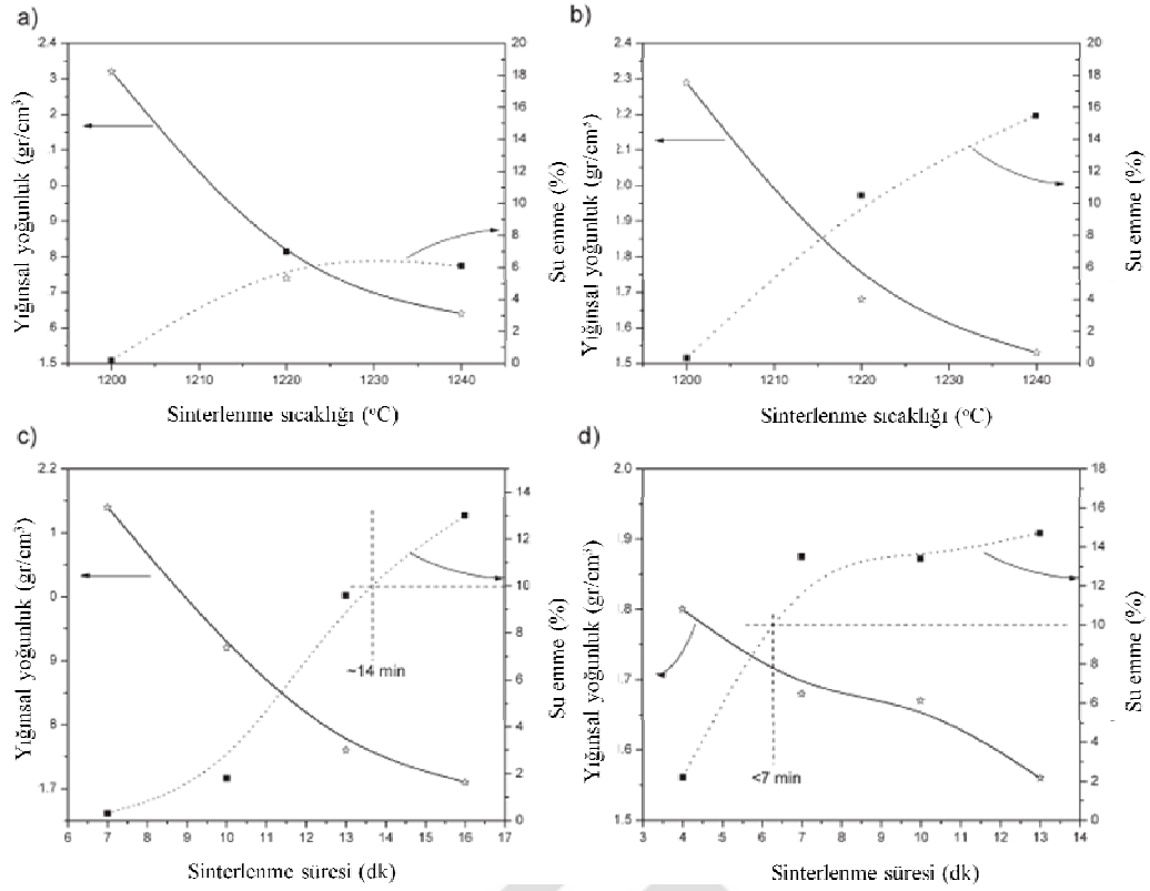
Şekil 5.5. CeO_2 katkısı ile köpükleştirme işleminde (a,b) sinterlenme sıcaklığı [(a) %4 CeO_2 ; (b) %7,4 CeO_2 ]; (c,d) sinterlenme süresi %4 CeO_2 ilavesi [(c) 1220^\circ C ; (d) 1240^\circ C ] etkisi.
