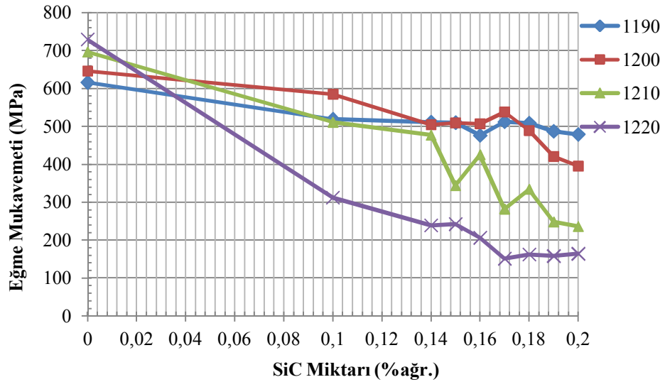
Şekil 7.45. Farklı sıcaklıklar için SiC ( d_{90} : \sim 9 \mu\text{m} ) miktarına bağlı eğme mukavemetindeki değişim
