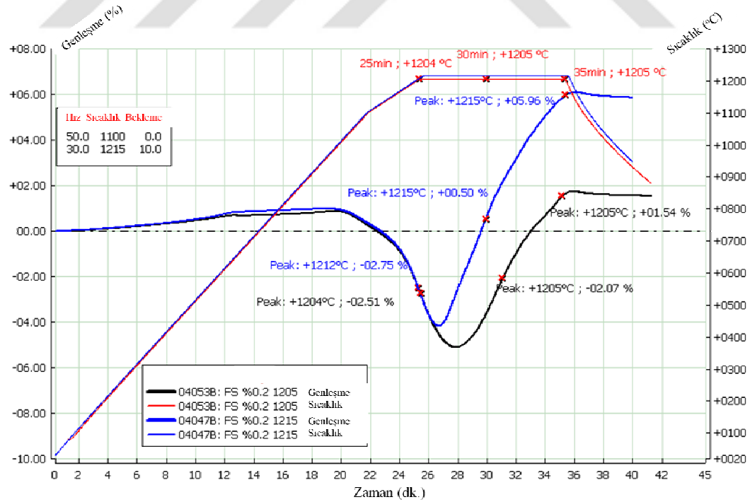
Şekil 7.19. %0,2 oranında saf SiC katkılı bünyenin 1205 ve 1215°C tepe sıcaklığında sinterlenme davranışının incelenmesi.
