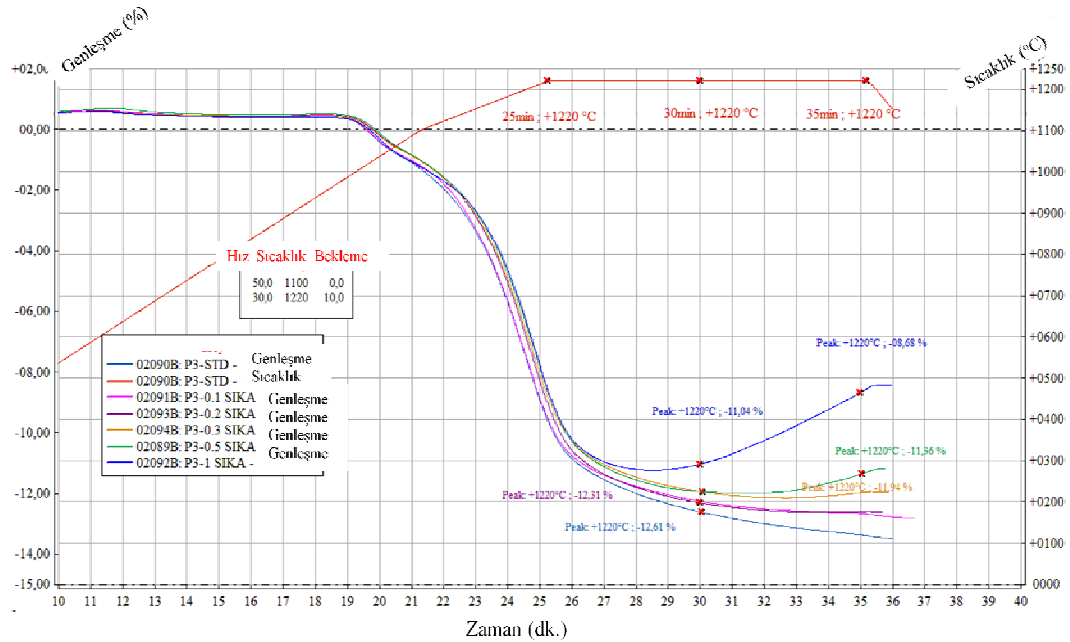
Şekil 7.86. P3 ve Sika kodlu SiC içeren P3 bünyelerinin 1220°C tepe sıcaklığında sinterlenme davranışının incelenmesi
