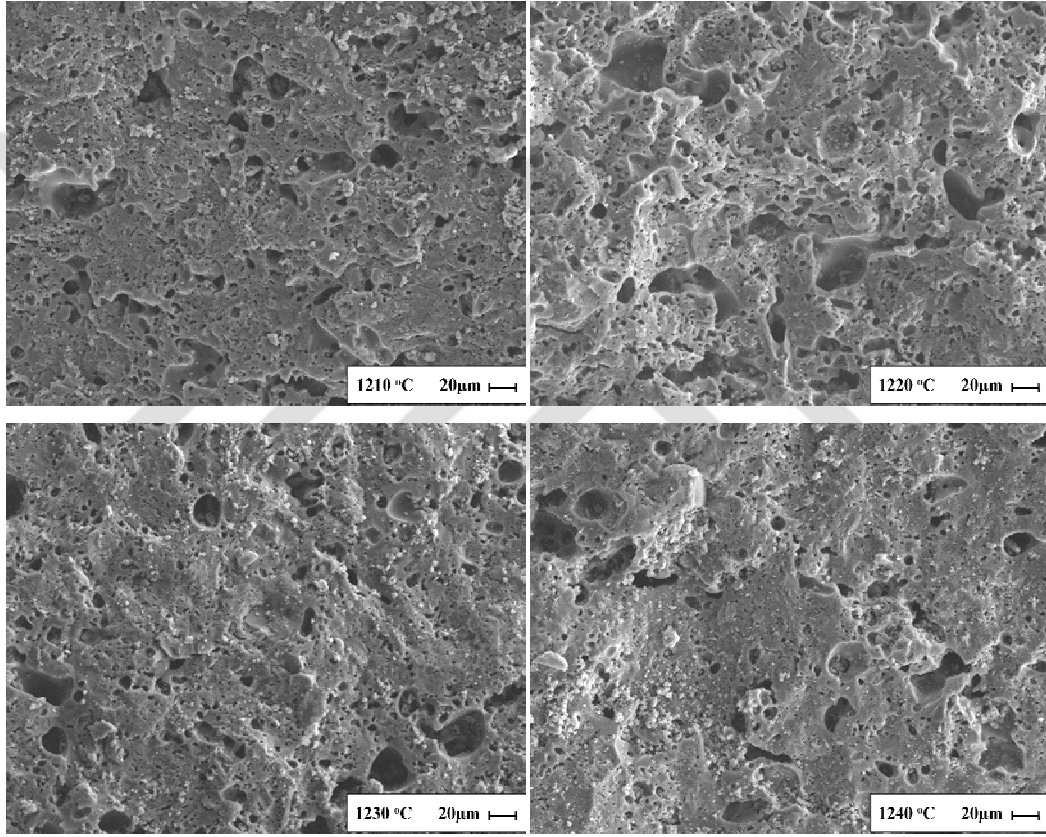
Görsel 7.35. %1 Sika katkılı P3 bünyesinin sıcaklığa bağlı mikroyapı gelişimi
