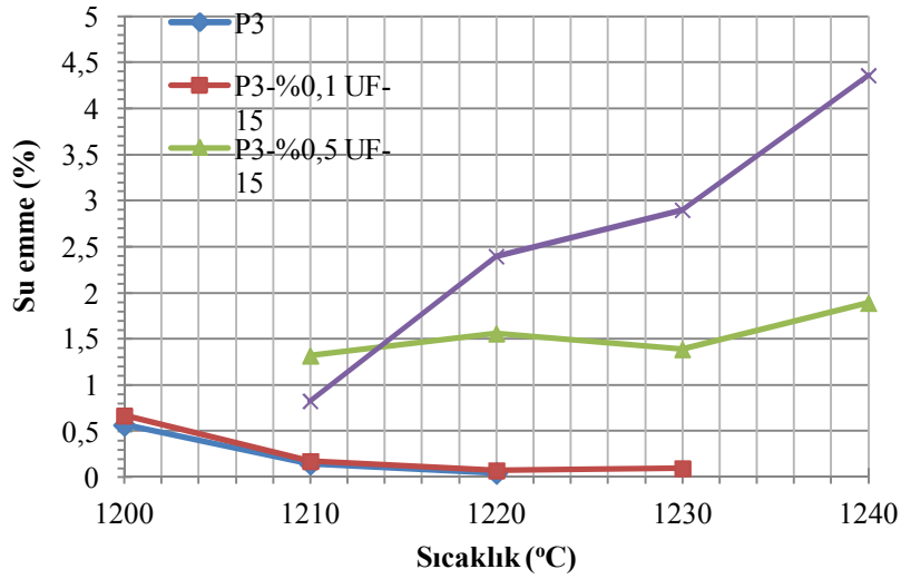
Şekil 7.80. P3 ve SiC (UF-15) katkılı P3 bünyelerinin sinterlenme sıcaklığına bağlı (%) su emme değerleri
