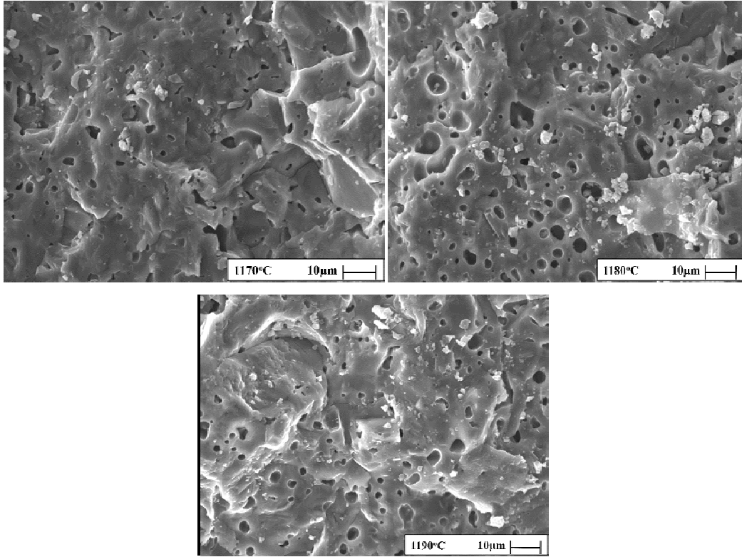
Görsel 7.20. Yüksek büyütmede STD+0,1 Sika kodlu karoların sıcaklığa bağlı mikroyapı gelişimi ( \rho_{1170} : 2,5gr/cm 3 , \rho_{1180} : 2,33gr/cm 3 , \rho_{1190} : 2,27gr/cm 3 )
