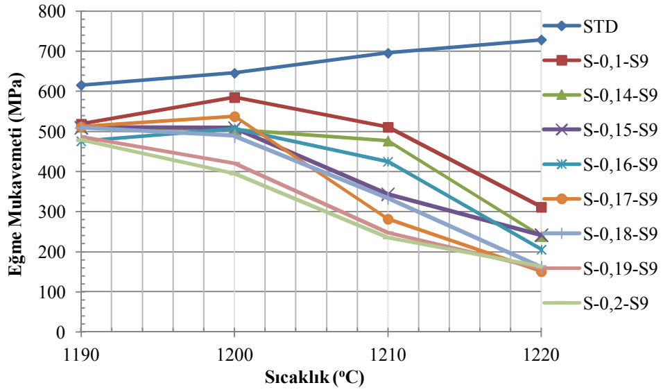
Şekil 7.44. Saf SiC ( d_{90} : \sim 9 \mu\text{m} ) içeren bünyelerin sıcaklığa bağlı eğme mukavemetindeki değişim
