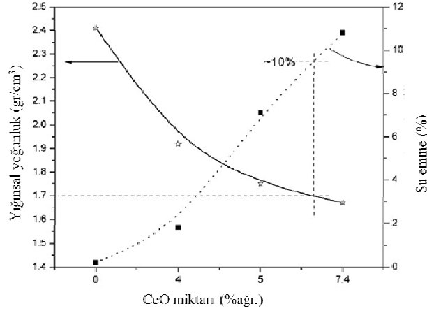
Şekil 5.4. CeO 2 katkısına bağlı olarak yoğunluk ve su emmedeki değişim. (Numuneler 1220°C'de 10dk bekleme ile sinterlenmiştir.) [92].
