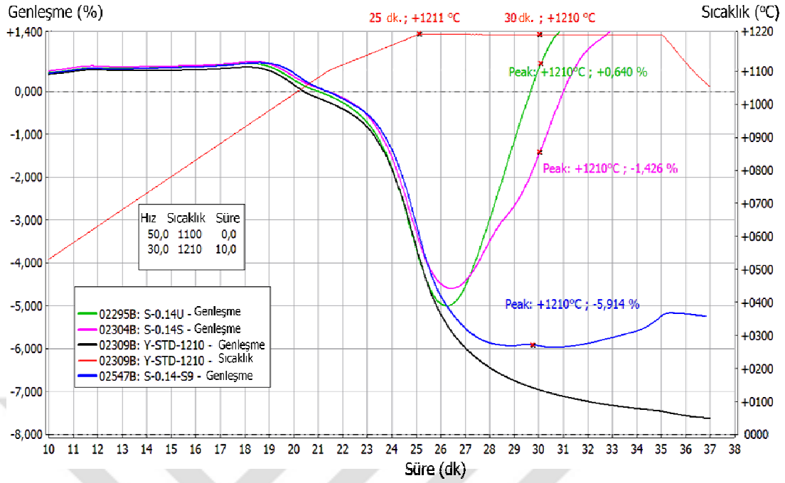
Şekil 7.52. Farklı tane boyutunda %0,14 oranında SiC (Sika, UF-15, SiC lab.) içeren bünyelerin 1210°C tepe sıcaklığında sinterlenme davranışının incelenmesi
