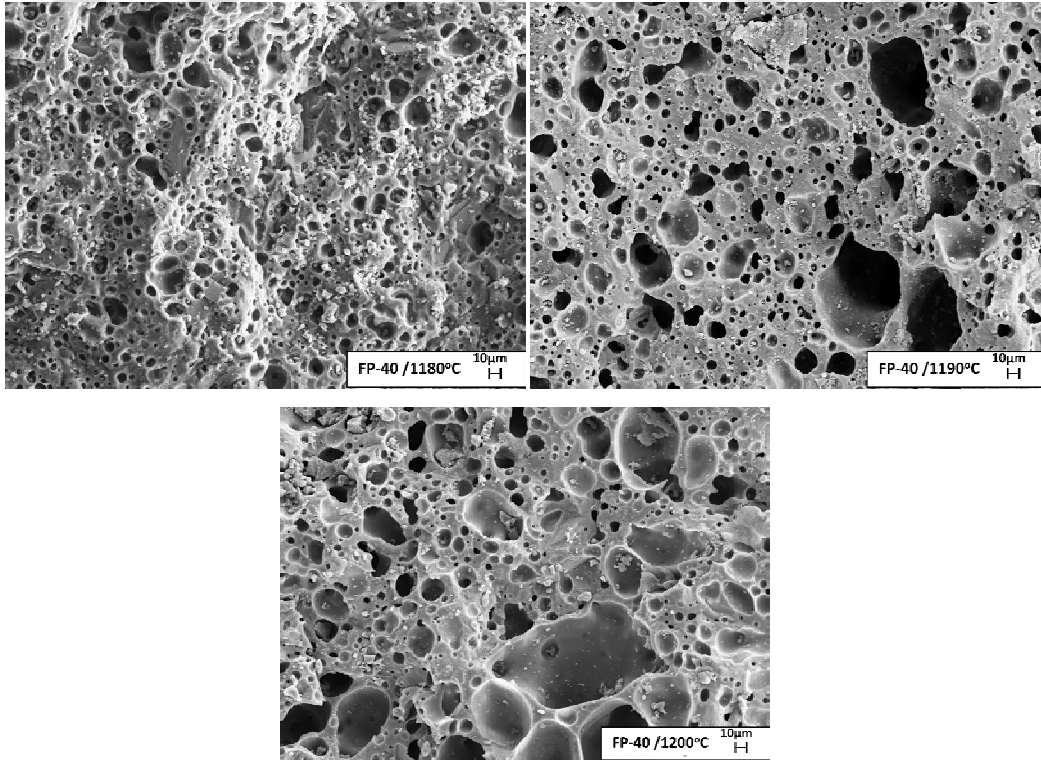
Görsel 7.3. Farklı sıcaklıklarda sinterlenen FP-40 bünyesi genel mikroyapı görüntüsü. (\rho_{1180}: 1,73\text{gr/cm}^3, \rho_{1190}: 1,39\text{gr/cm}^3, \rho_{1200}: 1,36\text{gr/cm}^3)
