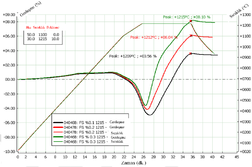
Şekil 7.22. %0,1, 0,2 ve 0,3 oranında saf SiC katkılı bünyelerin 1215°C tepe sıcaklığında sinterlenme eğrilerinin karşılaştırılması.
