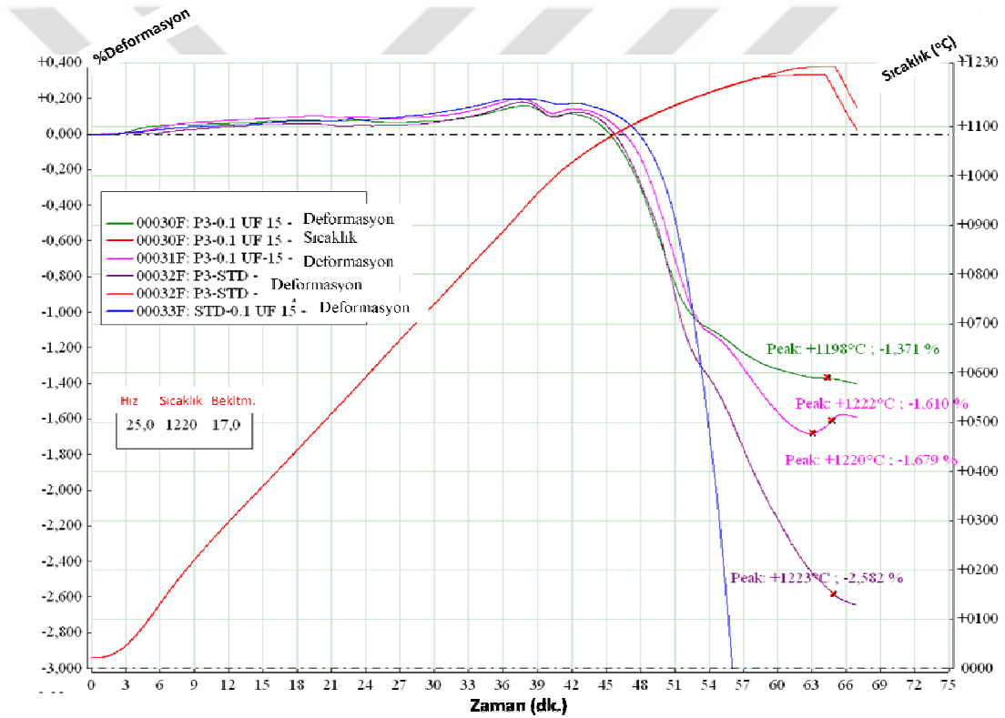
Şekil 7.91. Geliştirilen P3 ve %0,1UF-15 ilaveli P3 bünyesinin 1220°C’de deformasyon davranışının incelenmesi
