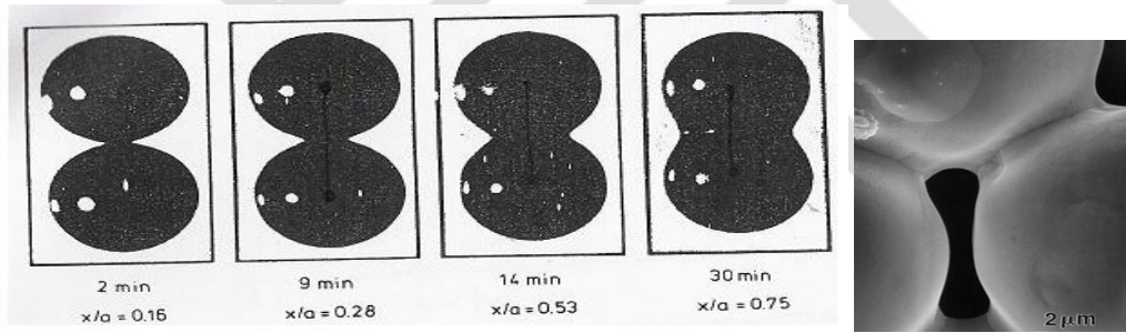
Şekil 4.2. Sinterlenme sırasında boyun oluşumu [52]
