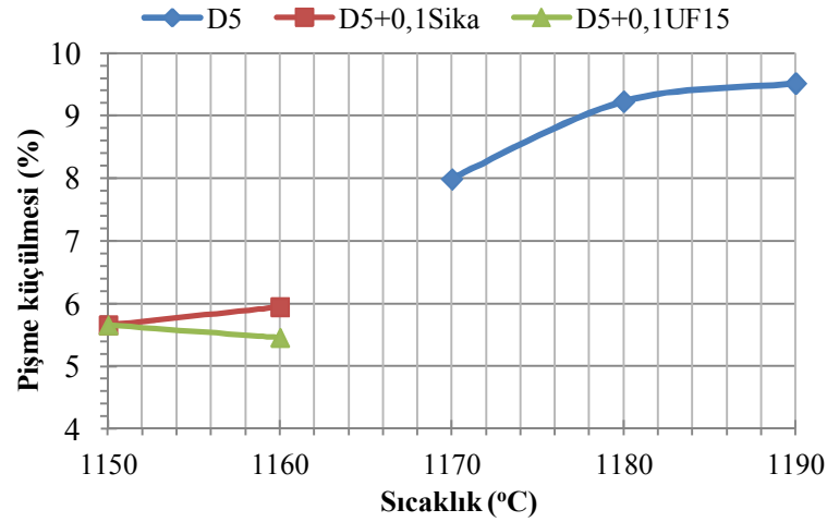
Şekil 7.66. D5 ve SiC katkılı D5 bünyelerin sıcaklığa bağlı pışme küçülmeleri
