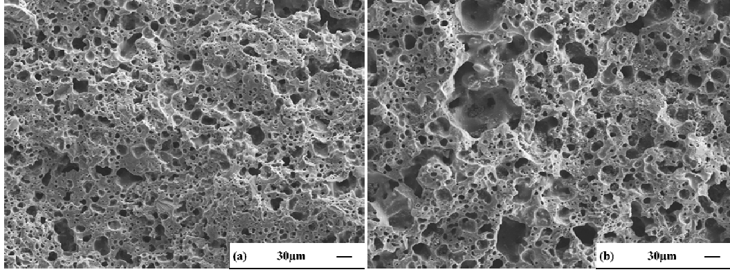
Görsel 7.17. (a)1210 ( \rho:1,67\text{gr/cm}^3 ), ve (b)1220°C ( \rho:1,64\text{gr/cm}^3 ), tepe sıcaklığında sinterlenen S-0,19-S9 kodlu bünyelerin genel mikroyapıları
