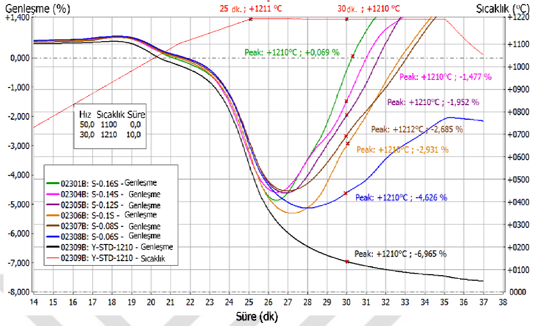
Şekil 7.46. Saf SiC (Sika) içeren bünyelerin 1210°C tepe sıcaklığında sinterlenme davranışının incelenmesi.
