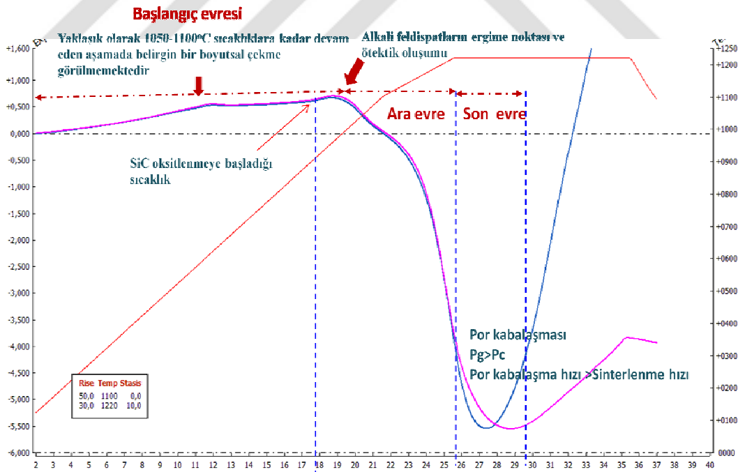
Şekil 7.50. Değişen oranlarda SiC ilave edilen bünyelerin sinterlenme aşamaları
