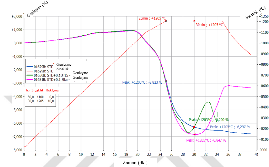
Şekil 7.70. STD ve SiC içeren STD bünyenin 1205°C tepe sıcaklığında sinterlenme davranışının incelenmesi
