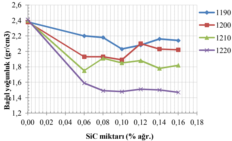
Şekil 7.29. Farklı sıcaklıklar için SiC (Sika) miktarına bağlı yoğunluktaki değişim
