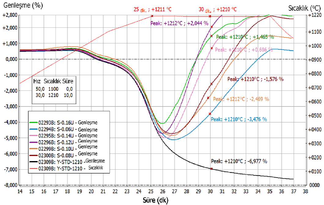
Şekil 7.47. Saf SiC (UF-15) içeren bünyelerin 1210°C tepe sıcaklığında sinterlenme davranışlarının incelenmesi
