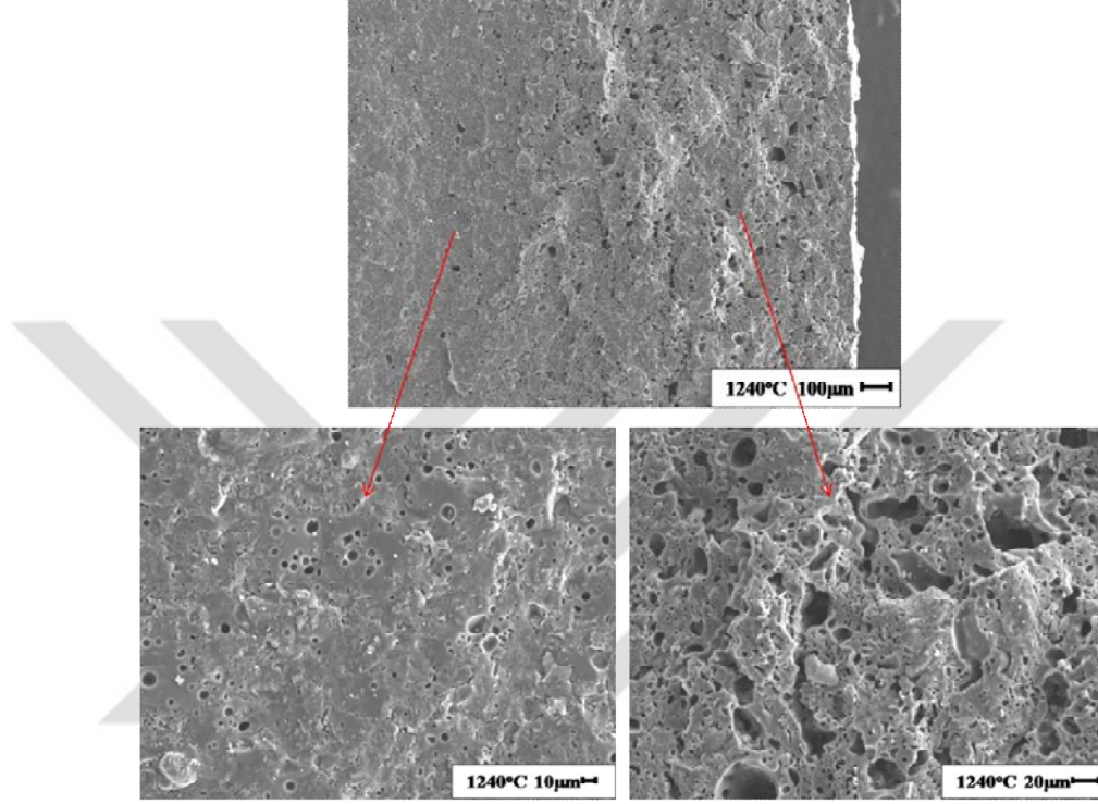
Görsel 7.39. %1 UF-15 katkılı P3 bünyesinin sıcaklığa bağlı mikroyapı gelişimi (1210°C; İç ve dış bölgelerde mikroyapı farkı)
