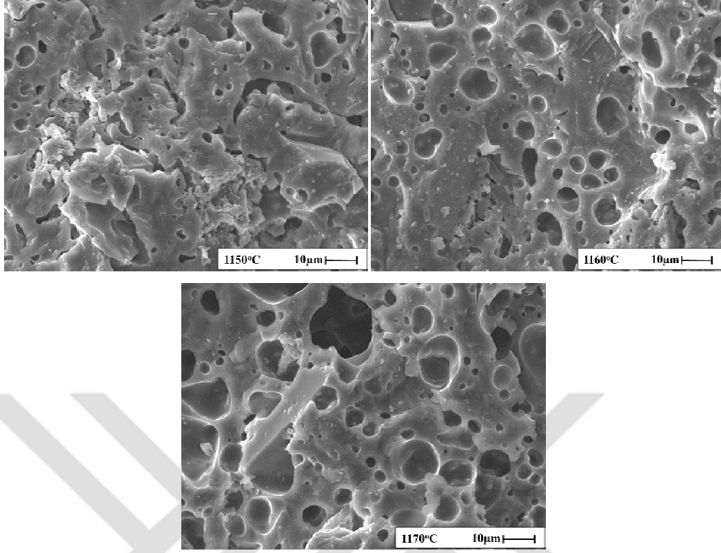
Görsel 7.30. Yüksek büyütmede D5+0,1UF15 kodlu karoların sıcaklığa bağlı mikroyapı gelişimi ( \rho_{1150}: 2,49 \text{ gr/cm}^3 , \rho_{1160}: 2,30 \text{ gr/cm}^3 , \rho_{1170}: 1,88 \text{ gr/cm}^3 )
