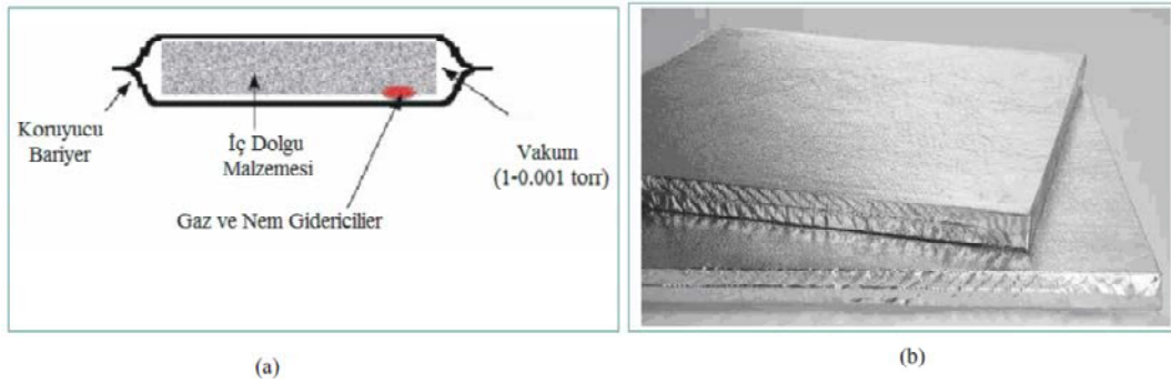
Şekil 3.8. Tipik bir vakum izolasyon paneli (a) iç yapısı (b) dış görüntüsü [20].
