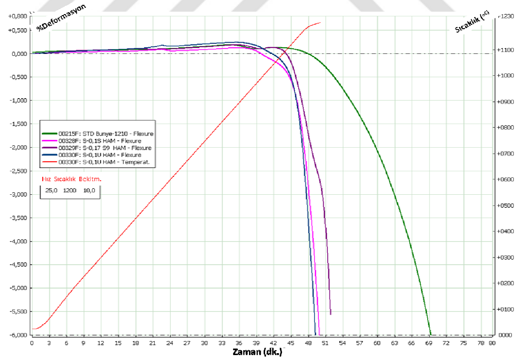
Şekil 7.56. %0,1 oranında Sika, UF-15 ve %0,17 oranında SiC-Lab. kodlu silisyum karbür katkılı bünyelerin zamana ve sıcaklığa bağlı deformasyon davranışı
