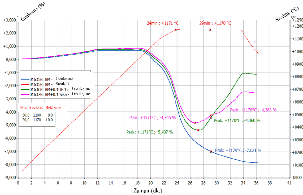
Şekil 7.71. BM ve SiC içeren BM bünyelerinin 1170°C tepe sıcaklığında sinterlenme davranışının incelenmesi
