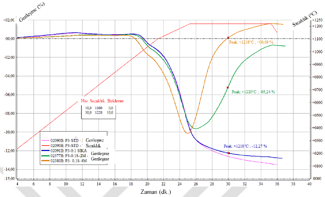
Şekil 7.90. %0,1 oranında Sika kodlu SiC ve %2 ve %4 oranında MO içeren P3 bünnyeleri sinterlenme davranışının karşılaştırılması
