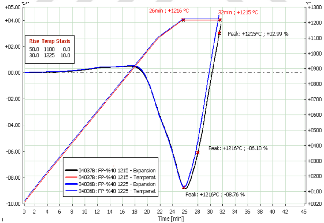
Şekil 7.15. %40 oranında parlatma atığı katkılı bünyenin 1215 ve 1225°C tepe sıcaklığında sinterlenme davranışının incelenmesi
