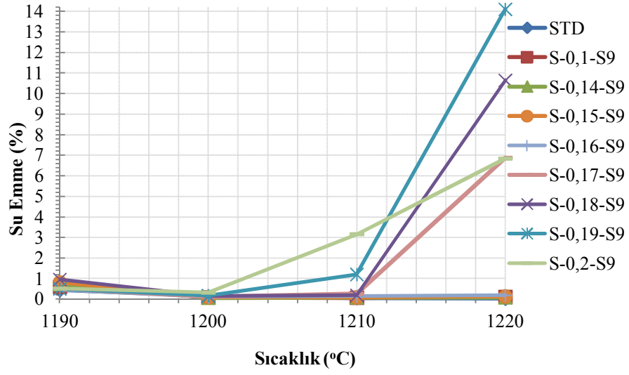
Şekil 7.40. Saf SiC ( d_{90} : \sim 9 \mu m ) içeren bünyelerin sıcaklığa bağlı % su emme değişimi
