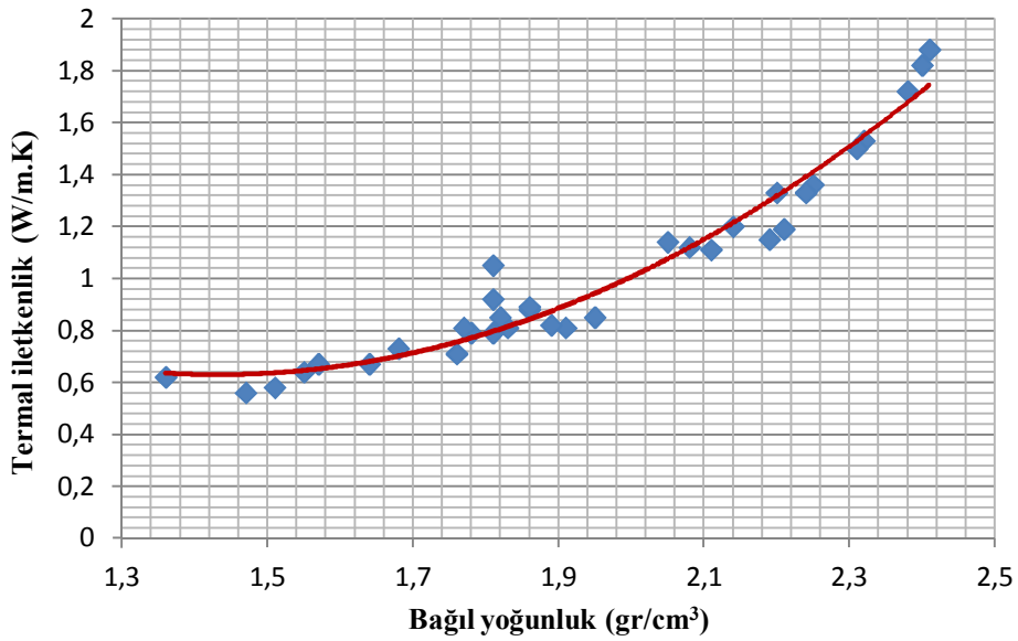
Şekil 7.57. SiC katkılı porselen karo bünyelerde yoğunluğa bağlı termal iletkenlik değişimi
