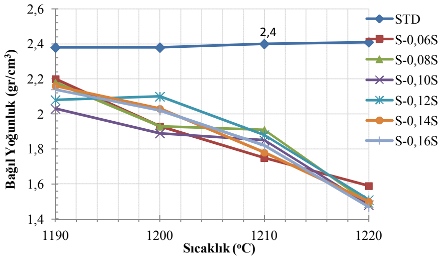
Şekil 7.28. Saf SiC (Sika) içeren bünyelerin sıcaklığa bağlı yoğunluk değerlerindeki değişim
