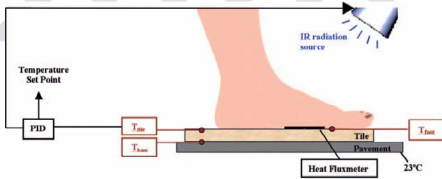
Şekil 5.2. Deneysel düzenek [80]
