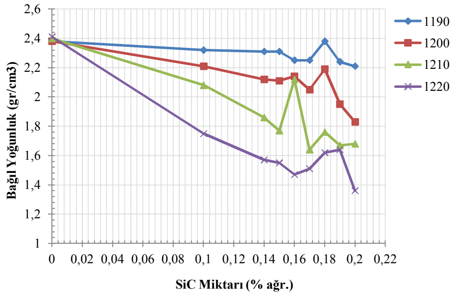
Şekil 7.43. Farklı sıcaklıklar için SiC ( d_{90} : \sim 9 \mu\text{m} ) miktarına bağlı yoğunluktaki değişim
