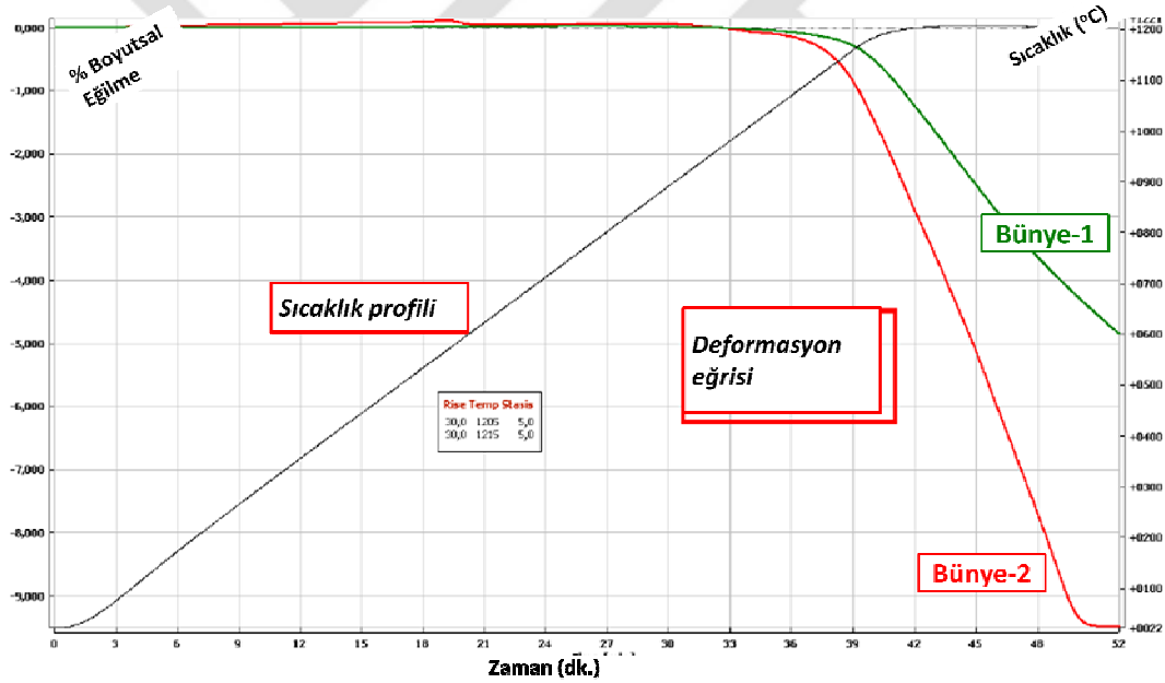
Şekil 7.53. İki farklı kompozisyona sahip porselen karo bünyenin deformasyon eğrisi [110].
