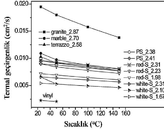
Şekil 3.1. Seramik yer karolarının sıcaklığa bağlı termal geçirgenlik değişimi [35].
