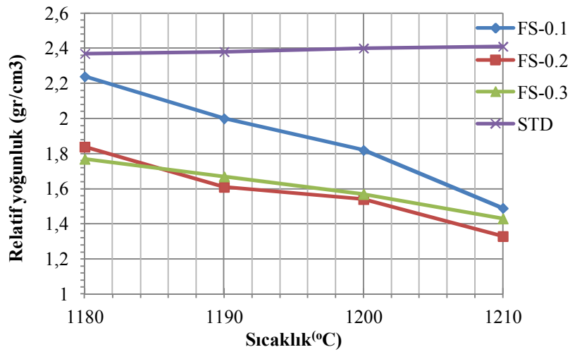
Şekil 7.7. Saf SiC katkılı bünyelerin katkı miktarına ve sıcaklığa bağlı yoğunluk değişimi
