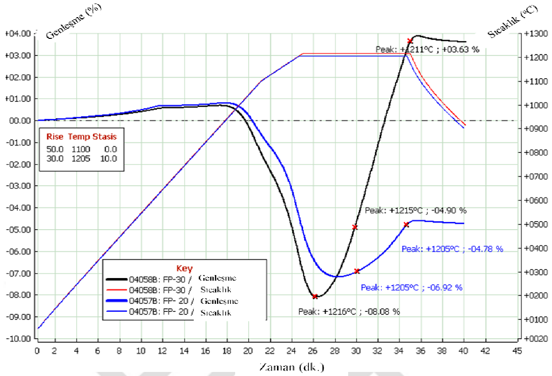
Şekil 7.14. %30 oranında parlatma atığı katkılı bünyenin 1205 ve 1215°C tepe sıcaklığında sinterlenme davranışının incelenmesi
