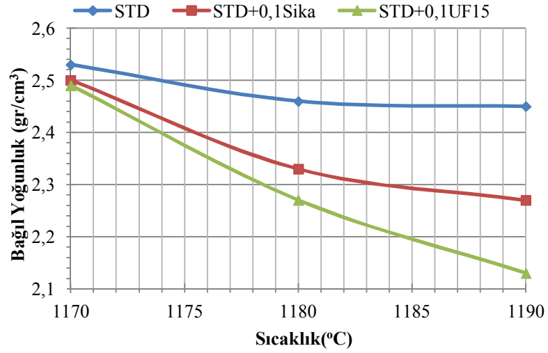
Şekil 7.61. STD ve SiC katkıli standart bünyelerin sıcaklığa bağlı yoğunluk değişimi
