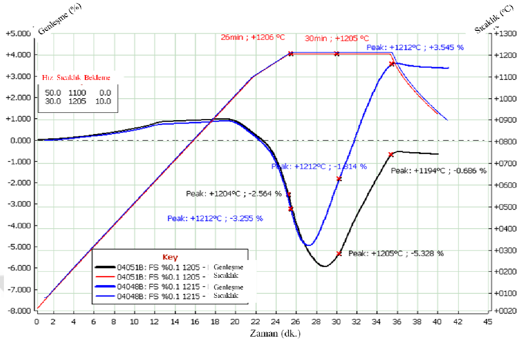
Şekil 7.18. %0,1 oranında saf SiC ilave edilmiş bünyenin 1205 ve 1215°C tepe sıcaklığında sinterlenme davranışının incelenmesi
