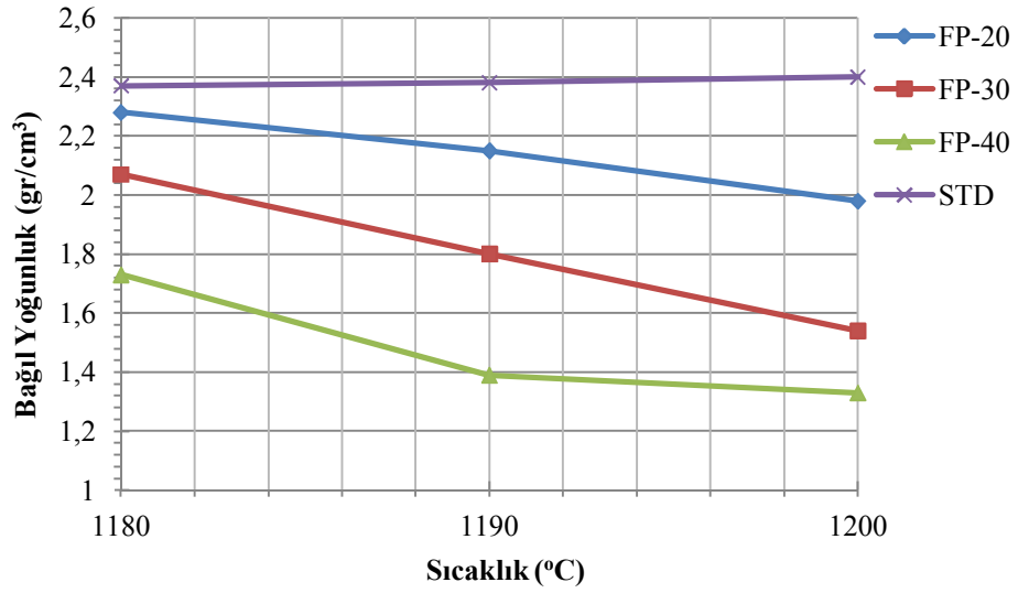
Şekil 7.2. Porselen karo parlatma atığı katkıli bünyelerin katkı miktarına ve sıcaklığa bağlı yoğunluk değişimi.
