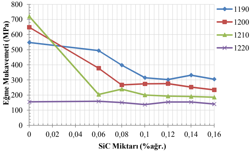
Şekil 7.37. Farklı sıcaklıklar için SiC (UF-15) miktarına bağlı eğme mukavemetindeki değişim
