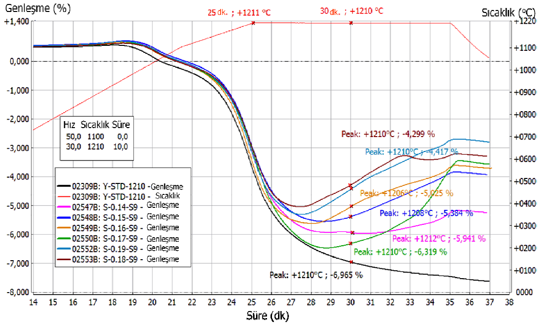
Şekil 7.51. Saf SiC (SiC-lab.) içeren bünyelerin 1210°C tepe sıcaklığında sinterlenme davranışının incelenmesi.
