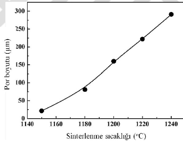
Şekil 5.9. Sinterlenme sıcaklığının por boyutuna etkisi (%2 SiC) [95].
