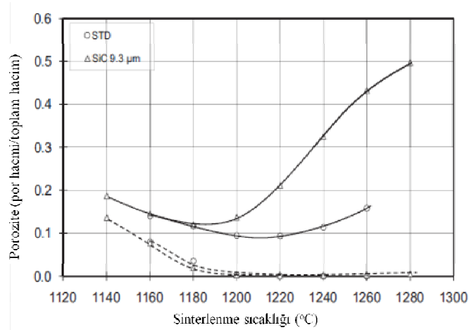
Şekil 5.6. Sıcaklığa bağlı toplam porozite ve açık porozite değişimi (STD ve %0,2 SiC içeren porselen karo) [94].
