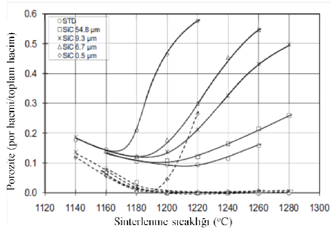
Şekil 5.7. Sıcaklığa bağlı toplam porozite ve açık porozite değişimi (STD ve farklı tane boyutunda SiC katkıli bünyeler) [94].
