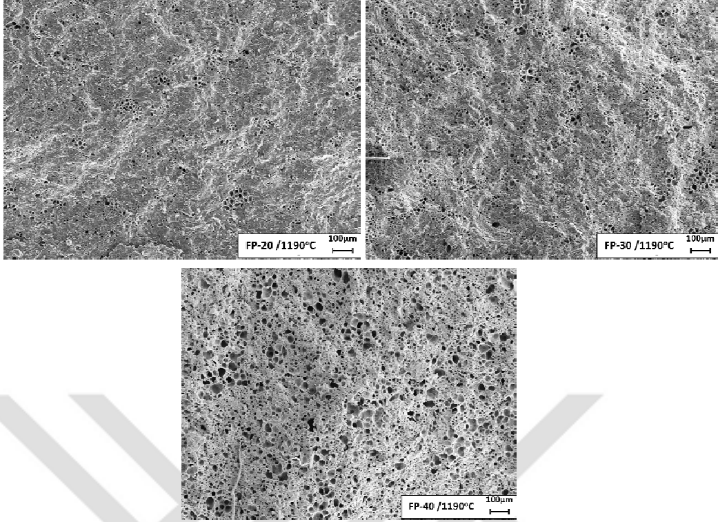
Görsel 7.4. FP-20 ( 2,15\text{gr/cm}^3 ), FP-30 ( 1,8\text{gr/cm}^3 ) ve FP-40 ( 1,39\text{gr/cm}^3 ) bünyeleri genel mikroyapı görüntüleri kıyaslaması.
