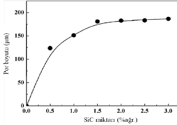
Şekil 5.11. SiC miktarının por boyutuna etkisi (1200°C, 20dk)
