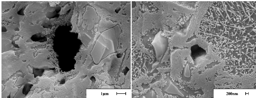
Görsel 7.31. P3 bünyesinin farklı büyütmelelerdeki mikroyapı görüntüsü (1220°C)
