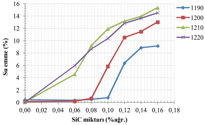
Şekil 7.27. Farklı sıcaklıklar için SiC (Sika) miktarına bağlı % su emme değişimi
