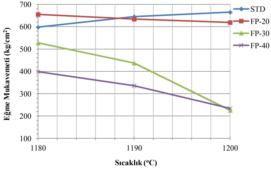
Şekil 7.3. Porselen karo parlatma atığı katkıli bünyelerin katkı miktarına ve sıcaklığa bağlı eğme mukavemeti değişimi
