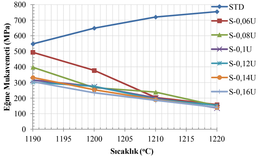
Şekil 7.36. Saf SiC (UF-15) içeren bünyelerin sıcaklığa bağlı eğme mukavemetindeki değişim
