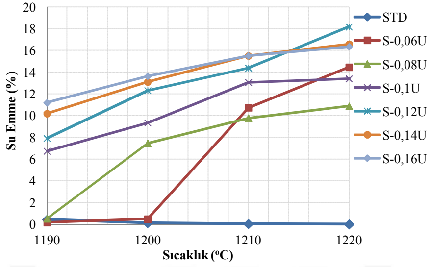
Şekil 7.32. Saf SiC (UF-15) içeren bünnyelerin sıcaklığa bağlı % su emme değişimi
