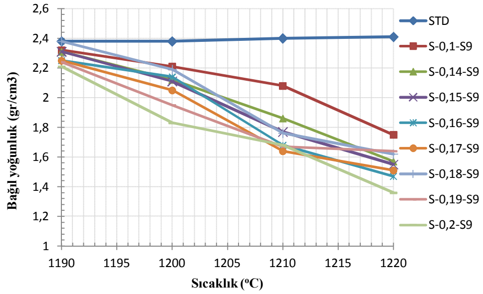
Şekil 7.42. Saf SiC ( d_{90} : \sim 9 \mu\text{m} ) içeren bünyelerin sıcaklığa bağlı yoğunluk değerlerindeki değişim
