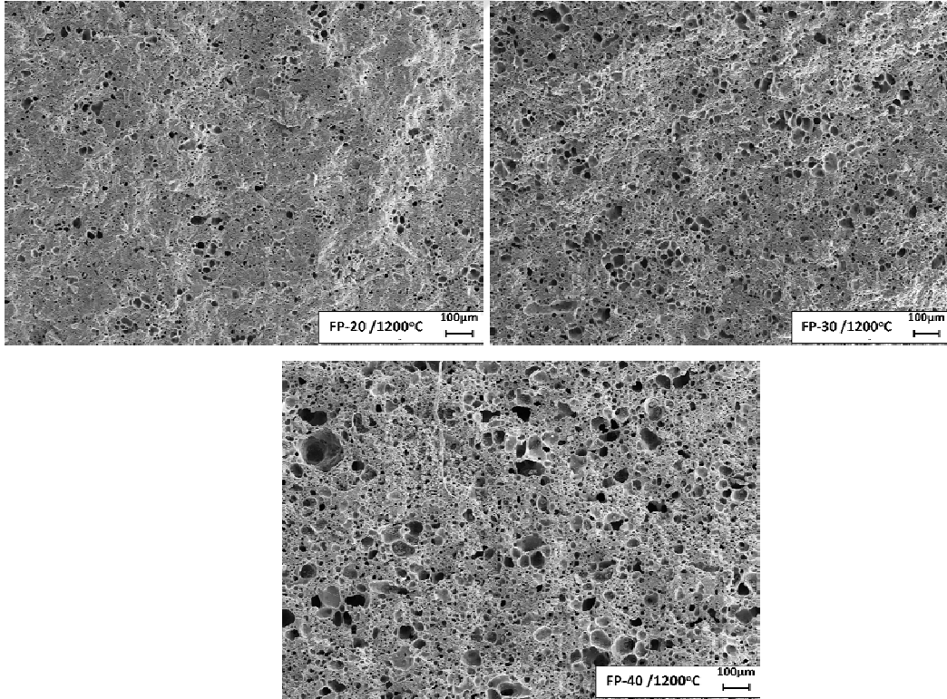
Görsel 7.5. FP-20 ( 1,98\text{gr/cm}^3 ), FP-30 ( 1,54\text{gr/cm}^3 ) ve FP-40 ( 1,33\text{gr/cm}^3 ) bünyeleri genel mikroyapı görüntüleri kıyaslaması
