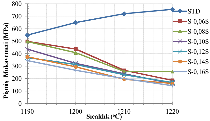
Şekil 7.30. Saf SiC içeren bünyelerin sıcaklığa bağlı eğme mukavemetindeki değişim
