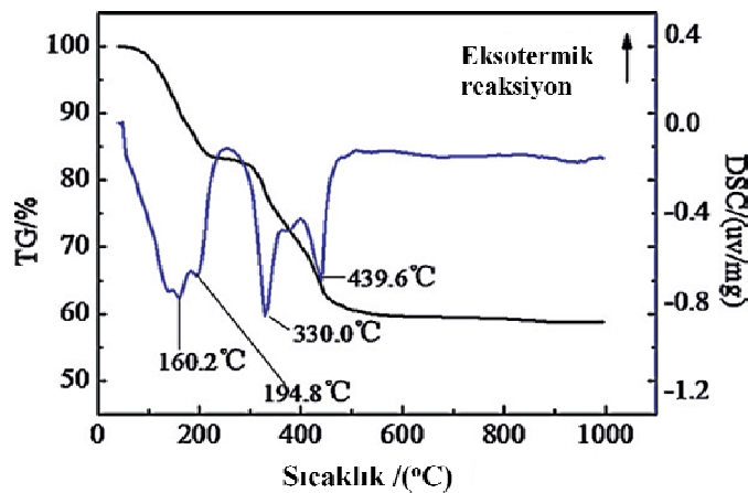
Şekil 7.85. Mağnezyum oksiklorit (MO) tozu TG-DSC eğrisi
