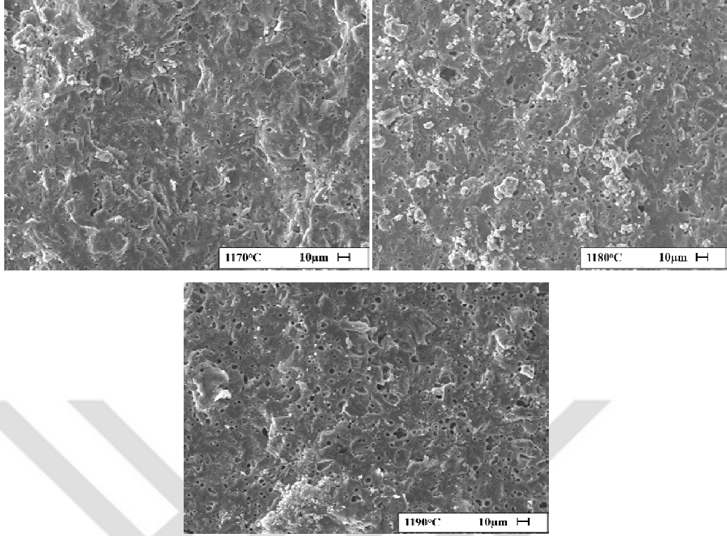
Görsel 7.19. STD+0,1 Sika kodlu karoların sıcaklığa bağlı mikroyapı gelişimi ( \rho_{1170} : 2,07gr/cm 3 , \rho_{1180} : 1,8gr/cm 3 , \rho_{1190} : 1,54gr/cm 3 )
