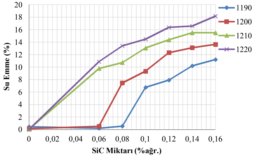
Şekil 7.33. Farklı sıcaklıklar için SiC (UF-15) miktarına bağlı % su emme değişimi
