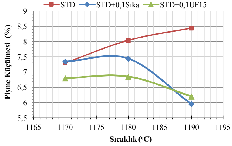
Şekil 7.59. STD ve SiC katkıli standart bünyelerin sıcaklığa bağlı pişme küçülmeleri
