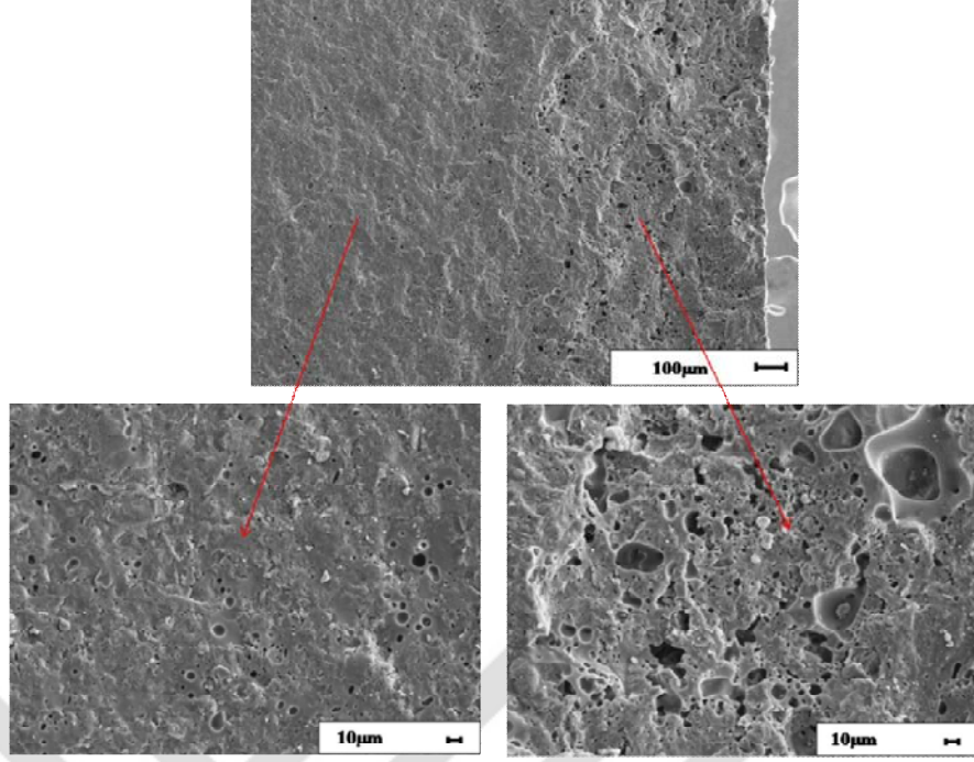
Görsel 7.37. %0,5 UF-15 katkılı P3 bünyesinin sıcaklığa bağlı mikroyapı gelişimi (1210°C; İç ve dış bölgelerde mikroyapı gelişimi farkı).
