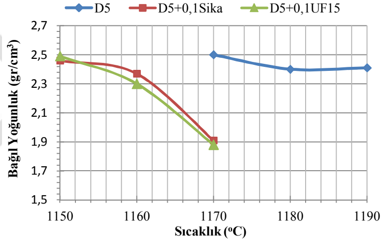
Şekil 7.68. D5 ve SiC katkılı D5 bünyelerinin sıcaklığa bağlı yoğunluk değişimi
