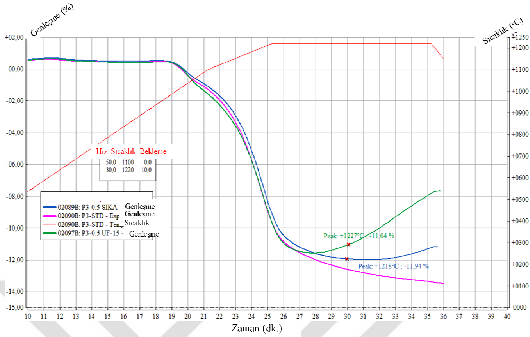
Şekil 7.88. %0,5 oranında Sika ve UF-15 kodlu SiC içeren P3 bün-yeleri sinterlenme davranışının karşılaştırılması.
