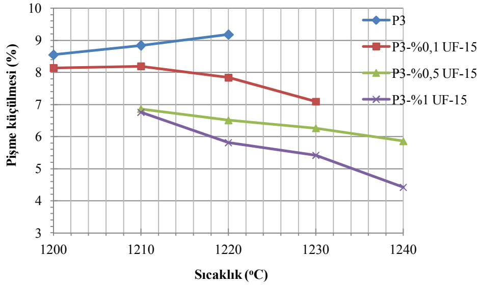
Şekil 7.78. P3 ve SiC (UF-15) katkı P3 bünyelerinin sinterlenme sıcaklığına bağlı pişme küçülmeleri (%).
