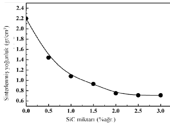
Şekil 5.10. SiC miktarına bağlı yoğunluktaki değişim (1220°C, 20dk)
