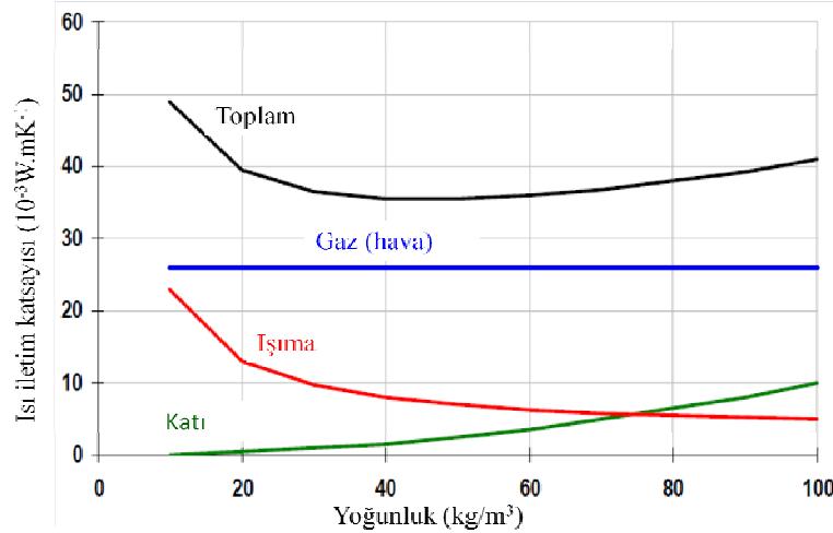
Şekil 3.7. Fiber ve köpür bazlı konvansiyonel ısı yalıtım malzemelerinde ısı transferi mekanizması.
