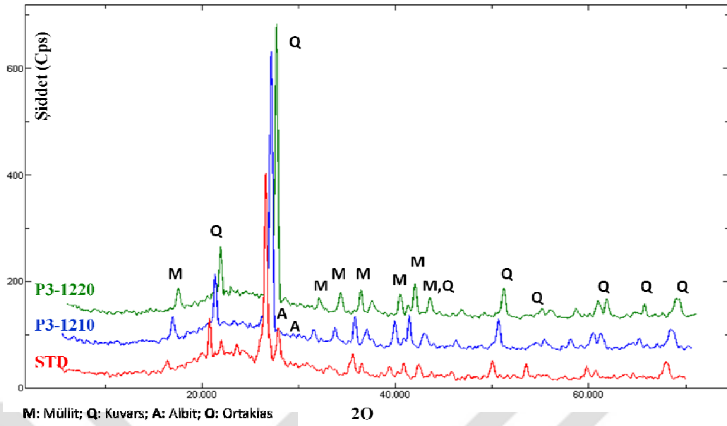
Şekil 7.76. STD ve P3 bünyesi mineralojik analizi
