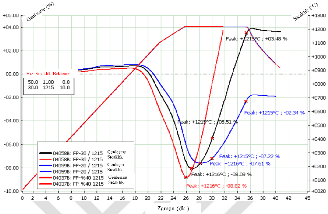
Şekil 7.17. %20, 30 ve 40 oranında parlatma atığı katkılı bünyelerin 1215°C tepe sıcaklığında sinterlenme eğrilerinin karşılaştırılması
