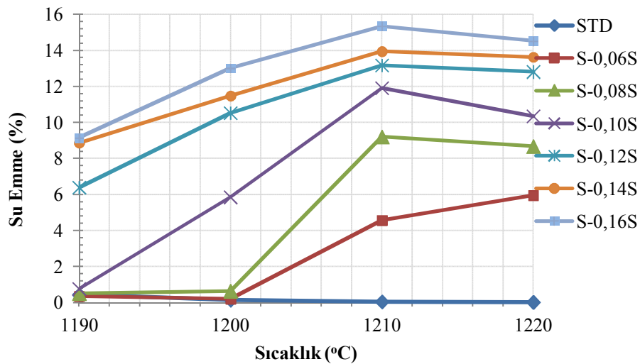
Şekil 7.26. Saf SiC (Sika) içeren standart bünyelerin sıcaklığa bağlı % su emme değişimi
