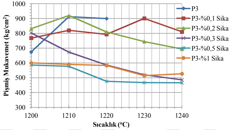
Şekil 7.83. P3 ve SiC (Sika) ilaveli P3 bünyelerinin sinterlenme sıcaklığına bağlı eğme mukavemeti değişimi.
