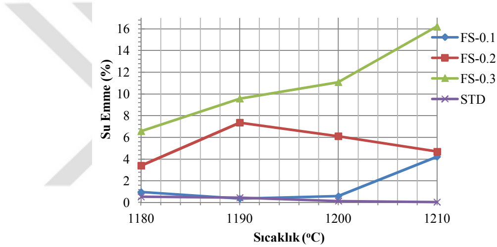
Şekil 7.6. Saf SiC katkılı bünyelerin katkı miktarına ve sıcaklığa bağlı su emme değerleri.
