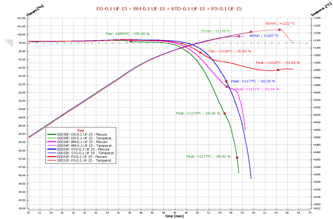
Şekil 7.92. Endüstriden temin edilen STD porselen karo bünye ile geliştirilen BM, D5 ve P3 bünyelerinin deformasyon davranışının karşılaştırmalı olarak incelenmesi
