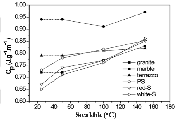
Şekil 3.2. Seramik yer karolarının sıcaklığa bağlı spesifik ısı değişimi ( C_p ) [35].
