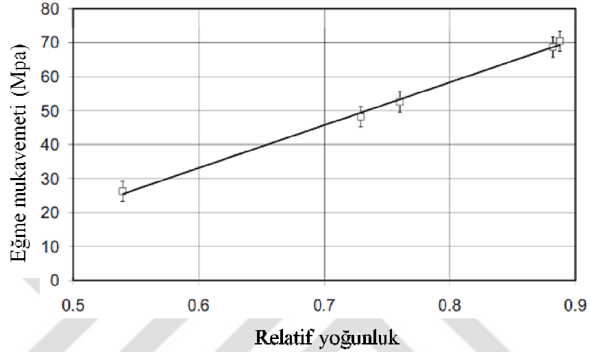
Şekil 7.4. Yoğunluğa bağlı eğme mukavemeti değişimi (Sıcaklık: 1200°C) [102].
