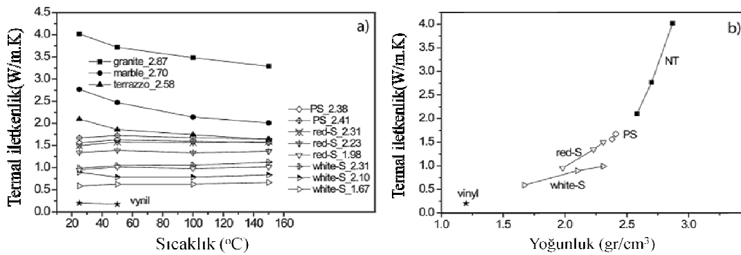
Şekil 3.3. Seramik yer karolarının oda sıcaklığında (a) sıcaklığa ve (b) yoğunluğa bağlı olarak değişen termal iletkenlik değerleri [35].
