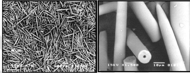
Görsel 5.1. Amorf silika fiberleri SEM görüntüsü (75X ve 1500X) [80]
