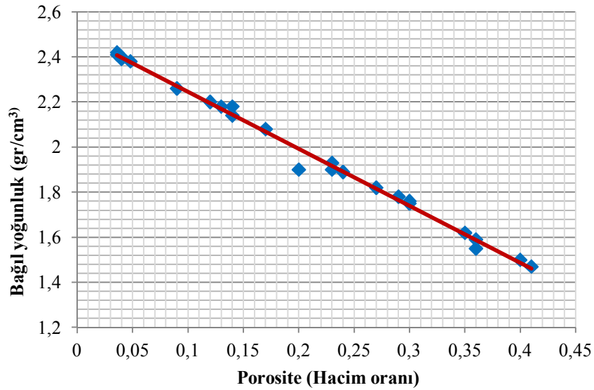
Şekil 7.38. Porozite hacmine bağlı bağıl yoğunluktaki değişim
