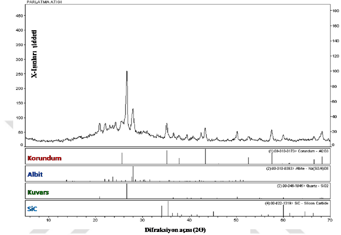
Şekil 6.1. Parlatma atığının minerolojik analizi
