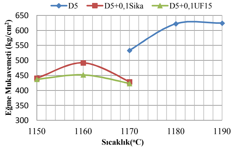
Şekil 7.69. D5 ve SiC katkılı D5 bünyelerinin sıcaklığa bağlı eğme mukavemeti
