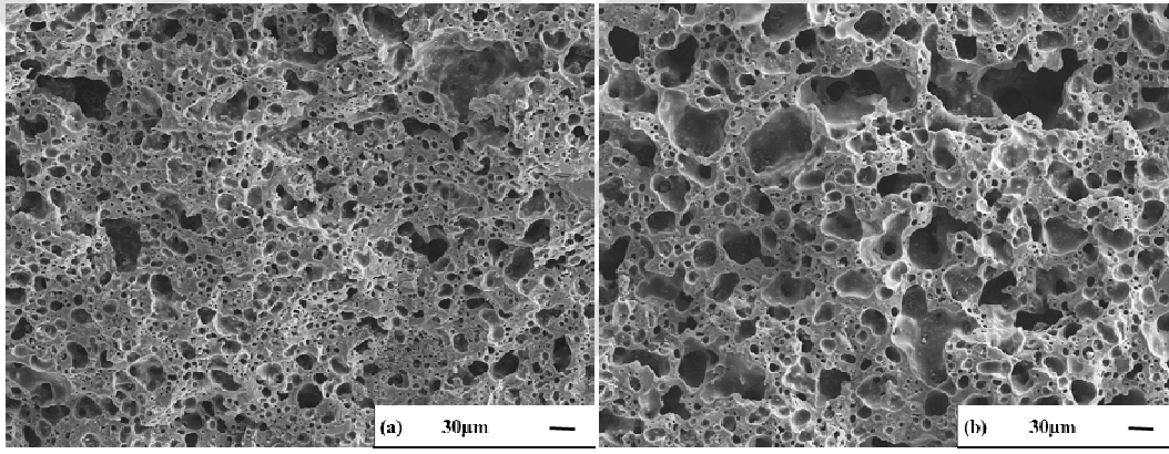
Görsel 7.15. (a) 1210 ( \rho: 1,64 \text{ gr/cm}^3 ), ve (b) 1220°C ( \rho: 1,51 \text{ gr/cm}^3 ), tepe sıcaklığında sinterlenen S-0,17-S9 kodlu bünyelerin genel mikroyapıları
