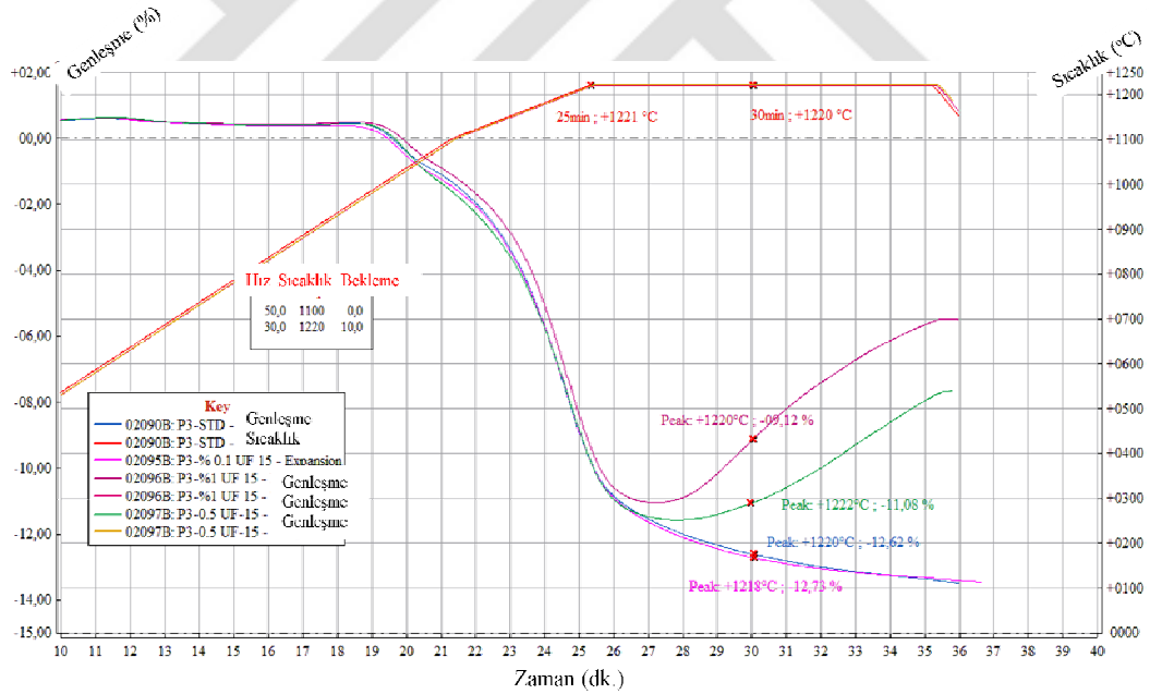
Şekil 7.87. P3 ve UF-15 kodlu SiC içeren P3 bünyelerinin 1220°C tepe sıcaklığında sinterlenme davranışının incelenmesi
