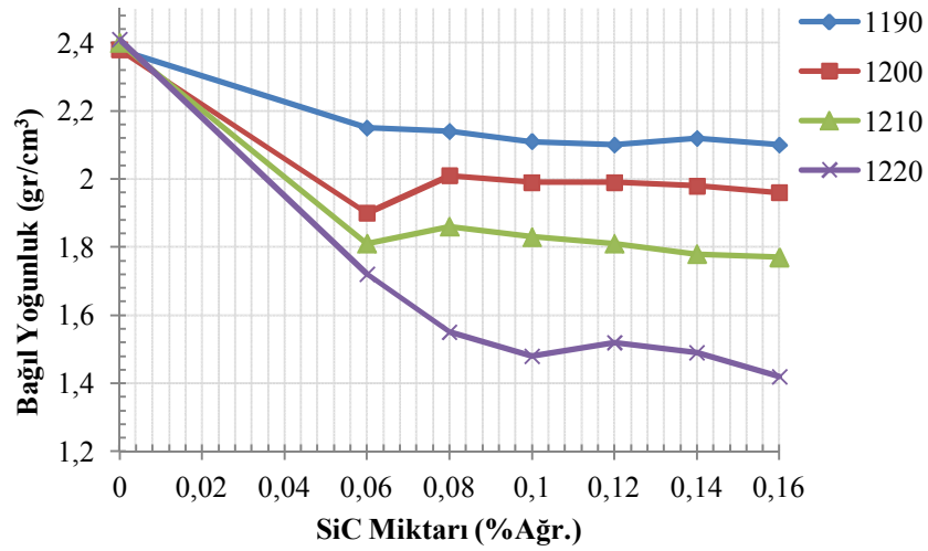
Şekil 7.35. Farklı sıcaklıklar için SiC (UF-15) miktarına bağlı yoğunluktaki değişim
