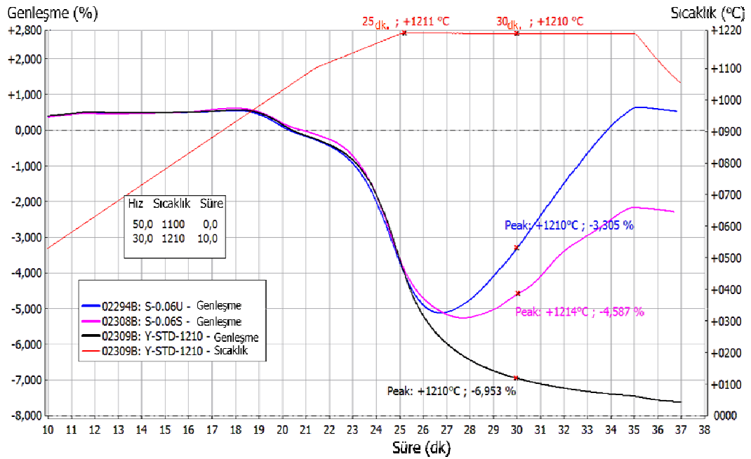
Şekil 7.48. Farklı tane boyutunda %0,06 oranında SiC (Sika, UF-15) içeren bünyelerin 1210°C tepe sıcaklığında sinterlenme davranışlarının incelenmesi
