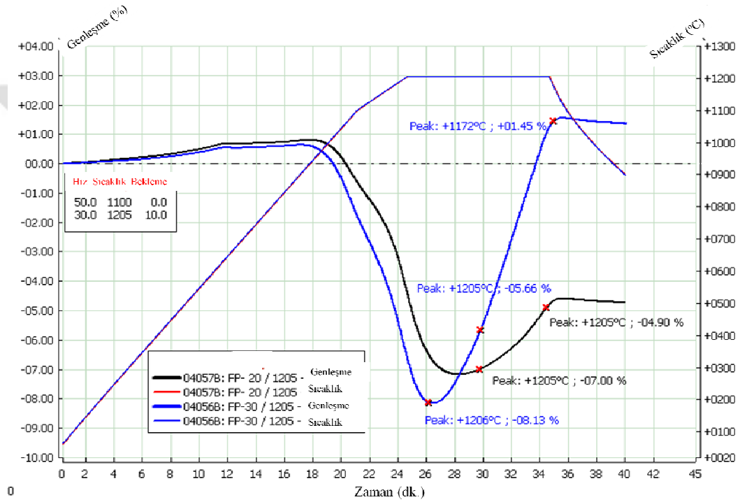
Şekil 7.16. %20 ve %30 oranında parlatma atığı katkılı bünyelerin 1205°C tepe sıcaklığında sinterlenme eğrilerinin karşılaştırılması
