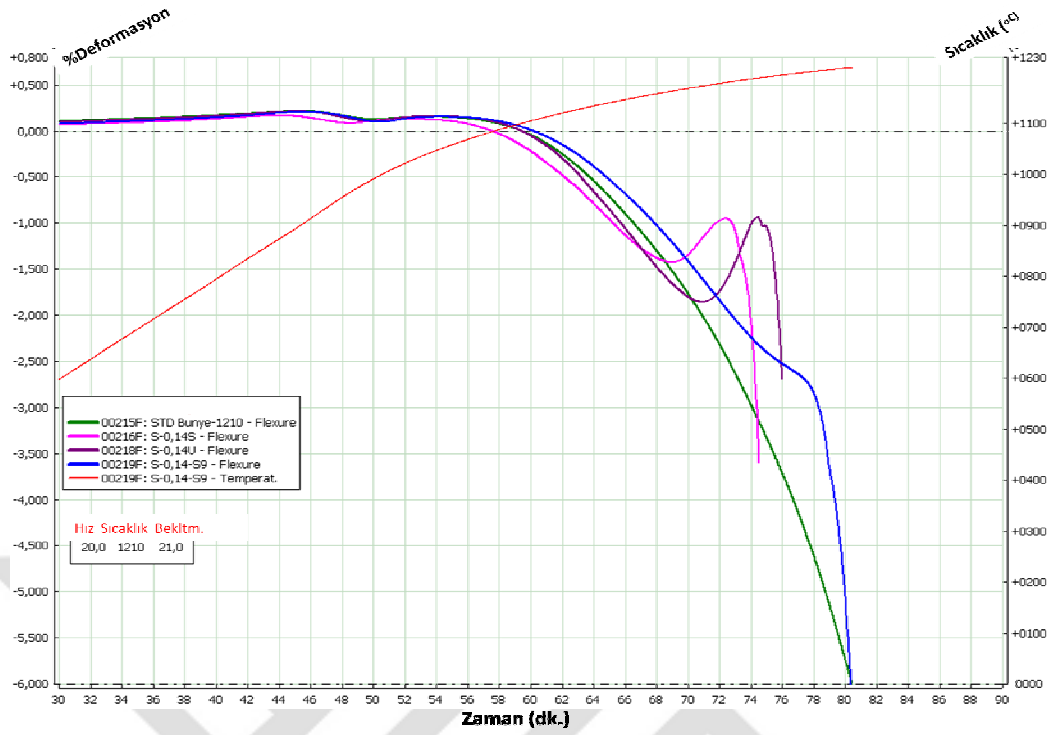
Şekil 7.55. %0,14 oranında Sika, UF-15 ve SiC-Lab. kodlu silisyum karbür katkılı bünyelerin zamana ve sıcaklığa bağlı deformasyon davranışı
