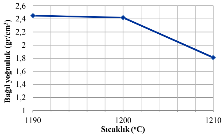
Şekil 7.10. %6 oranında \text{CeO}_2 katkılı bünyelerin katkı miktarına ve sıcaklığa bağlı yoğunluk değişimi
