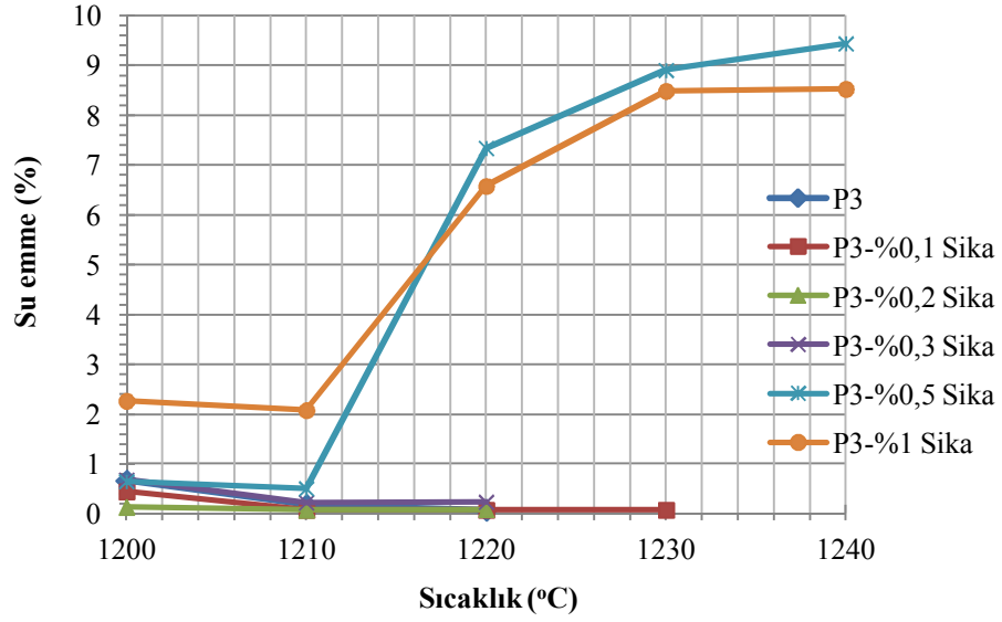
Şekil 7.79. P3 ve SiC (Sika) katkılı P3 bünyelerinin sinterlenme sıcaklığına bağlı (%) su emme değerleri
