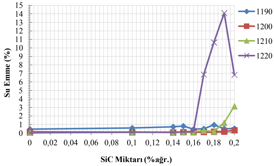
Şekil 7.41. Farklı sıcaklıklar için SiC ( d_{90} : \sim 9 \mu m ) miktarına bağlı % su emme değişimi
