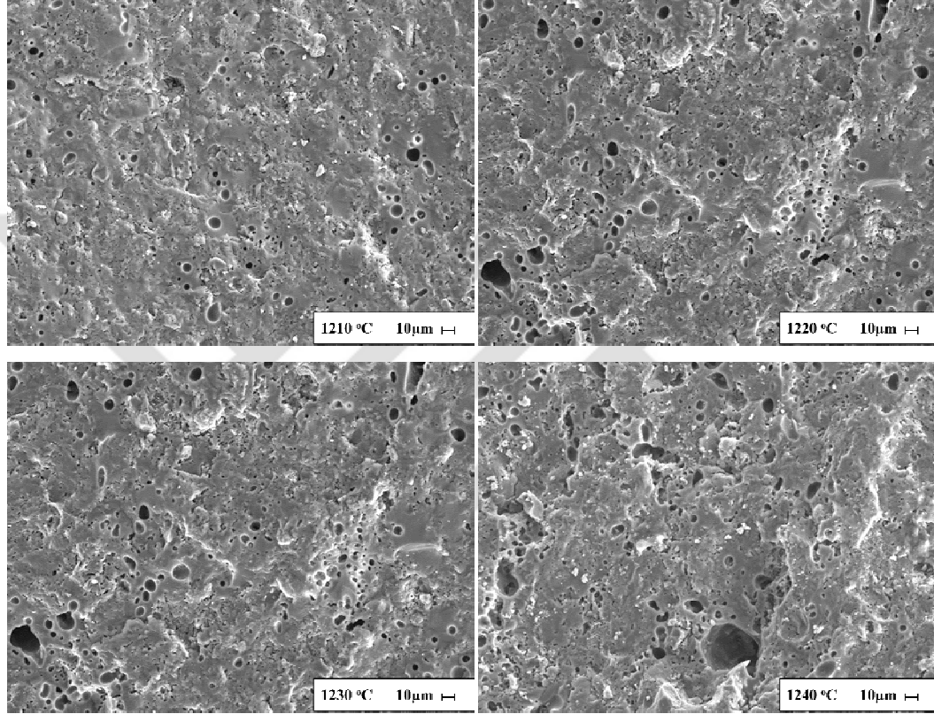
Görsel 7.36. %0,5 UF-15 kodlu SiC katkılı P3 bünyesinin sıcaklığa bağlı mikroyapı gelişimi
