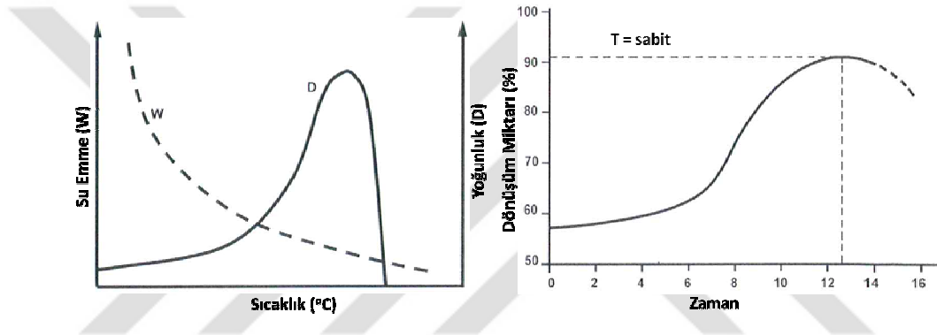
Şekil 4.5. (a) Vitrifikasyon diyagramı, (b) İzotermal dönüşüm diyagramı [73]
