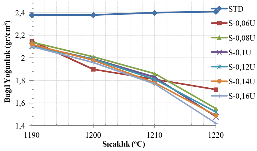
Şekil 7.34. Saf SiC (UF-15) içeren bünyelerin sıcaklığa bağlı yoğunluk değerlerindeki değişim
