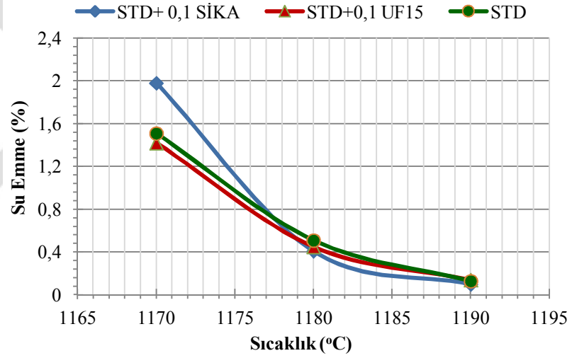
Şekil 7.60. STD ve SiC katkıli standart bünyelerin sıcaklığa bağlı % su emme değişimi
