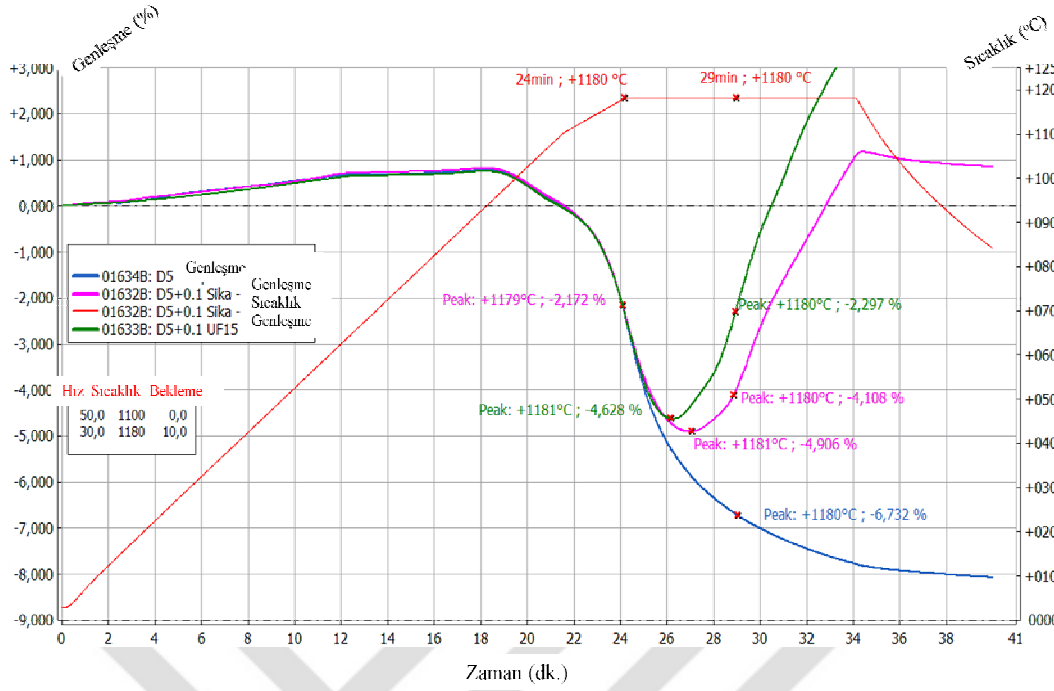
Şekil 7.72. D5 ve SiC içeren D5 bünyelerinin 1180°C tepe sıcaklığında sinterlenme davranışının incelenmesi
