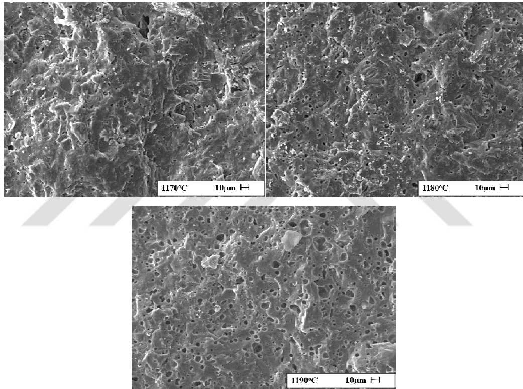
Görsel 7.21. STD+0,1UF-15 kodlu karoların sıcaklığa bağlı mikroyapı gelişimi ( \rho_{1170} :2,49gr/cm 3 , \rho_{1180} :2,27gr/cm 3 , \rho_{1190} :2,13gr/cm 3 )
