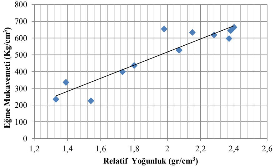
Şekil 7.5. Porselen karo parlatma atığı katkıli bünyelerde yoğunluğa bağlı eğme mukavemeti değişimi (Sinterlenme sıcaklığı: 1180, 1190, 1200°C)
