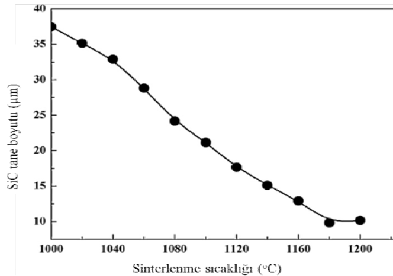
Şekil 5.8. Sinterlenme sıcaklığının SiC tane boyutuna etkisi [95].
