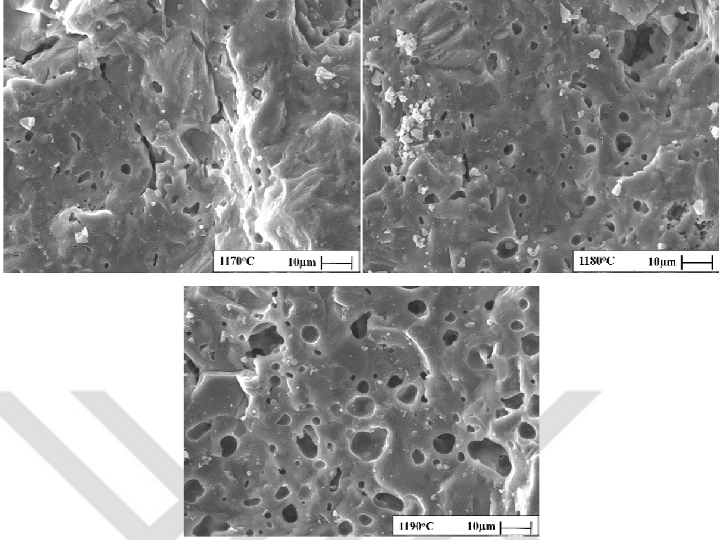
Görsel 7.22. Yüksek büyütmede STD+0,1UF-15 kodlu karoların sıcaklığa bağlı mikroyapı gelişimi ( \rho_{1170}: 2,49 \text{ gr/cm}^3 , \rho_{1180}: 2,27 \text{ gr/cm}^3 , \rho_{1190}: 2,13 \text{ gr/cm}^3 )
