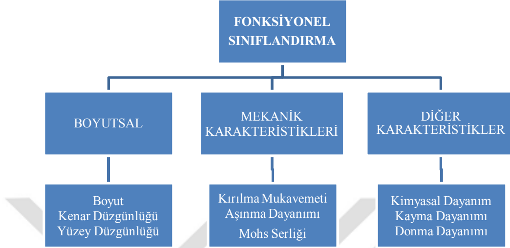
Şekil 2.1. Seramik karoların fonksiyonel sınıflandırması [5].
