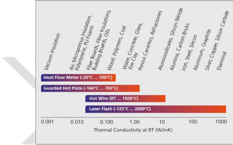
Şekil 3.4. Termal iletkenlik ölçüm metotları [40]
