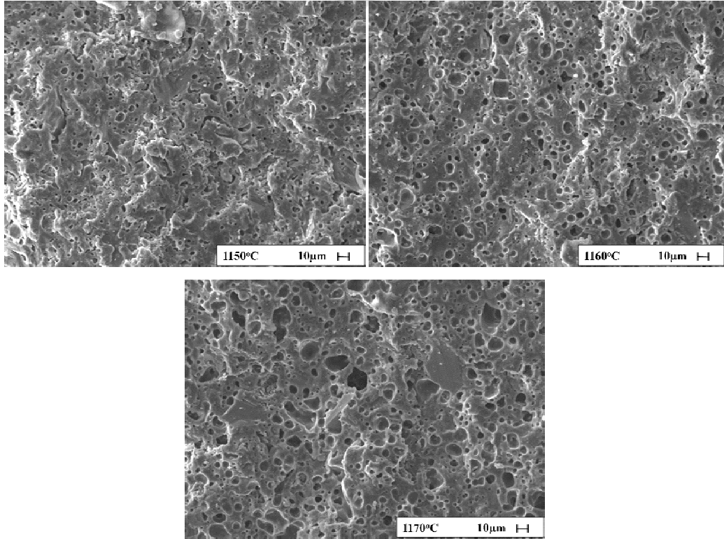
Görsel 7.29. D5+0,1UF15 kodlu karoların sıcaklığa bağlı mikroyapı gelişimi ( \rho_{1150} :2,49gr/cm 3 , \rho_{1160} :2,30gr/cm 3 , \rho_{1170} :1,88gr/cm 3 )
