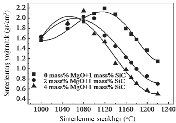
Şekil 5.14. Farklı oranlarda MO ve SiC içeren bünyelerin sinterlenme sıcaklığına bağlı yoğunluk değişimi [96].
