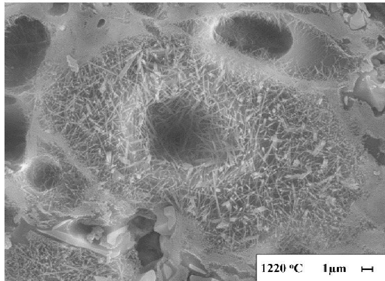
Görsel 7.34. %0,5 Sika katkılı P3 bünyesinde por etrafındaki müllit gelişimi
