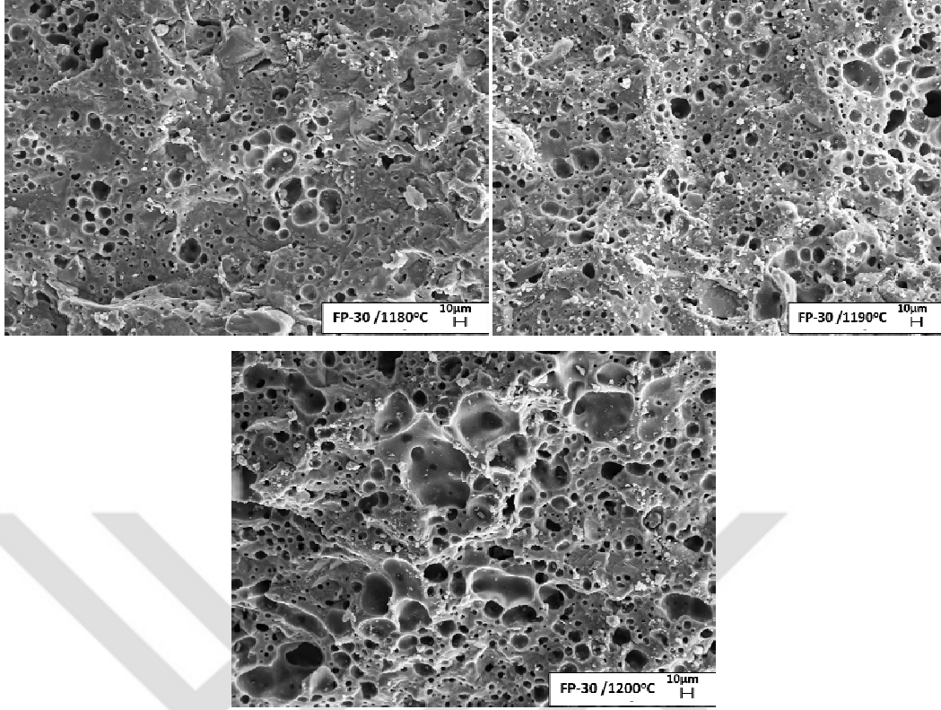
Görsel 7.2. Farklı sıcaklıklarda sinterlenen FP-30 bünyesi genel mikroyapı görüntüsü. (\rho_{1180}: 2,07\text{gr/cm}^3, \rho_{1190}: 1,8\text{gr/cm}^3, \rho_{1200}: 1,54\text{gr/cm}^3)
