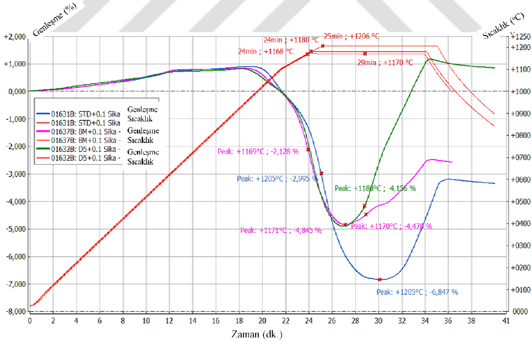
Şekil 7.73. %0,1 oranında Sika içeren D5, BM ve STD bünyelerinin sinterlenme davranışının karşılaştırılması
