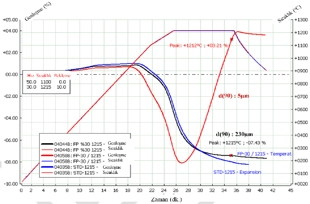
Şekil 7.23. %30 oranında farklı tane boyutuna sahip parlatma atığı katkılı bünyelerin ve standart bünyenin 1215°C tepe sıcaklığında sinterlenme eğrilerinin karşılaştırılması
