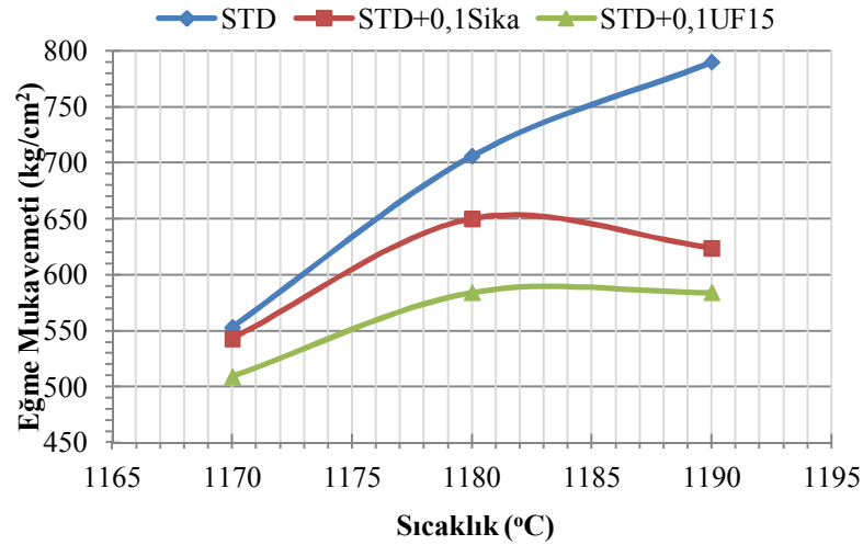
Şekil 7.62. STD ve SiC katkıli standart bünyelerin sıcaklığa eğme mukavemeti değişimi
