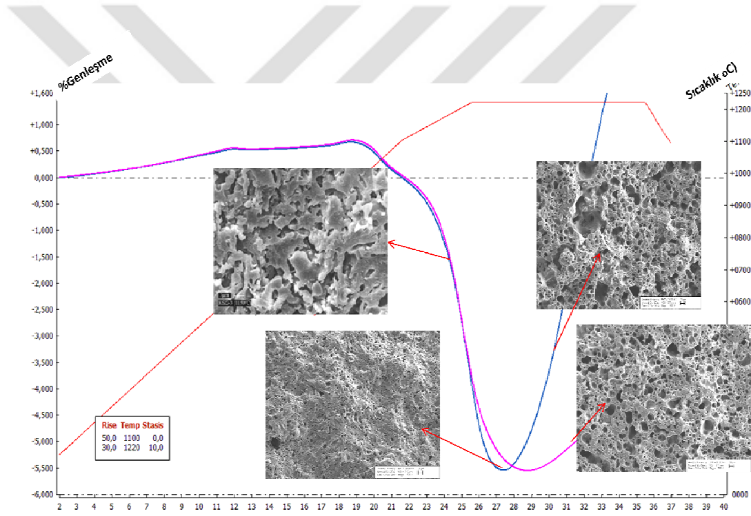
Görsel 7.18. 1220°C tepe sıcaklığında sinterlenen S-0,15-S9 ve S-0,19-S9 kodlu bünyelerinin sinterlenmeye bağlı mikroyapı gelişimleri
