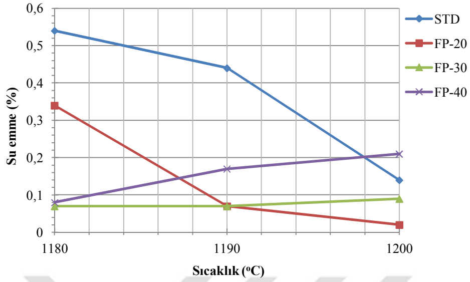
Şekil 7.1. Porselen karo parlatma atığı katkıli bünyelerin sıcaklığa bağlı su emme değerleri
