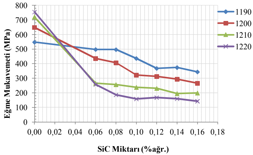
Şekil 7.31. Farklı sıcaklıklar için SiC (Sika) miktarına bağlı eğme mukavemetindeki değişim
