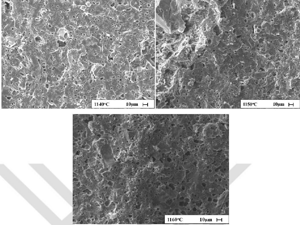
Görsel 7.23. BM+0,1Sika kodlu karoların sıcaklığa bağlı mikroyapı gelişimi ( \rho_{1140} :1,97gr/cm 3 , \rho_{1150} :2,30gr/cm 3 , \rho_{1160} :2,38gr/cm 3 )
