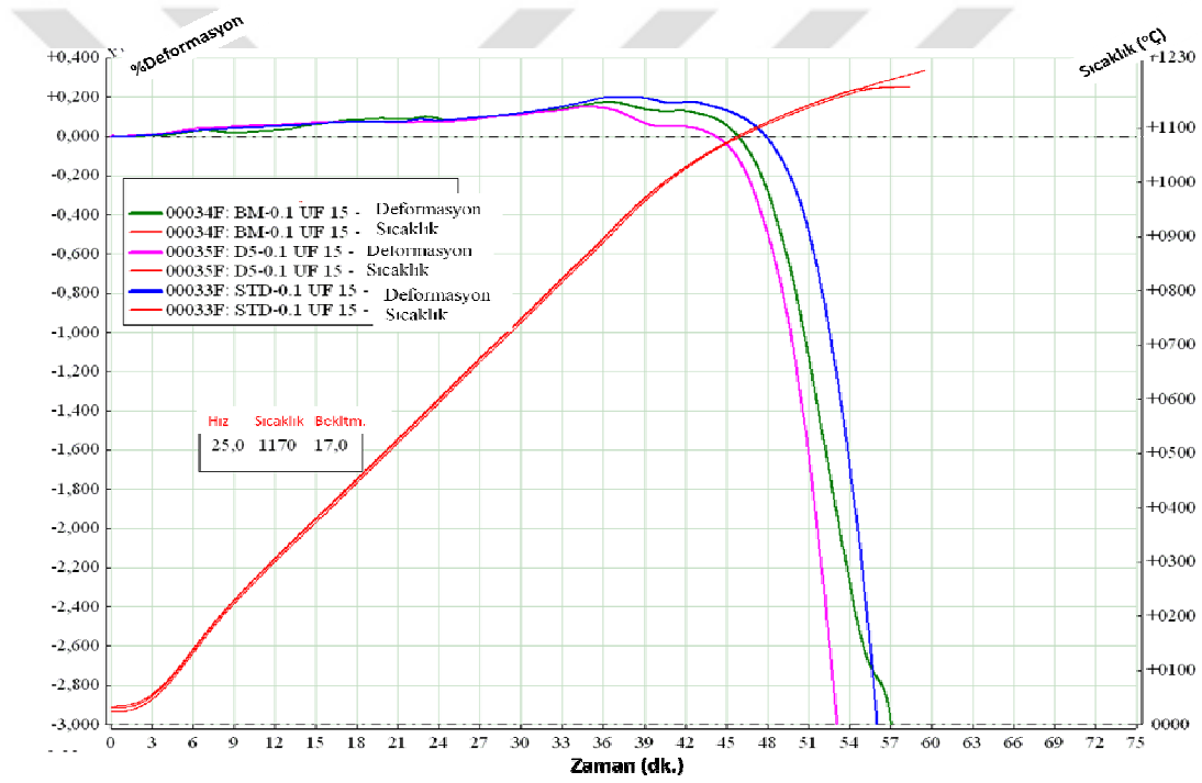
Şekil 7.75. %0,1 oranında Sika ve UF-15 kodlu silisyum karbür katkılı bünyelerin zamana ve sıcaklığa bağlı deformasyon davranışı
