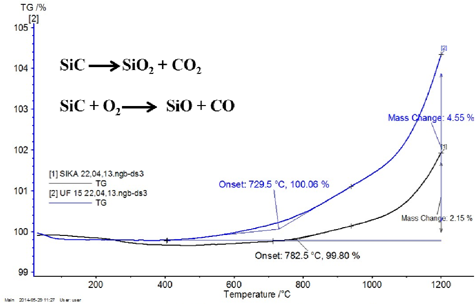
Şekil 7.25. Sika ve UF-15 kodlu SiC tozlarının sıcaklığa bağlı TG eğrisi
