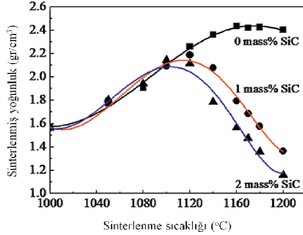
Şekil 5.13. %1 ve 2 oranında SiC ilave edilmiş bünyelerin sinterlenme sıcaklığına bağlı yoğunluk değişimi [96].
