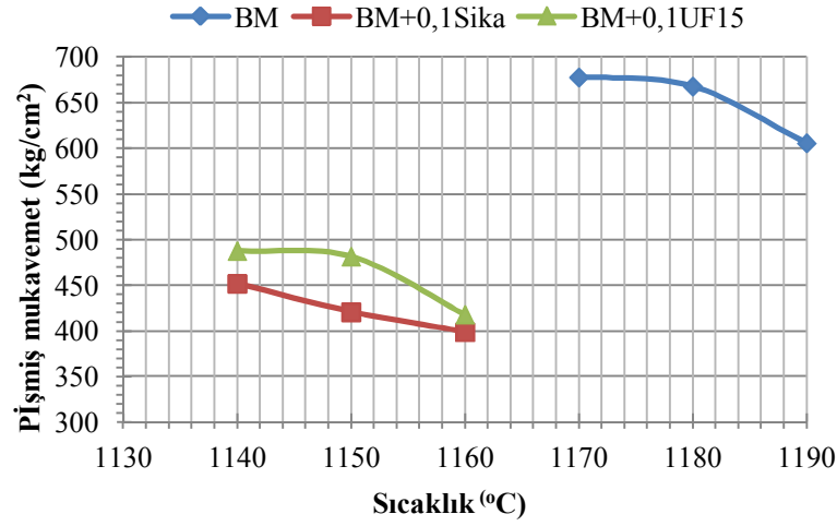
Şekil 7.65. BM ve SiC katkılı BM bünyelerinin sıcaklığa bağlı eğme mukavemeti
