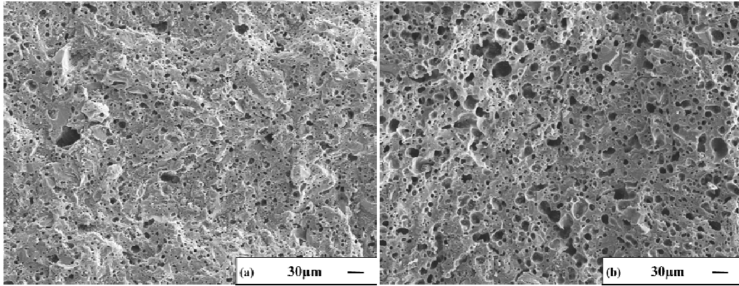
Görsel 7.12. (a)1210 ( \rho:1,86\text{gr/cm}^3 ), ve (b)1220°C ( \rho:1,57\text{gr/cm}^3 ), tepe sıcaklığında sinterlenen S-0,14-S9 kodlu bünyelerin genel mikroyapıları
