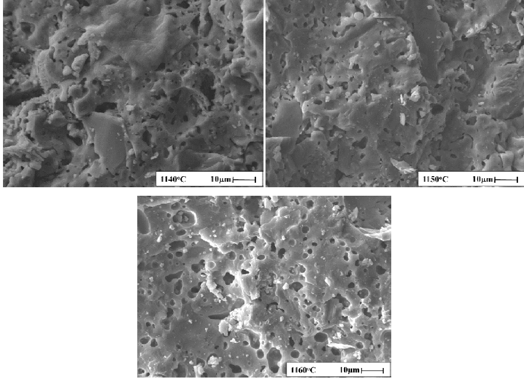
Görsel 7.26. Yüksek büyütmede BM+0,1UF15 kodlu karoların sıcaklığa bağlı mikroyapı gelişimi ( \rho_{1140} : 2,51gr/cm 3 , \rho_{1150} : 2,40gr/cm 3 , \rho_{1160} : 2,15gr/cm 3 )
