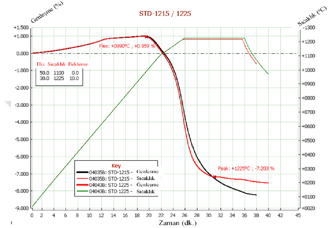
Şekil 7.12. Standart teknik porselen karonun 1215 ve 1225°C tepe sıcaklığında sinterlenme davranışının incelenmesi.
