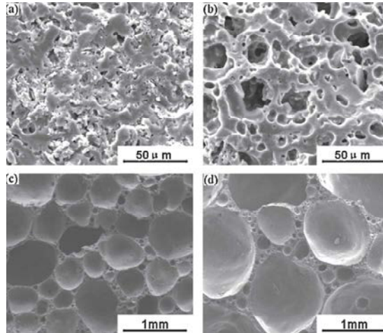
Görsel 5.3. Porselen karo atığı içeren bünyelerin sinterlenme sonrası SEM görüntüleri. (a) 1060^{\circ}\text{C} , (b) 1080^{\circ}\text{C} , (c) 1120^{\circ}\text{C} , (d) 1160^{\circ}\text{C} [96].
