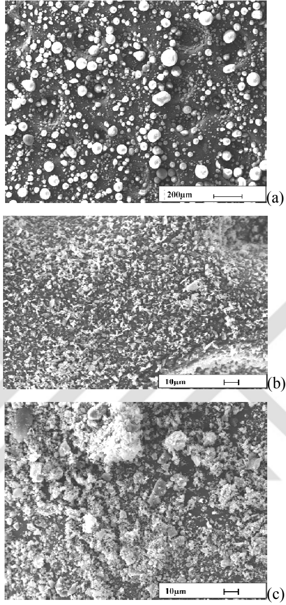
Görsel 6.1. Farklı tane boyutuna sahip saf SiC tozları mikroyapı görüntüleri (a) Sika, (b)UF-15, (c) SiC-Lab.
