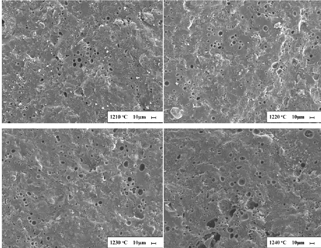
Görsel 7.38. %1 UF-15 ilaveli P3 bünyesinin sıcaklığa bağlı mikroyapı gelişimi
