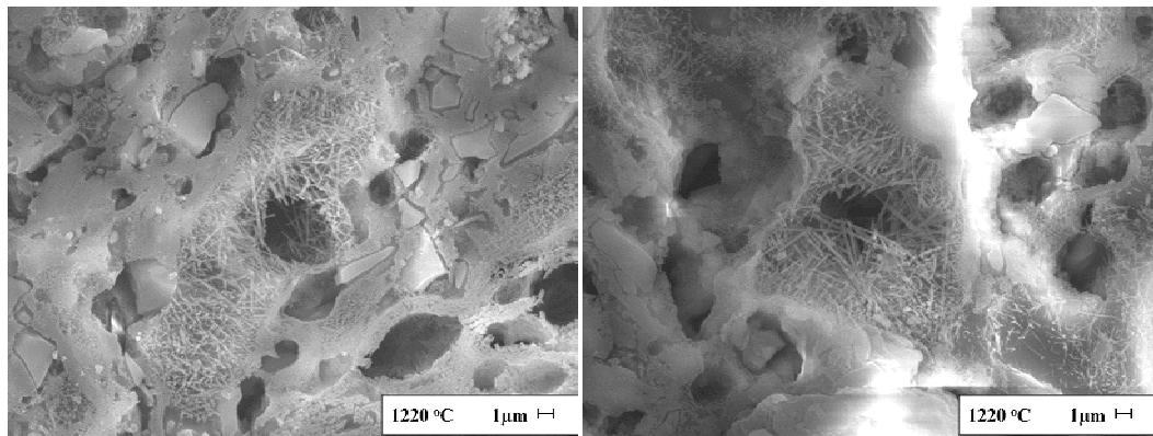
Görsel 7.40. %1 UF-15 katkılı P3 bünyesinde por etrafındaki müllit gelişimi
