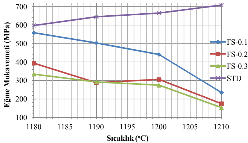
Şekil 7.8. Saf SiC katkılı bünyelerin katkı miktarına ve sıcaklığa bağlı eğme mukavemeti değişimi.
