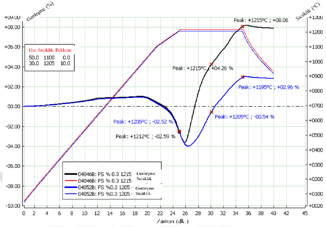
Şekil 7.20. %0,3 oranında saf SiC katkılı bünyenin 1205 ve 1215°C tepe sıcaklığında sinterlenme davranışının incelenmesi
