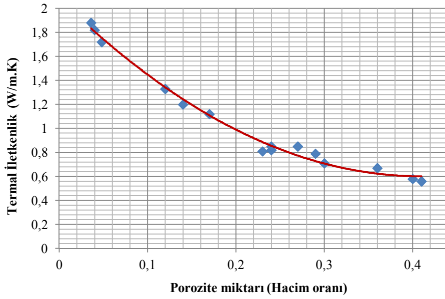
Şekil 7.58. SiC katkılı porselen karo bünyelerde por hacmine bağlı termal iletkenlik değişimi
