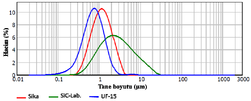
Şekil 6.2. Kullanılan SiC tozları tane boyut dağılımı
