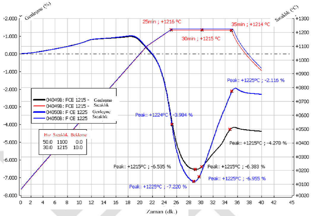
Şekil 7.24. %6 oranında CeO_2 ilaveli bünyenin 1215 ve 1225°C tepe sıcaklığında sinterlenme davranışının incelenmesi
