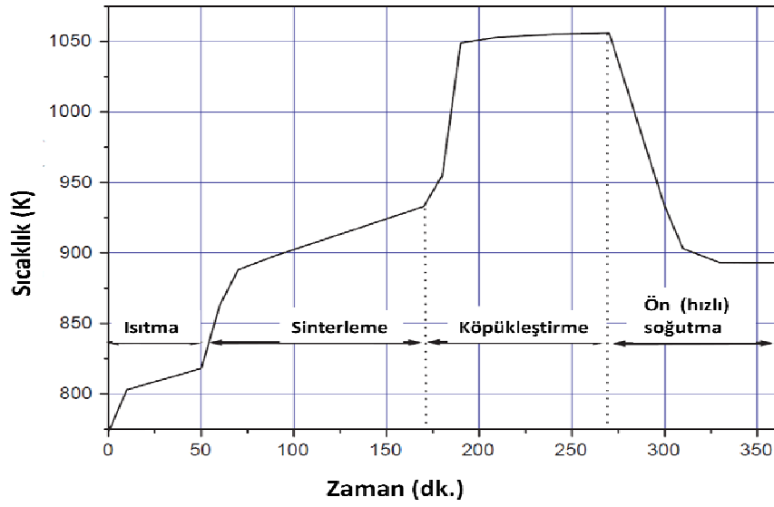
Şekil 5.1. Schulz [78] tarafından geliştirilen zaman ve sıcaklığa bağlı cam köpükleştirme aşamaları
