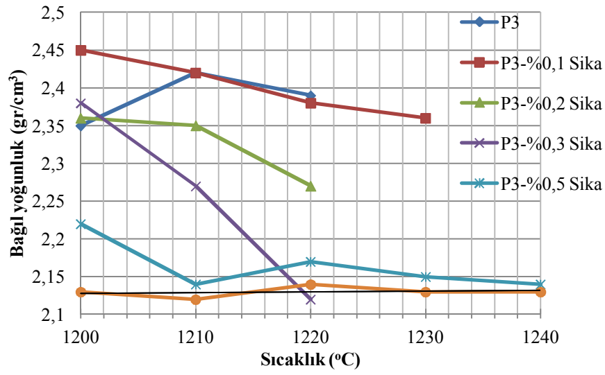
Şekil 7.81. P3 ve SiC (Sika) katkılı P3 bünyelerinin sinterlenme sıcaklığına bağlı yoğunluk değerleri
