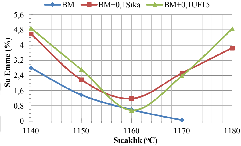
Şekil 7.63. BM ve SiC katkılı BM bünyelerinin sıcaklığa bağlı % su emme değişimi
