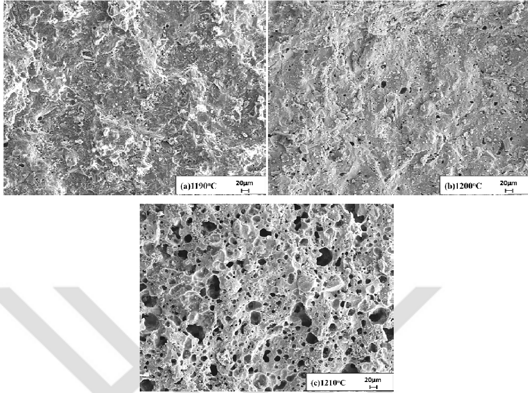
Şekil 7.10. FCe bünnyeleri ( \rho_{1190} : 2,45gr/cm 3 , \rho_{1200} : 2,42gr/cm 3 , \rho_{1210} : 1,81gr/cm 3 )
