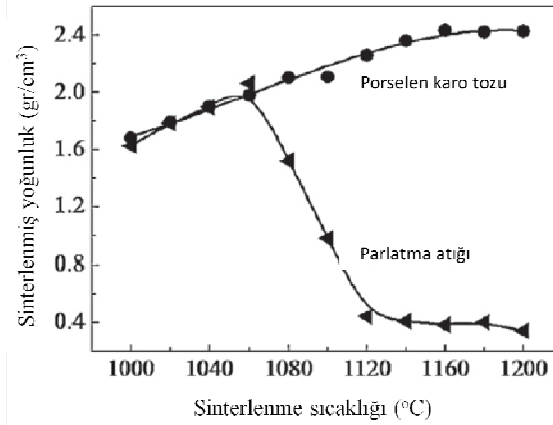
Şekil 5.12. Sıcaklığa bağlı pişmiş yoğunluk değişimi ( 5^{\circ}\text{C}/\text{dk} , 1000\text{-}1200^{\circ}\text{C} -20dk).
