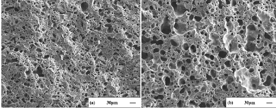
Görsel 7.14. (a) 1210 ( \rho: 1,68 \text{ gr/cm}^3 ), ve (b) 1220°C ( \rho: 1,47 \text{ gr/cm}^3 ), tepe sıcaklığında sinterlenen S-0,16-S9 kodlu bünyelerin genel mikroyapıları
