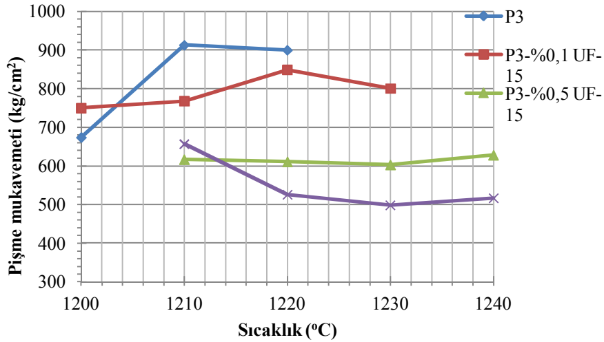
Şekil 7.84. P3 ve SiC (UF-15) ilaveli P3 bünyelerinin sinterlenme sıcaklığına bağlı eğme mukavemeti değişimi.
