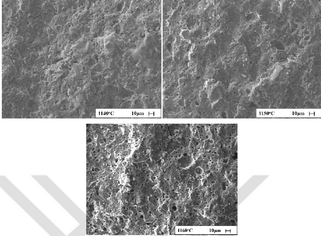
Görsel 7.25. BM+0,1UF15 kodlu karoların sıcaklığa bağlı mikroyapı gelişimi ( \rho_{1140} : 2,51gr/cm 3 , \rho_{1150} : 2,40gr/cm 3 , \rho_{1160} : 2,15gr/cm 3 )
