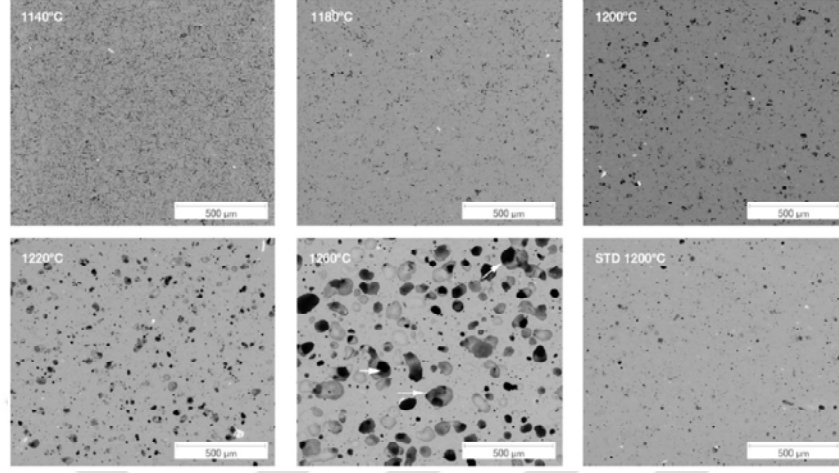
Görsel 5.2. STD ve %0,2 SiC ( d_{50} : 9,3 \mu\text{m} ) katkıli bünyelerin sıcaklığa bağlı mikroyapı gelişimi [94].
