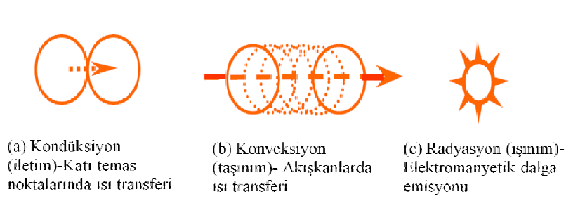
Şekil 3.5. Temel ısı transfer mekanizmaları; (a)Kondüksiyon, partiküller arası temas, (b)Konveksiyon, akışkan içerisinde iletim, (c) Işınım, elektromanyetik dalgalar ile iletim [42].
