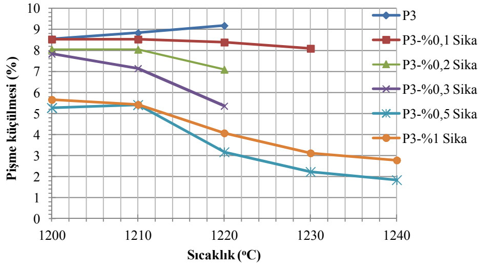
Şekil 7.77. P3 ve SiC (Sika) katkı P3 bünyelerinin sinterlenme sıcaklığına bağlı pişme küçülmeleri (%).
