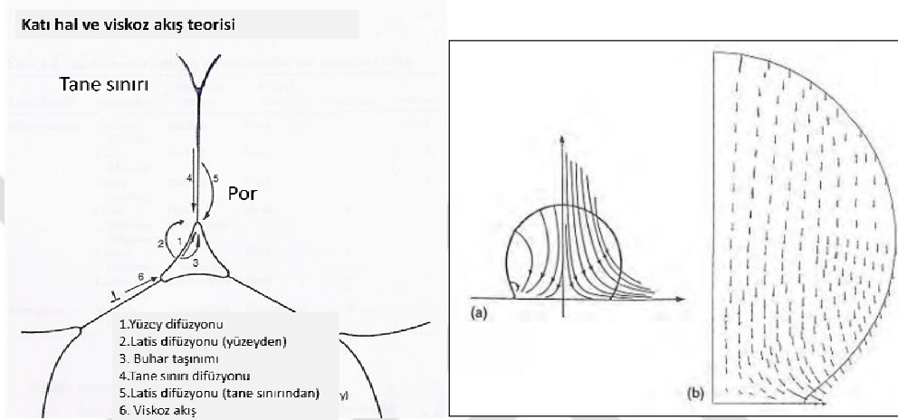
Şekil 4.1. Sinterlemenin ilk aşamalarında malzeme taşınım mekanizmaları [49].
