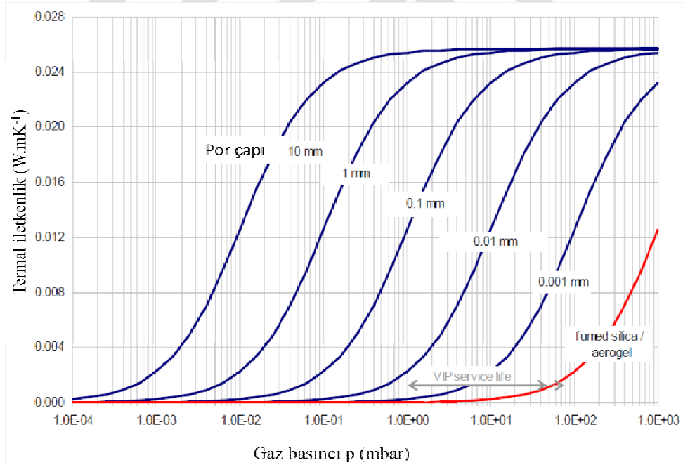
Şekil 3.6. Gaz basıncına ve por boyutuna bağlı termal iletkenlik değişimi [42-46].
