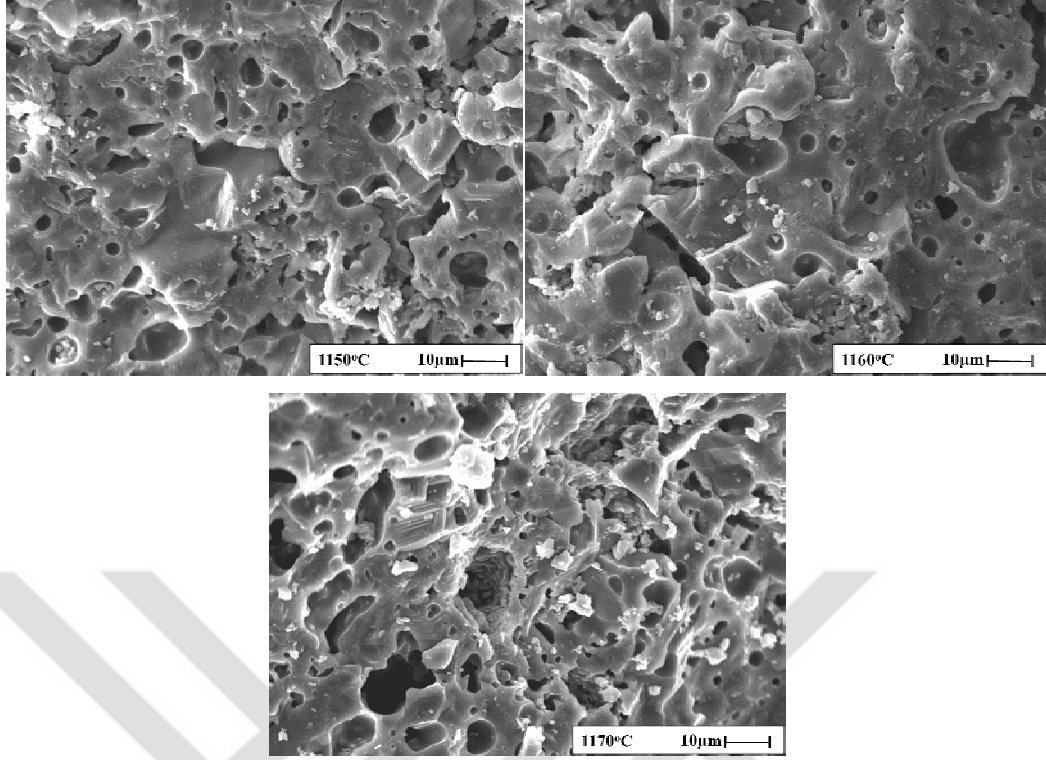
Görsel 7.28. Yüksek büyütmede D5+0,1Sika kodlu karoların sıcaklığa bağlı mikroyapı gelişimi ( \rho_{1150} :2,46gr/cm 3 , \rho_{1160} :2,37gr/cm 3 , \rho_{1170} :1,91gr/cm 3 )
