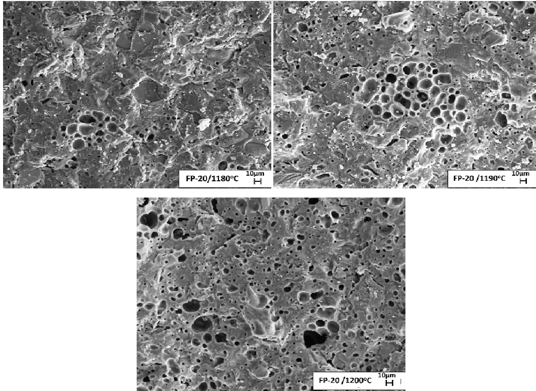
Görsel 7.1. Farklı sıcaklıklarda sinterlenen FP-20 bünyesi genel mikroyapı görüntüsü ( \rho_{1180} : 2,28gr/cm 3 , \rho_{1190} : 2,19gr/cm 3 , \rho_{1200} : 1,98gr/cm 3 )
