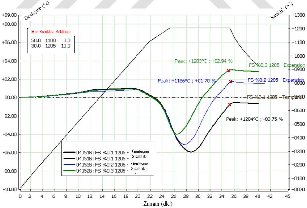
Şekil 7.21. % 0,1, 0,2 ve 0,3 oranında saf SiC katkılı bünyelerin 1205°C tepe sıcaklığında sinterlenme eğrilerinin karşılaştırılması
