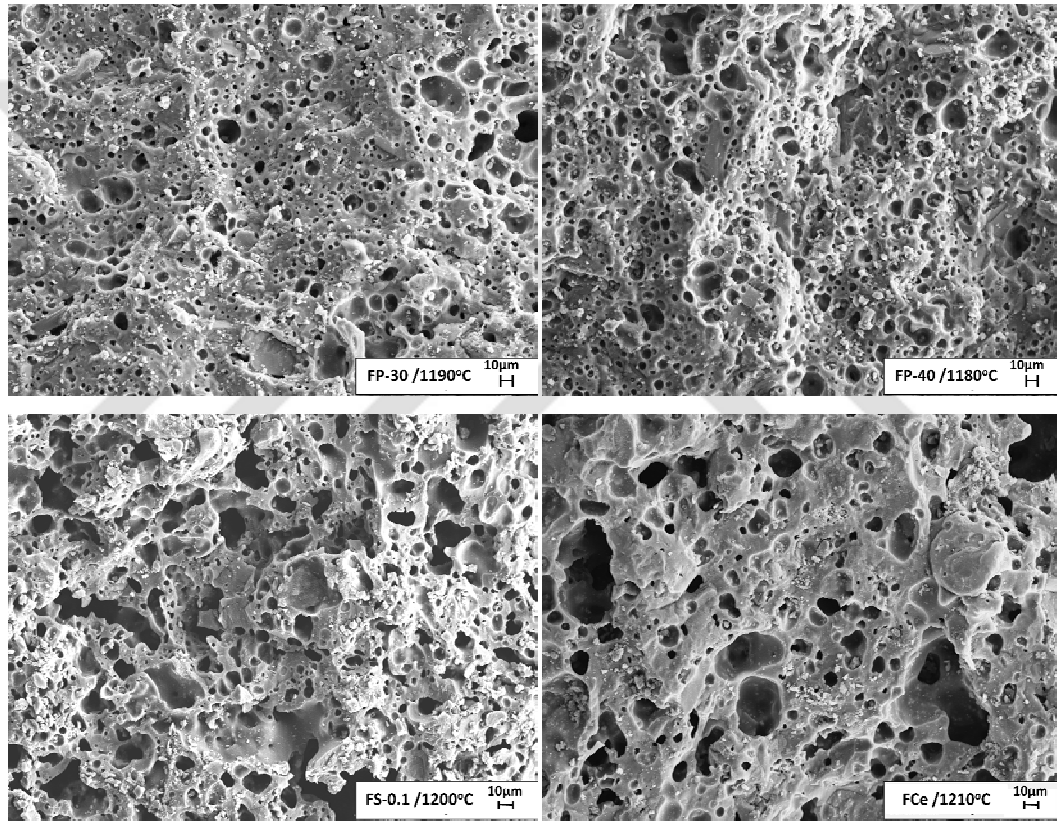
Şekil 7.11. FP-30 ( 1,8\text{gr/cm}^3 ); FP-40 ( 1,73\text{gr/cm}^3 ), FS-0.1 ( 1,82\text{gr/cm}^3 ) bünyeleri genel mikroyapı görüntüleri kıyaslaması
