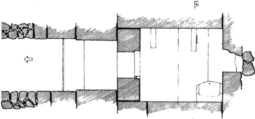
Resim 30. Bekçitepe Tmls Planı (Din 1993, Fig. 234.)
