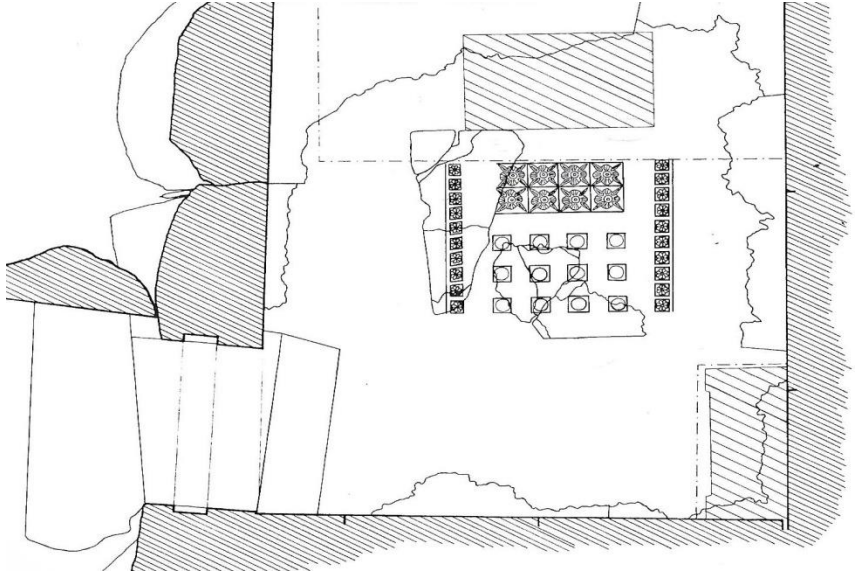
Resim 176. . Kızılbel Tmls, Mezar Odası Zemin Planı (Mellink 1998, Fig.3.1)
