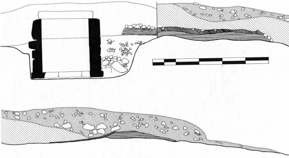
Resim 113. Kızılbel Tmls, Mezar Odası, Kesit (Mellink 1998, Pl. 2)
