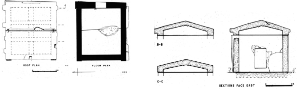
Resim 105. Müğren Tümlüsü, Mezar odasının W.W. Cummer'a ait Plan ve Kesitleri (Tiryaki 2015, Fig. 5a-b)
