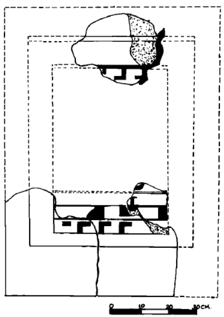
Resim 26. Hamamtepe Tümlüsü, Kapı Bloğu (Dinç-Önder 1992, Çiz.3).
