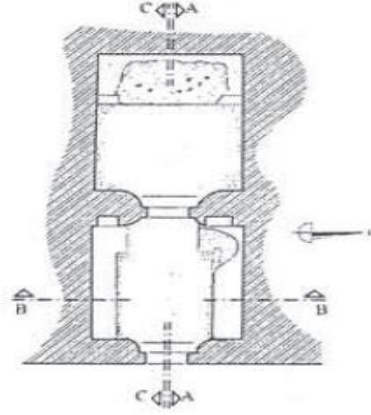
Resim 198. Baruthane Güney Tümlüsü Planı (Atasoy-Endoğlu-Dönmez 2005, Plan.1 )
