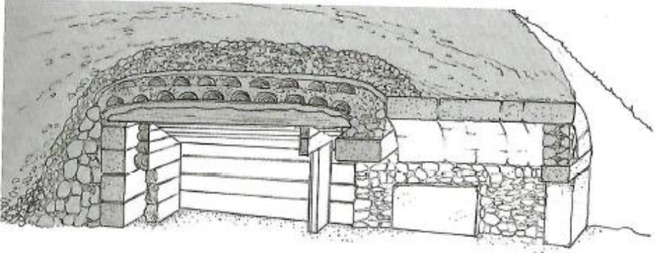
Resim 64. Tatarlı Tümülüsü, Kesit (von Kienlin 2010, Res.No.2)
