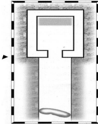
Resim 52. Aktepe Tümü, Mezar Odası Plan (Özgen-Öztürk 1996, Fig. 71).
