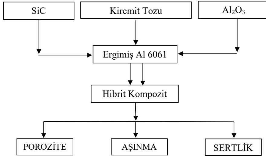
řekil 10: Kompozit üretim yöntemi ve aşamaları.
