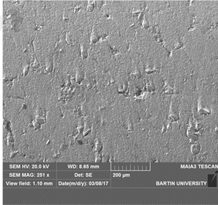
Şekil 20: Kompozitlerin elektron mikroskobu görüntüsü.
