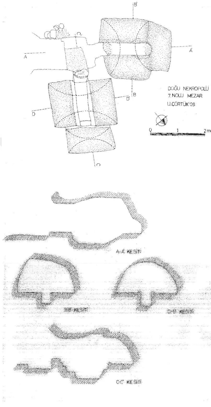
Res. 52: Tripolis Doğu Nekropolisi kaya mezarının çizimi 7 no.lu (2007-2009 Tripolis kazı arşivi)
