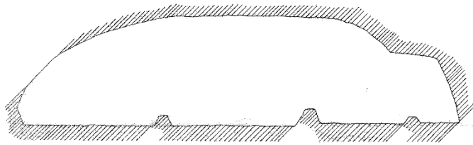
B.B' KESİTİ 3 NOLU MEZAR
