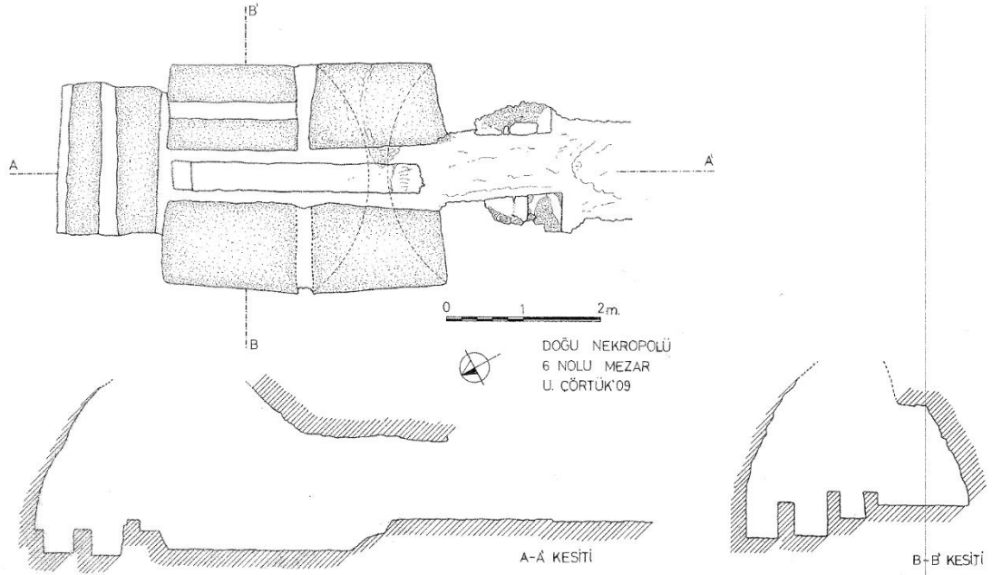
Res. 26: Tripolis Doğu Nekropolisi 6 no.lu kaya mezarının çizimi (2007-2009 Tripolis kazı arşivi)
