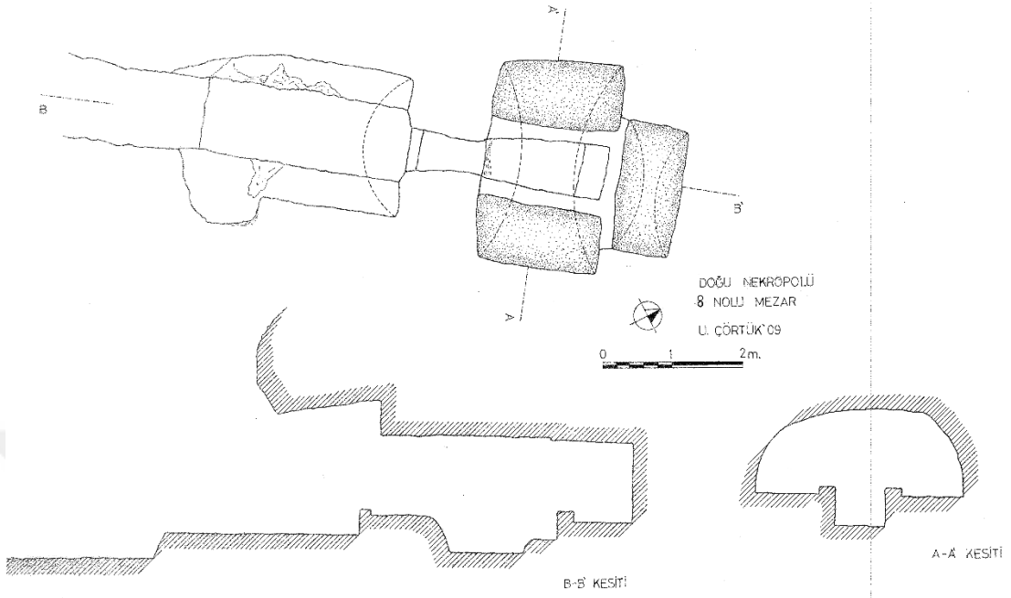
Res. 30: Tripolis Doğu Nekropolisi 8 no.lu kaya mezarı çizimi (2007-2009 Tripolis kazı arşivi)
