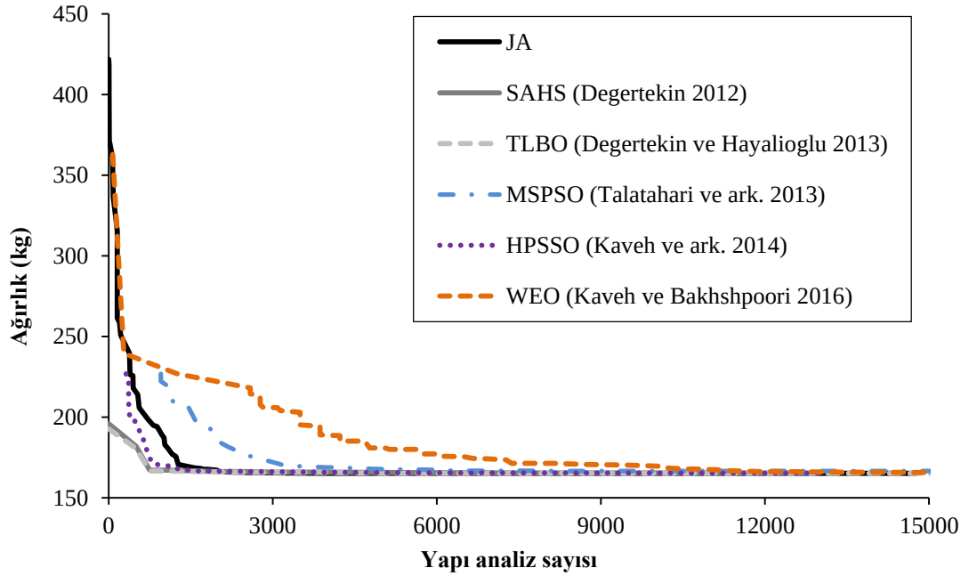
Şekil 4.14. 72 elemanlı sürekli tasarım değişkenli uzay kafes yapının optimizasyonunda yapı ağırlığının analiz sayısı ile değişimi (II. optimizasyon durumu)
