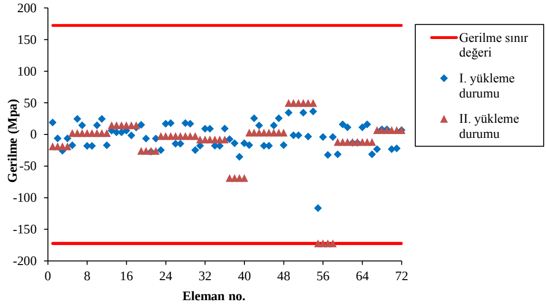
Şekil 4.8. 72 elemanlı sürekli tasarım değişkenli uzay kafes yapıda optimum tasarıma ait eleman gerilme değerleri (II. optimizasyon durumu)
