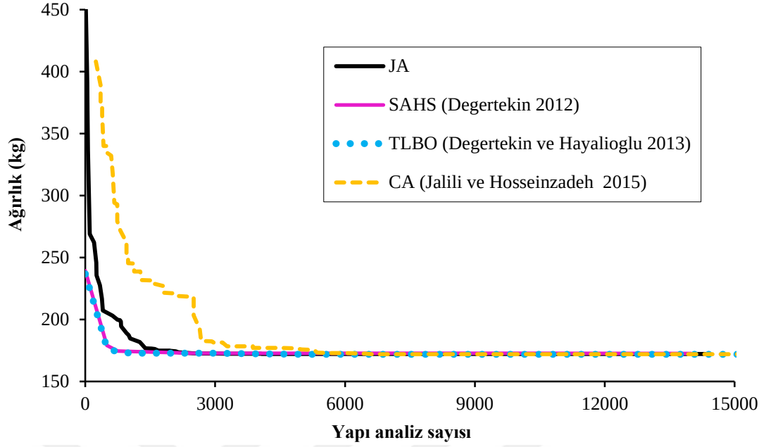
Şekil 4.13. 72 elemanlı sürekli tasarım değişkenli uzay kafes yapının optimizasyonunda yapı ağırlığının analiz sayısı ile değişimi (I. optimizasyon durumu)
