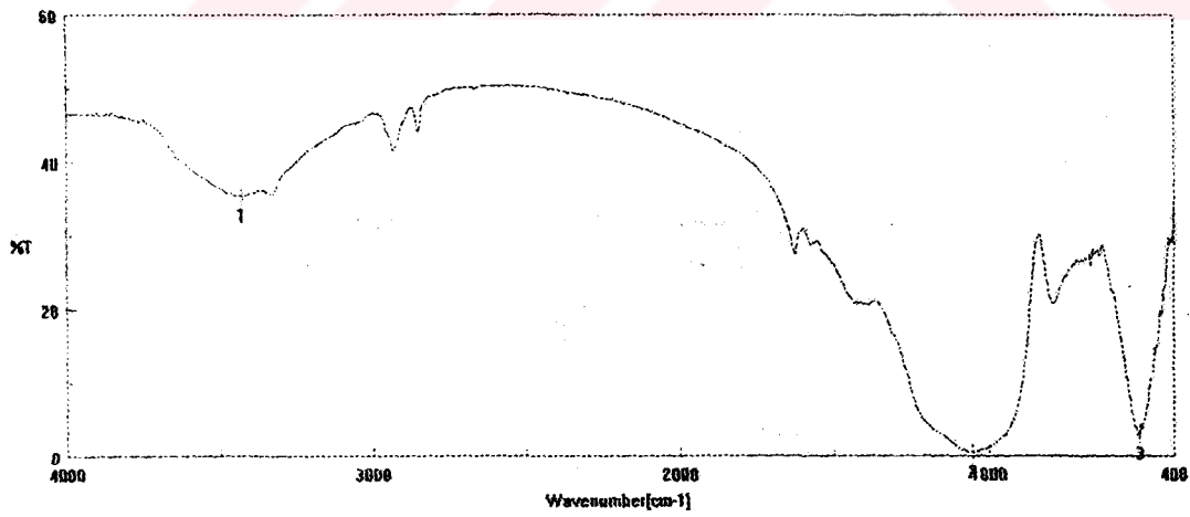
Şekil 3.8. Yüzeyi sistamin ile modifiye edilmiş cam mikroküreciklerin (NEL 1 D) infrared spektrumu
