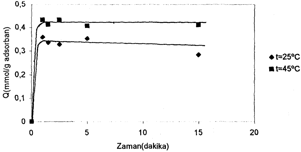
Şekil 3.19. Yüzeyi 2-aminoetantiyol ile modifiye edilmiş cam mikroküreciklere adsorplanan Cd(II) miktarının sıcaklık ile değişimi; Başlangıç derişimi : 100 ppm; pH : 4,60 Cam mikrokürecik miktarı : 50 mg;
