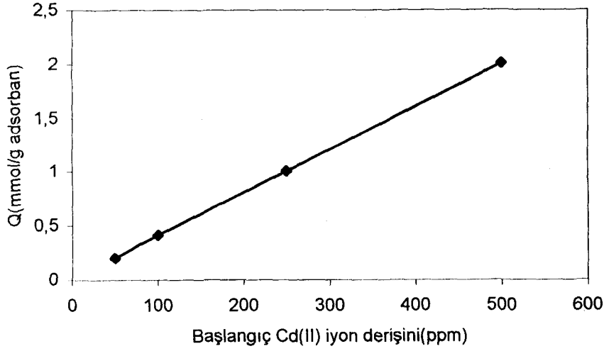
Şekil 3.12. Yüzeyi sistamin ile modifiye edilmiş cam mikroküreciklere adsorplanan Cd(II) miktarının Cd(II) başlangıç derişimi ile deęişimi; pH : 4,41; T : 25°C; Cam mikrokürecik miktarı : 50 mg; Zaman : 15 dakika
