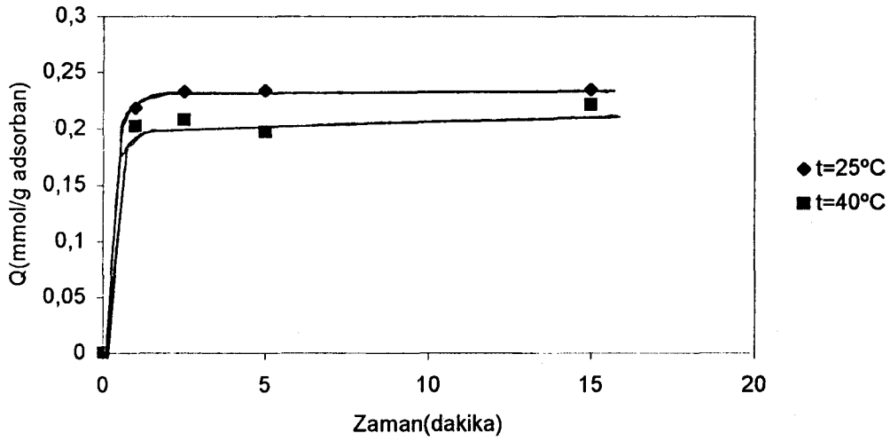
Şekil 3.23. Yüzeyi 2-aminoetantiyol ile modifiye edilmiş cam mikroküreciklere adsorplanan Pb(II) miktarının sıcaklık ile değişimi; Başlangıç derişimi : 100 ppm; pH : 6,10; Cam mikrokürecik miktarı : 50 mg;
