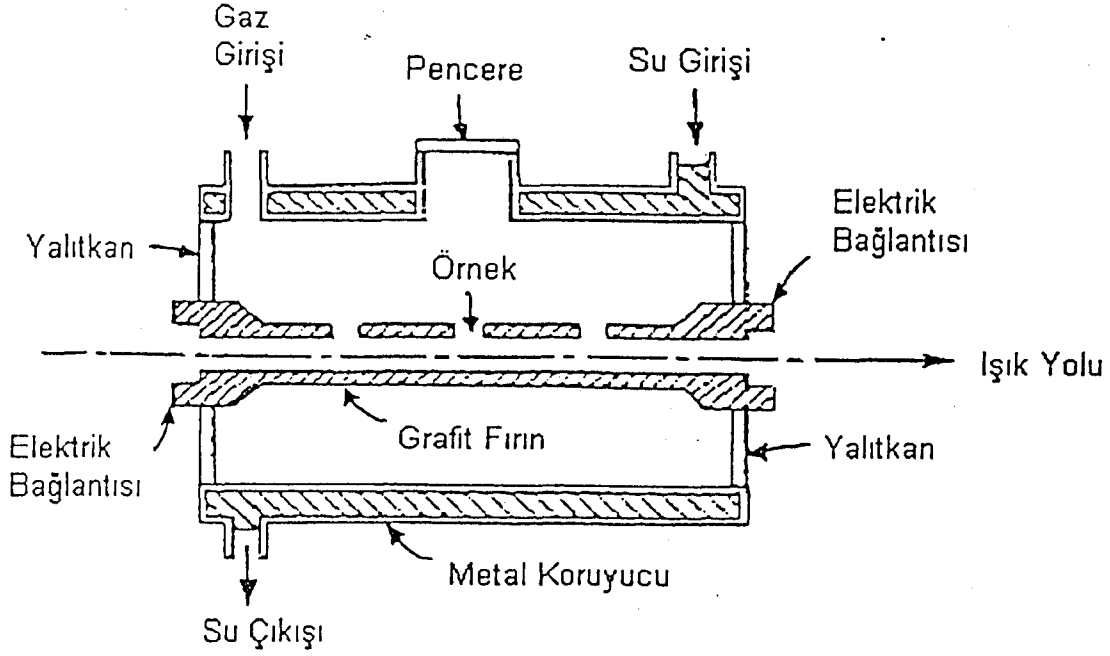
Şekil 1.18. Grafir fırın
