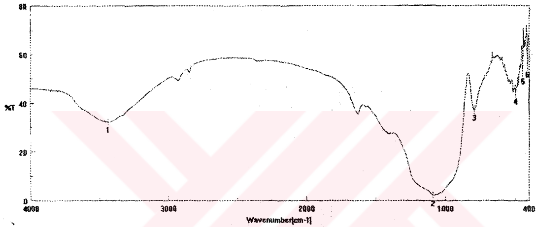
Şekil 3.5. Asit fonksiyonelliği kazandırılmış cam mikrokürecikleri (NED) infrared spektrumu
