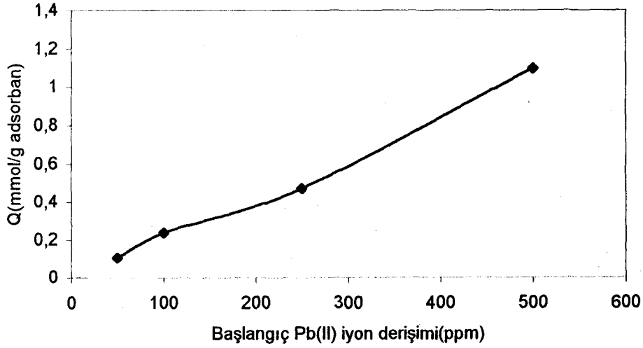
Şekil 3.24. Yüzeyi 2-aminoetantiyol ile modifiye edilmiş cam mikroküreciklere adsorplanan Pb(II) miktarının başlangıç derişimi ile deęişimi; pH : 6,10; T : 25°C; Cam mikrokürecik miktarı : 50 mg; Zaman : 15 dakika
