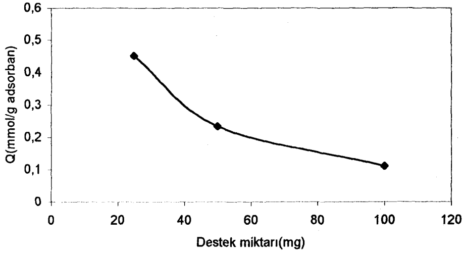
Şekil 3.25. Yüzeyi 2-aminoetantiyol ile modifiye edilmiş cam mikroküreciklere adsorplanan Pb(II) miktarının destek miktarı ile değişimi; Başlangıç derişimi : 100 ppm; pH : 6,10; T : 25°C; Zaman : 15 dakika
