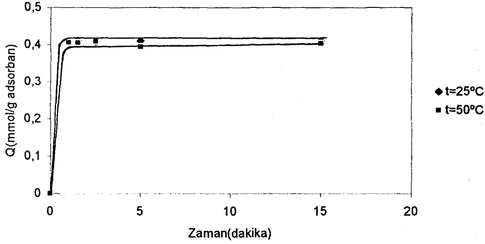
Şekil 3.11. Yüzeyi sistamin ile modifiye edilmiş cam mikroküreciklere adsorplanan Cd(II) miktarının sıcaklık ile değişimi; Başlangıç derişimi : 100 ppm; pH : 4,45 Cam mikrokürecik miktarı : 50 mg;
