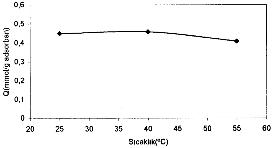
Şekil 3.15. Yüzeyi sistamin ile modifiye edilmiş cam mikroküreciklere adsorplanan Pb(II) miktarının sıcaklık ile değişimi; pH : 5,20; Başlangıç derişimi : 100 ppm; Cam mikrokürecik miktarı : 25 mg; Zaman : 15 dakika;
