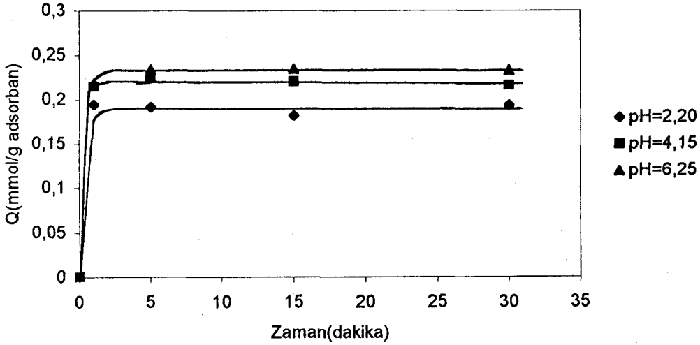
Şekil 3.22. Yüzeyi 2-aminoetantiyol ile modifiye edilmiş cam mikroküreciklere adsorplanan Pb(II) miktarının pH ile değişimi; Başlangıç derişimi : 100 ppm; T : 25°C; Cam mikrokürecik miktarı : 50 mg;
