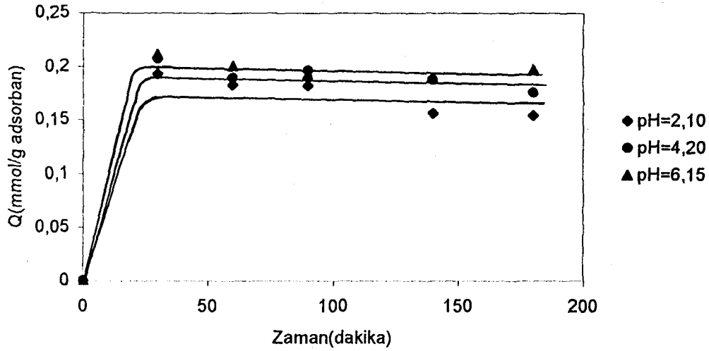
Şekil 3.14. Yüzeyi sistanın ile modifiye edilmiş cam mikroküreciklere adsorplanan Pb(II) miktarının pH ile değişimi; Başlangıç derişimi : 100 ppm; T : 25°C Cam mikrokürecik miktarı : 50 mg;
