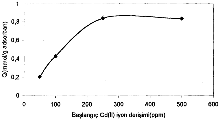
Şekil 3.20. Yüzeyi 2-aminoetantiyol ile modifiye edilmiş cam mikroküreciklere adsorplanan Cd(II) miktarının başlangıç derişimi ile değışimi; pH : 4,30; T : 25°C; Cam mikrokürecik miktarı : 50 mg; Zaman : 15 dakika
