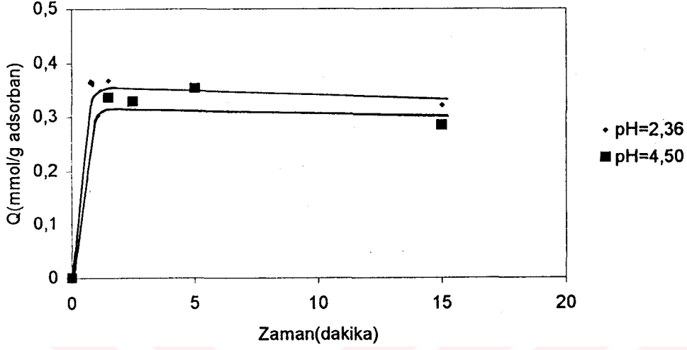
Şekil 3.18. Yüzeyi 2-aminoetantiyol ile modifiye edilmiş cam mikroküreciklere adsorplanan Cd(II) miktarının pH ile değişimi; Başlangıç derişimi : 100 ppm; T : 25°C Cam mikrokürecik miktarı : 50 mg;
