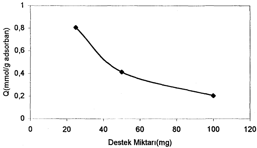
Şekil 3.13. Yüzeyi sistamin ile modifiye edilmiş cam mikroküreciklere adsorplanan Cd(II) miktarının destek miktarı ile değişimi; Başlangıç derişimi : 100 ppm; T : 25°C; pH : 4,41; Zaman : 15 dakika
