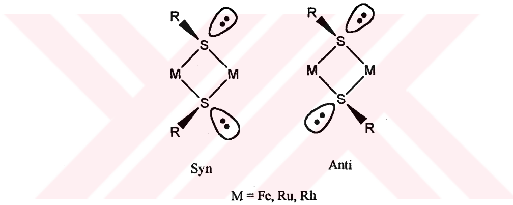
Şekil 1.1. Köprülü tiyolat ligandlarının stereoizomer yapıları
