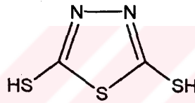
Şekil 1.15. 2,5-Dimerkapto-1,3,4-tiyodiazol yapısı
