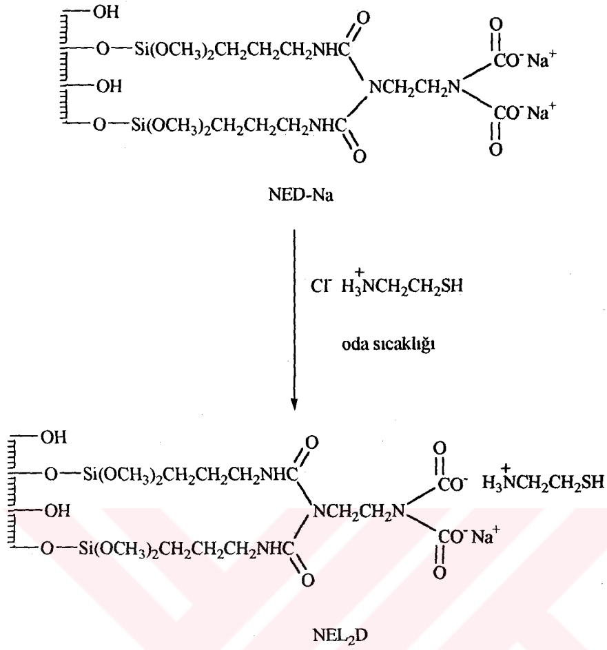
Şekil 3.7. 2-Aminoctantiyolün cama bağlanma reaksiyonu
