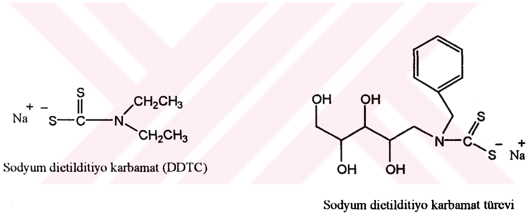
Şekil 1.2. Kükürt içeren ligandların yapı formülleri
