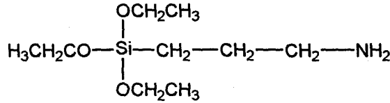
Şekil 1.12. 3-Aminopropiltrietoksisilan yapısı
