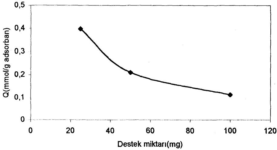
Şekil 3.17. Yüzeyi sistamin ile modifiye edilmiş cam mikroküreciklere adsorplanan Pb(II) miktarının destek miktarı ile değişimi; Başlangıç derişimi : 100 ppm; T : 25°C; pH : 5.15; Zaman : 15 dakika
