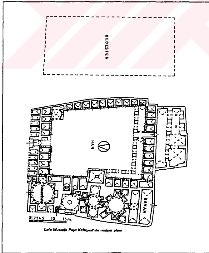
Çizim 2: Gaziantep Lala Mustafa Paşa Hanı Vaziyet Planı
