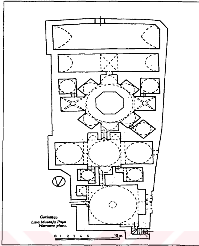
Çizim 1: Gaziantep Lala Mustafa Paşa Hamamı Planı
