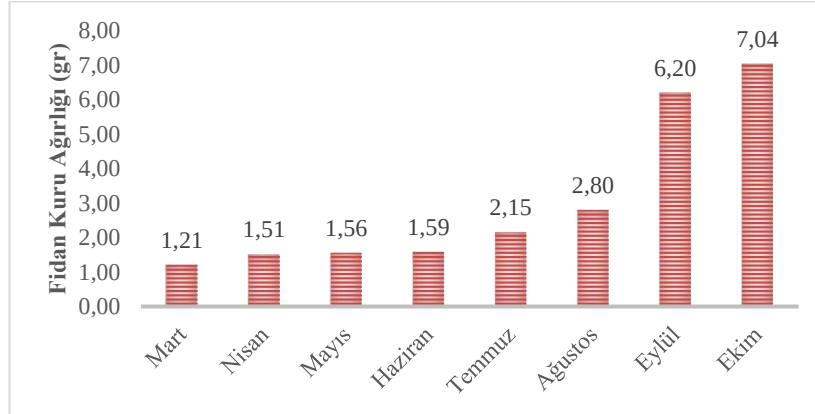
Şekil 4.20 Anadolu karaçamı fidanlarının fidan kuru ağırlığı periyodik gelişimi
