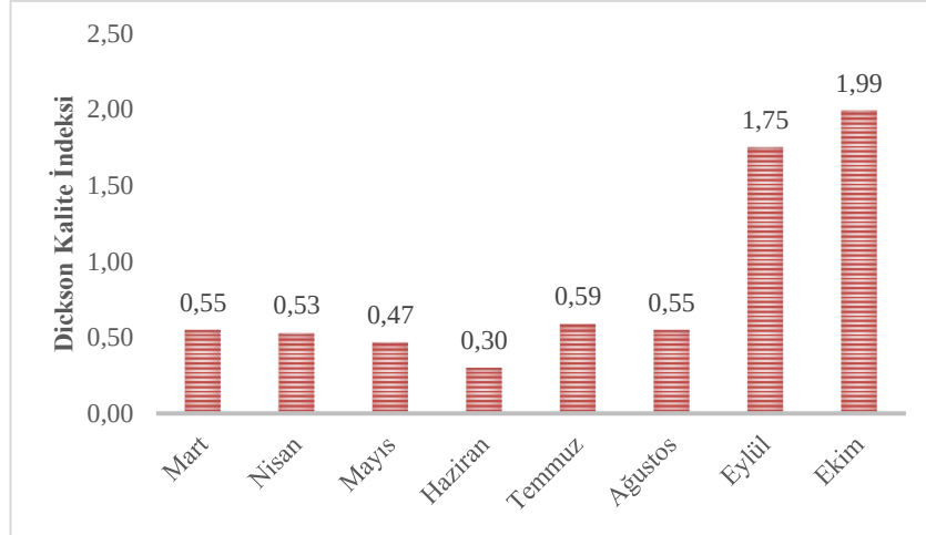
Şekil 4.23 Anadolu karaçamı fidanlarının Dickson kalite indisi değerleri periyodik değişimi
