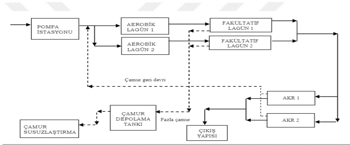
Şekil 2.3. Bursa Hamitler Sızıntı Suyu Arıtma Tesisi akım şeması (Kaşıkçı, 2010)
