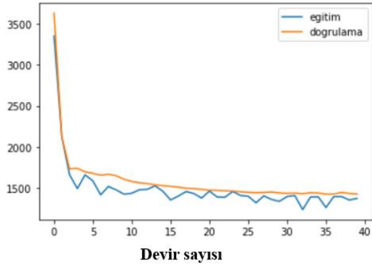
Şekil 4.4. CNN-LSTM’de devir sayısına göre kayıp fonksiyonunun değerleri (MSE)
