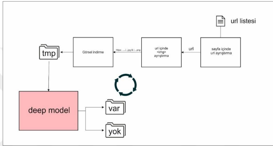
Şekil 6.2. Web crawler blok şeması
