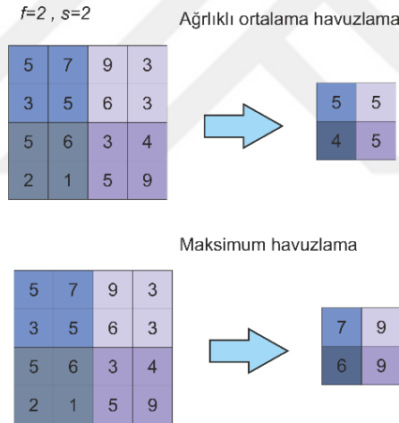
Şekil 5.6. Ortalama havuzlama ve maksimum havuzlama
