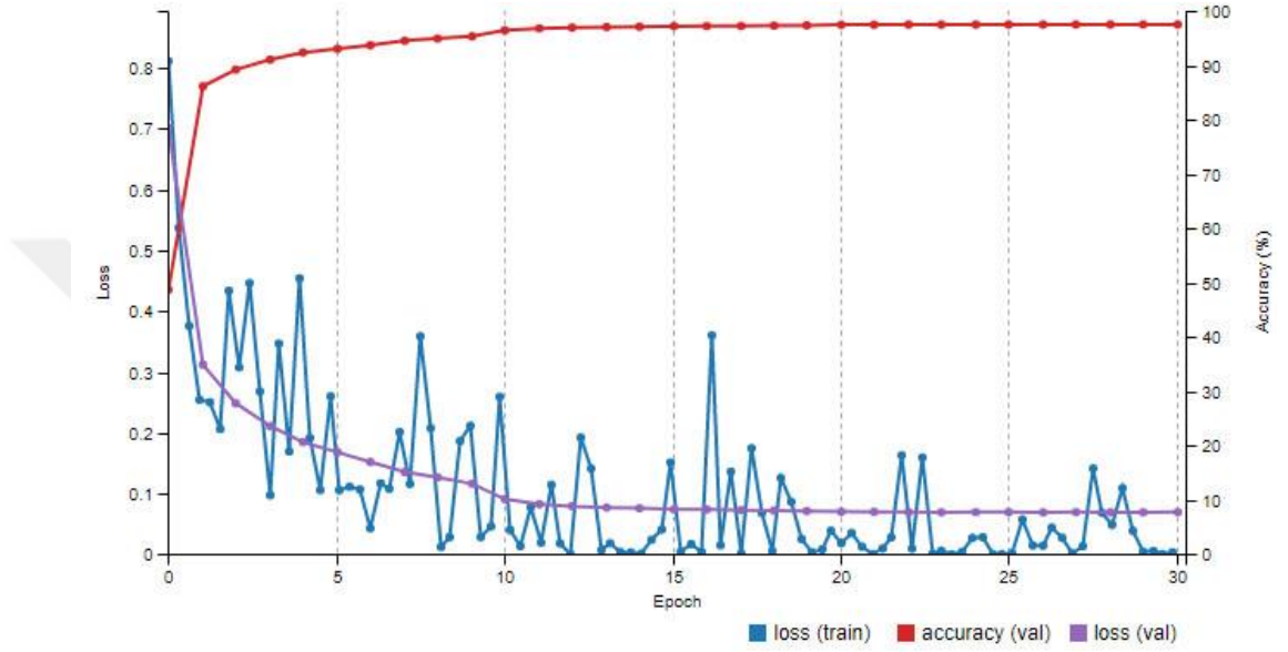
Şekil 6.19. Model_3 eğitim grafiği
