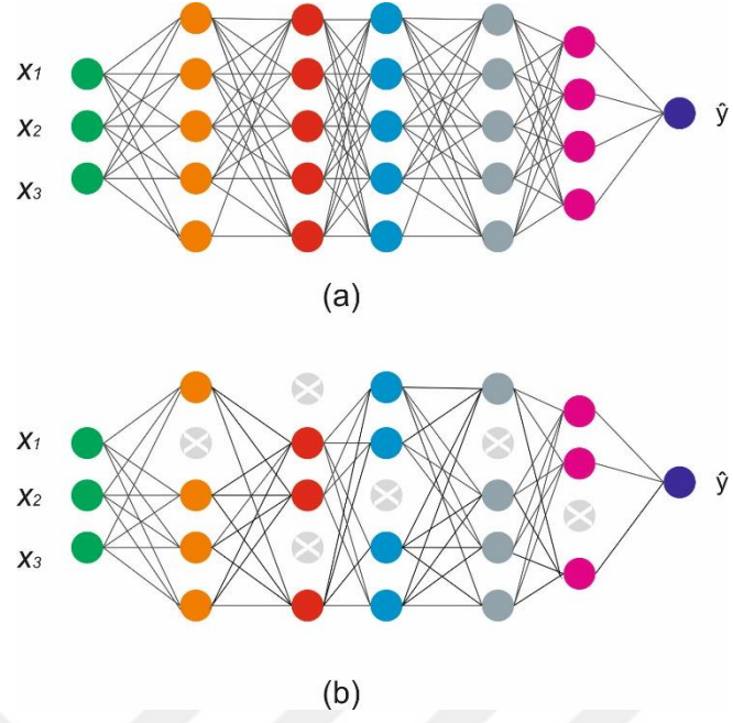
Şekil 4.11. Standart bir sinir ağı (a) Seyreltme işleminden sonra sinir ağı (b)
