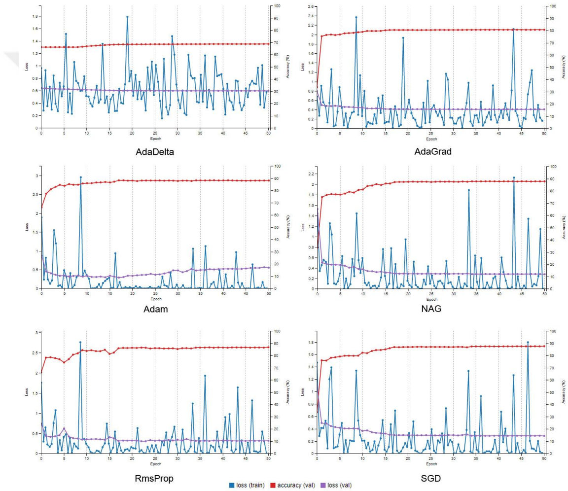
Şekil 6.11. db_00 veri seti ile AdaDelta, AdaGrad, Adam, NAG, RmsProp ve SGD Eniyileyici türlerinin eğitim karşılaştırmaları
