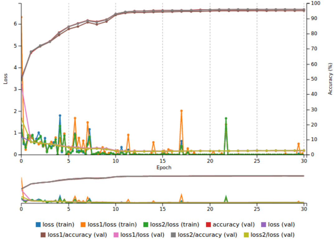
Şekil 4.10. Tur sayısı ve öğrenme başarısı arasındaki ilişki
