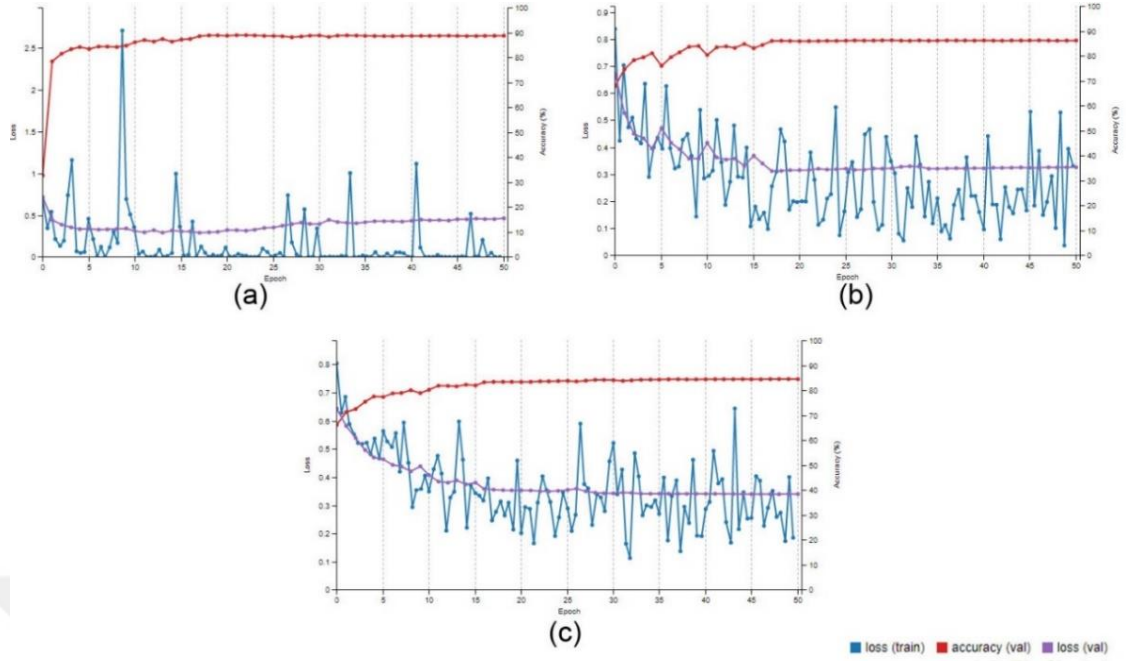
Şekil 6.10. 2 (a), 16 (b) ve 32 (c) yığın boyutlarının db_00 veri seti ve GoogLeNet kullanılarak kıyaslanması
