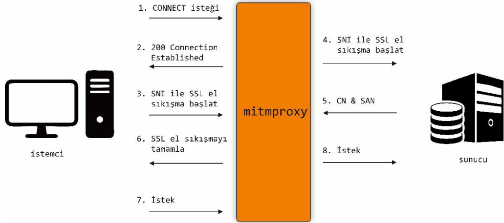
Şekil 6.26. Mitmproxy https bağlantı (Mitmproxy, 2021)
