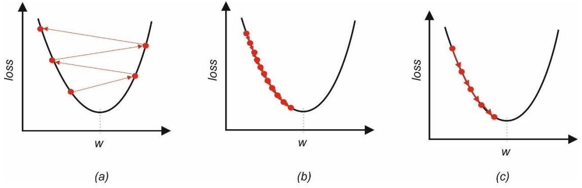
Şekil 4.9. (a) Yüksek öğrenme oranı (b) Düşük öğrenme oranı (c) Optimum öğrenme oranı (Akca, 2020)
