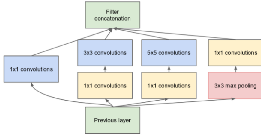
Şekil 5.14. Boyut küçültme ile başlangıç modülü
