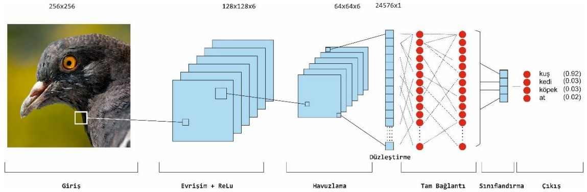
Şekil 5.8. ESA Katman yapısı
