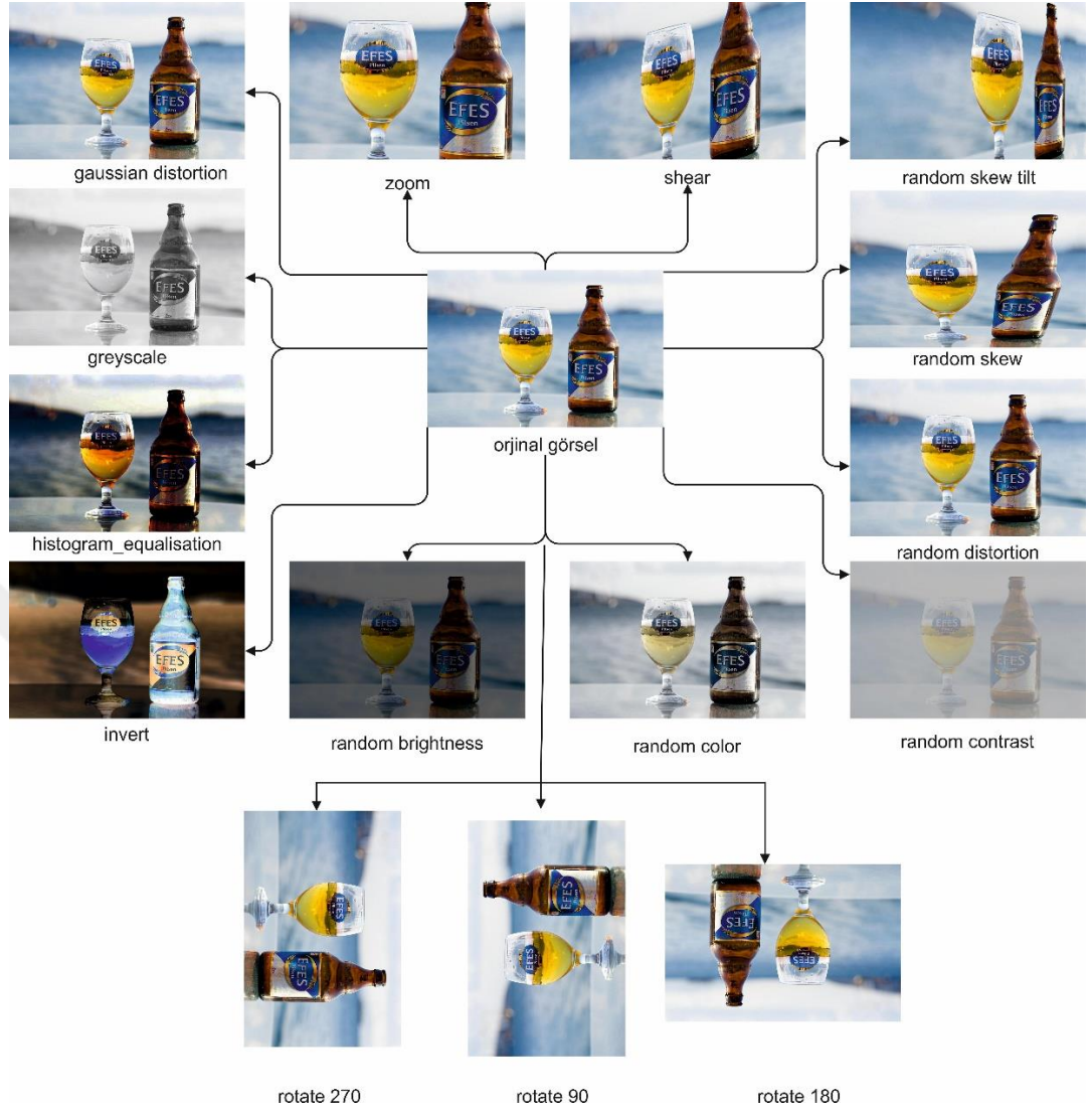
Şekil 6.6. Veri çoğaltma örnekleri
