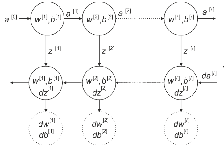
Şekil 3.4. İleri ve Geri besleme
