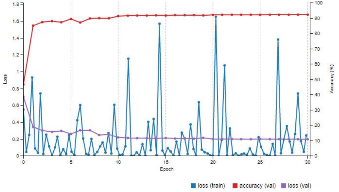
Şekil 6.17. Model_1 eğitim grafiği
