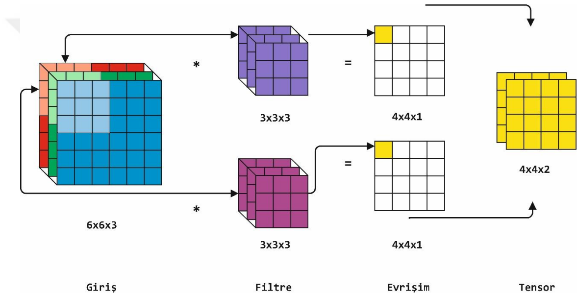
Şekil 5.7. Çok kanallı evrişim ve tensor yapısı
