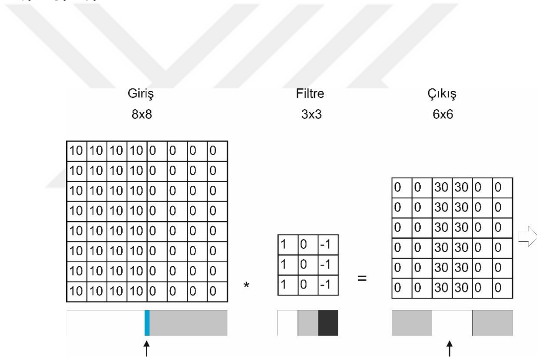
Şekil 5.3. Kenar bulma işlemi
