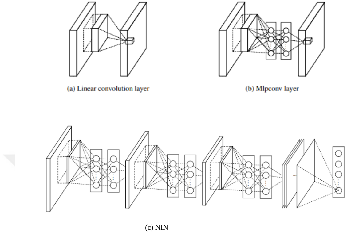
Şekil 5.11. (a) Doğrusal evrişim katmanı (b) MLP katmanı (c) Ağ içinde ağ yapısı
