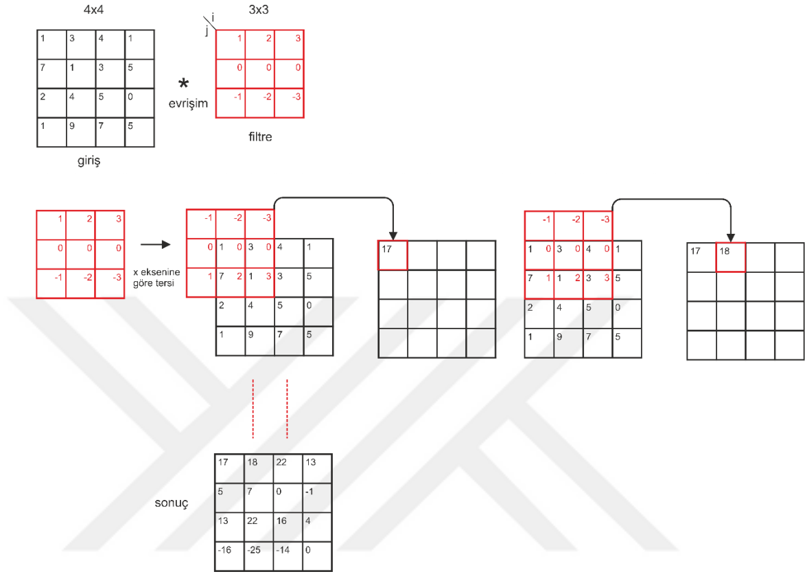
Şekil 5.2. İki boyutlu matris üzerinde evrişim işlem örneği
