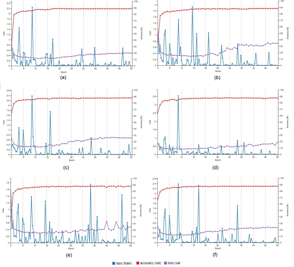
Şekil 6.13. Azalan Sönümleme (a) Sigmoid Sönümleme (b) Polinom Sönümleme (c) Devrik Sönümleme (d) Sabit (e) Üstel Sönümleme (f) temel öğrenme oranı ilkelerinin db_00 ile eğitim karşılaştırmaları
