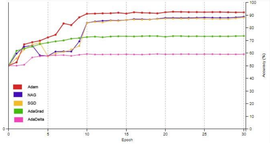
Şekil 4.6. Eniyileyici türleri kedi-köpek veri seti üzerindeki eğitiminin karşılaştırması
