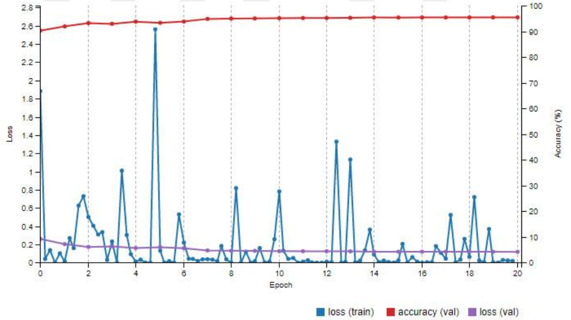
Şekil 6.18. Model_2 eğitim grafiği
