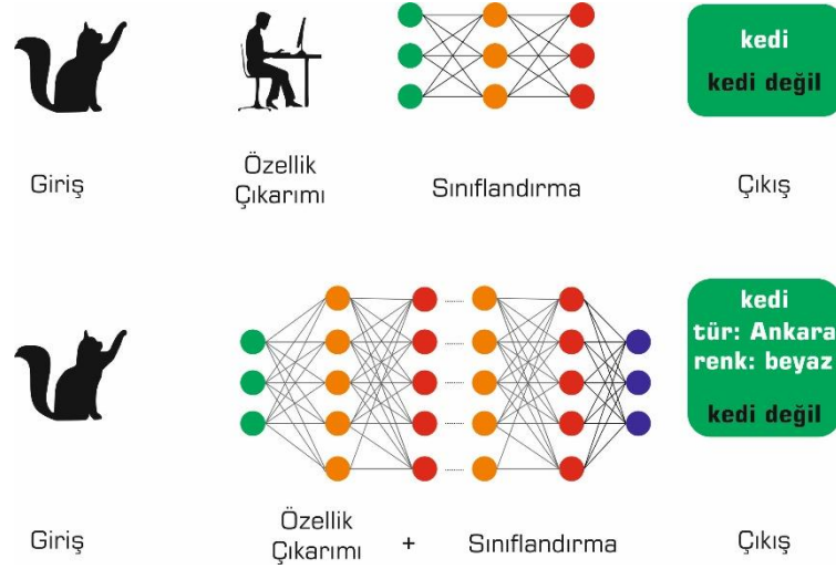
Şekil 3.1. Makine Öğrenmesi (üstte) ve Derin Öğrenme (altta)
