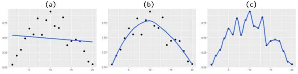
Şekil 4.8. Yetersiz Öğrenme (a), İyi Öğrenme (b), Aşırı Öğrenme (c)
