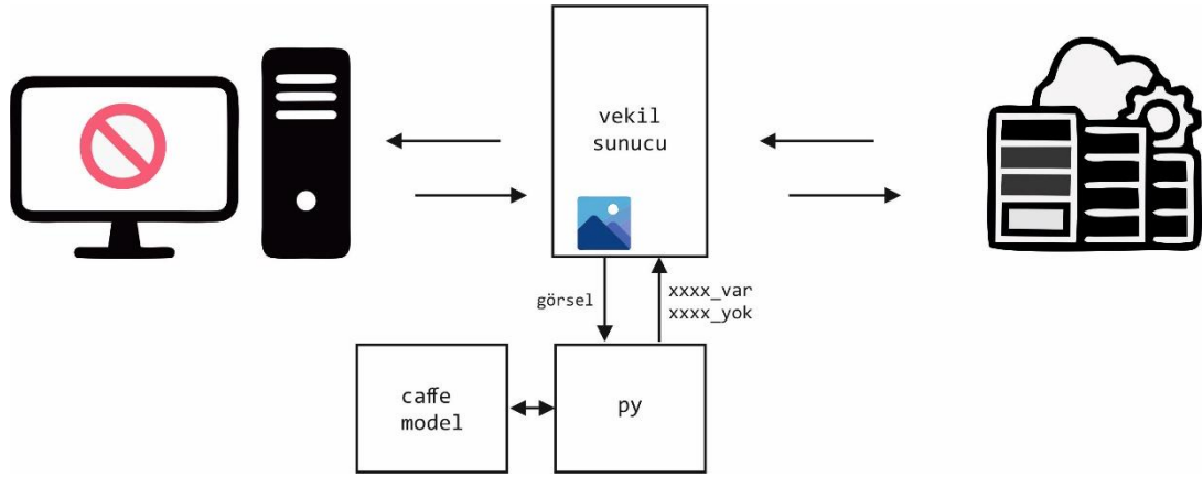
Şekil 6.25. Uygulama blok şeması
