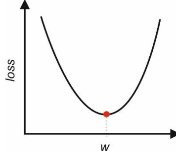
Şekil 4.4. Gradyan inişi
