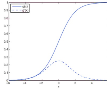
sigmoid
