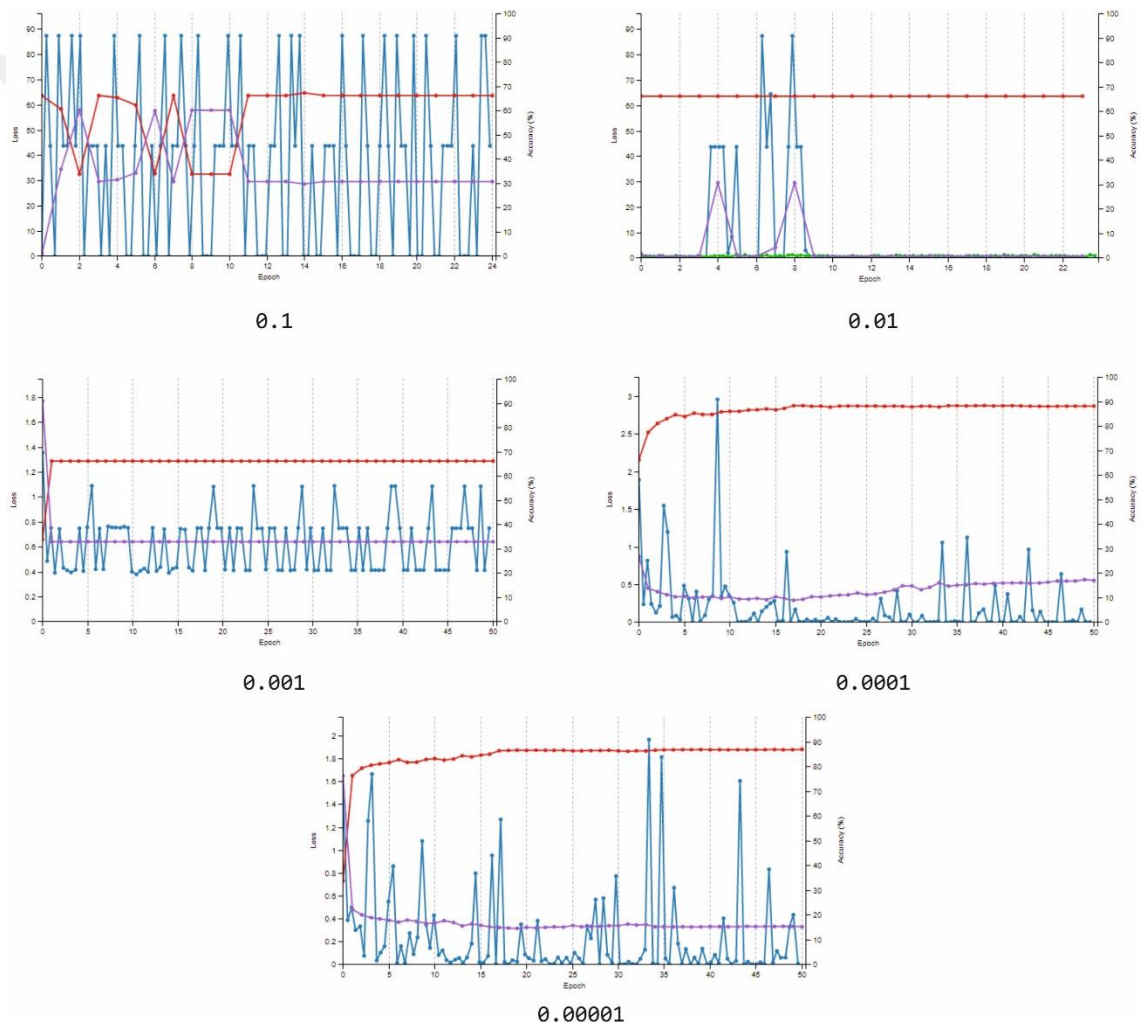
Şekil 6.14. Öğrenme katsayılarının karşılaştırılması
