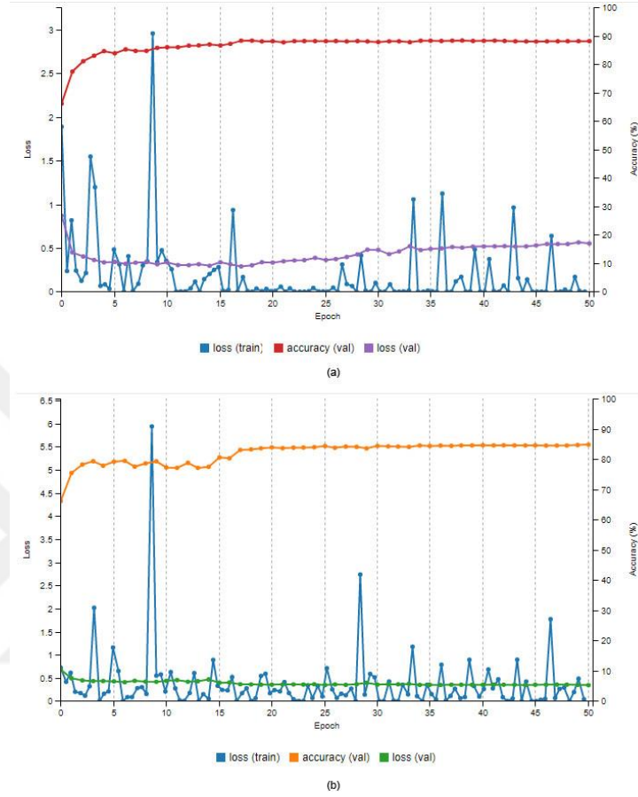
Şekil 6.9. db_00 veri seti kullanılarak GoogLeNet (a) ve AlexNet (b) karşılaştırması
