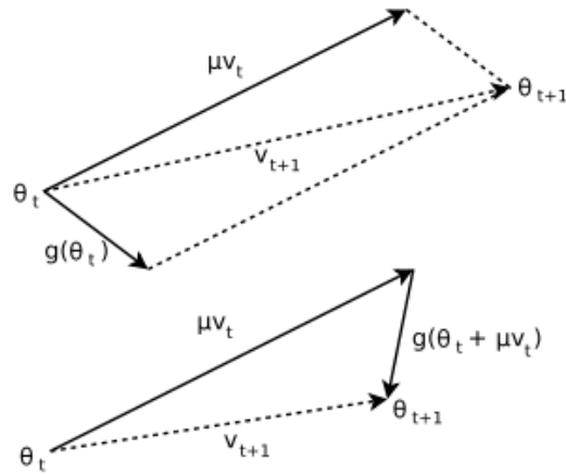
Şekil 4.7. Klasik momentum (üstte), Nesterov Hızlandırılmış Gradyan (altta)
