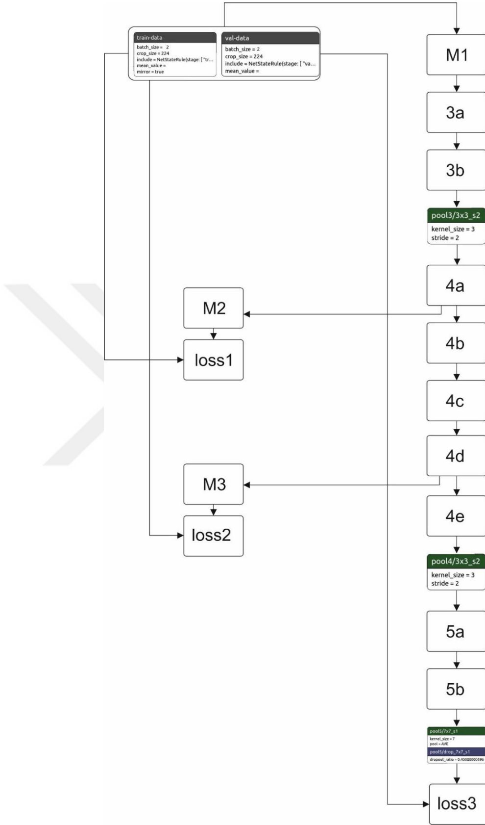
Şekil 6.15. GoogLeNet Inception Ağ Mimarisi
