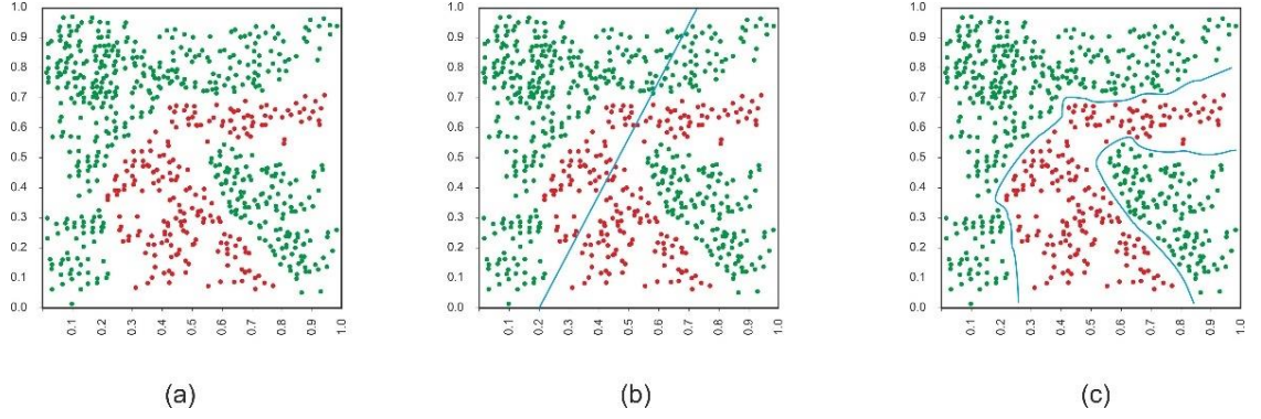
Şekil 4.2. Ham veri (a), Lineer aktivasyon fonksiyonu ile sınıflandırma (b), Lineer olmayan aktivasyon fonksiyonu ile sınıflandırma (c)
