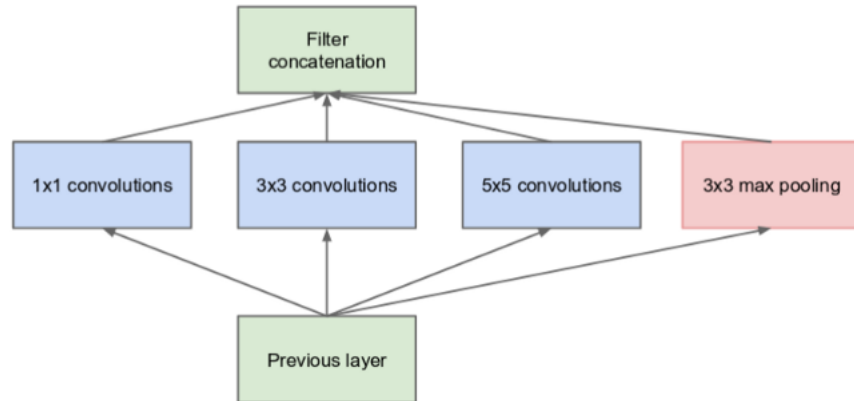
Şekil 5.13. Naif başlangıç modülü (Szegedy vd., 2014)
