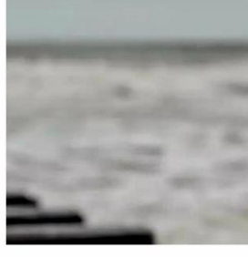
random_crop
