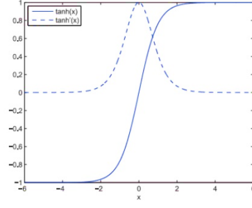
hiperbolik tanjant
