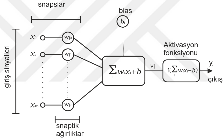
Şekil 2.2. Perseptron – algılayıcı
