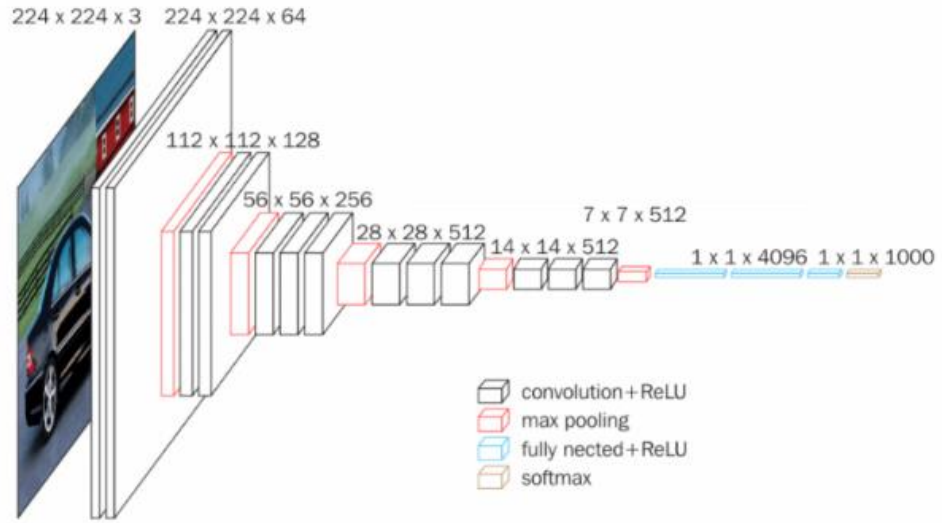
Şekil 5.10. VGG16 Mimarisi
