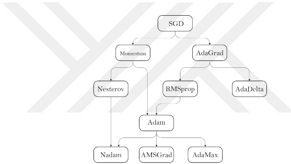
Şekil 4.5. Eniyileyici algoritmaları arasındaki ilişki haritası (Seyyarer vd, 2020)
