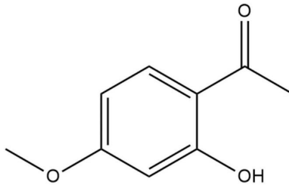
Paeonol
