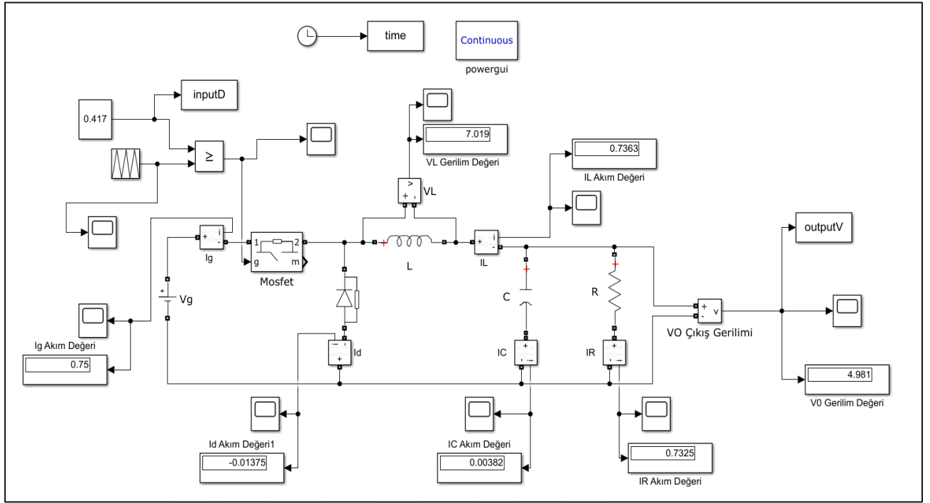
Şekil 3.7. Düşürücü tip DA-DA dönüştürücü simülasyon devresi
