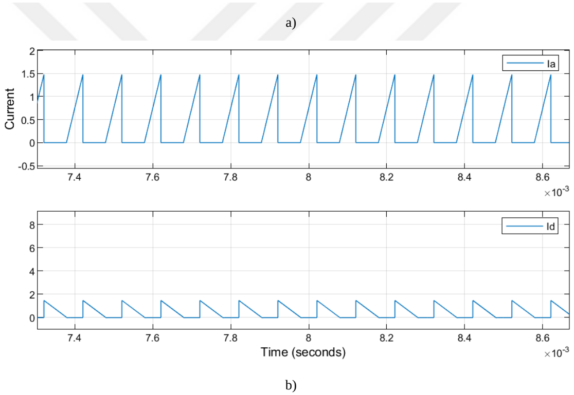
Şekil 4.3. Düşürücü tip DA-DA dönüştürücü referans simulink devresi mosfet ( I_a ) ve diyot ( I_d ) akım grafikleri a)normal görüntü, b)yakınlaştırılmış görüntü
