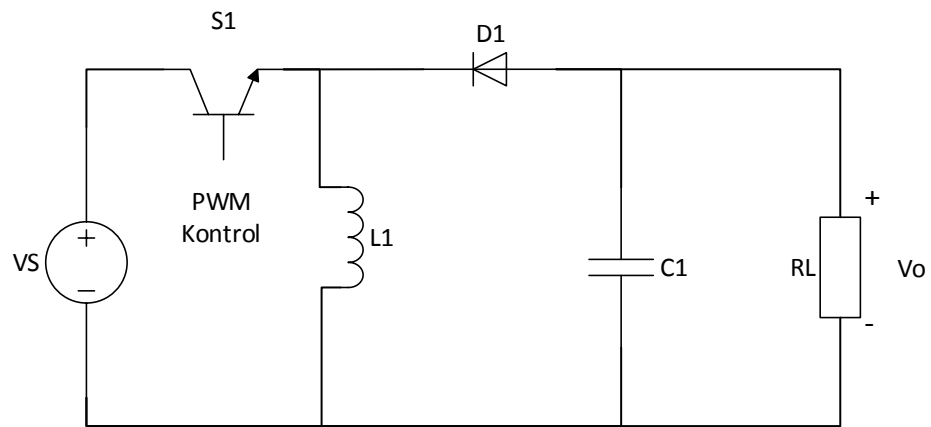
Şekil 2.9. Düşüren-yükselten dönüştürücü devresi
