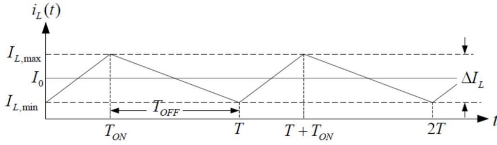
Şekil 3.3. Bobin akımı
