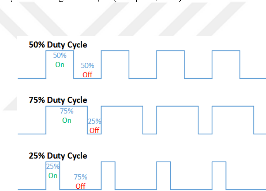
Şekil 2.24. Görev döngüsünün farklı yüzdelerde çalışma aralıkları
