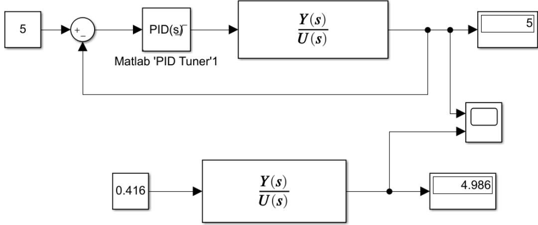
Şekil 4.18. Kontrolsüz ve PID kontrollü düşürücü tip DA-DA dönüştürücü blok diyagramı
