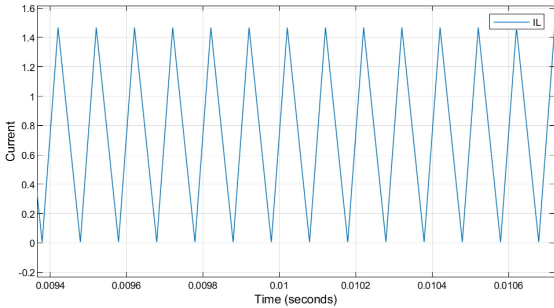
Şekil 4.2. Düşürücü tip DA-DA dönüştürücü referans simulink devresi bobin akım grafikleri a)normal görüntü, b)yakınlaştırılmış görüntü
