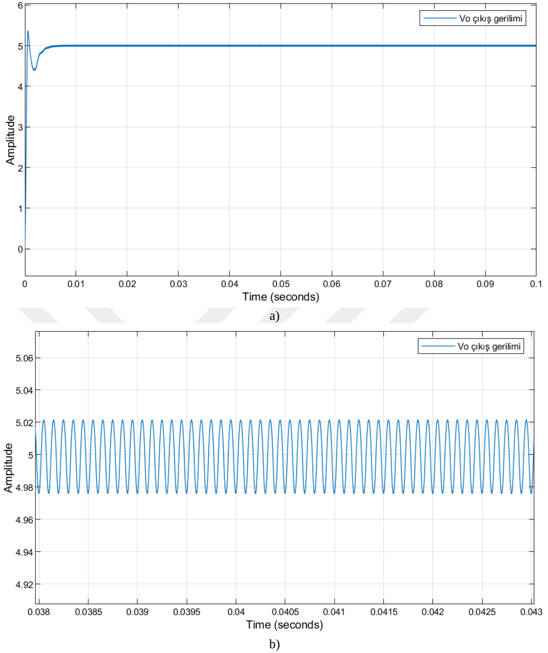
Şekil 4.15. PID kontrollü düşürücü dönüştürücü çıkış gerilim grafikleri a)normal görüntü, b)yakınlaştırılmış görüntü
