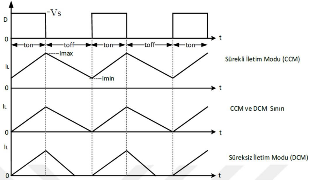
Şekil 2.2. DA-DA dönüştürücünün bobin akımına göre iletim durumları
