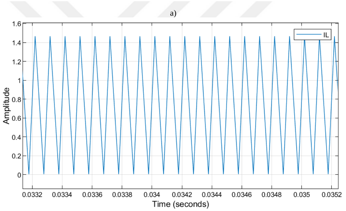
Şekil 4.16. PID kontrollü düşürücü tip DA-DA dönüştürücü bobin akım grafikleri a)normal görüntü, b)yakınlaştırılmış görüntü
