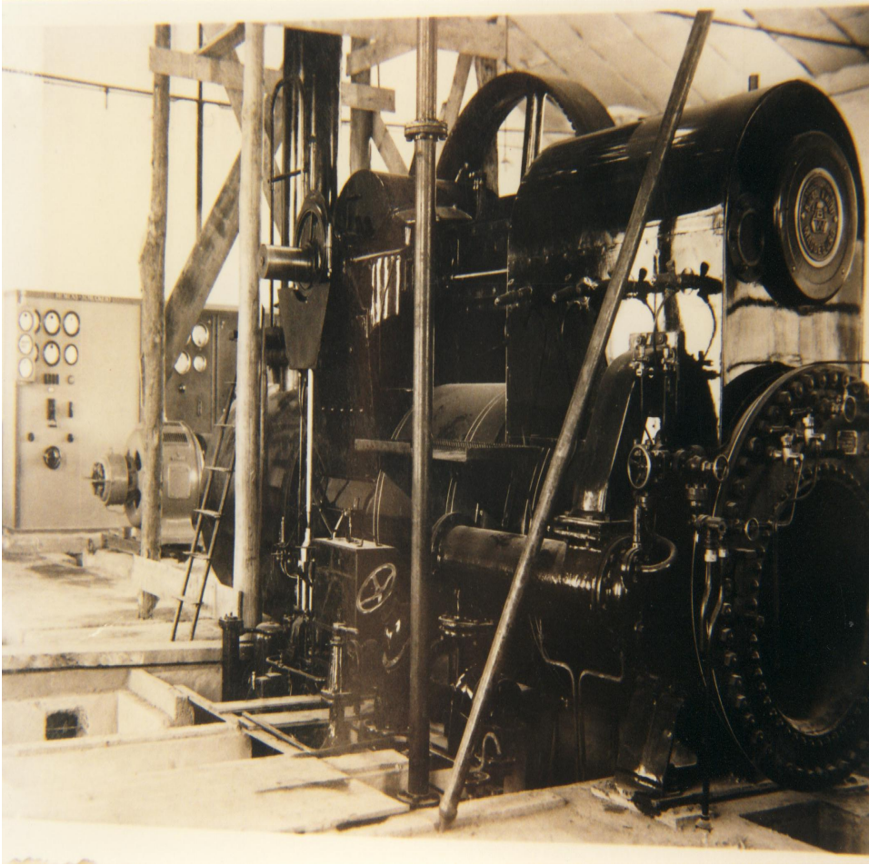
Fotoğraf 10. Lokomobil (elektrik fabrikası)
