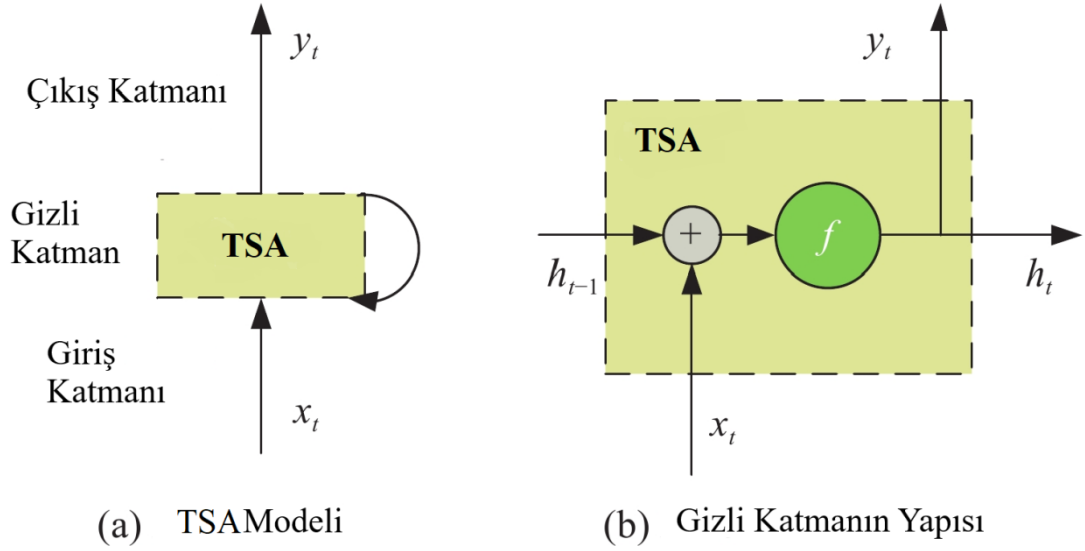
Şekil 2.2. TSA yapısı ve gizli katmanın yapısı (Liu vd. 2021)
