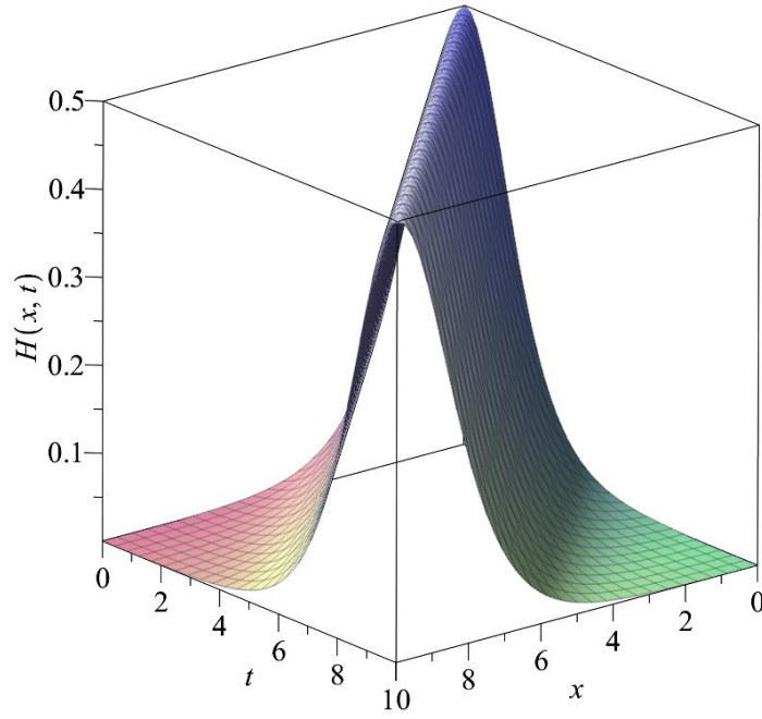
Şekil 7.2: Denklem (7.19) ile verilen H(x, t) fonksiyonun grafiği.
