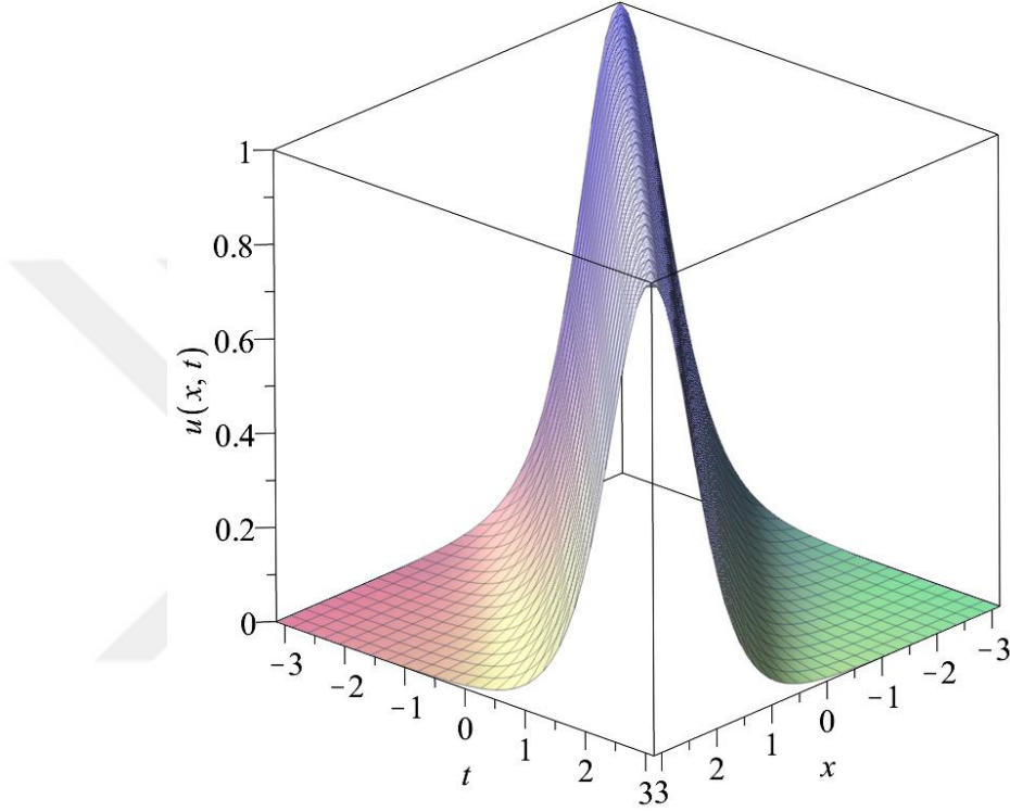
Şekil 2.2 Soliton çözümü u(x, t) = \text{sech}^2(x - t) , -\pi \leq x, t \leq \pi
