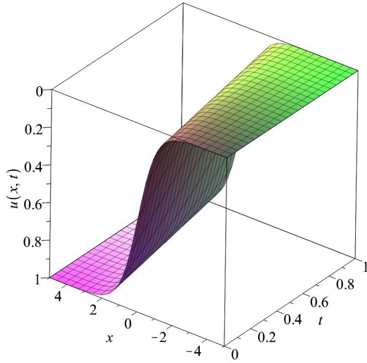
Şekil 3.5: Denklem (3.31a) ile verilen fonksiyonun grafiği.
