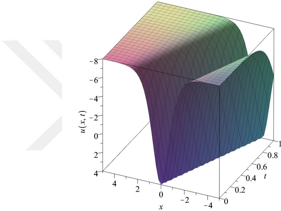
Şekil 3.3: Denklem (3.22a) ile verilen fonksiyonun grafiđi.
